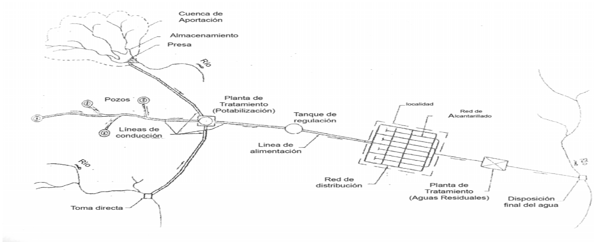
Figura 1.1 Estructura de un sistema hidráulico urbano típico
