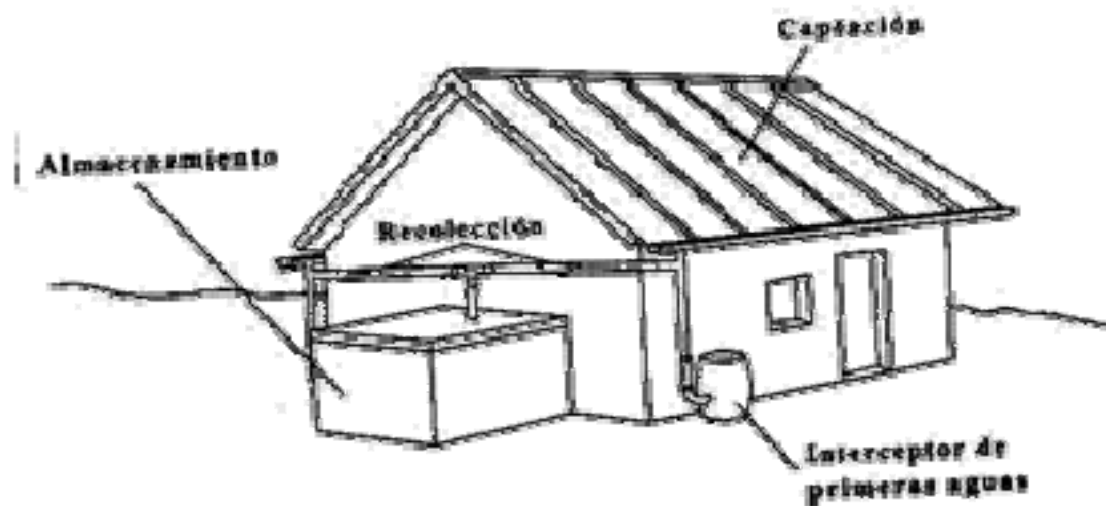
Figura 3.1 Captación en techo
