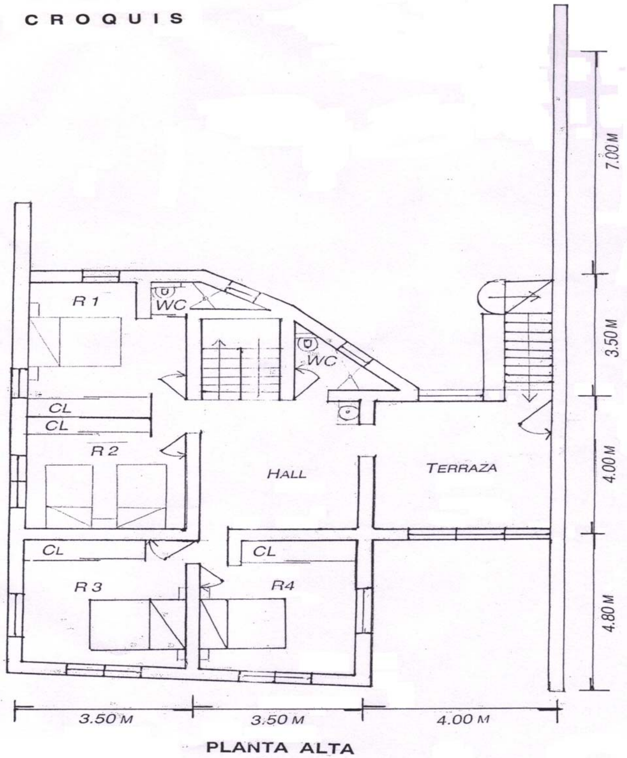
Figura 5.2 Croquis planta alta
