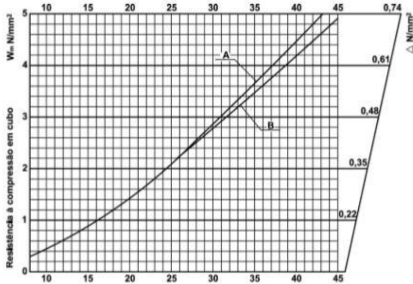
A - Ensayo en concreto B - Ensayo en muros
