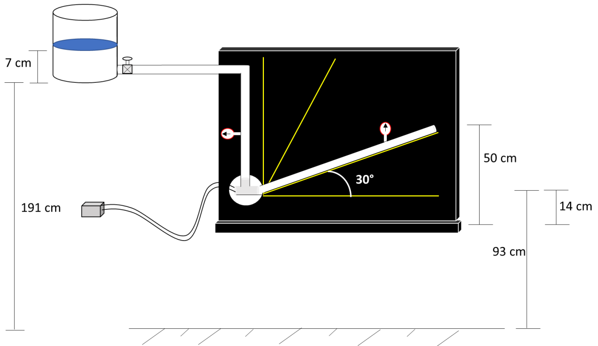
Figura 4.6. Esquema del modelo experimental con un ángulo de 30°.
