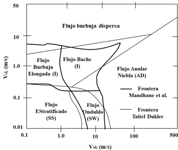
Figura 3.17. Mapa del patrón de flujo determinado por Taitel y Dukler en 1976, mediante un modelo teórico.
