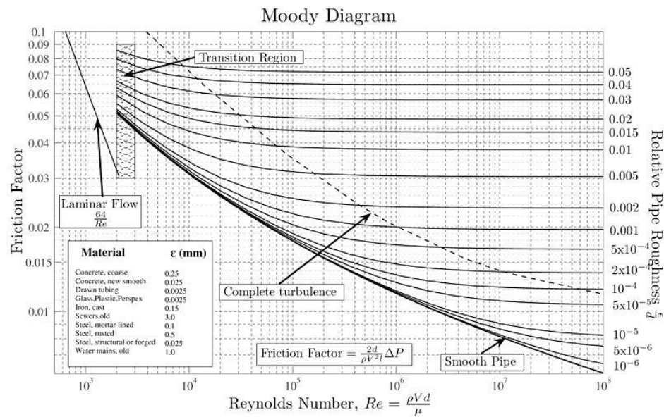
Figura 3.8. Gráfica doble logarítmica del Diagrama de Moody, útil para determinar el factor de fricción cuando se conocen la rugosidad relativa y el número de Reynolds.
