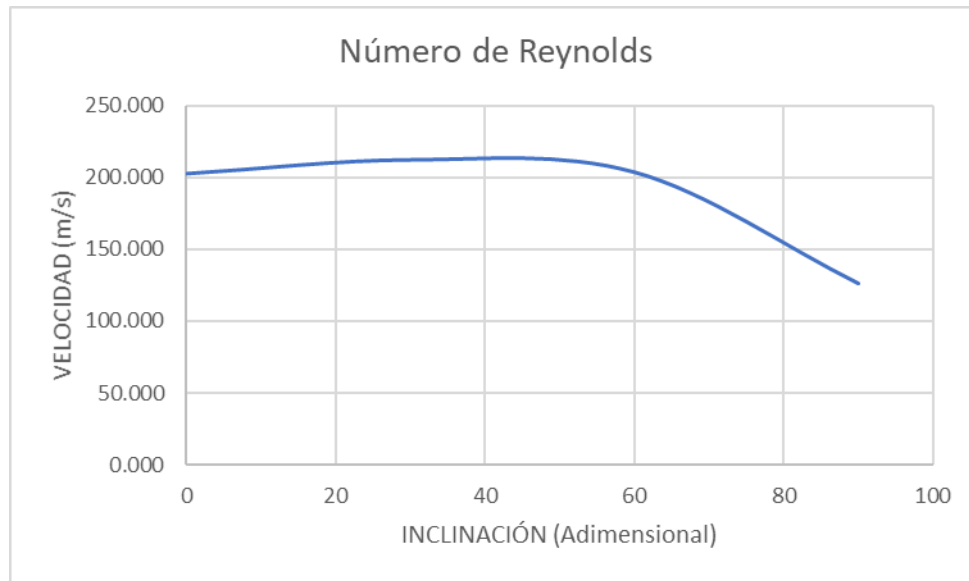
Figura 4.19. Comportamiento del número de Reynolds con respecto al ángulo de inclinación para un gasto alto.
