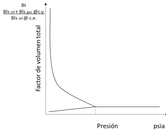
Figura 1.16. Gráfica del comportamiento del Bt con respecto a la presión.
