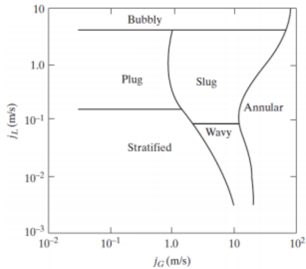
Figura 3.15. Mapa con la configuración de Mandhane.
