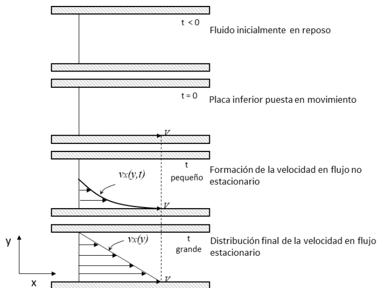
Figura 1.4. Formación del perfil de velocidades en estado estacionario para un fluido contenido entre dos placas.
