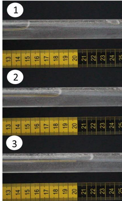
Figura 4.5. Fotografía donde se aprecia la formación del patrón de flujo estratificado dando como consecuencia el fenómeno de colgamiento.
