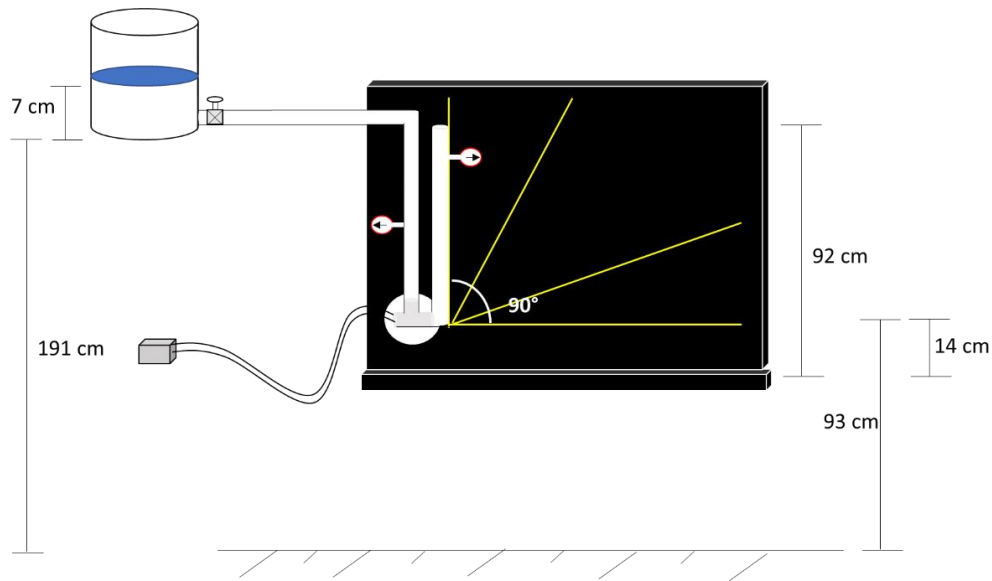
Figura 4.12. Esquema del modelo experimental con un ángulo de 90^\circ .
