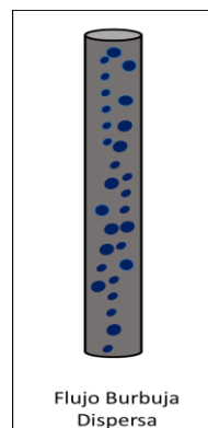
Figura 318. Esquema con el flujo burbuja dispersa, la fase gaseosa esta mezclada de manera homogénea dentro de la fase líquida, no se presenta resbalamiento entre las fases.
