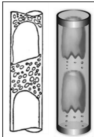
Figura 3.19. Es el esquema del flujo Bache (tapón) presente en una tubería vertical cuando el gasto de la fase gaseosa es más grande que la fase líquida.
