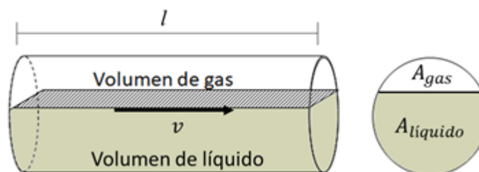
Figura 3.2. Esquema con la representación gráfica del colgamiento de la fase líquida, de un flujo multifásico en el interior de la tubería.
