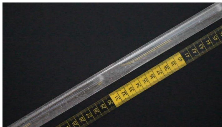
Figura 4.7. Fotografía donde se aprecia el Patrón de flujo intermitente de burbuja alargada.
