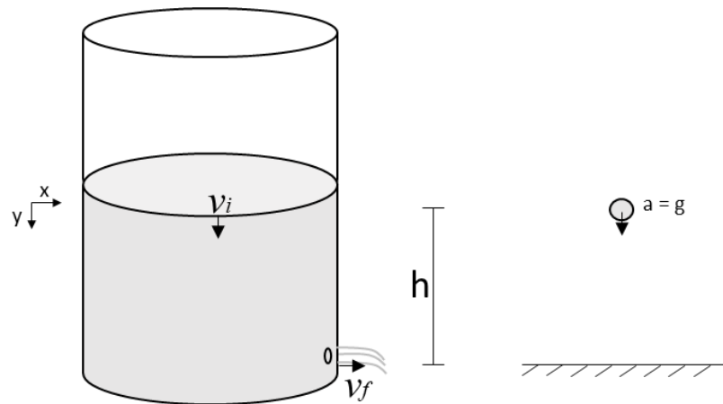
Figura 1.3. Esquema del experimento de Torricelli para determinar la velocidad de salida en un orificio por debajo de la superficie libre del líquido.
