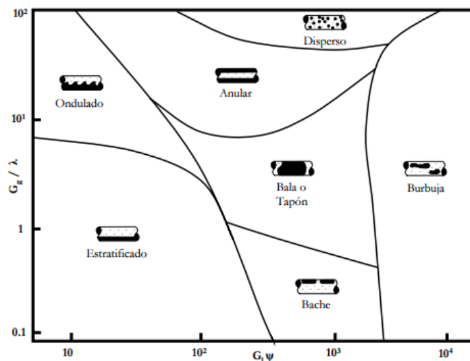
Figura 3.14. Gráfica del patrón de flujo del Mapa de Baker, se ilustran los tipos de flujo que se presentan dentro de la tubería.
