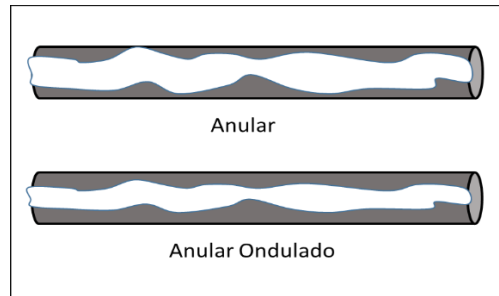
Figura 3.12. Esquema con los tipos de flujo anular y anular ondulado.
