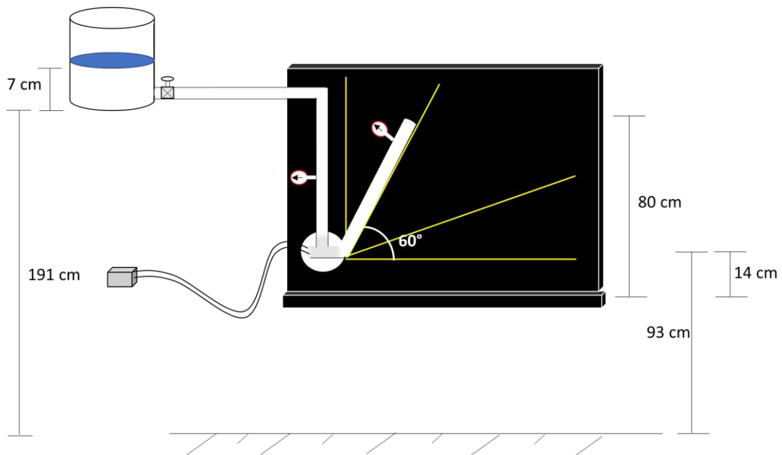
Figura 4.9. Esquema del modelo experimental con un ángulo de 60^\circ .
