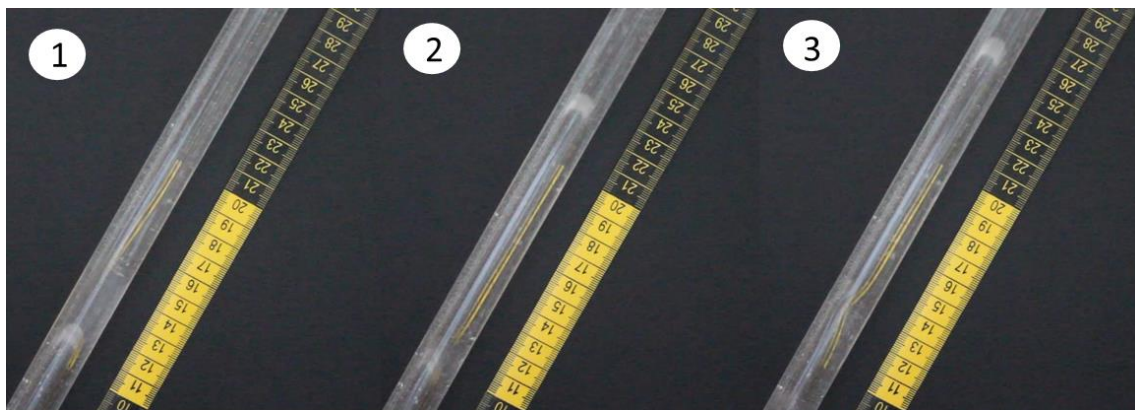
Figura 4.11. Fotografía donde se aprecia el Patrón de flujo tapón.
