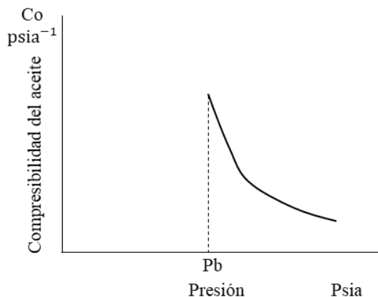
Figura 1.9. Gráfica del comportamiento de la compresibilidad del aceite respecto a la presión de yacimiento.
