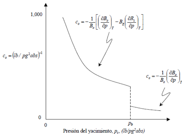
Figura 1.10. Gráfica del comportamiento de la compresibilidad del aceite respecto a la presión de yacimiento.
