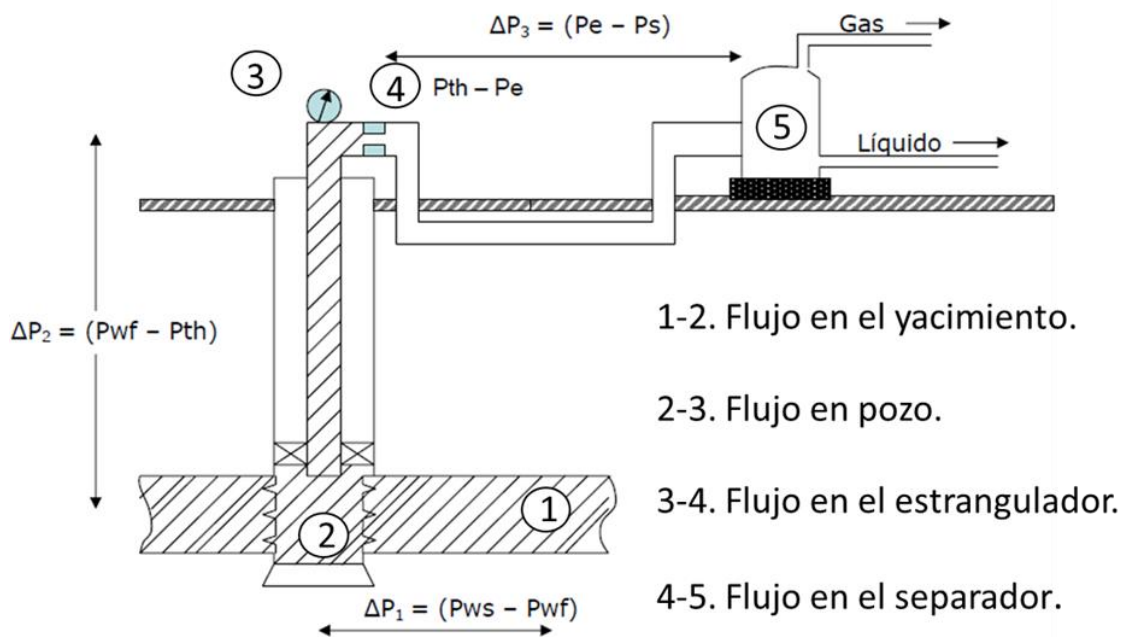
Figura 3.4. Esquema del sistema integral de producción.
