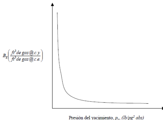
Figura 1.6. Gráfica del comportamiento del factor de volumen del gas con respecto a la presión de yacimiento.
