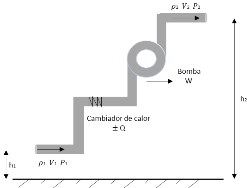
Figura 3.5. Diagrama de flujo en una tubería.
