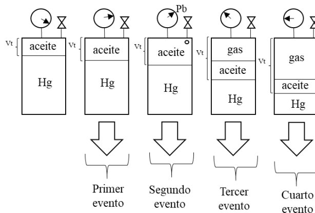
Figura 1.15. Método de separación instantánea (flash).
