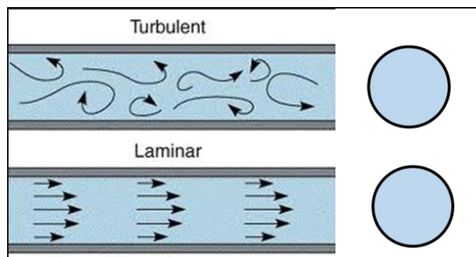
Figura 3.6. Esquema en el que se ilustra las líneas de corriente de un flujo laminar y un flujo turbulento a tubo lleno. En el caso de un flujo laminar se dice que el flujo tiene una velocidad media, no se tienen cambios en la temperatura, por lo tanto, la densidad es constante para ese instante.
