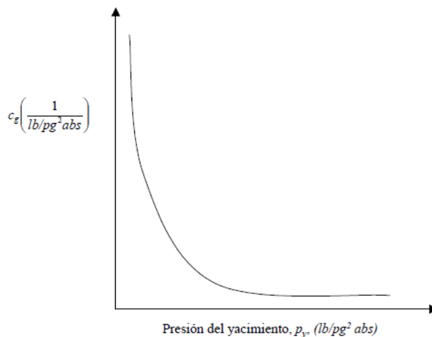
Figura 1.7. Gráfica del comportamiento del coeficiente de compresibilidad isotérmico del gas ideal con respecto a la presión de yacimiento.
