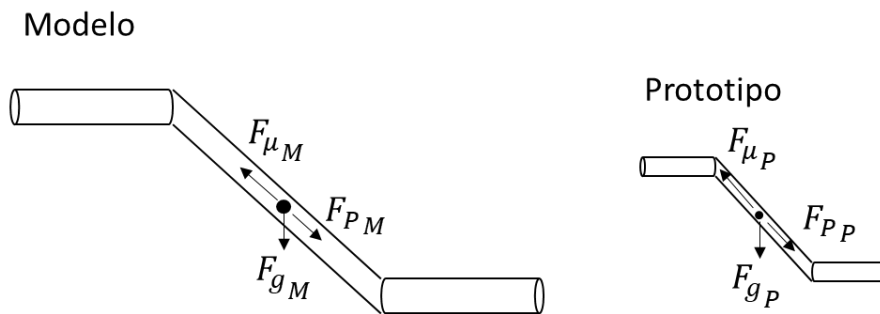
Figura 2.6. Similitud dinámica en una tubería.
