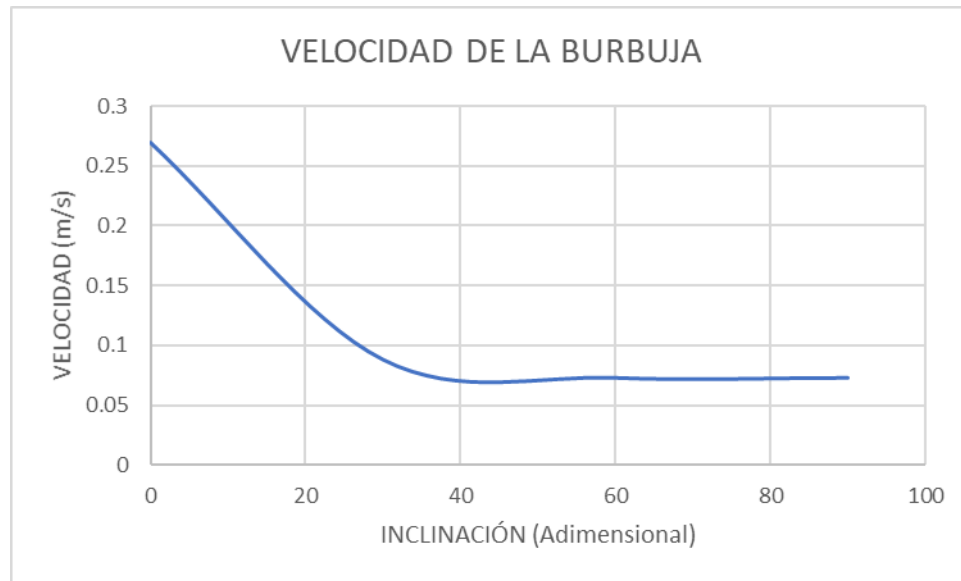
Figura 4.18. Comportamiento de la velocidad de burbuja con respecto al ángulo de inclinación para un gasto bajo.
