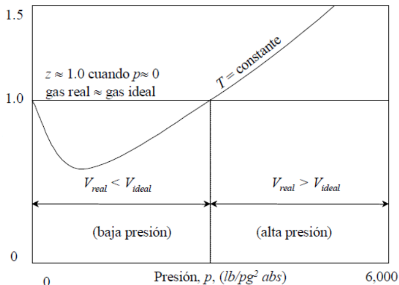
Figura 1.5. Gráfica del comportamiento del factor de desviación estándar con respecto a la presión de yacimiento.
