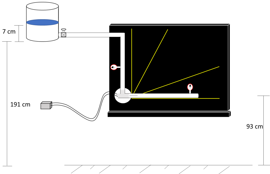
Figura 4.3. Esquema del modelo experimental con un ángulo de 0^\circ .
