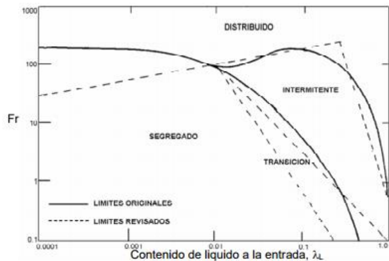
Figura 3.16. Mapa de la correlación de Beggs y Brill. Hace la correlación mediante el Número de Froude y el colgamiento en el interior de la tubería sin resbalamiento, \lambda = A_L/A_{Tubo} .
