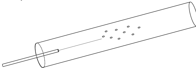
Figura 4.1. Esquema de una región del modelo experimental, donde se observa la inyección de aire al líquido a través de una aguja, formándose pequeñas burbujas de aire.
