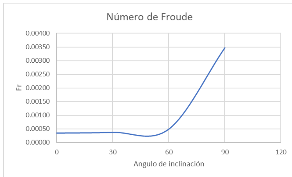
Figura 4.15. Comportamiento del número de Froude con respecto al ángulo de inclinación.
