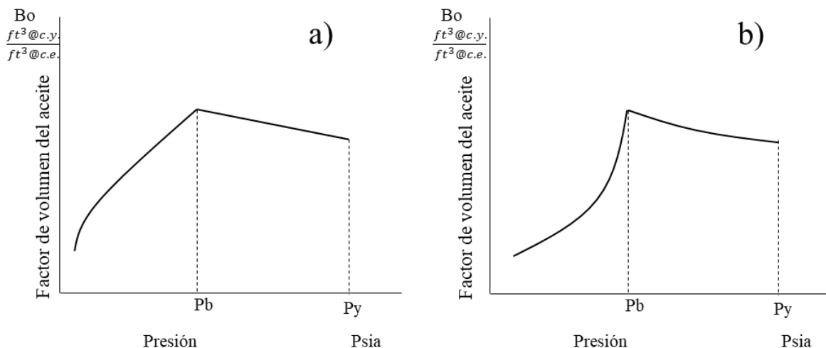
Figura 1.12. a) Gráfica del comportamiento del B_o contra la P_y de un yacimiento de aceite negro b) Gráfica del comportamiento del B_o contra la P_y de un yacimiento de aceite volátil.
