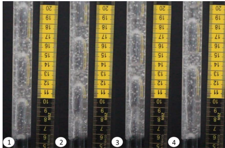
Figura 4.14. Fotografía donde se aprecia la formación del Patrón de flujo tapón.
