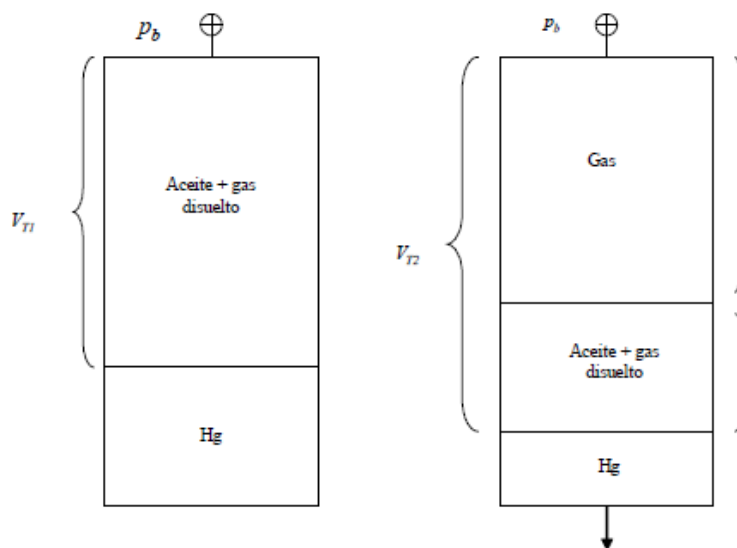
Figura 1.11. Ilustración de la compresibilidad del aceite, para una presión menor a la presión de burbuja.
