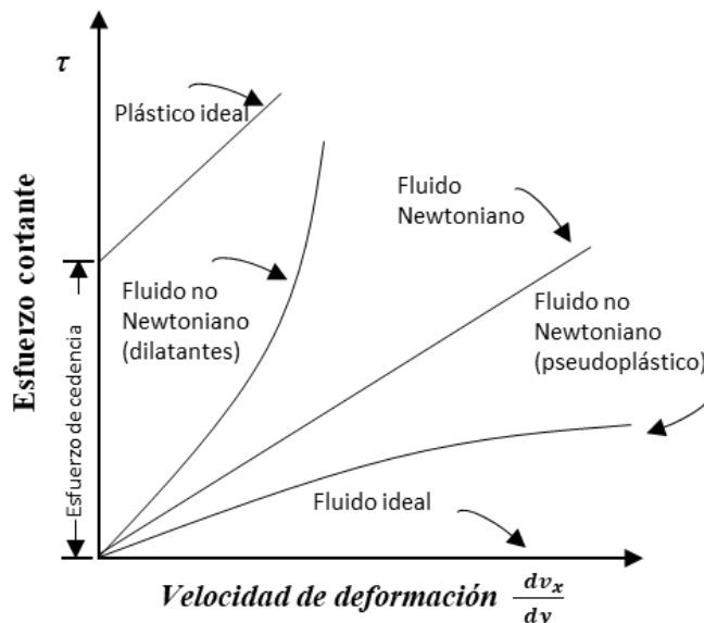
Figura 1.2. Gráfica de la clasificación de los fluidos respecto al esfuerzo cortante y su velocidad de deformación.
