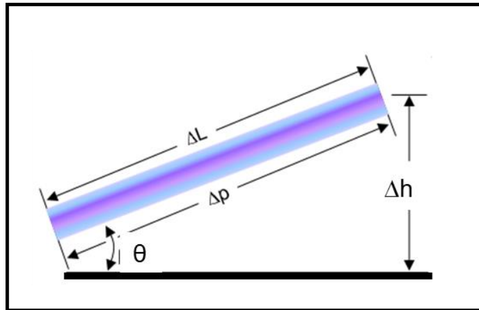
Figura 3.3. La imagen es el esquema donde se representan las características geométricas de una tubería inclinada que permiten determinar las pérdidas de presión por unidad de longitud.
