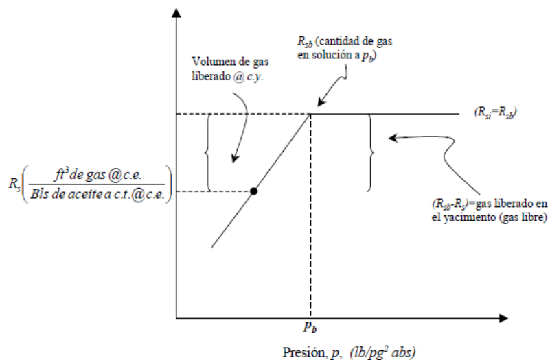
Figura 1.13. Gráfica del comportamiento de la R_s contra la P_y de un yacimiento de aceite negro.
