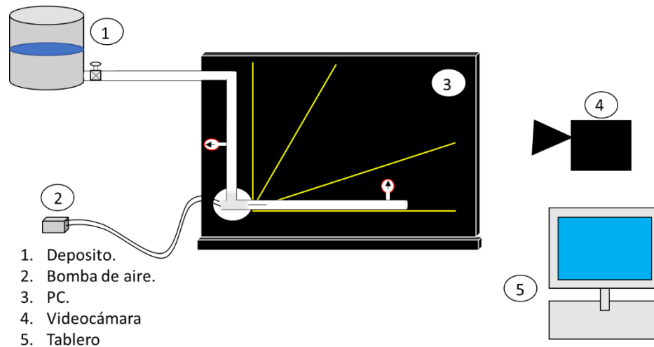
Figura 4.2. Esquema del modelo experimental.
