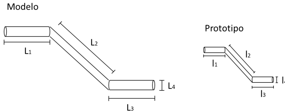
Figura 2.4. Similitud geométrica en una tubería.
