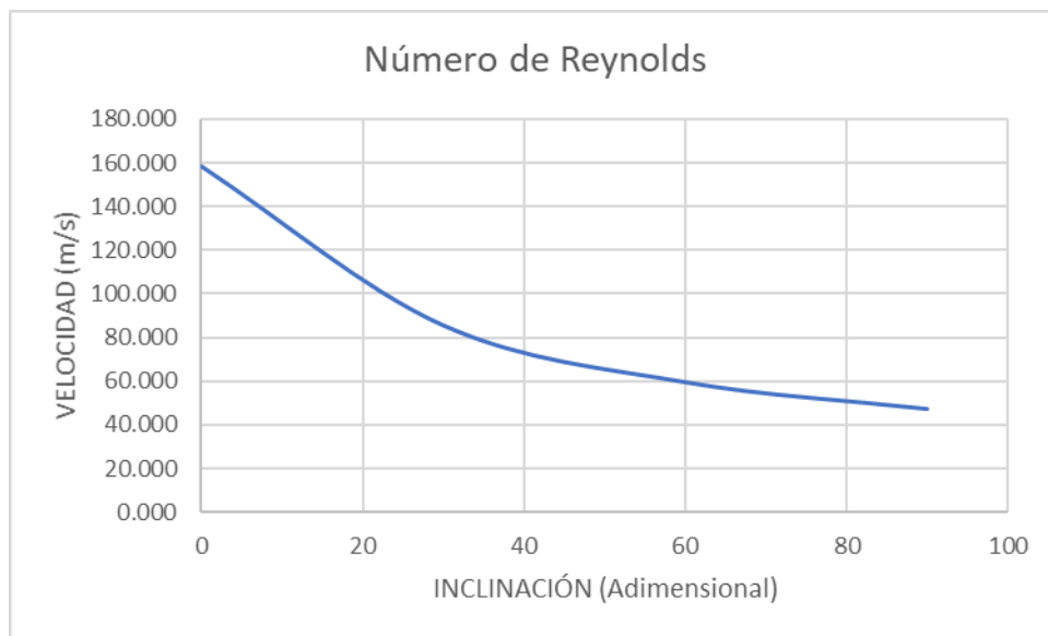
Figura 4.17. Comportamiento del número de Reynolds con respecto al ángulo de inclinación para un gasto bajo.
