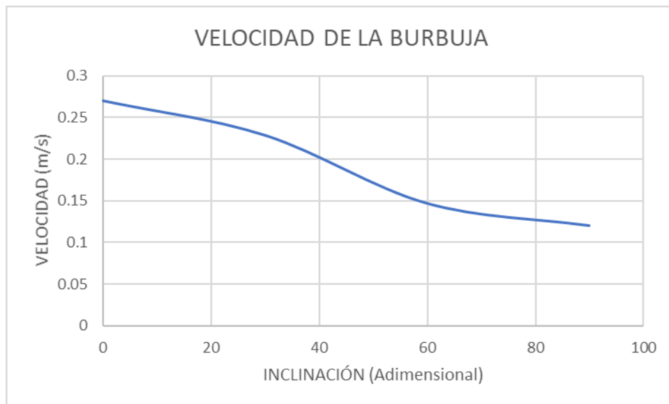
Figura 4.20. comportamiento de la velocidad de burbuja con respecto al ángulo de inclinación para un gasto alto.
