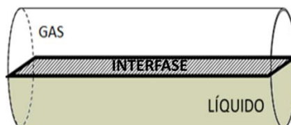
Figura 3.1. Representación de la interfase formada por un gas y un líquido.
