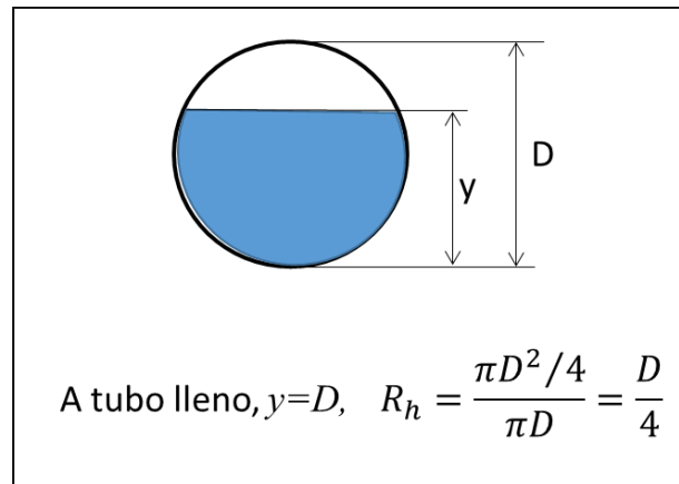
Figura 3.7. Esquema que ilustra el área mojada, el perímetro mojado que permiten definir el perímetro mojado en la tubería.
