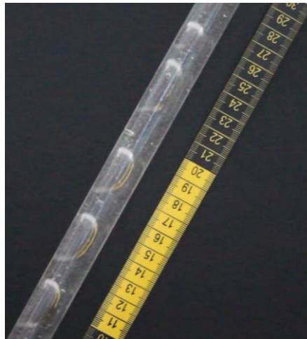
Figura 4.10. Fotografía donde se aprecia el Patrón de flujo intermitente de bache de líquido.
