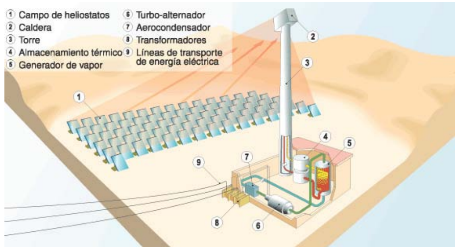
Figura I.10 Central solar fototérmica
