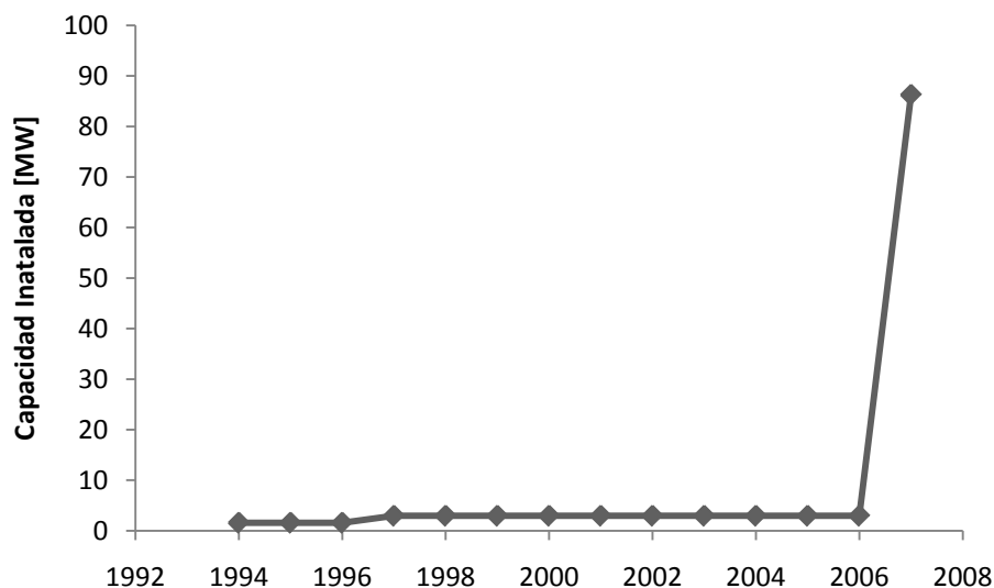
Figura IV.4 Capacidad Instalada en México (1994 a 2008)
