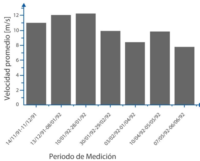
Figura III.12 Resultados obtenidos en La Mata, Oaxaca
