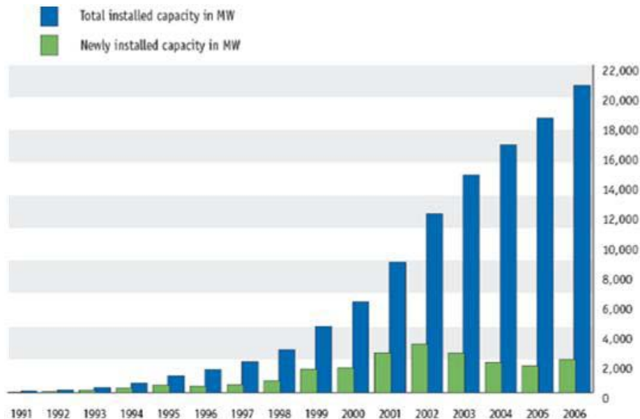
Figura II.6 Evolución de la energía eólica
