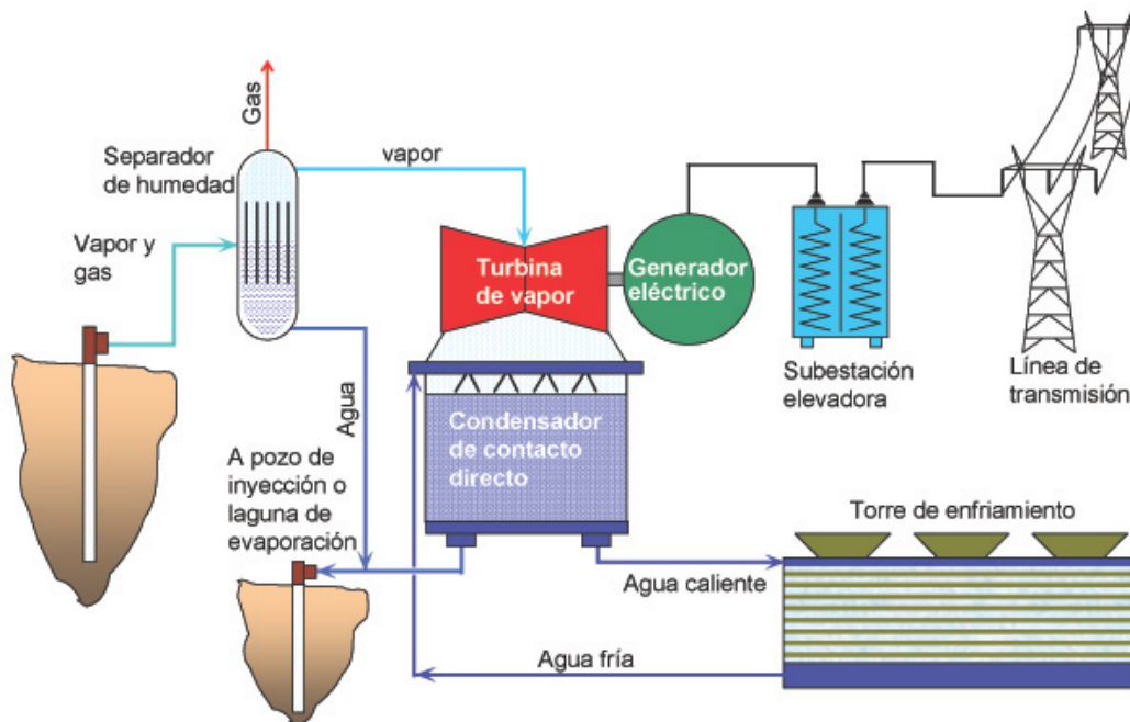
Figura I.8 Central geotermoeléctrica
