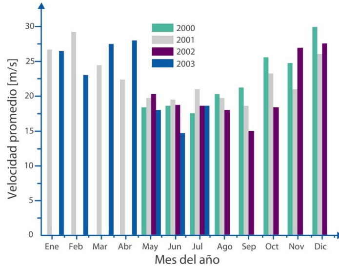
Figura III.16 Velocidad máxima del viento a 32 m de altura sobre el nivel del terreno
