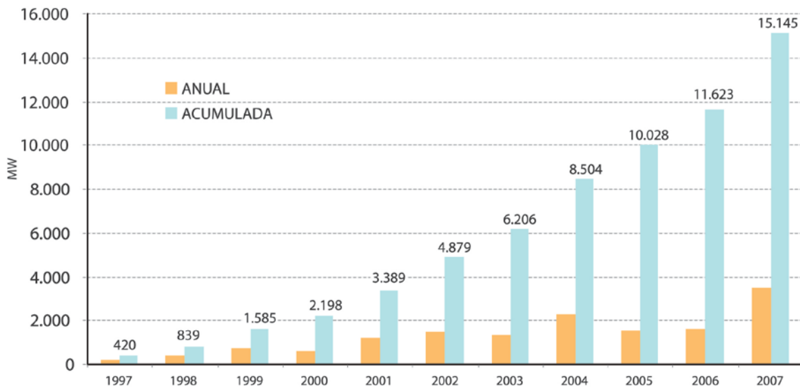
Figura II.2 Evolución anual de la capacidad eólica instalada
