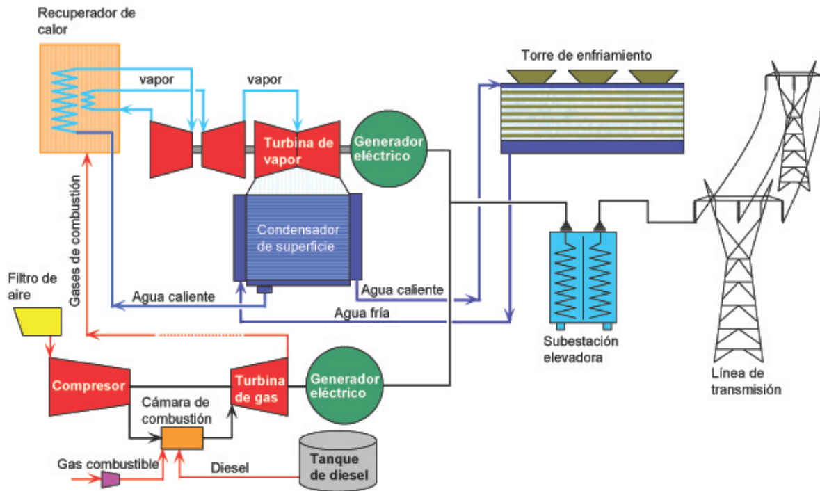
Figura I.5 Central de ciclo combinado
