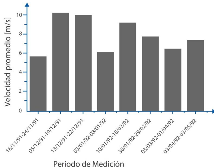
Figura III.14 Resultados obtenidos en Santo Domingo, Oaxaca
