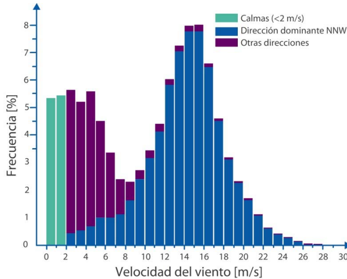
Figura III.17 Distribución de velocidad por rumbos
