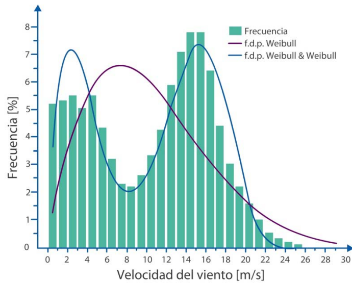
Figura III.18 Función de densidad de probabilidad
