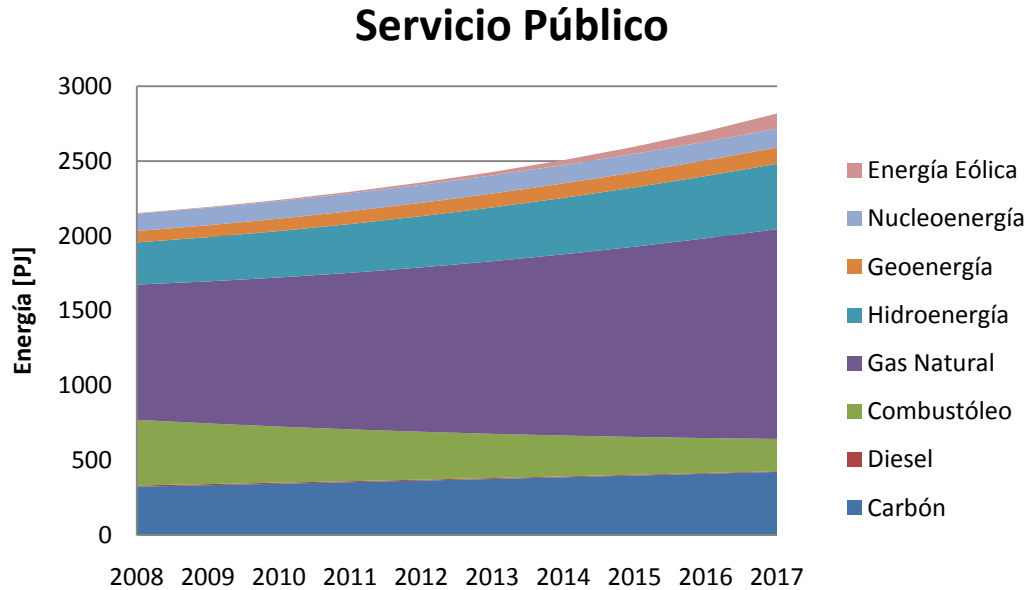
Figura V.6 Energía destinada a transformación de energía eléctrica periodo: 2007 – 2017
