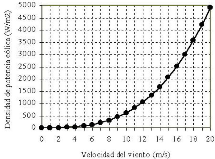
Figura III.7 Densidad de potencia eólica (para una densidad del aire igual a 1.225 \text{ kg/m}^3 )
