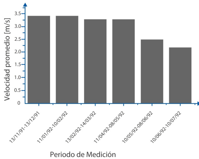
Figura III.13 Resultados obtenidos en Rancho Salinas, Oaxaca
