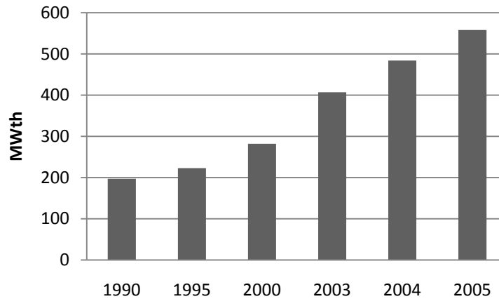
Figura II.4 Evolución de la capacidad instalada con tecnología fototérmica
