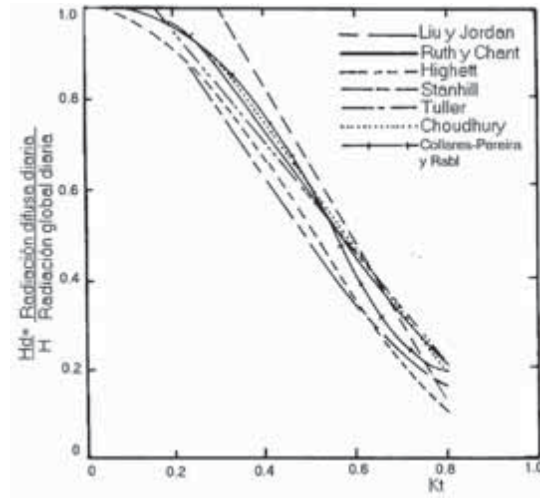
Figura III.9 Comparación de diferentes modelos de radiación difusa
