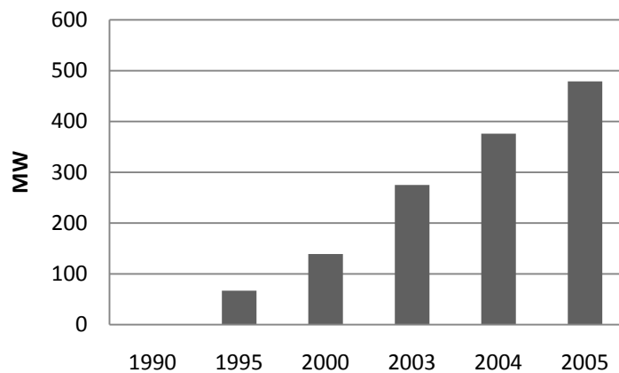
Figura II.12 Evolución de la energía fotovoltaica
