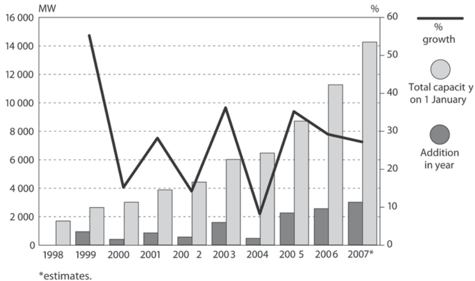
Figura II.10 Evolución de la capacidad instalada eólica
