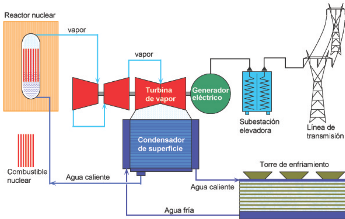
Figura I.6 Central nucleoeléctrica
