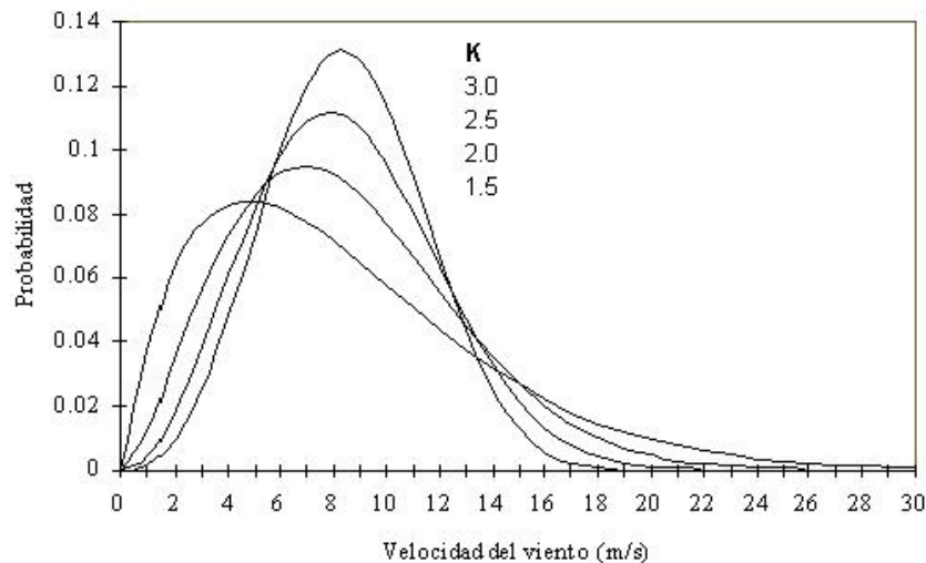
Figura III.5 Ejemplo de una familia de curvas de la función de densidad de probabilidad de Weibull para una velocidad media de 8 m/s
