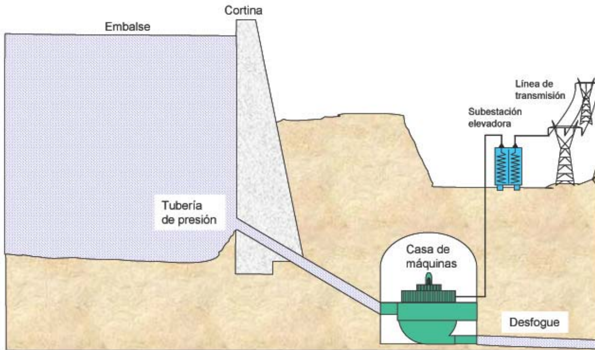
Figura I.7 Central hidroeléctrica
