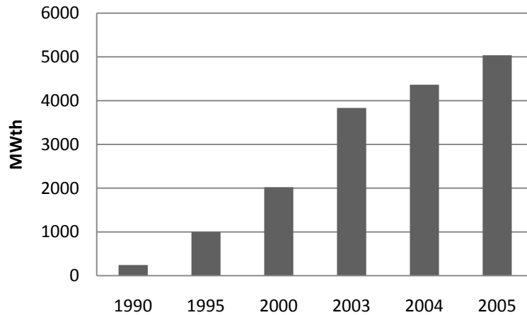
Figura II.7 Evolución de la energía fototérmica
