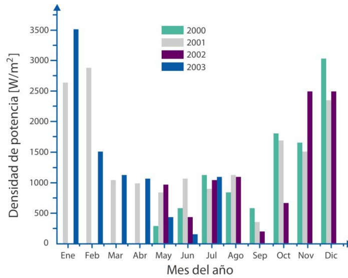
Figura III.19 Densidad de potencia
