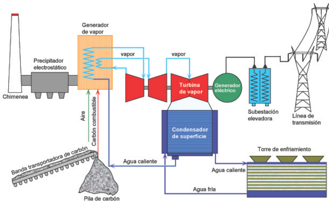
Figura I.2 Central carboeléctrica
