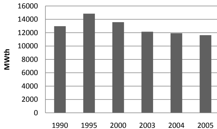
Figura II.11 Evolución de la energía fototérmica
