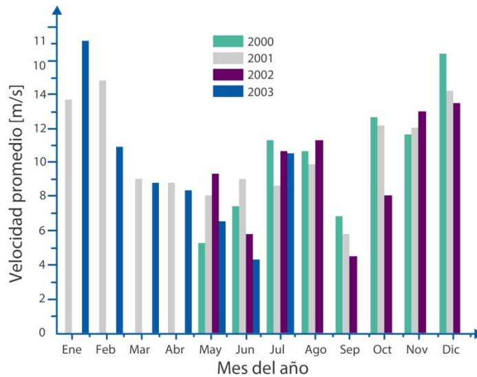
Figura III.15 Velocidad media del viento a 32 m de altura sobre el nivel del terreno
