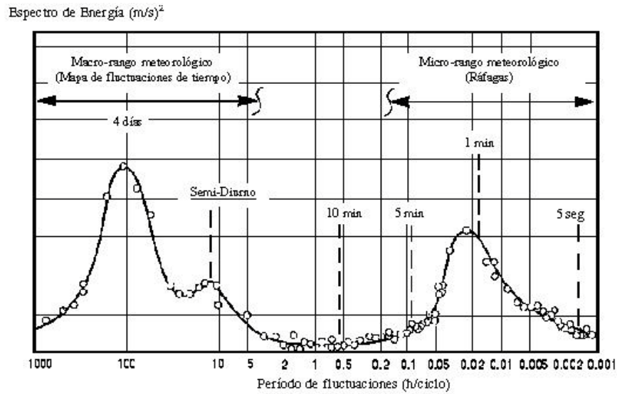
Figura III.2 Espectro energético del viento
