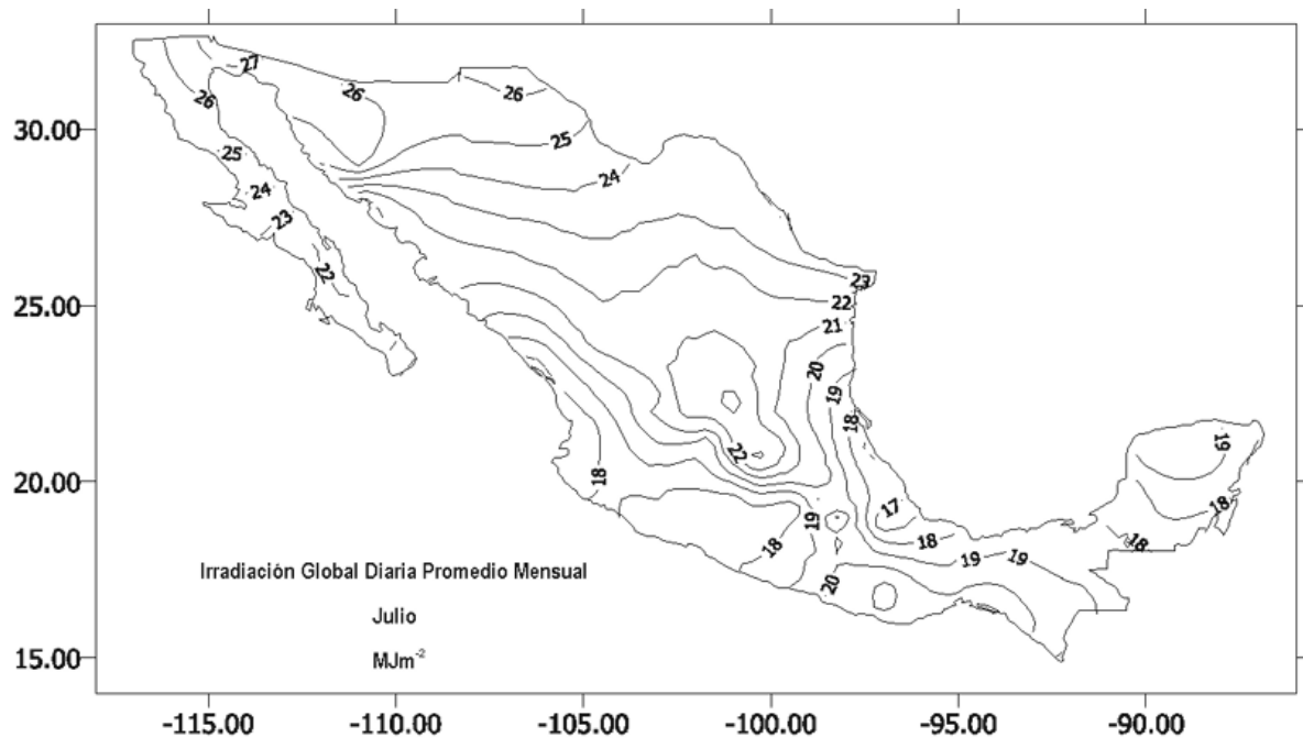
Figura III.21 Irradiación global diaria promedio mensual (MJm -2 ), en julio
