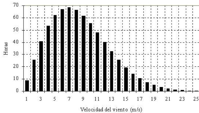
Figura III.3 Ejemplo del histograma de velocidad de viento para un período mensual
