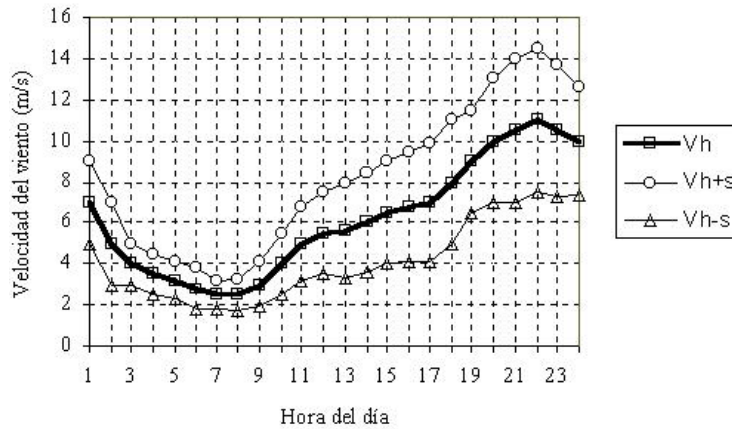
Figura III.4 Ejemplo del patrón diario de velocidad de viento para un período mensual
