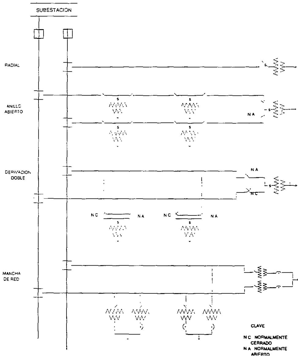
Figura 1 - Estructuras de alimentación.
