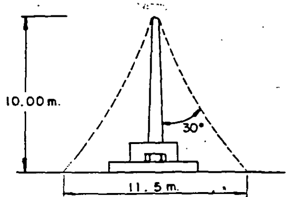
Figura 1A - ZONA DE PROTECCION DE LOS ELECTRODOS
