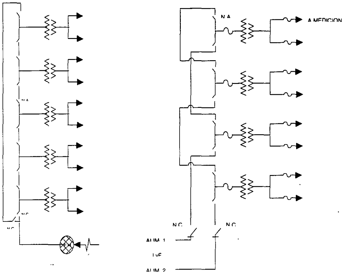
a) Un usuario en M.T. con transformadores en varios niveles.
