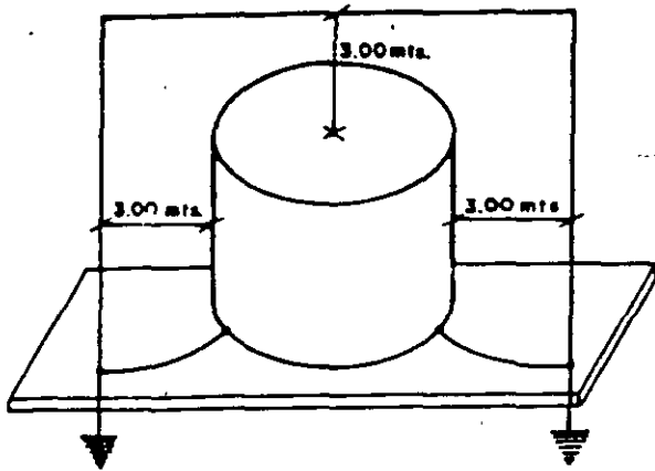
Figura 5 - DEPOSITO DE COMBUSTIBLE CON BLINDAJE
