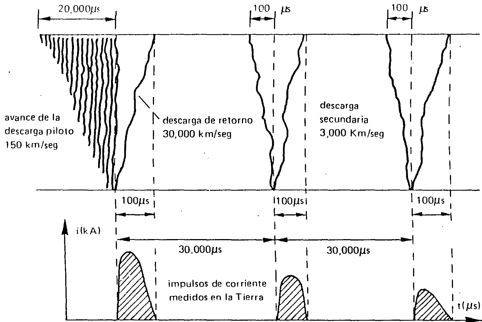
Figura 10.12 Representación esquemática del proceso de descarga de una nube de tormenta según Schonland y Collens.
