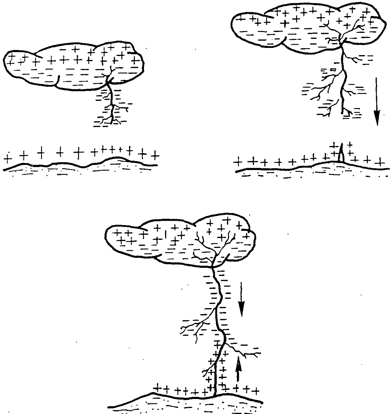
Figura 10.11 Formación del canal plasmático nube-tierra según Schonland. A medida que avanza la descarga piloto las cargas (+) sobre la superficie terrestre se aglomeran, hasta que finalmente le salen al encuentro a las cargas (-), quedando así establecido el referido canal.
