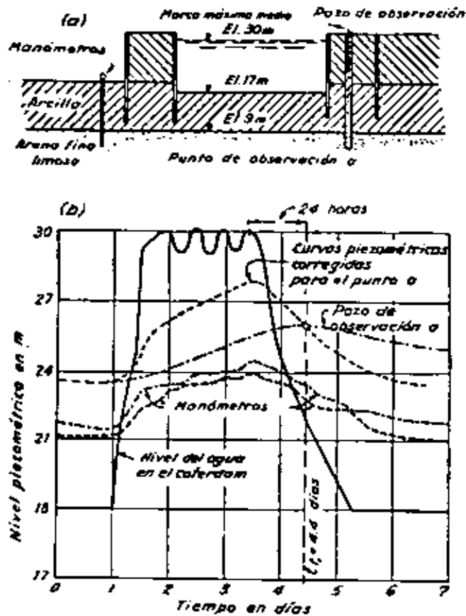
Fig. 69.1. (a) Sección transversal de una ataguia apoyada en arcilla que descansa sobre arena; (b) niveles piezométricos correspondientes al nivel del agua en la arena (según Fitz Hugh et al., 1947).
