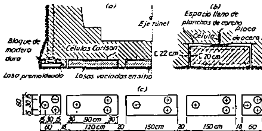
Fig. 67.2. Instalación usada para medir la presión de contacto en la base del túnel del subterráneo de Chicago. (a) Media sección transversal por el intradós mostrando las losas de medición; (b) sección transversal de detalle de una losa; (c) planta con la disposición de las losas (según Terraghi, 1943a).
