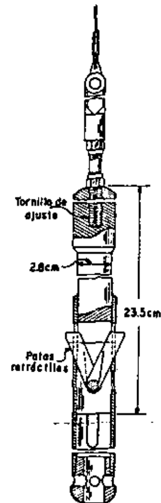
Figura XIII-3. El torpedo para medir asentamientos (Ref. 1).
