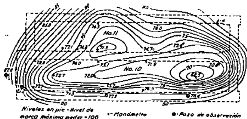
Fig. 69.5. Curvas de igual nivel piezométrico para el estrato de arena situado debajo de los diques de carena de fig. 69.1 (a).
