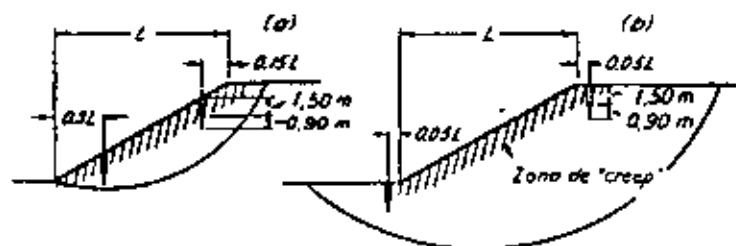
Fig. 66.8. Posición de los puntos de observación para detectar el movimiento de un talud. (a) Si se espera un deslizamiento por un círculo de pie; (b) si puede producirse una rotura por la base.
