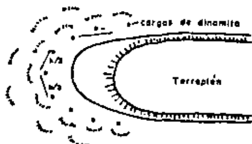
Figura III-9. Desplazamiento de tubas por barrenación en el frente de avance (Ref. 20).
