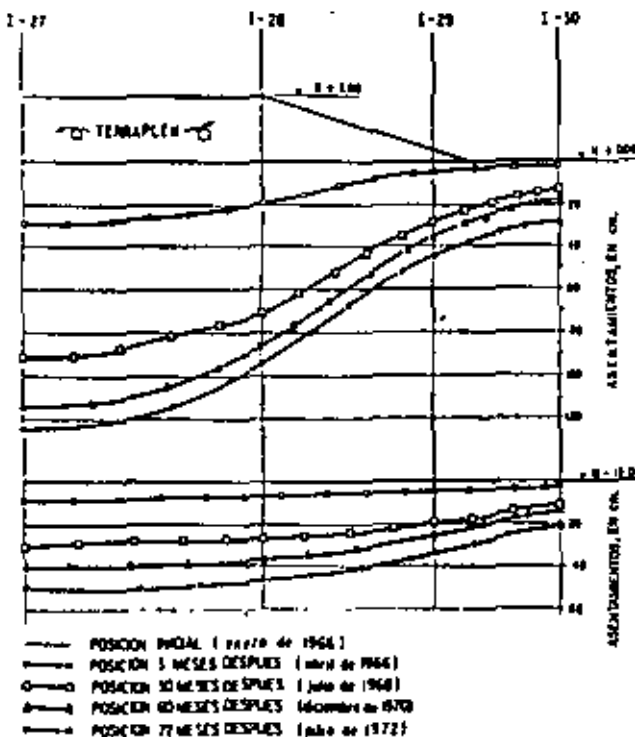
Figura VI-44. Resultados de medición con torpedos de asentamiento, en una sección del mismo terraplén de prueba a que se refiere la figura VI-43.
