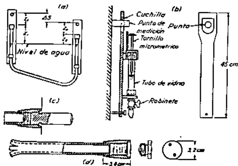
Fig. 66.2. (a) Diagrama esquemático de un nivel de agua; (b) detalle de los tubos de vidrio y del tornillo micrométrica utilizados para medir; (c) punto de observación; (d) detalle de la tapa de protección utilizada antes de empujar el caño en su lugar (según Terzaghi, 1938b).
