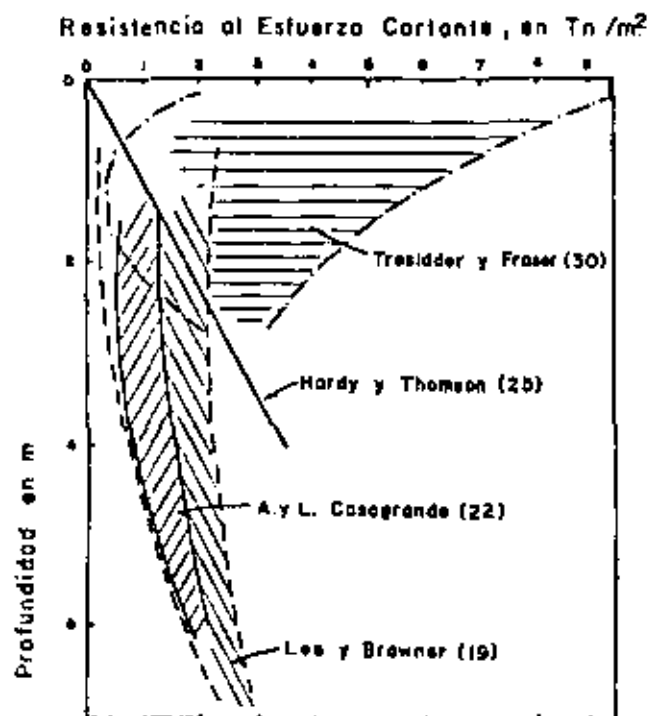
Figura III-7. Resistencia al esfuerzo cortante vs. profundidad, en turbas (Mediciones con veta en el lugar) (Ref. 20).
