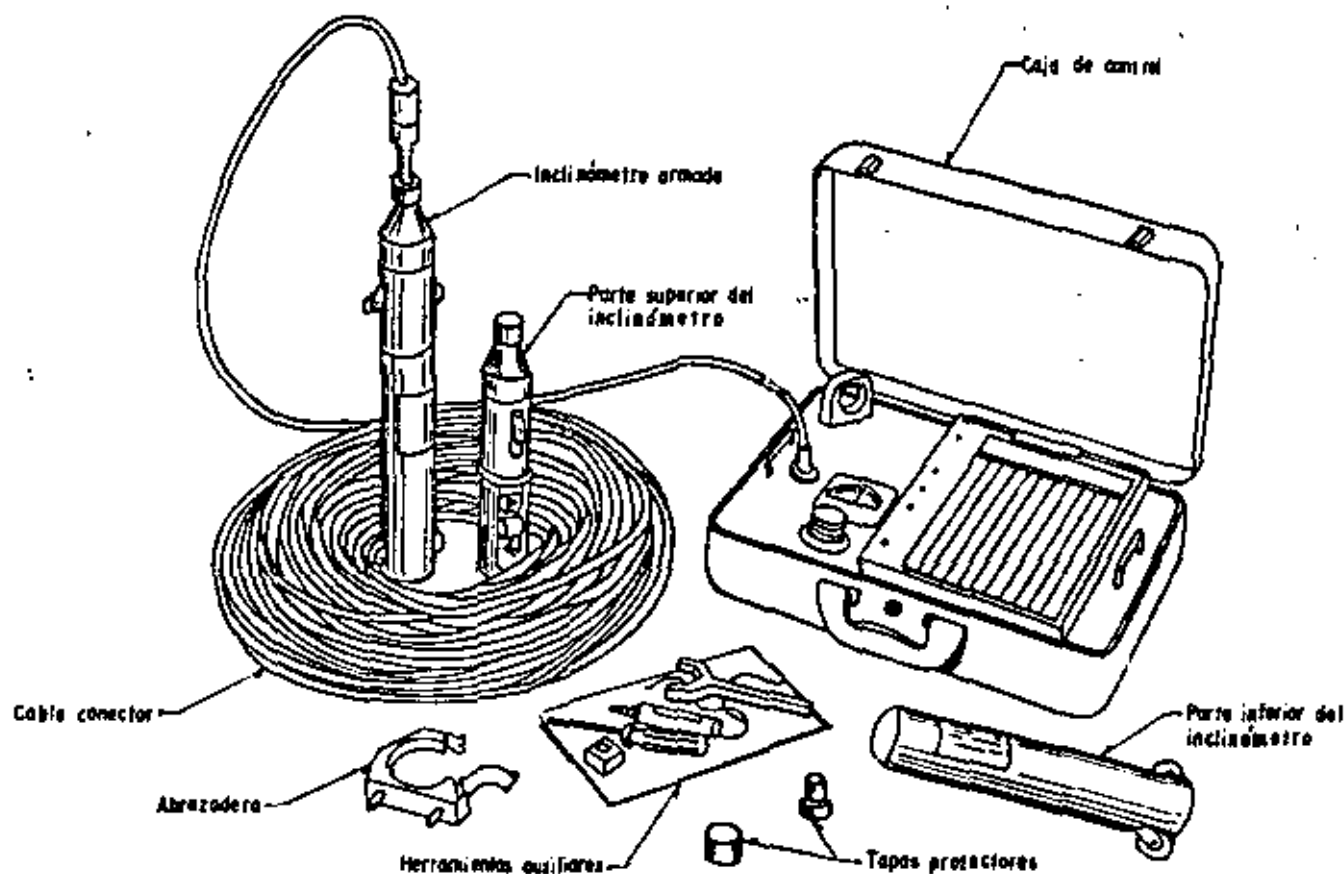
Figura XIII-5. Inclinómetro completo.
