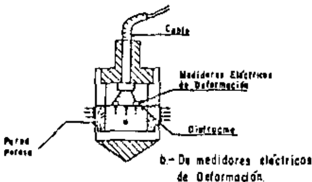
Figura XIII-17. Piezómetros eléctricos
