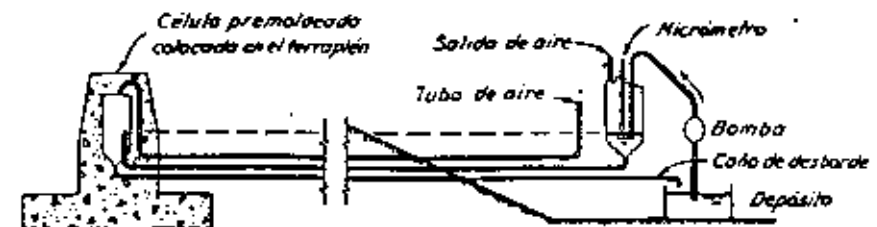
Fig. 66.6. Nivel de agua para medir el asentamiento de un punto en el interior de una presa (según Mallet y Pacquant, 1951).
