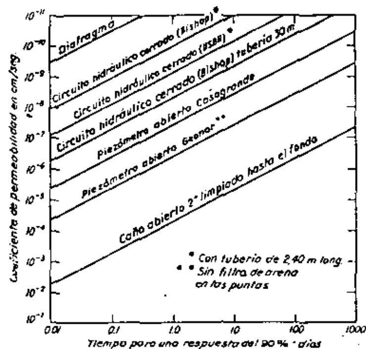
Fig. 68.5. Retardo aproximado de los diferentes tipos de piezómetros (según Ilvarev, 1951; Penman, 1961; Brooker y Lindberg, 1963, y otros).
