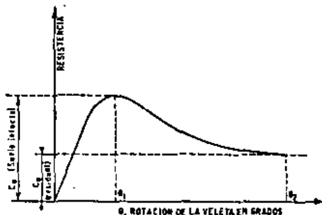
Figura VI-41. Curva típica de resistencia de una arcilla blanda con pruebas de veleta (Ref. 71).
