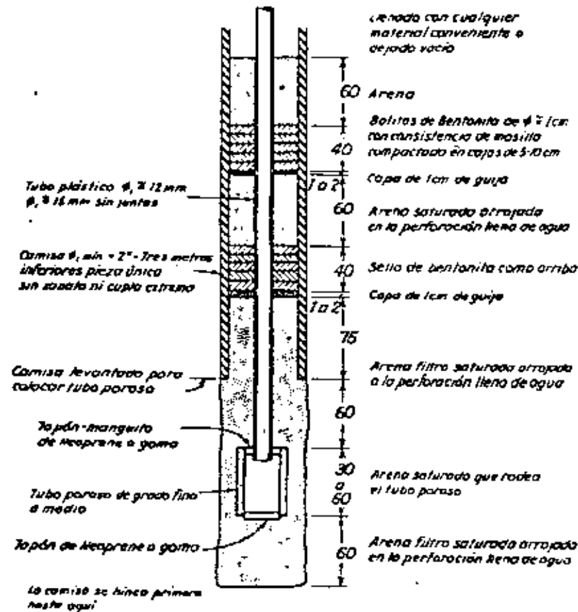
Fig. 68.1. Piezómetro abierto tipo Casagrande (según A. Casagrande, 1949).
