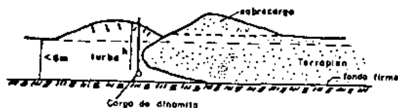
Figura III-9. Desplazamiento de tubas por barrenación en el frente de avance (Ref. 20).
