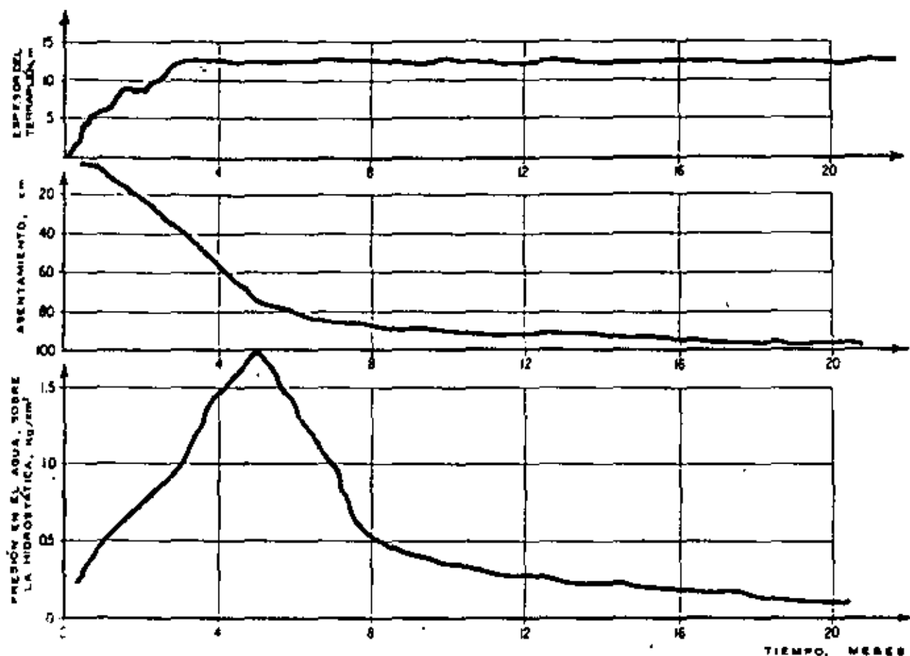
Figura XIII-19. Comparación entre la colocación de la carga, el asentamiento y la evolución de las lecturas piezométricas en el terraplén de acero a un paso a desnivel.
