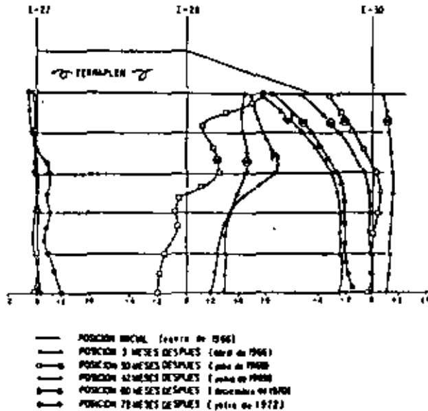
NOTAS: 1.- El inclinómetro I-28 se corrió a los 42 meses de haber los instalados, 2.- En el inclinómetro I-27, solo se dejaron los gráficos para 3, 30 y 72 meses.
