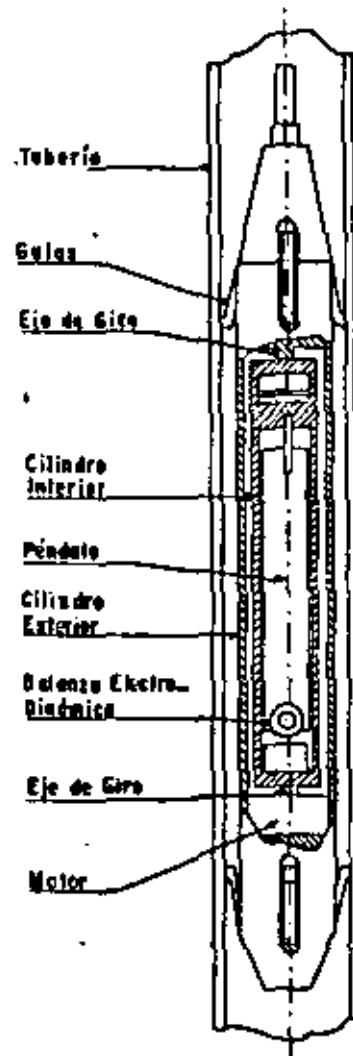
Figura XIII-11. Inclinómetro tipo Geconsult (Ref. 20).
