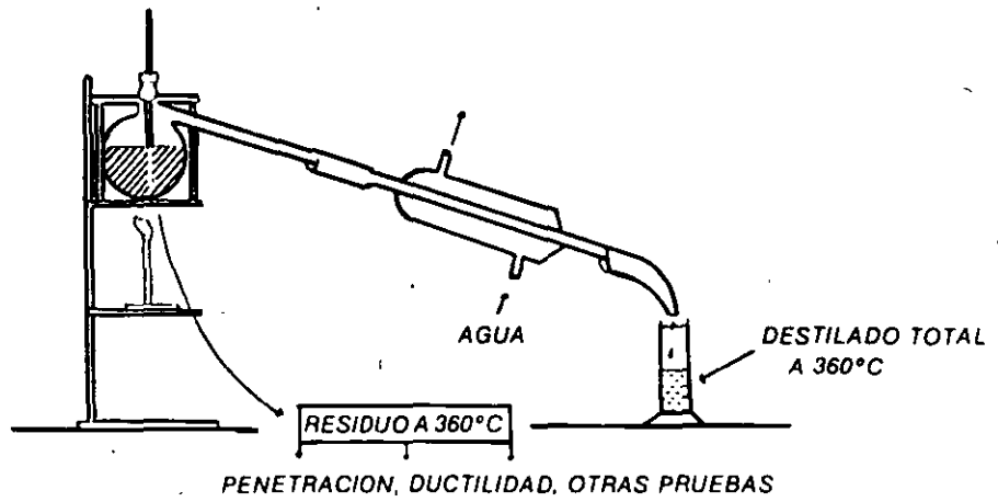
FIGURA 14. PRUEBA DE DESTILACION
