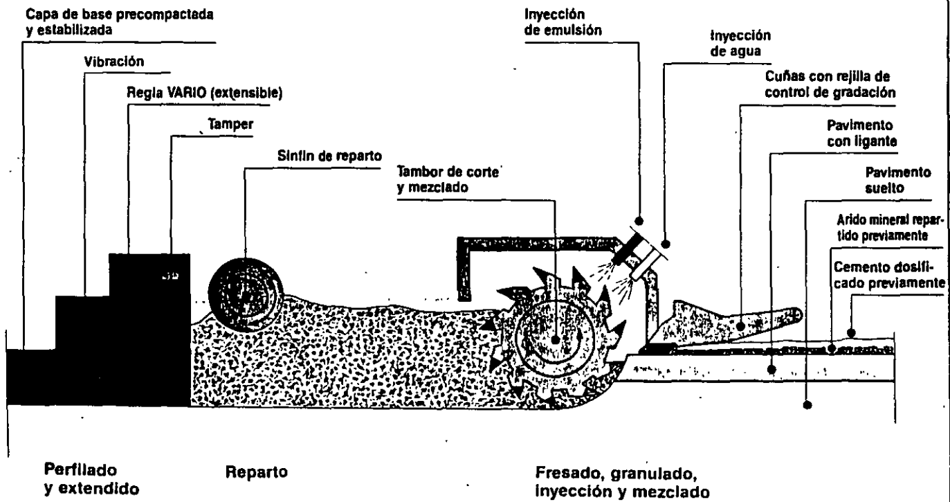
Principio de trabajo del proceso tal como lo realiza la recicladora en frío 2100 DCR.
