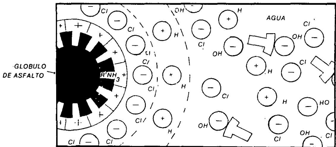
FIGURA 18. ESQUEMA DE LA ESTRUCTURA DE UNA EMULSION CATIONICA
