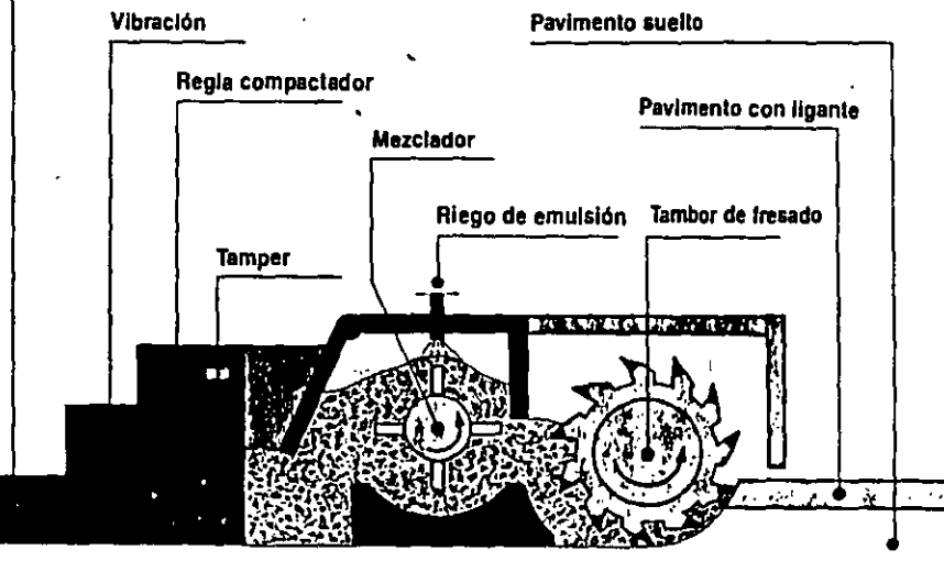
Tratamiento superficial a todo el ancho de calzada.
