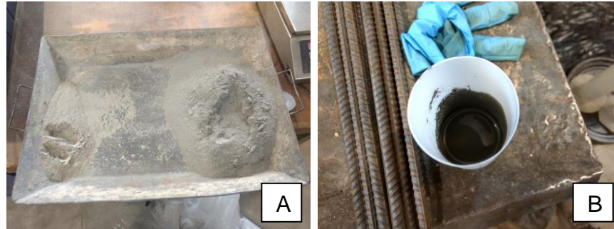
Figura 3.10. Agregados y jales antes de ser mezclados con agua (A). Llenado de moldes cilíndricos (B).
