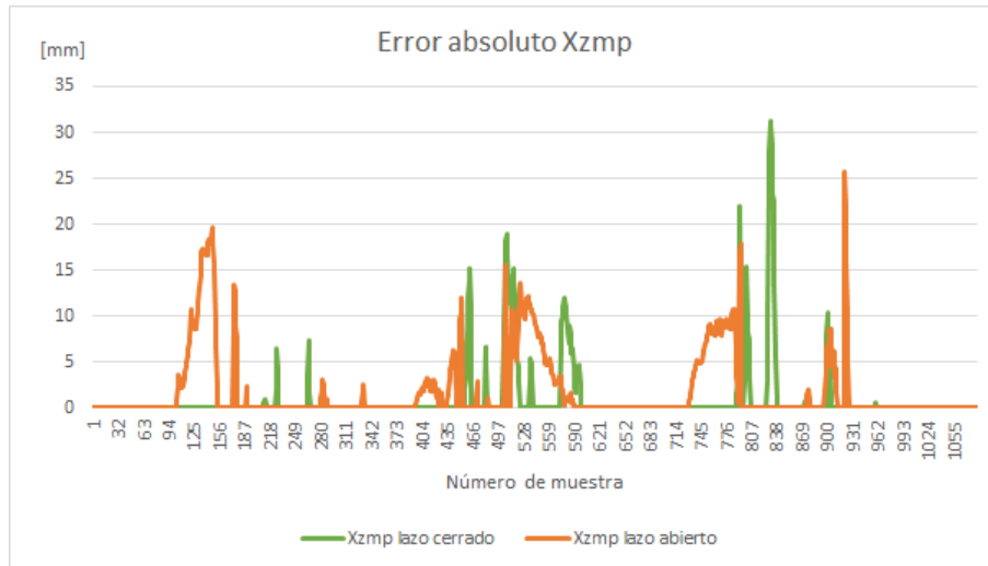
Figura 5.39. Error absoluto en Xzmp durante caminata en superficie inclinada menos cinco grados en dirección roll
