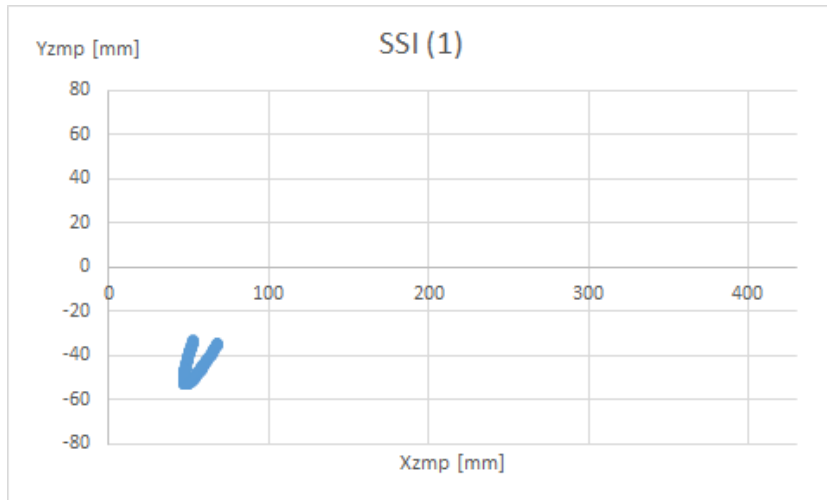
Figura 3.23. ZMP de referencia en XY durante SSI (1)
