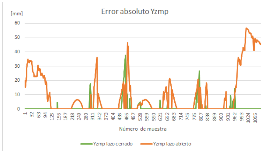
Figura 5.40. Error absoluto en Yzmp durante caminata en superficie inclinada menos cinco grados en dirección roll
