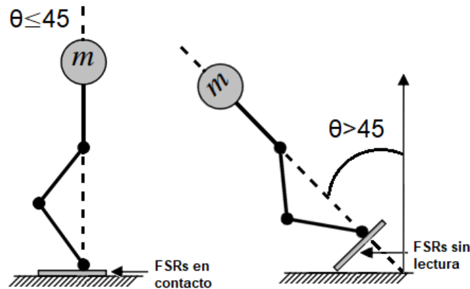
Figura 3.38. Representación de caída del robot 6
