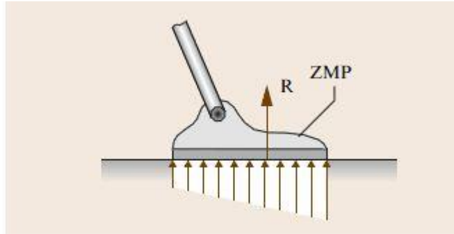
Figura 2.3. Vista lateral de ubicación de ZMP en suela de un robot bípedo [50]
