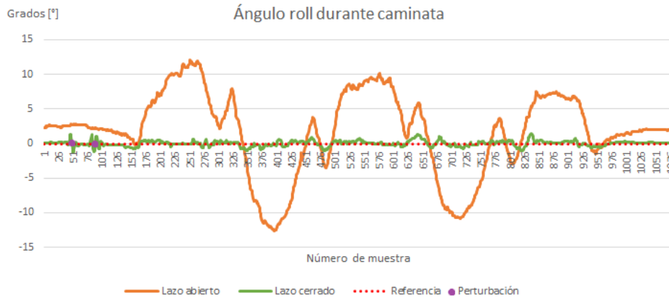
Figura 5.2. Ángulos roll de la cadera durante la caminata sobre superficie horizontal
