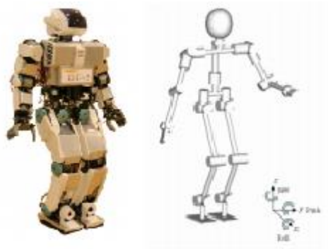
Figura 1.11. Fotografía y estructura de KHR-1 [27]
