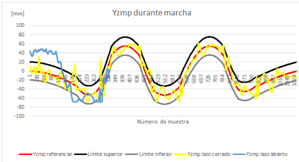
Figura 5.44. Coordenada Y del ZMP durante caminata con carga
