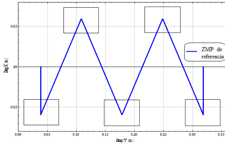
Figura 2.13. ZMP propuesto para diseño de caminata de robot bípodo Scout [3]
