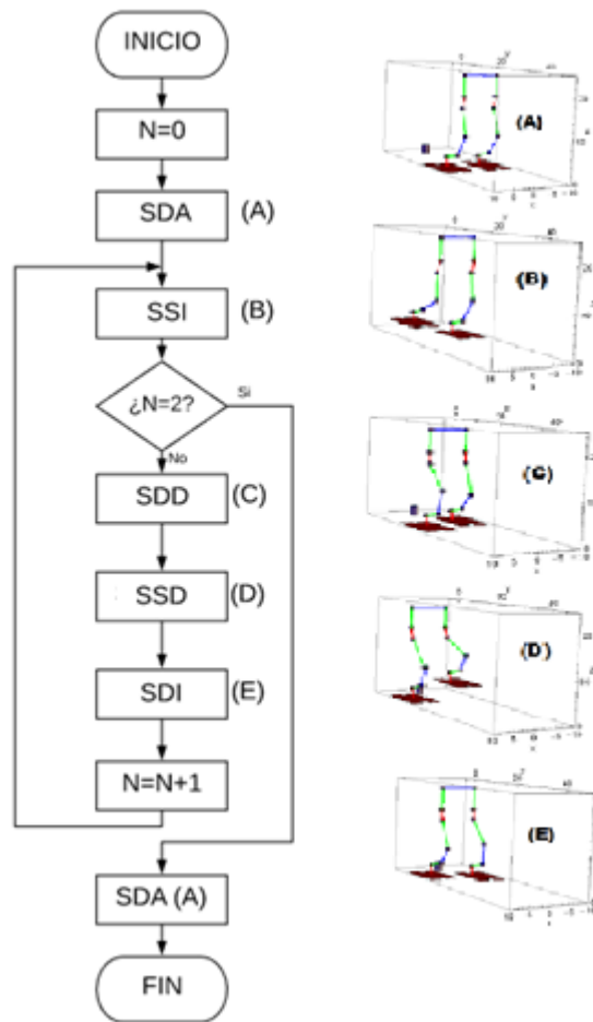
Figura 2.17. Diagrama de flujo de caminata diseñada con representación simulada y algoritmo Diagrama basado en [83]
