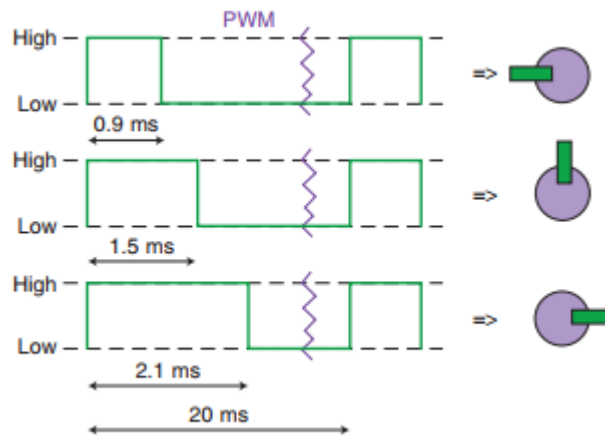
Figura 2.6. Ejemplo de funcionamiento de servo a través de PWM [55]
