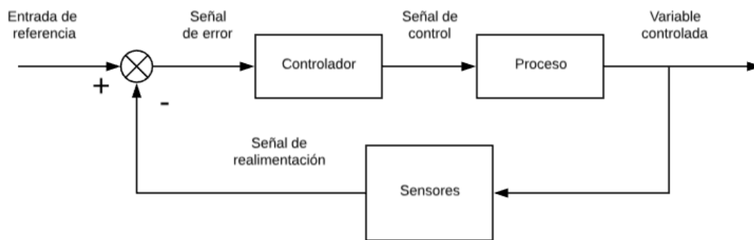
Figura 4.3. Ejemplo de diagrama de bloques de un sistema de lazo cerrado
