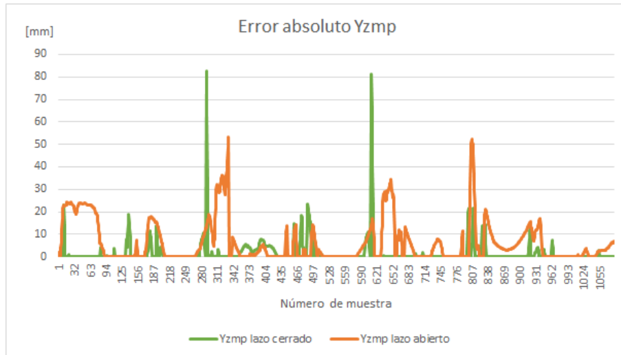
Figura 5.34. Error absoluto en Yzmp durante caminata en superficie inclinada menos cinco grados en dirección roll
