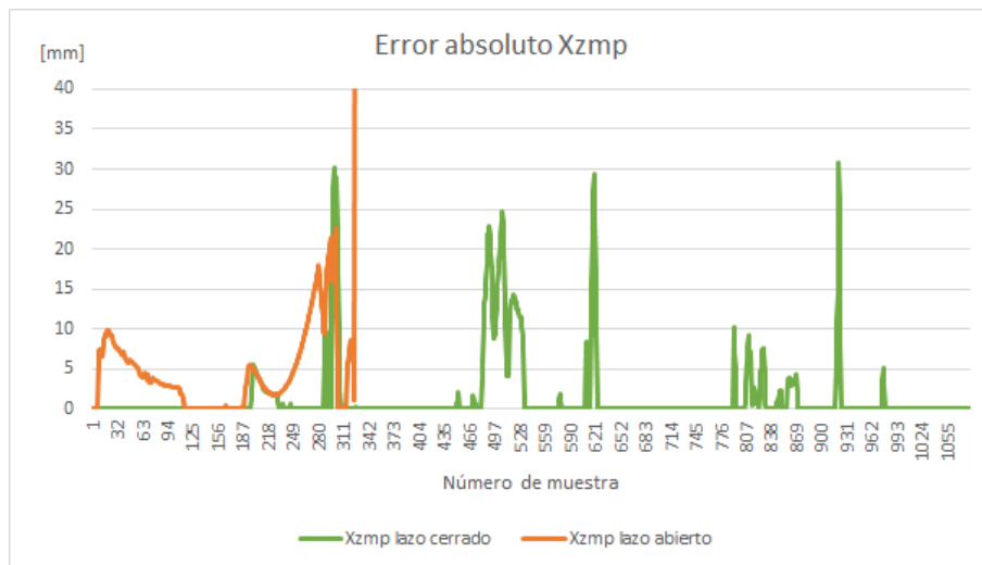
Figura 5.46. Error absoluto en Xzmp durante caminata con carga
