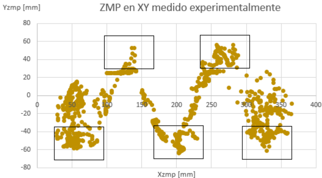
Figura 3.13. ZMP experimental en ejes XY
