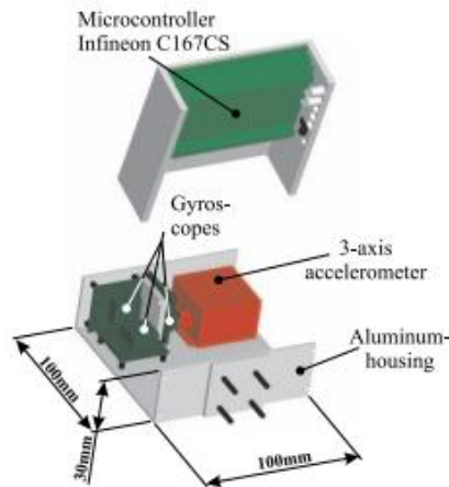
Figura 1.26. Unidad de medición inercial de robot Johnnie [41]
