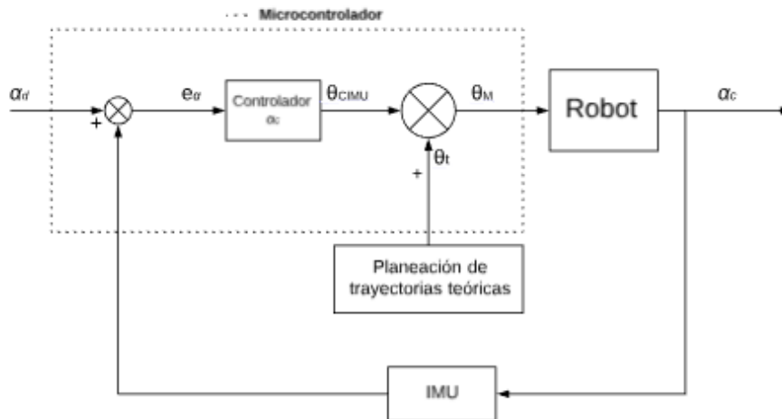
Figura 4.4. Diagrama de bloques del sistema de control de ángulos de la cadera del robot bípedo
