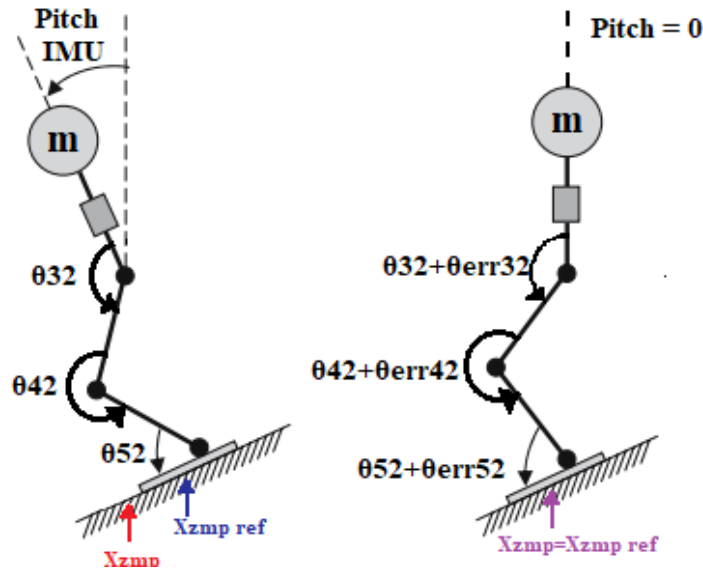
Figura 4.8. Corrección de postura de robot bípedo en plano sagital 7
