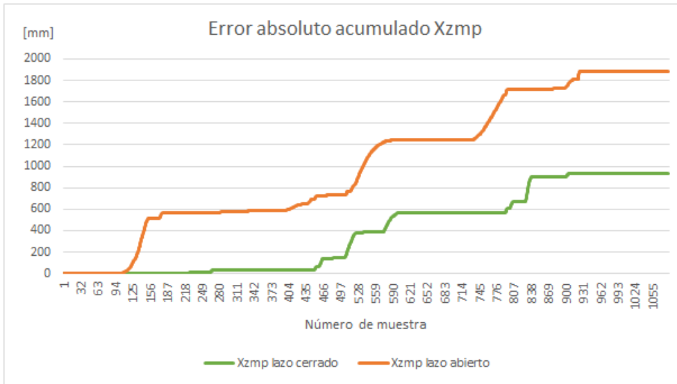
Figura 5.41. Error absoluto acumulado en Xzmp durante caminata en superficie inclinada cinco grados en dirección roll
