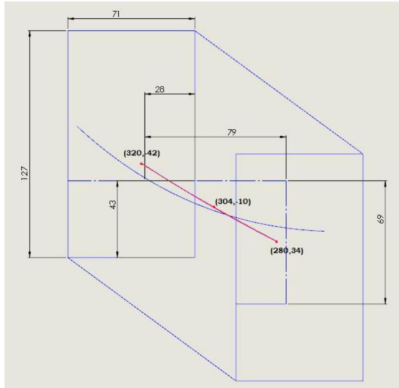
Figura 3.20. Propuesta de trayectoria de ZMP en SDI (2)
