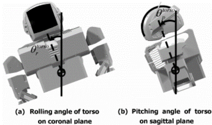
Figura 1.28. Medición inercial en robot KHR-2 [43]
