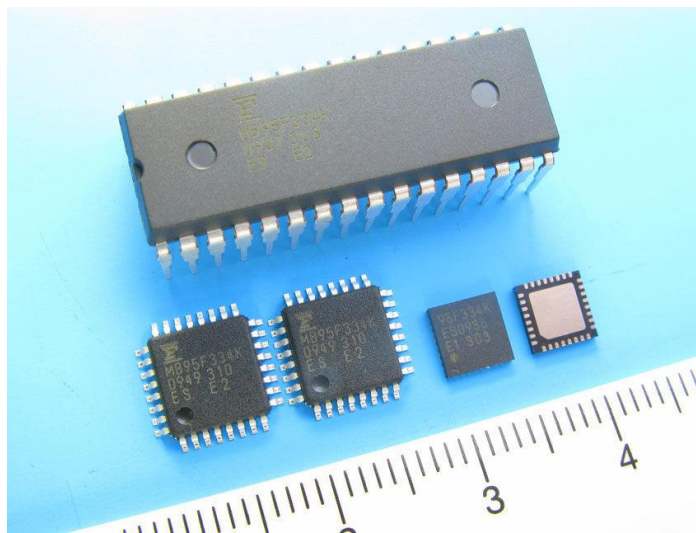
Figura 2.9. Ejemplos de microcontroladores en diferentes presentaciones [57]
