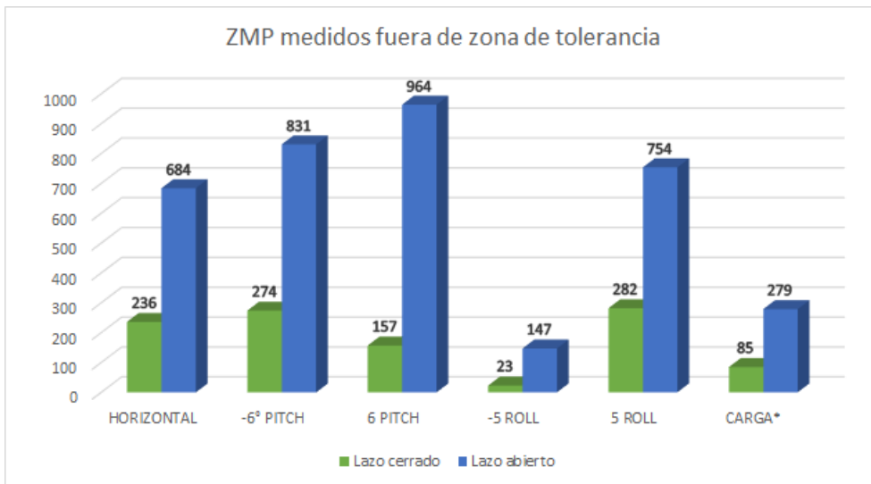
Figura 5.50. ZMP medidos fuera de zona de tolerancia en lazo abierto y cerrado
