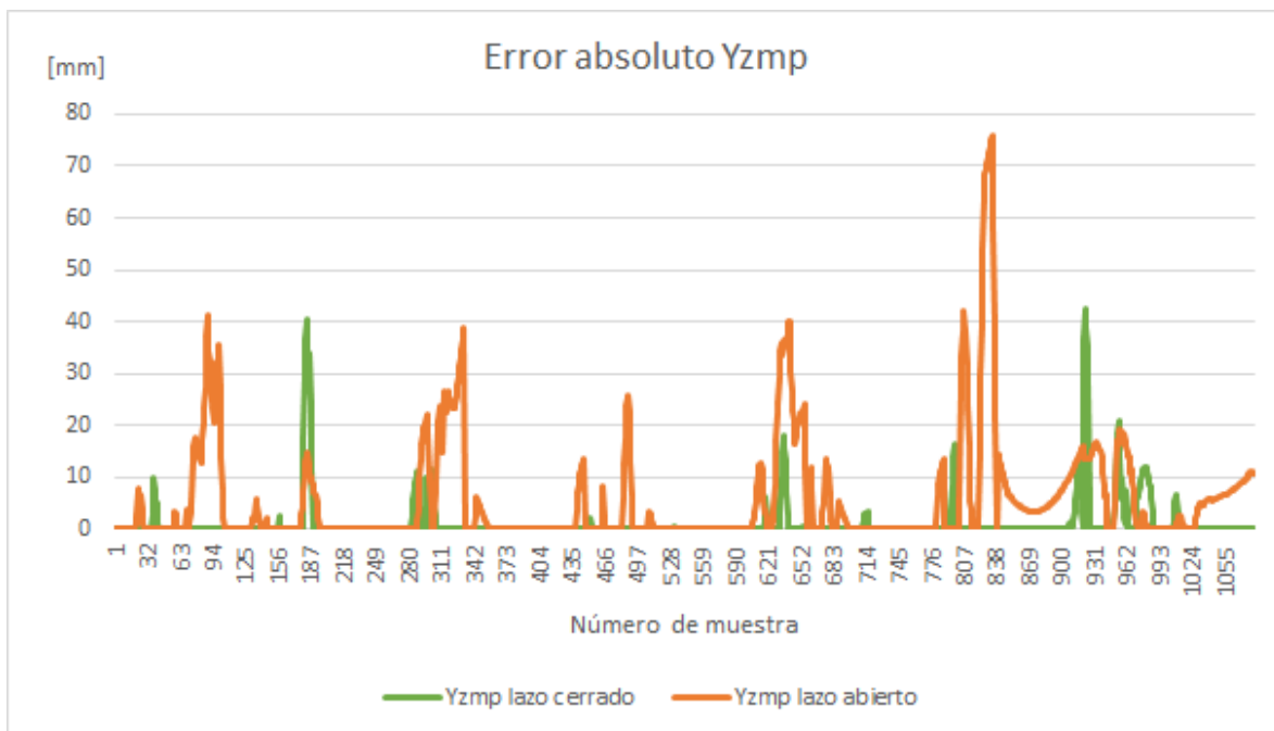
B. Error absoluto en Yzmp durante caminata en superficie inclinada seis grados en dirección pitch
