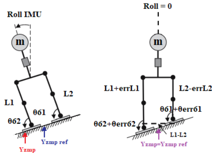
Figura 4.9. Corrección de postura de robot bípedo en plano coronal 8
