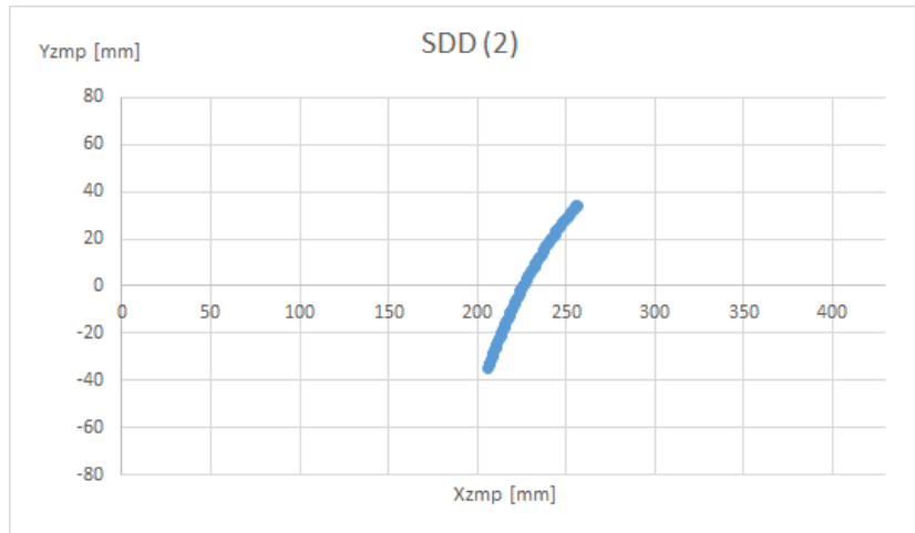
Figura 3.28. ZMP de referencia en XY durante SDD (2)
