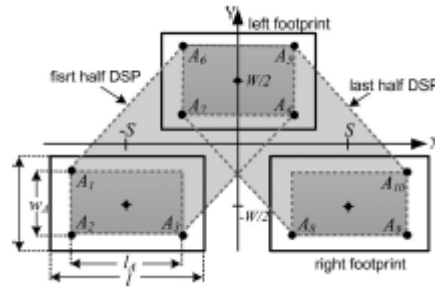
Figura 1.22. Ejemplo de AZR dentro de polígonos de soporte [39]
