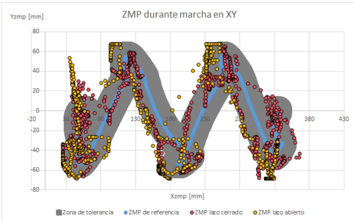
Figura 5.27. ZMP en XY durante caminata en superficie inclinada seis grados en dirección pitch
