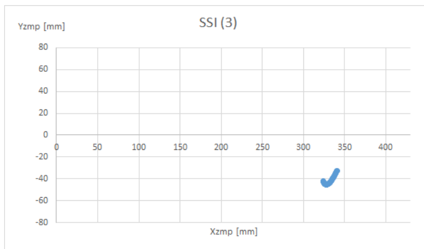
Figura 3.31. ZMP de referencia en XY durante SSI (3)
