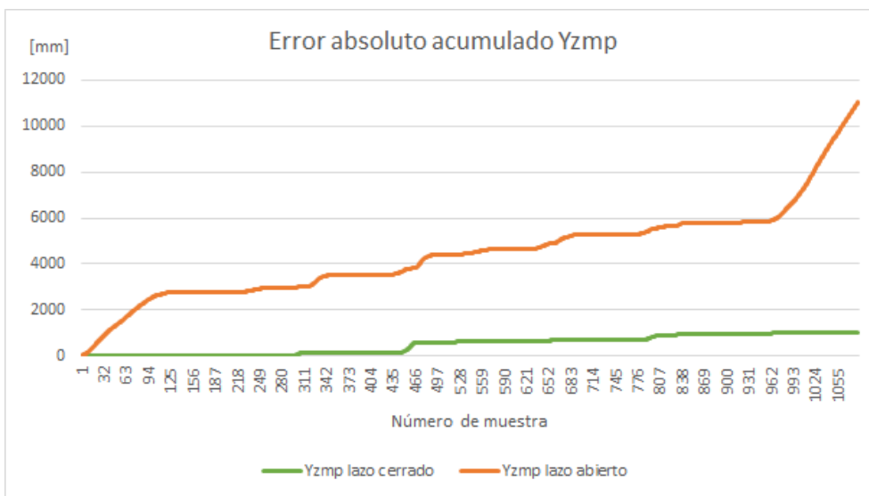
Figura 5.42. Error absoluto acumulado en Yzmp durante caminata en superficie inclinada cinco grados en dirección roll
