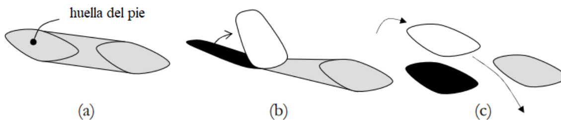
Figura 2.4. Ejemplos de polígonos de soporte [47]
