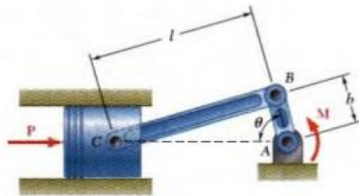
Figura 2.7. Sistema biela-manivela de 1 GDL [48]
