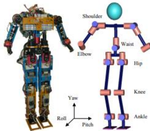
Figura 1.11. Fotografía y estructura de KHR-1 [27]
