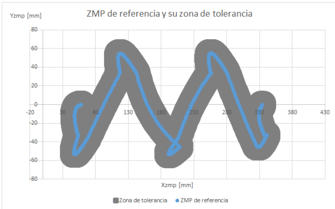
Figura 3.35. Conjunto de puntos de ZMP permisibles durante la marcha
