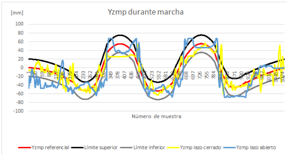
Figura 5.13. Coordenada Y del ZMP durante caminata en superficie horizontal
