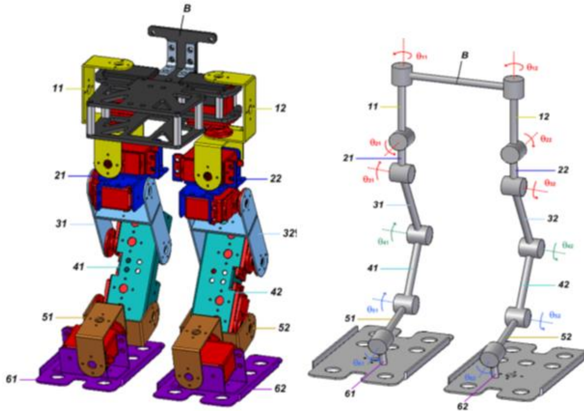
Figura 1.2. Diseño asistido por computadora del robot bípedo y su modelo simplificado [1].
