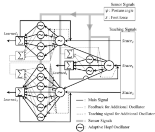
Figura 1.30. Estructura de red de controlador CPG con osciladores [44]
