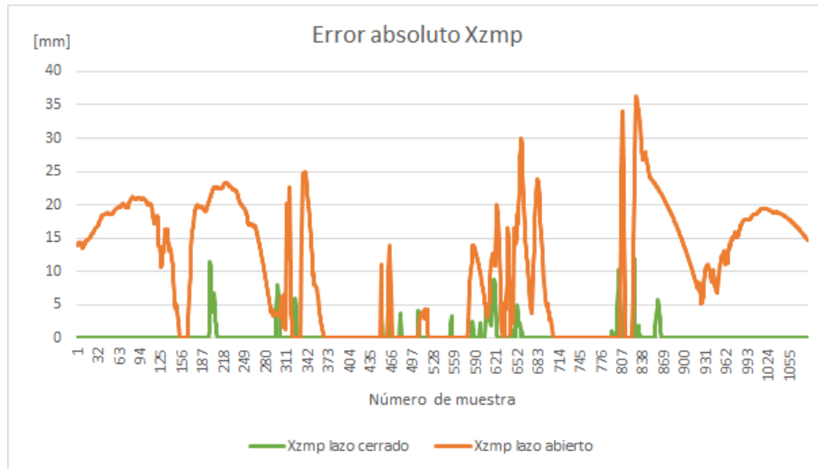
Figura 5.22. Error absoluto en Xzmp durante caminata en superficie inclinada menos seis grados en dirección pitch
