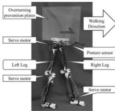
Figura 1.31. Robot de 7 GDL con sensor de postura [44]
