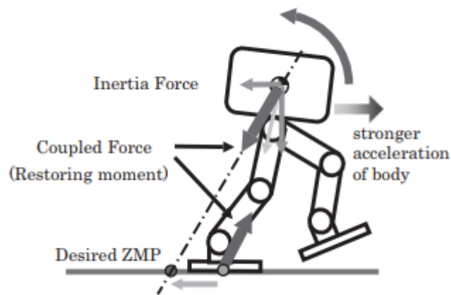
Figura 1.9. Aplicación de un ZMP deseado como parámetro de control en ASIMO [15]
