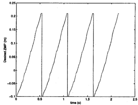
Figura 1.20. Coordenada X del ZMP deseado de un robot de 7 GDL durante la marcha [36]
