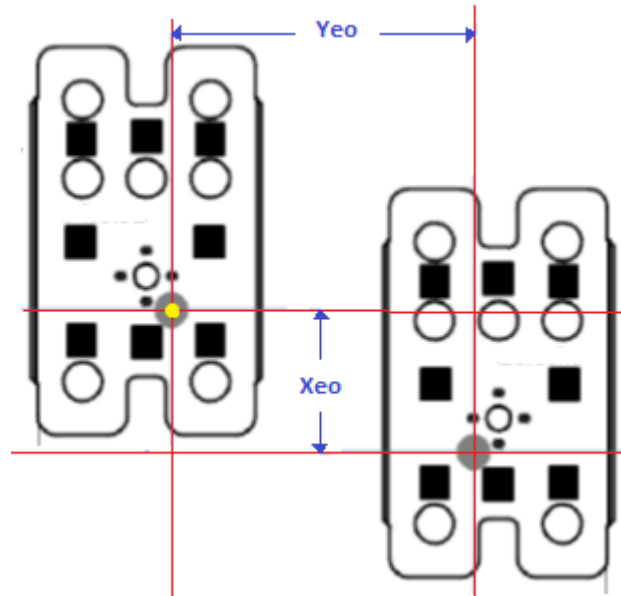
Figura 3.10. Representación de distancias X_{eo} e Y_{eo} 4
