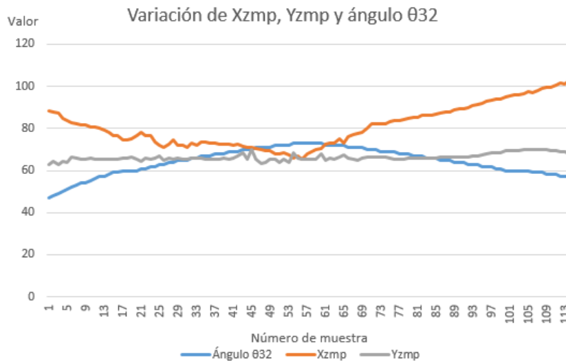
Figura 4.7. Efecto del giro del ángulo del motor 32 en las coordenadas del ZMP en SSD
