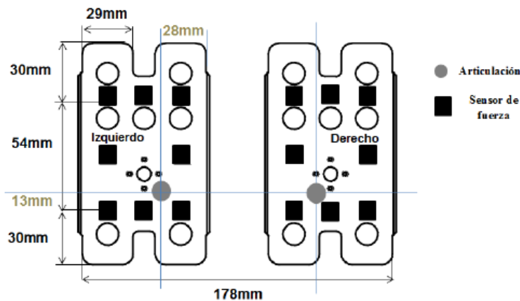
Figura 2.20. Sistema de arreglos de sensores de fuerza en la planta de los pies del robot bípedo [4]
