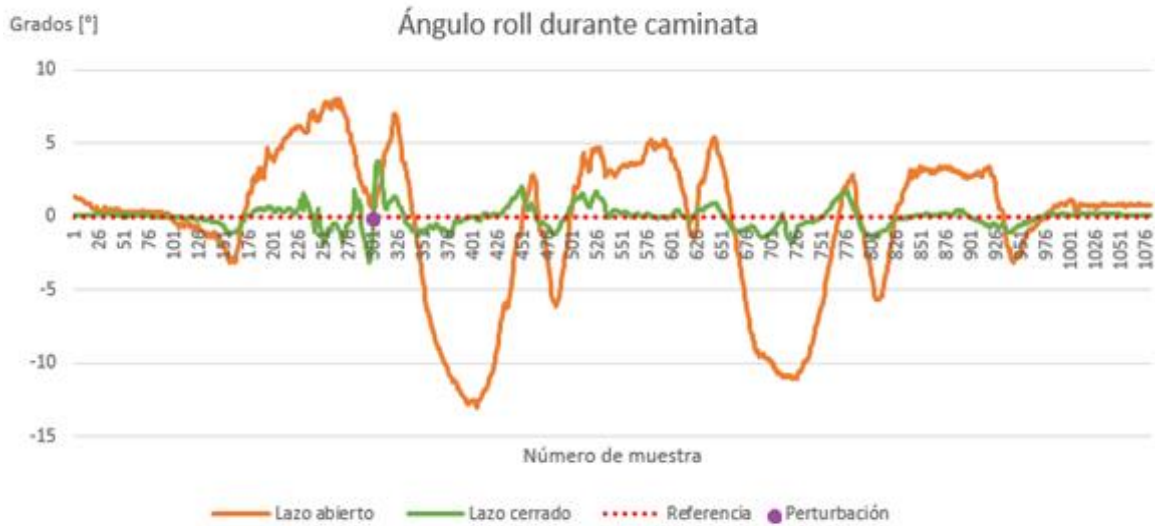
Figura 5.4. Ángulos roll de la cadera durante la caminata sobre superficie inclinada menos cinco grados en dirección pitch
