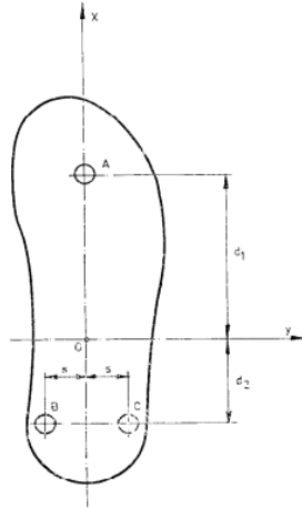
Figura 1.17. Posición de componentes en medición del ZMP en 1972 [34]
