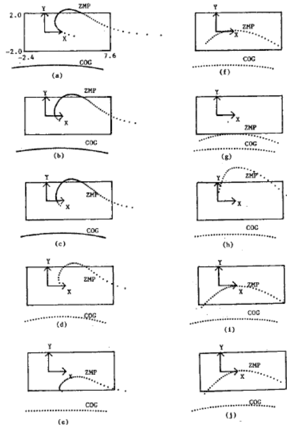
Figura 1.19. Diseño de trayectorias del ZMP durante la fase de soporte simple en 1990 [35]
