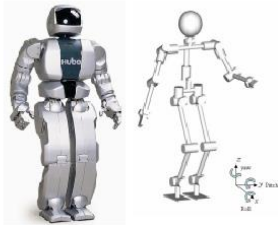
Figura 1.13. Fotografía y estructura de HUBO [29]
