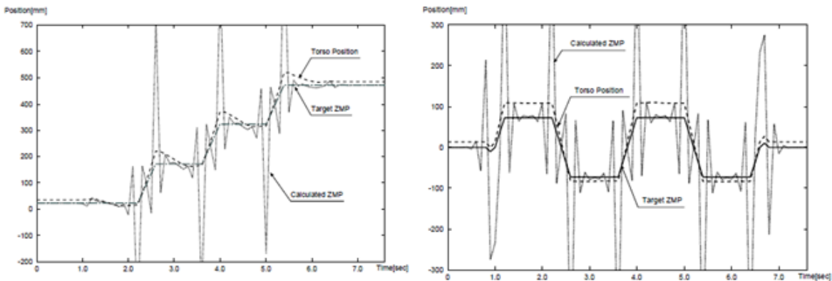
Figura 1.21. Resultado de aplicación de un sistema de control de ZMP en robot h5 [37]
