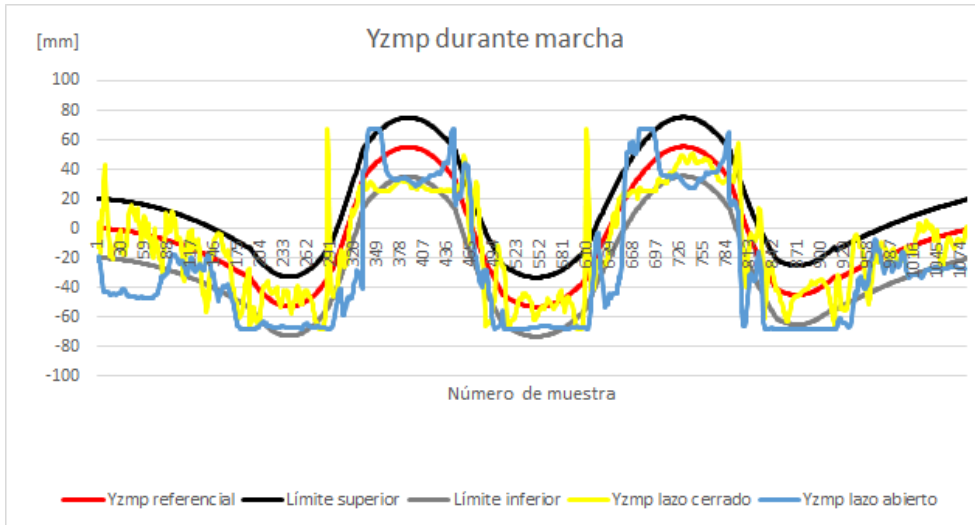
Figura 5.31. Coordenada Y del ZMP durante caminata en superficie inclinada menos cinco grados en dirección roll
