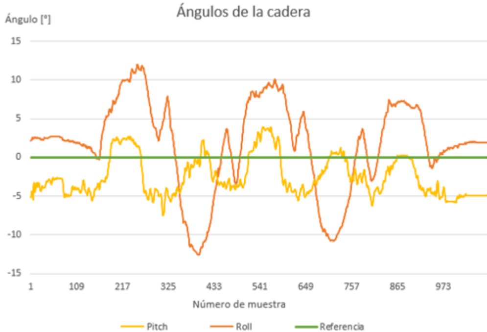
Figura 3.6. Ángulos medidos pitch y roll de la cadera durante marcha
