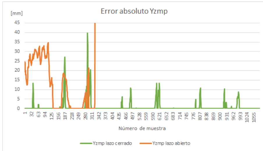
Figura 5.47. Error absoluto en Yzmp durante caminata con carga
