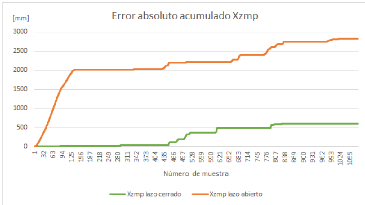
D. Error absoluto acumulado en Xzmp durante caminata en superficie inclinada menos seis grados en dirección roll
