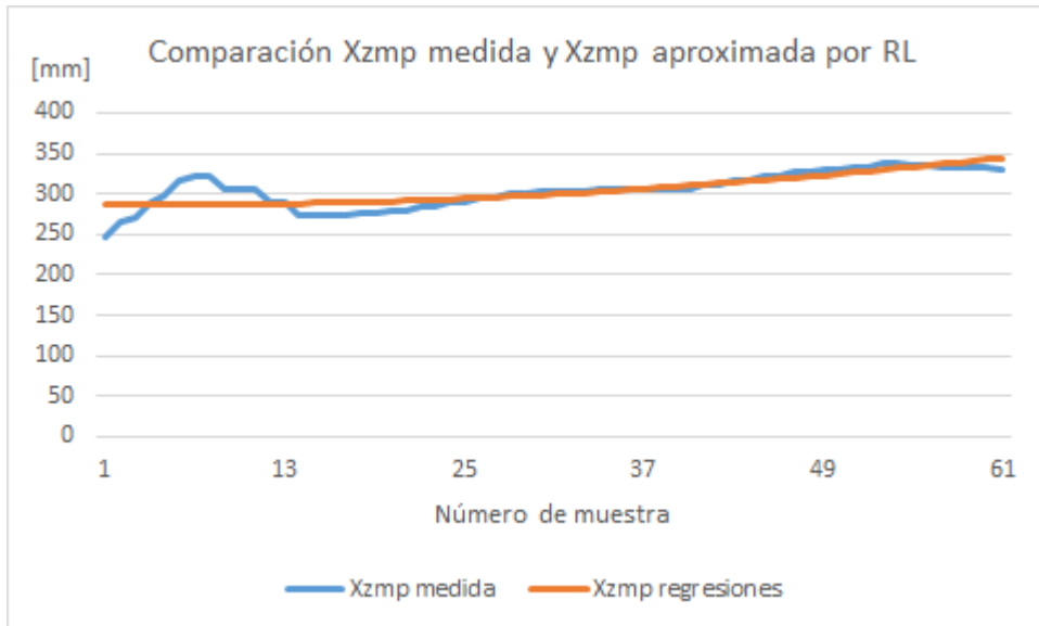
Figura 3.14. Xzmp medido y Xzmp aproximado por regresión lineal en fase SDI (2)
