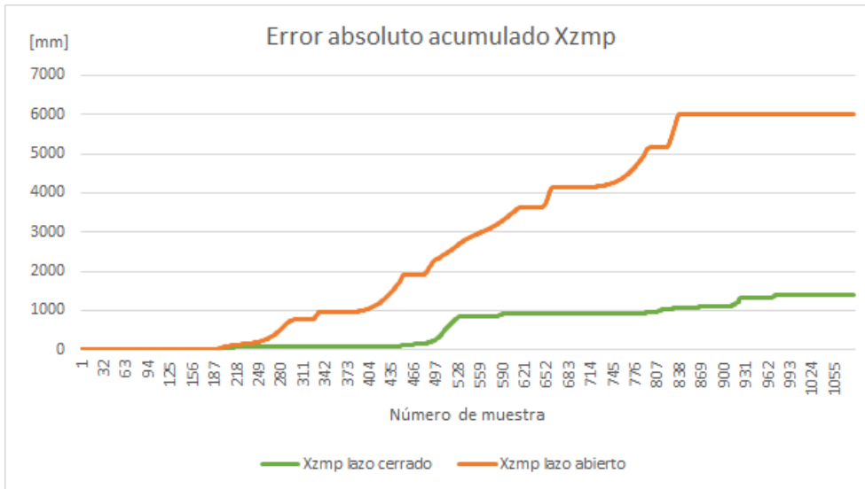
Figura 5.29. Error absoluto acumulado en Xzmp durante caminata en superficie inclinada seis grados en dirección pitch
