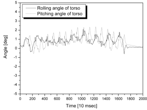
Figura 1.29. Ángulos de torso de KHR-2 durante caminata [43]
