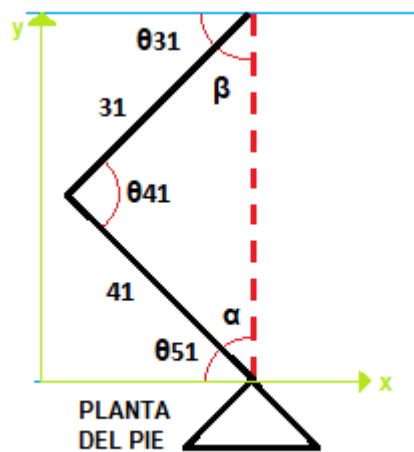
Figura 3.5. Representación cinemática de los eslabones de la rodilla
