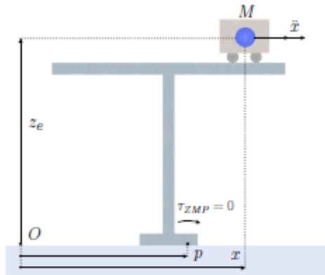
Figura 2.11. Representación de modelo simplificado carro-mesa [12]
