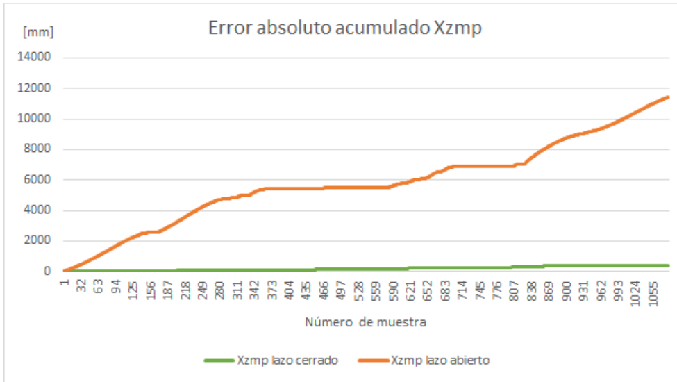
Figura 5.24. Error absoluto acumulado en Xzmp durante caminata en superficie inclinada menos seis grados en dirección pitch
