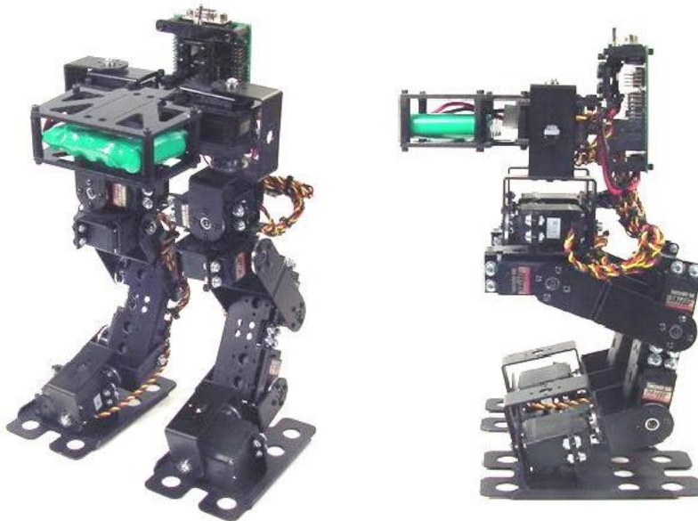
Figura 1.1. Vista isométrica y lateral del robot bípedo Scout [2]
