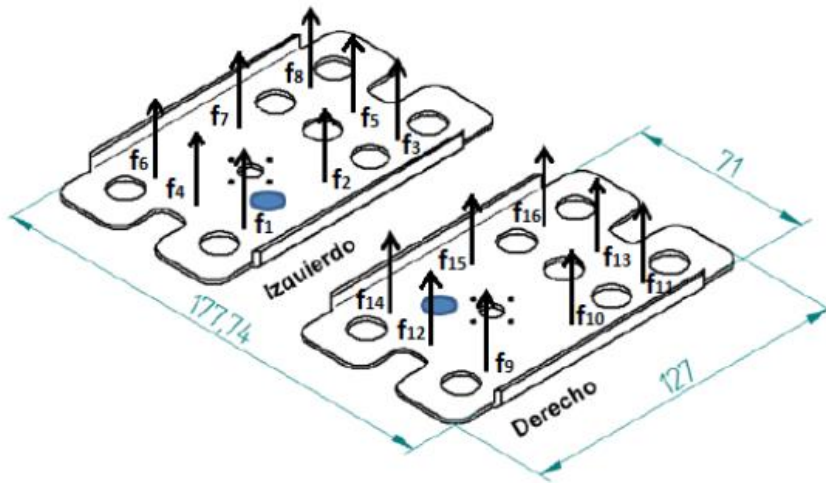
Figura 3.9. Representación de fuerzas de reacción en las plantas del pie del robot bípedo [4]
