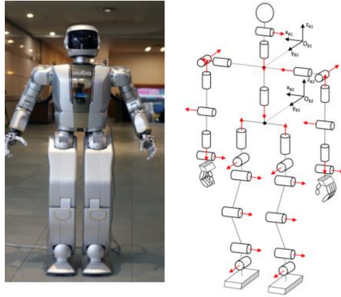
Figura 1.15. Fotografía y estructura de HUBO2 [31]
