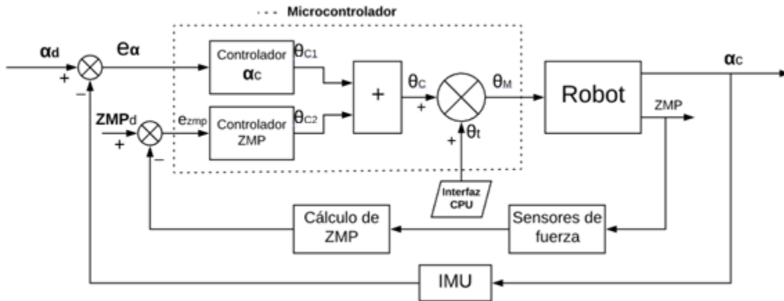
Figura 6.1. Diagrama de bloques de sistema de control de ZMP, pitch y roll
