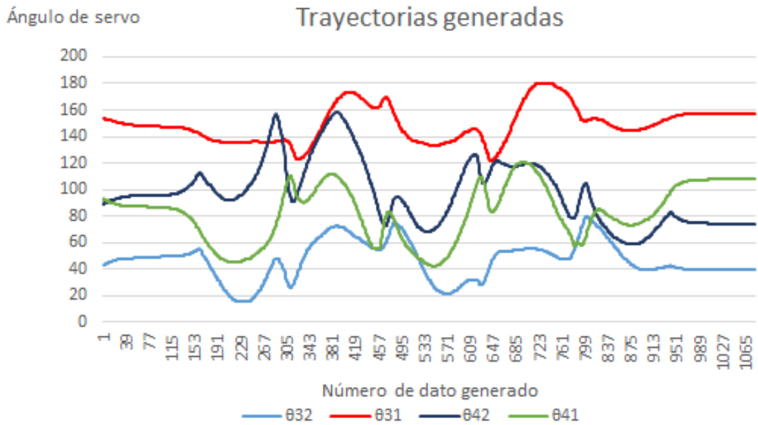
Figura 2.15. Trayectoria de ángulos de servomotores de las articulaciones 32, 31, 42 y 41
