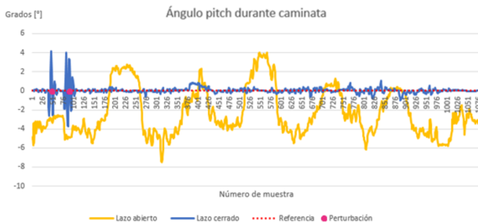
Figura 5.1. Ángulos pitch de la cadera durante la caminata sobre superficie horizontal
