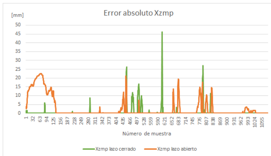
Figura 5.33. . Error absoluto en Xzmp durante caminata en superficie inclinada menos cinco grados en dirección roll
