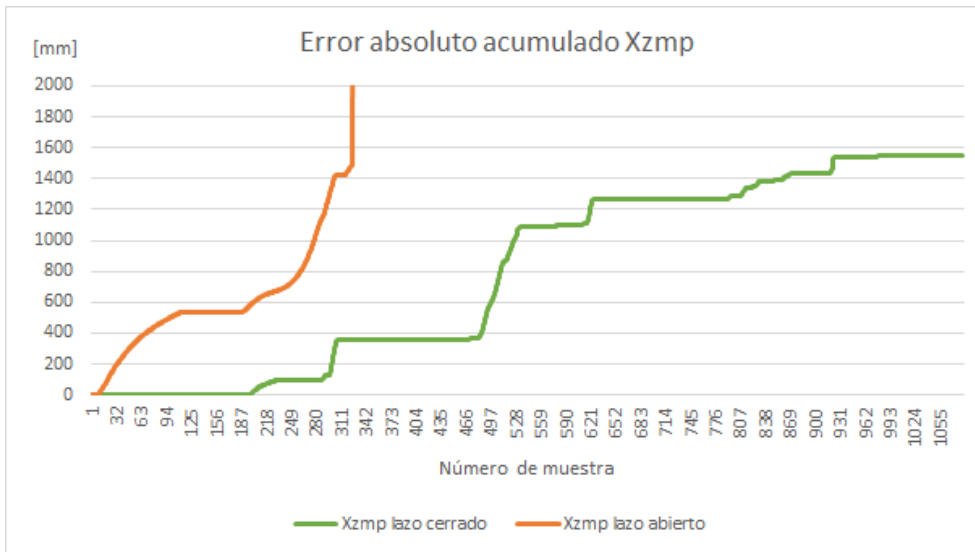
Figura 5.48. Error absoluto acumulado en Xzmp durante caminata con carga
