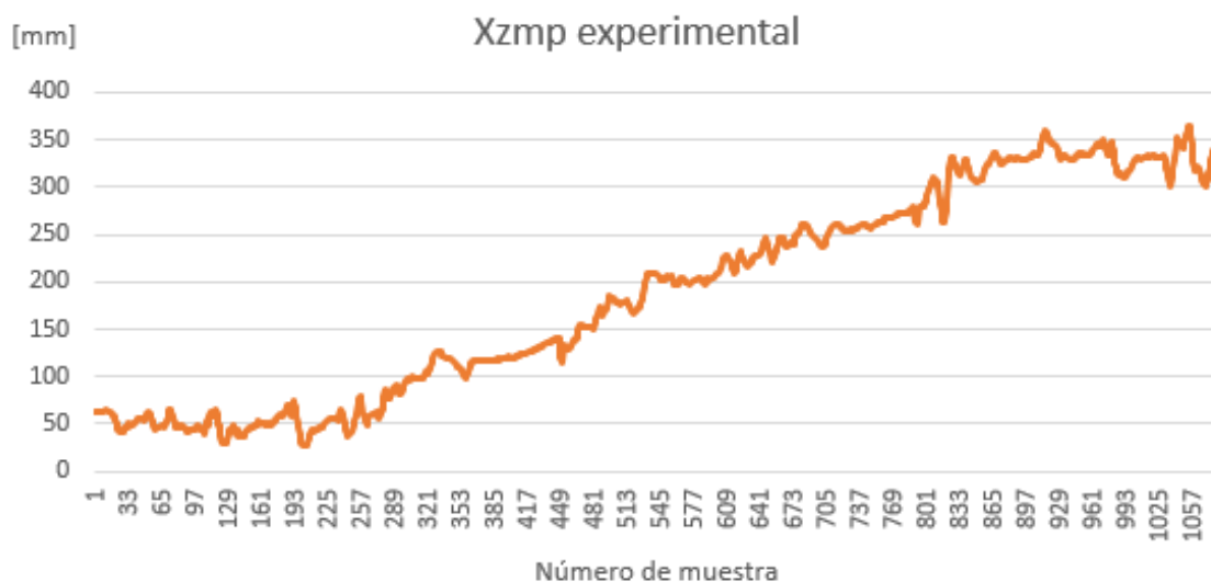
Figura 3.11. Coordenada X de ZMP experimental durante caminata
