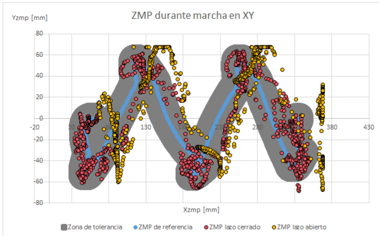
Figura 5.21. ZMP en XY durante caminata en superficie inclinada menos seis grados en dirección pitch
