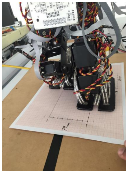
Figura 3.7. Medición experimental de longitud y ancho de paso
