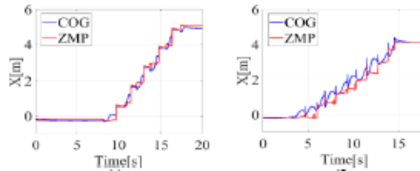
Figura 1.25. Aplicación de sistema de control de ZMP en un mecanismo de 4 GDL [40]
