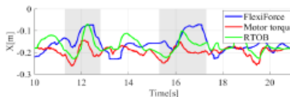
Figura 1.24. Resultado de obtención de ZMP por diferentes métodos [40]
