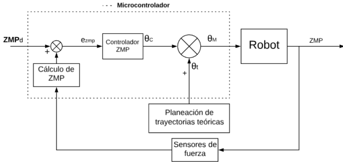
Figura 4.5. Diagrama de bloques del sistema de control del ZMP del robot bípedo
