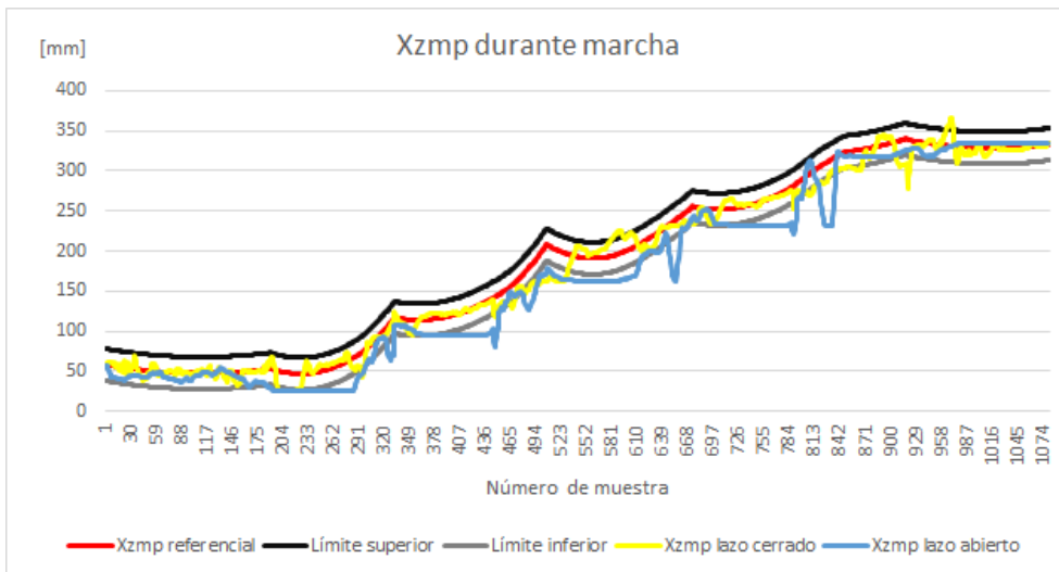
Figura 5.25. Coordenada X del ZMP durante caminata en superficie inclinada seis grados en dirección pitch
