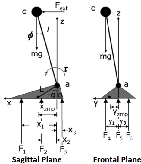
Figura 3.8. Análisis de cálculo de ZMP en planos sagital y frontal [4]
