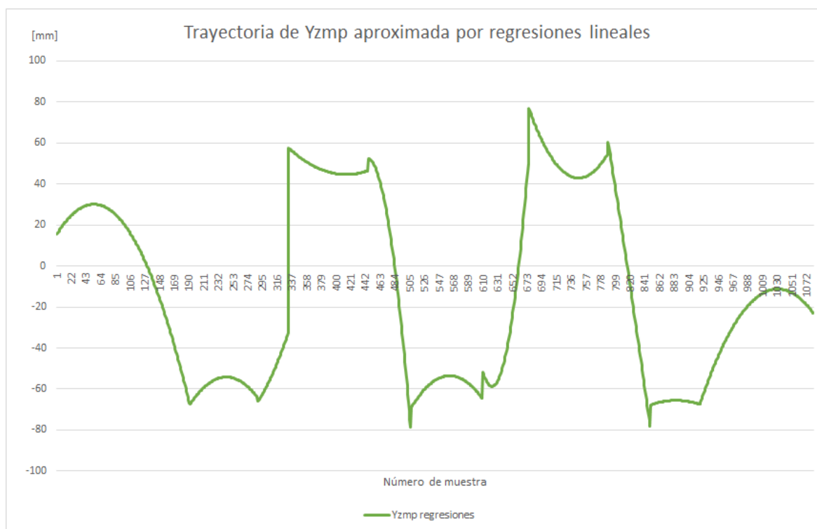
Figura 3.18. Yzmp aproximada por regresiones lineales durante la marcha
