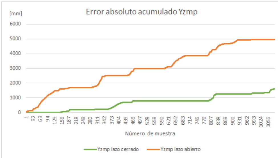
Figura 5.18. Error absoluto acumulado en Yzmp durante caminata en superficie horizontal
