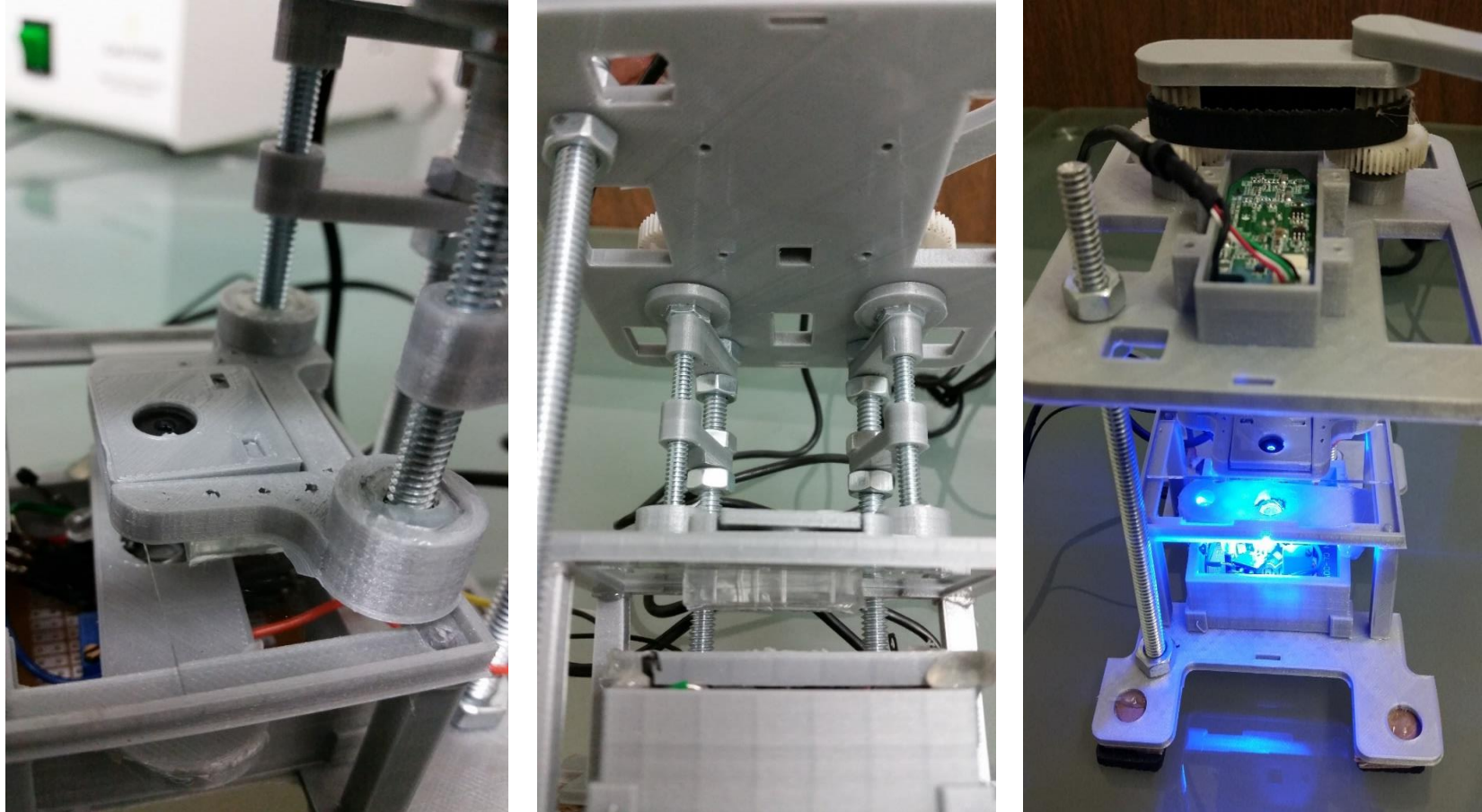
FIGURA 0-2. DE IZQUIERDA A DERECHA, LAS FOTOGRAFÍAS MUESTRAN PARTES IMPORTANTES DEL DISEÑO DEL PROTOTIPO : LA ETAPA ÓPTICA DONDE SE RESGUARDA LA LENTE, EL SISTEMA DE TRANSMISIÓN DE MOVIMIENTO QUE PERMITE EL AJUSTE DE LA DISTANCIA FOCAL Y EL ORIFICIO DONDE PARA LA LUZ AL SENSOR EN LA PARTE DE ARRIBA, Y UNA FOTOGRAFÍA CON PERSPECTIVA DONDE SE MUESTRAN LAS BASES, LA COLOCACIÓN DEL CHIP DE LA CÁMARA, LA PLATINA Y LA ILUMINACIÓN ENCENDIDA.
