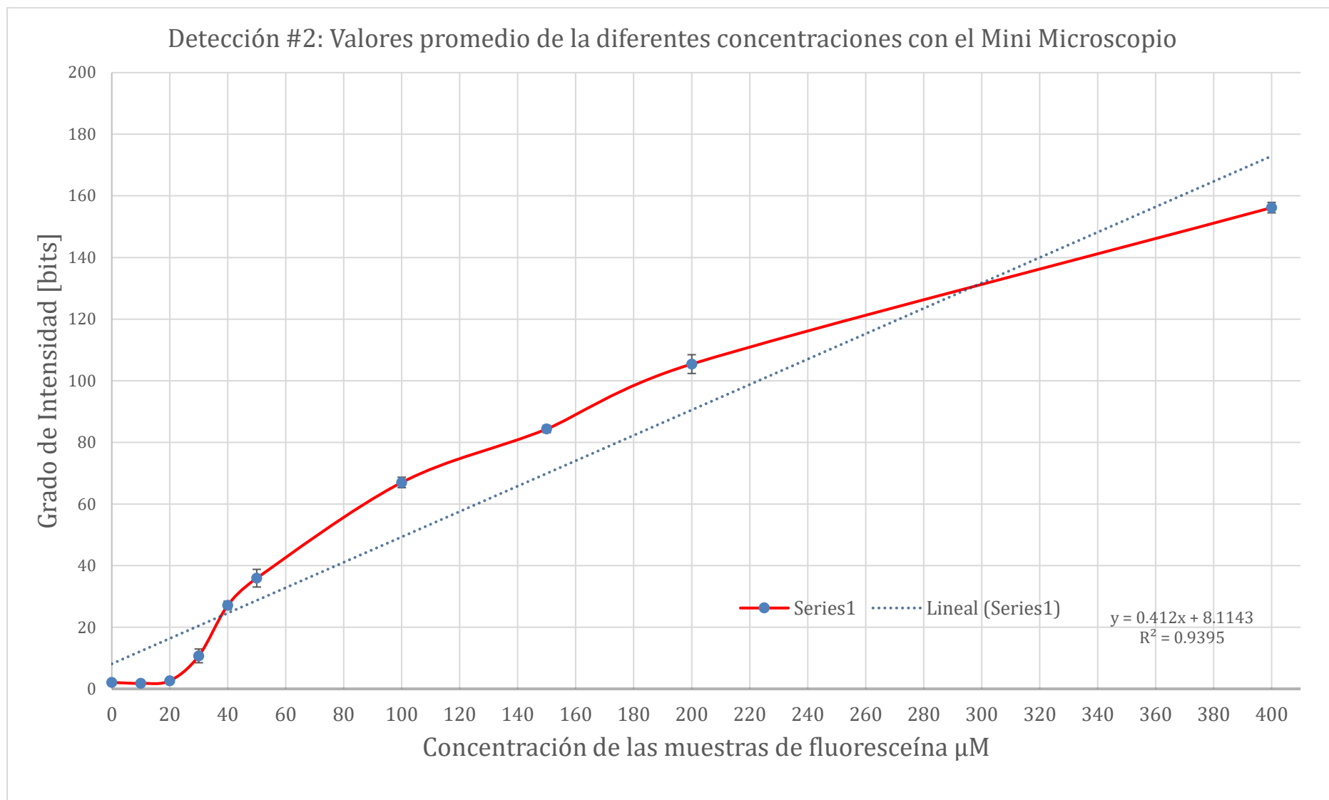
FIGURA 4-10. GRÁFICA QUE DEL COMPORTAMIENTO DE LOS VALORES PROMEDIO DE LAS IMÁGENES TOMADAS CON EL MINI MICROSCOPIO DE DETECCIÓN DE FLUORESCENCIA A PH 8.0.
