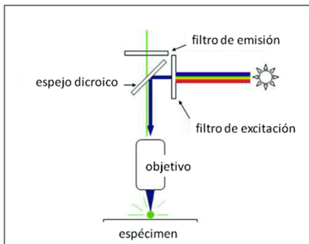
FIGURA 1-12. DIAGRAMA DEL EJEMPLO DEL MICROSCOPIO DE FLUORESCENCIA.
