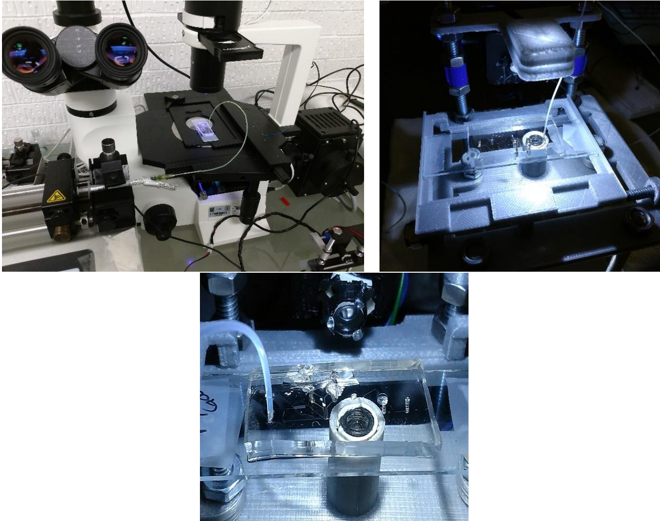
FIGURA 0-19. PARA REALIZAR LOS EXPERIMENTOS ES NECESARIO COLOCAR EL CHIP DE MICRO FLUÍDICA EN LA PLATINA DE LOS MICROSCOPIOS Y ÉSTAS IMÁGENES NOS MUESTRAN CÓMO ES QUE FUE LLEVADO A CABO EN AMBOS. ÉSTE CHIP ESTA EMBEBIDO EN UN PORTAOBJETOS CONVENCIONAL Y PARA AMBOS CASOS, EL CHIP TIENE INSERTADA YA LA MANGUERA DE INYECCIÓN DE FLUORESCÉINA.
