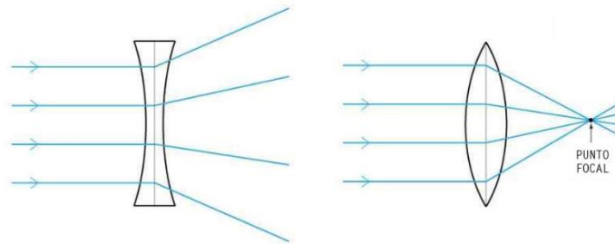
FIGURA 1-5. IMAGEN QUE MUESTRA EL COMPORTAMIENTO DE LAS LENTES NEGATIVAS (IZQUIERDA) Y POSITIVAS (DERECHA) CON LOS RAYOS DE LUZ INCIDENTES [6].
