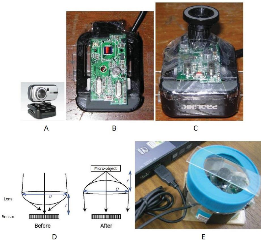
FIGURA 1-14. A) IMAGEN DE CÁMARA WEB, B) CÁMARA WEB REMOVIDA DE LA CARATULA FRONTAL, C) COLOCACIÓN DEL LENTE INVERTIDO D) DIAGRAMA EXPLICATIVO DE COMO AL INVERTIR EL LENTE DE LA CÁMARA WEB, LA FUNCIÓN SE INVIERTE, EN VEZ DE TOMAR UNA GRAN IMAGEN Y REDUCIRLA PARA EL SENSOR, TOMA UNA IMAGEN PEQUEÑA Y LA MAGNIFICA. E) PROTOTIPO FINAL DE MICROSCOPIO DE LENTE INVERTIDO [13].
