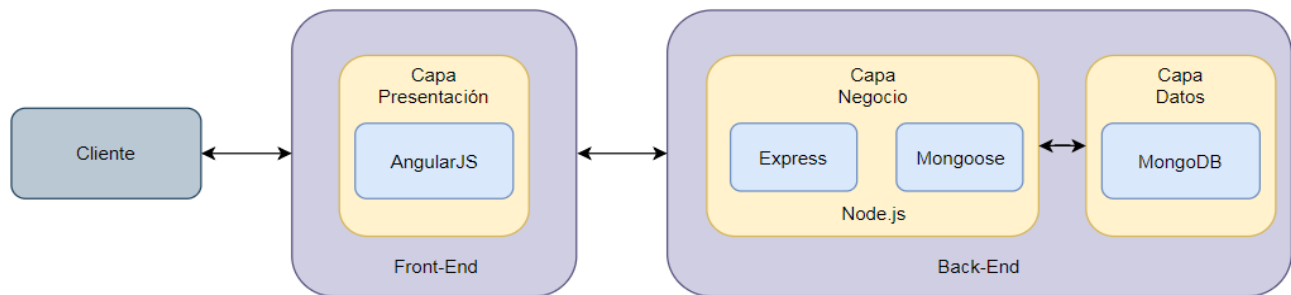
Figura 4.3 Diagrama de capas del sistema de punto de venta
