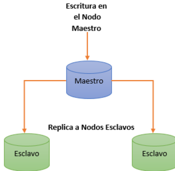
Figura 2.42 Replicación con escritura en el nodo maestro
