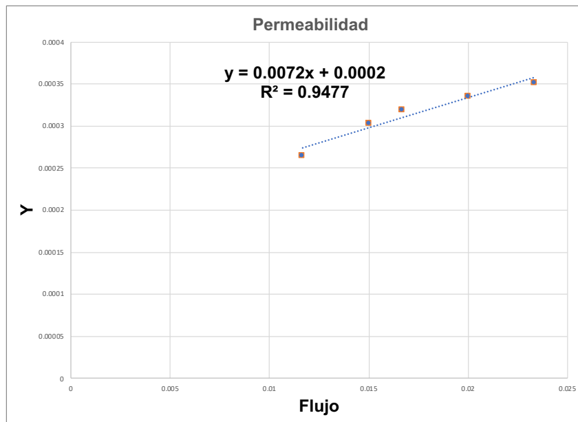
Gráfico 11.- Datos para el calculo de la permeabilidad “Surfactante (2)”.
