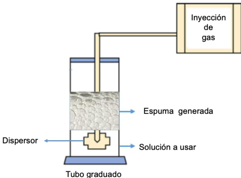
Figura 9.- Diagrama del experimento en tubo de ensayo.
