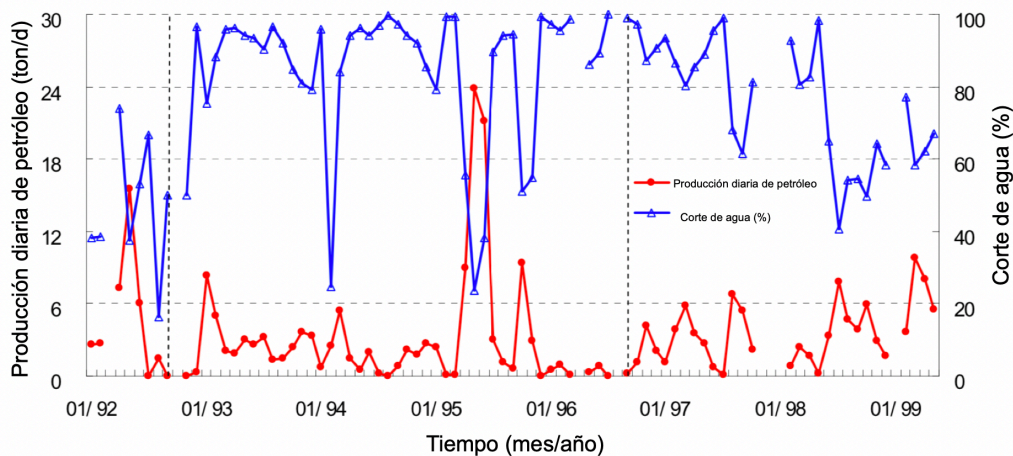
Figura 12.- Curva de producción del pozo 19-162. 21
