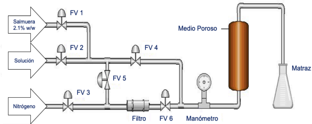
Figura 10.- Diagrama del experimento en medio poroso.
