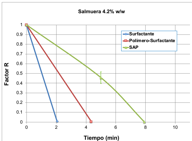
Gráfico 3.- Estabilidad de las espumas en salmuera sintética al 4.2% w/w.
