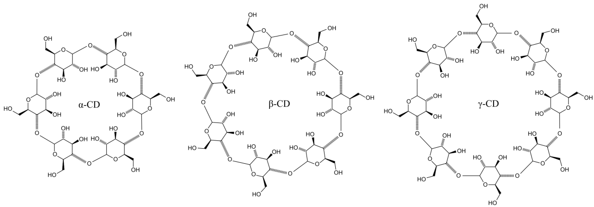
Figura 6.- Estructura de las ciclodextrinas; \alpha -CD, \beta -CD y \gamma -CD con 6, 7 y 8 subunidades de glucosa, respectivamente. 15
