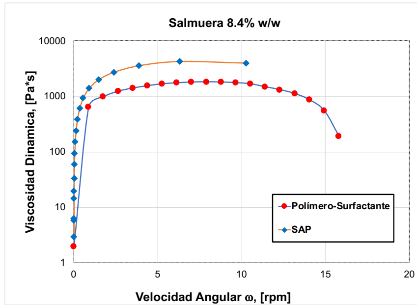
Gráfico 22.- Comportamiento de la viscosidad aparente de los sistemas SAP y Polímero-Surfactante en salmuera 8.4% w/w.
