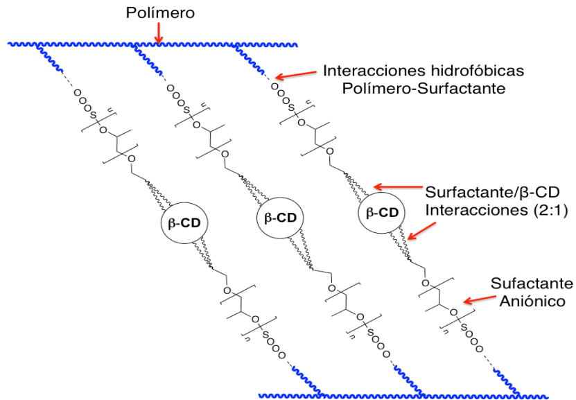
Figura 7.- Estructura propuesta de la red SAP, modificado de "Formulation of a self-assembling polymeric network system for enhanced oil recovery applications". 11
