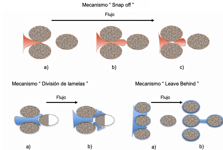
Figura 8.- Mecanismos de Formación de Espumas en Medios Porosos, modificado de "Efecto de la concentración del químico disperso en la formación de espumas en medios porosos". 8
