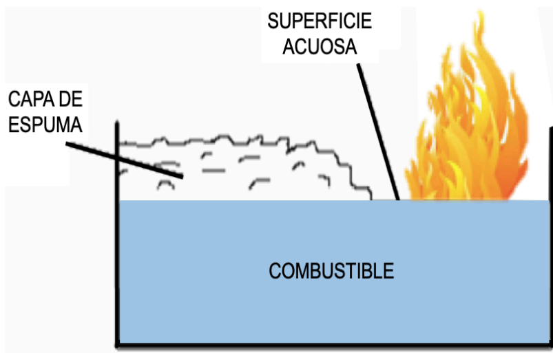
Figura 5.- Mecanismo de acción de la espuma en contraincendios. 14
