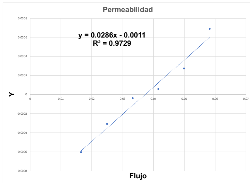
Gráfico 15.- Datos para el calculo de la permeabilidad “SAP (2)”.
