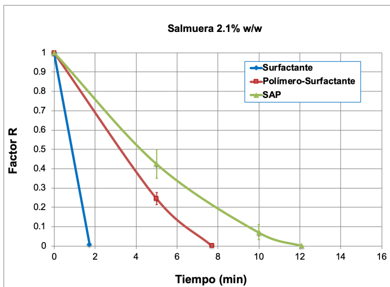
Gráfico 2.- Estabilidad de las espumas en salmuera sintética al 2.1% w/w.
