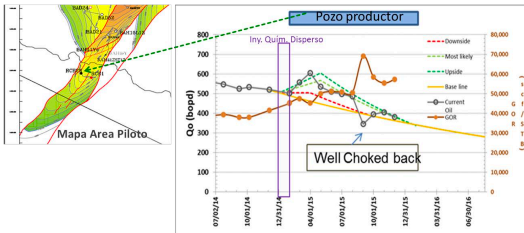
Figura 11.- Área piloto y comportamiento del pozo productor influenciado por la inyección de espuma. 8
