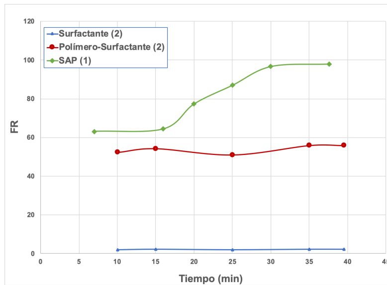
Gráfico 6.- Comportamiento del Factor de Resistencia grupo 1.
