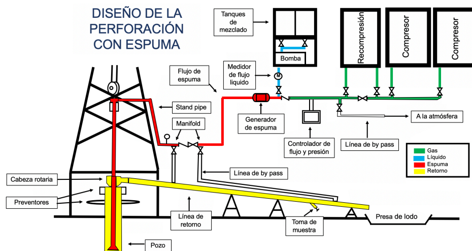
Figura 4.- Infraestructura superficial para la perforación con espuma. 12
