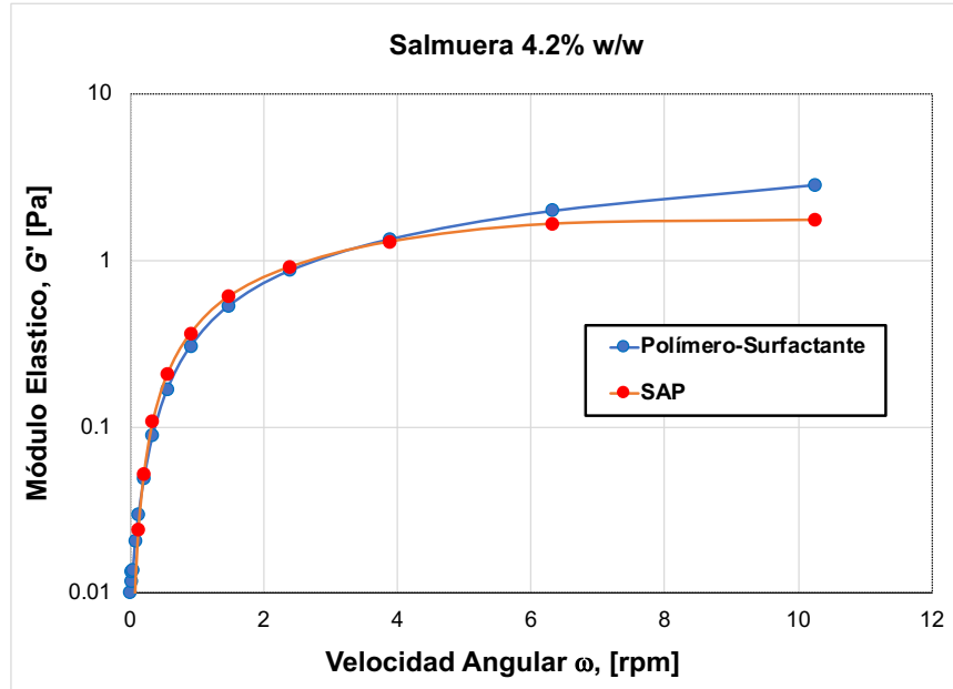
Gráfico 21.- Comportamiento del módulo elástico de los sistemas SAP y Polímero-Surfactante en salmuera 4.2% w/w.
