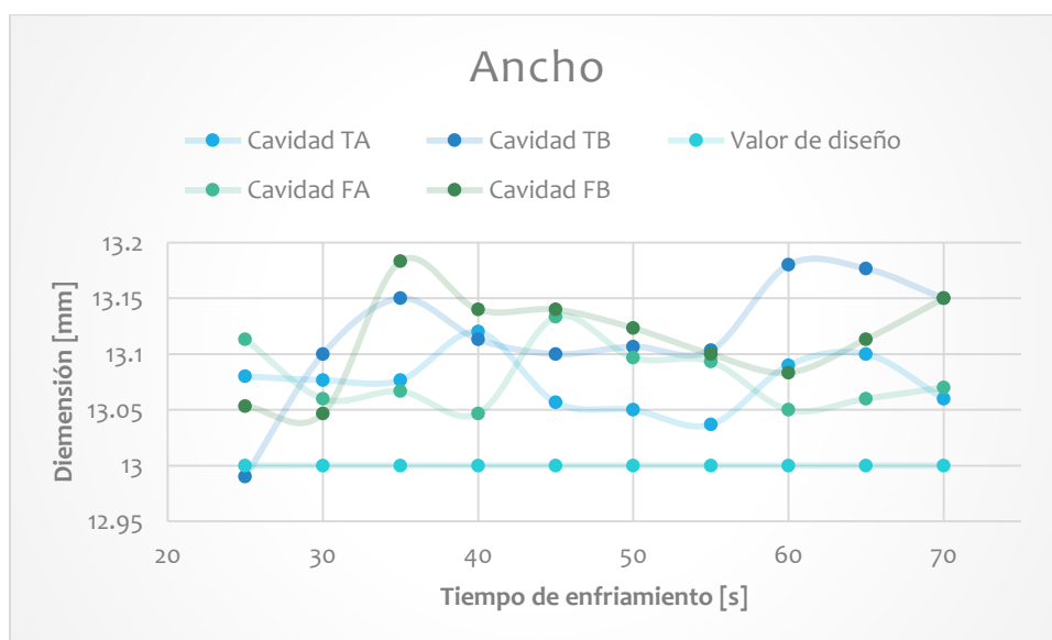
Gráfica 6. Tiempo de enfriamiento probetas de tracción
