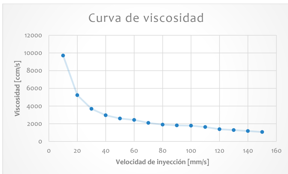
Gráfica 26. Curva de viscosidad molde 4.
