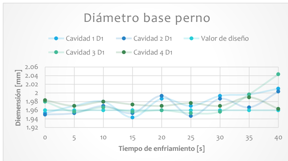
Gráfica 23. Tiempo de enfriamiento dimensión 1
