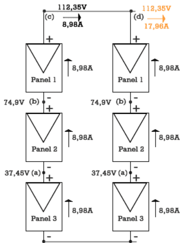
Ilustración 16 Conexión Mixta
