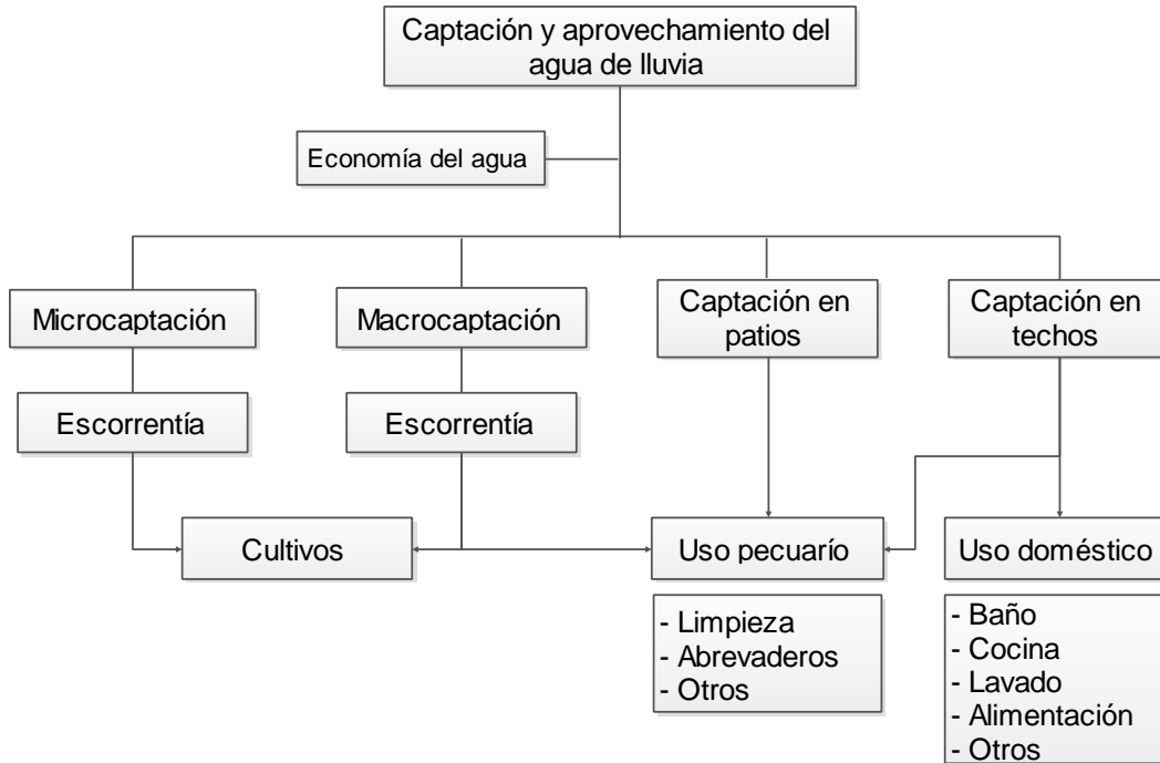
Figura 1.10. Técnicas de captación pluvial.
