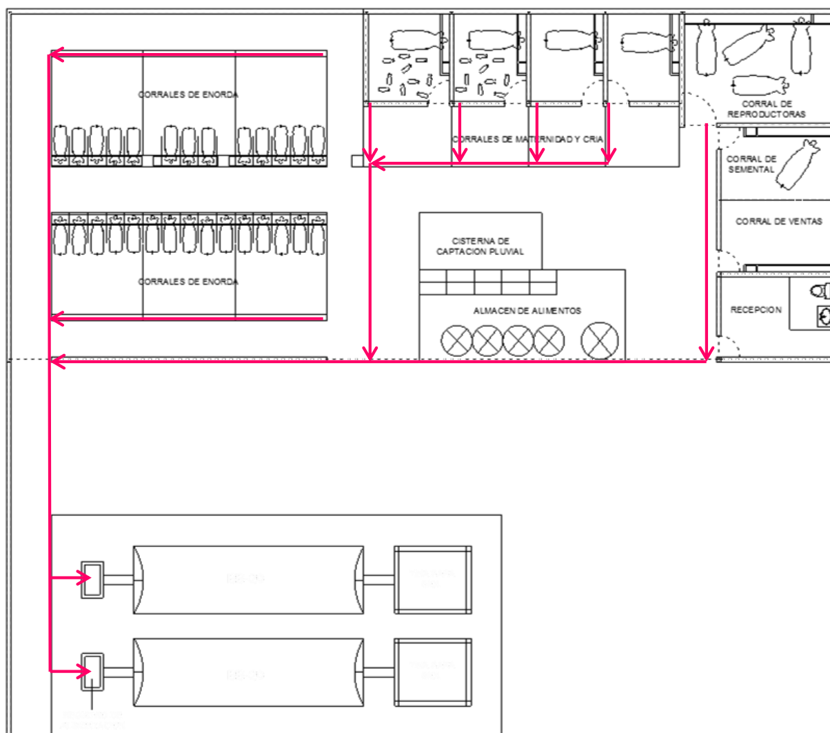
Figura 4.15. Ubicación del modelo BB-40 y sistema de captación de residuos.
