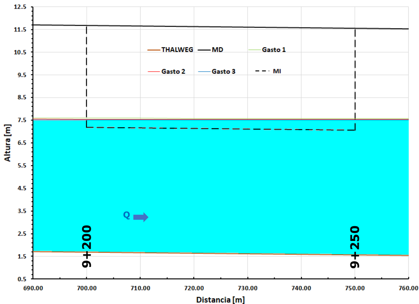
FIGURA 5.5 Perfiles hidráulicos, para los tres gastos, obtenidos con el método numérico de Runge-Kutta.
