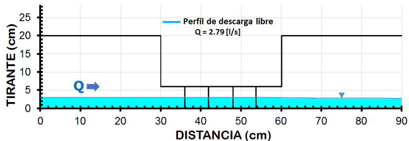
FIGURA 3.15 Gráfica del perfil de descarga libre.
