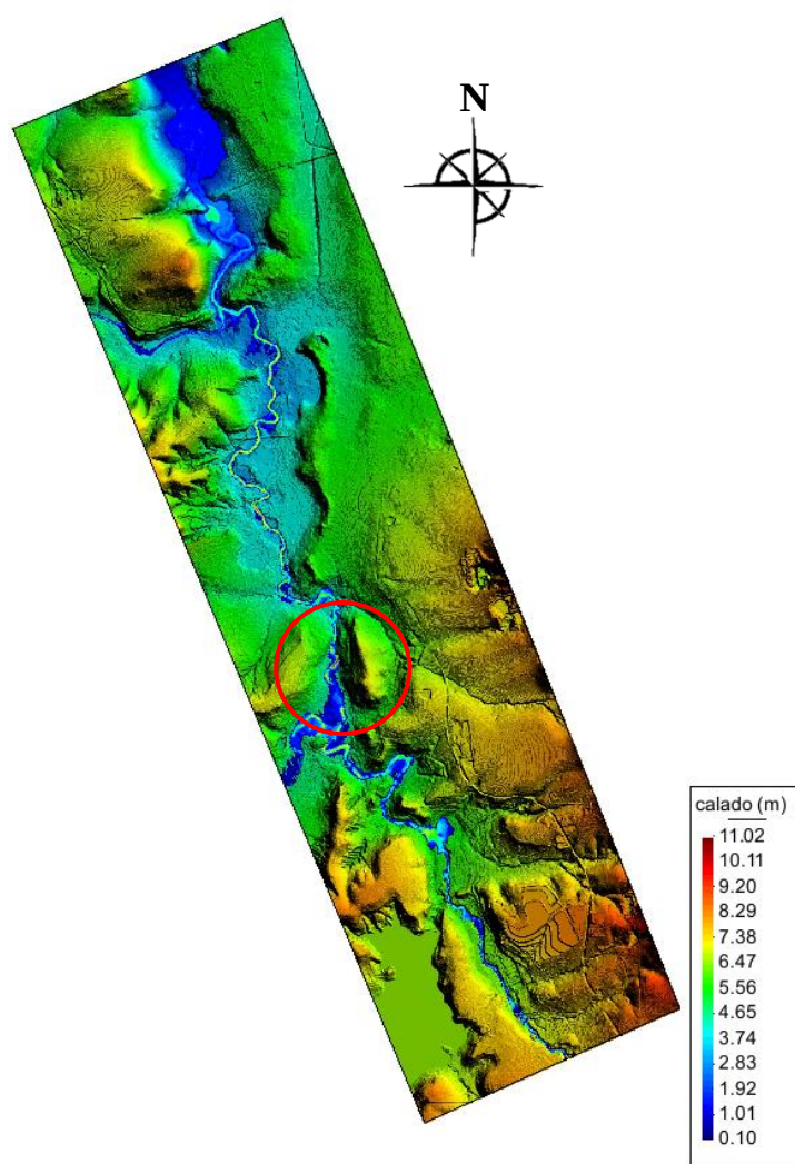
FIGURA 5.3 Resultado de una simulación matemática en 2D del río Tula para un gasto de 450 \text{ m}^3/\text{s} realizada con el paquete Iber®.
