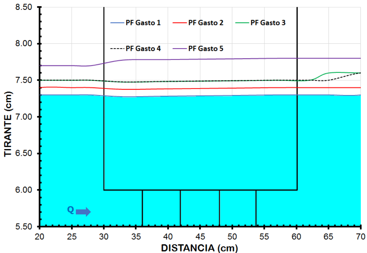
FIGURA 4.2 Perfiles hidráulicos calculados con el método numérico de Runge-Kutta.
