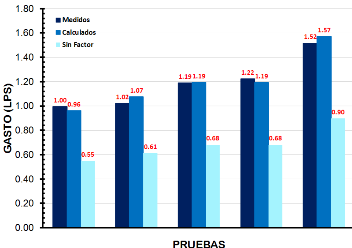
FIGURA 4.3 Comparativa de caudales de desbordamiento medidos contra calculados.
