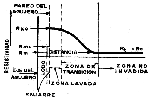
DISTRIBUCION RADIAL DE RESISTIVIDADES ( R_{mf} \gg R_w , ESTRATO CON AGUA)
