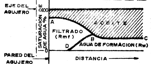
DISTRIBUCION RADIAL DE FLUIDOS EN LA VECINDAD DEL AGUJERO, ESTRATO CON ACEITE (CUALITATIVO)
