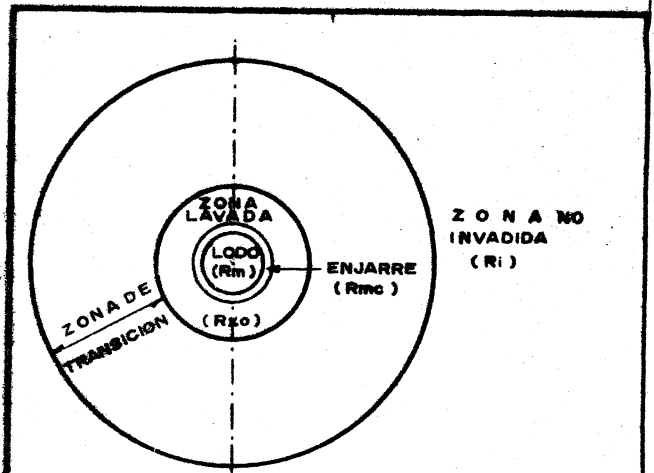
SECCION HORIZONTAL A TRAVES DE UN ESTRATO PERMEABLE CON AGUA.
