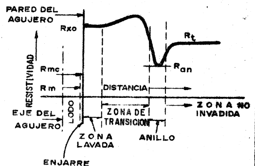
DISTRIBUCION RADIAL DE RESISTIVIDADES ( R_{mf} \gg R_w , ESTRATO CON ACEITE, S_w \ll 50\% )
