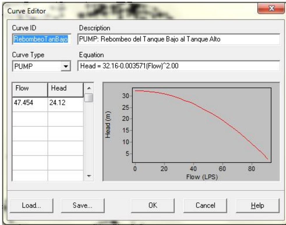
Figura 2.1 Curva del rebombeo del tanque bajo al tanque alto
