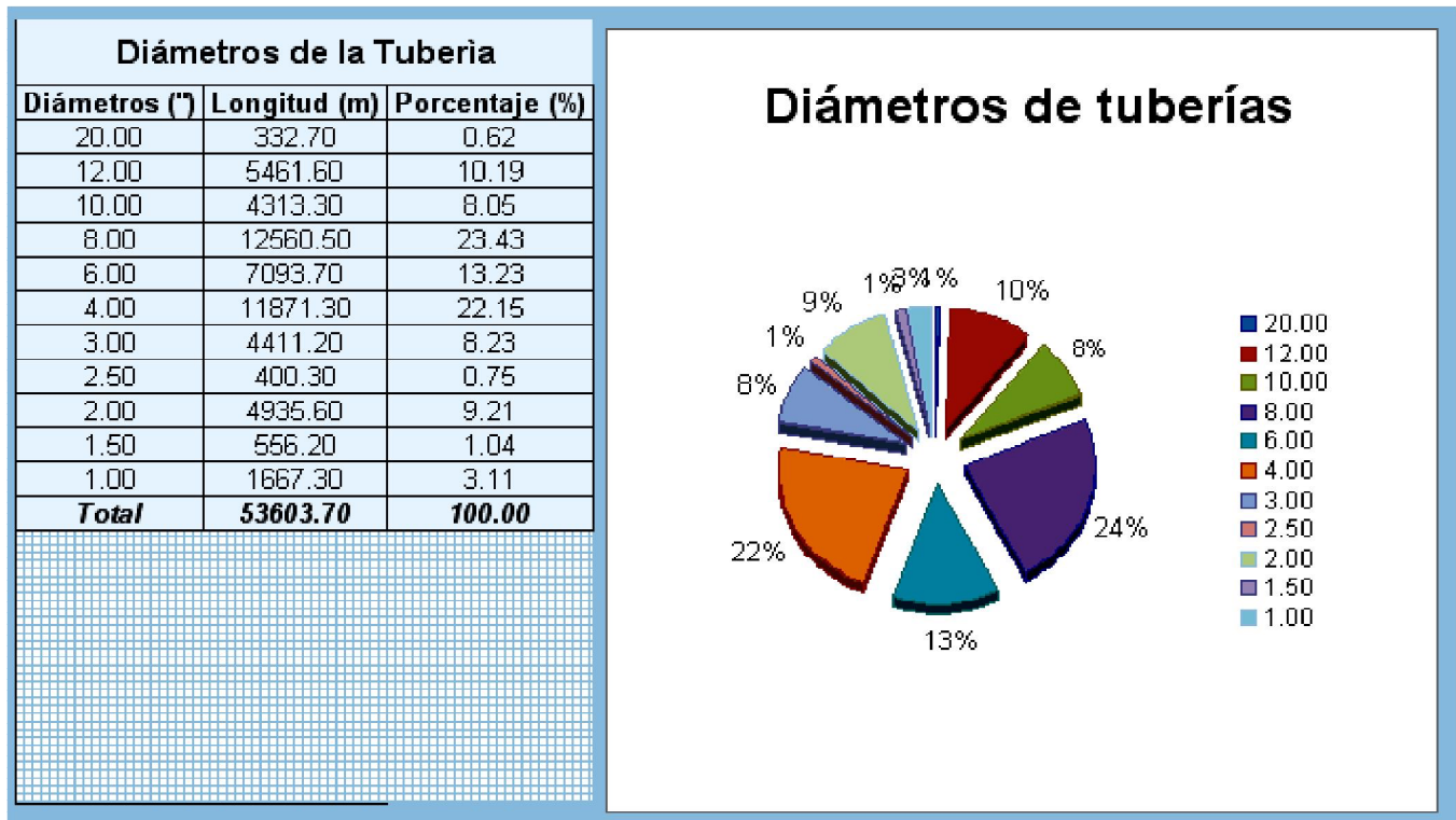
Figura 1.10 Porcentaje de los diámetros que comprende la red de distribución (Cortesía PUMAGUA)
