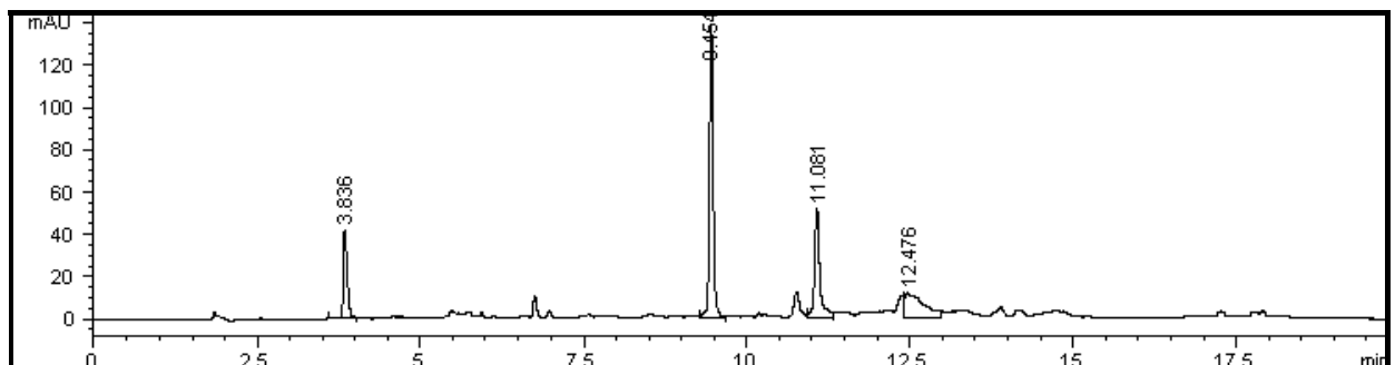
Fig. C.4i Cromatograma de microcistina.
