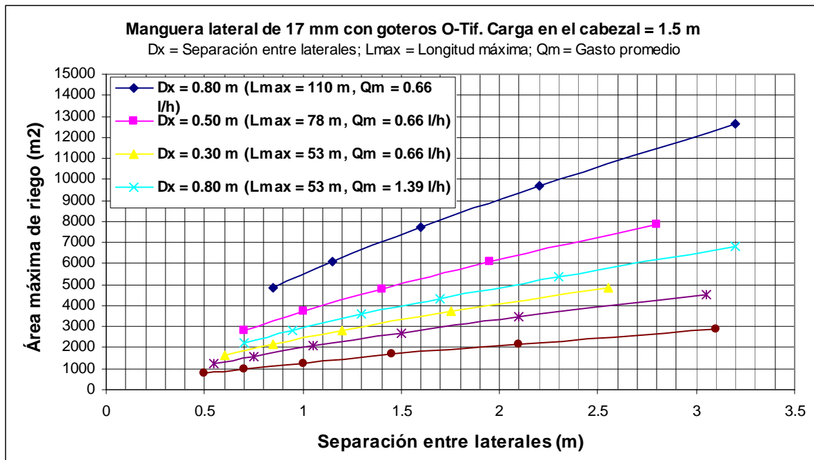
Figura 15. Áreas máximas de riego
