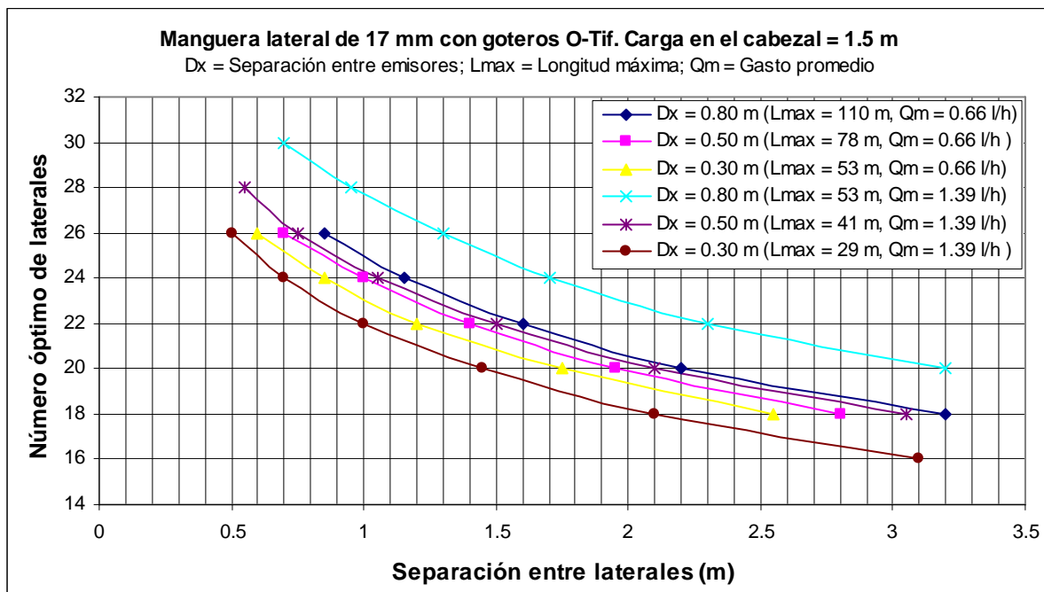
Figura 14. Gráfica para el diseño de los laterales
