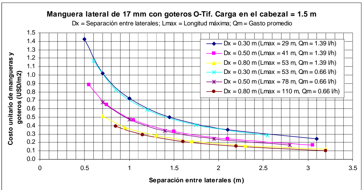
Figura 13. Costo unitario con manguera de 17mm de diámetro exterior
