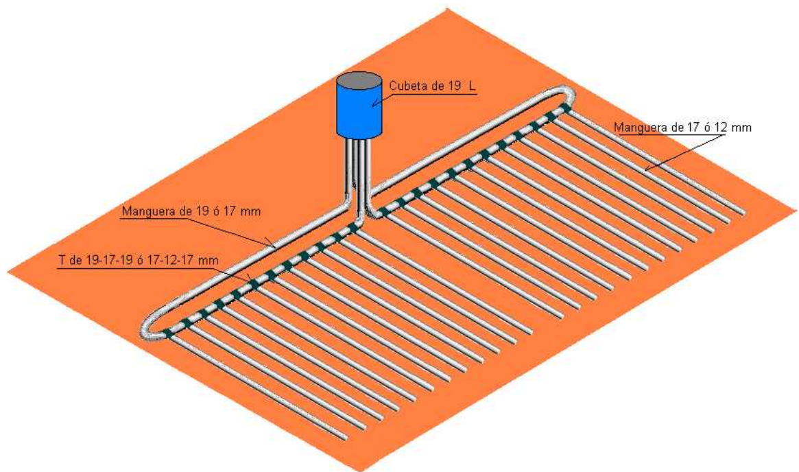
Figura 8. Tendido de las mangueras para la segunda etapa
