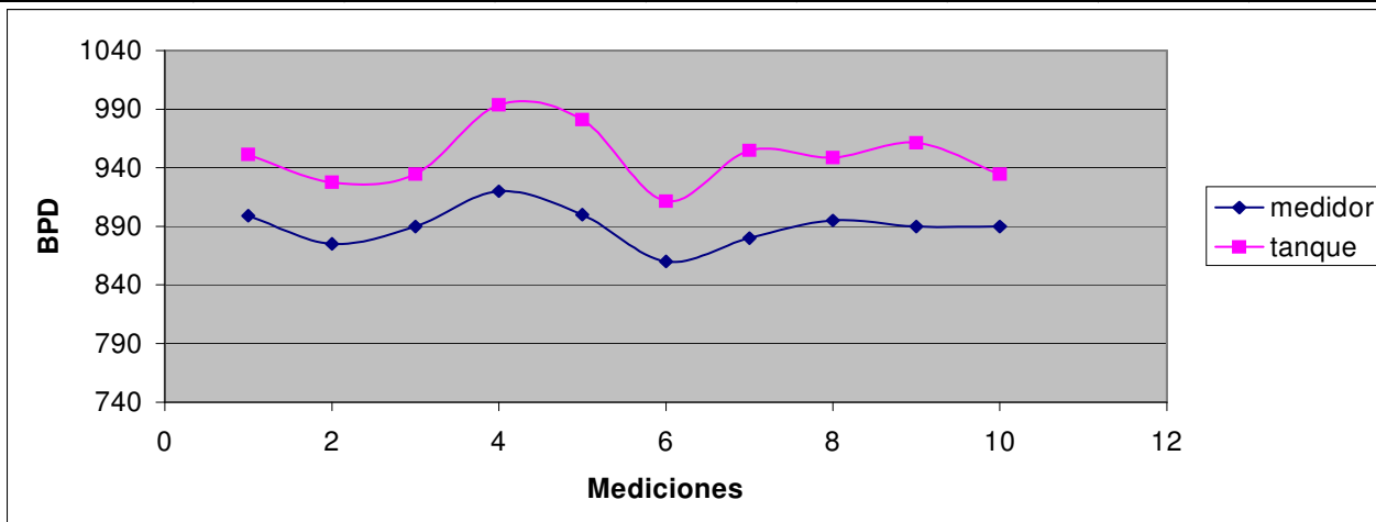
Figura C.12.-Medición de líquidos con medidor electrónico y en tanque de almacenamiento, Samaria No. 101
