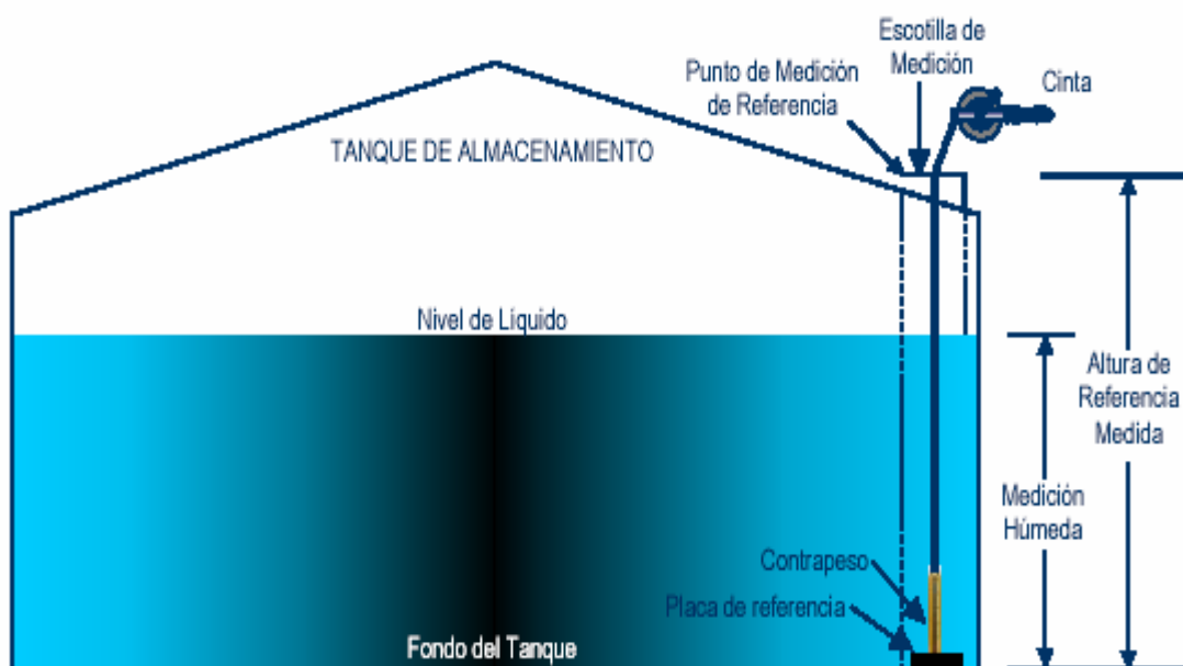
Figura. II.6.- Medición húmeda 7
