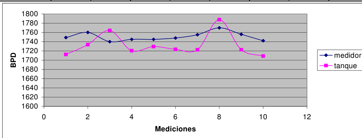
Figura C.11.- Medición de líquidos con medidor electrónico y en tanque de almacenamiento, Samaria No. 99
