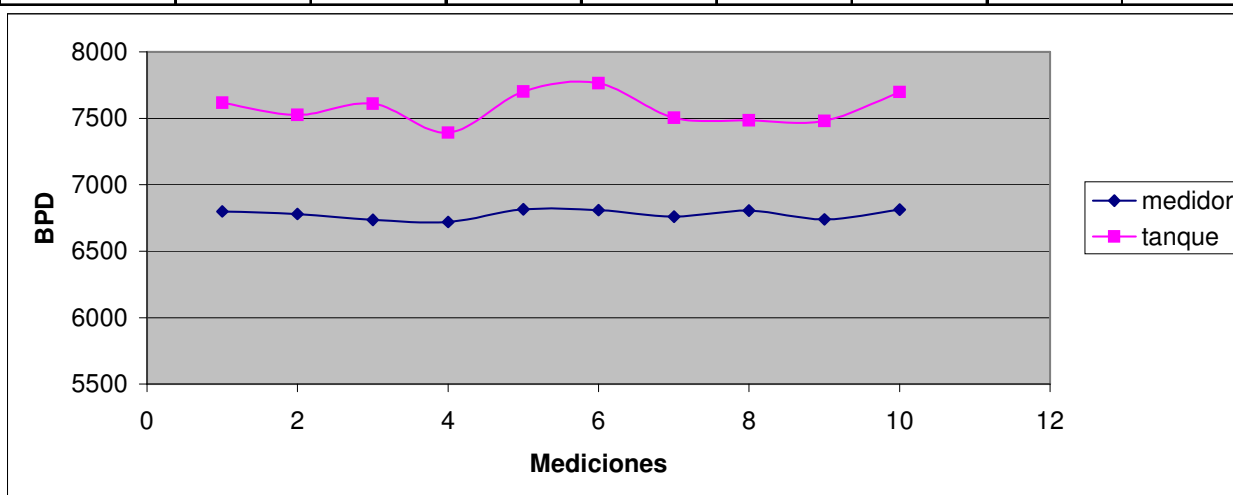
Figura C.5.-Medición de líquidos con medidor electrónico y en tanque de almacenamiento, Samaria No. 85
