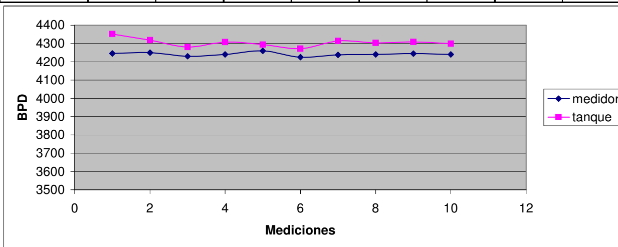
Figura C.6.-Medición de líquidos con medidor electrónico y en tanque de almacenamiento, Samaria No. 87
