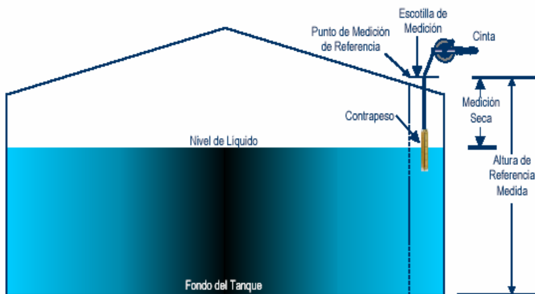
Figura. II.7.- Medición seca 7
