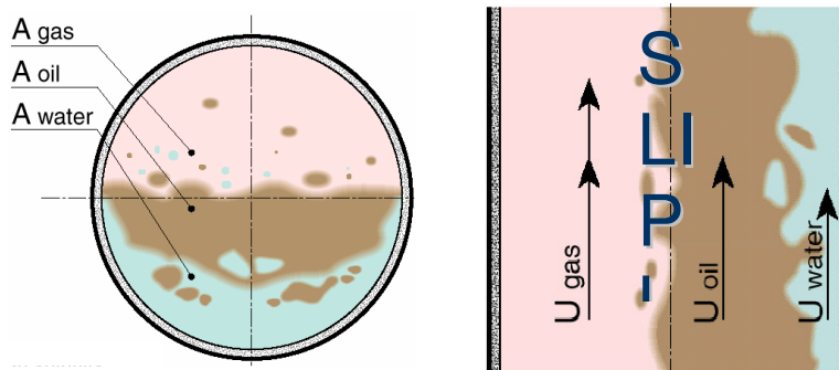
Figura IV.5.- Distribución de fases de flujo
