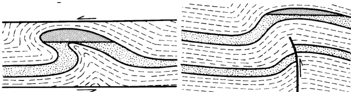
Figura 1.6. Tipos de Pliegues.
