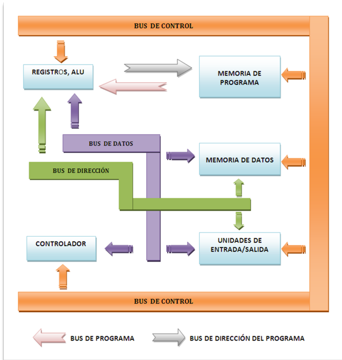
Figura 3. Arquitectura Harvard
