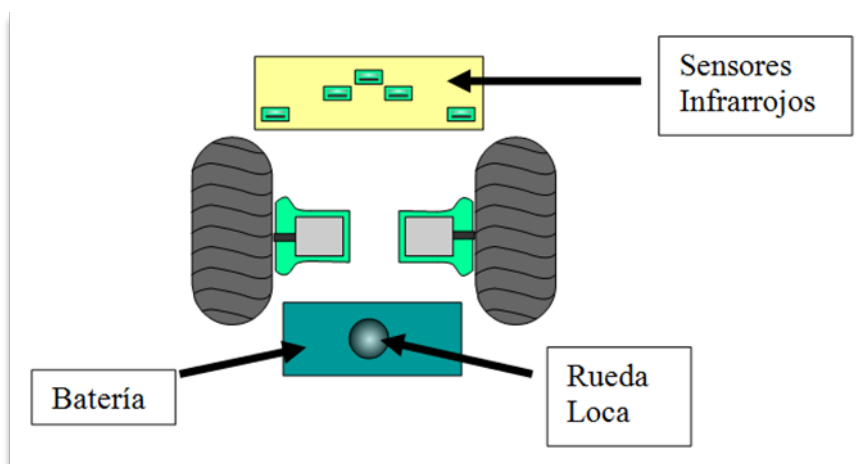
Figura 21. Sección inferior del robot vista desde abajo
