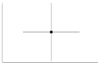
Figura 24. Cursor crosshair
