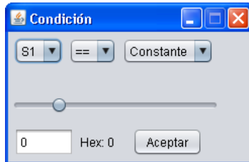
Figura 48. Bloque condicional
