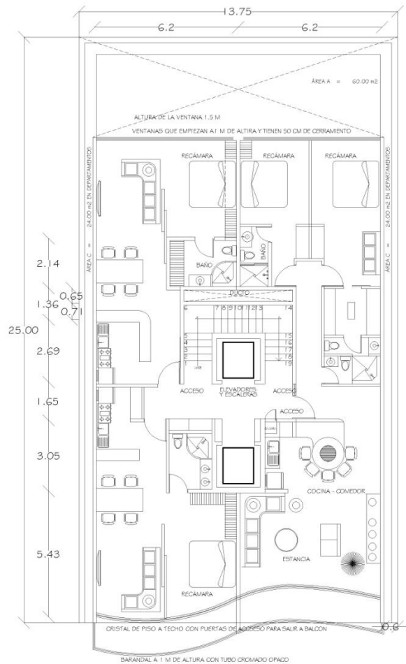
PLANTA TIPO SUITES OPCIÓN SUITE DE 100 M2 CON 2 RECAMARAS NIVEL 5 (+13.40m) NORTE
