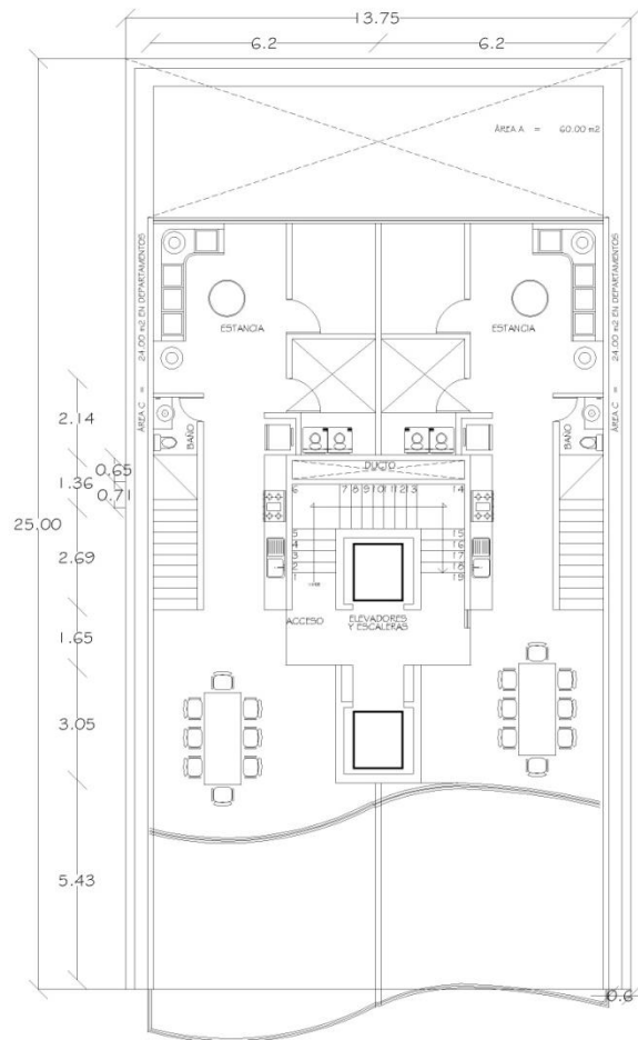
PLANTA BAJA PENTHOUSE NIVEL 19 (+57.50m) NORTE
