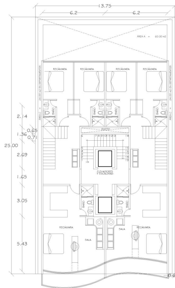
PLANTA ALTA PENTHOUSE NIVEL 20 (+60.65m) NORTE
