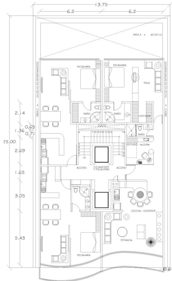
PLANTA TIPO SUITES OPCIÓN SUITE DE 100 M2 CON UNA RECAMARA NIVEL 5 (+13.40m) NORTE 0 1m 2m 3m 4m 5m 10m ESCALA GRÁFICA (metros)
