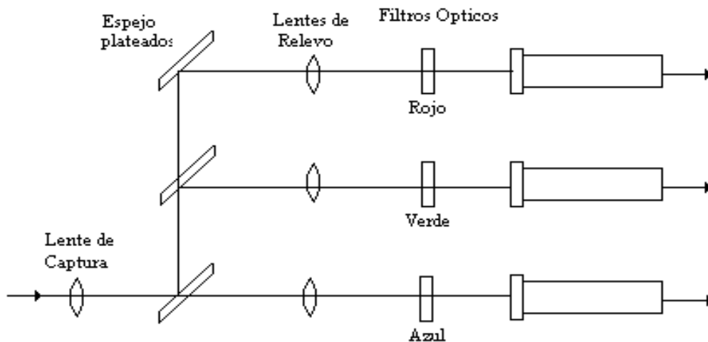
Figura 7. Componentes básicos de una cámara de color
