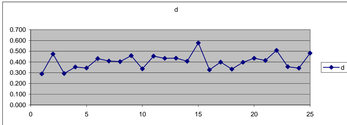
Fig. 16. Dependencia de los parámetros de elipses de dispersión de umbrales diferenciales en el Diagrama de Colores Básicos de Color XYZ CIE-1931[5].
