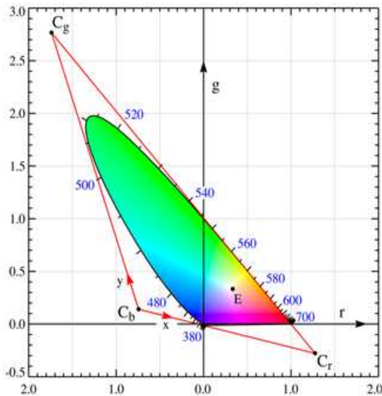
Figura 15. Espacio de color CIE 1931
