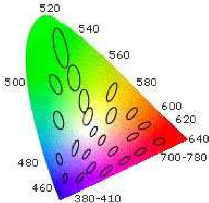
Figura 14. Espacio de color XYZ de la CIE
