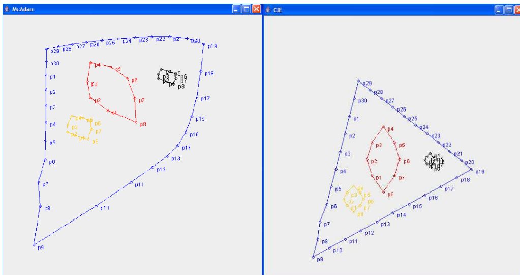
Figura 32. Las 3 Elipse contenidas en el espacio CIE 1931 a la izquierda en el espacio de McAdam y a la derecha en el espacio CIE XYZ (1931)
