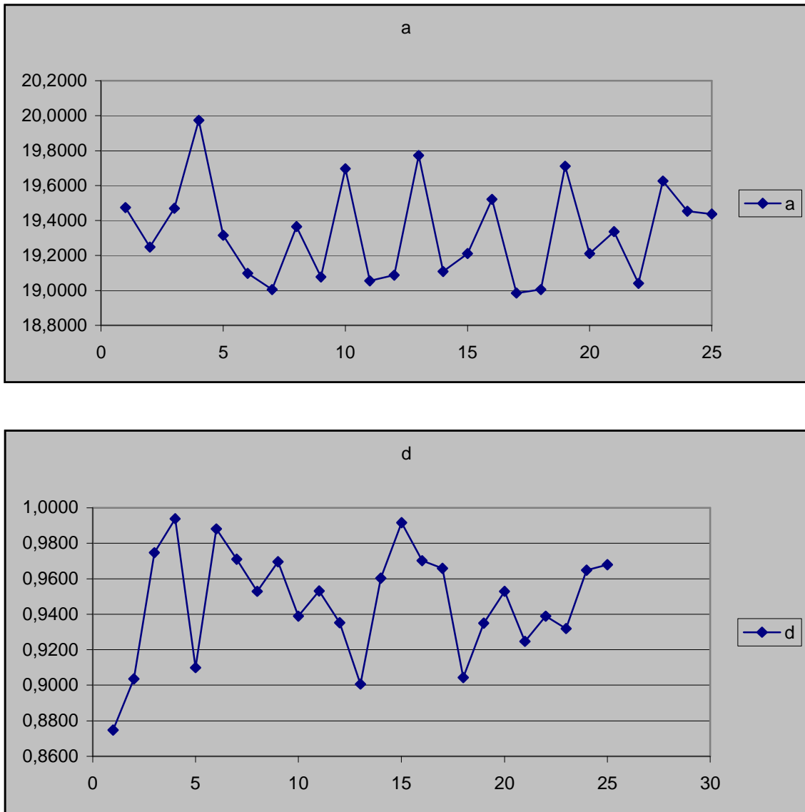
Fig. 23. Dependencia de los parámetros de las elipses de dispersión de umbrales diferenciales de saturación de color en el diagrama Curvilíneo de Color \xi, \eta, Mc Adam[6]
