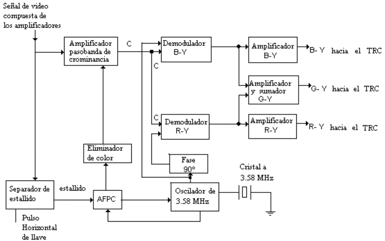
Figura 13. Sintonización de señal a color
