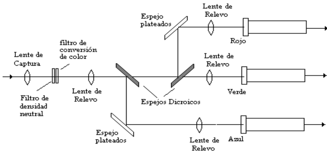
Figura 8. Arreglo de espejos dicróicos
