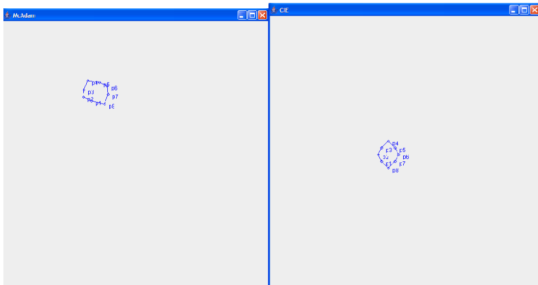
Figura 30. Elipse 2 en el espacio CIE 1931 a la izquierda y a la derecha ya transformada al espacio de McAdam
