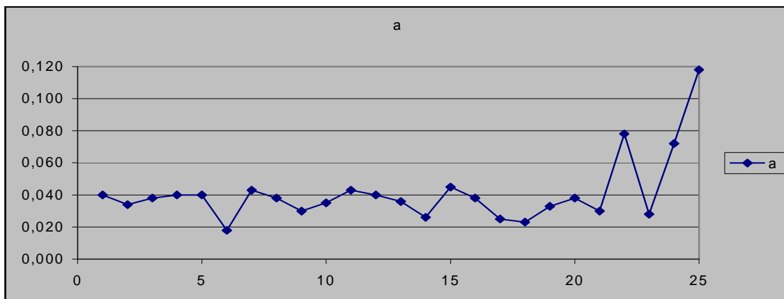
Fig. 16. Dependencia de los parámetros de elipses de dispersión de umbrales diferenciales en el Diagrama de Colores Básicos de Color XYZ CIE-1931[5].
