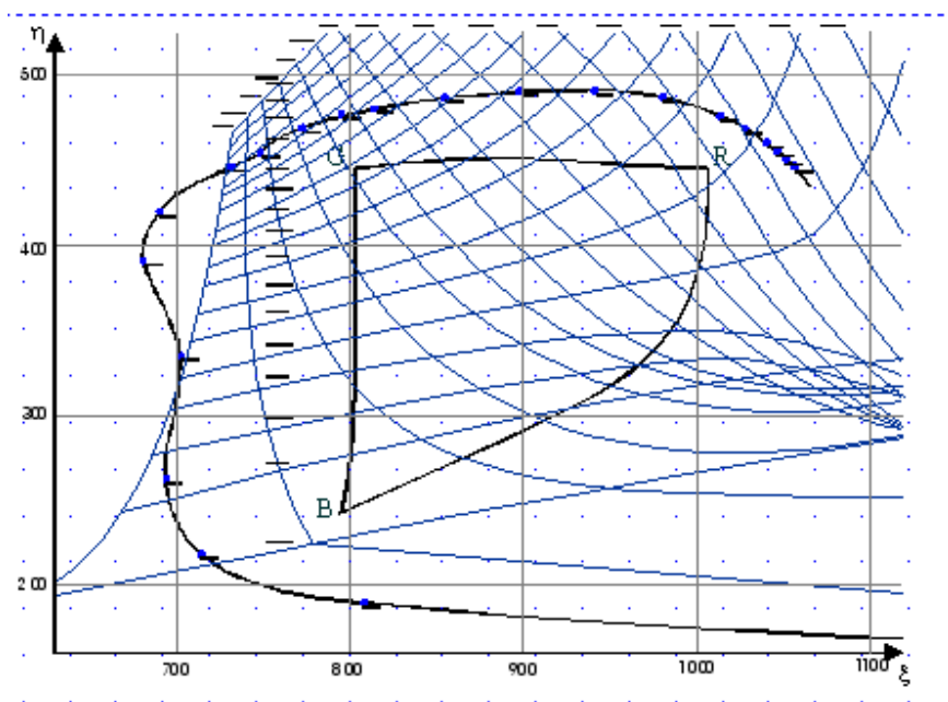
Figura 28. Espacio de Color Curvilíneo McAdam
