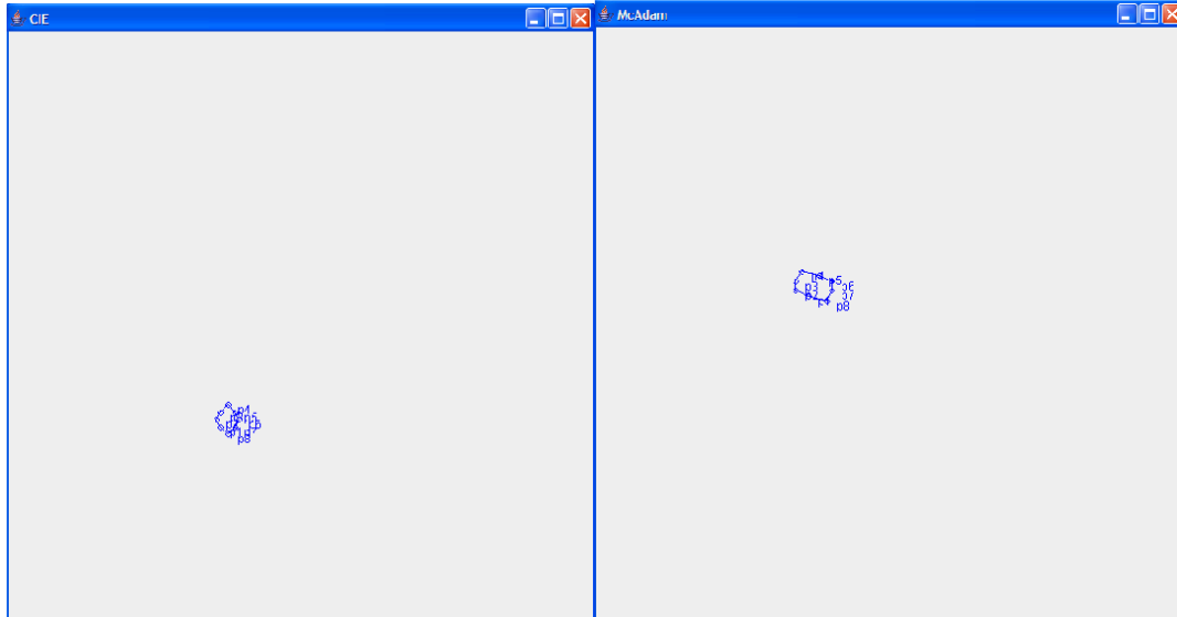
Figura 31. Elipse 3 en el espacio CIE 1931 a la izquierda y a la derecha ya transformada al espacio de McAdam
