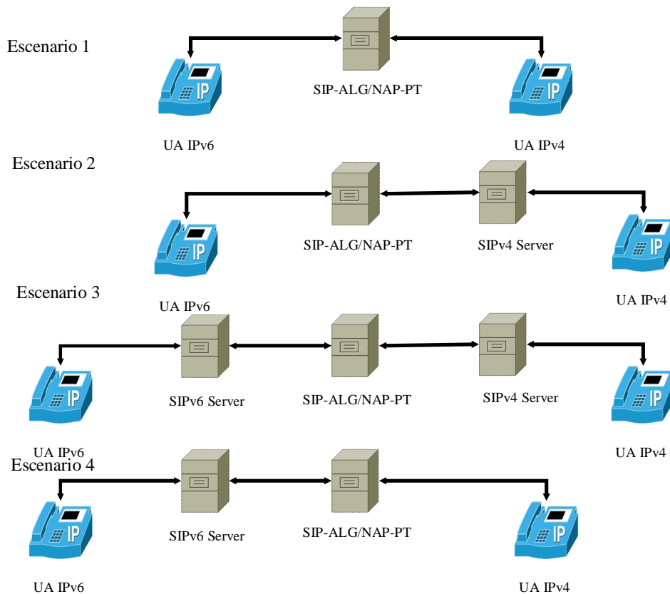
Fig 7.8 Escenario de desarrollo para SIPv6
