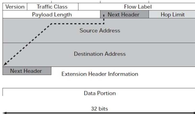
Figura 4.8 Encabezado IPv6.
