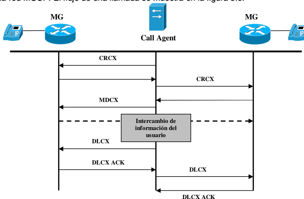
Figura 3.9 Conexiones y llamadas MGCP
