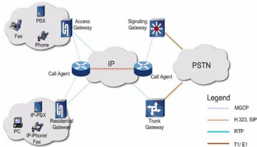
Figura 3.8 Arquitectura MGCP
