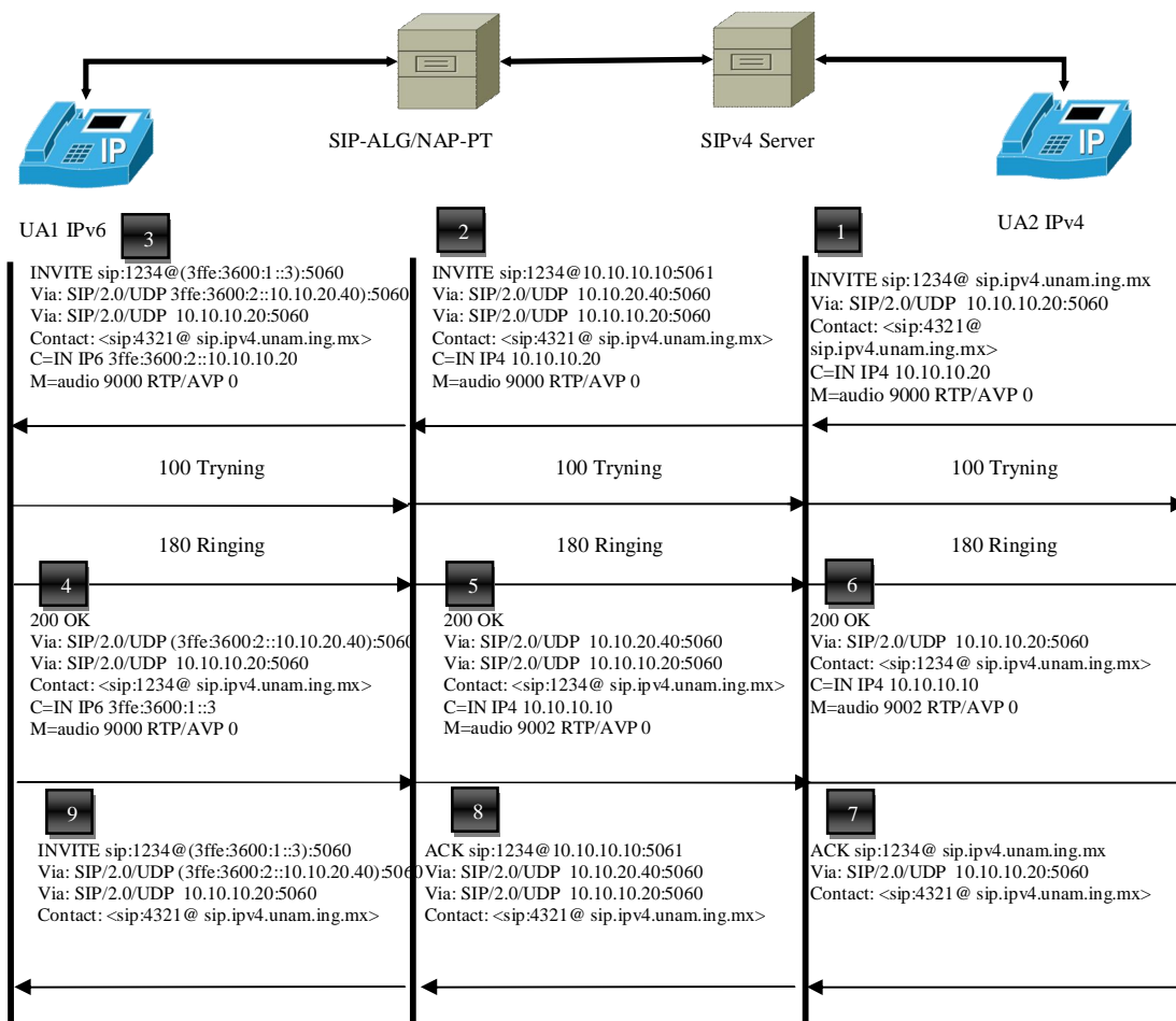
Figura 7.9 Flujo de una llamada SIPv6
