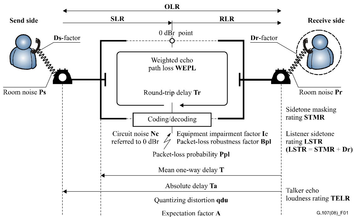
Figura 2.12 Factor de determinación de índice de calidad.
