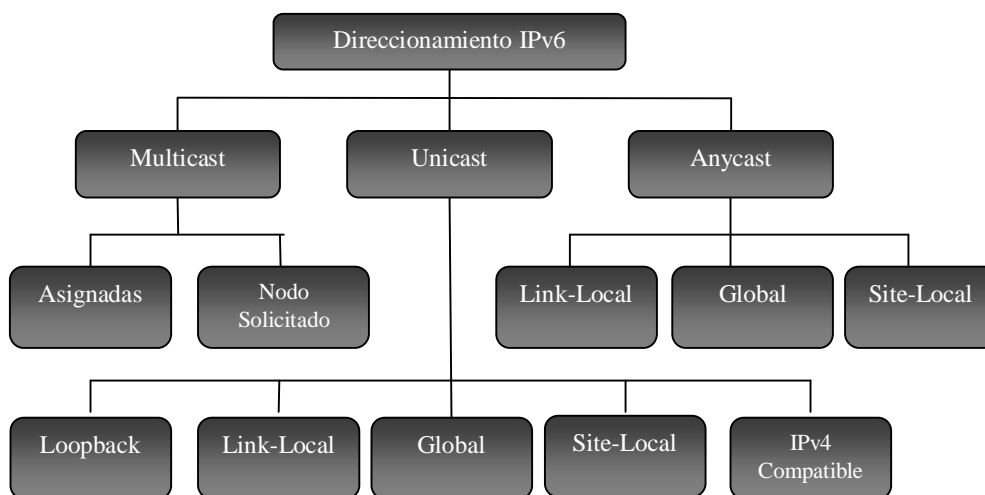
Figura 5.3 Direcciones IPv6
