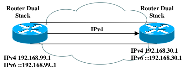
Figura 6.14 Túnel automático con direcciones Ipv4 compatibles
