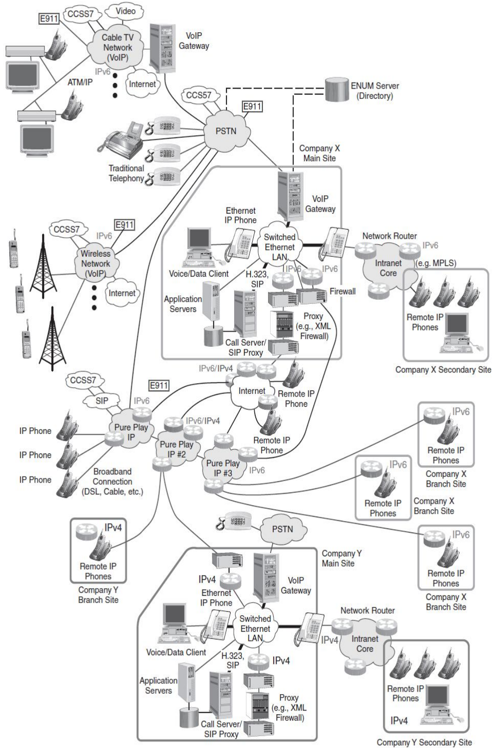
Figura 7.2 Arquitectura VoIPv6
