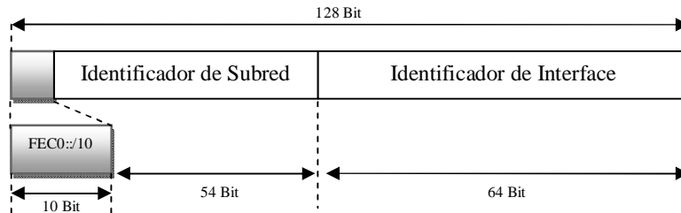
Figura 5.5 Dirección Site-Local.
