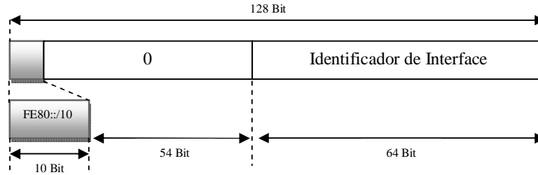
Figura 5.4 Dirección Link-Local
