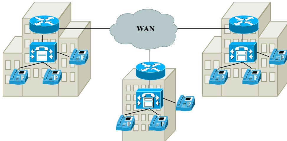
Figura 3.18 Esquema Distribuido.
