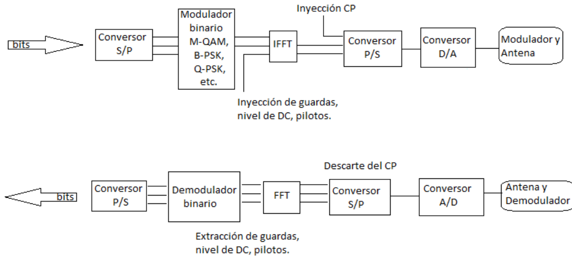
Figura 9 Diagrama a bloques del modulador OFDM [4]
