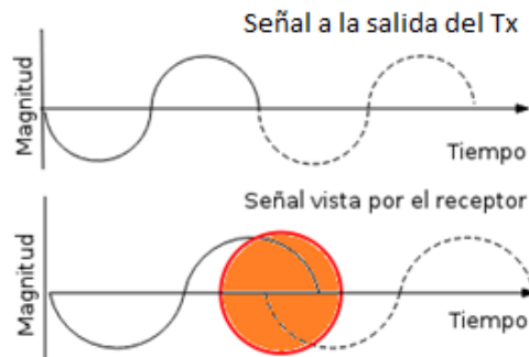
Figura 7 Señal distorsionada por ISI (en el dominio del tiempo)
