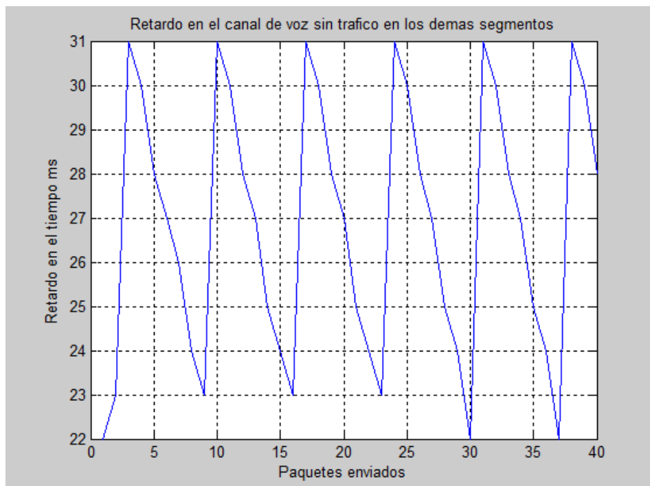
Figura 46 Gráfica de los retardos de los paquetes ping
