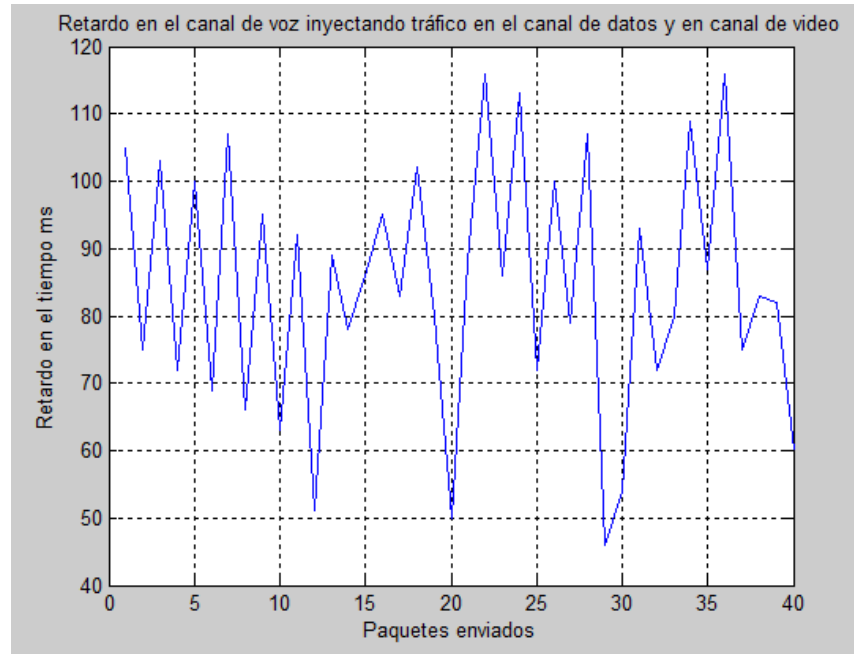
Figura 54 Gráfica de los retardos de los paquetes ping
