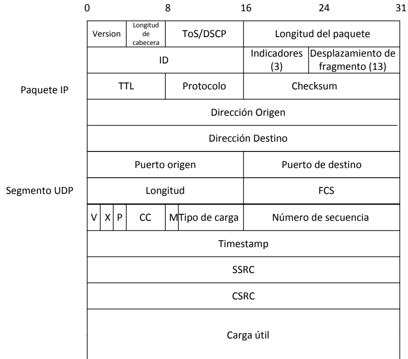
Figura 13 Encabezados de protocolo RTP, UDP e IP
