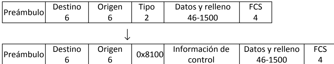
Figura 8 Trama 802.1Q [17]
