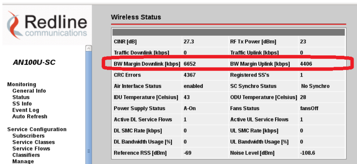
Figura 41 Máxima tasa de transmisión indicada por la BS
