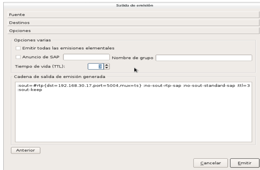
Figura 34 Opciones de red
