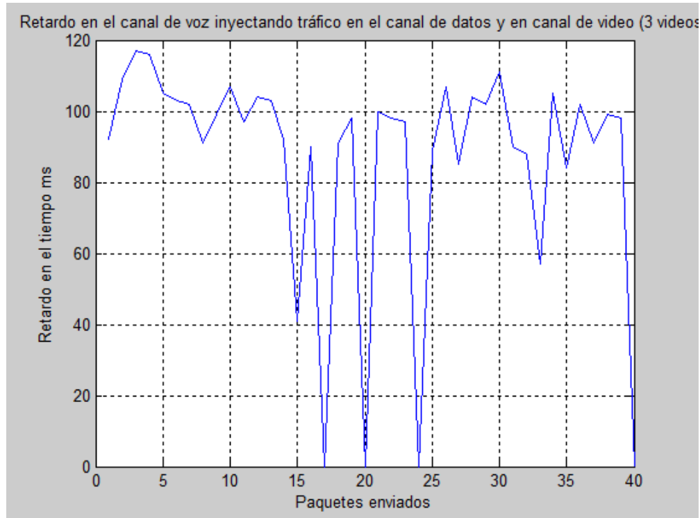
Figura 66 Gráfica de los retardos de los paquetes ping
