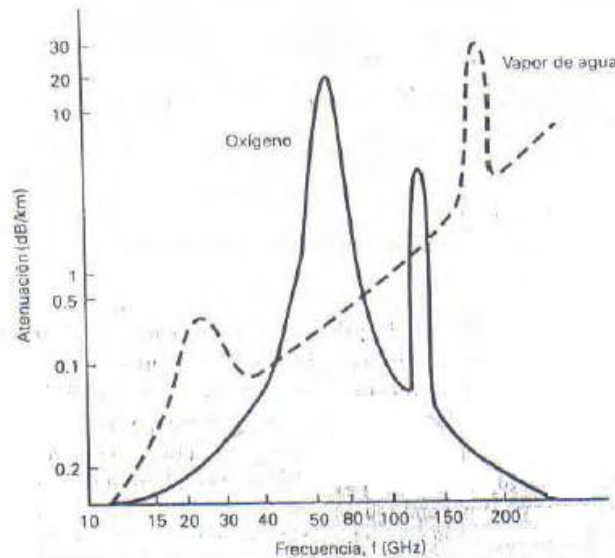
Figura 6 Atenuación de las ondas radioeléctricas debido a la presencia de oxígeno y de vapor de agua [6]
