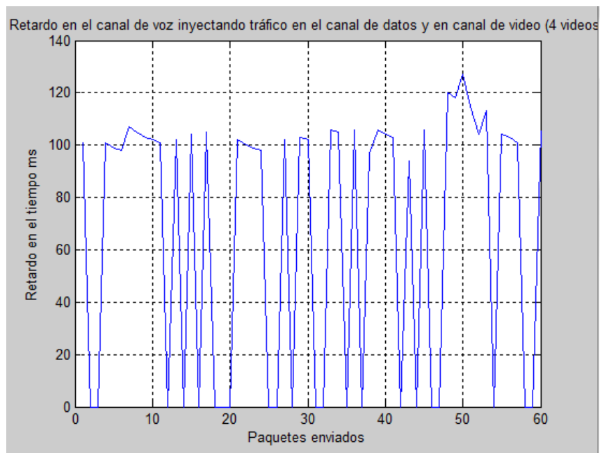
Figura 72 Gráfica de los retardos de los paquetes ping
