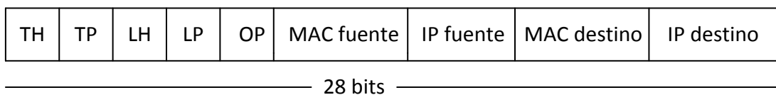
Figura 11 Paquete ARP
