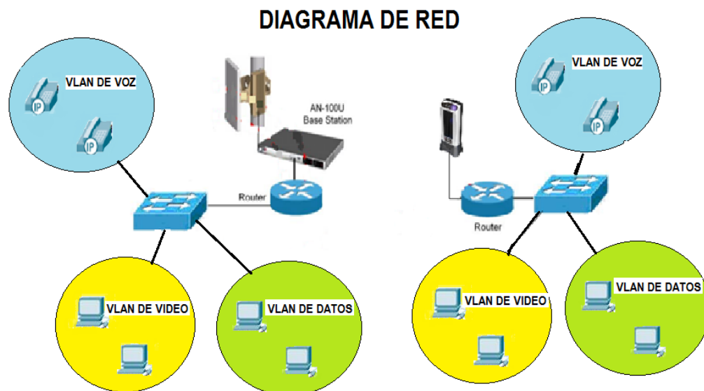
Figura 36 Topología implementada
