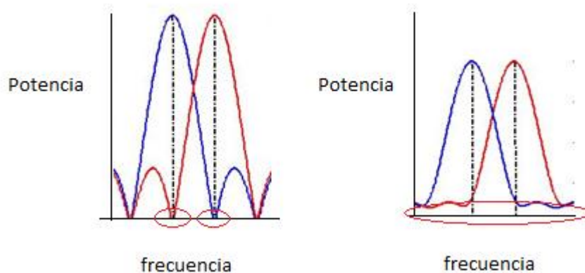
Figura 8 Ejemplo de ICI
