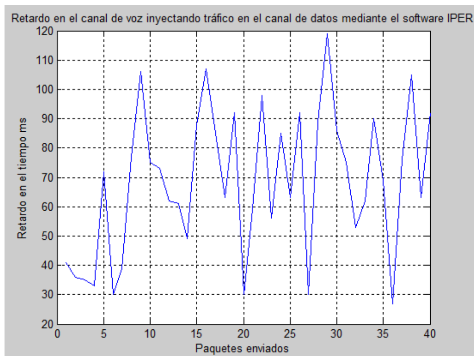
Figura 50 Gráfica de los retardos de los paquetes ping
