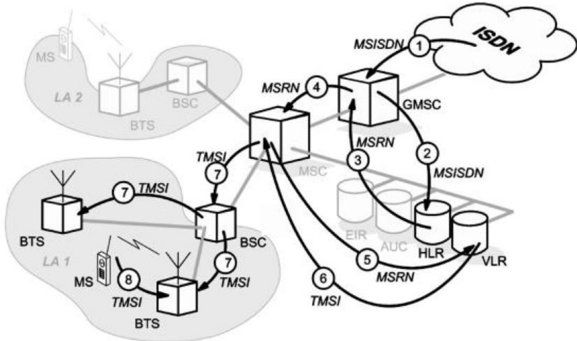
Figura 3.8 Principio de encaminamiento de las llamadas a abonados móviles.
