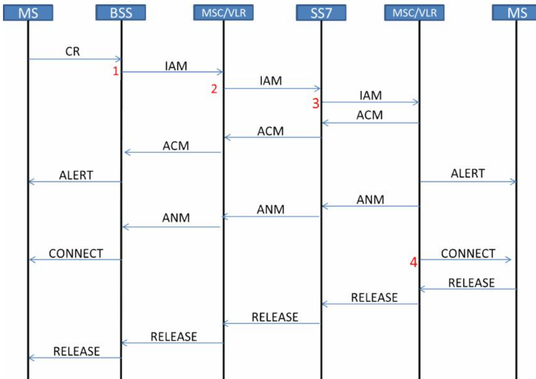
Figura 4.5 MOC Flujo de señalización.
