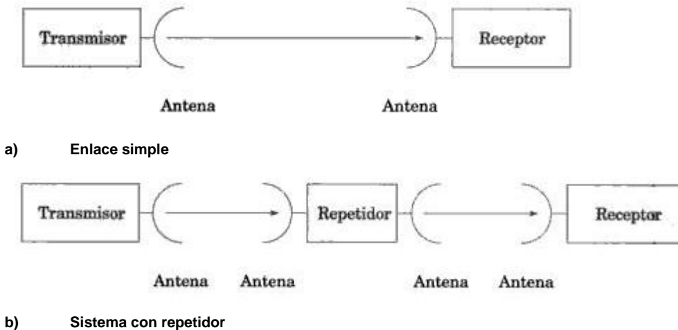
Figura 2.19 Sistemas de Comunicación por Microondas.
