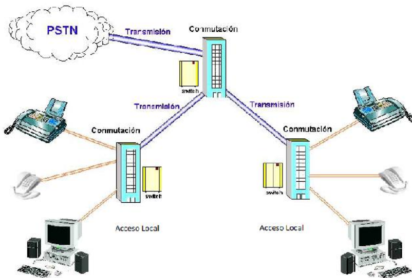
Figura 1.5 Sistema tradicional de telefonía.
