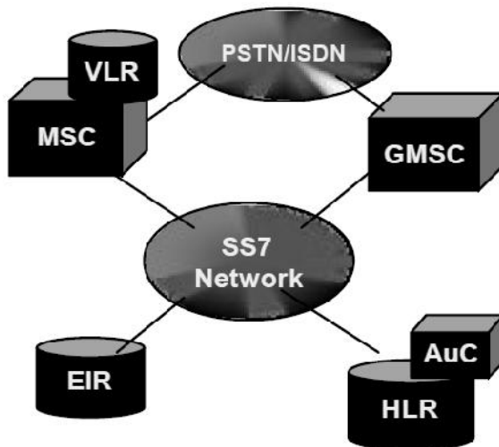
Figura 2.12 Registro de Identificación de Equipo, (EIR, Equipment Identity Register) y Puerta de acceso MSC (GMSC, Gateway MSC).
