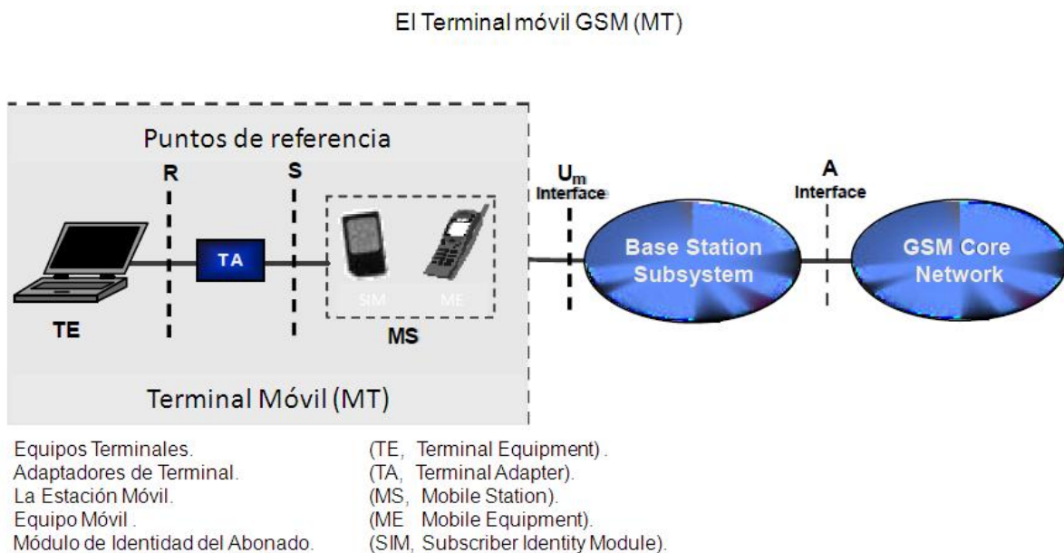
Figura 2.9 El Terminal móvil.
