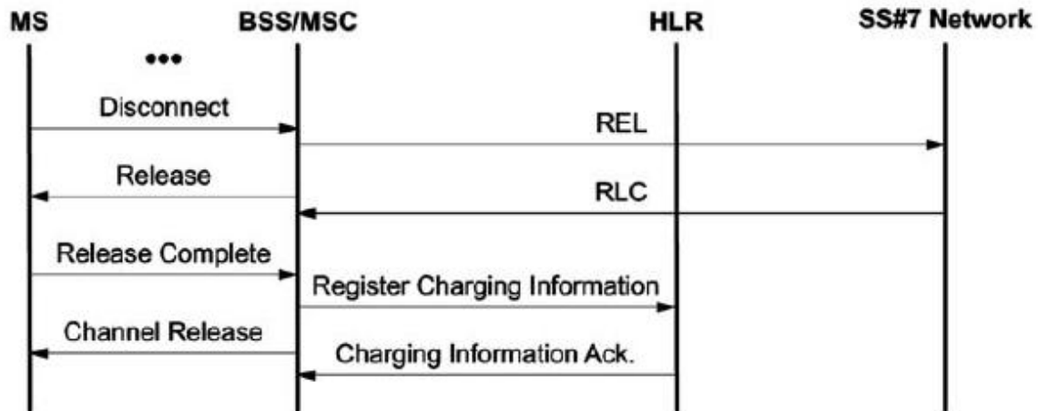
Figura. 3.9 Inicio de llamada móvil, terminación y almacenamiento de información de cargo.
