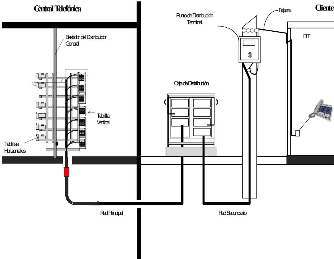
Figura 1.6 Diagrama de elementos en una red telefónica pública conmutada para un abonado.
