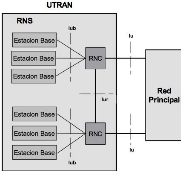
Figura 2.24 Arquitectura General UTRAN.
