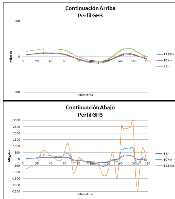
Figura 33.- Perfil GH3. Imagen de las gráficas de las continuaciones arriba y las continuaciones abajo aplicados a los valores de gravedad observada.
