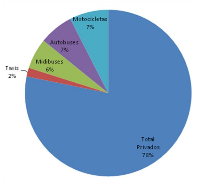
Figura 5.10 Estructura de las emisiones de GEI (CO 2 eq) para el transporte de pasajeros en la ZMG (2007, por modo)
