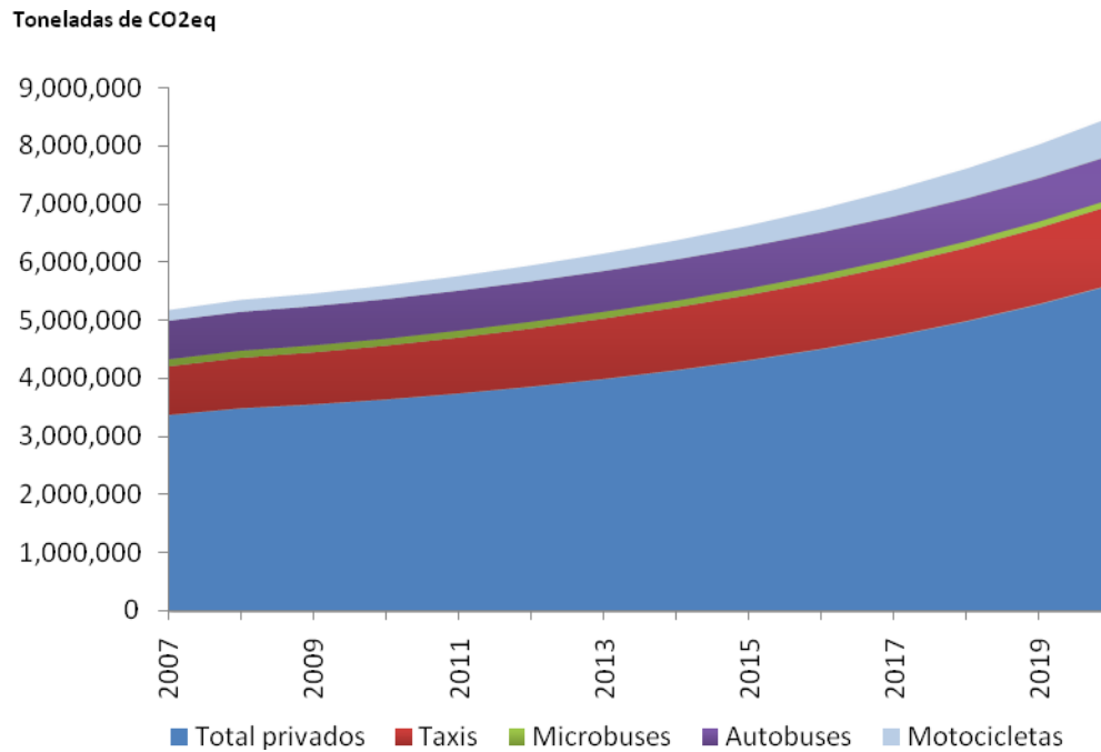
Figura 6.19. Emisiones equivalentes de CO 2 , ZMM (escenario base)
