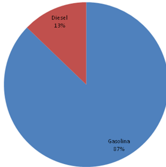
Figura 6.13 Estructura de las emisiones de GEI (CO 2 eq) para el transporte de pasajeros en la ZMM (2007, por combustible)
