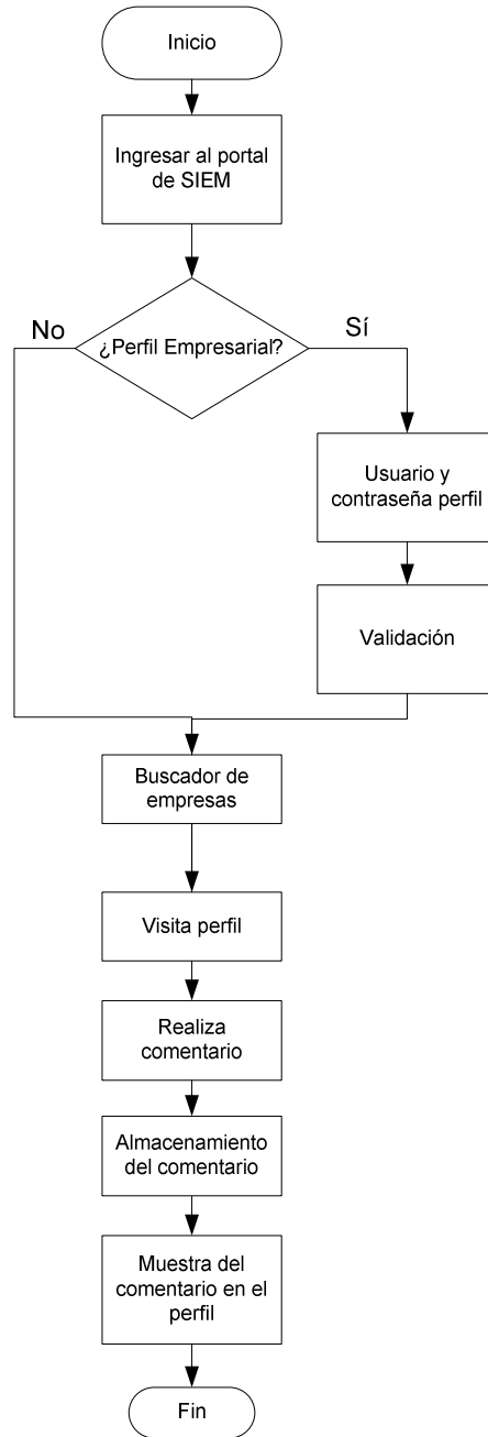
Figura 4.2: Diagrama de flujo de comentarios.
