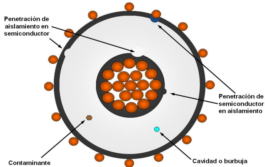
Figura 1.19.- Defectos y consecuencias de los aislamientos
