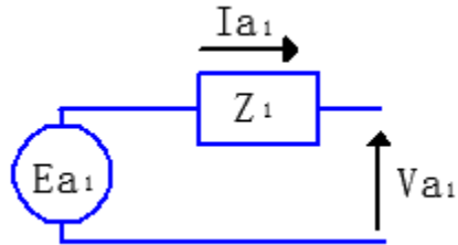
Figura A.8.- Circuito equivalente de secuencia positiva
