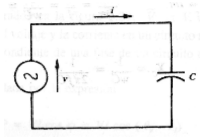
Figura 3.7.- Circuito capacitivo
