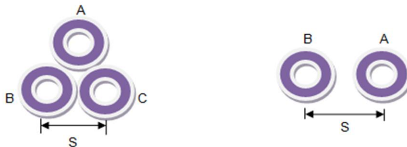
Figura 3.10.- Formación triangular o equidistante
