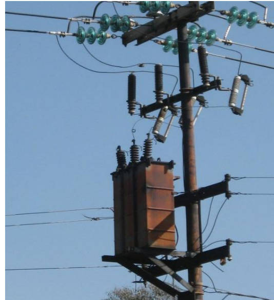
Figura AN.15.- Corrosión en los transformadores
