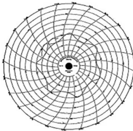
Figura 5-8 Inadecuado gasto de inyección de gas
