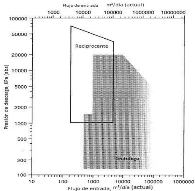
Figura. 1-18 Envoltura operativa del compresor.
