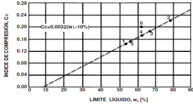
Figura 1.11 Relación entre el índice de compresión y el limite líquido para arcillas normalmente consolidadas de Medellín (Maturana, 1994).
