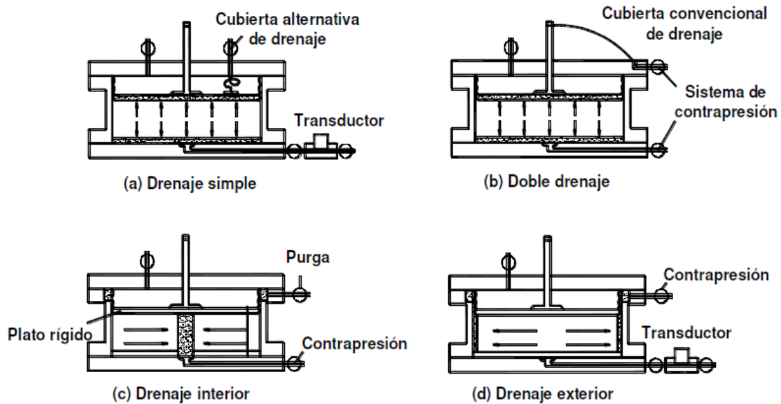
Figura 1.9 Drenaje y medición de presión de poro, de acuerdo con los cuatro tipos de pruebas que pueden desarrollarse (Rowe, 1966).
