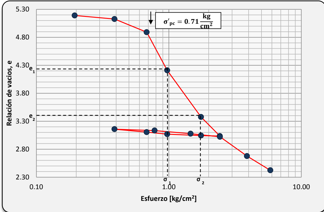
Figura A. 9 Curva de compresibilidad 9: Relación de vacíos acumulada vs esfuerzo efectivo, e=5.26 , C_c=3.27 y \sigma'_{pc}=0.71 .
