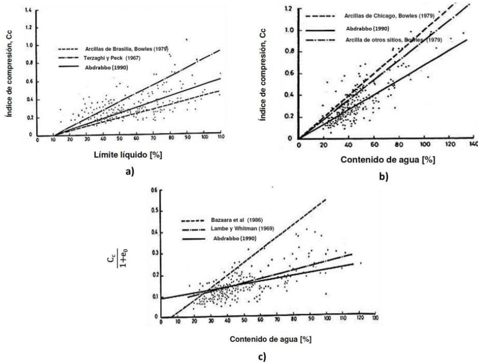
Figura 1.10 a) Índice de compresión vs límite líquido, b) Índice de compresión vs contenido de agua, c) C_c/1+e_0 vs contenido de agua (Abdrabbo, 1990).
