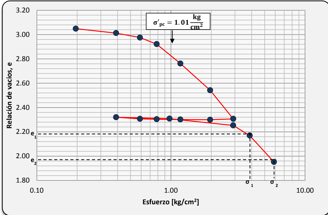
Figura A. 27 Curva de compresibilidad 27: Relación de vacíos acumulada vs esfuerzo efectivo, e=3.10 , C_c=1.21 y \sigma'_{pc}=1.01 .
