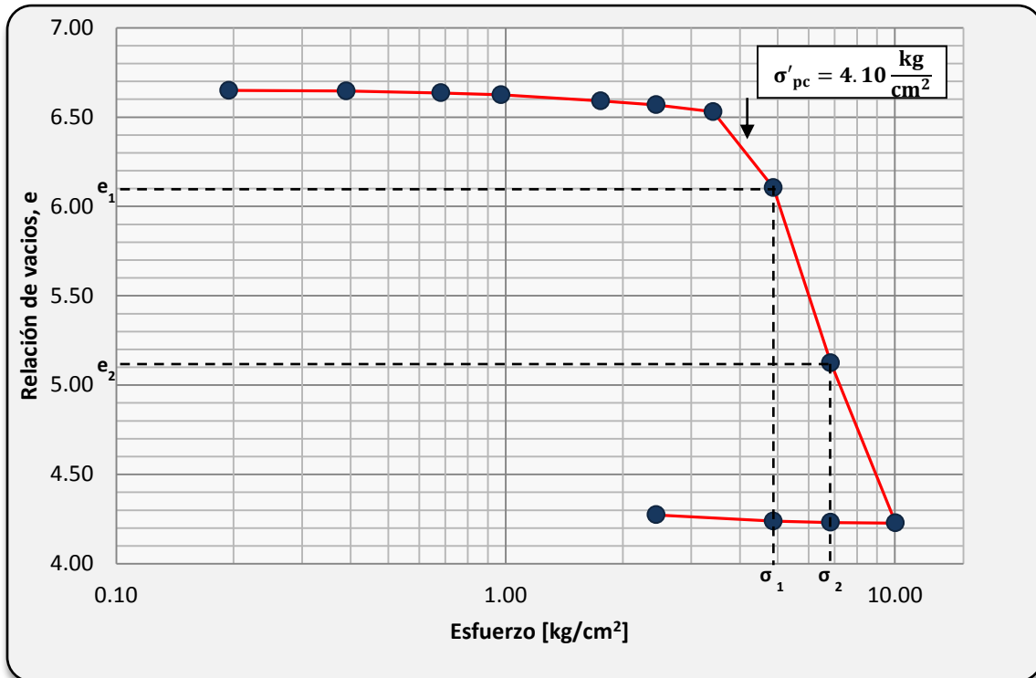
Figura A. 19 Curva de compresibilidad 19: Relación de vacíos acumulada vs esfuerzo efectivo, e=6.65 , C_c=6.66 y \sigma'_{pc}=4.10 .
