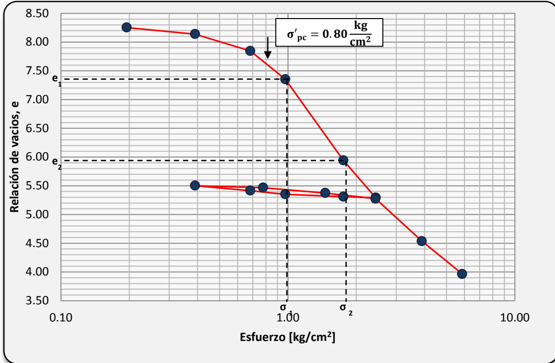
Figura A. 11 Curva de compresibilidad 11: Relación de vacíos acumulada vs esfuerzo efectivo, e=8.38 , C_c=5.52 y \sigma'_{pc}=0.80 .
