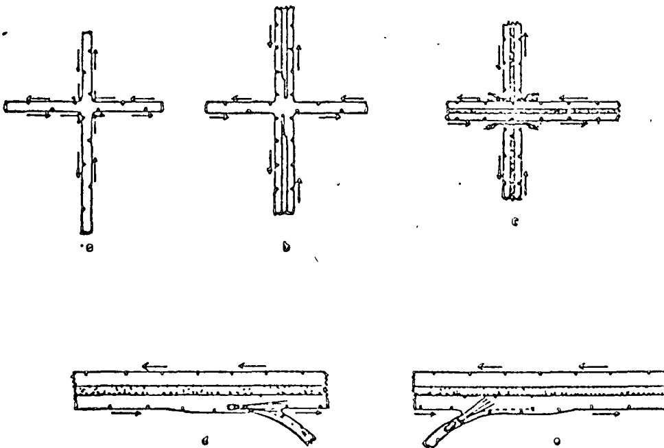
Posición de los luminarios en diferentes tipos de intersecciones
