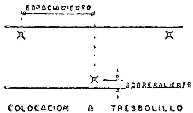
Diferentes formas de colocacion de luminarios
