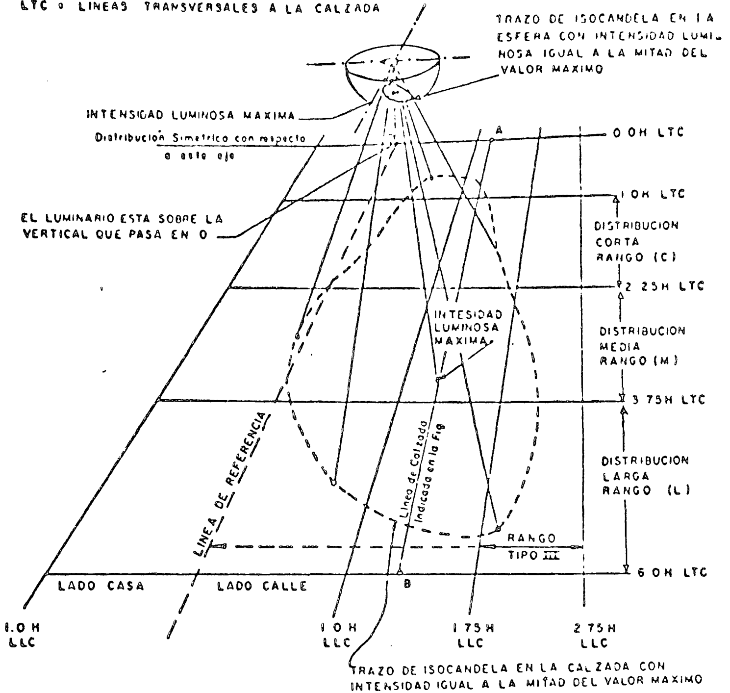
Diagrama que representa la proyección de la intensidad luminosa máxima y el trazo de isocandela, para un luminaire que tiene un tipo III de distribución media, en la esfera imaginaria y en la calzada.
