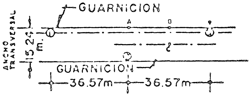
FIG. B. Separación longitudinal en tresbolillo
