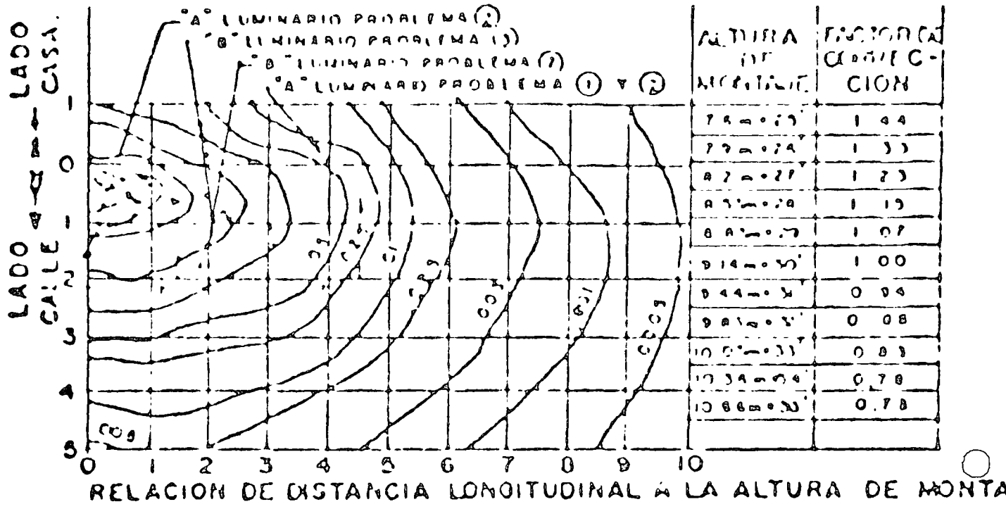
FIG. A. Ejemplo de diagrama de isobriancie, de bujias-pie horizontales sobre superficie de pavimento para un luminario que proporciona una distribución tipo III. Lámpara de 10,000 lúmenes iniciales, factor de conservación del luminario omitido
