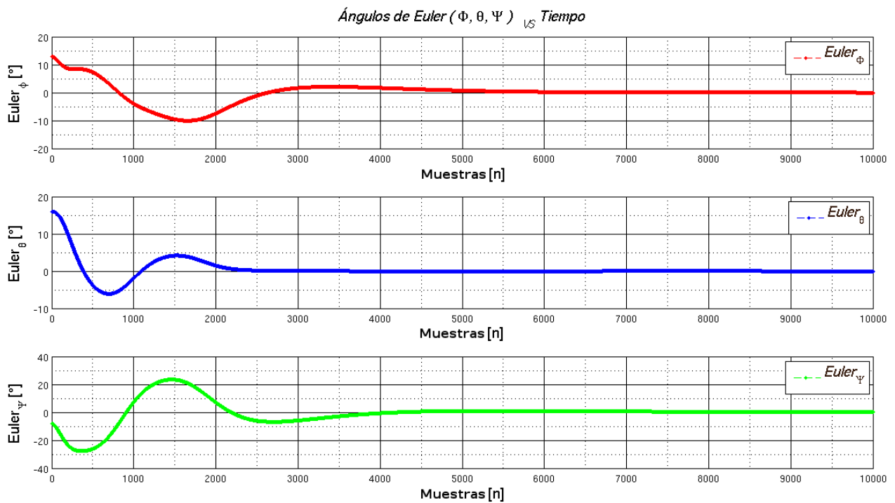
Figura 3.17: Gráfica de ângulos de Euler para valores iniciais \phi = 12.825 , \theta = 15.987 , \psi = -8.197 generada por Matlab, por separado.
