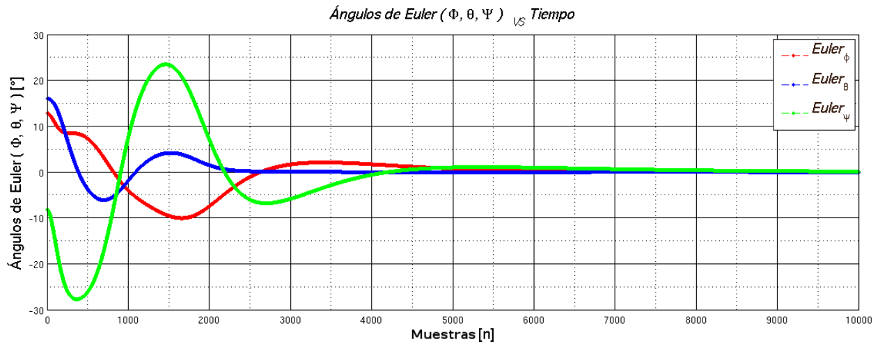
Figura 3.16: Gráfica de ângulos de Euler para valores iniciais \phi = 12.825 , \theta = 15.987 , \psi = -8.197 generada por Matlab.
