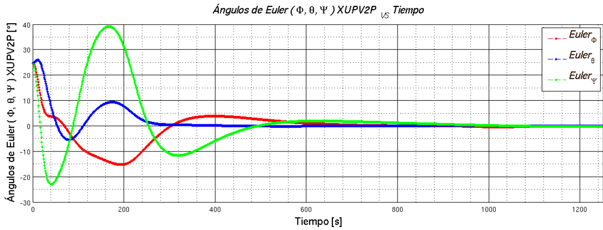
Figura 3.36: Gráfica de ângulos de Euler para valores iniciais \phi = 25 , \theta = 25 , \psi = 25 gerada por XUPV2P.
