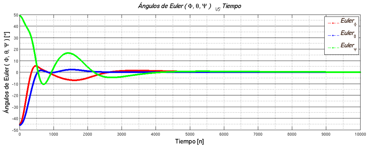
Figura 3.13: Gráfica de ângulos de Euler para valores iniciais \phi = -45.125 , \theta = -45.987 , \psi = 48.978 gerada por Matlab.
