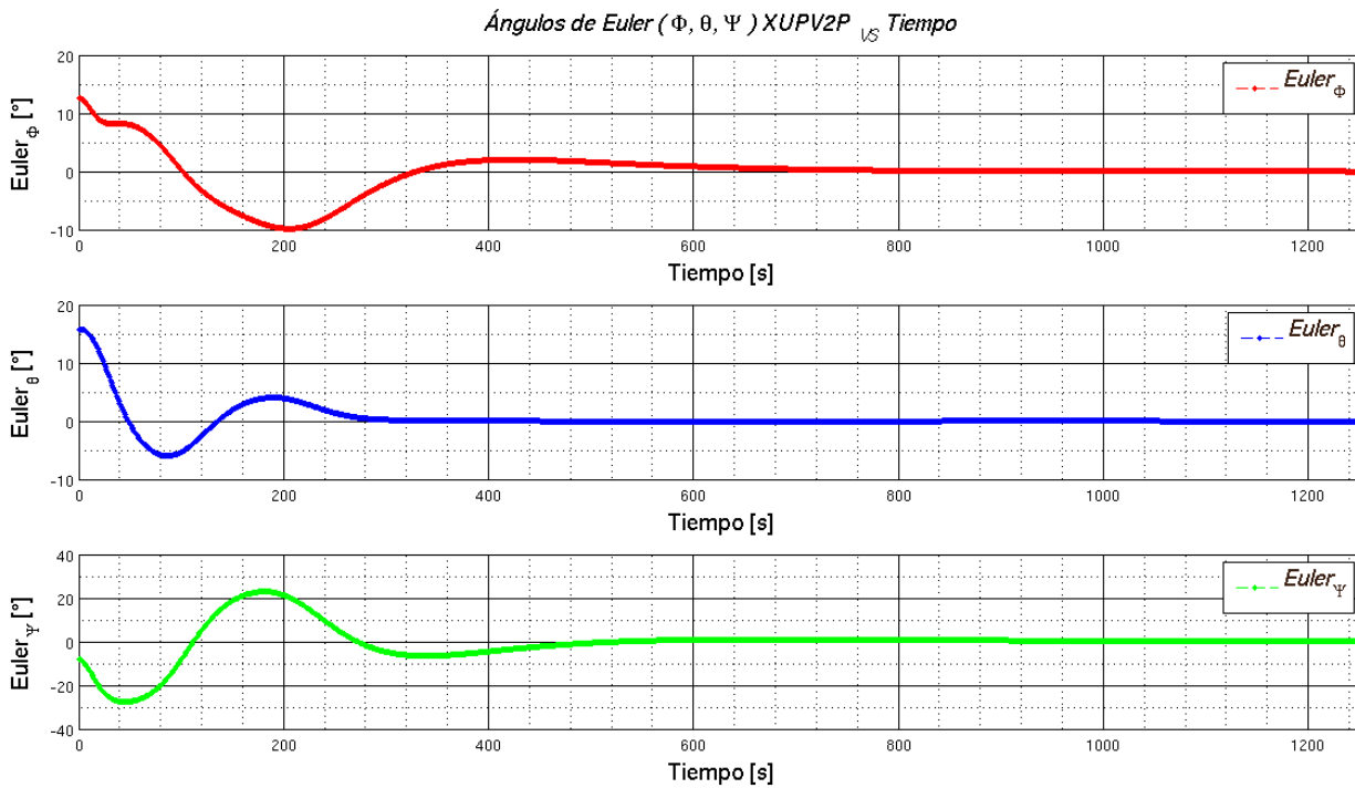
Figura 3.31: Gráfica de ângulos de Euler para valores iniciais \phi = 12.825 , \theta = 15.987 , \psi = -8.197 generada por XUPV2P, por separado.
