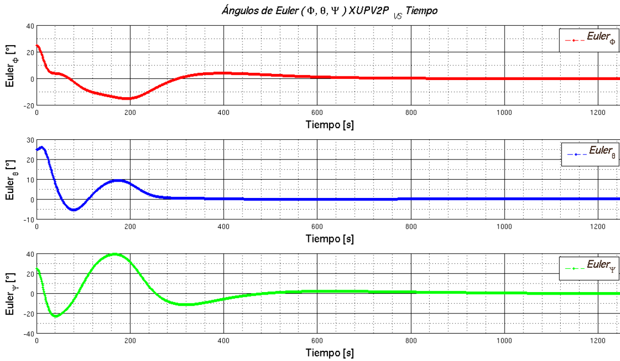
Figura 3.37: Gráfica de ângulos de Euler para valores iniciais \phi = 25 , \theta = 25 , \psi = 25 gerada por XUPV2P, por separado.
