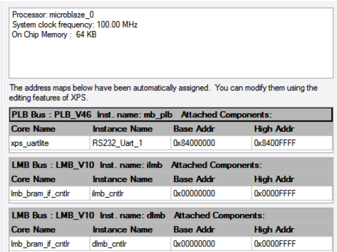
Figura 3.10: Mapa de memoria de configuración, velocidad de reloj y cantidad de memoria de la implementación.
