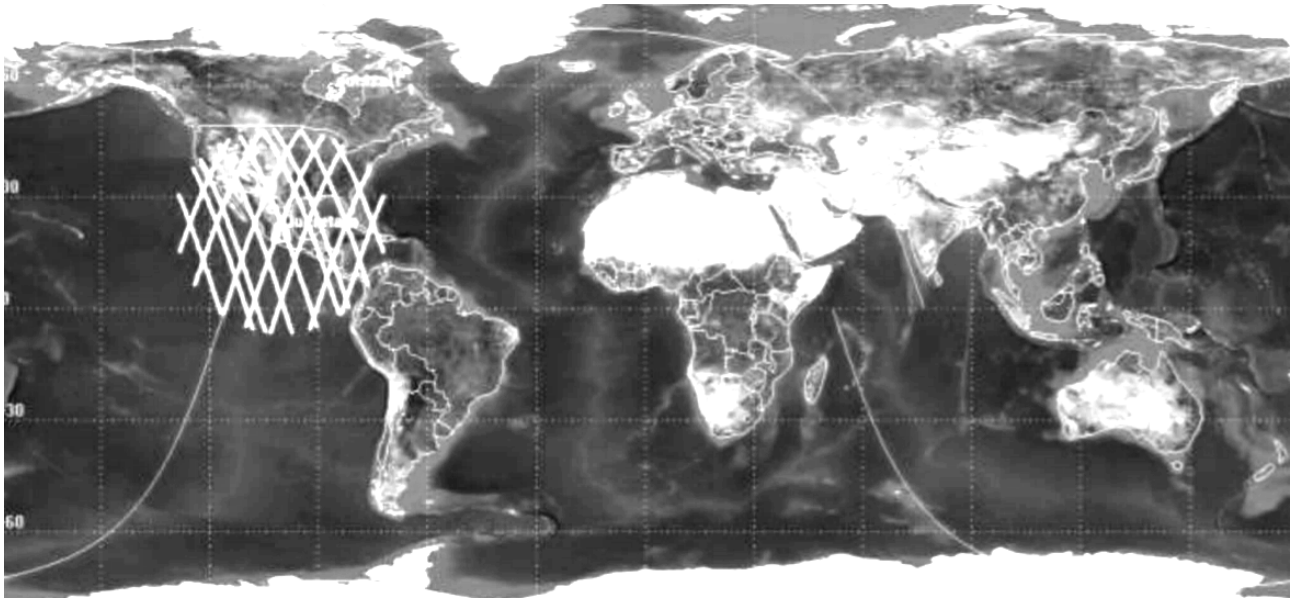
Figura 1.4: Simulación orbital Satélite Quetzal 800 km 105^\circ de inclinación [2]
