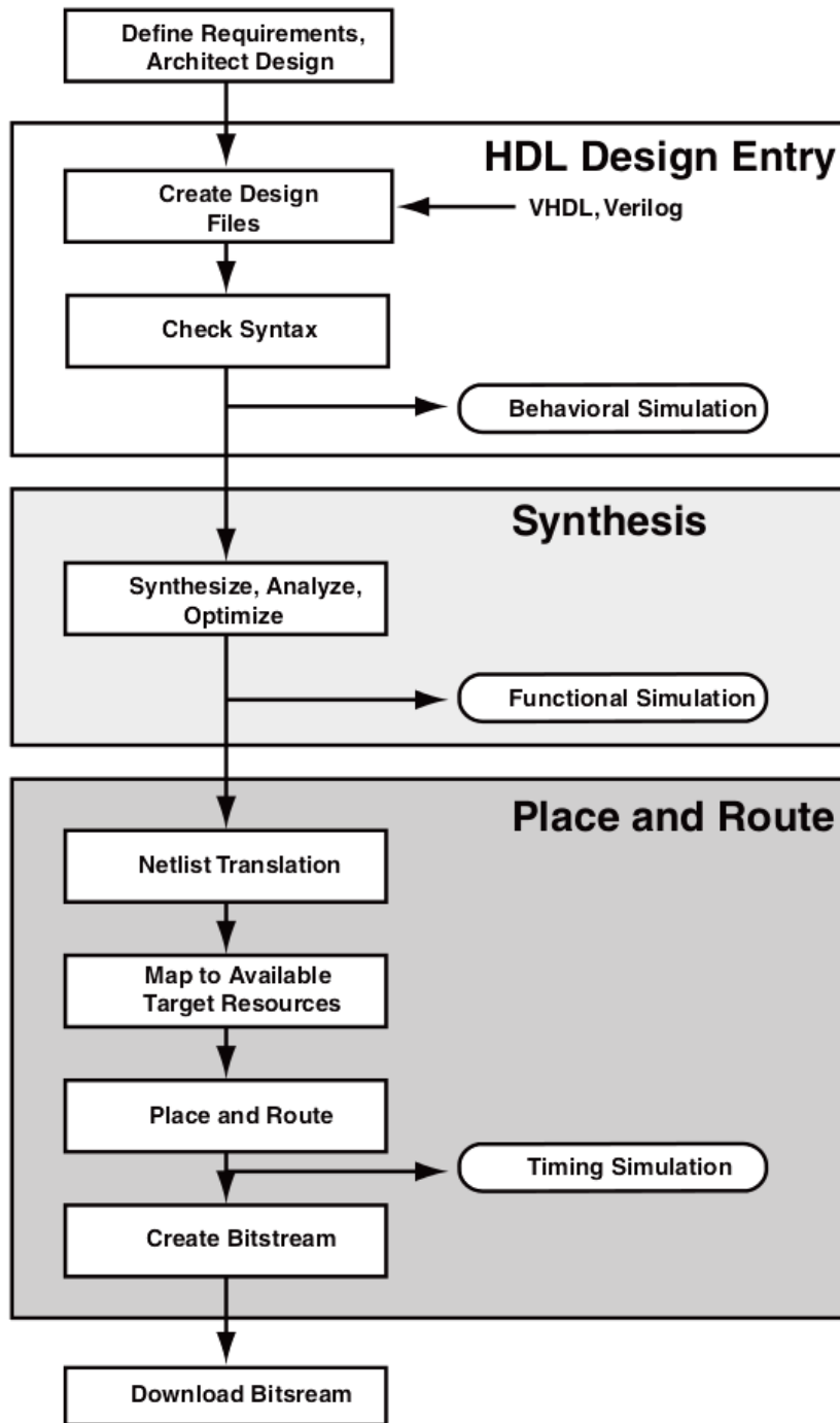
Figura 3.4: Diagrama de flujo de implementación de un diseño en FPGA [5].
