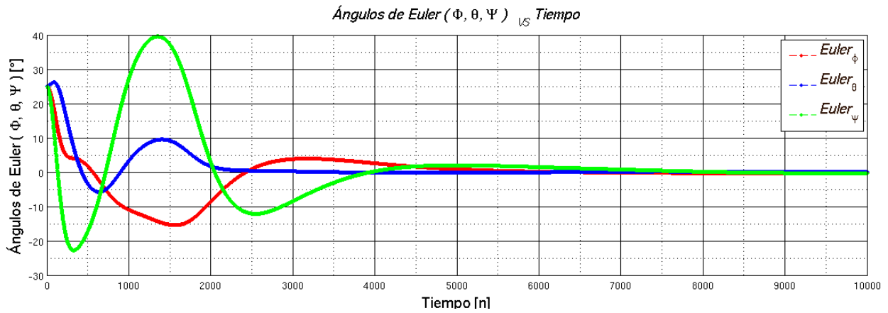
Figura 3.22: Gráfica de ángulos de Euler para valores iniciales \phi = 25, \theta = 25, \psi = 25 generada por Matlab.
