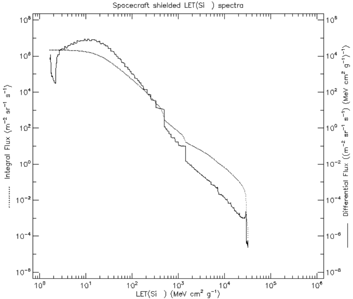
Figura 2.5: Flujo de partículas de alta energía para un volumen sensible paralelepípedo rectangular de 3.87\mu m \times 3.87\mu m \times 2.0\mu m . Estimada con SPENVIS usando el algoritmo constant LET (CREME) para la misión Quetzal.
