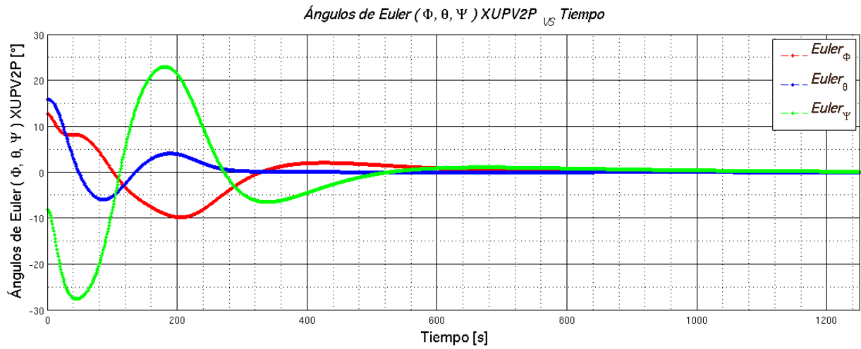
Figura 3.30: Gráfica de ângulos de Euler para valores iniciais \phi = 12.825 , \theta = 15.987 , \psi = -8.197 generada por XUPV2P.
