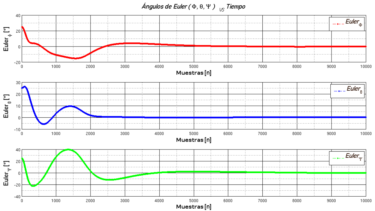
Figura 3.23: Gráfica de ángulos de Euler para valores iniciales \phi = 25, \theta = 25, \psi = 25 generada por Matlab, por separado.
