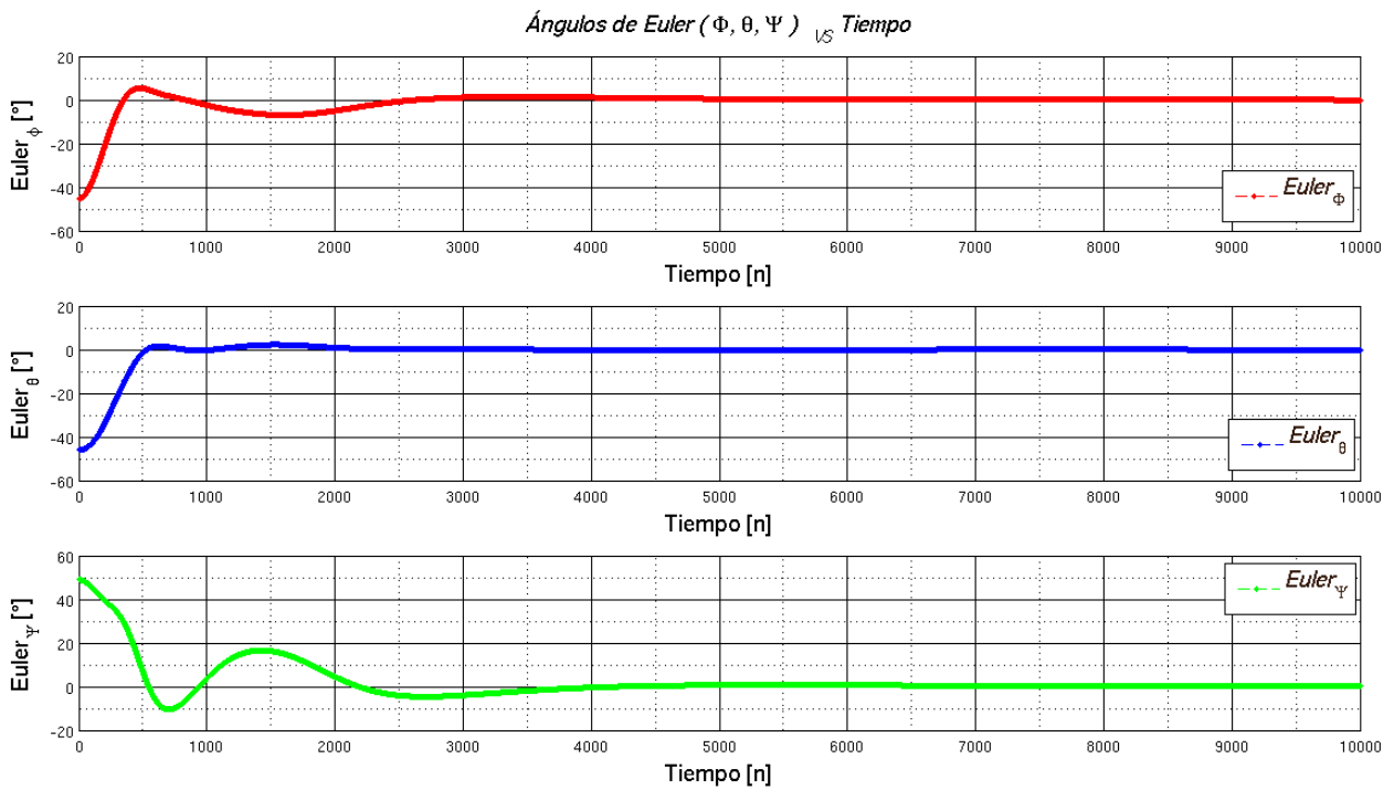
Figura 3.14: Gráfica de ângulos de Euler para valores iniciais \phi = -45.125 , \theta = -45.987 , \psi = 48.978 gerada por Matlab, por separado.
