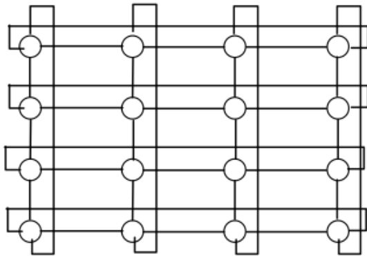
Figura 2.7 Malla
