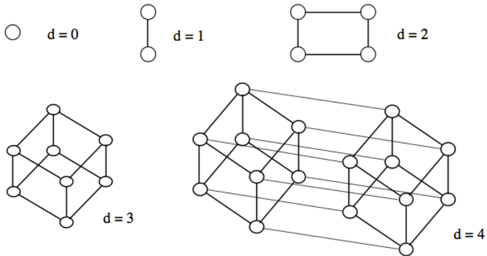
Figura 2.11 Hipercubo
