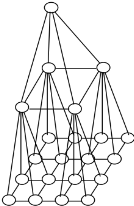
Figura 2. 9 Piramidal
