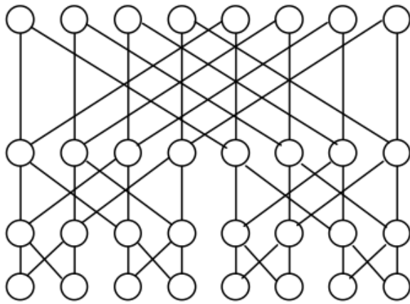
Figura 2.10 Mariposa
