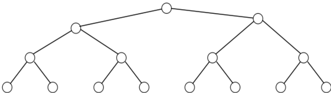
Figura 2.8 Árbol binario
