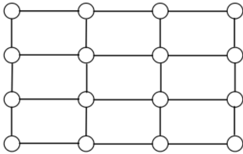
Figura 2.6 Malla
