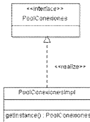
FIGURA V.5 - DIAGRAMA DE CLASES: POOLCONEXIONES SINGLETON
