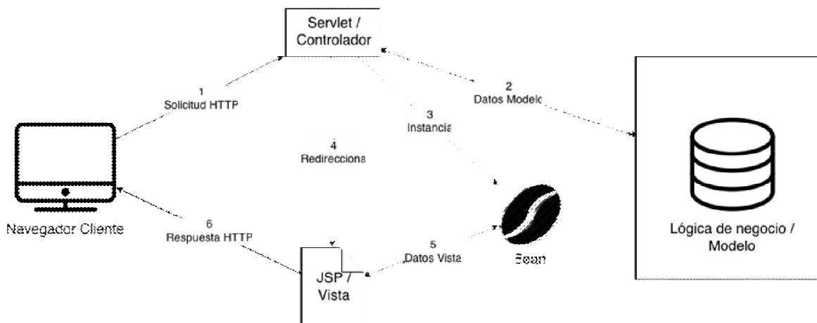
FIGURA IV.13 - MODELO 2
