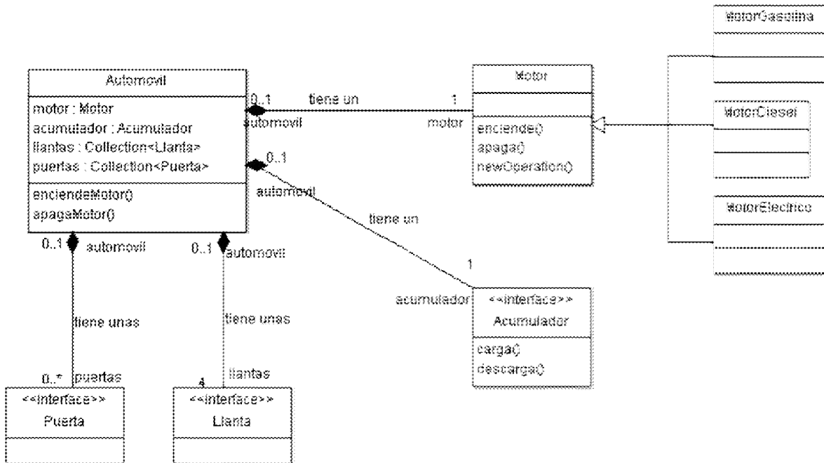
FIGURA III.10 - DIAGRAMA DE CLASES AUTOMOVIL Y LAS PARTES QUE LO COMPONEN
