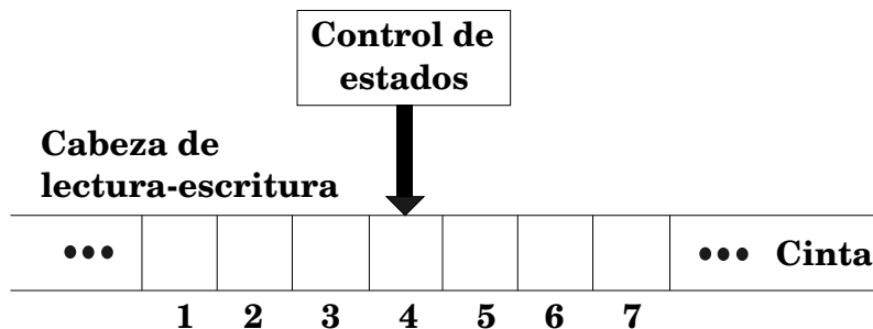
Figura 1.3: Máquina de Turing Determinista de una cinta (MTD). Consiste en un control de estados , una cabeza de lectura-escritura y una cinta infinita dividida en celdas, las cuales pueden contener cualquier símbolo definido dentro del alfabeto de la cinta [Gar79].
