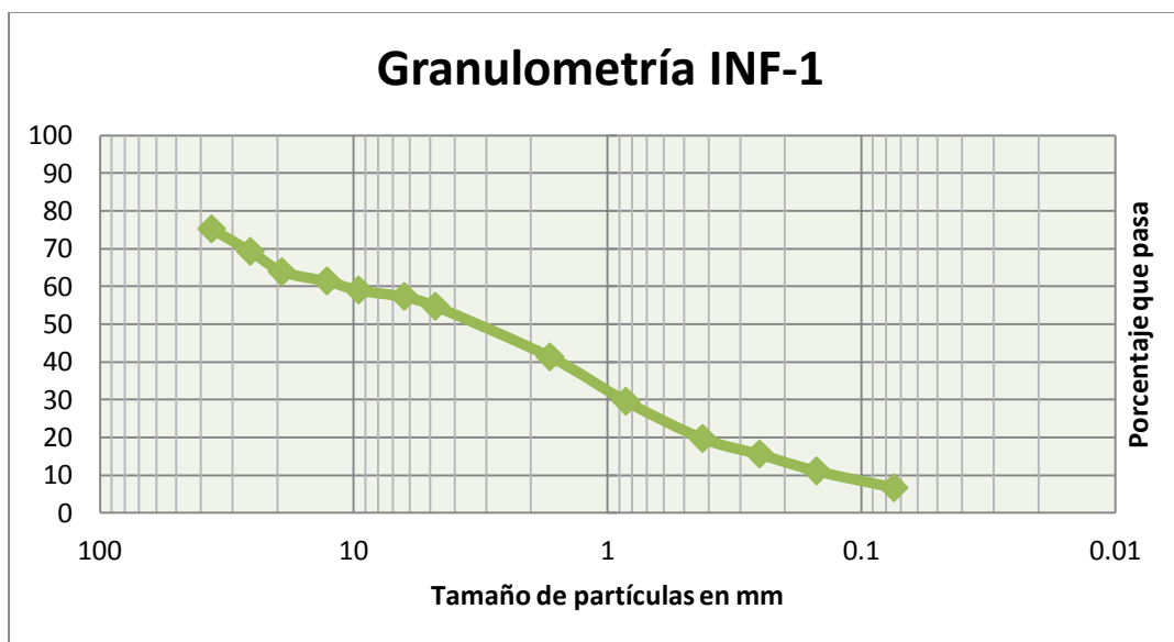
Figura 4.3.2 Curva granulométrica del suelo INF-1
