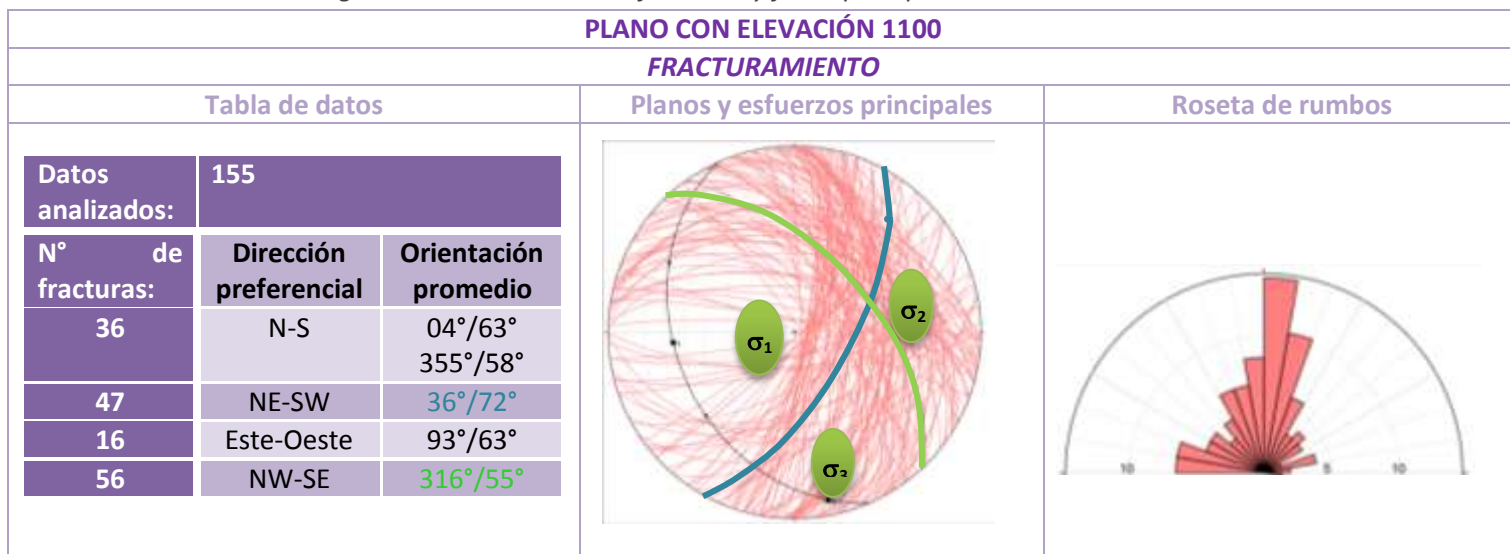
Figura 4.4.2 Análisis de fracturas y fallas para plano con elevación 1100
