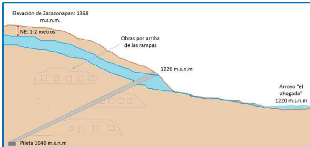
Figura 4.1.7 Circulación de agua dentro de las obras de la mina. (Neri, 2014).
