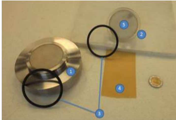
Figura 3.2.9 Material para llevar a cabo el montaje de la pastilla de roca a la cámara.
