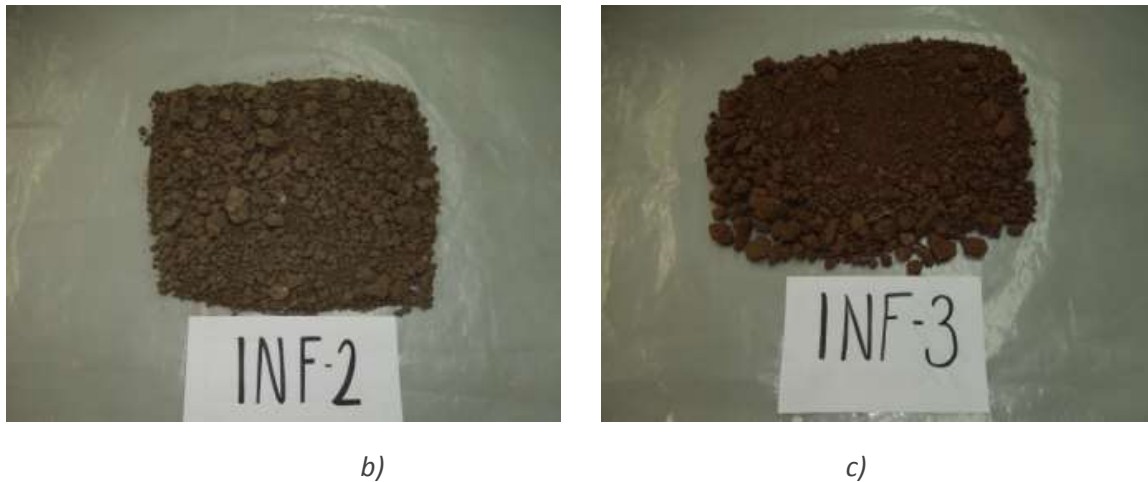
Figura 3.3.6 Muestra de suelo representativa para analizar la granulometría a) INF-1, b) INF-2 y c) INF-3.
