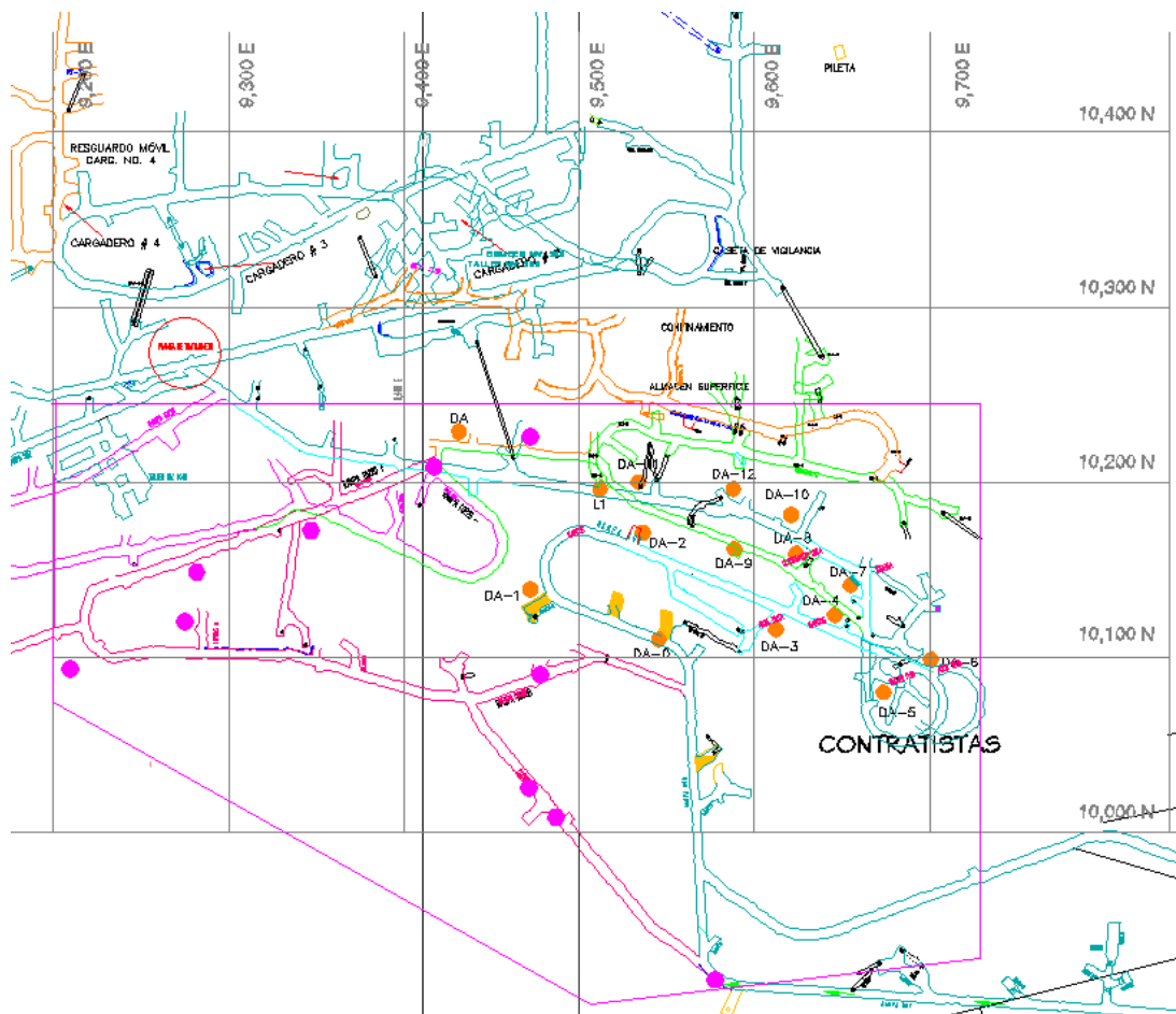
Figura 3.1.9 Delimitación de subcuenca dentro de las obras de la mina, enmarcada en color magenta, ubicada en coordenadas locales por minera Tizapa.
