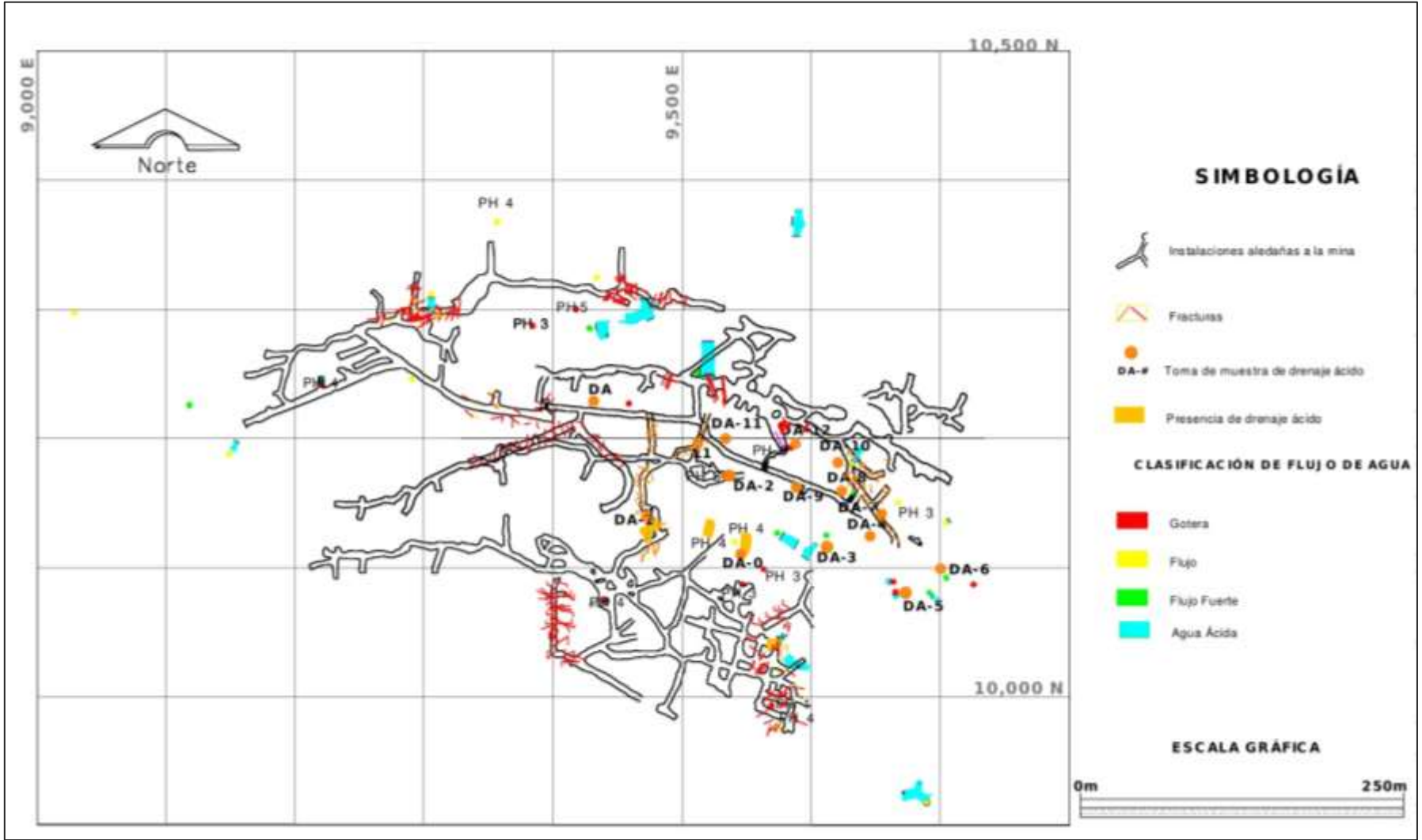
Figura 4.4.1 Plano de fracturamiento en las obras aledañas de la mina
