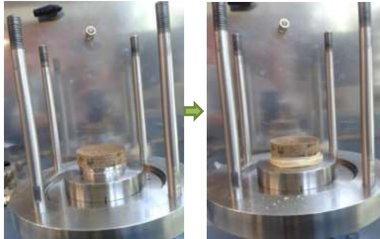
Figura 3.2.11 Colocación de la membrana de látex a la pastilla para el montaje en la cámara.
