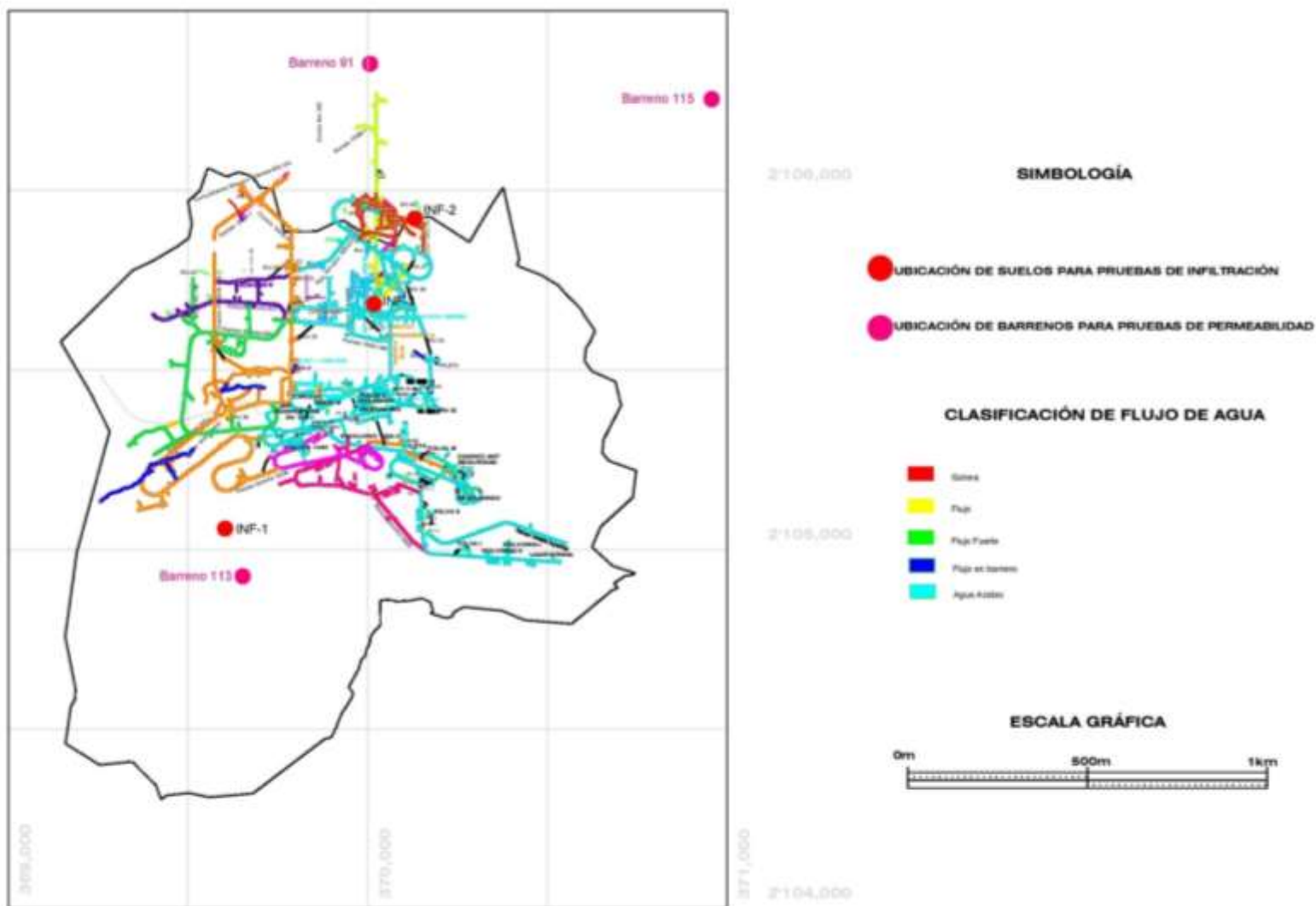
Figura 3.1.2 Ubicación de sitios de infiltración y permeabilidad
