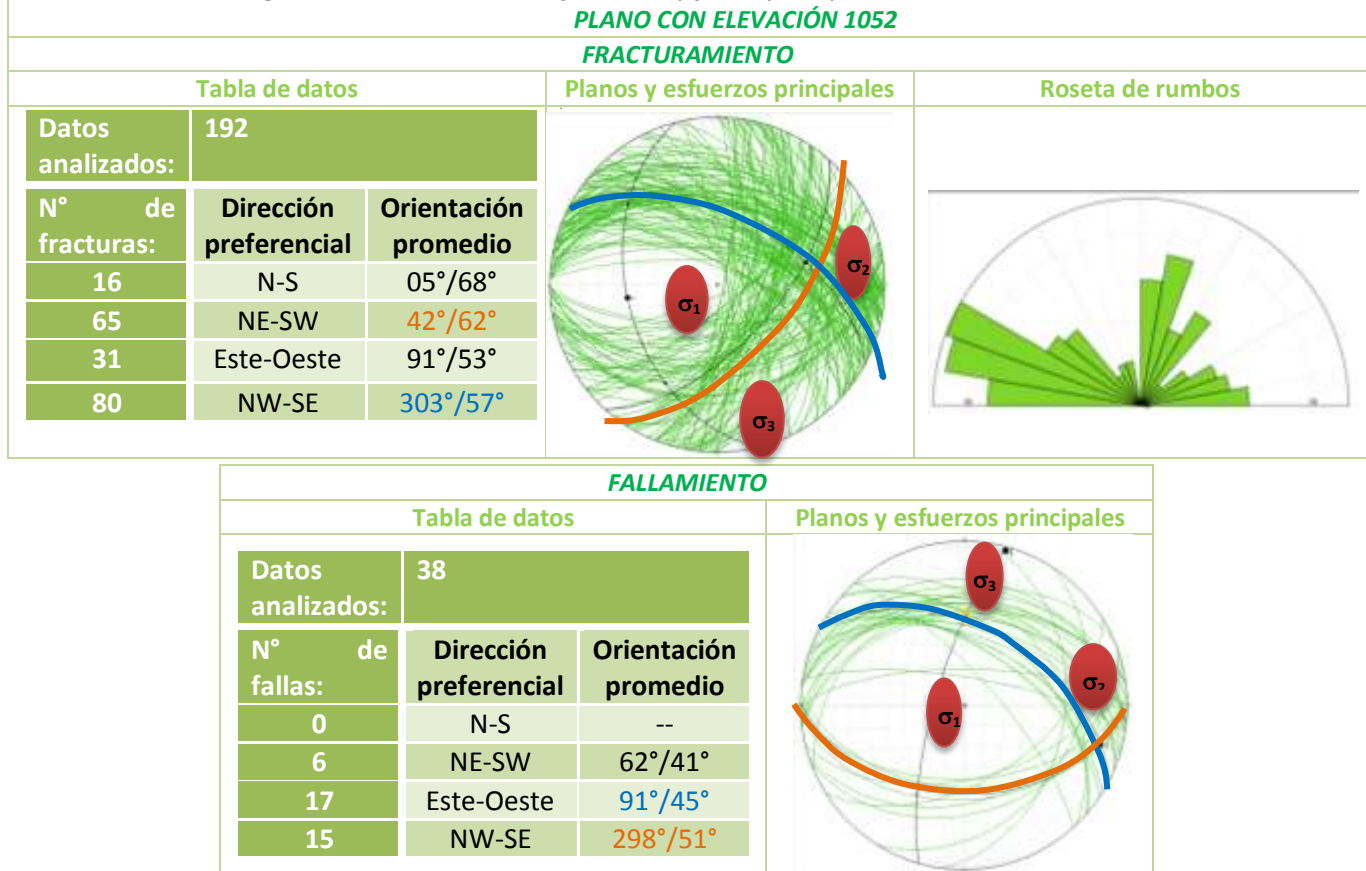
Figura 4.4.1 Análisis de fracturas y fallas para plano con elevación 1052
