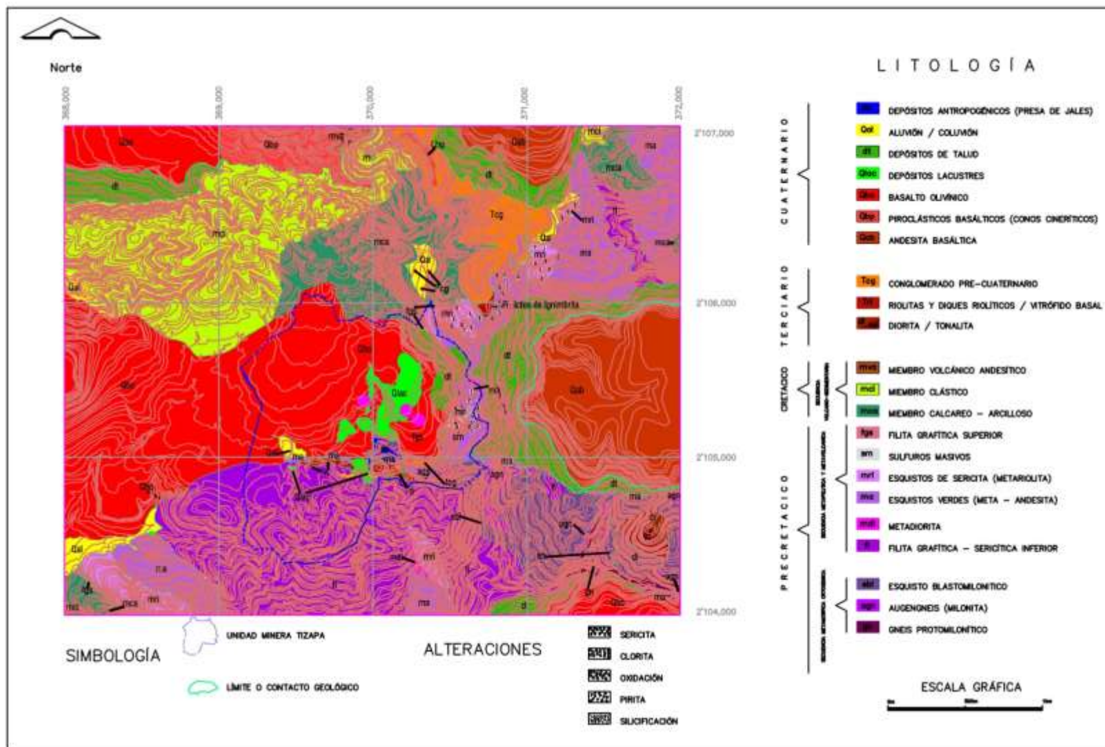
Figura 2.2.1 Geología de la mina Tizapa
