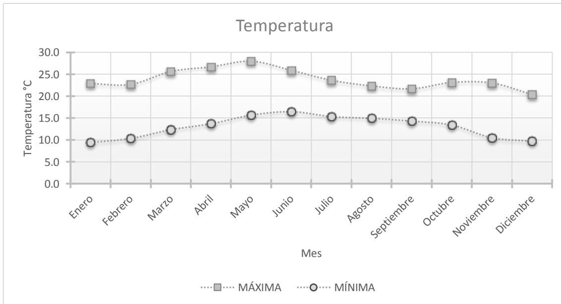
Figura 2.3.3 Temperatura máxima y mínima promedio por mes (años 1997 a 2012). Estación meteorológica de Tizapa
