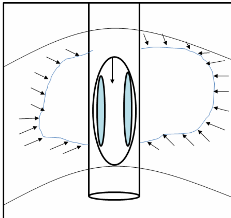
Figura 1.18. Tratamiento con fracturamiento hidráulico 19 .
