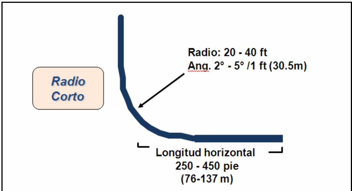
Figura 1.9. Pozo horizontal radio corto.
