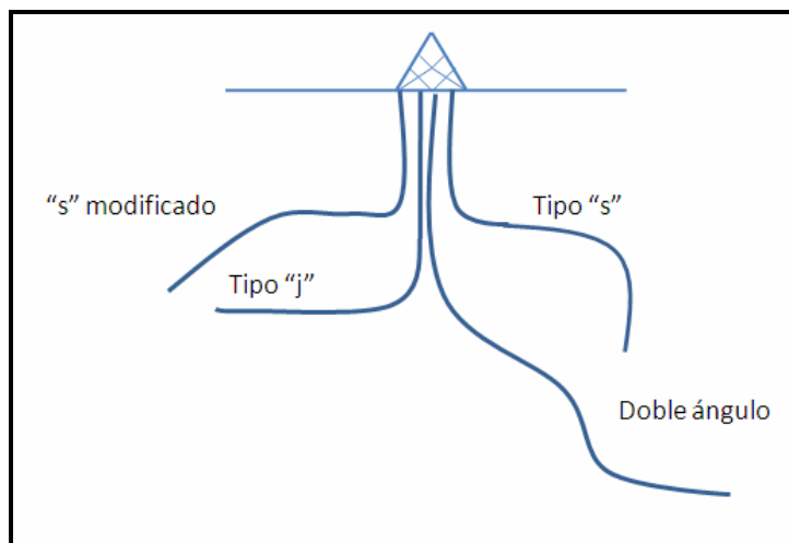
Figura 1.3. Trayectorias más comunes en los pozos direccionales 7 .
