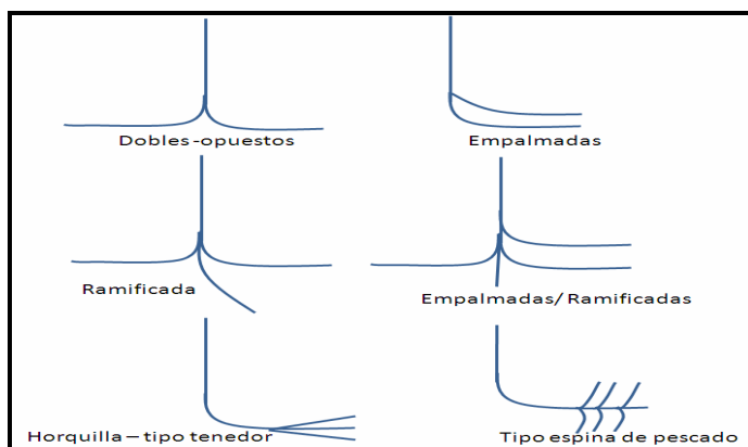
Figura 1.4. Presenta algunas de las posibles geometrías de pozos multilaterales 8 .
