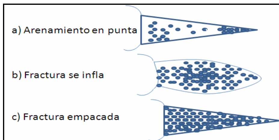
Figura 1.29. Crecimiento del espesor de la fractura mediante el arenamiento controlado en la punta de la fractura.
