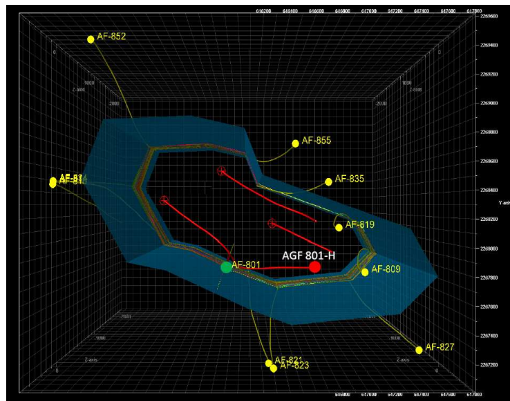
Figura 2.2. Pozo horizontal 801-H ubicado en el campo Agua Fría 62 .
