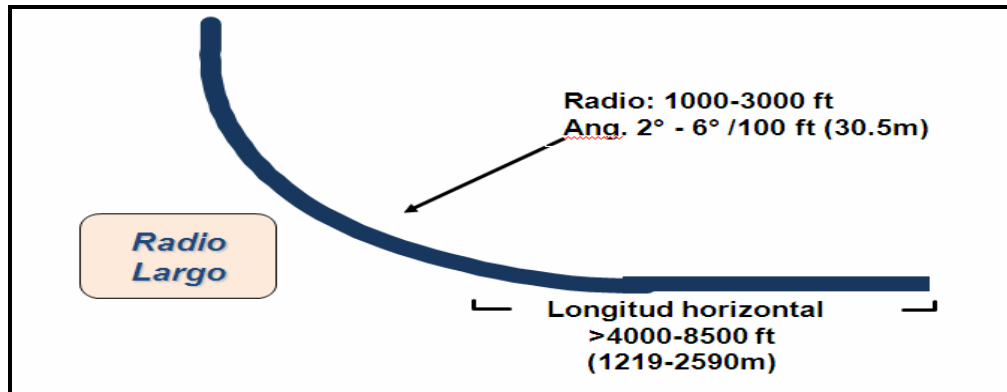
Figura 1.11. Pozo horizontal radio largo.
