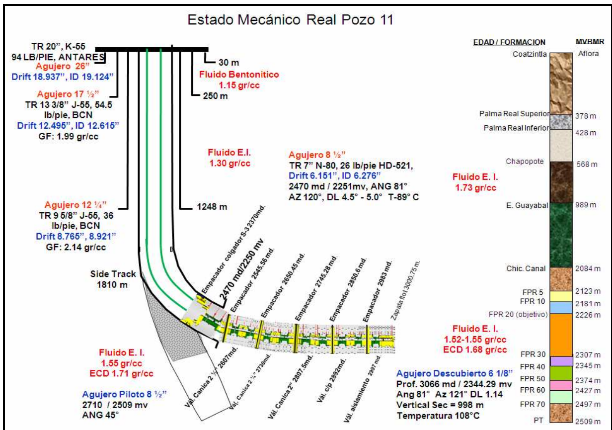
Figura 4.11. Estado mecánico programado, tomado del programa de perforación del pozo 11 85 .
