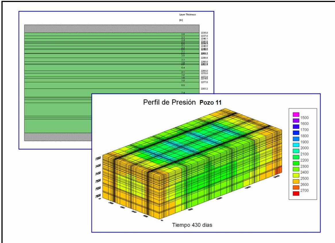
Figura 4.8. Simulación de la presión esperada en el pozo 11 82 .
