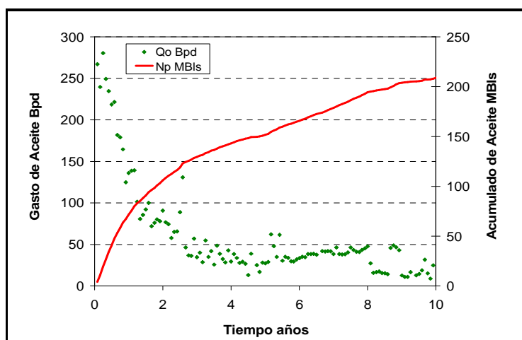
Figura 2.6. Producción acumulada en 10 años, Pozo Horizontal 3 67 .
