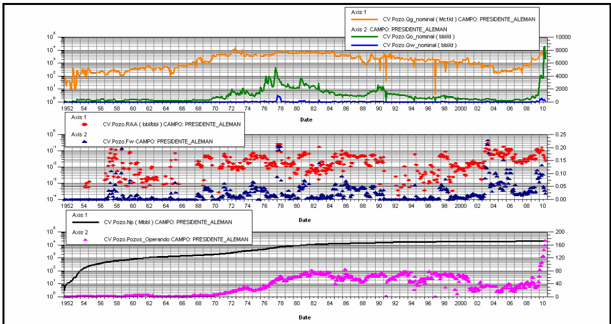
Figura 4.2. Historia de producción del campo al mes de noviembre del 2010 76 .
