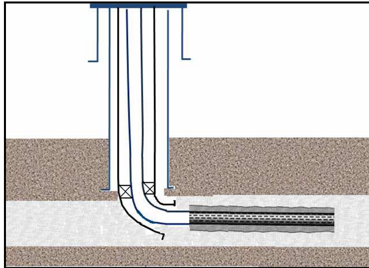
Figura 1.13. Terminación con Liners Ranurados.
