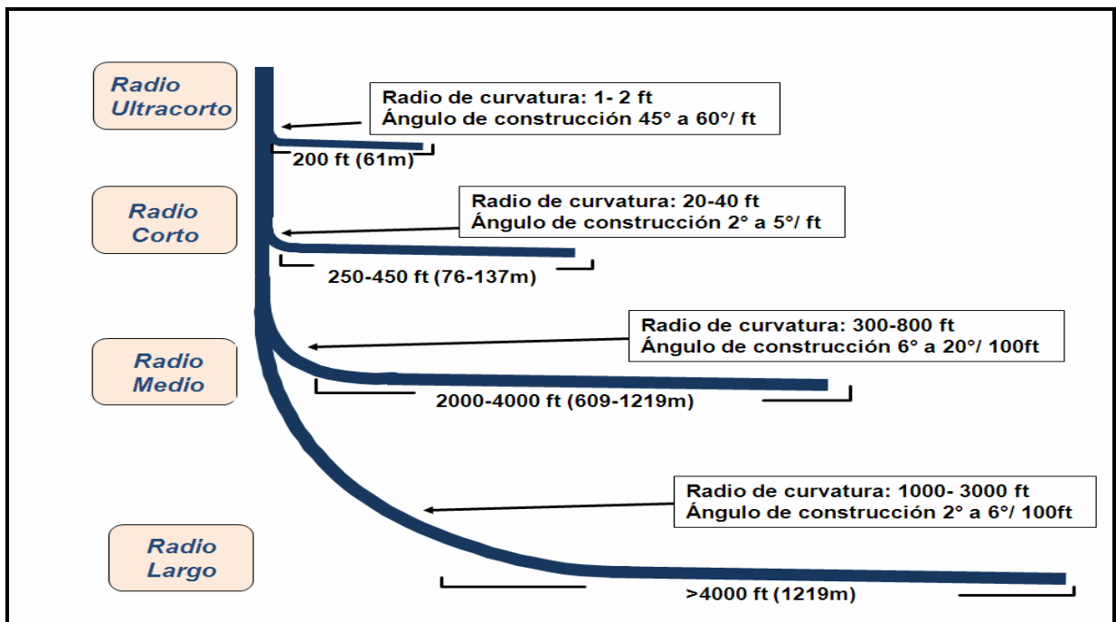
Figura 1.7. Clasificación de los pozos horizontales 14 .
