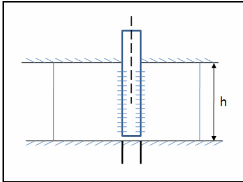
Figura 1.1. Pozo vertical perforado perpendicularmente al plano del yacimiento 3 .
