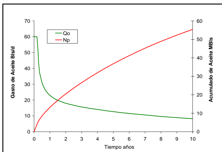
Figura 2.10. Producción acumulada esperada a 10 años Pozo Horizontal 8 71 .
