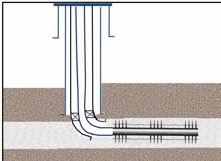
Figura 1.15. Terminación con liner, cementado y disparado.
