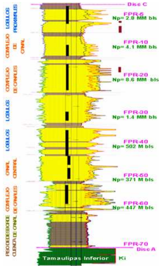
Figura A-4.2. Columna estratigráfica del campo Presidente Alemán
