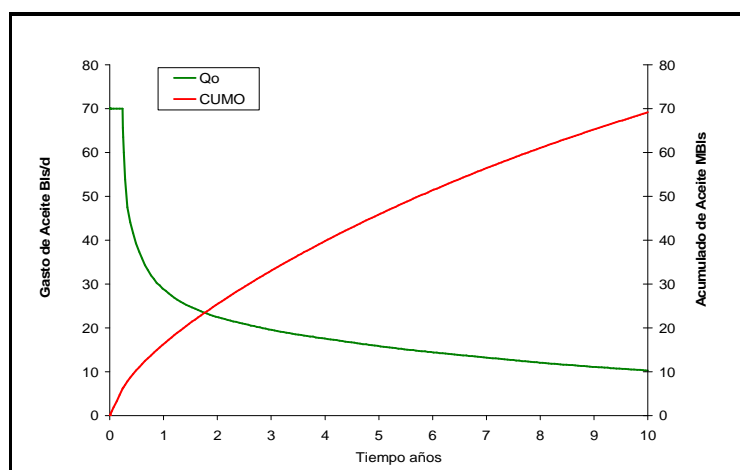
Figura 2.11. Producción acumulada esperada a 10 años Pozo Horizontal 9 72 .
