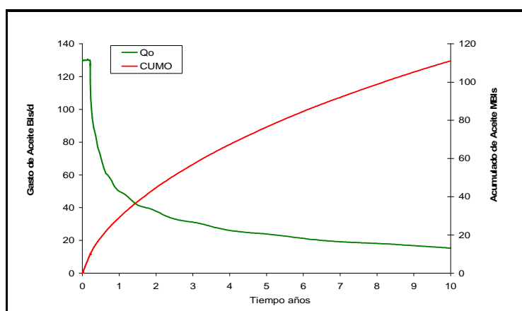
Figura 2.9. Producción acumulada esperada a 10 años, Pozo Horizontal 7 70 .
