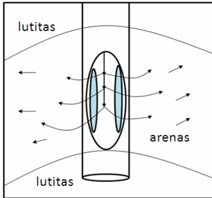
Figura 1.24. Introducción de material sustentante en la fractura 35 .
