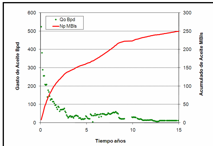
Figura 2.5. Producción acumulada en 15 años pozo horizontal 2 66 .
