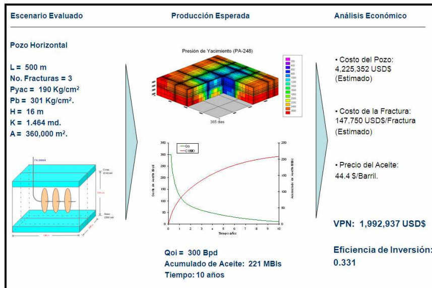
Figura 4.10. Producción acumulada en 10 años pozo 11 84 .
