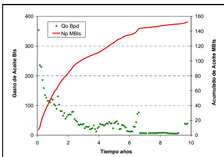
Figura 2.7. Producción acumulada en 10 años, Pozo Horizontal 4 68 .
