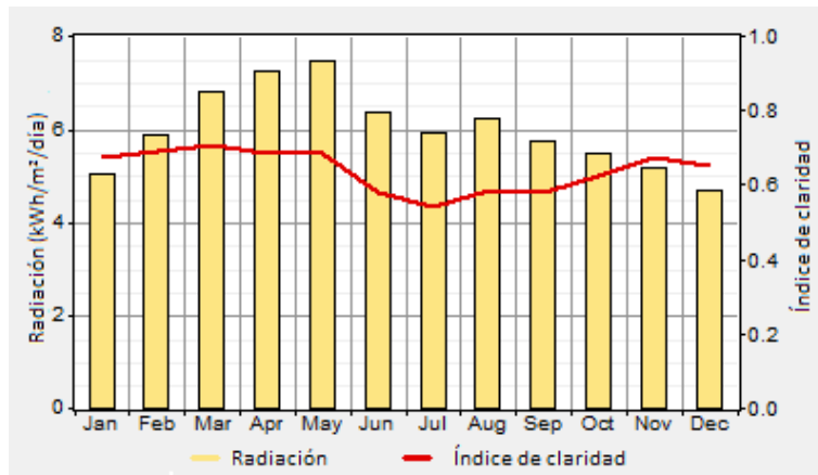
Gráfica B.7 Radiación solar e índice de claridad para el Estado de Guanajuato.
