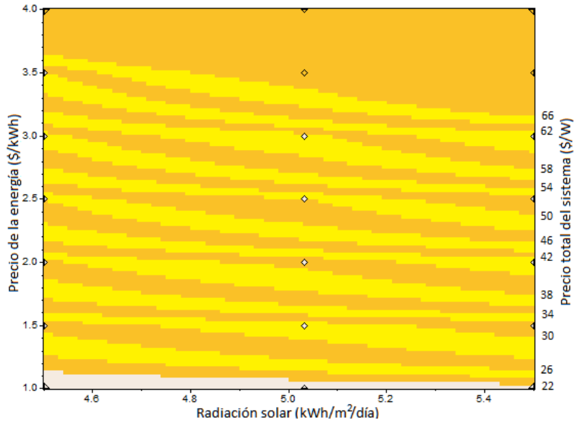
Gráfica B.12 Precios máximos del arreglo de paneles fotovoltaicos, bajo diferentes rangos de radiación solar y precios de energía eléctrica, para los cuales es rentable su instalación en Monterrey.
