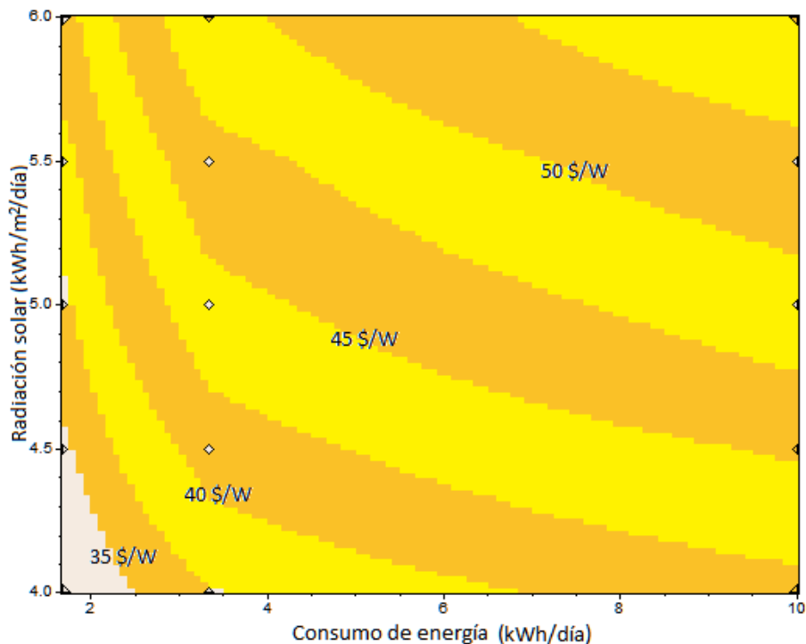
Gráfica 5.9 Precios máximos del arreglo para los cuales es rentable la instalación de paneles fotovoltaicos en Tarifa 2.
