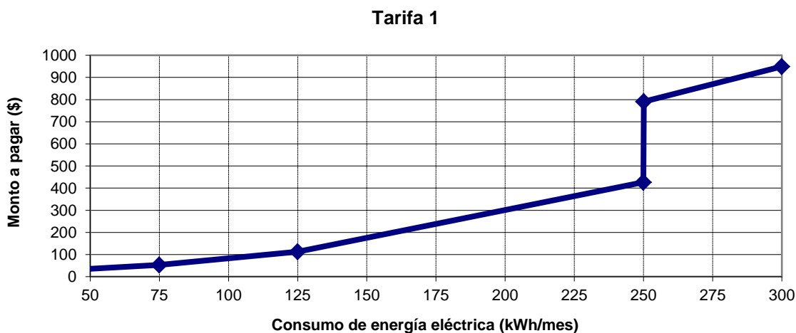
Gráfica 4.1 Monto a pagar sin IVA por la energía eléctrica consumida durante un mes para la Tarifa 1 con precios de febrero del 2011.
