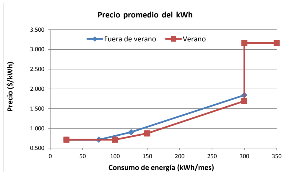
Gráfica 4.4 Precio promedio del kWh en base al consumo de energía eléctrica mensual para temporada de verano (rojo) y temporada fuera de verano (azul).
