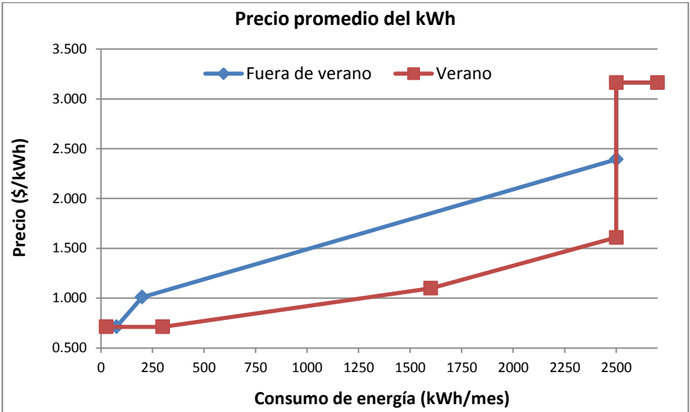
Gráfica 4.14 Precio promedio del kWh en base al consumo de energía eléctrica mensual para temporada de verano (rojo) y fuera de verano (azul).
