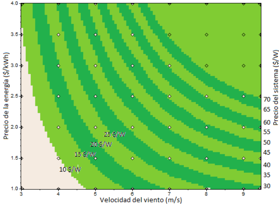
Gráfica 6.1 Precios máximos del arreglo para los cuales es rentable la instalación de aerogeneradores.
