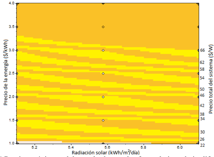
Gráfica B.24 Precios máximos del arreglo de paneles fotovoltaicos, bajo diferentes rangos de radiación solar y precios de energía eléctrica, para los cuales es rentable su instalación en Zacatecas.
