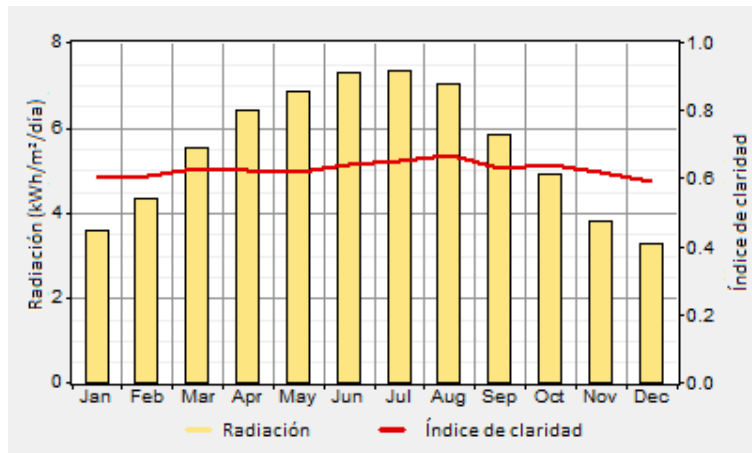
Gráfica B.15 Radiación solar e índice de claridad para el Estado de Coahuila.
