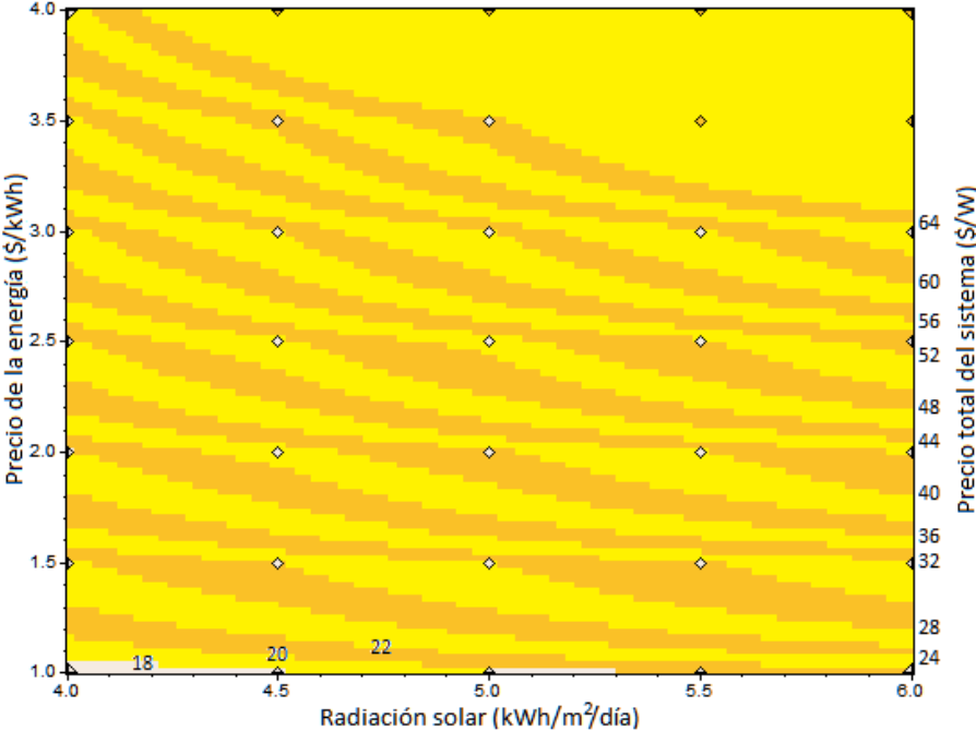
Gráfica 5.10 Precios máximos del arreglo para los cuales es rentable la instalación de paneles fotovoltaicos.
