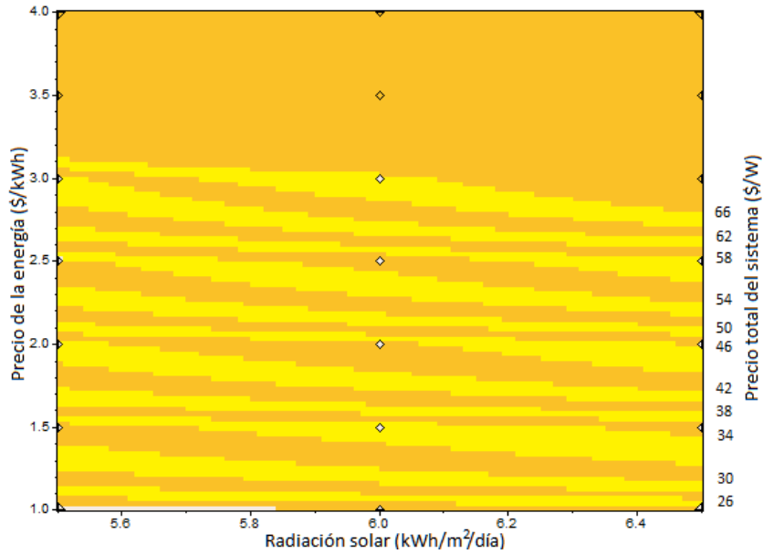
Gráfica B.8 Precios máximos del arreglo de paneles fotovoltaicos, bajo diferentes rangos de radiación solar y precios de energía eléctrica, para los cuales es rentable su instalación en Guanajuato.
