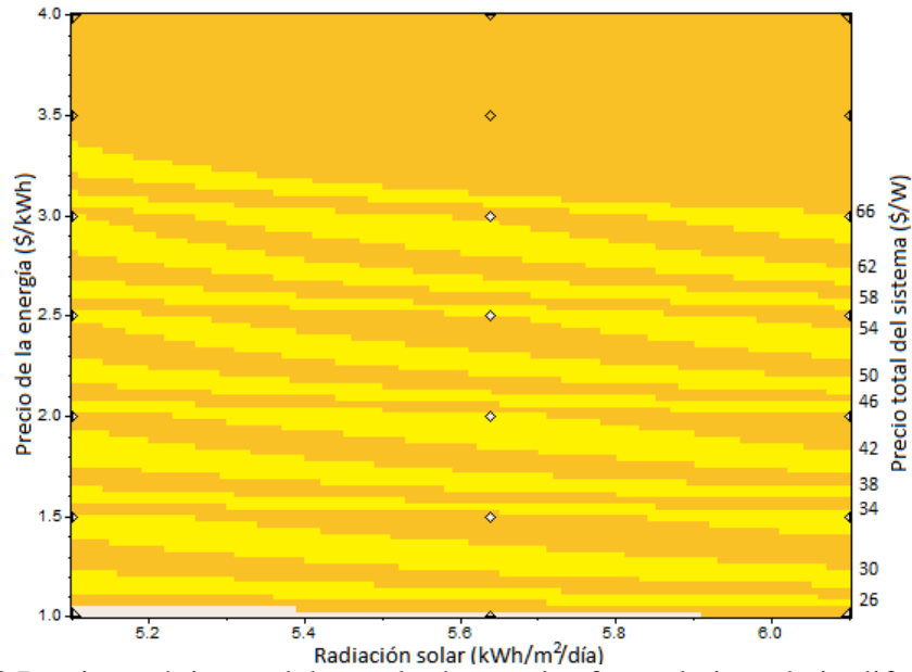
Gráfica B.18 Precios máximos del arreglo de paneles fotovoltaicos, bajo diferentes rangos de radiación solar y precios de energía eléctrica, para los cuales es rentable su instalación en San Luis Potosí.
