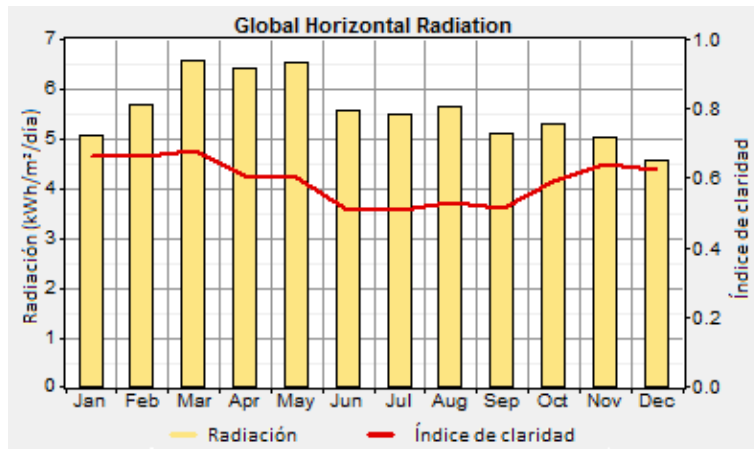
Gráfica B.9 Radiación solar e índice de claridad para el Estado de Guerrero.
