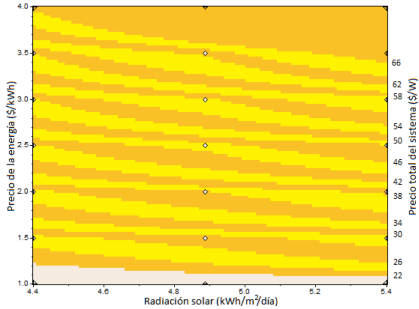
Gráfica B.22 Precios máximos del arreglo de paneles fotovoltaicos, bajo diferentes rangos de radiación solar y precios de energía eléctrica, para los cuales es rentable su instalación en Veracruz.
