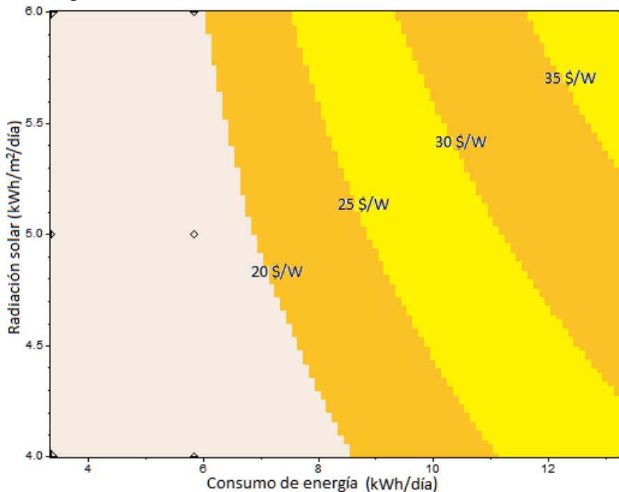
Gráfica 5.3 Precios máximos del arreglo para los cuales es rentable la instalación de paneles fotovoltaicos en casas habitación con Tarifa 1B.
