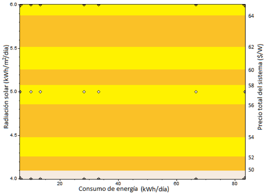
Gráfica 5.8 Precios máximos del arreglo para los cuales es rentable la instalación de paneles fotovoltaicos en casas habitación con Tarifa DAC.
