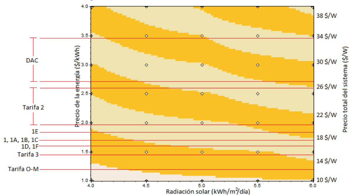
Gráfica C.3 Precios máximos del arreglo para los cuales es rentable la instalación de paneles fotovoltaicos con una TREMA=18%.
