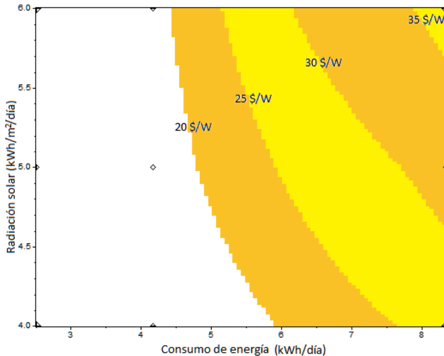
Gráfica 5.1 Precios máximos del arreglo para los cuales es rentable la instalación de paneles fotovoltaicos en casas habitación con Tarifa 1.
