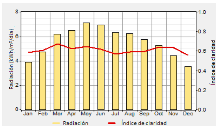
Gráfica B.23 Radiación solar e índice de claridad para el Estado de Zacatecas.
