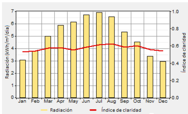
Gráfica B.11 Radiación solar e índice de claridad para el Estado de Monterrey.
