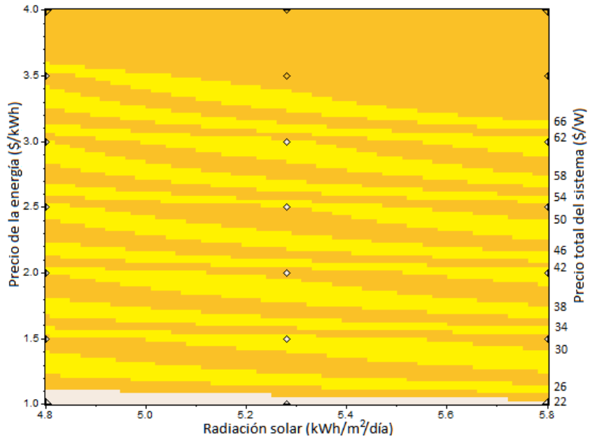
Gráfica B.4 Precios máximos del arreglo de paneles fotovoltaicos, bajo diferentes rangos de radiación solar y precios de energía eléctrica, para los cuales es rentable su instalación en Chiapas.
