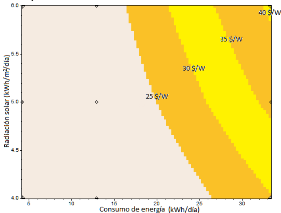
Gráfica 5.5 Precios máximos del arreglo para los cuales es rentable la instalación de paneles fotovoltaicos en casas habitación con Tarifa 1D.
