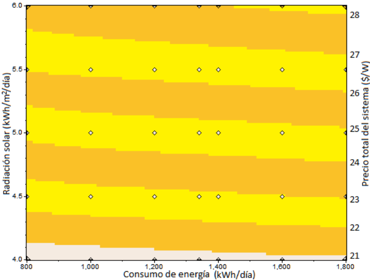
Gráfica 5.12 Precios máximos del arreglo para los cuales es rentable la instalación de paneles fotovoltaicos en el hotel.
