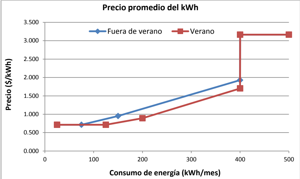
Gráfica 4.6 Precio promedio del kWh en base al consumo de energía eléctrica mensual durante temporada de verano (rojo) y temporada fuera de verano (azul).
