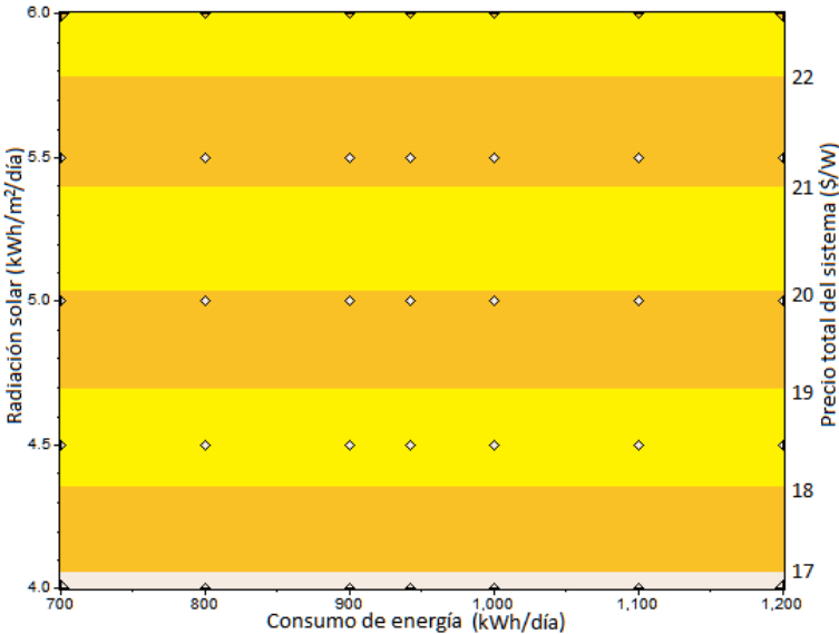
Gráfica 5.13 Precios máximos del arreglo para los cuales es rentable la instalación de paneles fotovoltaicos en el club.
