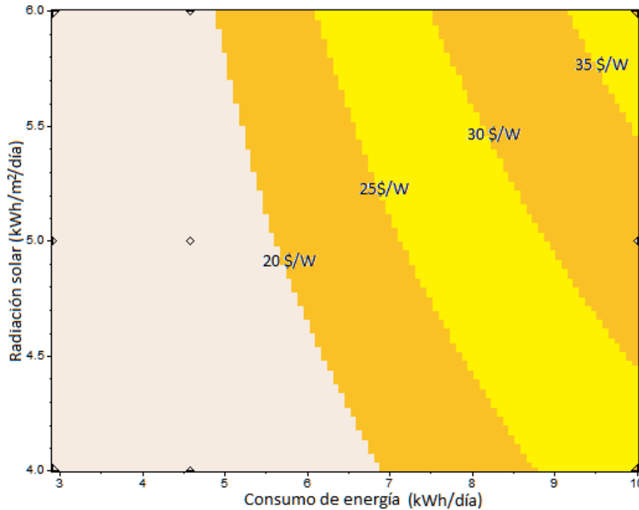
Gráfica 5.2 Precios máximos del arreglo para los cuales es rentable la instalación de paneles fotovoltaicos en casas habitación con Tarifa 1A.
