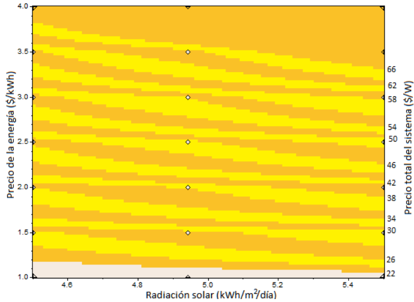
Gráfica B.2 Precios máximos del arreglo de paneles fotovoltaicos, bajo diferentes rangos de radiación solar y precios de energía eléctrica, para los cuales es rentable su instalación en Campeche.
