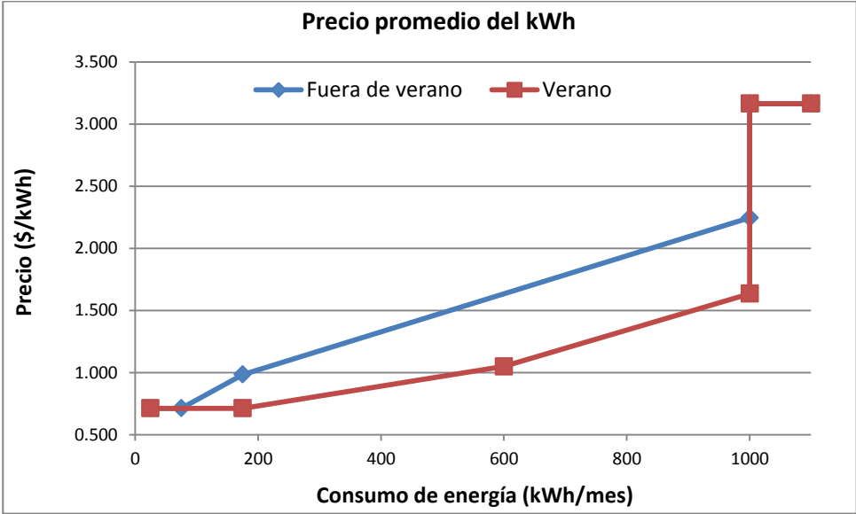
Gráfica 4.10 Precio promedio del kWh en base al consumo de energía eléctrica mensual para temporada de verano (rojo) y fuera de verano (azul).
