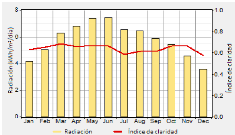
Gráfica B.5 Radiación solar e índice de claridad para el Estado de Chihuahua.
