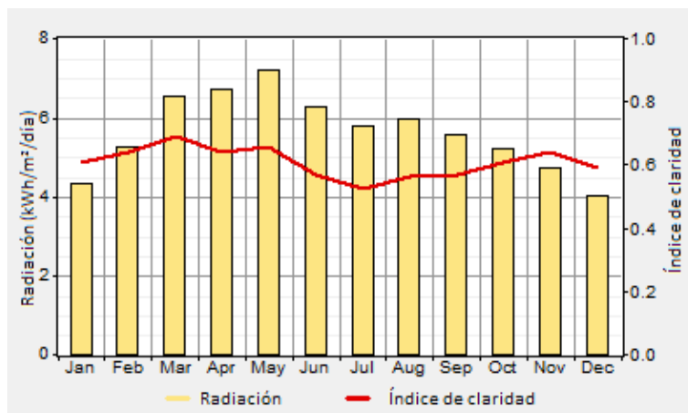
Gráfica B.17 Radiación solar e índice de claridad para el Estado de San Luis Potosí.
