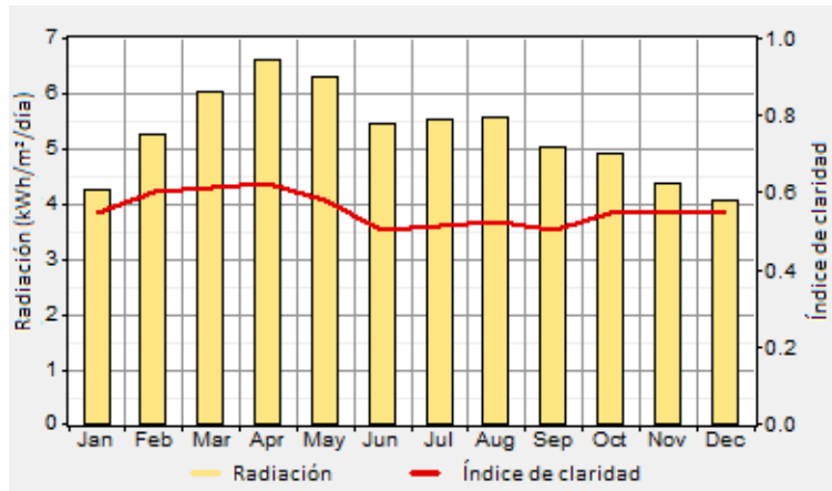
Gráfica B.3 Radiación solar e índice de claridad para el Estado de Chiapas.
