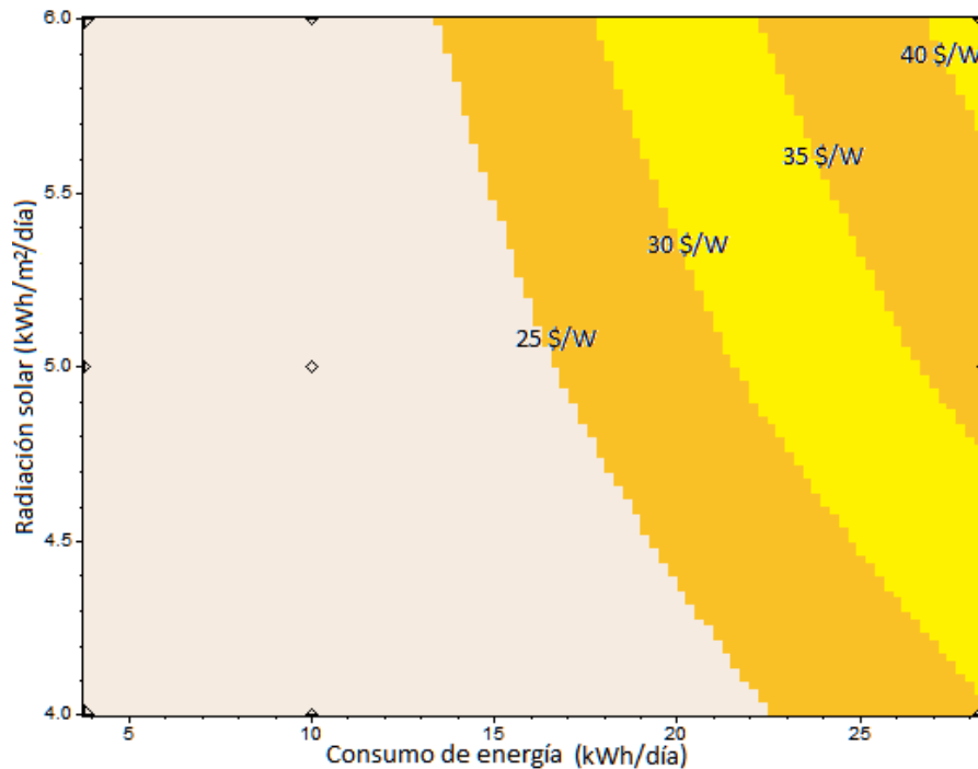
Gráfica 5.4 Precios máximos del arreglo para los cuales es rentable la instalación de paneles fotovoltaicos en casas habitación con Tarifa 1C.
