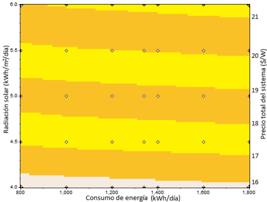
Gráfica 5.14 Precios máximos del arreglo para los cuales es rentable la instalación de paneles fotovoltaicos en el hotel.
