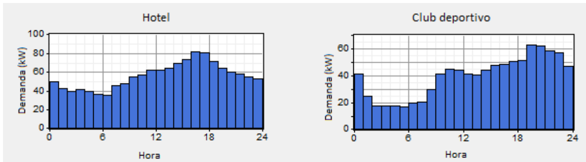
Gráfica 5.11 Curvas de demanda de electricidad para un hotel y un club deportivo
