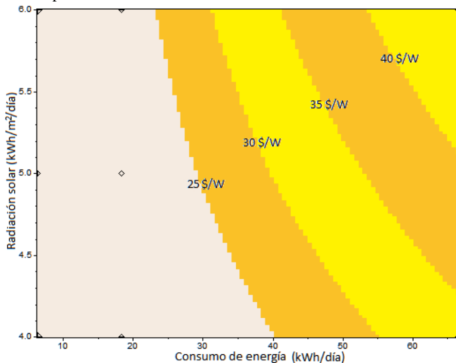
Gráfica 5.6 Precios máximos del arreglo para los cuales es rentable la instalación de paneles fotovoltaicos en casas habitación con Tarifa 1E.
