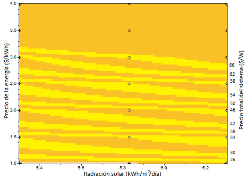
Gráfica B.14 Precios máximos del arreglo de paneles fotovoltaicos, bajo diferentes rangos de radiación solar y precios de energía eléctrica, para los cuales es rentable su instalación en Nayarit.
