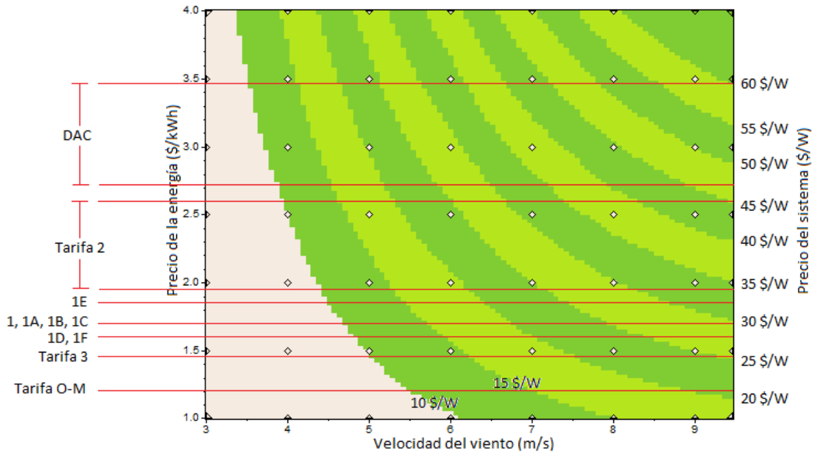
Gráfica C.4 Precios máximos del arreglo para los cuales es rentable la instalación de aerogeneradores con una TREMA=18%.
