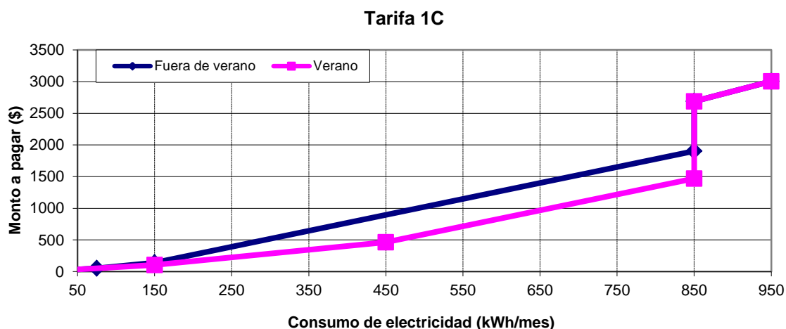
Gráfica 4.7 Comparación del monto a pagar sin IVA por la energía eléctrica consumida durante un mes en verano (rosa) y fuera de verano (azul) para la Tarifa 1C con precios de febrero del 2011.
