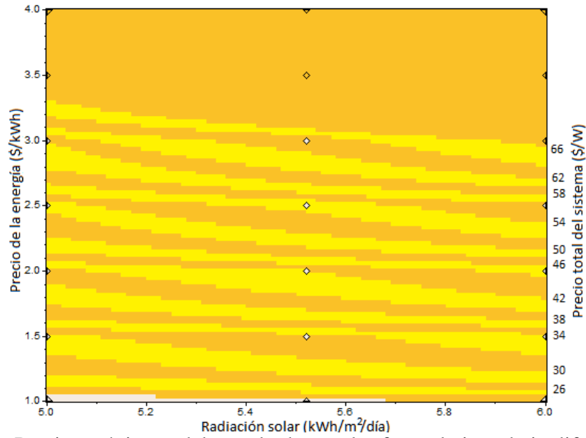
Gráfica B.16. Precios máximos del arreglo de paneles fotovoltaicos, bajo diferentes rangos de radiación solar y precios de energía eléctrica, para los cuales es rentable su instalación en Coahuila.
