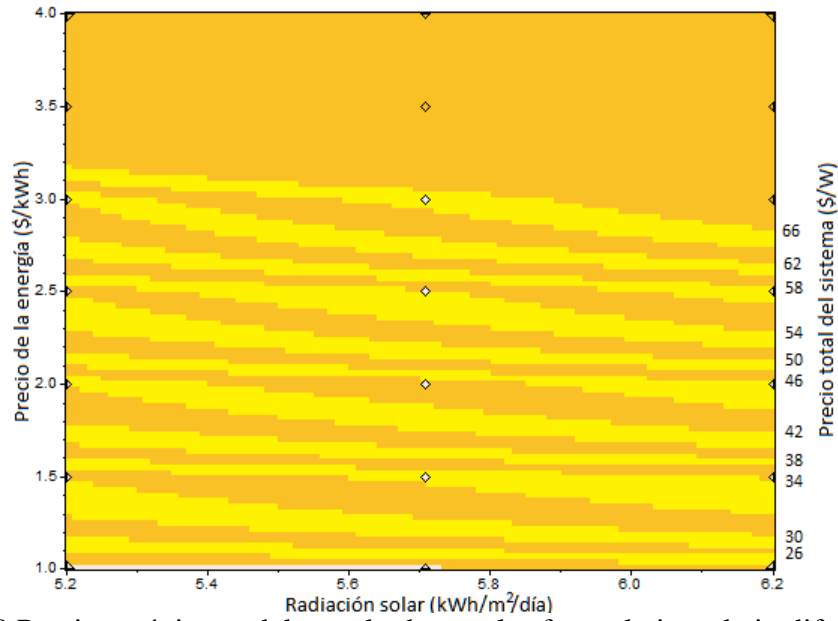
Gráfica B.20 Precios máximos del arreglo de paneles fotovoltaicos, bajo diferentes rangos de radiación solar y precios de energía eléctrica, para los cuales es rentable su instalación en Sonora.
