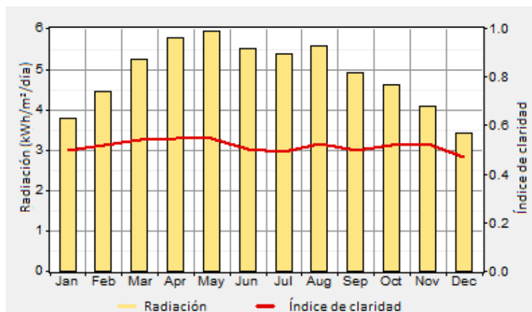
Gráfica B.21 Radiación solar e índice de claridad para el Estado de Veracruz.
