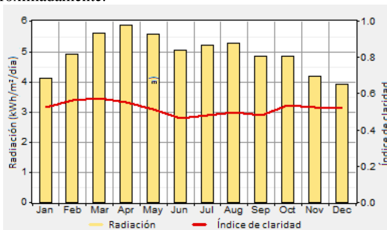
Gráfica B.1 Radiación solar e índice de claridad para el Estado de Campeche.
