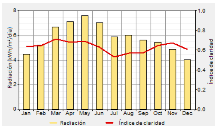
Gráfica B.13 Radiación solar e índice de claridad para el Estado de Nayarit.
