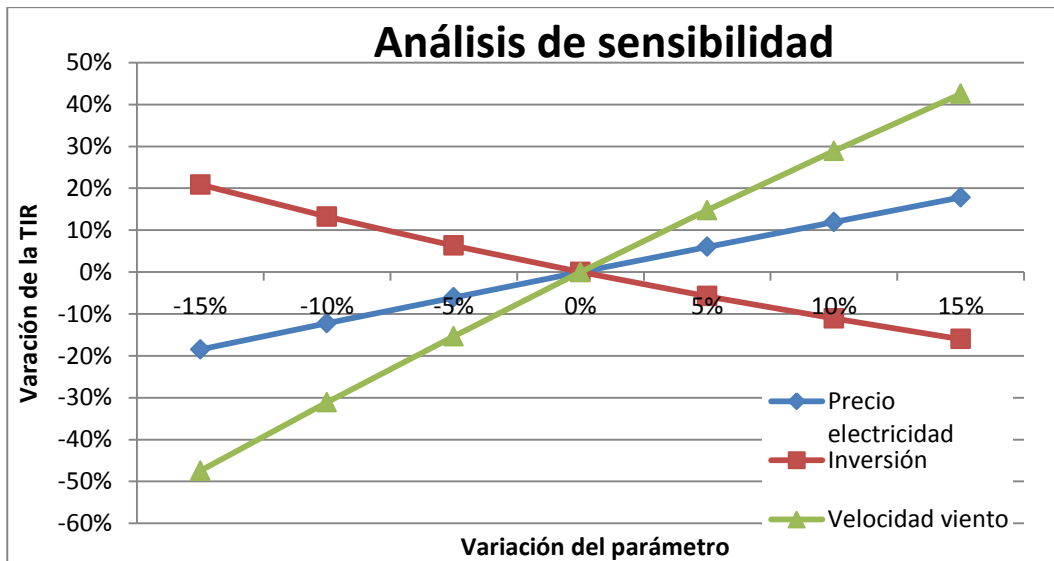
Gráfica 6.2 Análisis de sensibilidad para los aerogeneradores.
