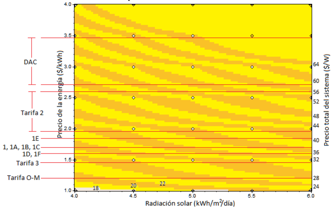
Gráfica C.1 Precios máximos del arreglo para los cuales es rentable la instalación de paneles fotovoltaicos.
