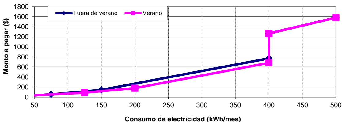
Gráfica 4.5 Comparación del monto a pagar sin IVA por la energía eléctrica consumida durante un mes en verano (rosa) y fuera de verano (azul) para la Tarifa 1B con precios de febrero del 2011.
