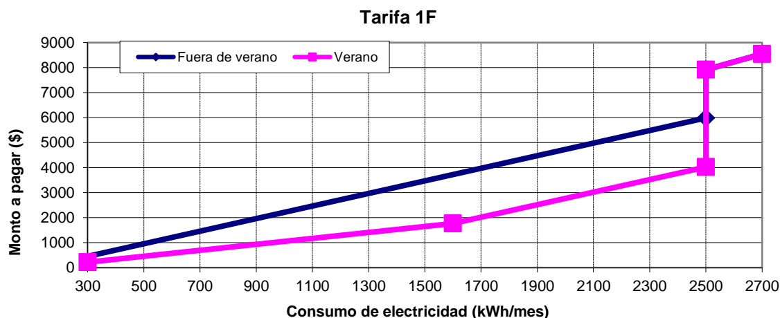
Gráfica 4.13 Comparación del monto a pagar sin IVA por la energía eléctrica consumida durante un mes en verano (rosa) y fuera de verano (azul) para la Tarifa 1F con precios de febrero del 2011.
