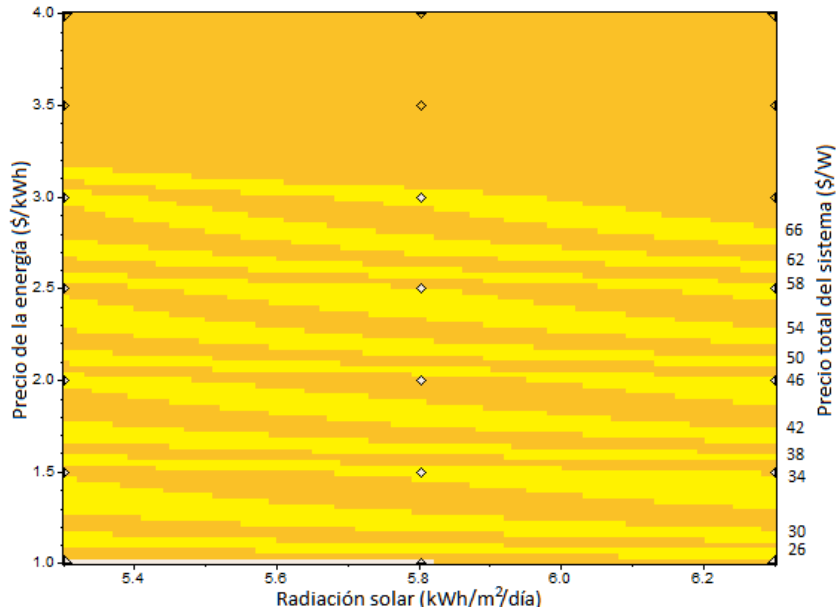
Gráfica B.6 Precios máximos del arreglo de paneles fotovoltaicos, bajo diferentes rangos de radiación solar y precios de energía eléctrica, para los cuales es rentable su instalación en Chihuahua.
