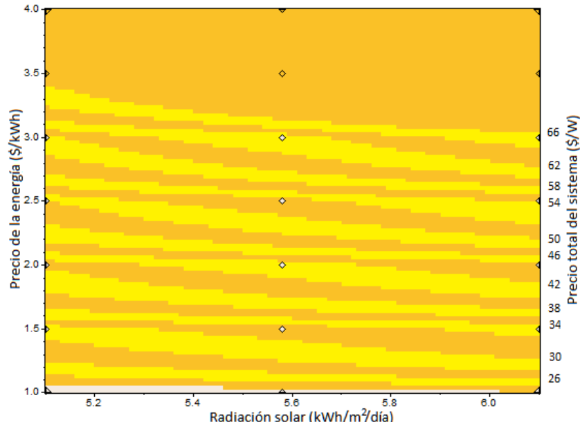
Gráfica B.10 Precios máximos del arreglo de paneles fotovoltaicos, bajo diferentes rangos de radiación solar y precios de energía eléctrica, para los cuales es rentable su instalación en Guerrero.
