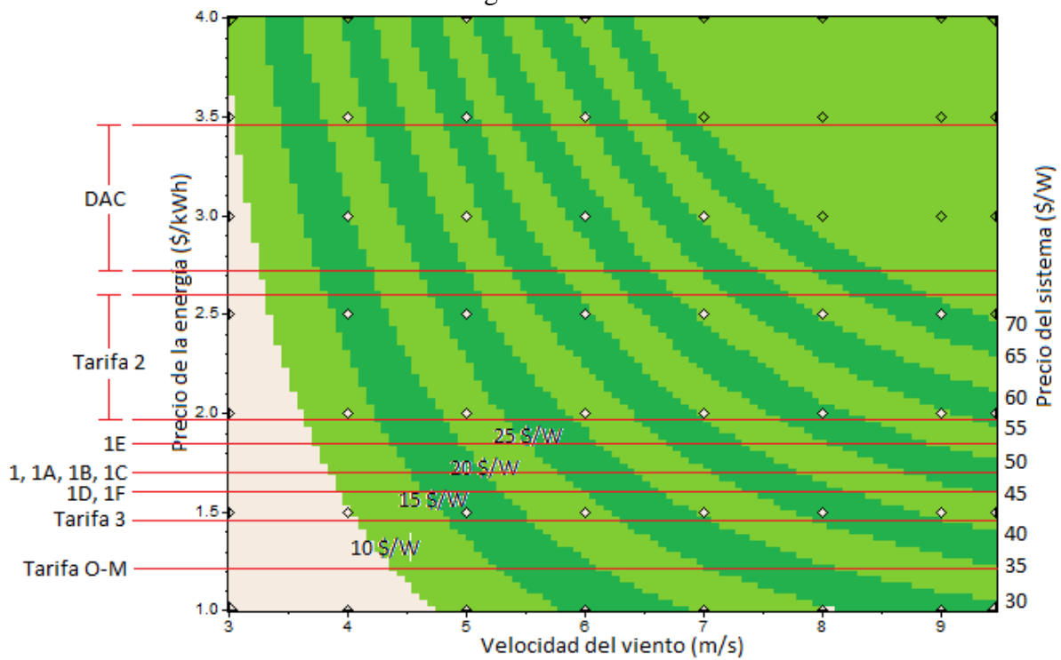
Gráfica C.2 Precios máximos del arreglo para los cuales es rentable la instalación de aerogeneradores.
