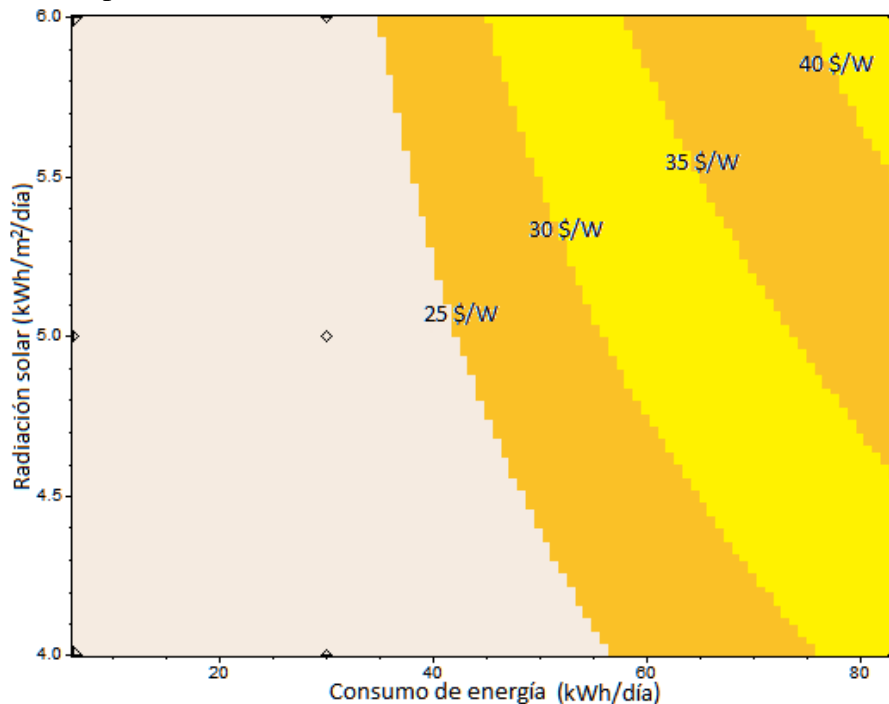
Gráfica 5.7 Precios máximos del arreglo para los cuales es rentable la instalación de paneles fotovoltaicos en casas habitación con Tarifa 1F.
