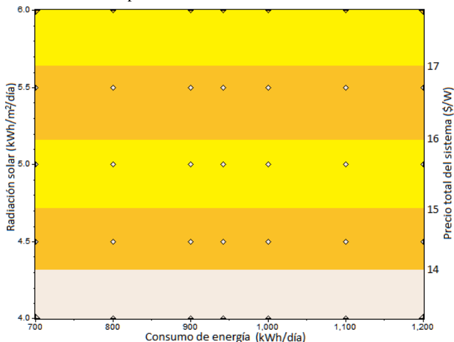
Gráfica 5.15 Precios máximos del arreglo para los cuales es rentable la instalación de paneles fotovoltaicos en el club.
