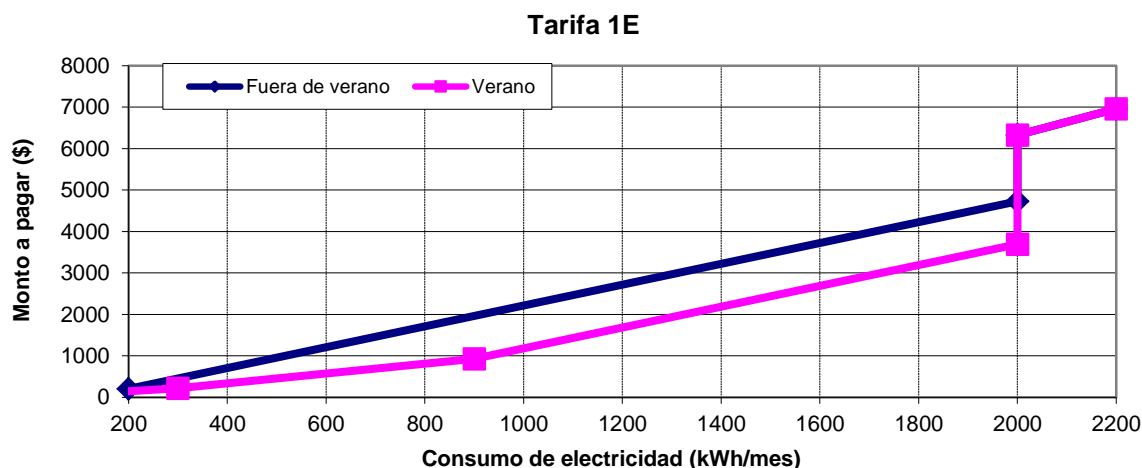
Gráfica 4.11 Comparación del monto a pagar sin IVA por la energía eléctrica consumida durante un mes en verano (rosa) y fuera de verano (azul) para la Tarifa 1E con precios de febrero del 2011.
