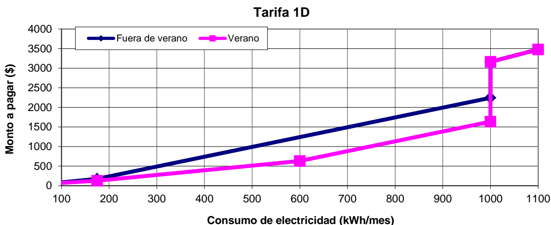
Gráfica 4.9 Comparación del monto a pagar sin IVA por la energía eléctrica consumida durante un mes en verano (rosa) y fuera de verano (azul) para la Tarifa 1D con precios de febrero del 2011.
