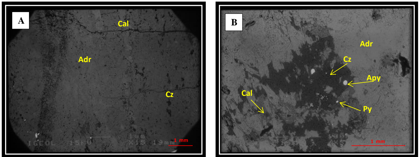
Fotografía 8. A imagen general de la muestra analizada; B se observa cristales brillantes de forma redondeada que corresponde a la arsenopirita, se observa un cristal brillante de forma anedral de grano fino al cual corresponde a una pirita, de color gris oscuro se aprecian cristales anhedrales que corresponde a un cuarzo, de color gris medio se observa una calcita de forma subhedral y de gris claro se aprecia un granate andradita
