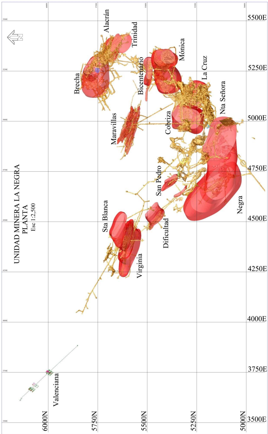
Figura 8. Plano vista en planta de los cuerpos mineralizados de la unidad minera La Negra. Escala 1 : 2,500. (Torres,2014)
