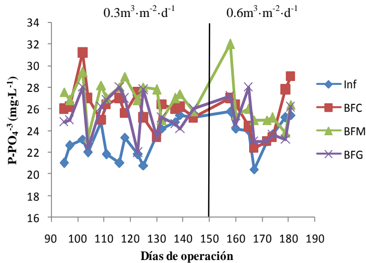
Figura 28. Comportamiento de los P-PO_4^{-3} con respecto al tiempo de operación de los biofiltros durante las etapas experimentales ( 0.3m^3 \cdot m^{-2} \cdot d^{-1} y 0.6m^3 \cdot m^{-2} \cdot d^{-1} ).
