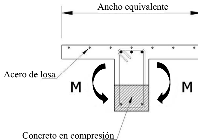
Fig 2.22c Contribución a la resistencia por momento flexionante negativo del acero de refuerzo de la losa
