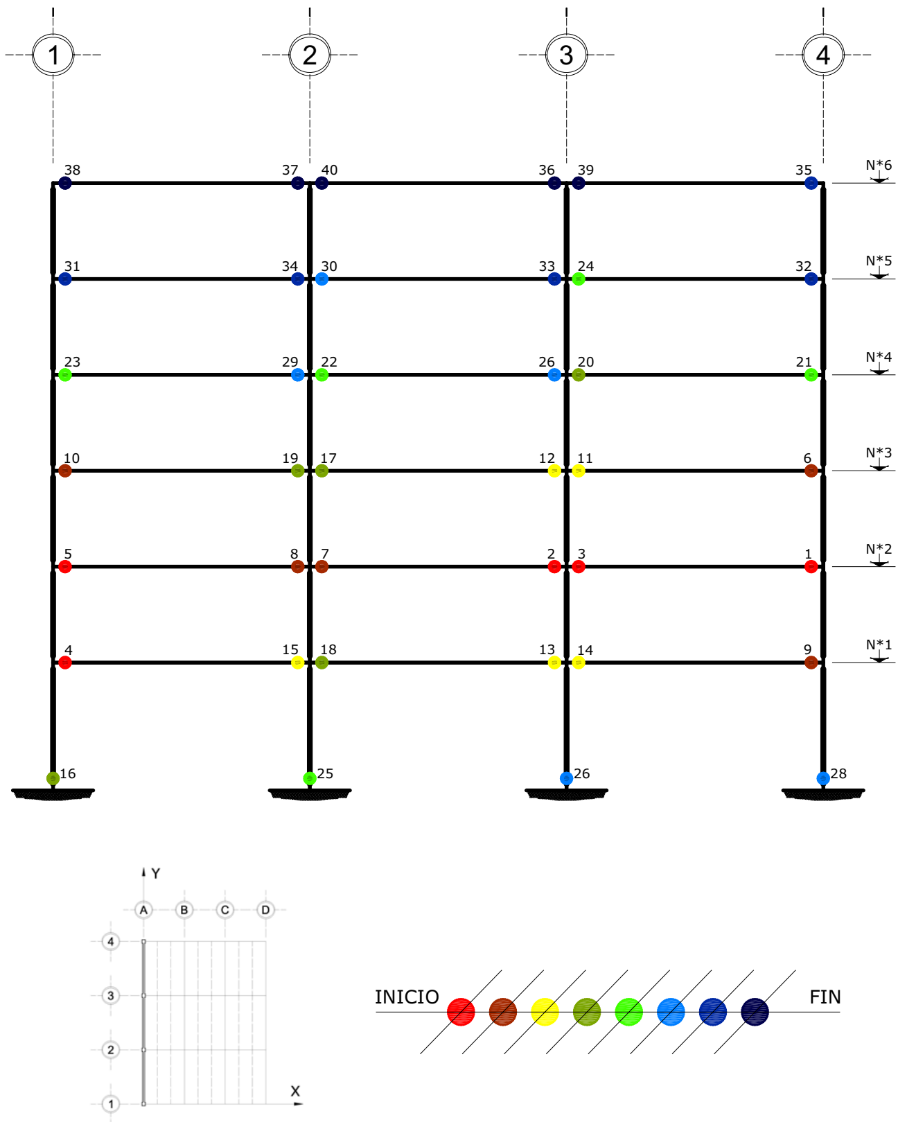
Fig 4.209 Ubicación y secuencia de formación de articulaciones plásticas, análisis Push-over, con sobre-resistencias, edificio de 6 niveles, eje A, caso D2
