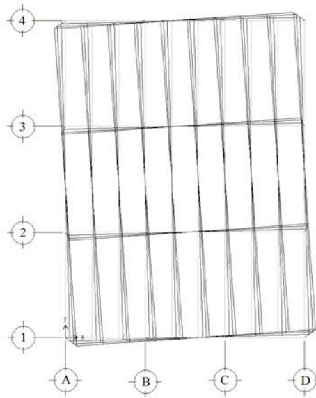
Fig 3.8 Deformada en planta del primer modo de vibración de torsión, edificio de 3 niveles
