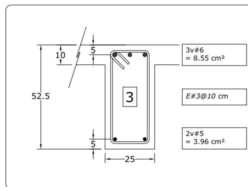
Fig 3.62 Tipos de armados de refuerzo longitudinal y transversal resultantes en los extremos de las vigas del eje A, caso B1 (Q = 4)
