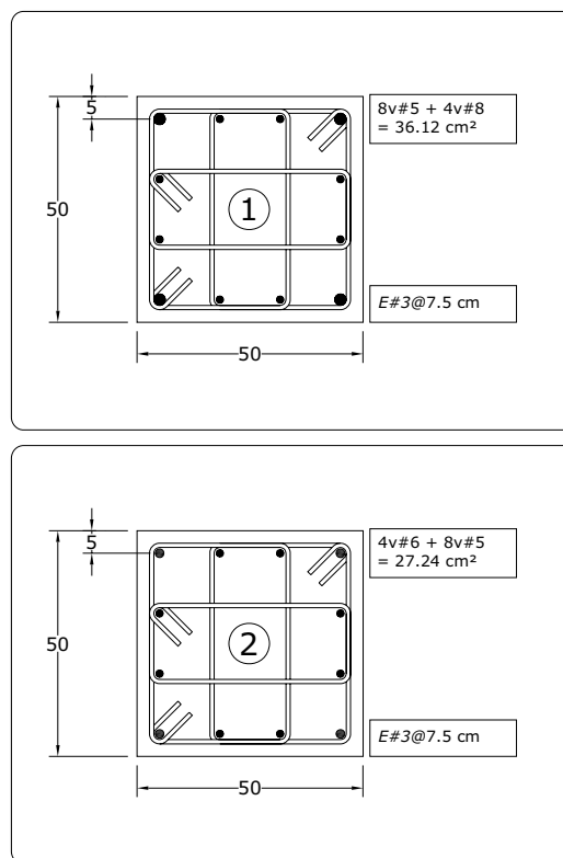
Fig 3.61 Tipos de armados de refuerzo longitudinal y transversal resultantes en los extremos de las columnas del eje 2, caso B1 ( Q = 4 )
