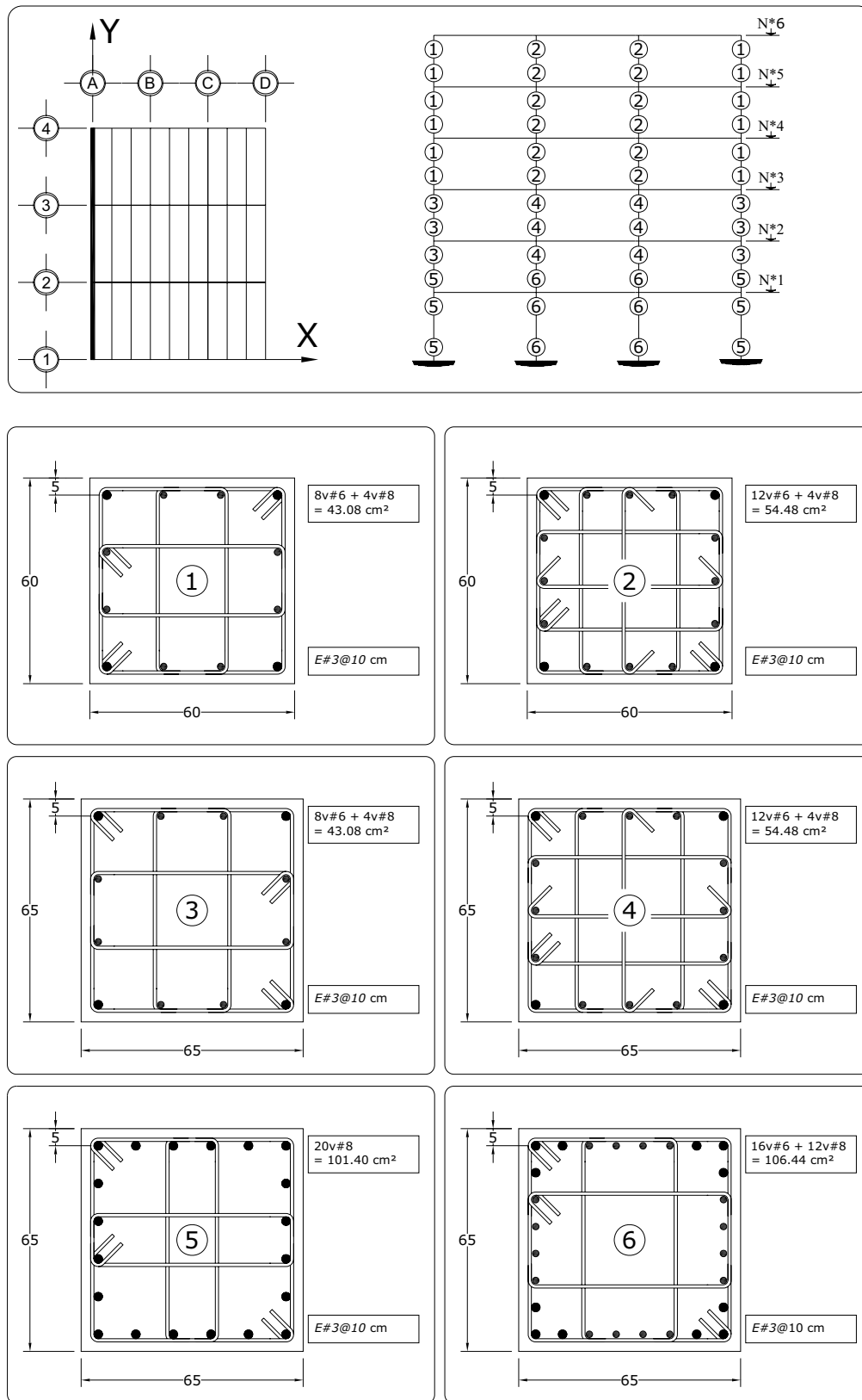
Fig 3.99 Tipos de armados de refuerzo longitudinal y transversal resultantes en los extremos de las columnas del eje A, caso C1 ( Q = 2 )
