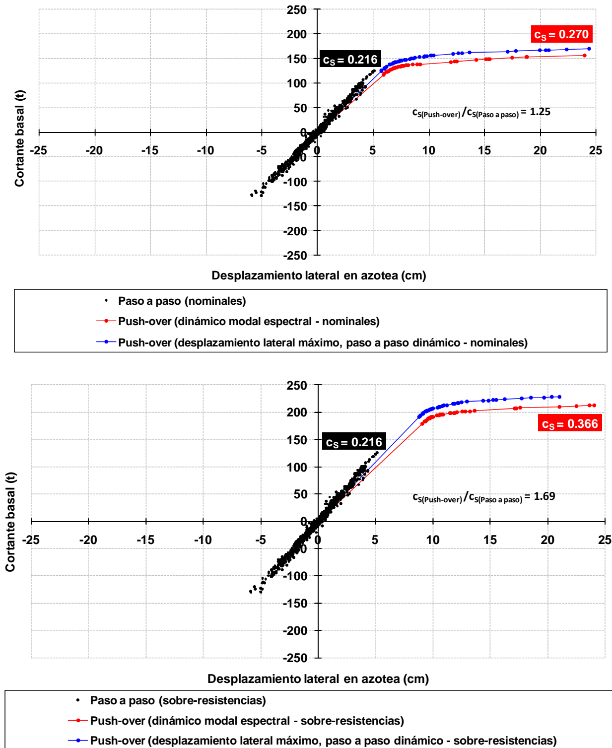
Fig 5.8 Comparación de las curvas fuerza cortante basal - desplazamiento lateral de azotea de los análisis dinámico inelástico paso a paso (con el registro SCT EW-85) y estático no-lineal Push-over (con el perfil de cargas laterales del análisis dinámico modal espectral y del dinámico inelástico paso a paso cuando ocurre el desplazamiento lateral máximo), sin y con sobre-resistencias, caso C2 del eje 2 del edificio de 6 niveles
