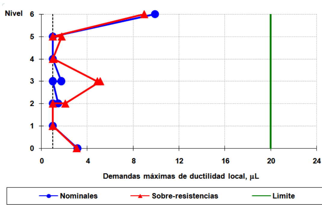
Fig 4.182 Demandas máximas de ductilidad local desarrolladas en columnas del eje 2, caso C2, análisis Push-over (sin y con sobre-resistencias), perfil de cargas laterales del análisis dinámico modal espectral, diseño Apéndice A, NTC-Sismo del RDF-04, edificio de 6 niveles
