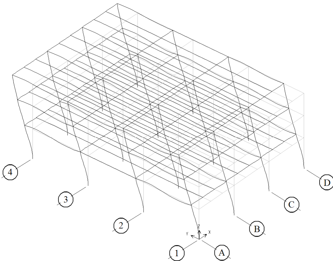
Fig 3.4 Deformada en elevación del primer modo de vibración, dirección larga, edificio de 3 niveles
