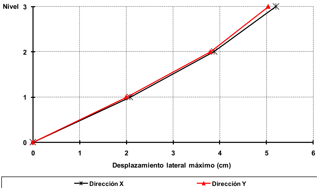
Fig 3.26 Desplazamientos laterales máximos, análisis dinámico modal espectral (rige condición de servicio), edificio de 3 niveles, caso B1 ( Q = 4 )
