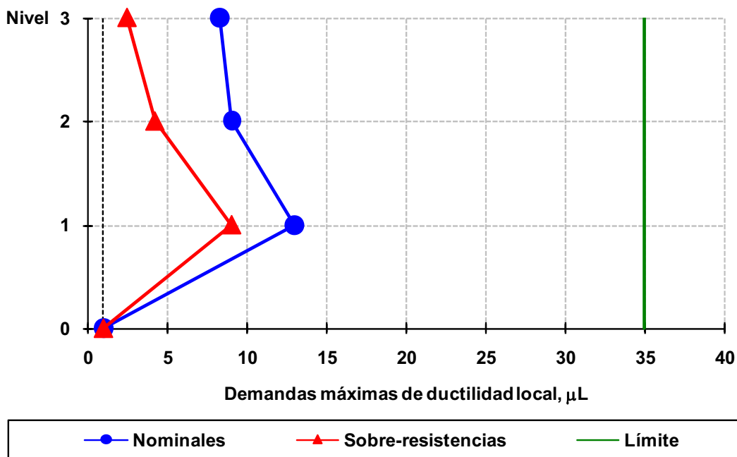
Fig 4.172 Demandas máximas de ductilidad local desarrolladas en vigas del eje 2, caso B2, análisis Push-over (sin y con sobre-resistencias), perfil de cargas laterales del análisis dinámico modal espectral, diseño Apéndice A, NTC-Sismo del RDF-04, edificio de 3 niveles
