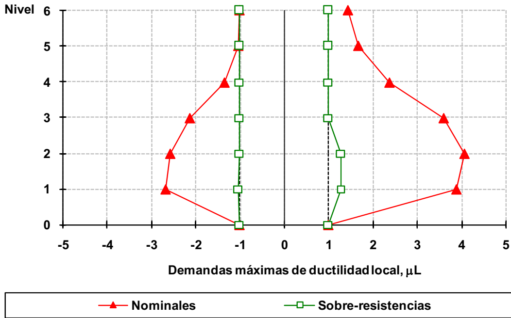
Fig 4.96 Demandas máximas de ductilidad local desarrolladas en vigas del eje 2, caso D2, análisis paso a paso elástico e inelástico (sin y con sobre-resistencias), NTC-Sismo del RDF-04, edificio de 6 niveles
