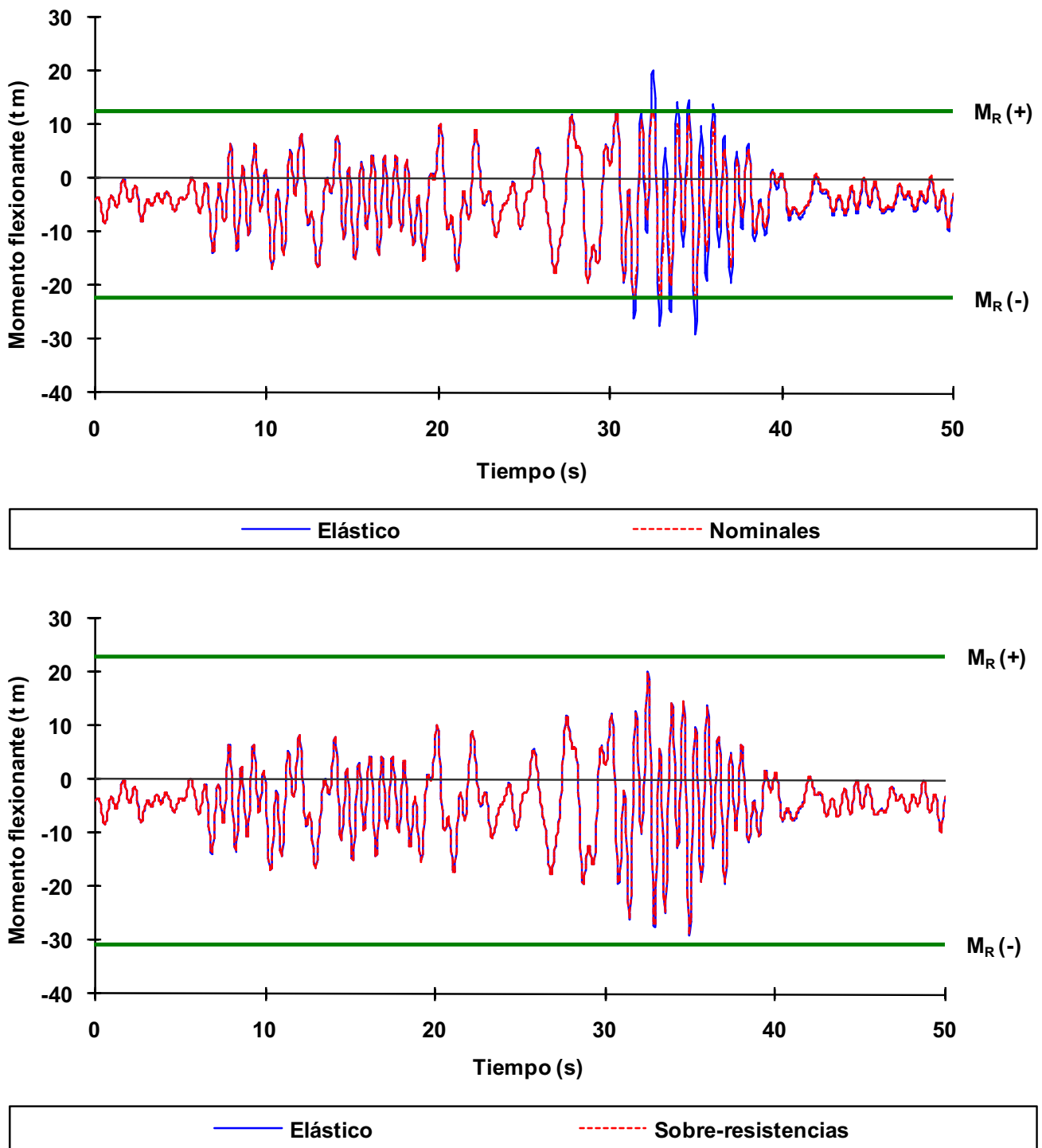
Fig 4.59 Historias de momentos flexionantes del extremo izquierdo de la viga 7 del nivel 1 del eje A, caso A2, análisis paso a paso elástico e inelástico (sin y con sobre-resistencias), diseño Apéndice A, NTC-Sismo del RDF-04, edificio de 3 niveles
