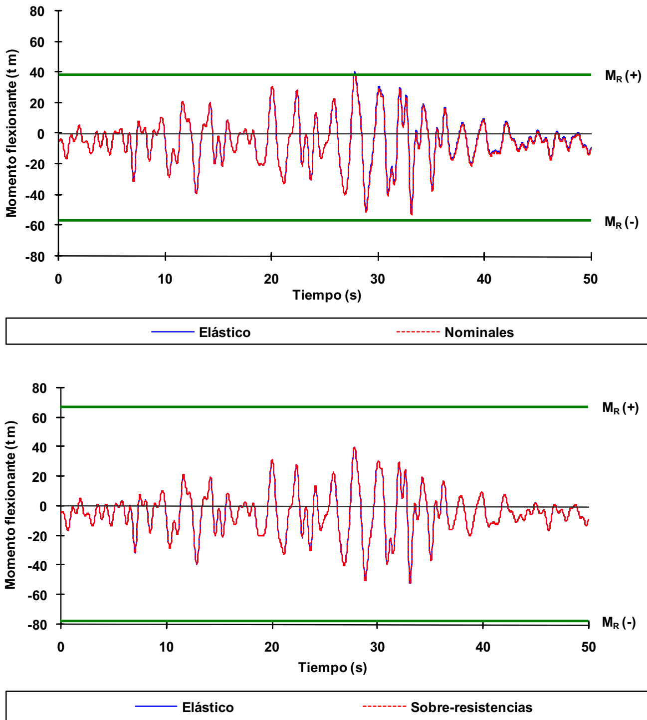
Fig 4.63 Historias de momentos flexionantes del extremo izquierdo de la viga 16 del nivel 1 del eje A, caso C2, análisis paso a paso elástico e inelástico (sin y con sobre-resistencia), diseño Apéndice A, NTC-Sismo del RDF-04, edificio de 6 niveles
