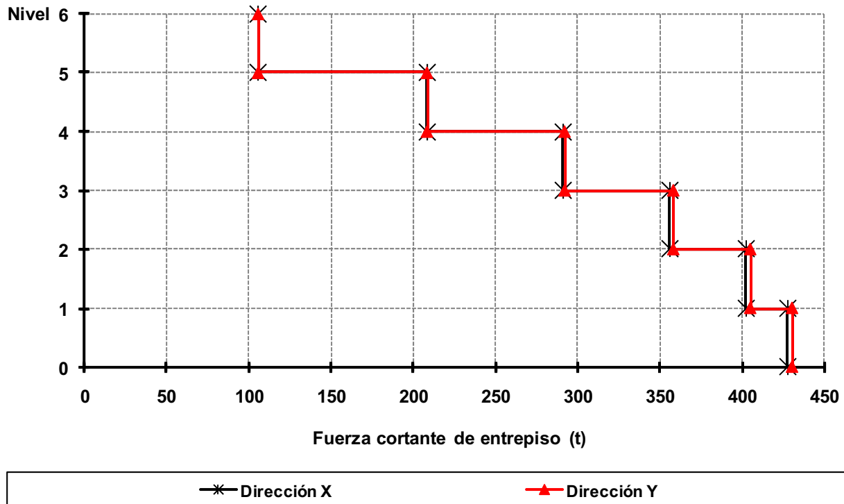
Fig 3.36 Fuerzas cortantes de entrepiso, análisis dinámico modal espectral, edificio de 6 niveles, caso C1 ( Q = 2 )
