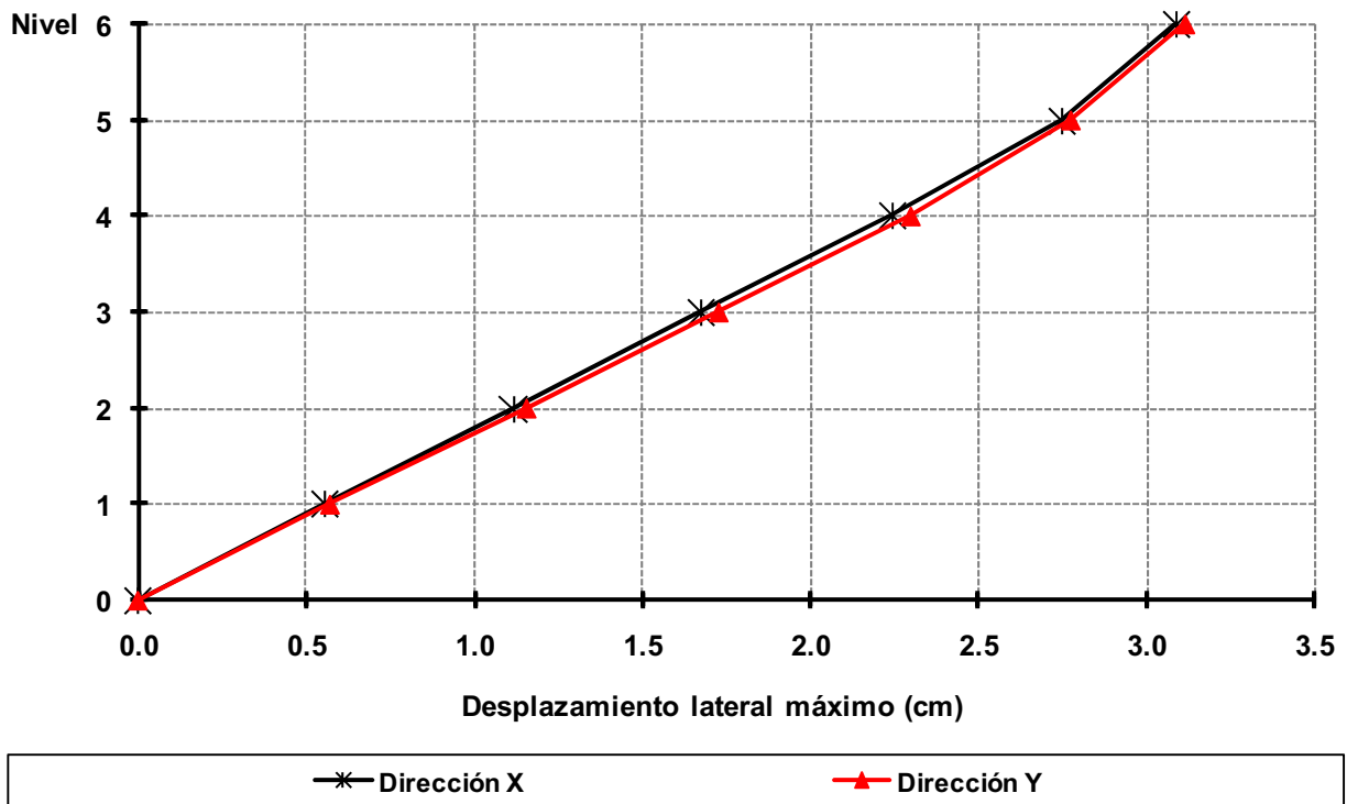
Fig 3.31a Desplazamientos laterales máximos, análisis dinámico modal espectral (condición de servicio), edificio de 6 niveles, caso D2 ( Q = 4 )
