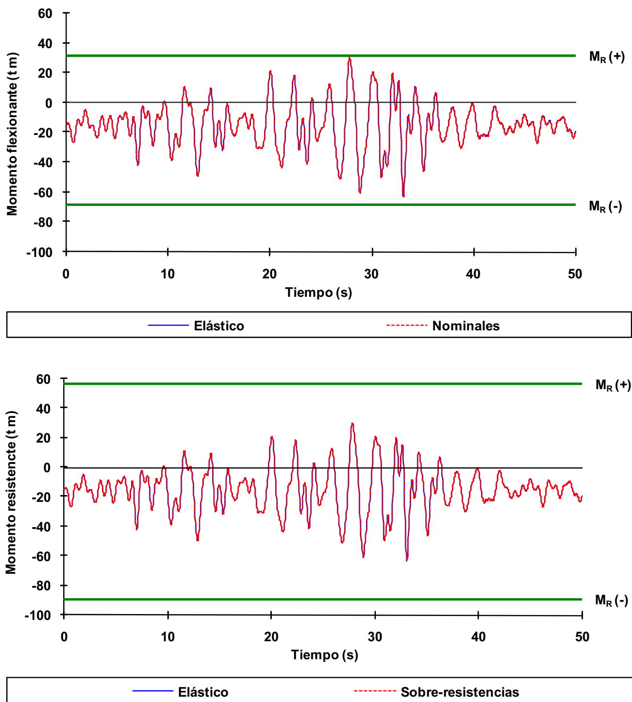
Fig 4.62 Historias de momentos flexionantes del extremo izquierdo de la viga 16 del nivel 1 del eje 2, caso C2, análisis paso a paso elástico e inelástico (sin y con sobre-resistencias), diseño Apéndice A, NTC-Sismo del RDF-04, edificio de 6 niveles
