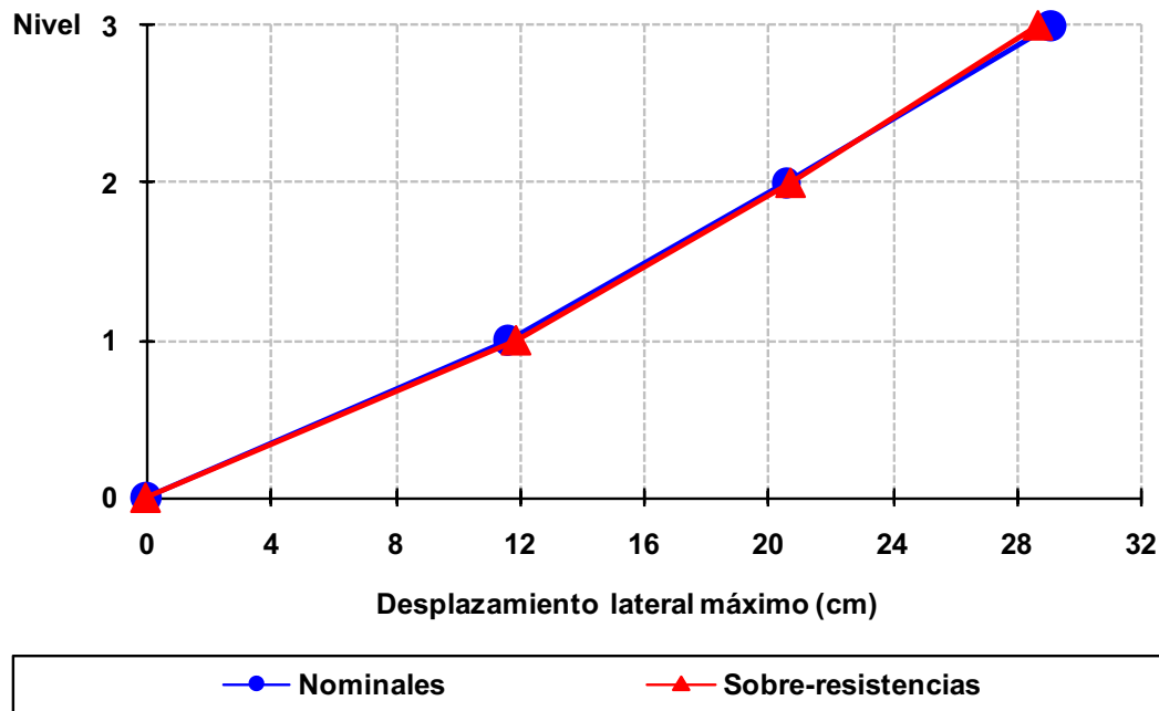
Fig 4.157 Desplazamientos laterales máximos del eje A, caso B2, análisis Push-over (sin y con sobre-resistencias), perfil de cargas laterales del análisis dinámico modal espectral, diseño Apéndice A, NTC-Sismo del RDF-04, edificio de 3 niveles
