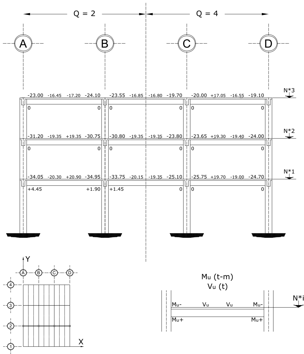
Fig 3.48 Momentos flexionantes y fuerzas cortantes últimos de vigas, eje 2, casos A1 ( Q = 2 ) y B1 ( Q = 4 )
