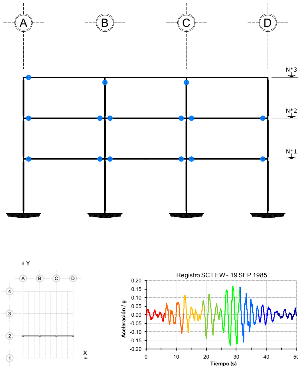
Fig 4.122 Ubicación y secuencia de formación de articulaciones plásticas, análisis paso a paso, resistencias nominales, edificio de 3 niveles, eje 2, caso A2
