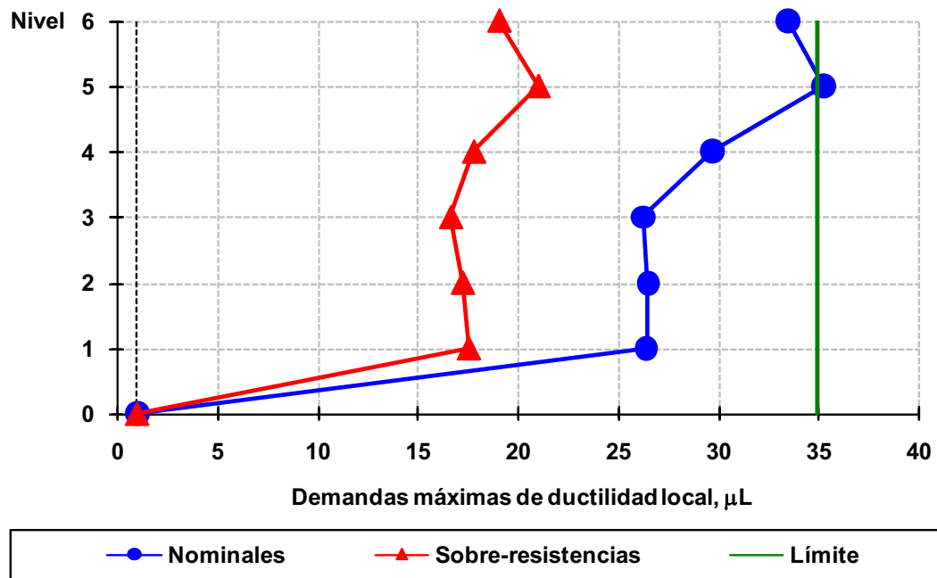
Fig 4.177 Demandas máximas de ductilidad local desarrolladas en vigas del eje A, caso D2, análisis Push-over (sin y con sobre-resistencias), perfil de cargas laterales del análisis dinámico modal espectral, diseño Apéndice A, NTC-Sismo del RDF-04, edificio de 6 niveles
