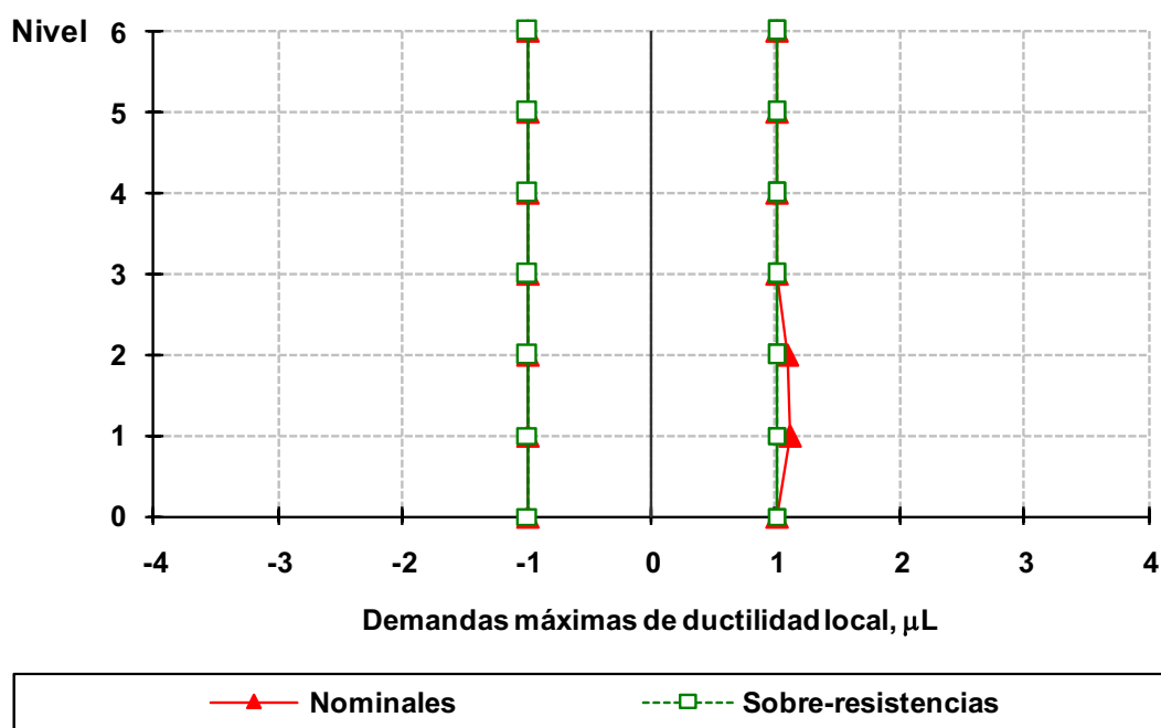
Fig 4.94 Demandas máximas de ductilidad local desarrolladas en vigas del eje 2, caso C2, análisis paso a paso elástico e inelástico (sin y con sobre-resistencias), NTC-Sismo del RDF-04, edificio de 6 niveles
