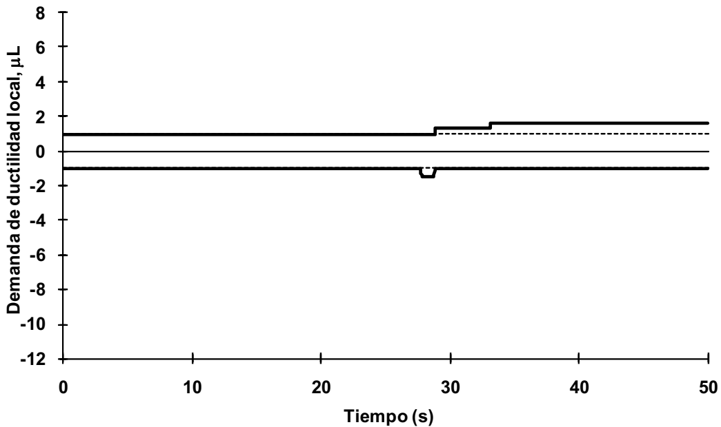
Fig 4.113 Demanda de ductilidad local desarrollada en el extremo izquierdo de la viga 16 del nivel 1, eje A, caso D2, análisis paso a paso inelástico (con sobre-resistencias), NTC-Sismo del RDF-04, edificio de 6 niveles
