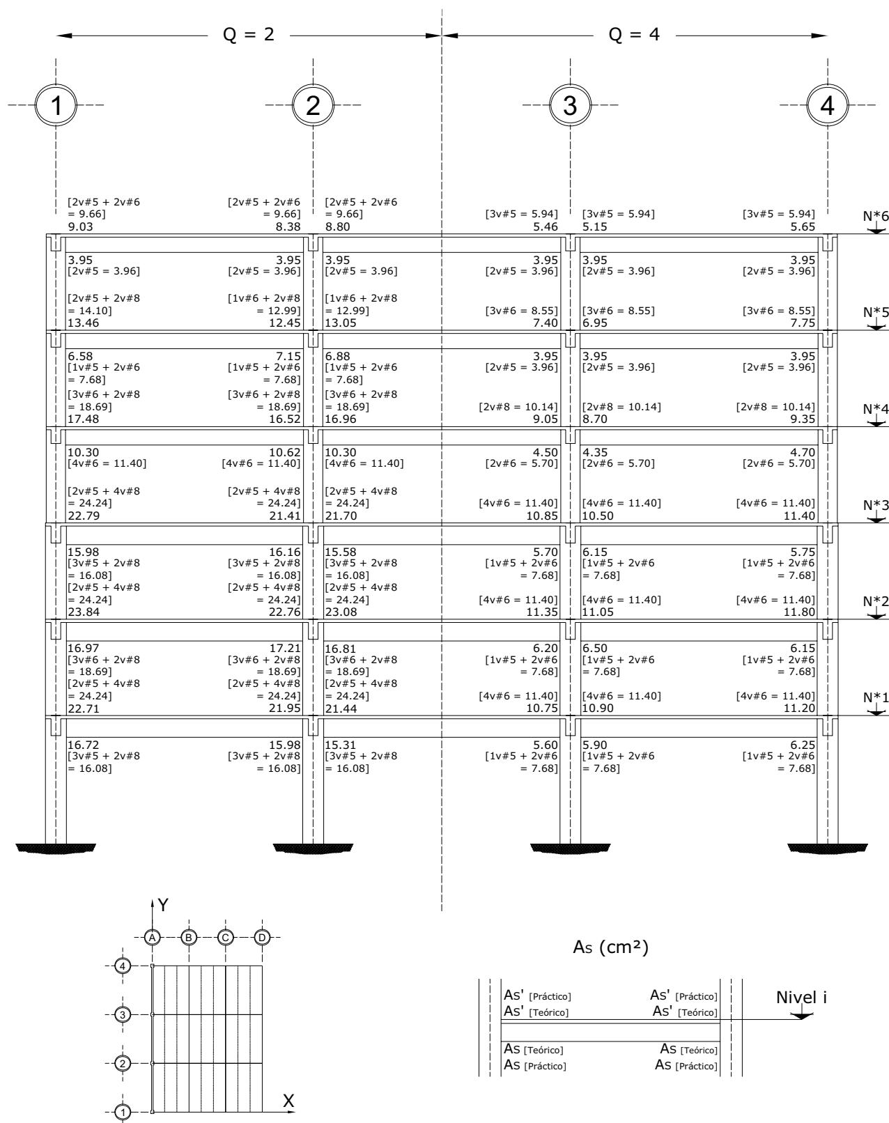
Fig 3.114 Acero de refuerzo longitudinal teórico y práctico necesario en vigas, eje A, casos C2 (Q = 2) y D2 (Q = 4)
