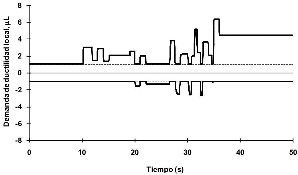
Fig 4.104 Demanda de ductilidad local desarrollada en el extremo izquierdo de la viga 7 del nivel 1, eje A, caso B2, análisis paso a paso inelástico (sin sobre-resistencias), NTC-Sismo del RDF-04, edificio de 3 niveles
