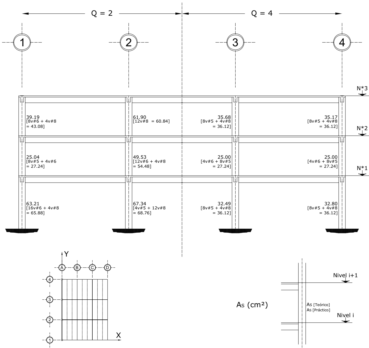
Fig 3.55a Acero de refuerzo longitudinal teórico y práctico necesario en columnas, eje A, casos A1 (Q = 2) y B1 (Q = 4)
