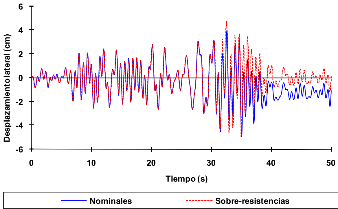
Fig 4.19 Historias de desplazamientos laterales de azotea, eje A, caso A2, análisis paso a paso elástico e inelástico (sin y con sobre-resistencias), diseño Apéndice A, NTC-Sismo del RDF-04, edificio de 3 niveles
