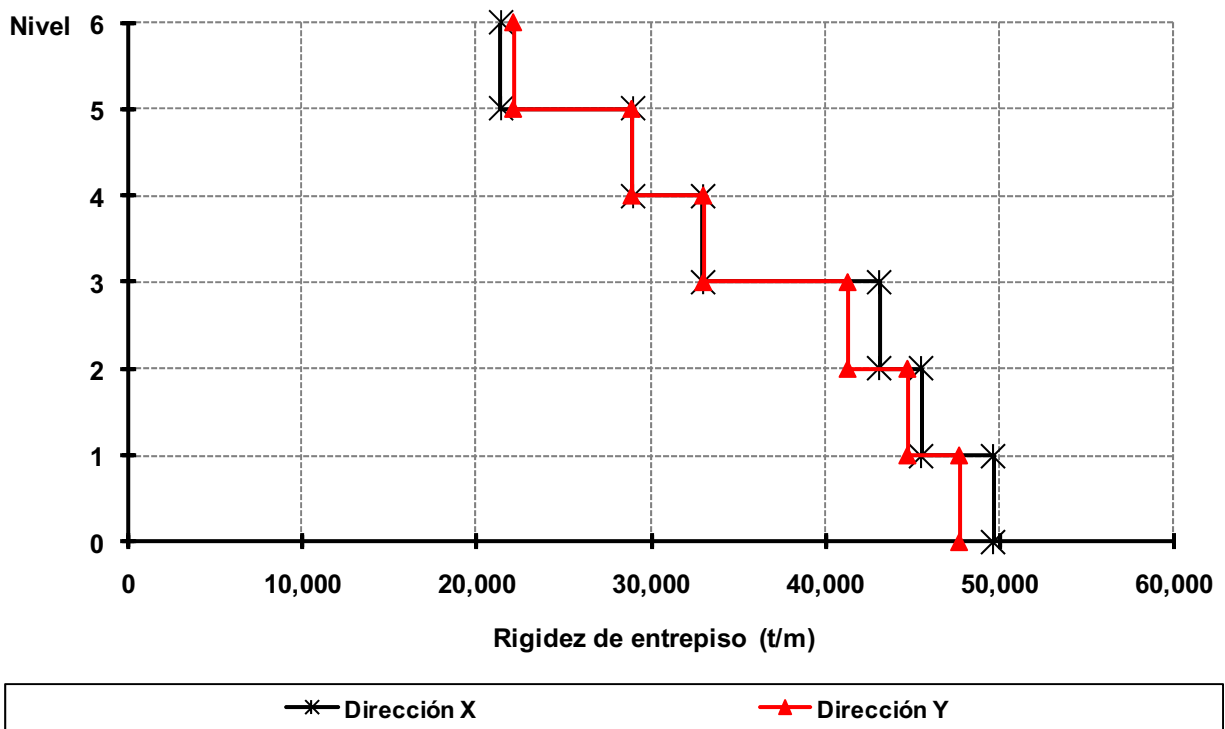
Fig 3.46 Rigideces de entrapiso, edificio 6 niveles, caso D1 (Q = 4)
