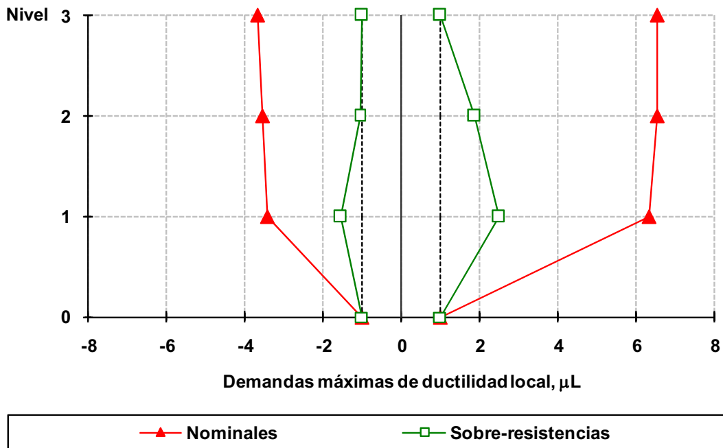
Fig 4.93 Demandas máximas de ductilidad local desarrolladas en vigas del eje A, caso B2, análisis paso a paso elástico e inelástico (sin y con sobre-resistencias), NTC-Sismo del RDF-04, edificio de 3 niveles
