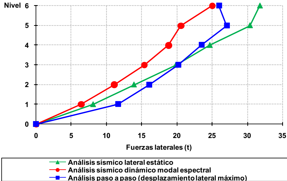
Fig 4.149 Distribución del perfil de fuerzas laterales debidas a diferentes condiciones de análisis sísmico del eje A, caso C2, (con sobre-resistencias), diseño según el Apéndice A de las NTC-Sismo del RDF-04, edificio de 6 niveles
