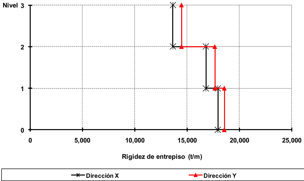
Fig 3.40 Rigideces de entrepiso, edificio 3 niveles, caso A1 (Q = 2)
