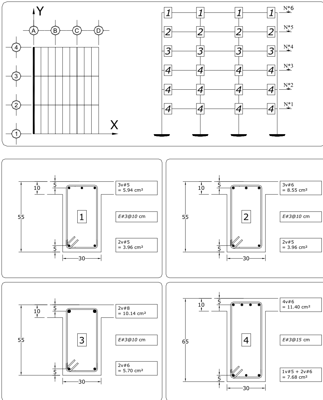
Fig 3.122 Tipos de armados de refuerzo longitudinal y transversal resultantes en los extremos de las vigas del eje A, caso D2 (Q = 4)
