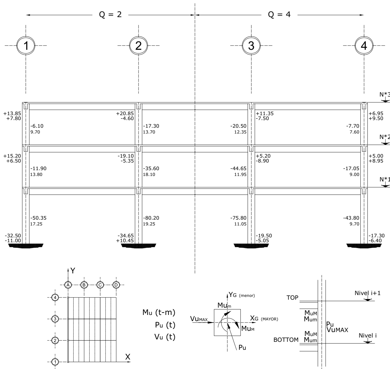
Fig 3.71 Elementos mecánicos últimos en columnas, eje A, casos A2 y B2
