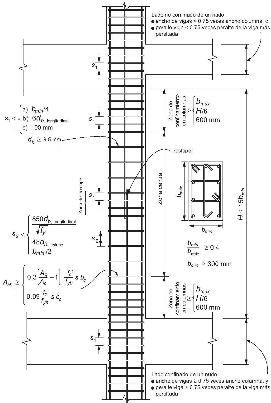
Fig 2.25 Detallado de elementos a flexocompresión de marcos dúctiles
