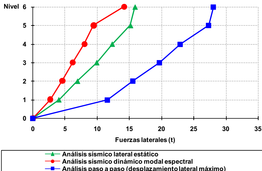
Fig 4.151 Distribución del perfil de fuerzas laterales debidas a diferentes condiciones de análisis sísmico del eje 2, caso D2, (con sobre-resistencias), diseño según el Apéndice A de las NTC-Sismo del RDF-04, edificio de 6 niveles
