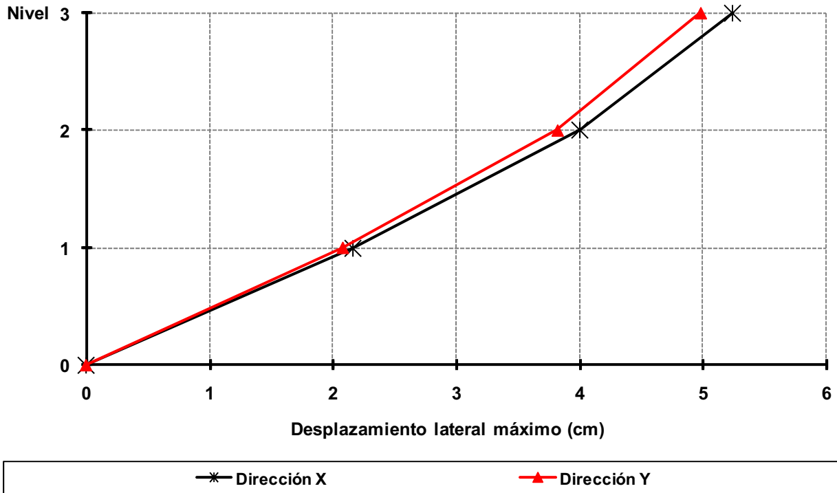
Fig 3.24 Desplazamientos laterales máximos, análisis dinámico modal espectral (rige condición de servicio), edificio de 3 niveles, caso A1 ( Q = 2 )
