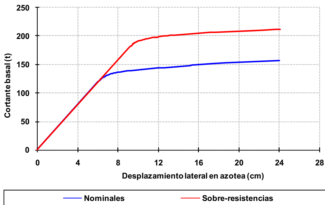
Fig 4.190 Relaciones fuerza cortante basal - desplazamiento horizontal en azotea, eje 2, caso C2, análisis Push-over (sin y con sobre-resistencias), perfil de cargas laterales del análisis dinámico modal espectral, diseño Apéndice A, NTC-Sismo del RDF-04, edificio de 6 niveles
