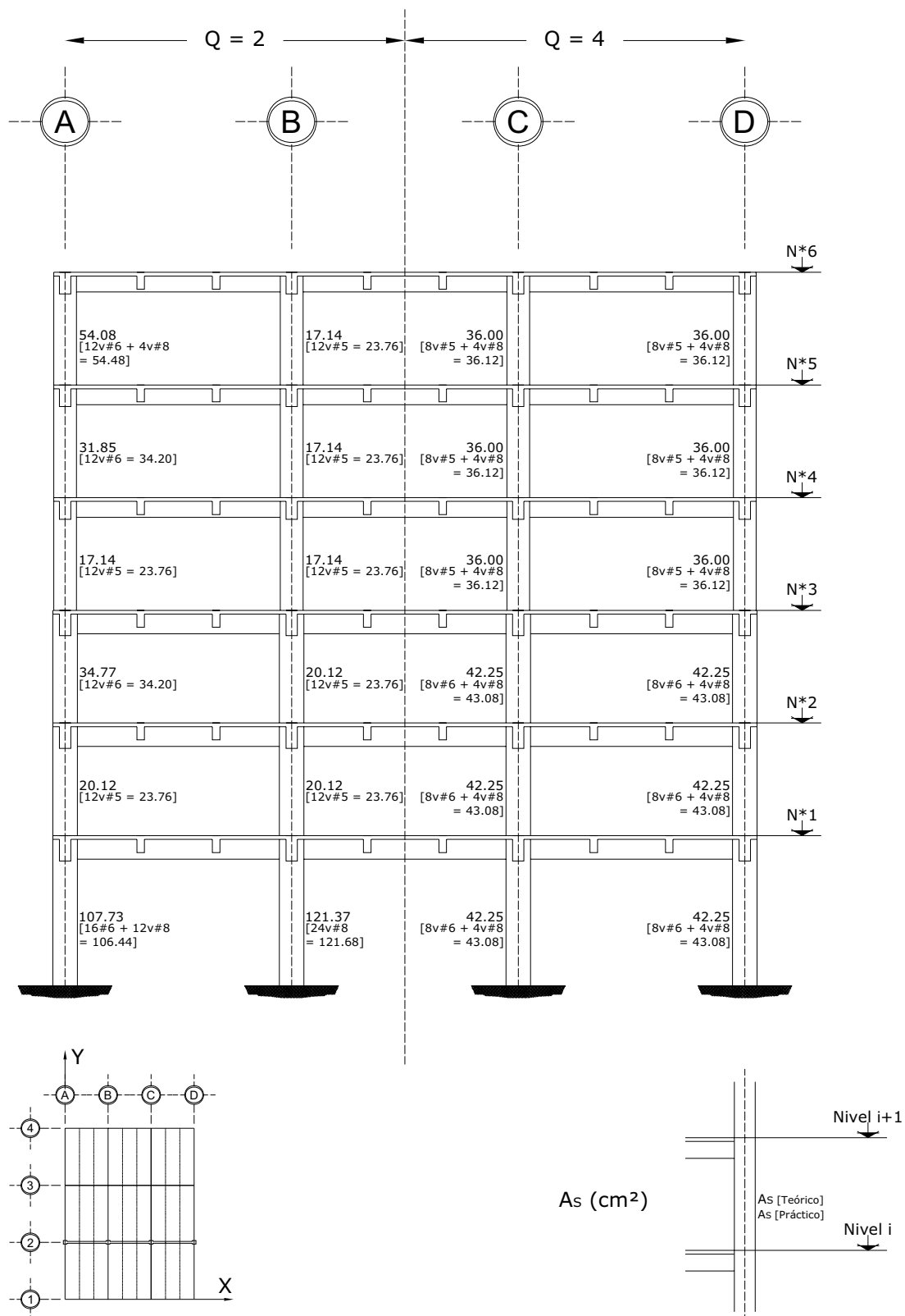
Fig 3.93a Acero de refuerzo longitudinal teórico y práctico necesario en columnas, eje 2, casos C1 (Q = 2) y D1 (Q = 4)
