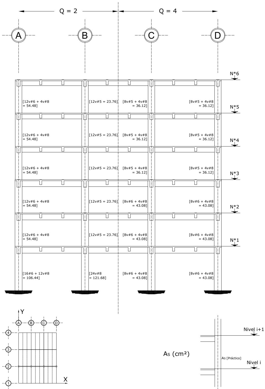
Fig 3.93b Acero de refuerzo longitudinal teórico y práctico necesario en columnas, eje 2, casos C1 ( Q = 2 ) y D1 ( Q = 4 )
