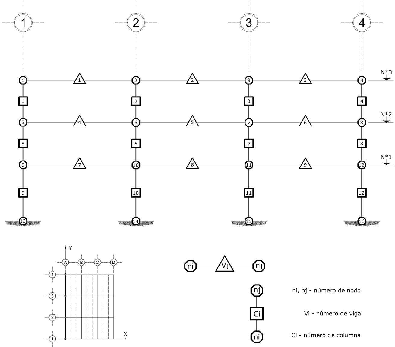
Fig 4.3 Numeración de nudos y barras en el modelo matemático bidimensional para el análisis paso a paso y el análisis tipo push-over, edificios de 3 niveles, eje A (dirección larga), casos A1 y A2 ( Q = 2 ), B1 y B2 ( Q = 4 )
