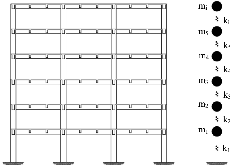
Fig 2.2 Simplificación de una estructura en un sistema de masas y resortes
