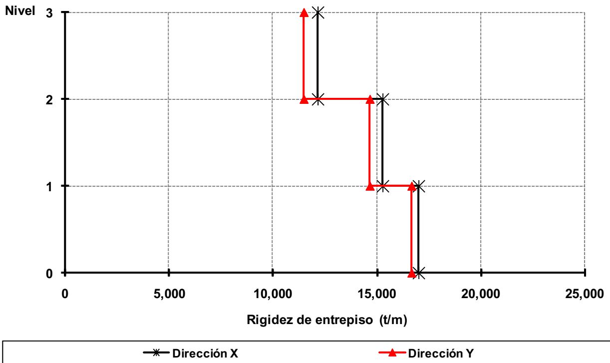
Fig 3.43 Rigideces de entrepiso, edificio 3 niveles, caso B2 (Q = 4)
