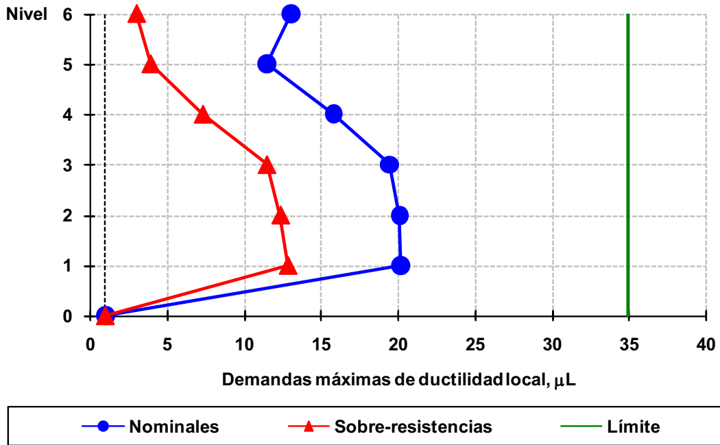
Fig 4.176 Demandas máximas de ductilidad local desarrolladas en vigas del eje 2, caso D2, análisis Push-over (sin y con sobre-resistencias), perfil de cargas laterales del análisis dinámico modal espectral, diseño Apéndice A, NTC-Sismo del RDF-04, edificio de 6 niveles
