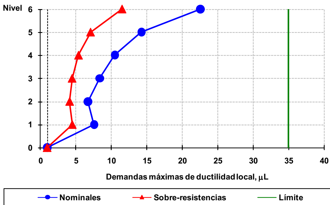
Fig 4.175 Demandas máximas de ductilidad local desarrolladas en vigas del eje A, caso C2, análisis Push-over (sin y con sobre-resistencias), perfil de cargas laterales del análisis dinámico modal espectral, diseño Apéndice A, NTC-Sismo del RDF-04, edificio de 6 niveles
