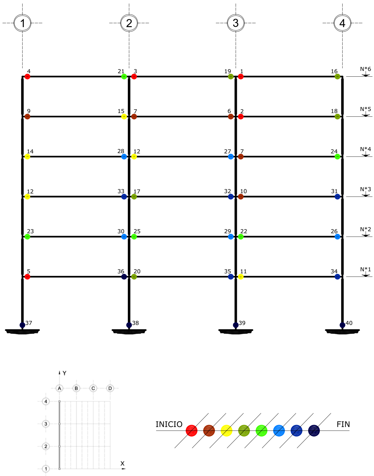
Fig 4.204 Ubicación y secuencia de formación de articulaciones plásticas, análisis Push-over, resistencias nominales, edificio de 6 niveles, eje A, caso C2
