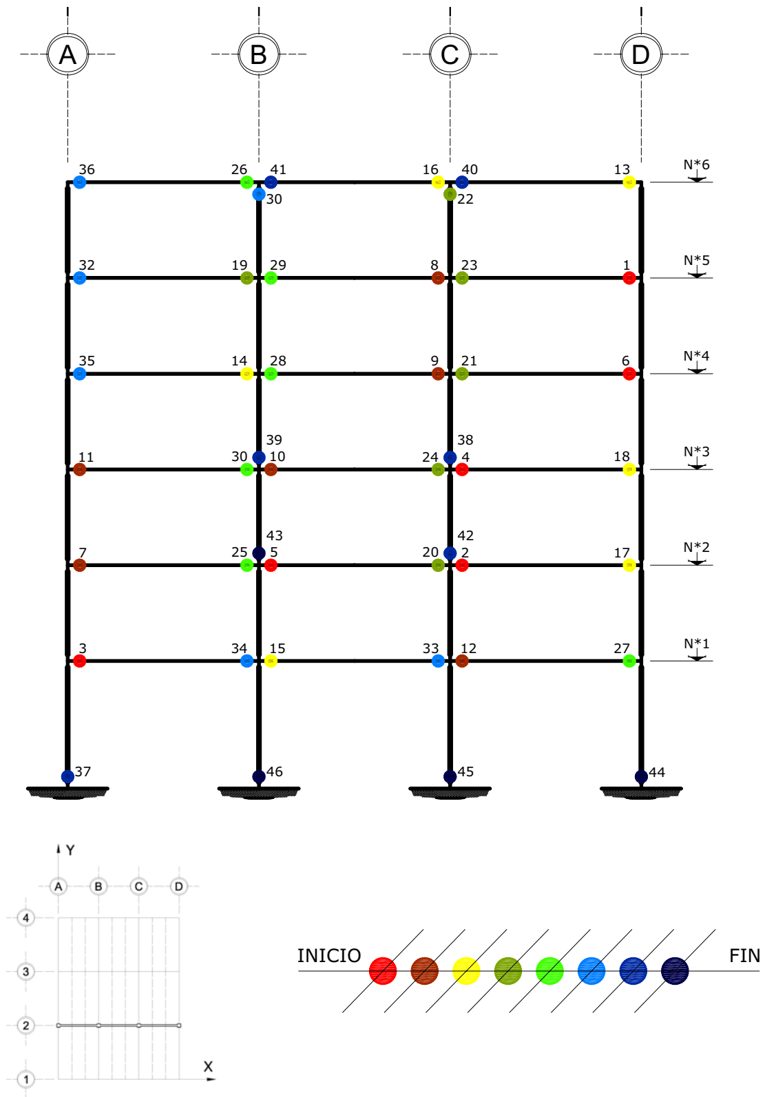
Fig 4.202 Ubicación y secuencia de formación de articulaciones plásticas, análisis Push-over, resistencias nominales, edificio de 6 niveles, eje 2, caso C2
