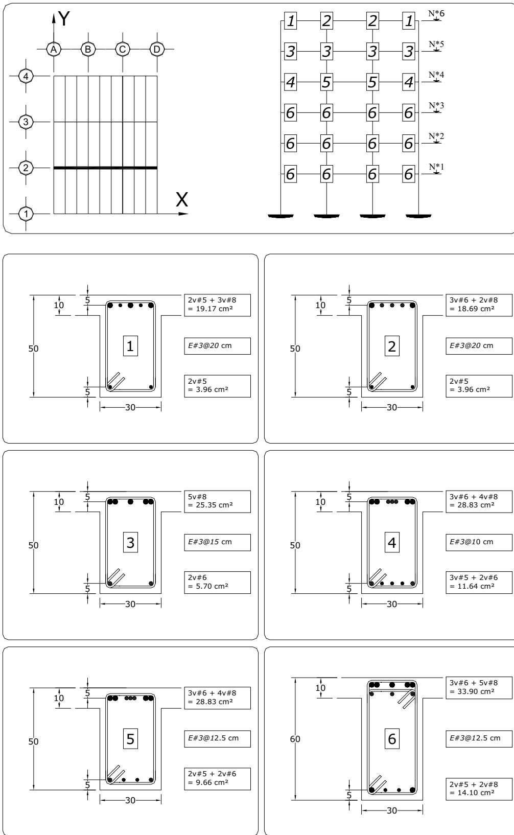
Fig 3.116 Tipos de armados de refuerzo longitudinal y transversal resultantes en los extremos de las vigas del eje 2, caso C2 (Q = 2)
