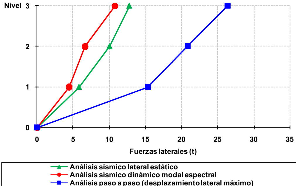
Fig 4.145 Distribución del perfil de fuerzas laterales debidas a diferentes condiciones de análisis sísmico del eje A, caso B2, (con sobre-resistencias), diseño según el Apéndice A de las NTC-Sismo del RDF-04, edificio de 3 niveles
