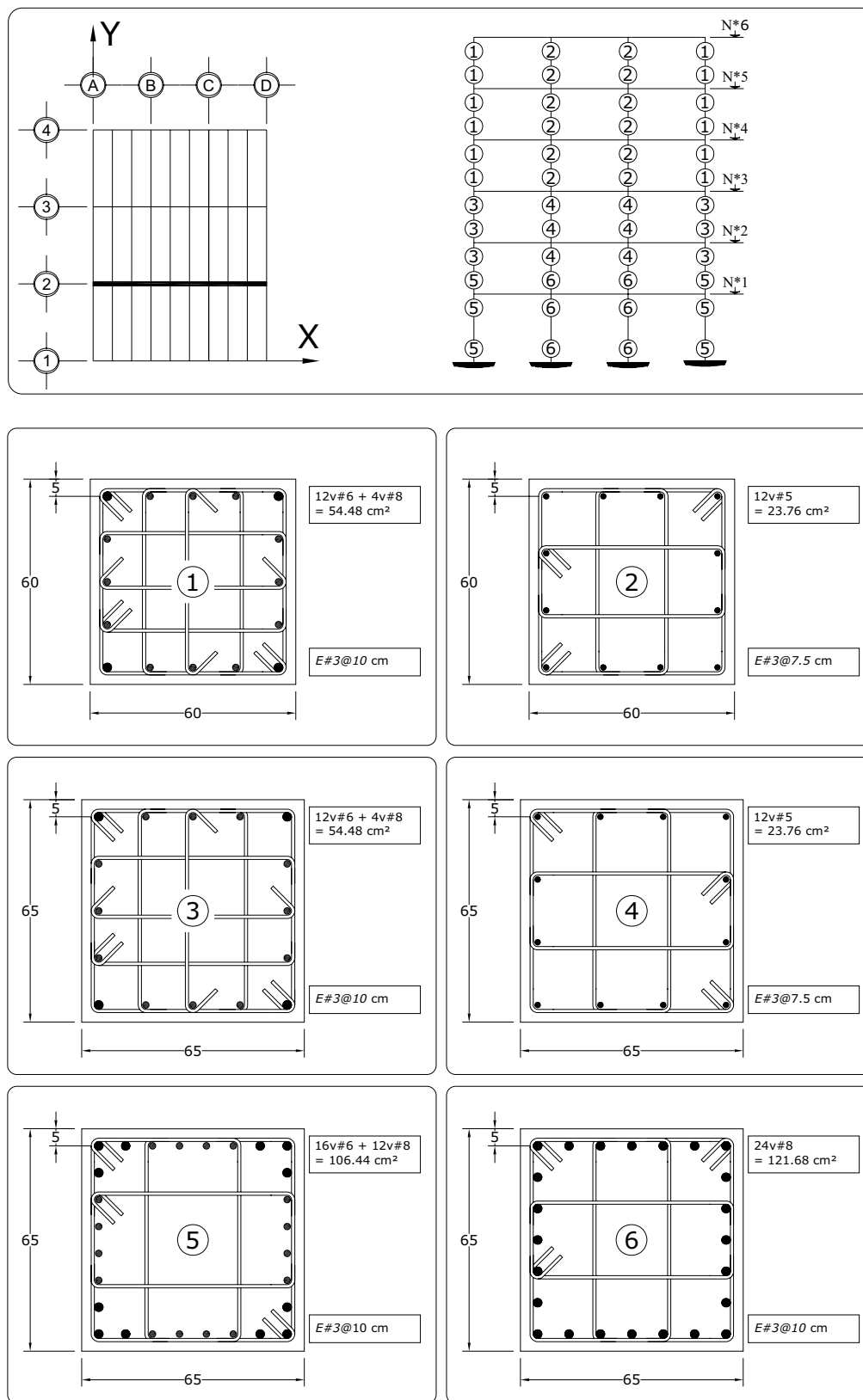
Fig 3.97 Tipos de armados de refuerzo longitudinal y transversal resultantes en los extremos de las columnas de 1 eje 2, caso C1 (Q = 2)
