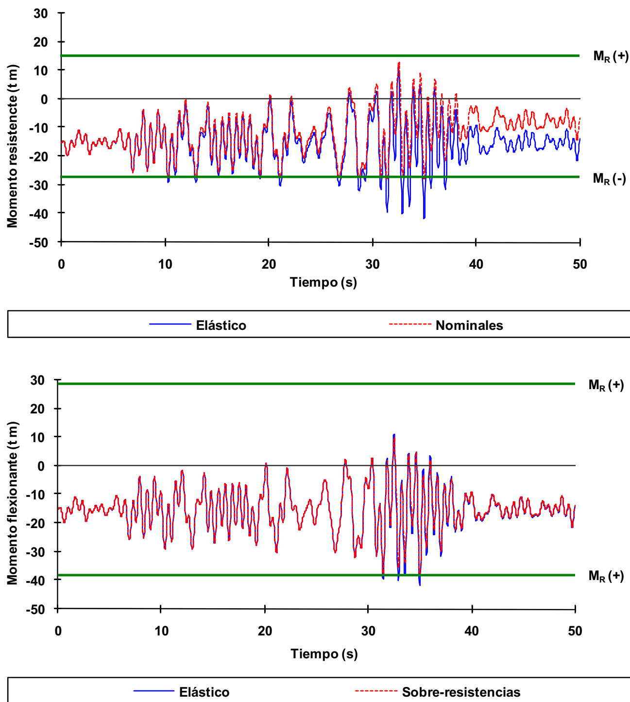
Fig 4.60 Historias de momentos flexionantes del extremo izquierdo de la viga 7 del nivel 1 del eje 2, caso B2, análisis paso a paso elástico e inelástico (sin y con sobre-resistencias), diseño Apéndice A, NTC-Sismo del RDF-04, edificio de 3 niveles
