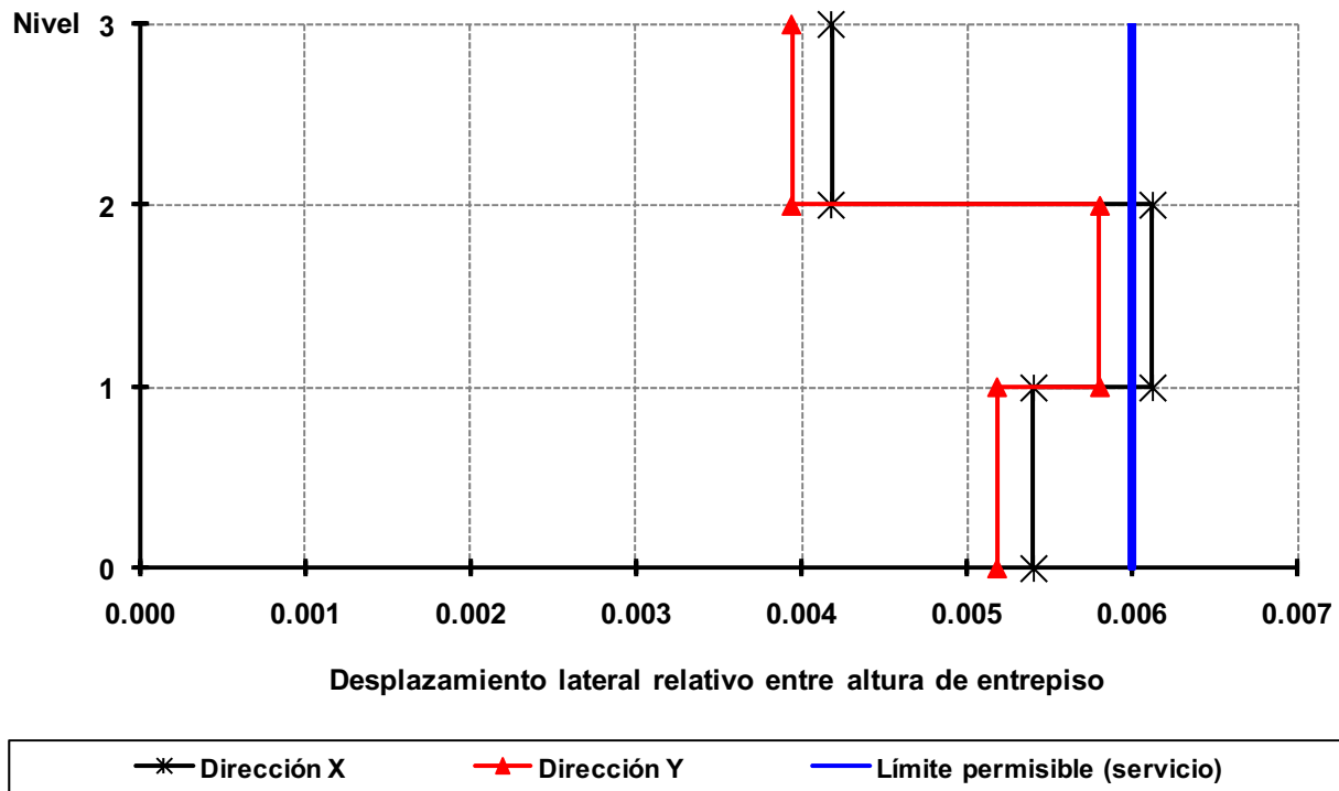
Fig 3.16 Relaciones desplazamiento lateral relativo entre altura de entrepiso (rige condición de servicio), análisis dinámico modal espectral, edificio de 3 niveles, caso A1 ( Q = 2 )
