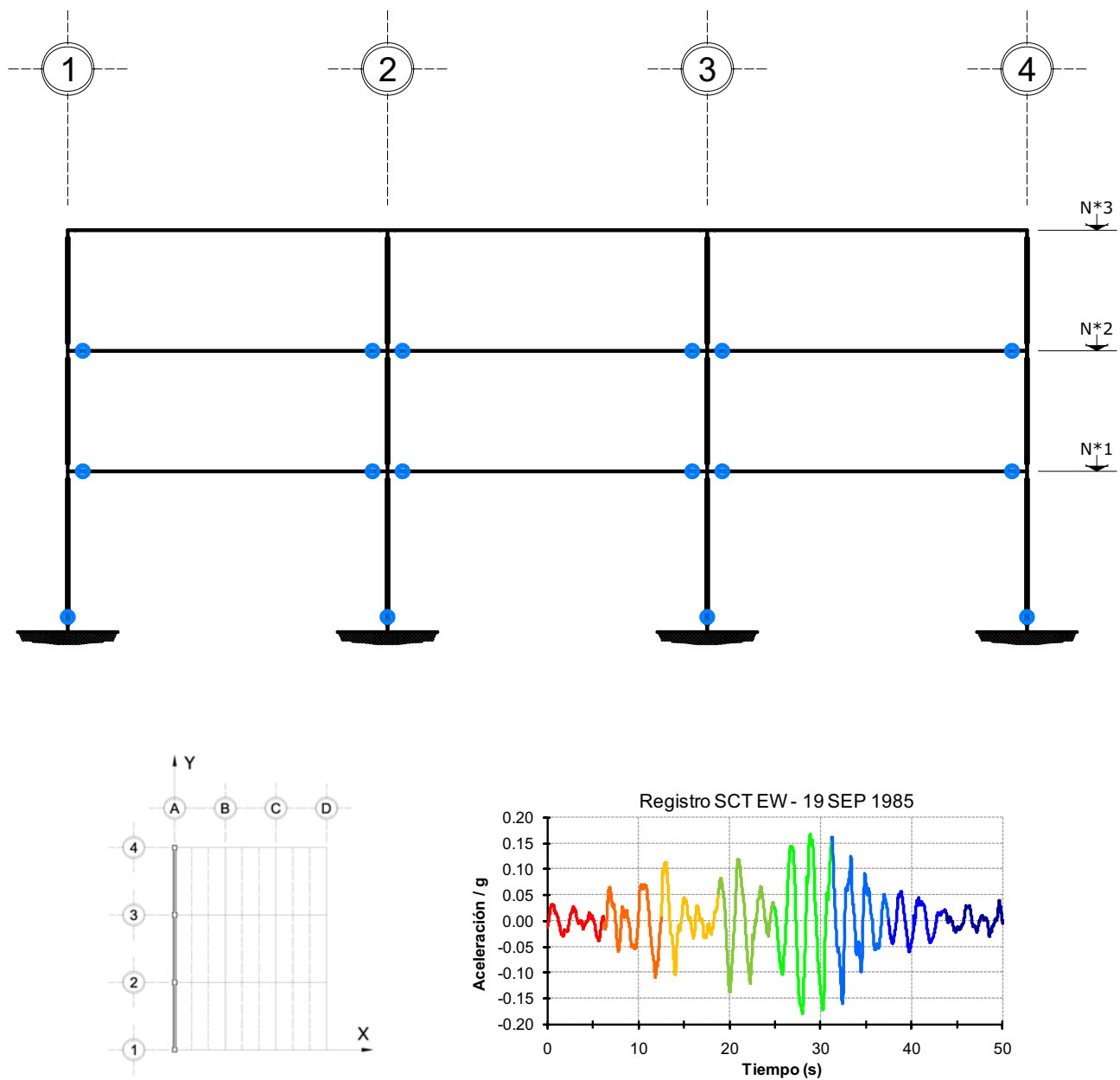
Fig 4.129 Ubicación y secuencia de formación de articulaciones plásticas, análisis paso a paso, con sobre-resistencias, edificio de 3 niveles, eje A, caso B2
