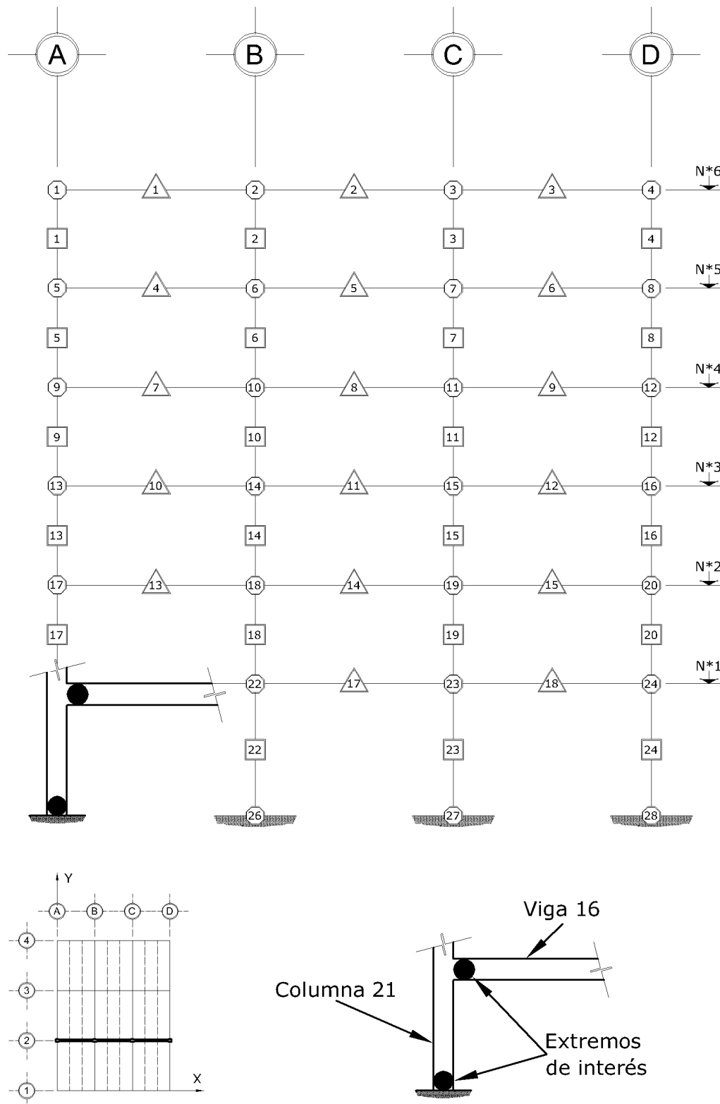
Fig 4.8 Identificación de los extremos en secciones estructurales de la viga 16 y la columna 21 para el estudio de las historias en el tiempo de las respuestas de los análisis paso a paso elásticos e inelásticos (sin y con sobre-resistencias), edificios de 6 niveles, eje 2 (dirección corta), casos C1 y C2 ( Q = 2 ), D1 y D2 ( Q = 4 )
