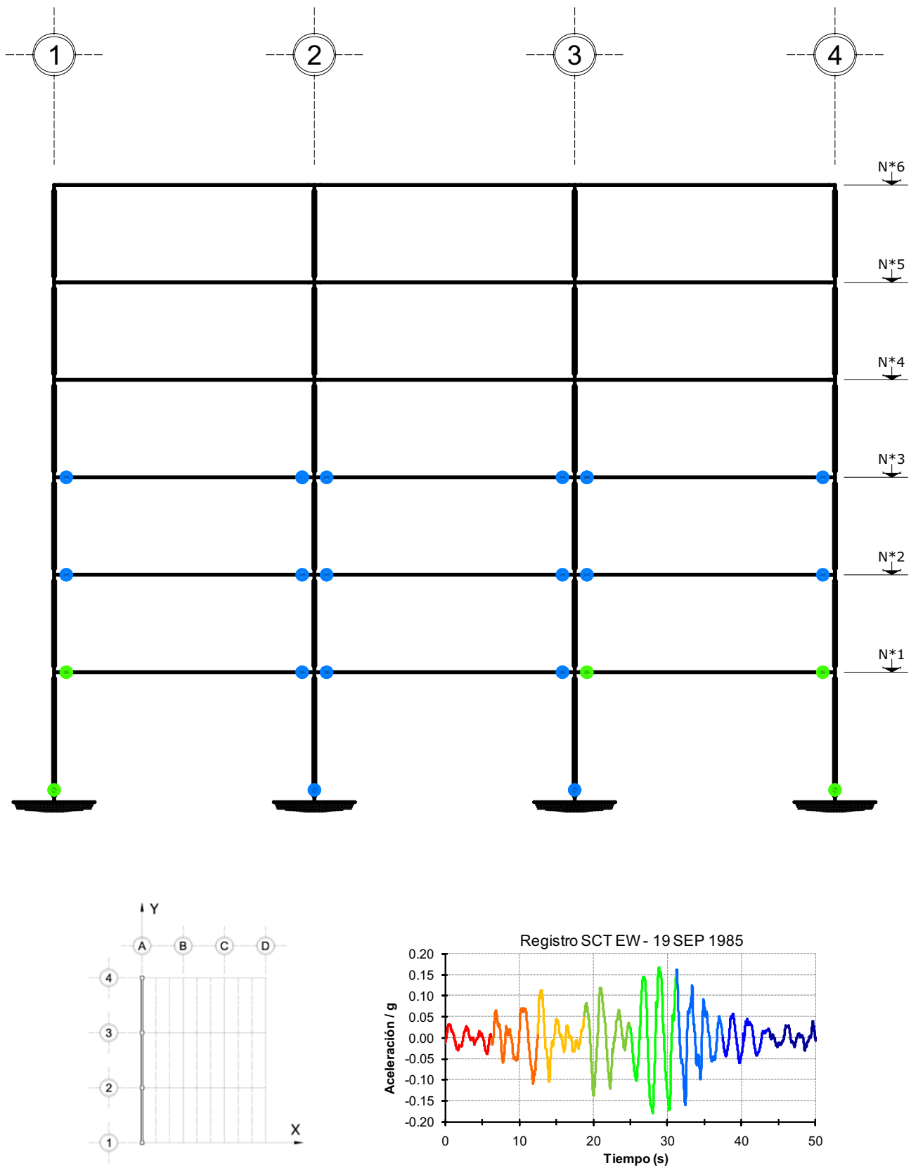
Fig 4.137 Ubicación y secuencia de formación de articulaciones plásticas, análisis paso a paso, con sobre-resistencias, edificio de 6 niveles, eje A, caso D2
