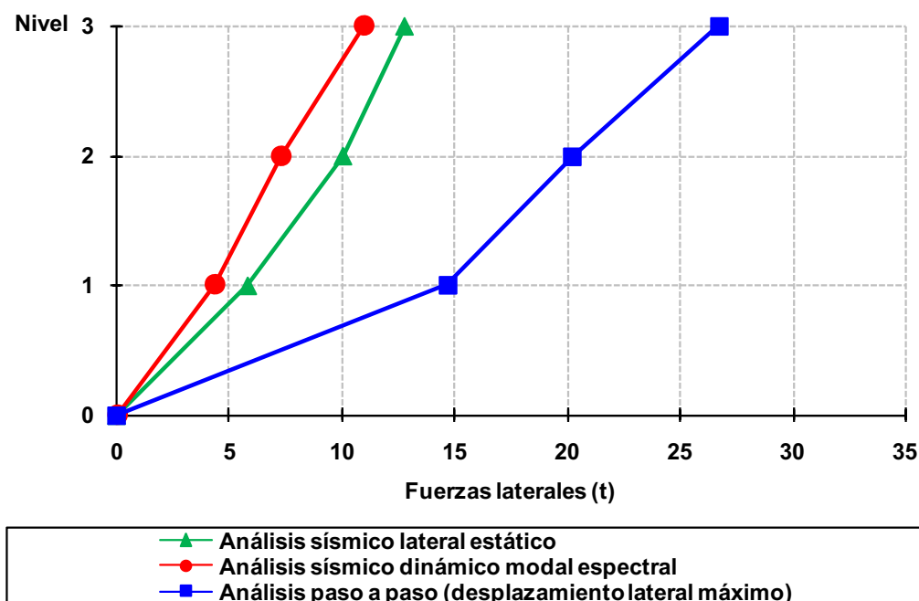
Fig 4.142 Distribución del perfil de fuerzas laterales debidas a diferentes condiciones de análisis sísmico del eje 2, caso B2, (sin sobre-resistencias), diseño según el Apéndice A de las NTC-Sismo del RDF-04, edificio de 3 niveles
