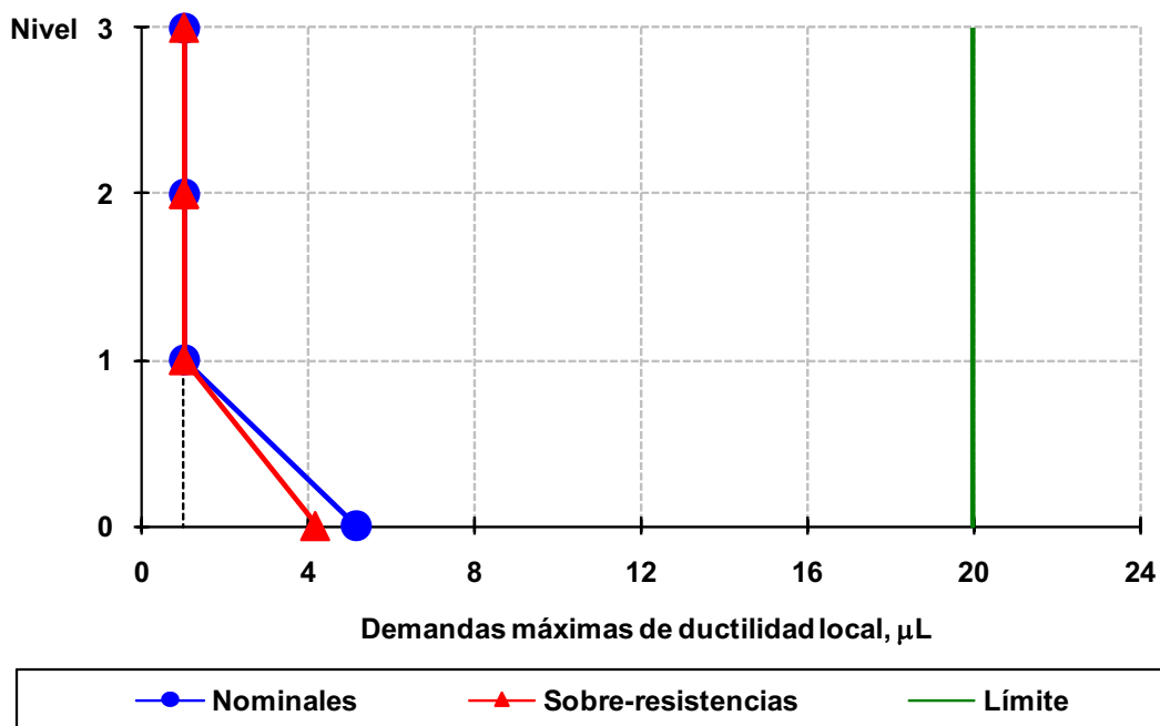
Fig 4.179 Demandas máximas de ductilidad local desarrolladas en columnas del eje A, caso A2, análisis Push-over (sin y con sobre-resistencias), perfil de cargas laterales del análisis dinámico modal espectral, diseño Apéndice A, NTC-Sismo del RDF-04, edificio de 3 niveles
