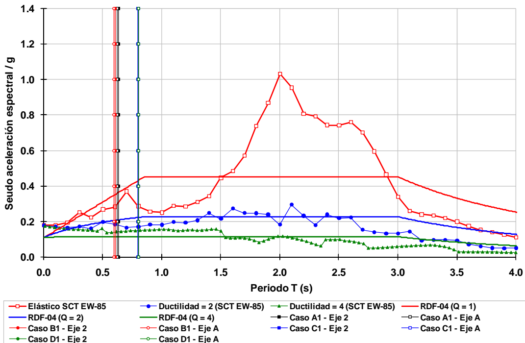
Fig 5.1 Espectros de respuesta SCT EW-85 (ductilidades 1, 2 y 4, con amortiguamiento del 5%) y de diseño ( Q=1, 2 y 4 ) del Cuerpo Principal (zona sísmica III b ) de las NTC-Sismo del RDF-04, y ubicación de los periodos fundamentales de vibración de los diferentes modelos de estudio de 3 niveles
