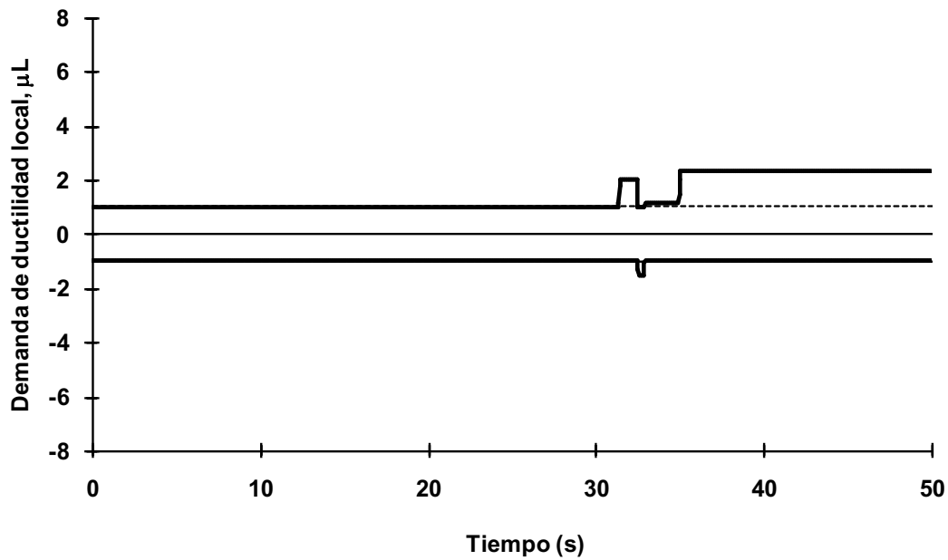
Fig 4.105 Demanda de ductilidad local desarrollada en el extremo izquierdo de la viga 7 del nivel 1, eje A, caso B2, análisis paso a paso inelástico (con sobre-resistencias), NTC-Sismo del RDF-04, edificio de 3 niveles
