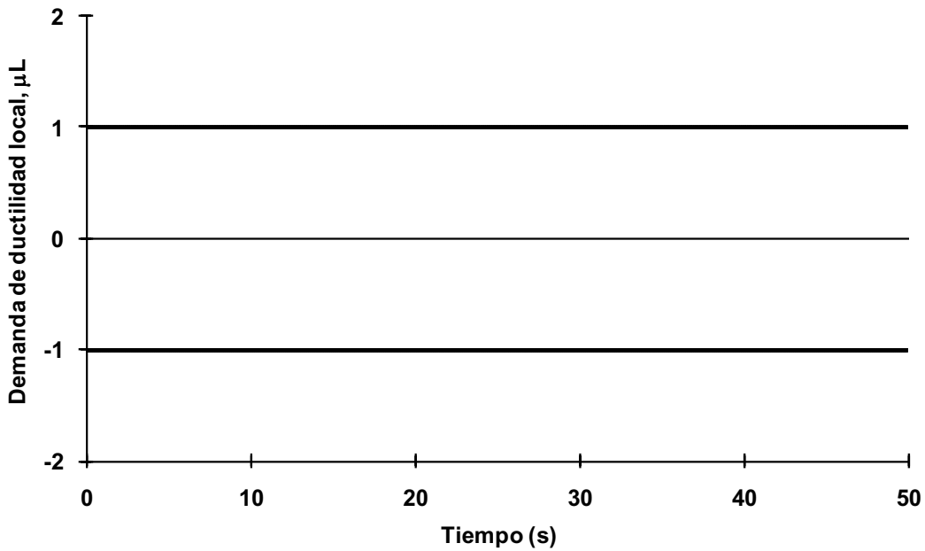
Fig 4.109 Demanda de ductilidad local desarrollada en el extremo izquierdo de la viga 16 del nivel 1, eje A, caso C2, análisis paso a paso inelástico (con sobre-resistencias), NTC-Sismo del RDF-04, edificio de 6 niveles
