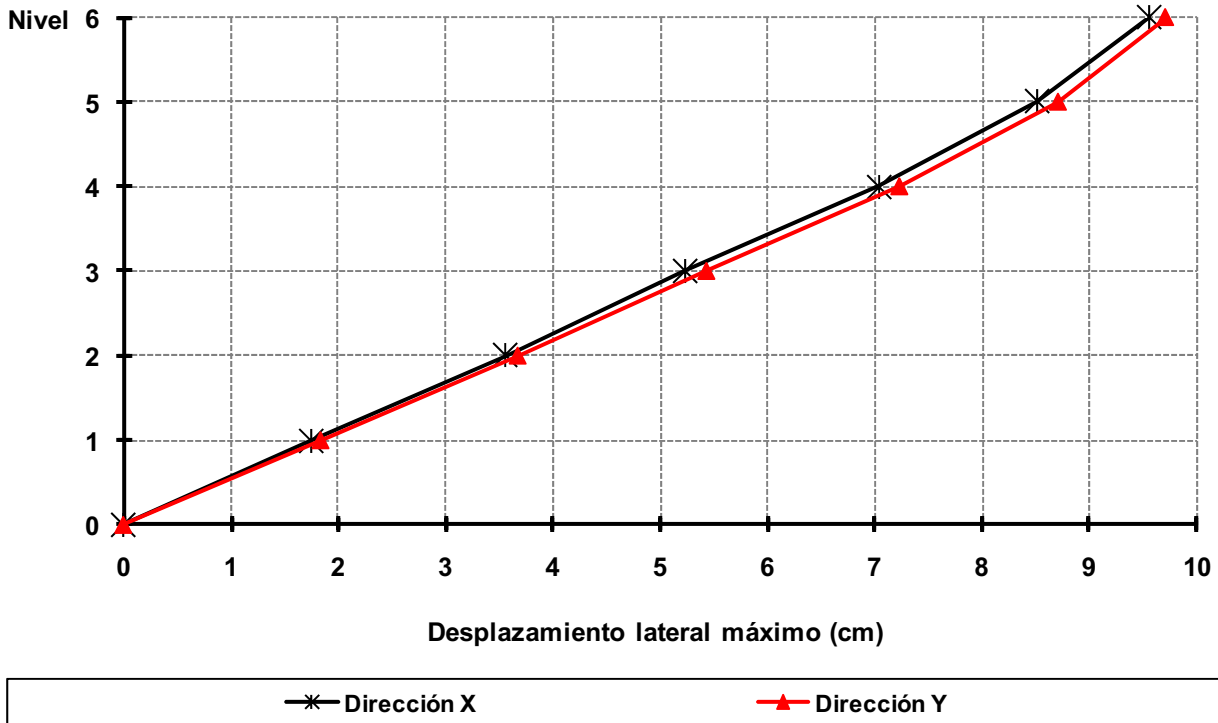
Fig 3.30 Desplazamientos laterales máximos, análisis dinámico modal espectral (rige condición de servicio), edificio de 6 niveles, caso D1 ( Q = 4 )
