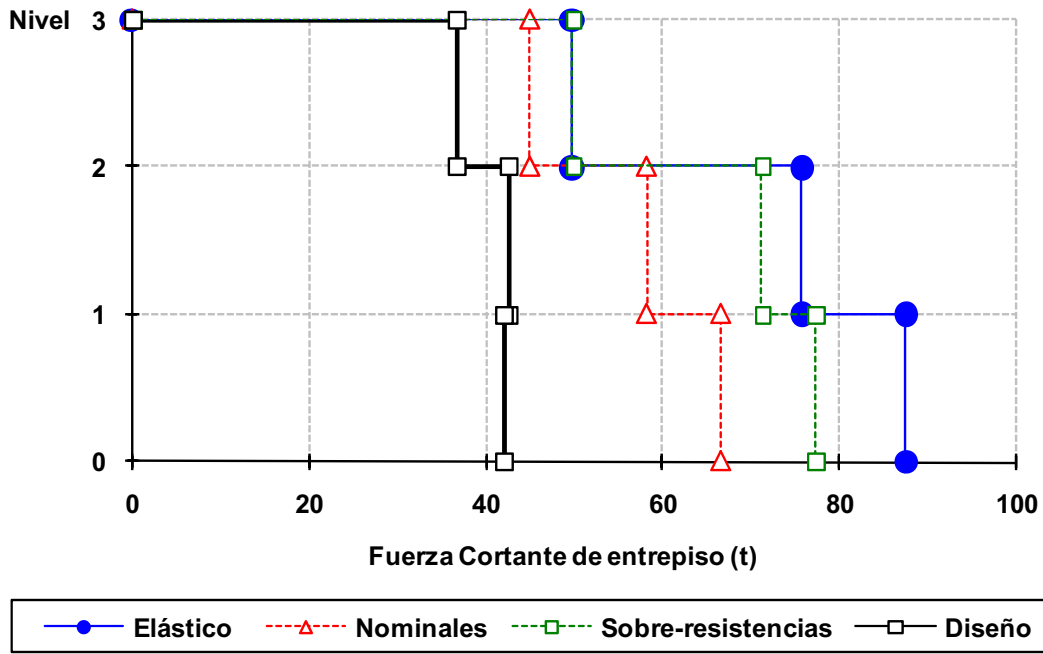
Fig 4.36 Envolventes de fuerzas cortantes de entrepiso del eje 2, caso B2, análisis paso a paso elástico e inelástico (sin y con sobre-resistencias) y modal espectral, NTC-Sismo del RDF-04, edificio de 3 niveles
