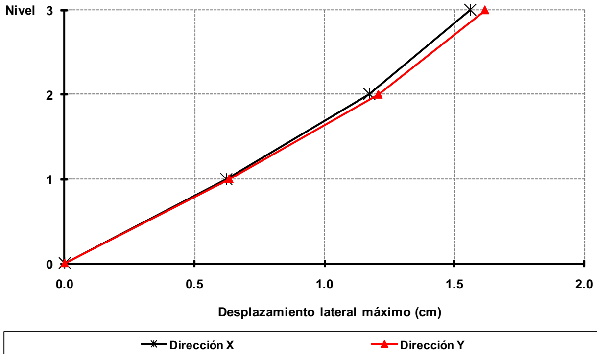
Fig 3.27a Desplazamientos laterales máximos, análisis dinámico modal espectral (condición de servicio), edificio de 3 niveles, caso B2 ( Q = 4 )
