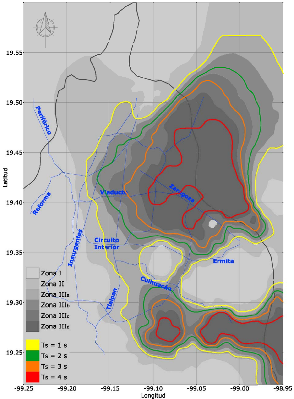
Fig 2.9 Periodos dominantes del movimiento del suelo, T_s (s), en la ciudad de México para fines del diseño por sismo, según el Apéndice A de las NTC-Sismo del RDF-04
