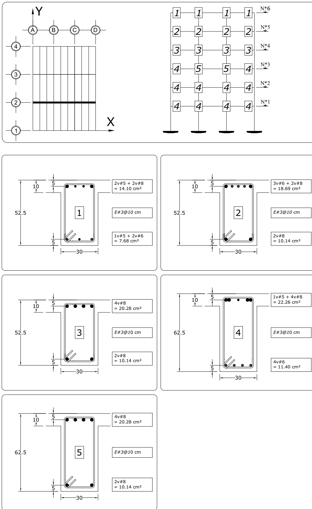
Fig 3.100 Tipos de armados de refuerzo longitudinal y transversal resultantes en los extremos de las vigas del eje 2, caso D1 (Q = 4)
