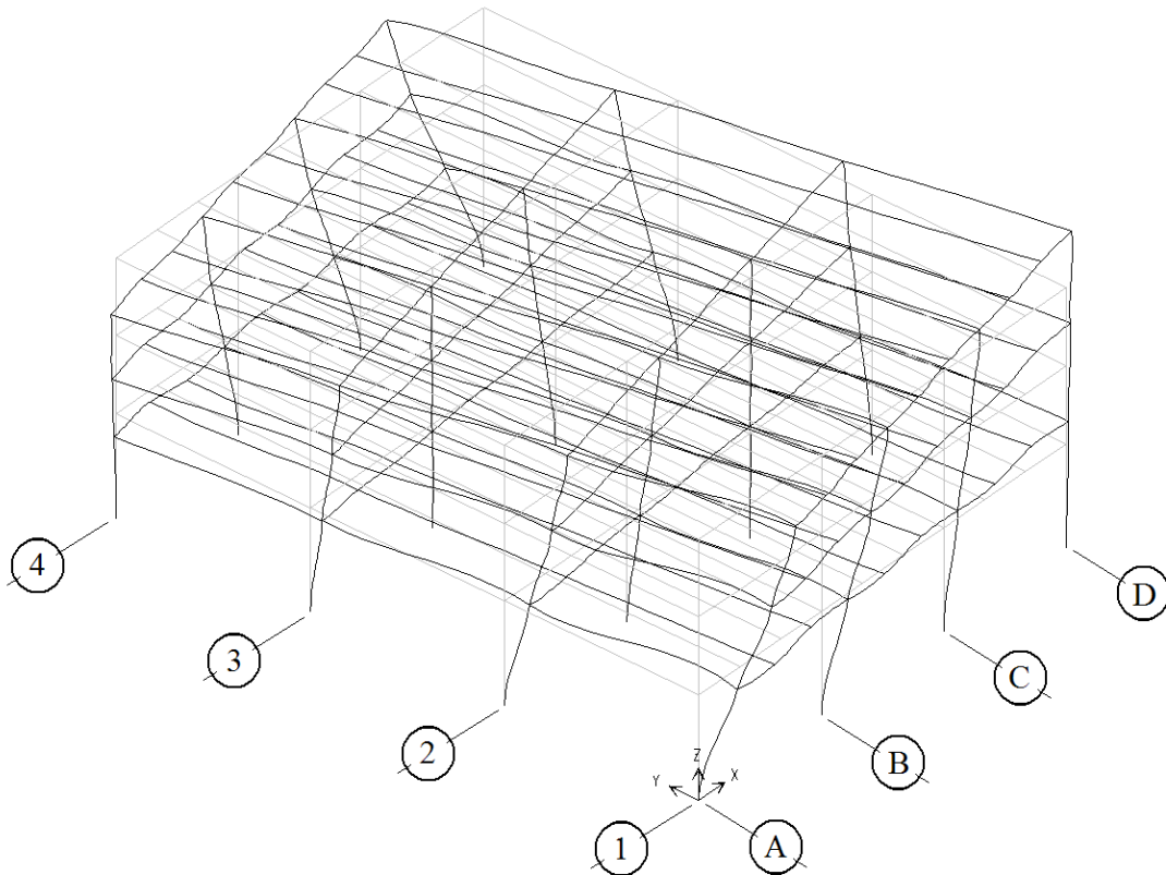
Fig 3.9 Deformada en perspectiva del primer modo de vibración en torsión, edificio de 3 niveles
