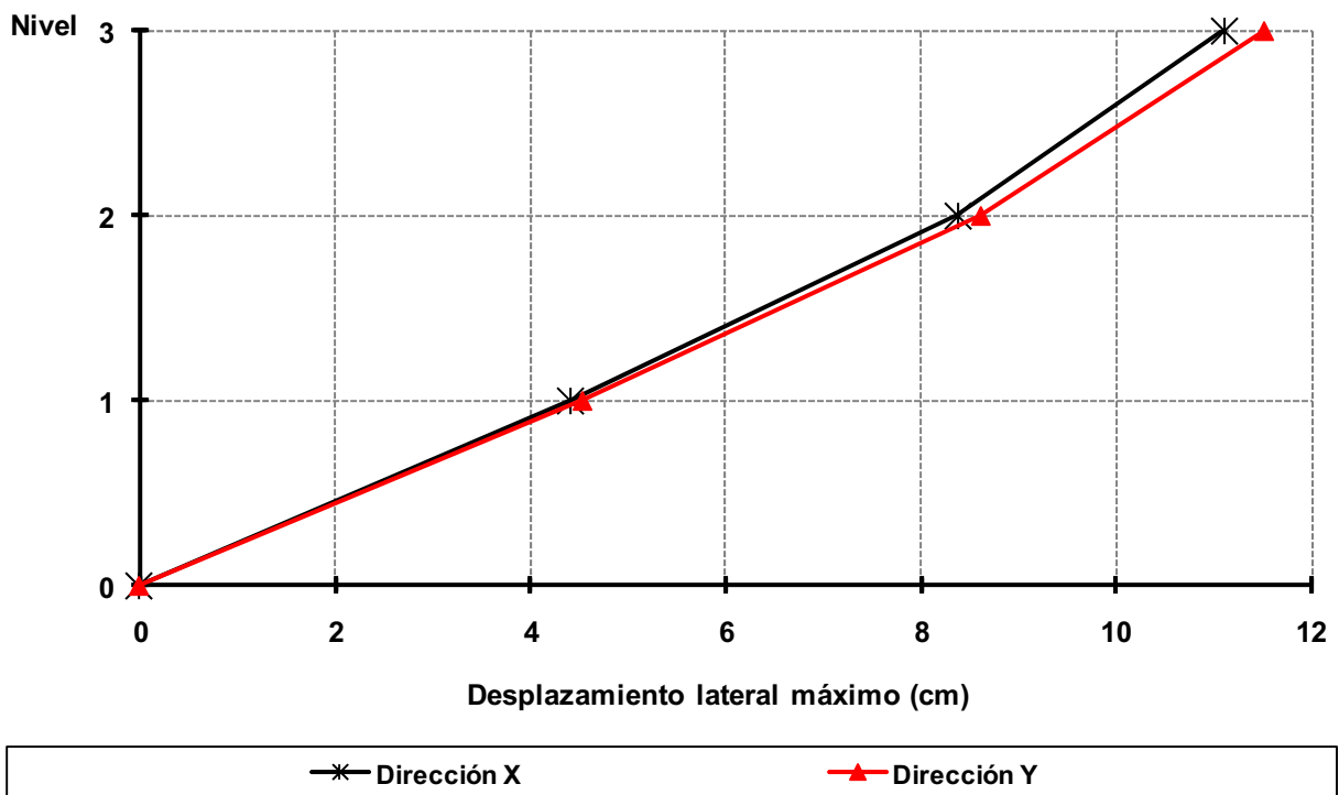
Fig 3.25b Desplazamientos laterales máximos, análisis dinámico modal espectral (condición de colapso), edificio de 3 niveles, caso A2 ( Q = 2 )
