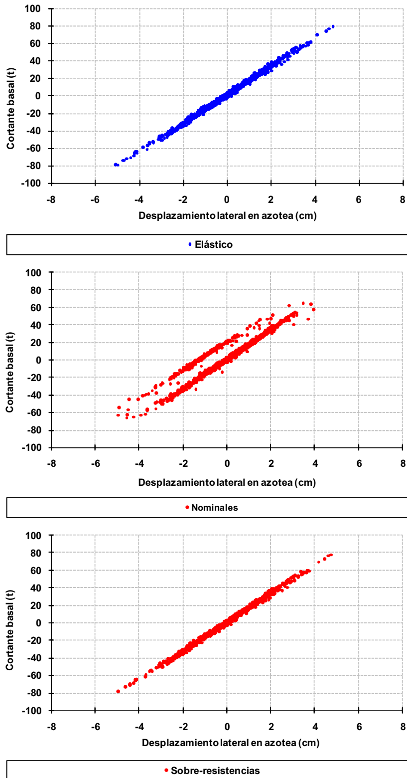
Fig 4.51 Relaciones fuerza cortante basal - desplazamiento horizontal en azotea, eje A, caso A2, análisis paso a paso elástico e inelástico (sin y con sobre-resistencias), diseño Apéndice A, NTC-Sismo del RDF-04, edificio de 3 niveles
