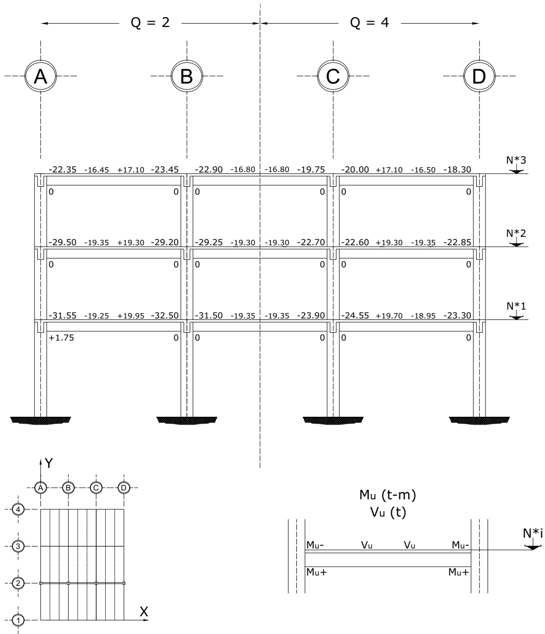
Fig 3.68 Momentos flexionantes y fuerzas cortantes últimos de vigas, eje 2, casos A2 ( Q = 2 ) y B2 ( Q = 4 )
