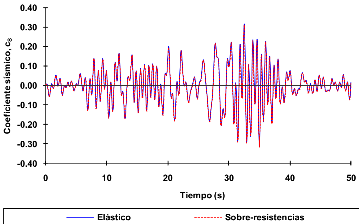
Fig 4.42 Historias de coeficientes sísmicos ( c_s ), eje 2, caso A2, análisis paso a paso elástico e inelástico (sin y con sobre-resistencias), diseño Apéndice A, NTC-Sismo del RDF-04, edificio de 3 niveles
