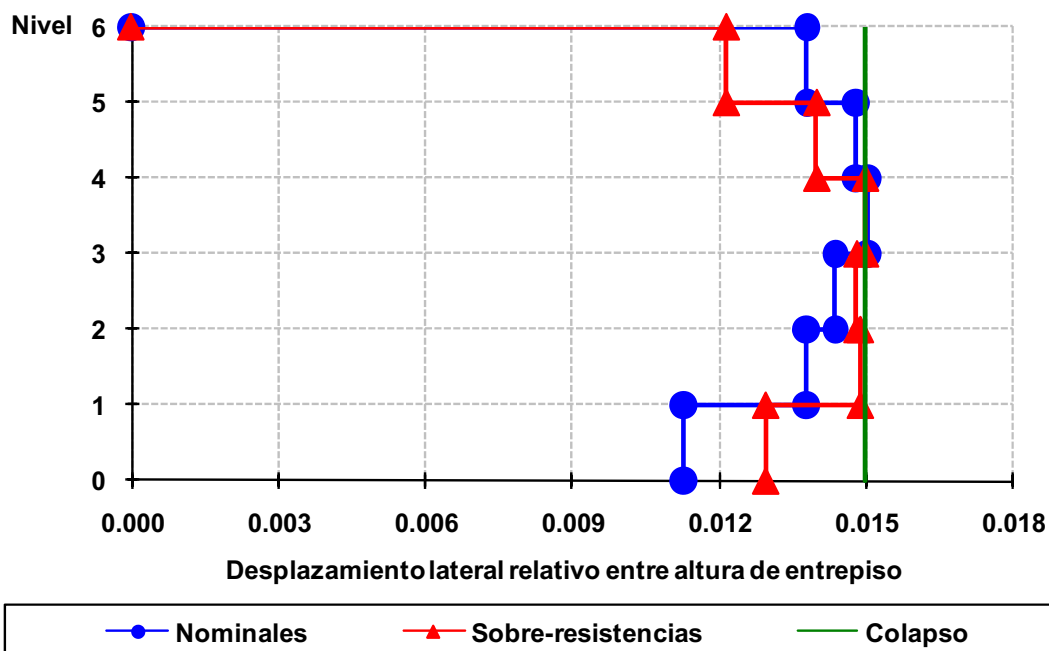
Fig 4.167 Relaciones desplazamiento lateral relativo entre altura de entrepiso del eje A, caso C2, análisis Push-over (sin y con sobre-resistencias), perfil de cargas laterales del análisis dinámico modal espectral, diseño Apéndice A, NTC-Sismo del RDF-04, edificio de 6 niveles
