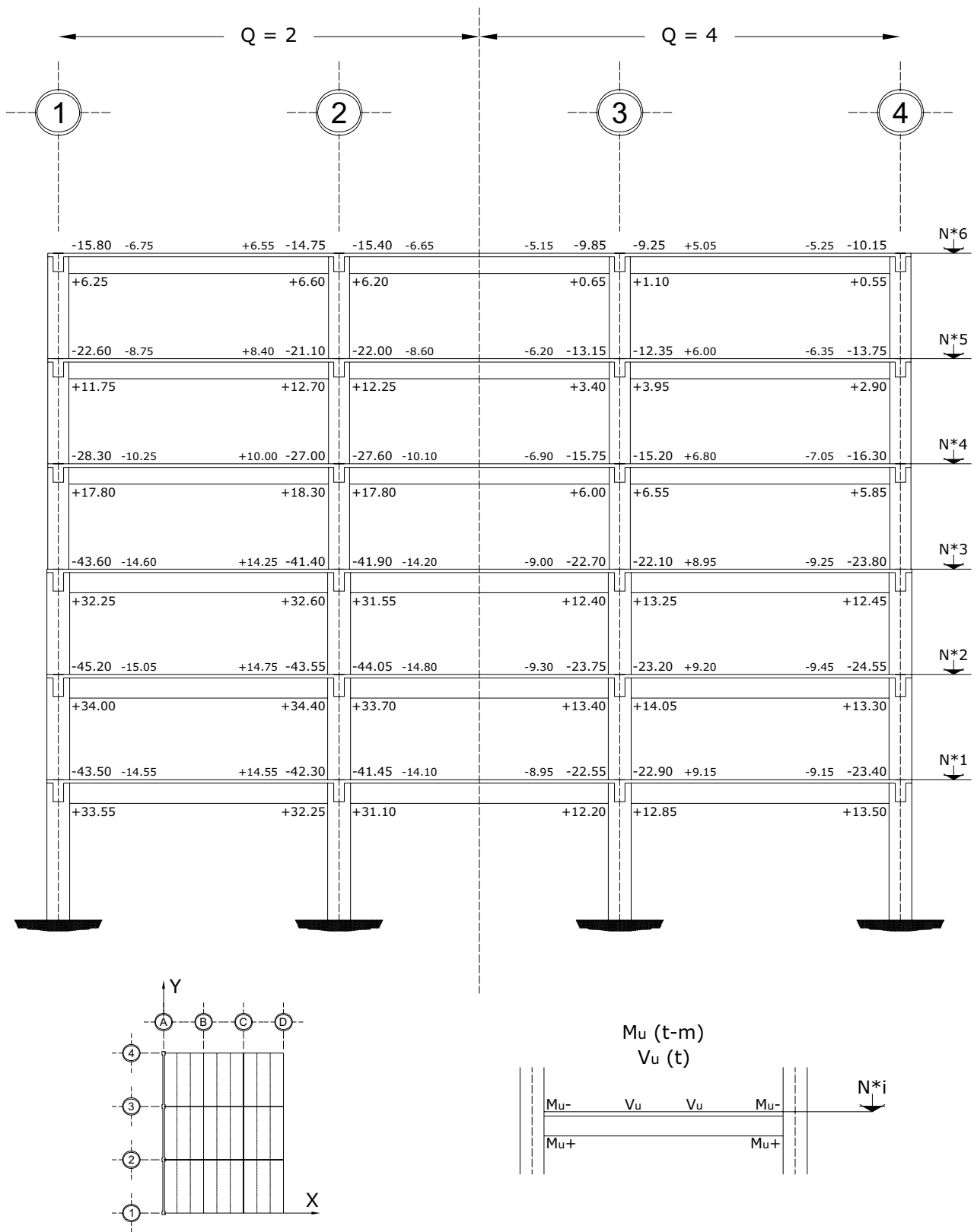
Fig 3.110 Momentos flexionantes y fuerzas cortantes últimos de vigas, eje A, casos C2 ( Q = 2 ) y D2 ( Q = 4 )
