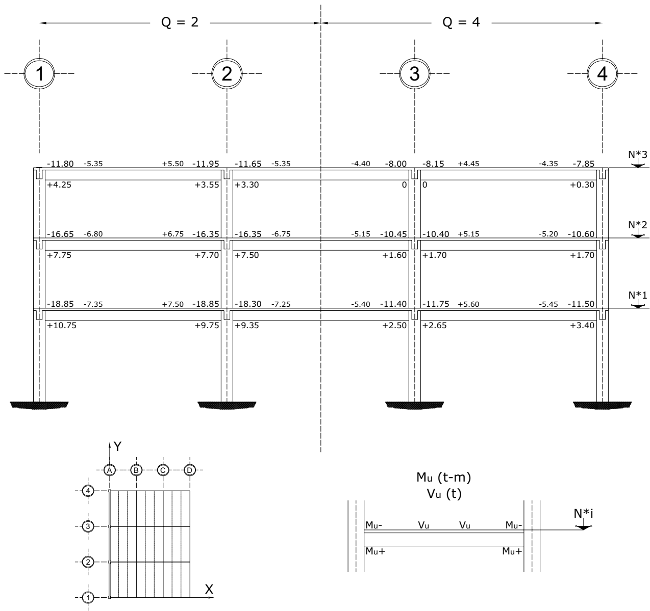
Fig 3.70 Momentos flexionantes y fuerzas cortantes últimos de vigas, eje A, casos A2 ( Q = 2 ) y B2 ( Q = 4 )
