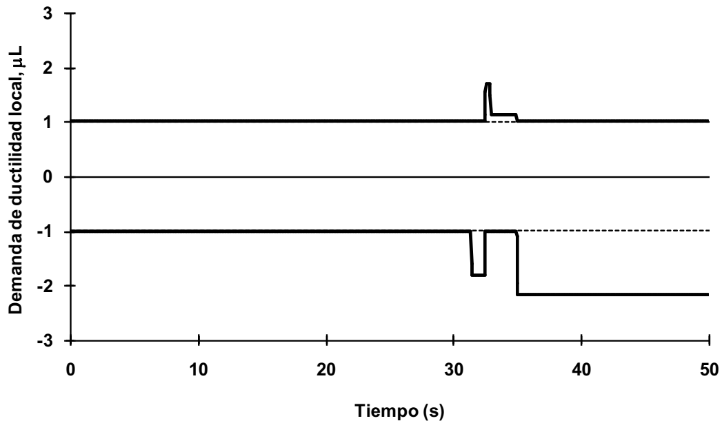
Fig 4.100 Demanda de ductilidad local desarrollada en el extremo izquierdo de la viga 7 del nivel 1, eje A, caso A2, análisis paso a paso inelástico (sin sobre-resistencias), NTC-Sismo del RDF-04, edificio de 3 niveles
