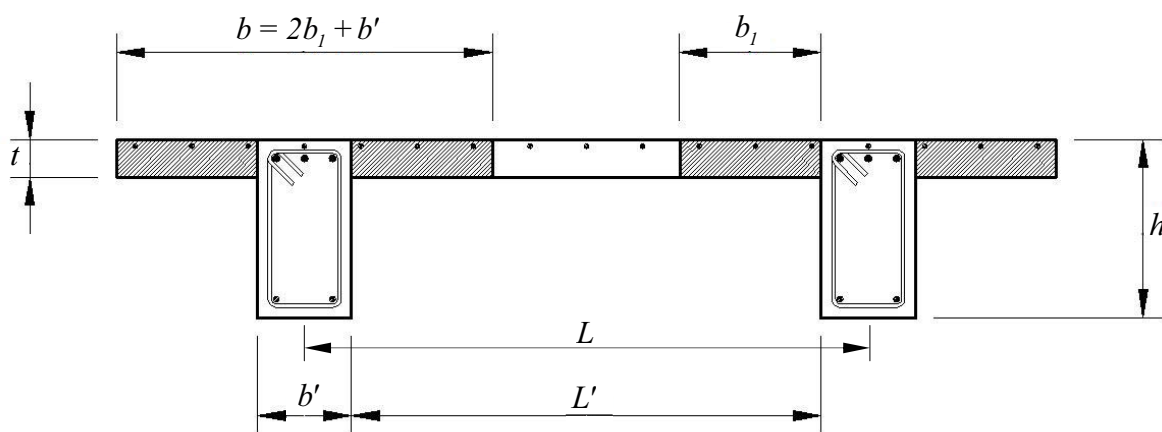
Fig 2.22a Ancho equivalente del patín a compresión con que contribuye la losa a la resistencia de flexión de la viga T
