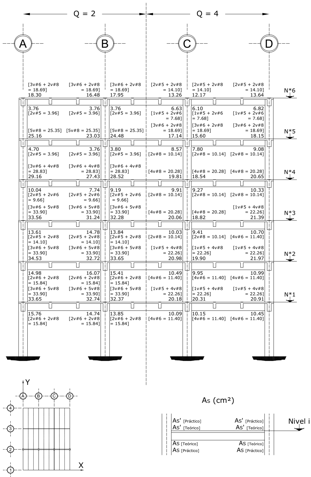
Fig 3.92 Acero de refuerzo longitudinal teórico y práctico necesario en vigas, eje 2, casos C1 (Q = 2) y D1 (Q = 4)
