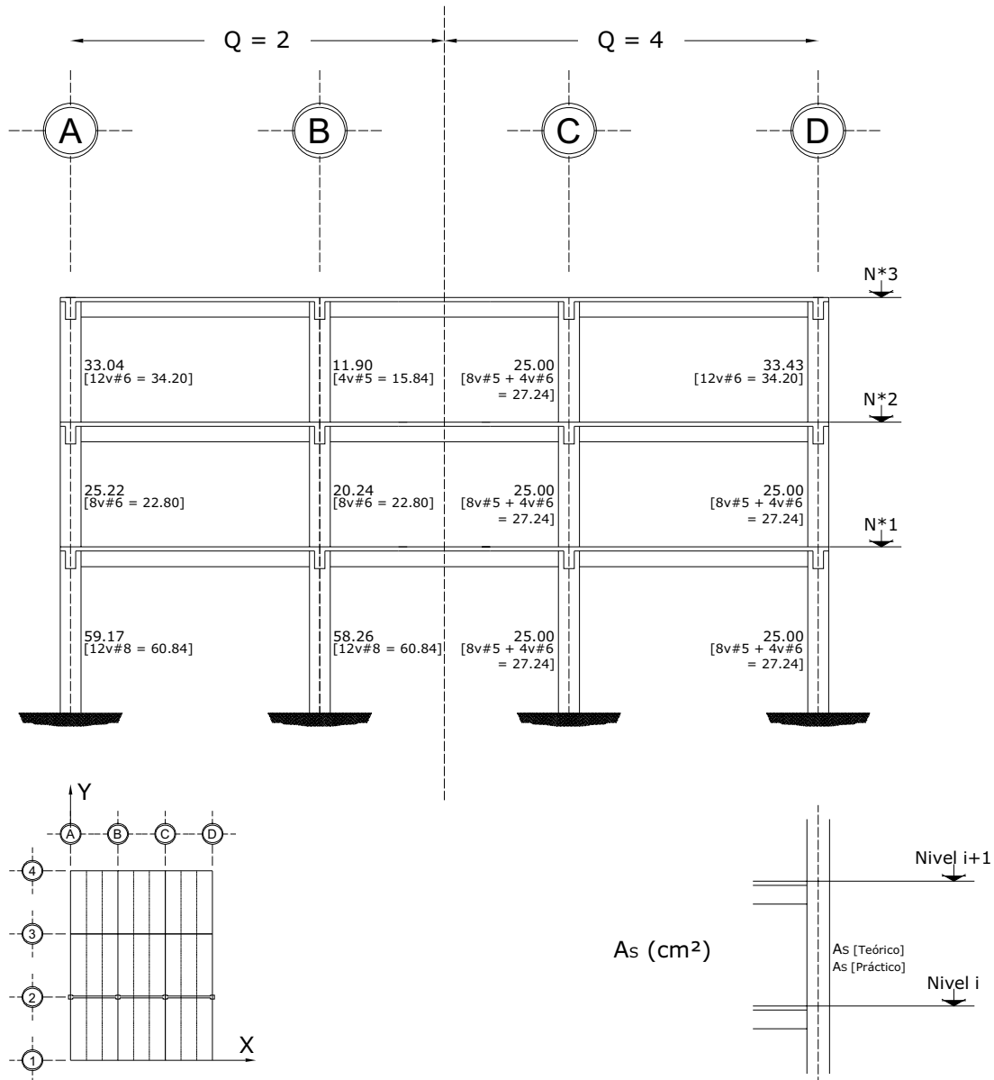
Fig 3.73a Acero de refuerzo longitudinal teórico y práctico necesario en columnas, eje 2, casos A2 ( Q = 2 ) y B2 ( Q = 4 )
