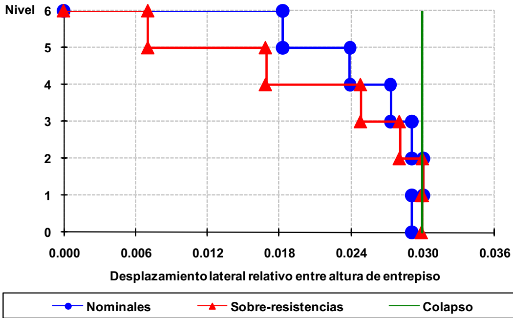
Fig 4.168 Relaciones desplazamiento lateral relativo entre altura de entrepiso del eje 2, caso D2, análisis Push-over (sin y con sobre-resistencias), perfil de cargas laterales del análisis dinámico modal espectral, diseño Apéndice A, NTC-Sismo del RDF-04, edificio de 6 niveles
