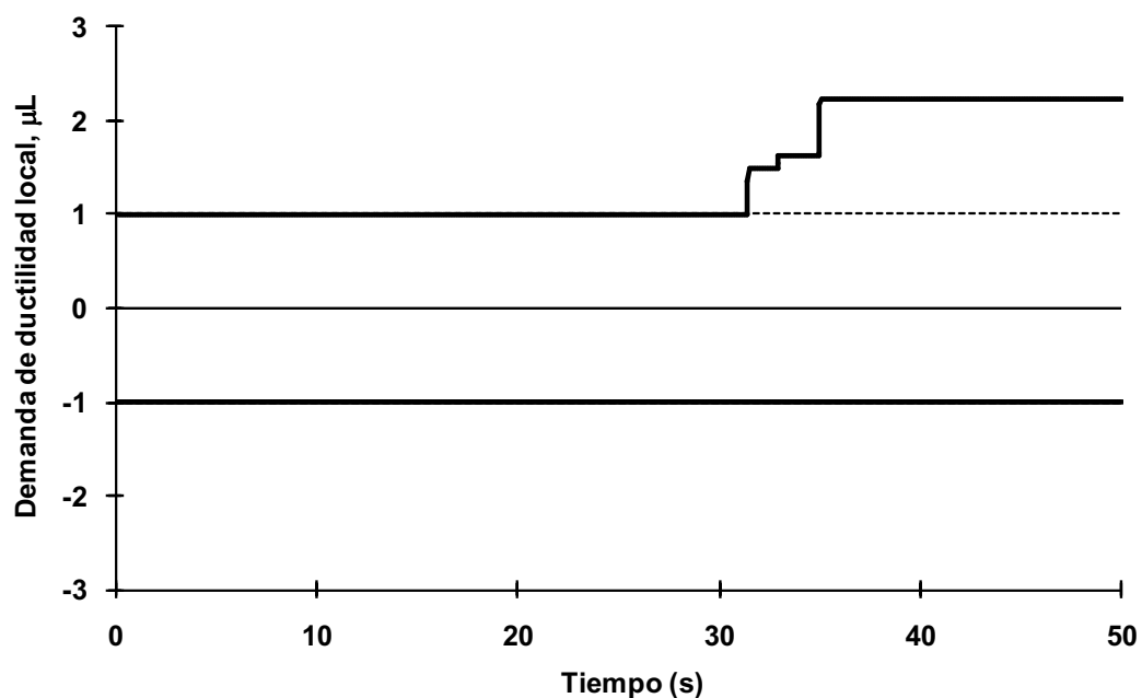
Fig 4.98 Demanda de ductilidad local desarrollada en el extremo izquierdo de la viga 7 del nivel 1, eje 2, caso A2, análisis paso a paso inelástico (sin sobre-resistencias), NTC-Sismo del RDF-04, edificio de 3 niveles
