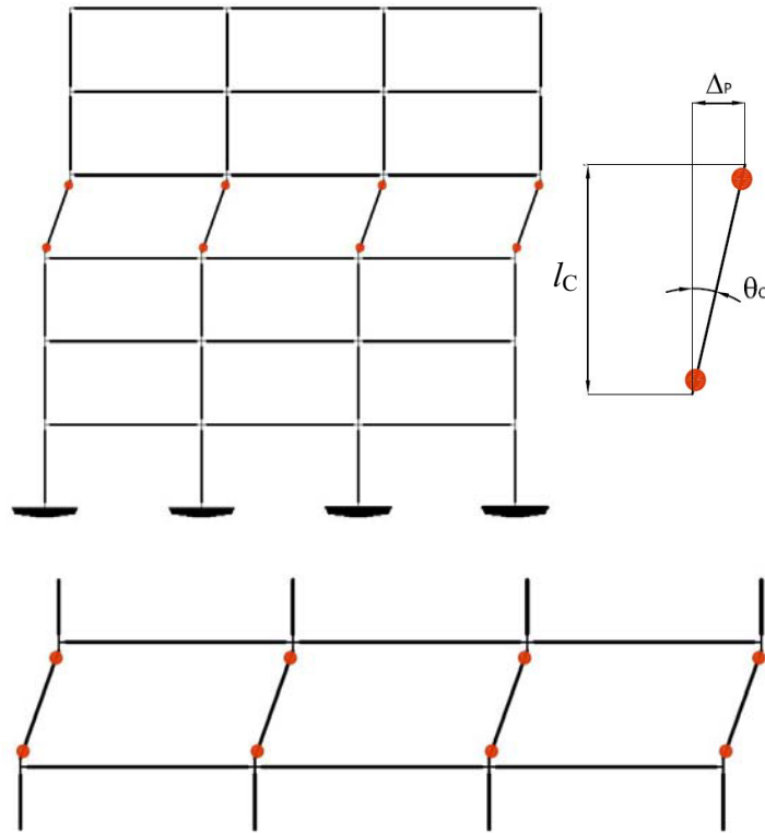
Fig 2.18 Mecanismo de falla de un entrepiso con columnas débiles y vigas fuertes
