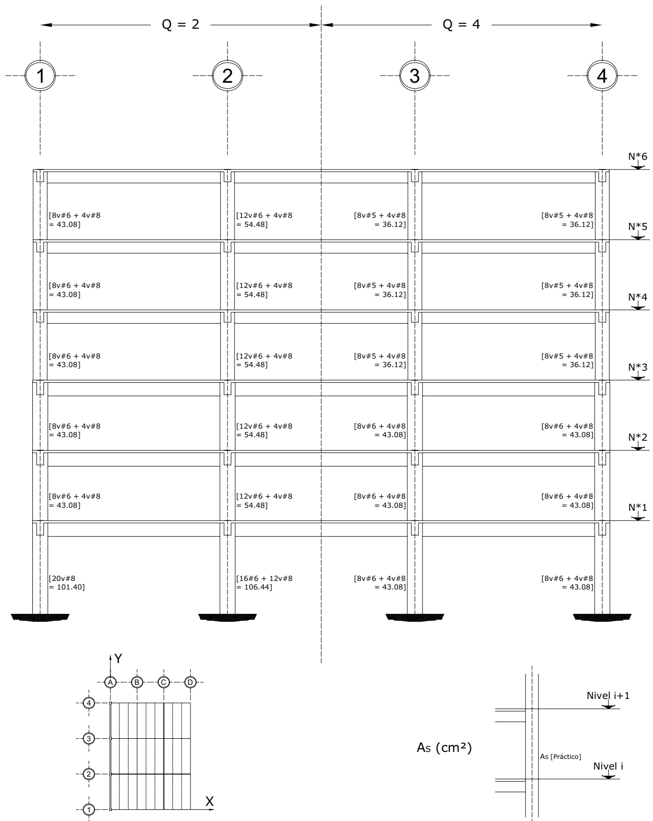
Fig 3.75b Acero de refuerzo longitudinal teórico y práctico necesario en columnas, eje A, casos C1 (Q = 2) y D1 (Q = 4)
