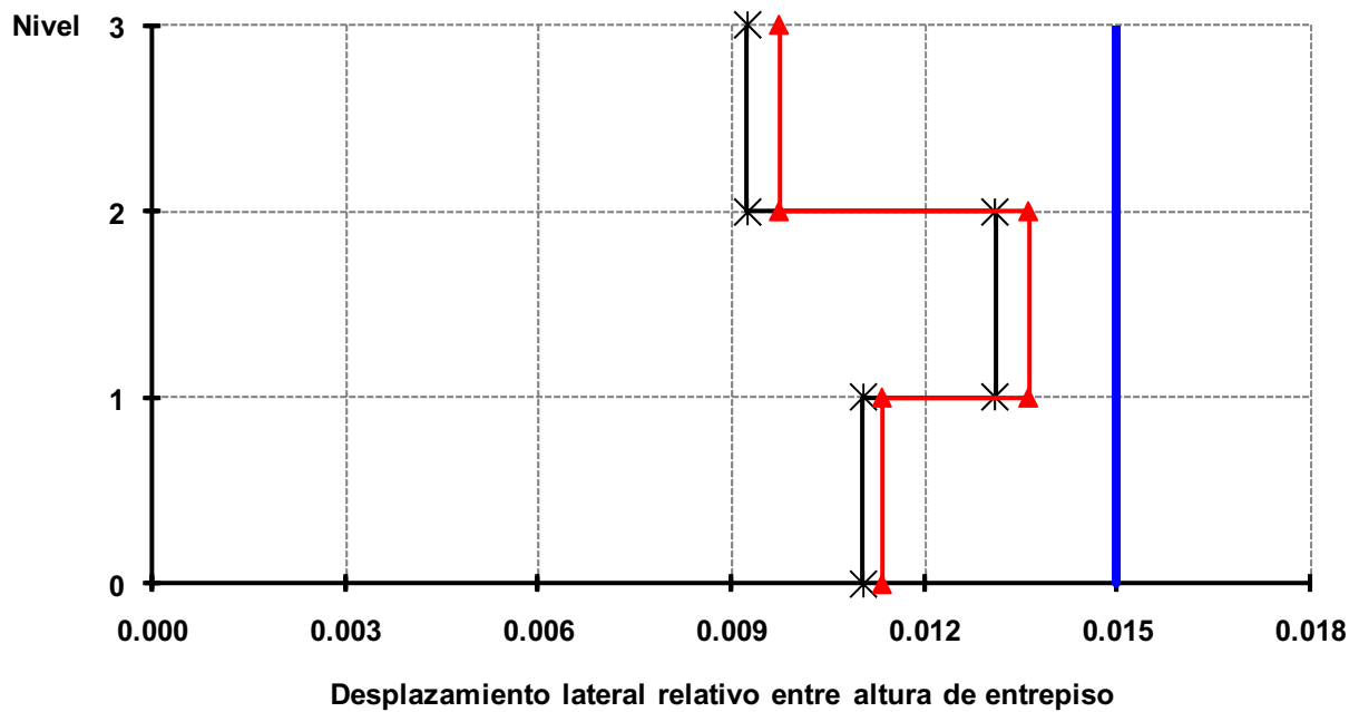
Fig 3.17b Relaciones desplazamiento lateral relativo entre altura de entrepiso (condición de colapso), análisis dinámico modal espectral, edificio de 3 niveles, caso A2 ( Q = 2 )
