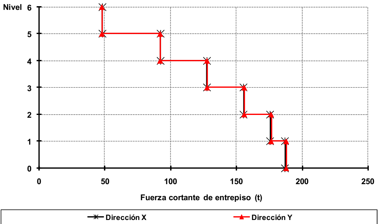
Fig 3.39 Fuerzas cortantes de entrepiso, análisis dinámico modal espectral, edificio de 6 niveles, caso D2 (Q = 4)
