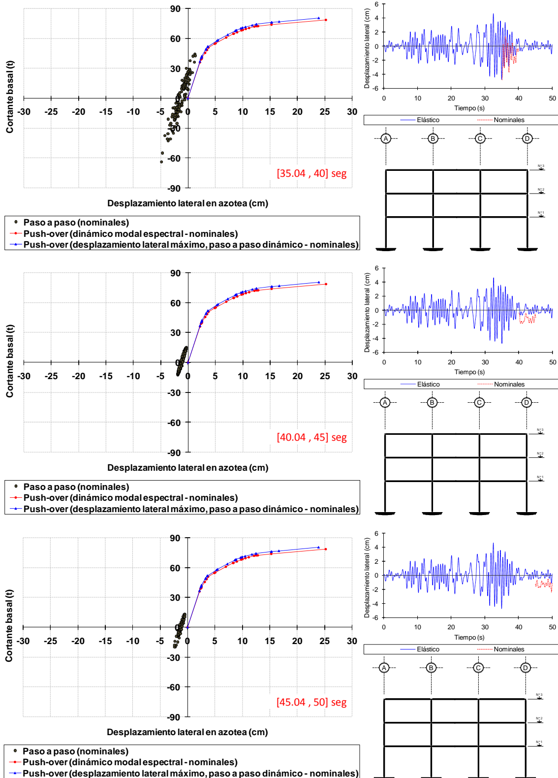
Fig 5.6c Comparación de la intensidad de la respuesta inelástica fuerza cortante basal - desplazamiento lateral de azotea para varios intervalos del tiempo (35 a 50 segundos) de los análisis paso a paso contra análisis estático no-lineal Push-over, resistencias nominales, caso B2 del eje 2 del edificio de 3 niveles
