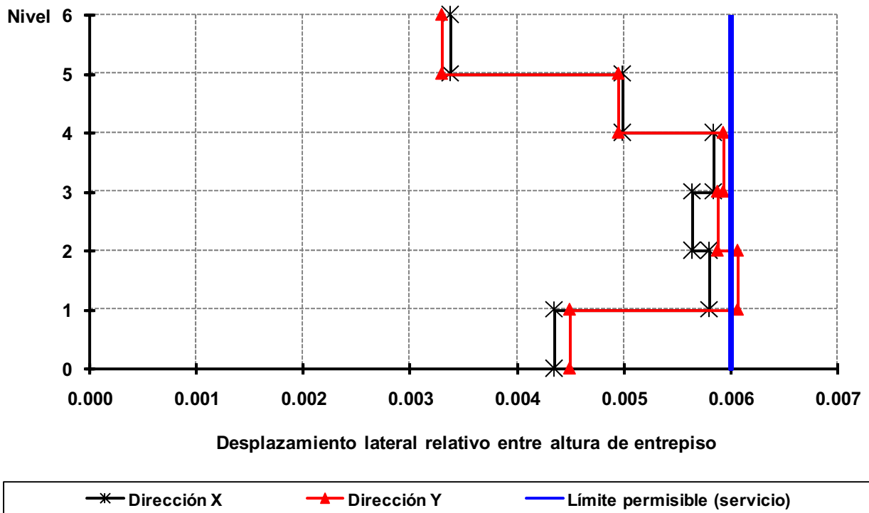
Fig 3.20 Relaciones desplazamiento lateral relativo entre altura de entrepiso (rige condición de servicio), análisis dinámico modal espectral, edificio de 6 niveles, caso C1 ( Q = 2 )
