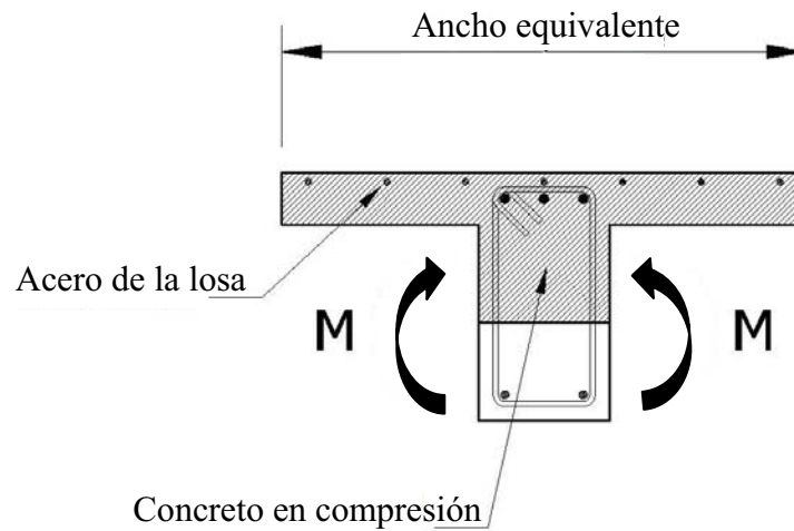
Fig 2.22b Contribución de los patines de la losa a la resistencia ante la acción de momento flexionante positivo
