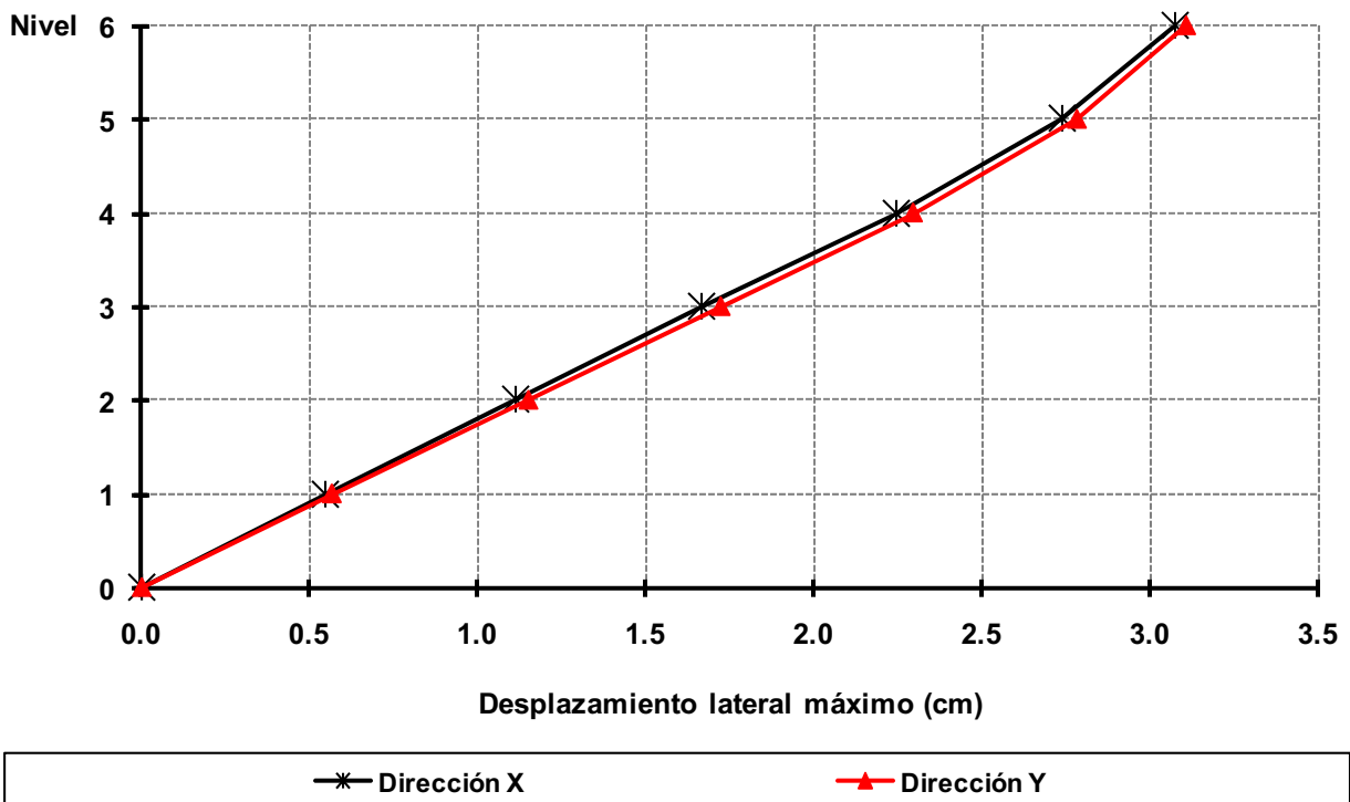
Fig 3.29a Desplazamientos laterales máximos, análisis dinámico modal espectral (condición de servicio), edificio de 6 niveles, caso C2 ( Q = 2 )
