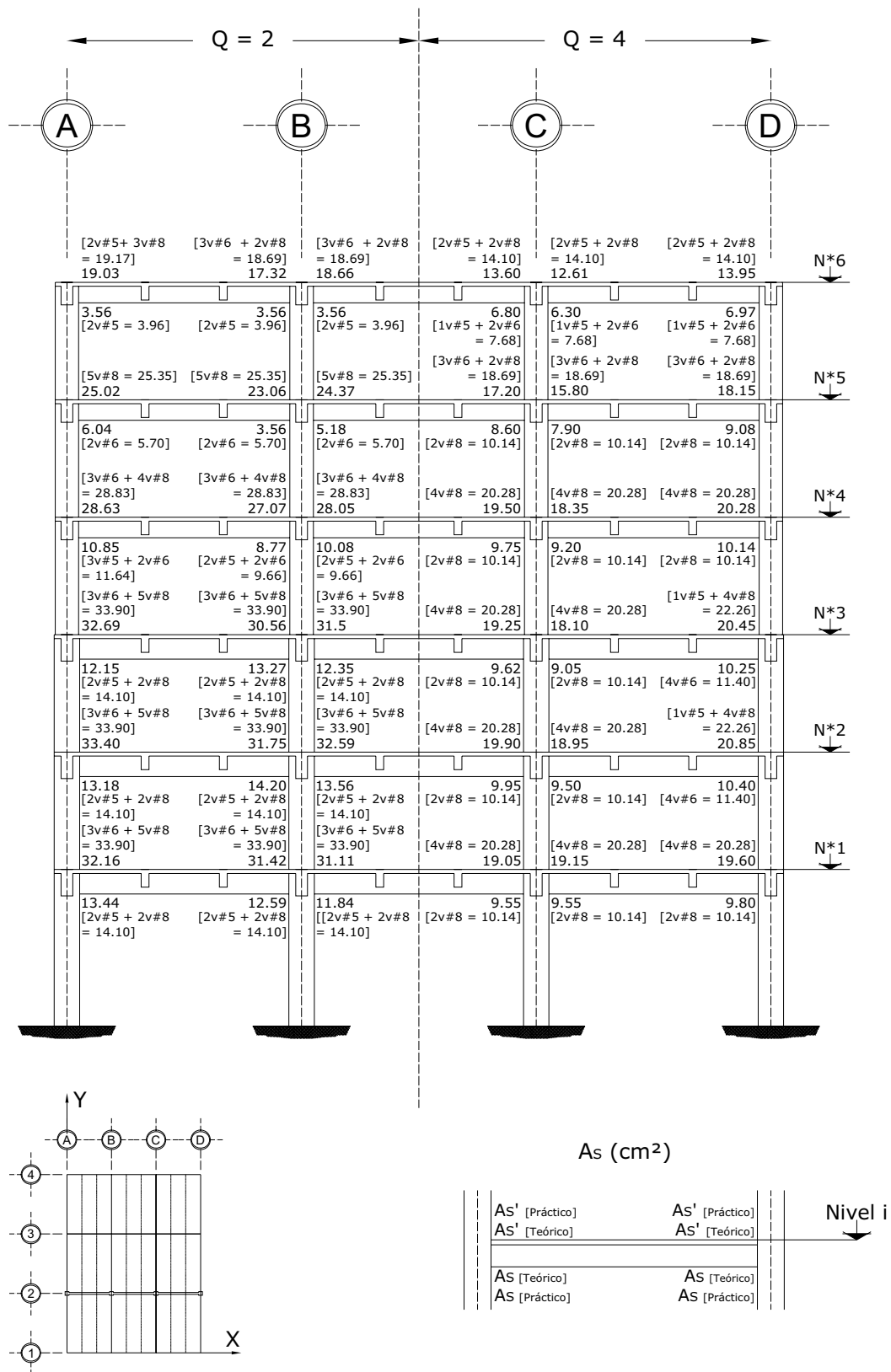
Fig 3.112 Acero de refuerzo longitudinal teórico y práctico necesario en vigas, eje 2, casos C2 ( Q = 2 ) y D2 ( Q = 4 )
