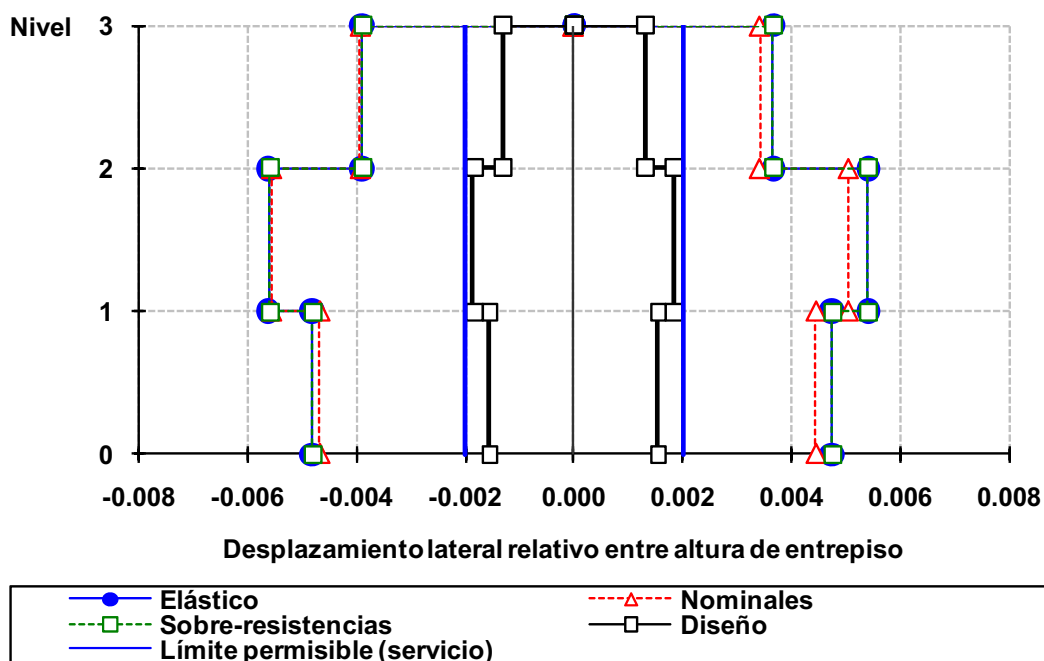
Fig 4.26 Relaciones desplazamiento lateral relativo entre altura de entrepiso del eje 2, caso A2, análisis paso a paso elástico e inelástico (sin y con sobre-resistencias) y modal espectral, NTC-Sismo del RDF-04, edificio de 3 niveles
