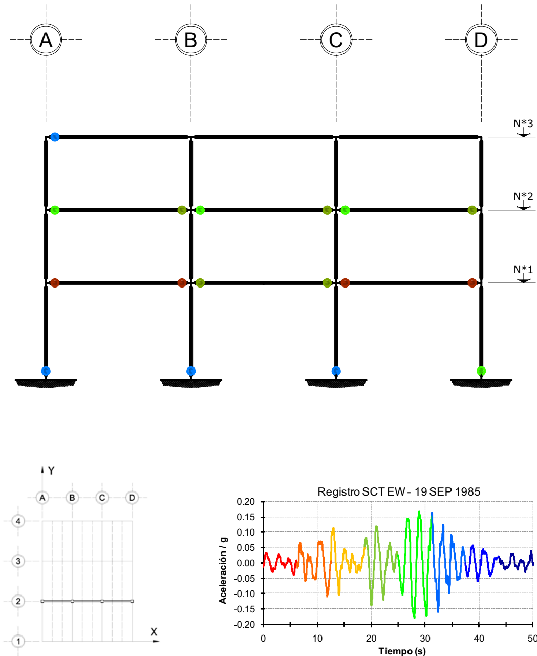
Fig 4.126 Ubicación y secuencia de formación de articulaciones plásticas, análisis paso a paso, resistencias nominales, edificio de 3 niveles, eje 2, caso B2
