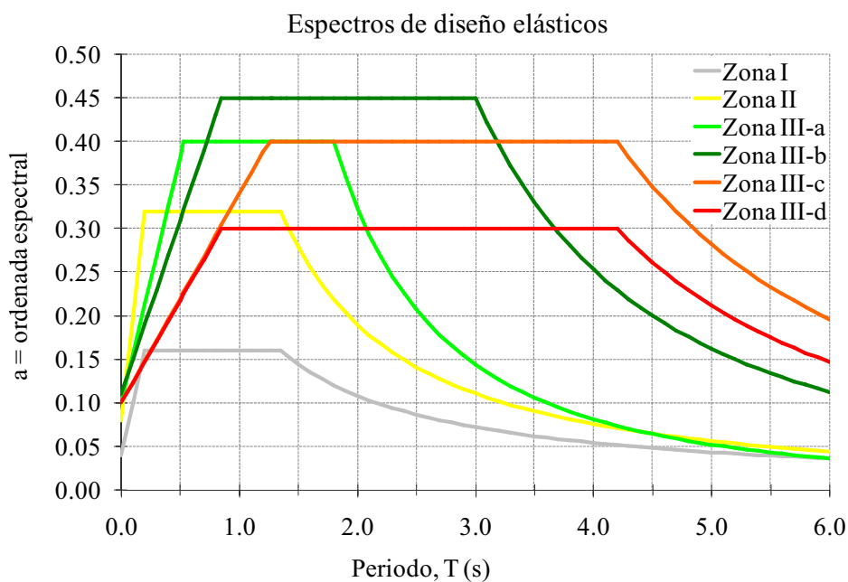
Fig 2.8b Espectros de diseño elásticos correspondientes a las diferentes zonas sísmicas del Valle de México, según el Cuerpo Principal de las NTC-Siismo del RDF-04
