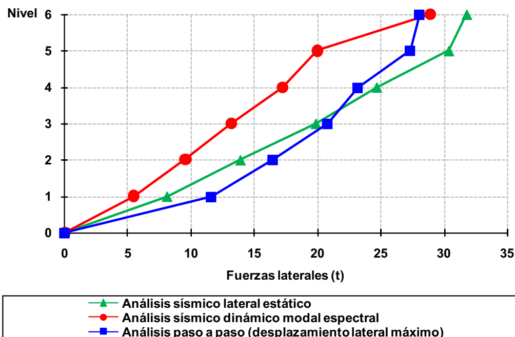
Fig 4.146 Distribución del perfil de fuerzas laterales debidas a diferentes condiciones de análisis sísmico del eje 2, caso C2, (sin sobre-resistencias), diseño según el Apéndice A de las NTC-Sismo del RDF-04, edificio de 6 niveles
