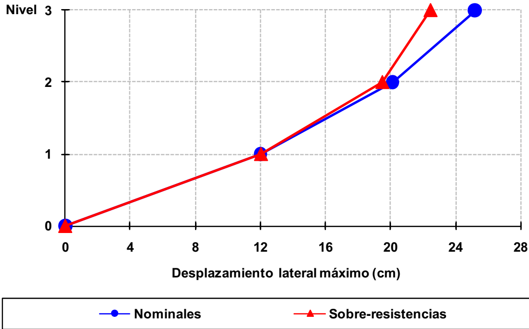
Fig 4.156 Desplazamientos laterales máximos del eje 2, caso B2, análisis Push-over (sin y con sobre-resistencias), perfil de cargas laterales del análisis dinámico modal espectral, diseño Apéndice A, NTC-Sismo del RDF-04, edificio de 3 niveles
