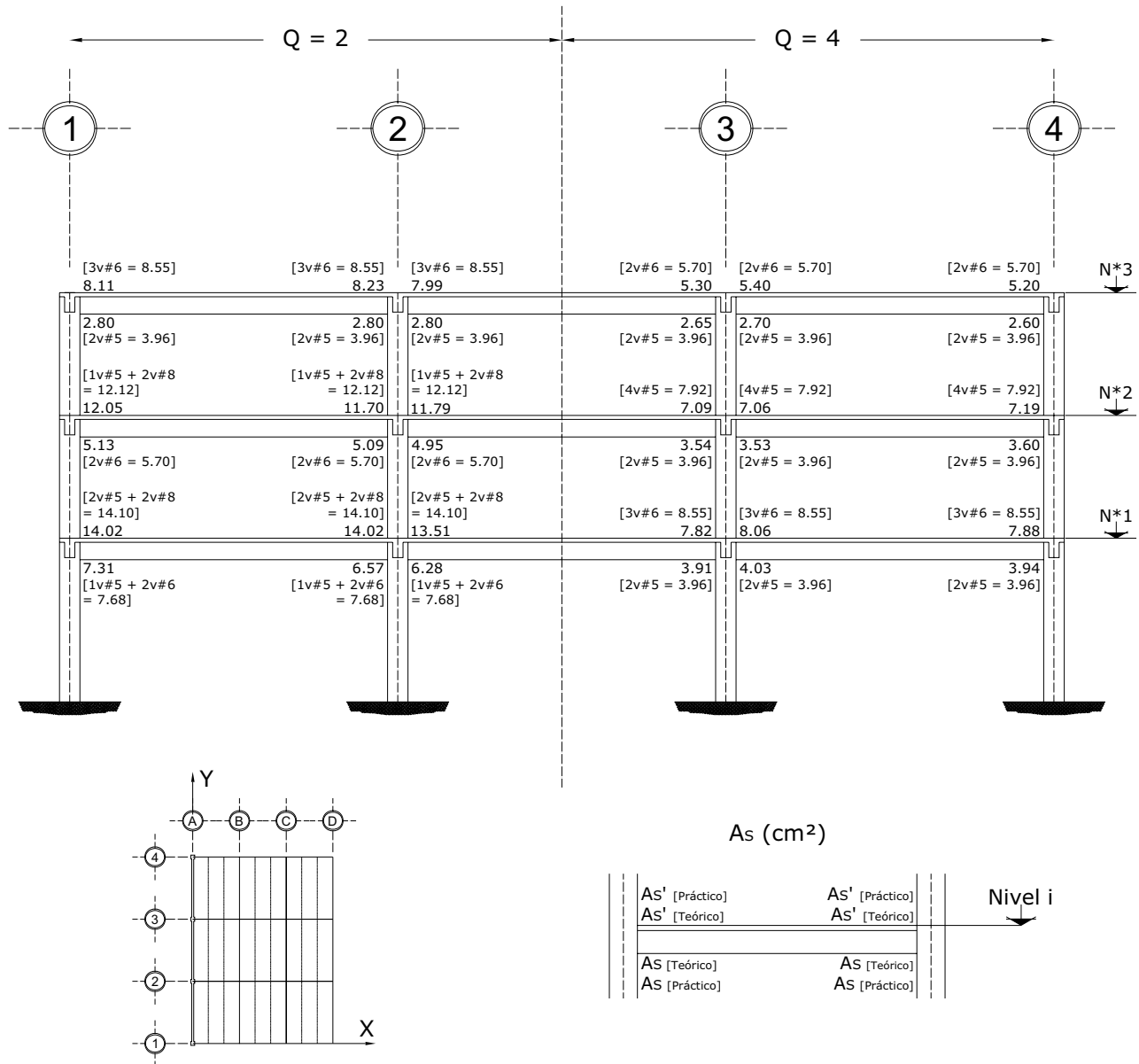
Fig 3.74 Acero de refuerzo longitudinal teórico y práctico necesario en vigas, eje A, casos A2 ( Q = 2 ) y B2 ( Q = 4 )
