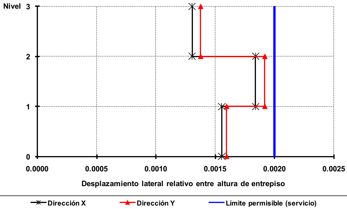
Fig 3.19a Relaciones desplazamiento lateral relativo entre altura de entrepiso (condición de servicio), análisis dinámico modal espectral, edificio de 3 niveles, caso B2 (Q = 4)
