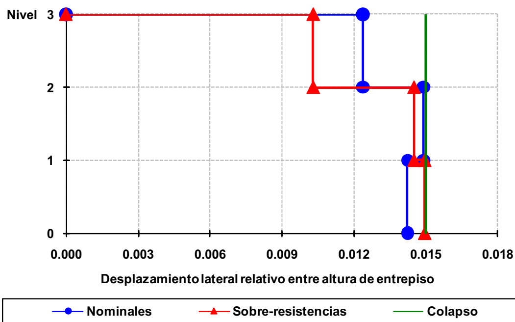
Fig 4.162 Relaciones desplazamiento lateral relativo entre altura de entrepiso del eje 2, caso A2, análisis Push-over (sin y con sobre-resistencias), perfil de cargas laterales del análisis dinámico modal espectral, diseño Apéndice A, NTC-Sismo del RDF-04, edificio de 3 niveles
