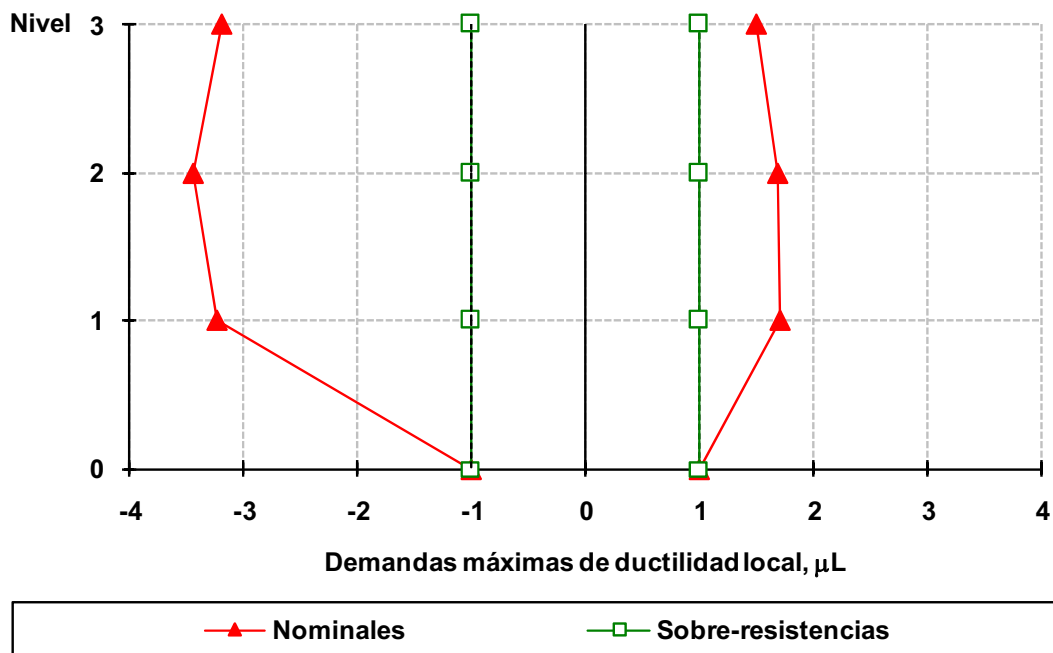
Fig 4.91 Demandas máximas de ductilidad local desarrolladas en vigas del eje A, caso A2, análisis paso a paso elástico e inelástico (sin y con sobre-resistencias), NTC-Sismo del RDF-04, edificio de 3 niveles
