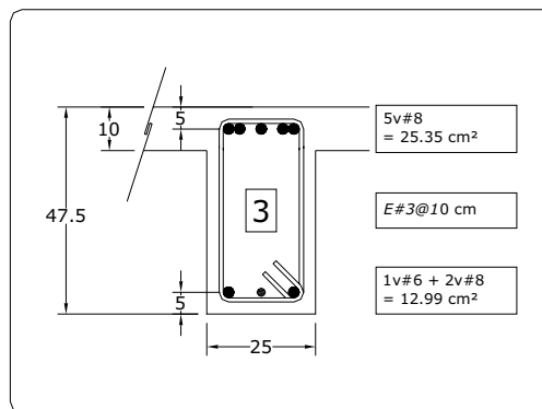
Fig 3.56 Tipos de armados de refuerzo longitudinal y transversal resultantes en los extremos de las vigas del eje 2, caso A1 (Q = 2)
