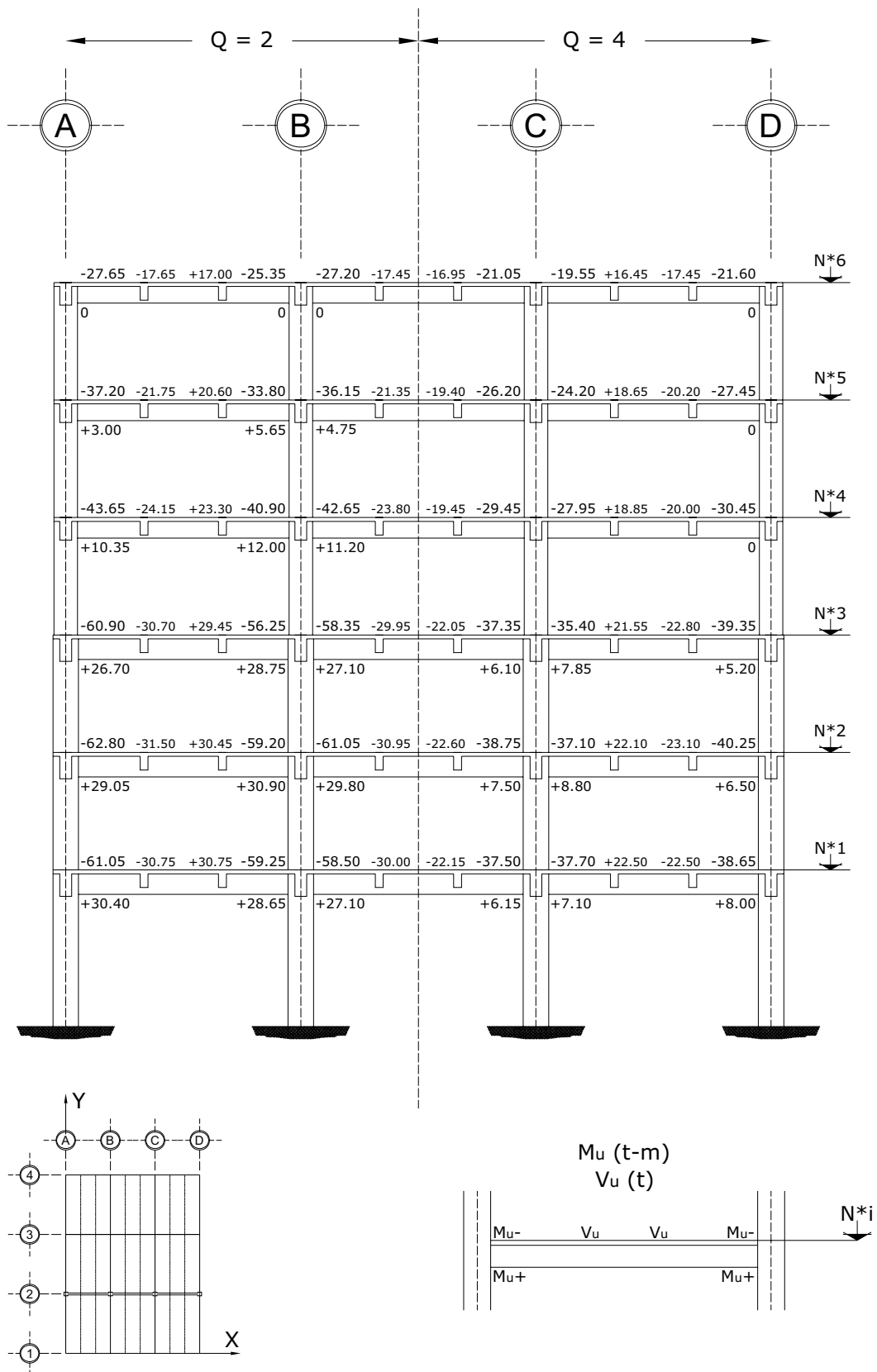
Fig 3.88 Momentos flexionantes y fuerzas cortantes últimos de vigas, eje 2, casos C1 (Q = 2) y D1 (Q = 4)
