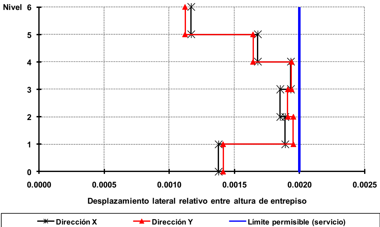
Fig 3.23a Relaciones desplazamiento lateral relativo entre altura de entrepiso (condición de servicio), análisis dinámico modal espectral, edificio de 6 niveles, caso D2 (Q = 4)
