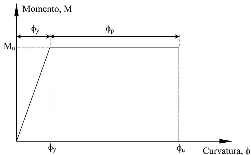
Fig 2.16 Curva idealizada momento-curvatura
