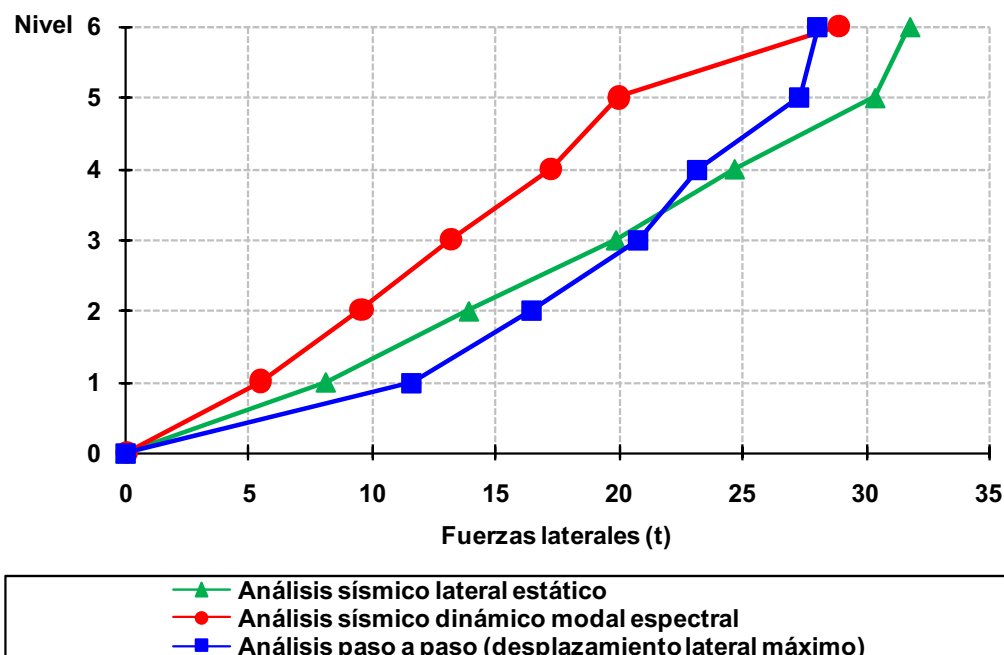
Fig 4.147 Distribución del perfil de fuerzas laterales debidas a diferentes condiciones de análisis sísmico del eje 2, caso C2, (con sobre-resistencias), diseño según el Apéndice A de las NTC-Sismo del RDF-04, edificio de 6 niveles
