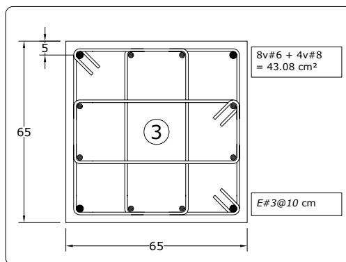
Fig 3.103 Tipos de armados de refuerzo longitudinal y transversal resultantes en los extremos de las columnas del eje A, caso D1 (Q = 4)
