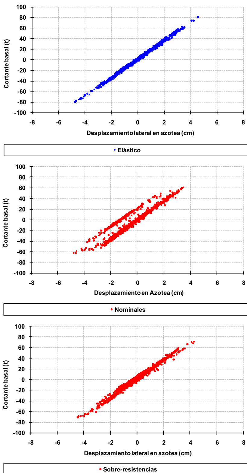
Fig 4.52 Relaciones fuerza cortante basal - desplazamiento horizontal en azotea, eje 2, caso B2, análisis paso a paso elástico e inelástico (sin y con sobre-resistencias), diseño Apéndice A, NTC-Sismo del RDF-04, edificio de 3 niveles
