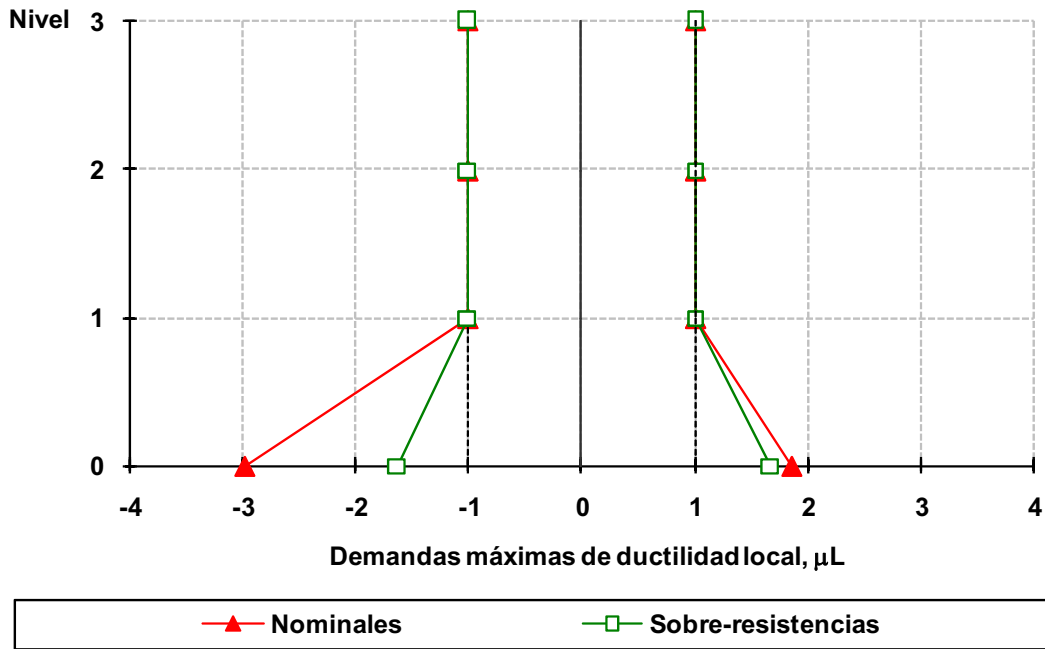
Fig 4.116 Demandas máximas de ductilidad local desarrolladas en columnas del eje 2, caso B2, análisis paso a paso elástico e inelástico (sin y con sobre-resistencias), NTC-Sismo del RDF-04, edificio de 3 niveles
