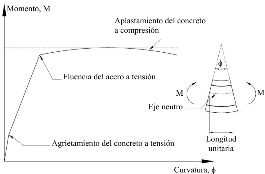
Fig 2.15 Relación típica de momento contra curvatura para un miembro a flexión de concreto reforzado
