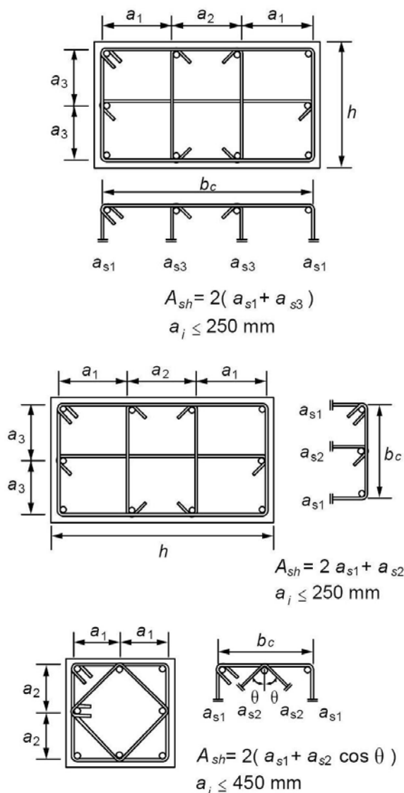
Fig 2.26 Detallado del refuerzo transversal de elementos a flexocompresión
