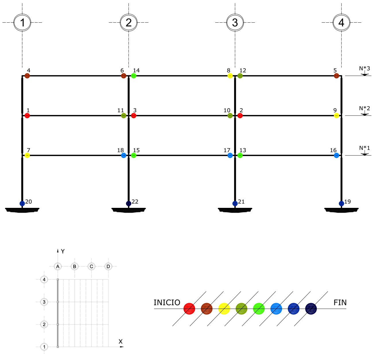
Fig 4.196 Ubicación y secuencia de formación de articulaciones plásticas, análisis Push-over, resistencias nominales, edificio de 3 niveles, eje A, caso A2
