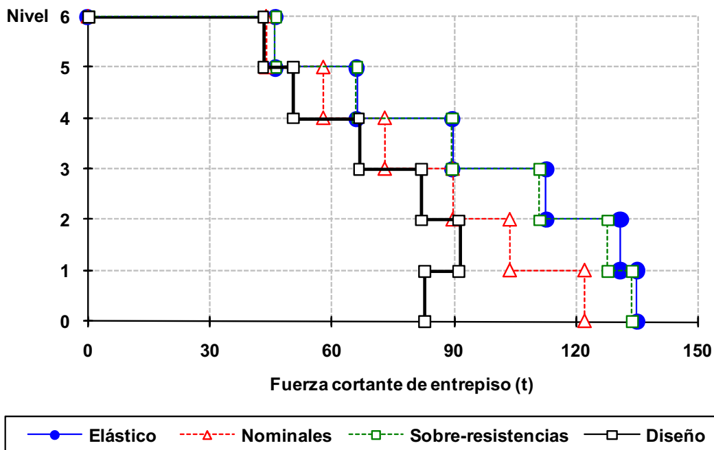
Fig 4.40 Envolventes de fuerzas cortantes de entrepiso del eje 2, caso D2, análisis paso a paso elástico e inelástico (sin y con sobre-resistencias) y modal espectral, NTC-Sismo del RDF-04, edificio de 6 niveles
