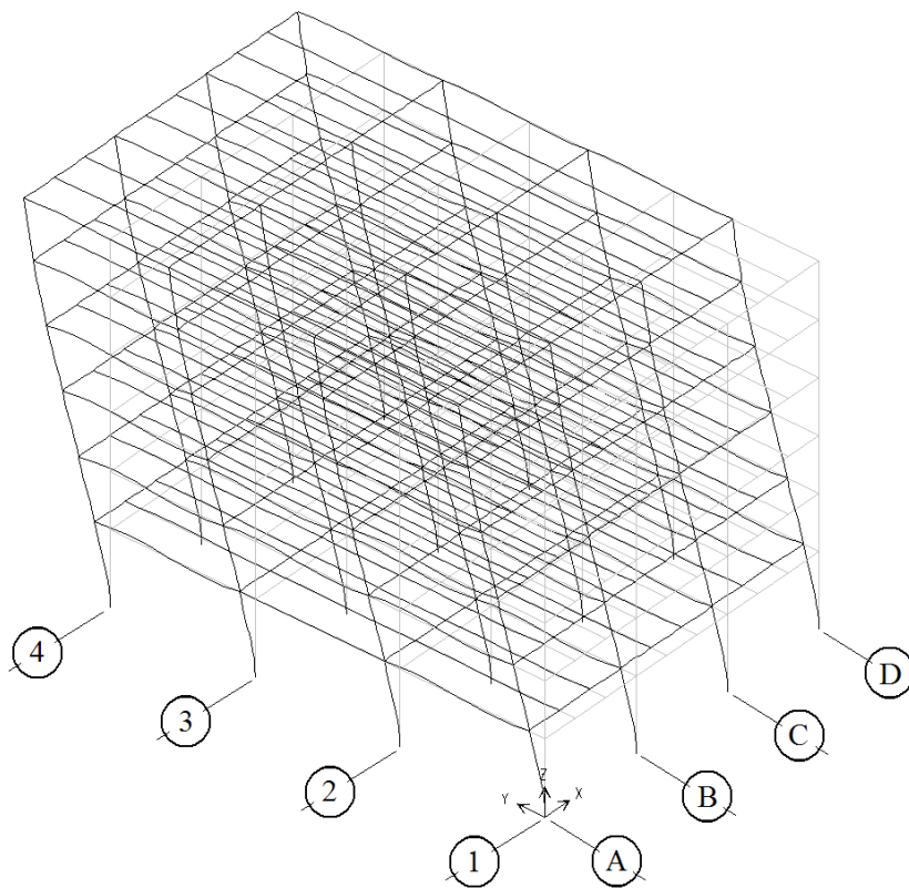
Fig 3.11 Deformada en perspectiva del primer modo de vibración, dirección larga, edificio de 6 niveles
