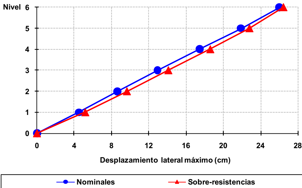
Fig 4.159 Desplazamientos laterales máximos del eje A, caso C2, análisis Push-over (sin y con sobre-resistencias), perfil de cargas laterales del análisis dinámico modal espectral, diseño Apéndice A, NTC-Sismo del RDF-04, edificio de 6 niveles
