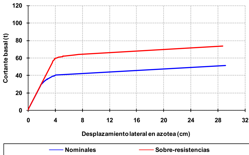
Fig 4.189 Relaciones fuerza cortante basal - desplazamiento horizontal en azotea, eje A, caso B2, análisis Push-over (sin y con sobre-resistencias), perfil de cargas laterales del análisis dinámico modal espectral, diseño Apéndice A, NTC-Sismo del RDF-04, edificio de 3 niveles
