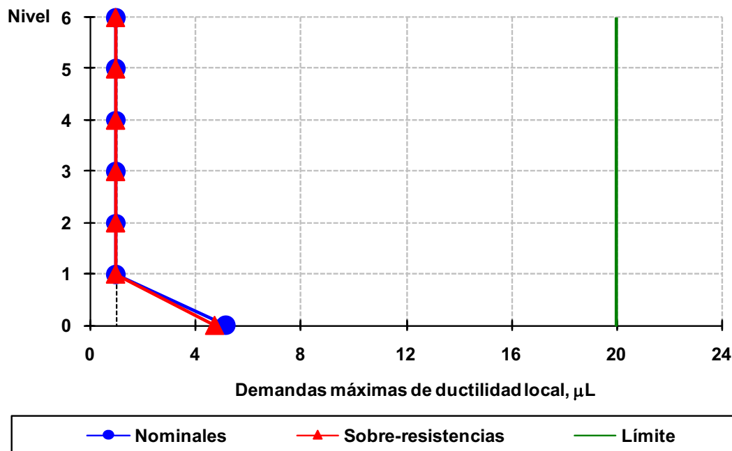
Fig 4.183 Demandas máximas de ductilidad local desarrolladas en columnas del eje A, caso C2, análisis Push-over (sin y con sobre-resistencias), perfil de cargas laterales del análisis dinámico modal espectral, diseño Apéndice A, NTC-Sismo del RDF-04, edificio de 6 niveles
