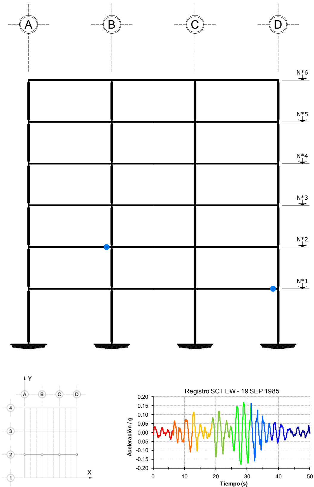
Fig 4.130 Ubicación y secuencia de formación de articulaciones plásticas, análisis paso a paso, resistencias nominales, edificio de 6 niveles, eje 2, caso C2
