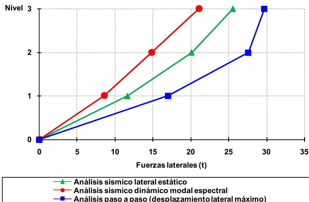
Fig 4.138 Distribución del perfil de fuerzas laterales debidas a diferentes condiciones de análisis sísmico del eje 2, caso A2, (sin sobre-resistencias), diseño según el Apéndice A de las NTC-Sismo del RDF-04, edificio de 3 niveles
