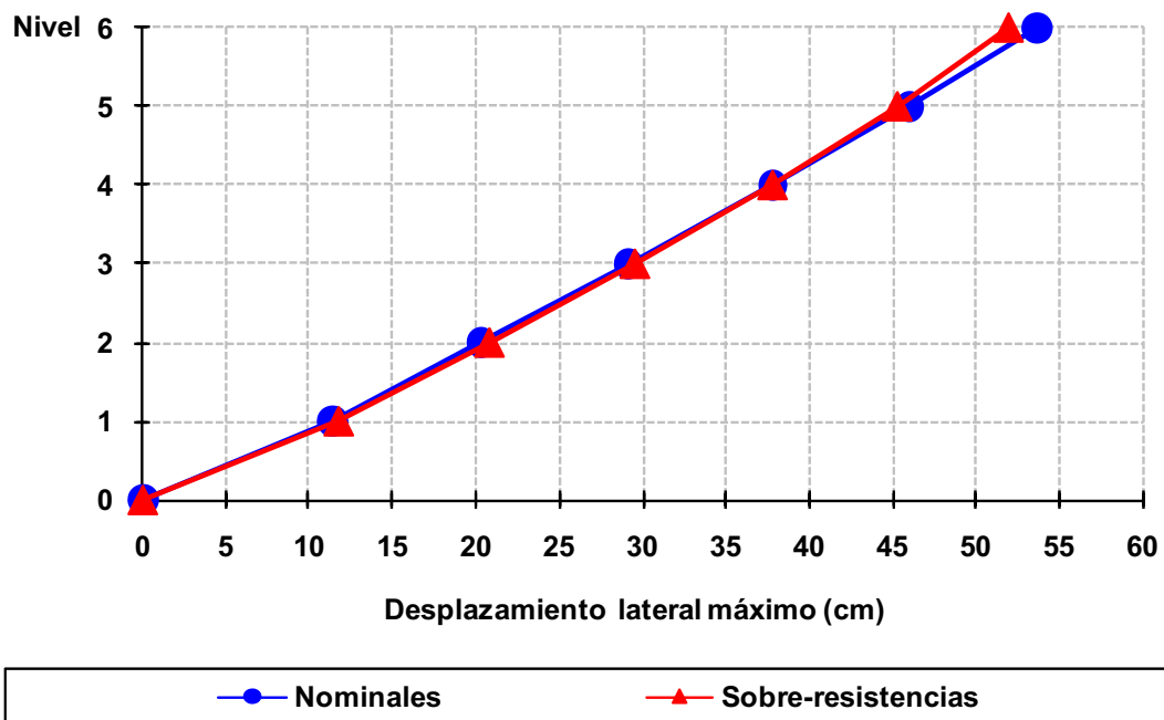
Fig 4.161 Desplazamientos laterales máximos del eje A, caso D2, análisis Push-over (sin y con sobre-resistencias), perfil de cargas laterales del análisis dinámico modal espectral, diseño Apéndice A, NTC-Sismo del RDF-04, edificio de 6 niveles
