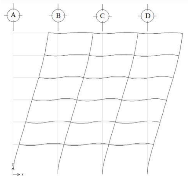
Fig 3.12 Deformada en elevación del primer modo de vibración, dirección corta, edificio de 6 niveles
