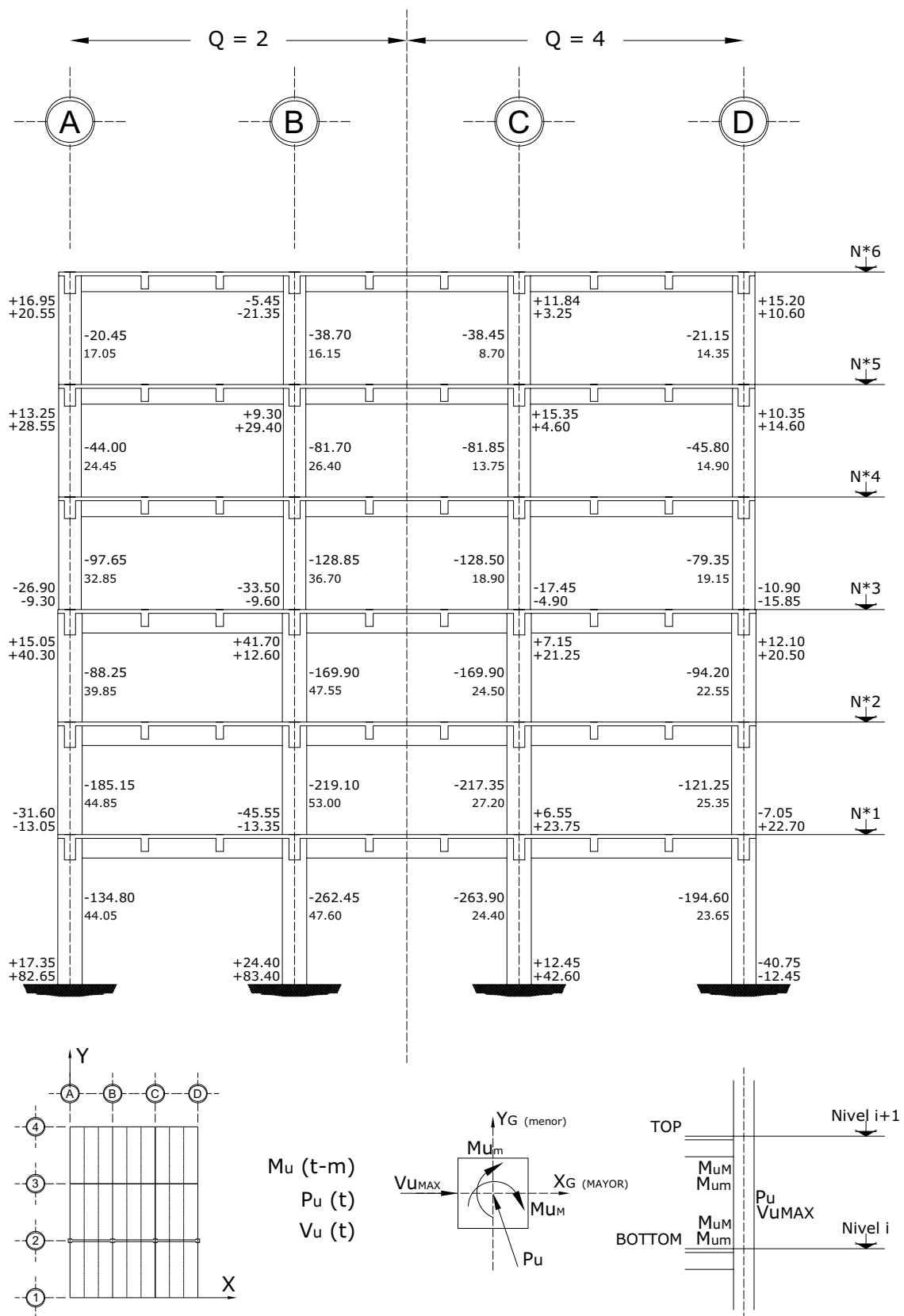
Fig 3.89 Elementos mecánicos últimos en columnas, eje 2, casos C1 ( Q = 2 ) y D1 ( Q = 4 )
