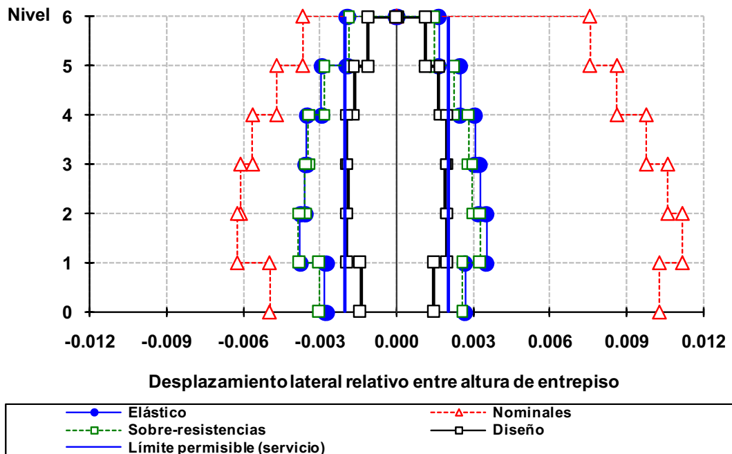
Fig 4.33 Relaciones desplazamiento lateral relativo entre altura de entrepiso del eje A, caso D2, análisis paso a paso elástico e inelástico (sin y con sobre-resistencias) y modal espectral, NTC-Sismo del RDF-04, edificio de 6 niveles
