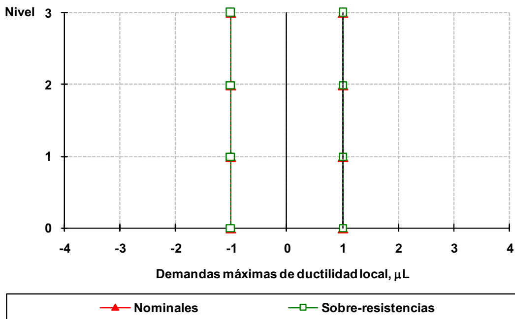
Fig 4.115 Demandas máximas de ductilidad local desarrolladas en columnas del eje A, caso A2, análisis paso a paso elástico e inelástico (sin y con sobre-resistencias), NTC-Sismo del RDF-04, edificio de 3 niveles
