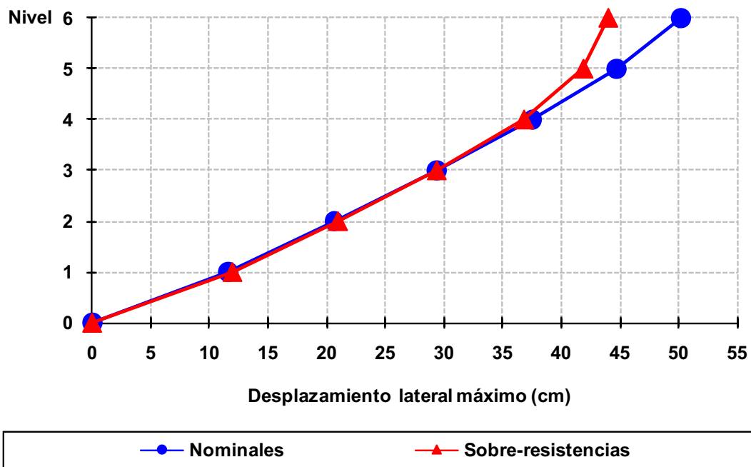
Fig 4.160 Desplazamientos laterales máximos del eje 2, caso D2, análisis Push-over (sin y con sobre-resistencias), perfil de cargas laterales del análisis dinámico modal espectral, diseño Apéndice A, NTC-Sismo del RDF-04, edificio de 6 niveles
