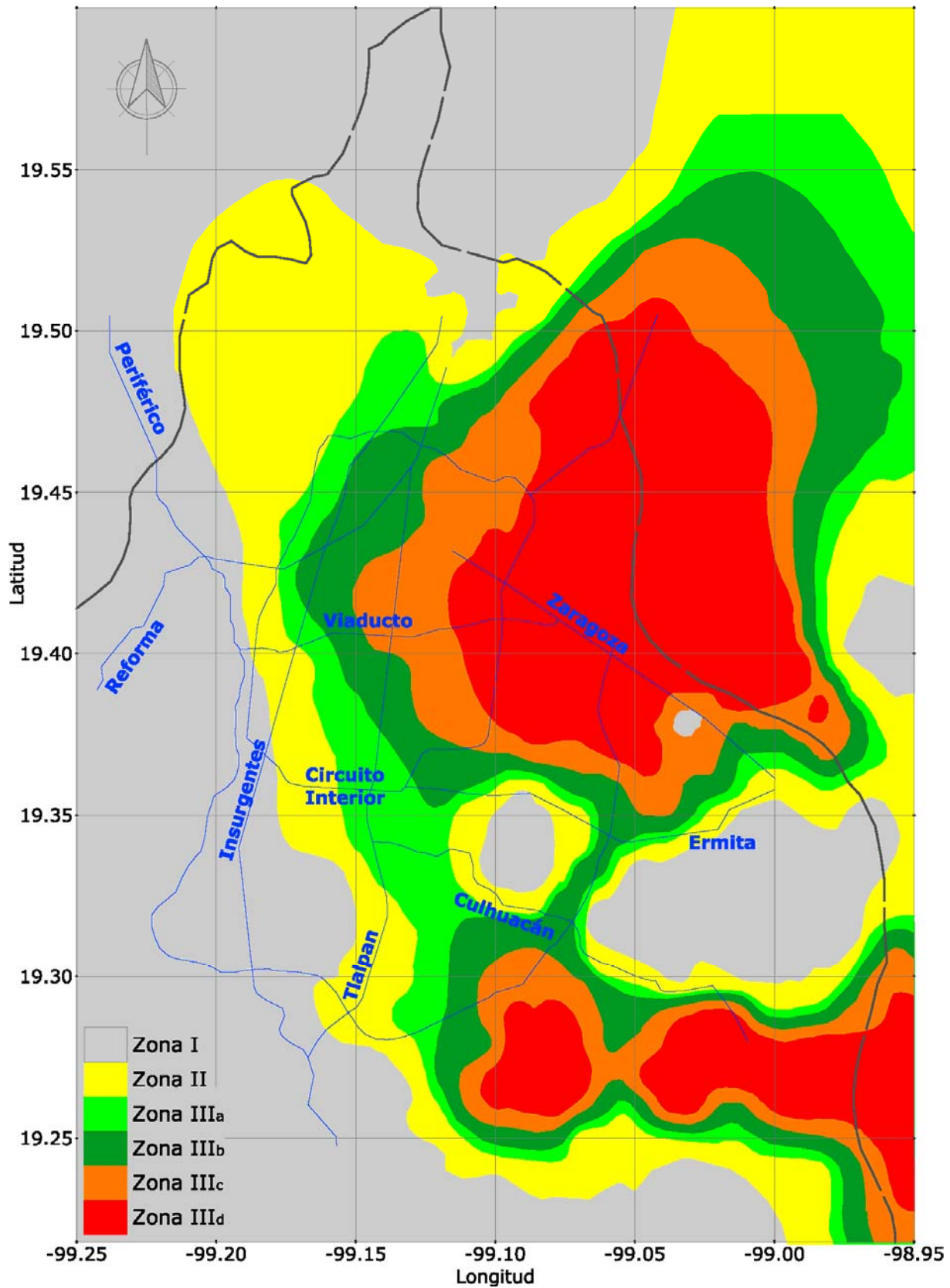
Fig 2.7 Zonificación de la ciudad de México para fines de diseño por sismo, según el Cuerpo Principal de las NTC-Sismo del RDF-04
