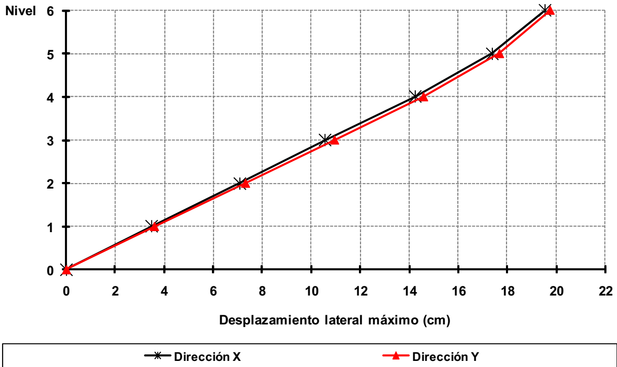
Fig 3.29b Desplazamientos laterales máximos, análisis dinámico modal espectral (condición de colapso), edificio de 6 niveles, caso C2 ( Q = 2 )
