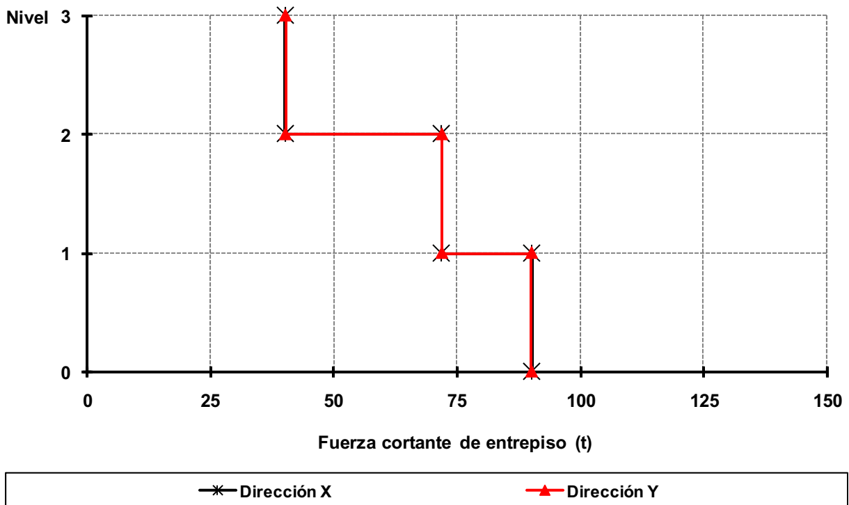
Fig 3.35 Fuerzas cortantes de entrepiso, análisis dinámico modal espectral, edificio de 3 niveles, caso B2 (Q = 4)
