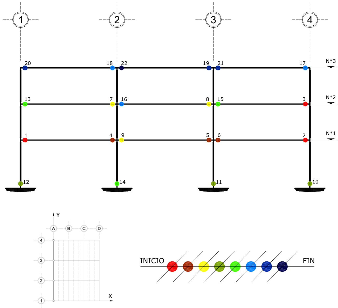
Fig 4.201 Ubicación y secuencia de formación de articulaciones plásticas, análisis Push-over, con sobre-resistencias, edificio de 3 niveles, eje A, caso B2
