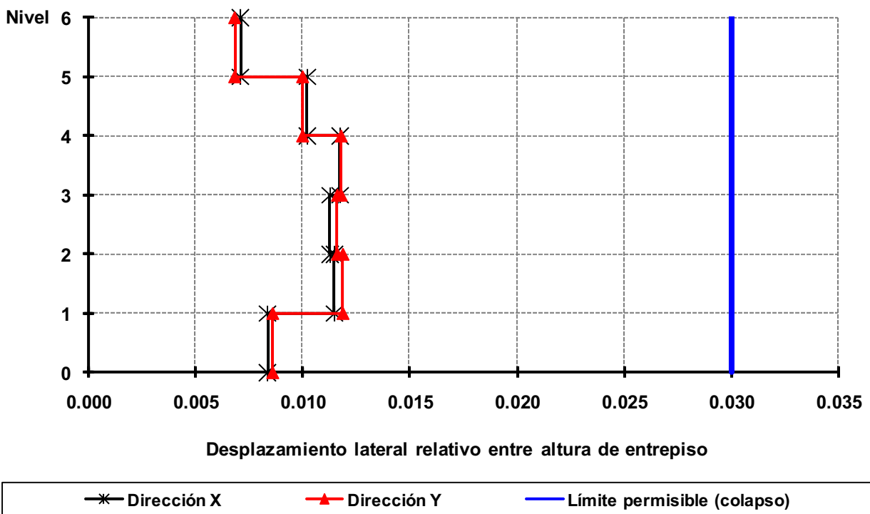
Fig 3.23b Relaciones desplazamiento lateral relativo entre altura de entrepiso (condición de colapso), análisis dinámico modal espectral, edificio de 6 niveles, caso D2 (Q = 4)
