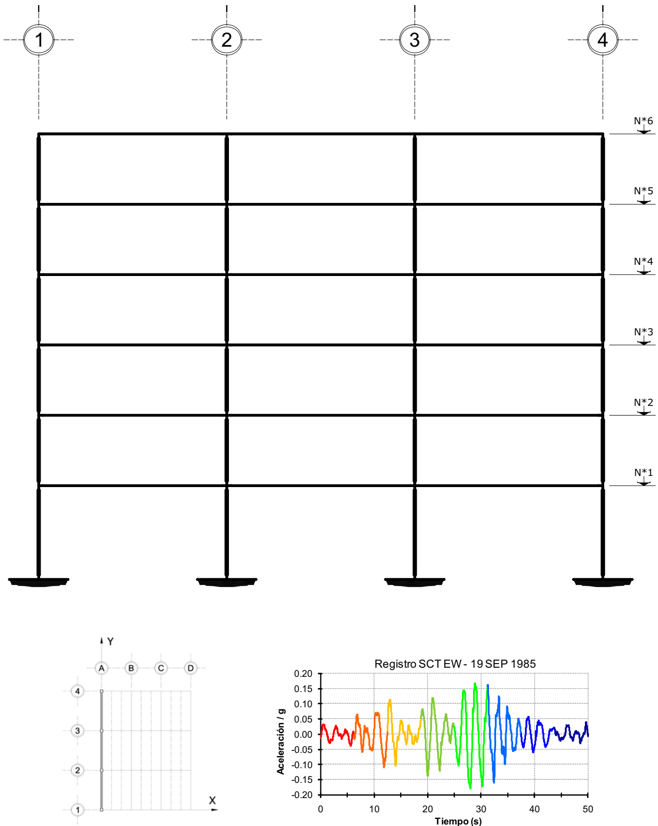
Fig 4.133 Ubicación y secuencia de formación de articulaciones plásticas, análisis paso a paso, con sobre-resistencias, edificio de 6 niveles, eje A, caso C2
