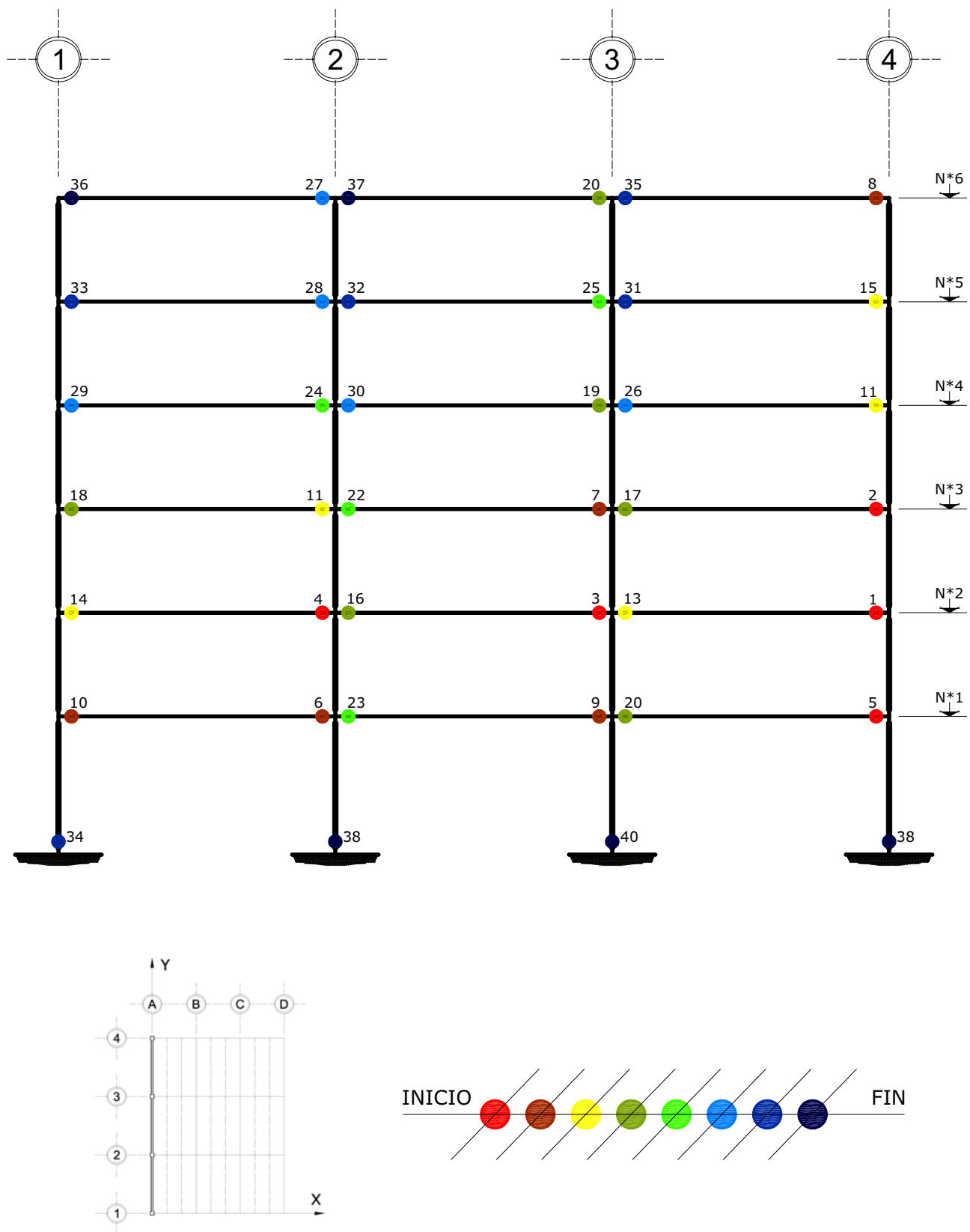
Fig 4.208 Ubicación y secuencia de formación de articulaciones plásticas, análisis Push-over, resistencias nominales, edificio de 6 niveles, eje A, caso D2
