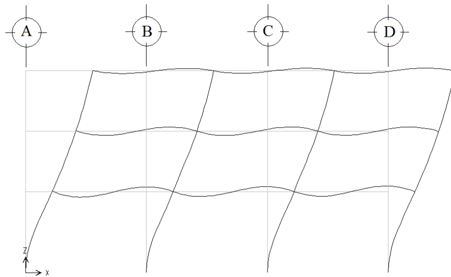
Fig 3.6 Deformada en elevación del primer modo de vibración, dirección corta, edificio de 3 niveles
