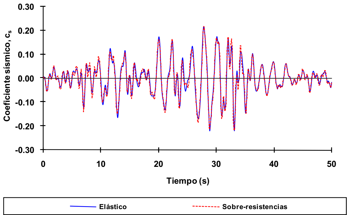
Fig 4.49 Historias de coeficientes sísmicos ( c_s ), eje A, caso D2, análisis paso a paso elástico e inelástico (sin y con sobre-resistencias), diseño Apéndice A, NTC-Sismo del RDF-04, edificio de 6 niveles
