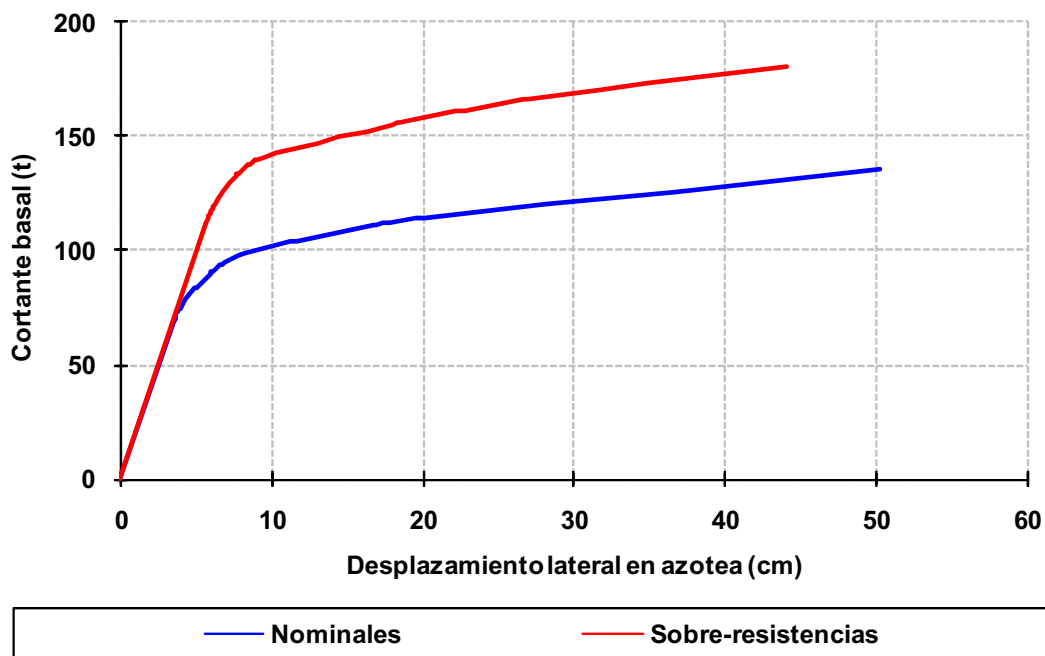
Fig 4.192 Relaciones fuerza cortante basal - desplazamiento horizontal en azotea, eje 2, caso D2, análisis Push-over (sin y con sobre-resistencias), perfil de cargas laterales del análisis dinámico modal espectral, diseño Apéndice A, NTC-Sismo del RDF-04, edificio de 6 niveles
