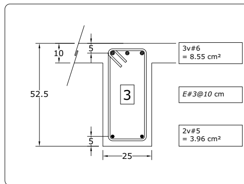
Fig 3.82 Tipos de armados de refuerzo longitudinal y transversal resultantes en los extremos de las vigas del eje A, caso B2 (Q = 4)
