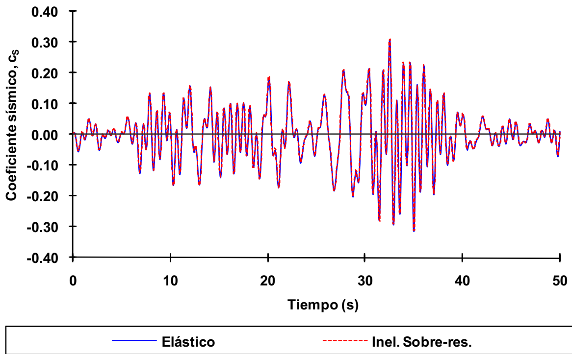
Fig 4.43 Historias de coeficientes sísmicos ( c_s ), eje A, caso A2, análisis paso a paso elástico e inelástico (sin y con sobre-resistencias), diseño Apéndice A, NTC-Sismo del RDF-04, edificio de 3 niveles
