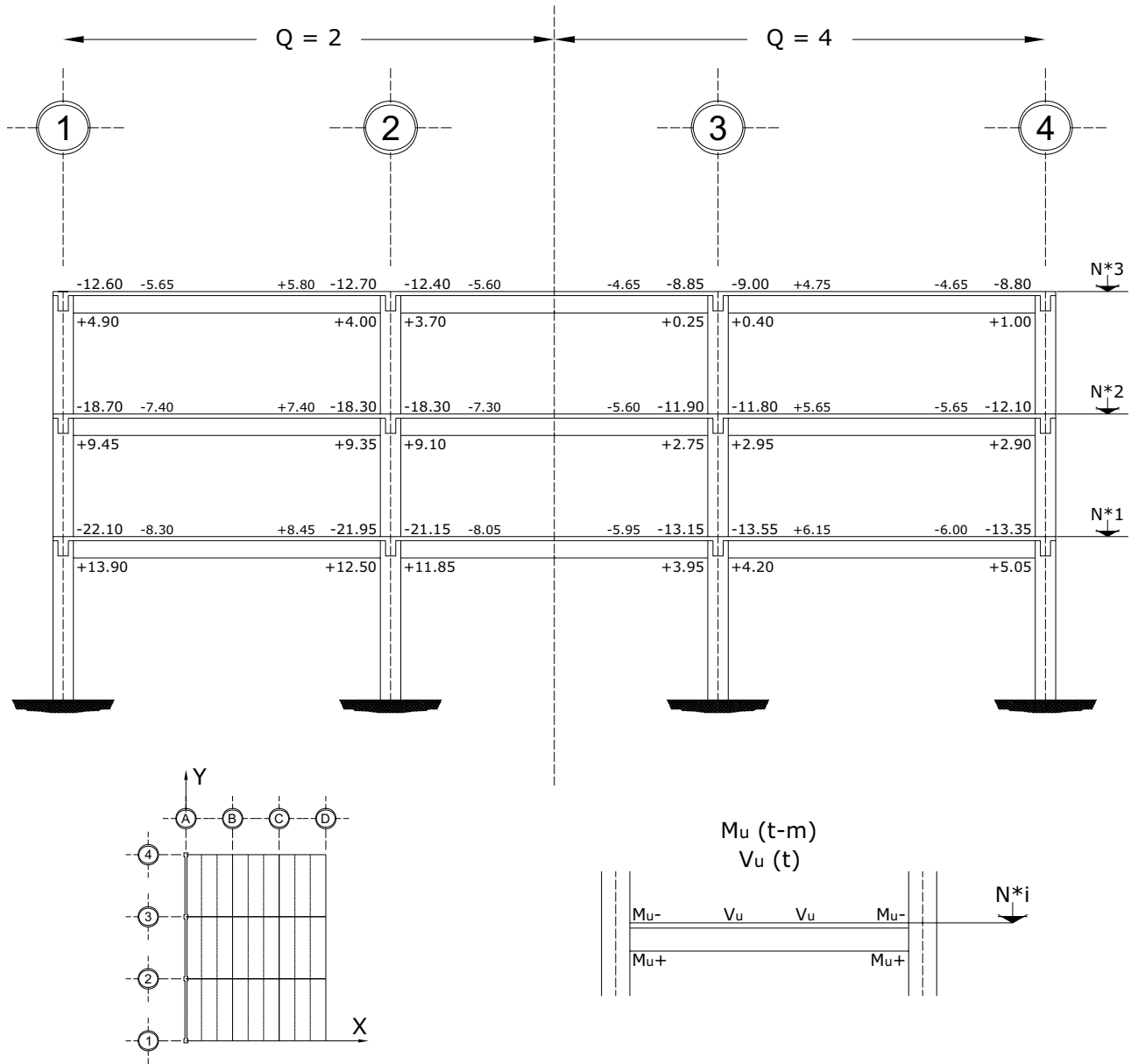
Fig 3.50 Momentos flexionantes y fuerzas cortantes últimos de vigas, eje A, casos A1 (Q = 2) y B1 (Q = 4)
