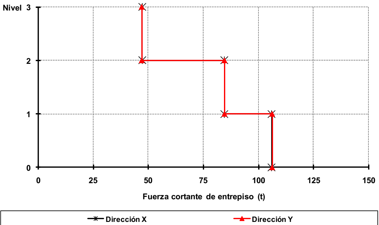
Fig 3.34 Fuerzas cortantes de entrepiso, análisis dinámico modal espectral, edificio de 3 niveles, caso B1 (Q = 4)
