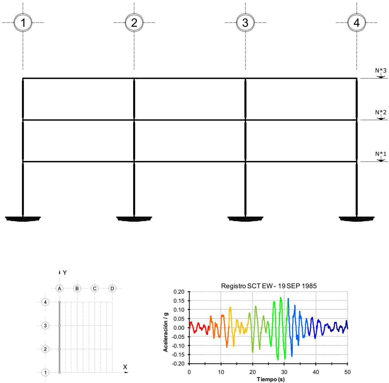
Fig 4.125 Ubicación y secuencia de formación de articulaciones plásticas, análisis paso a paso, con sobre-resistencias, edificio de 3 niveles, eje A, caso A2
