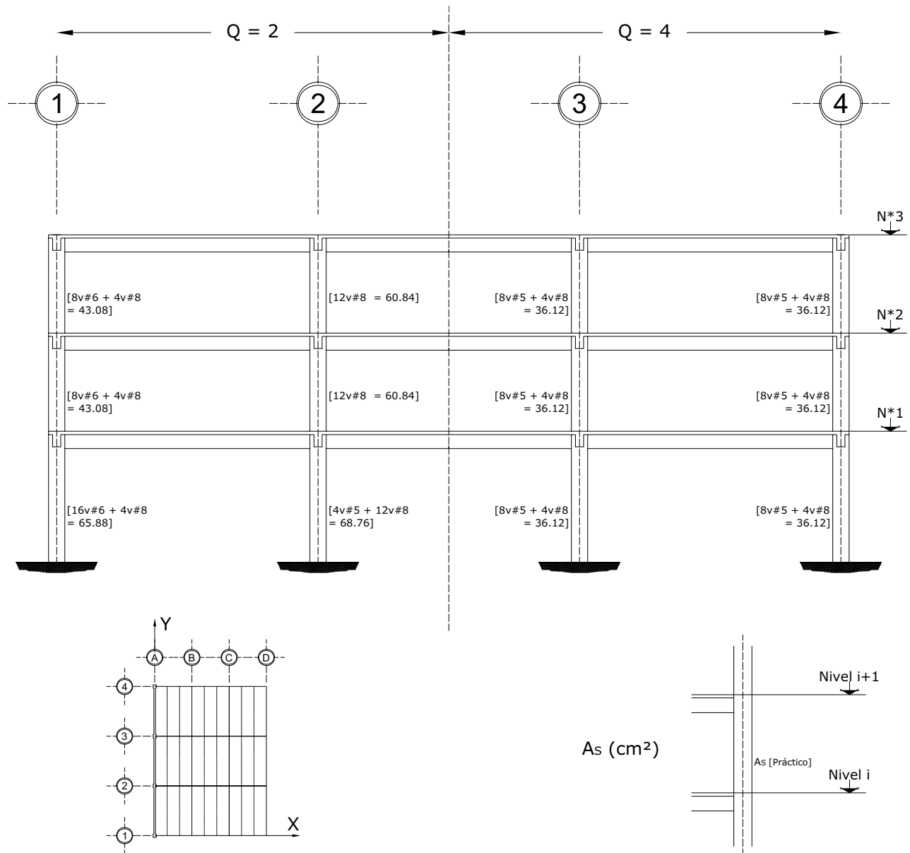
Fig 3.55b Acero de refuerzo longitudinal teórico y práctico necesario en columnas, eje A, casos A1 ( Q = 2 ) y B1 ( Q = 4 )
