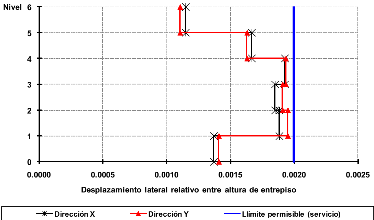
Fig 3.21a Relaciones desplazamiento lateral relativo entre altura de entrepiso (condición de servicio), análisis dinámico modal espectral, edificio de 6 niveles, caso C2 ( Q = 2 )
