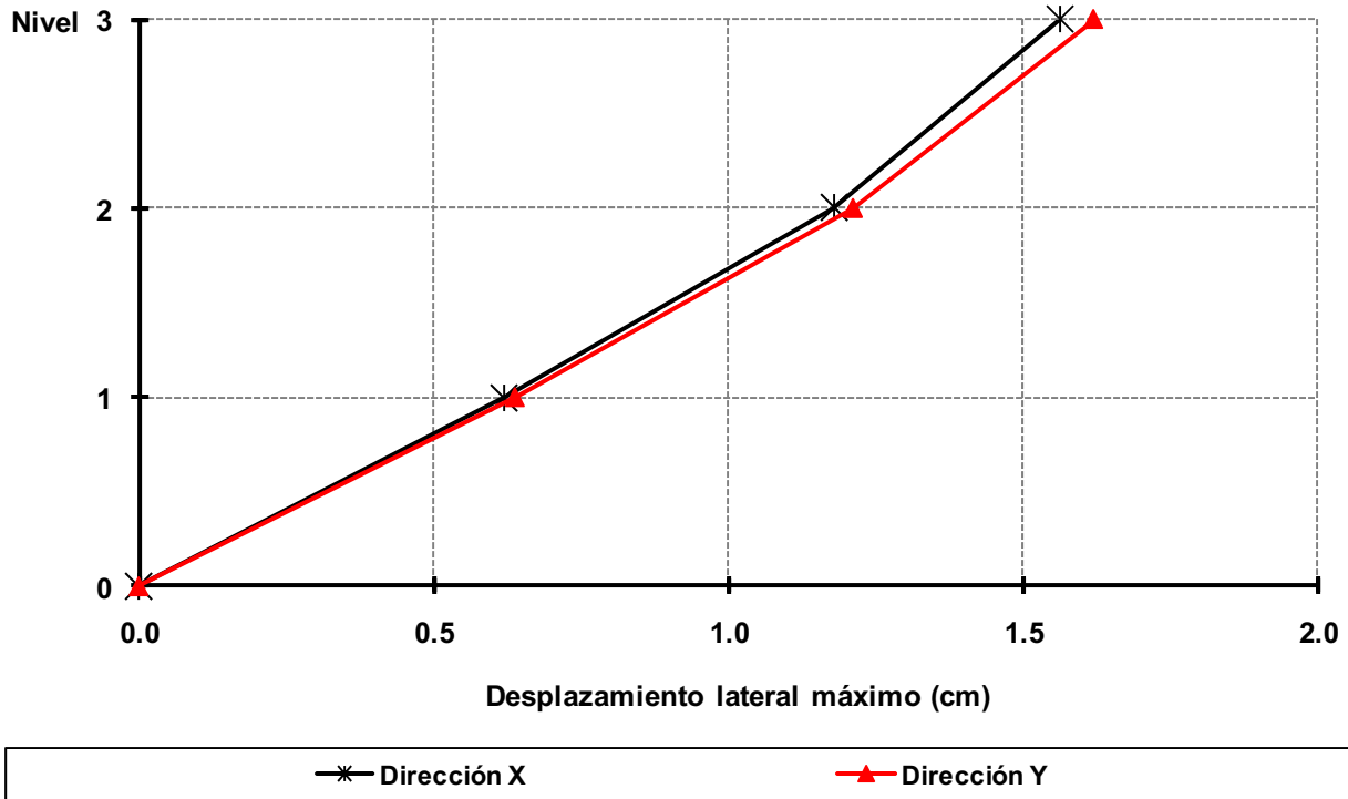
Fig 3.25a Desplazamientos laterales máximos, análisis dinámico modal espectral (condición de servicio), edificio de 3 niveles, caso A2 ( Q = 2 )
