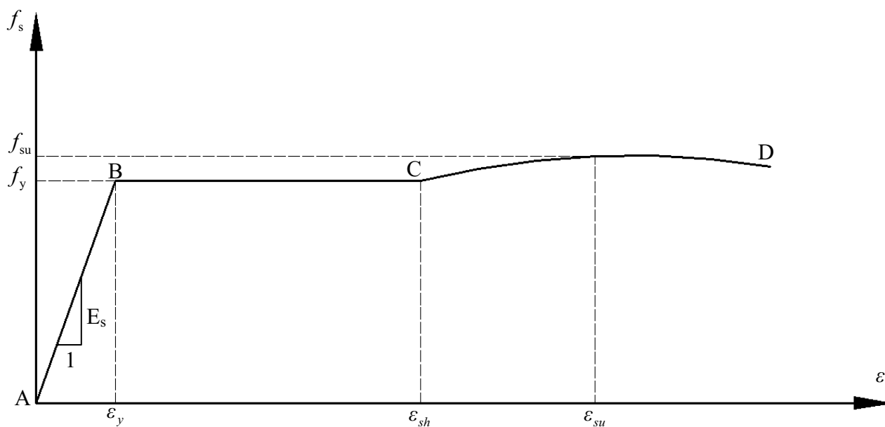
Fig 2.21 Gráfica esfuerzo-deformación EPD
