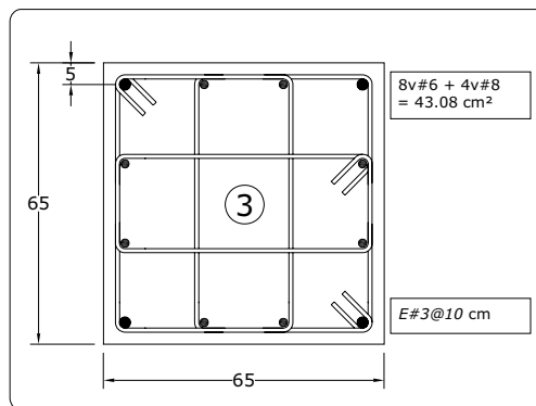
Fig 3.101 Tipos de armados de refuerzo longitudinal y transversal resultantes en los extremos de las columnas del eje 2, caso D1 (Q = 4)
