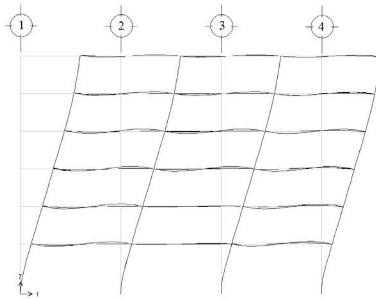
Fig 3.10 Deformada en elevación del primer modo de vibración, dirección larga, edificio de 6 niveles
