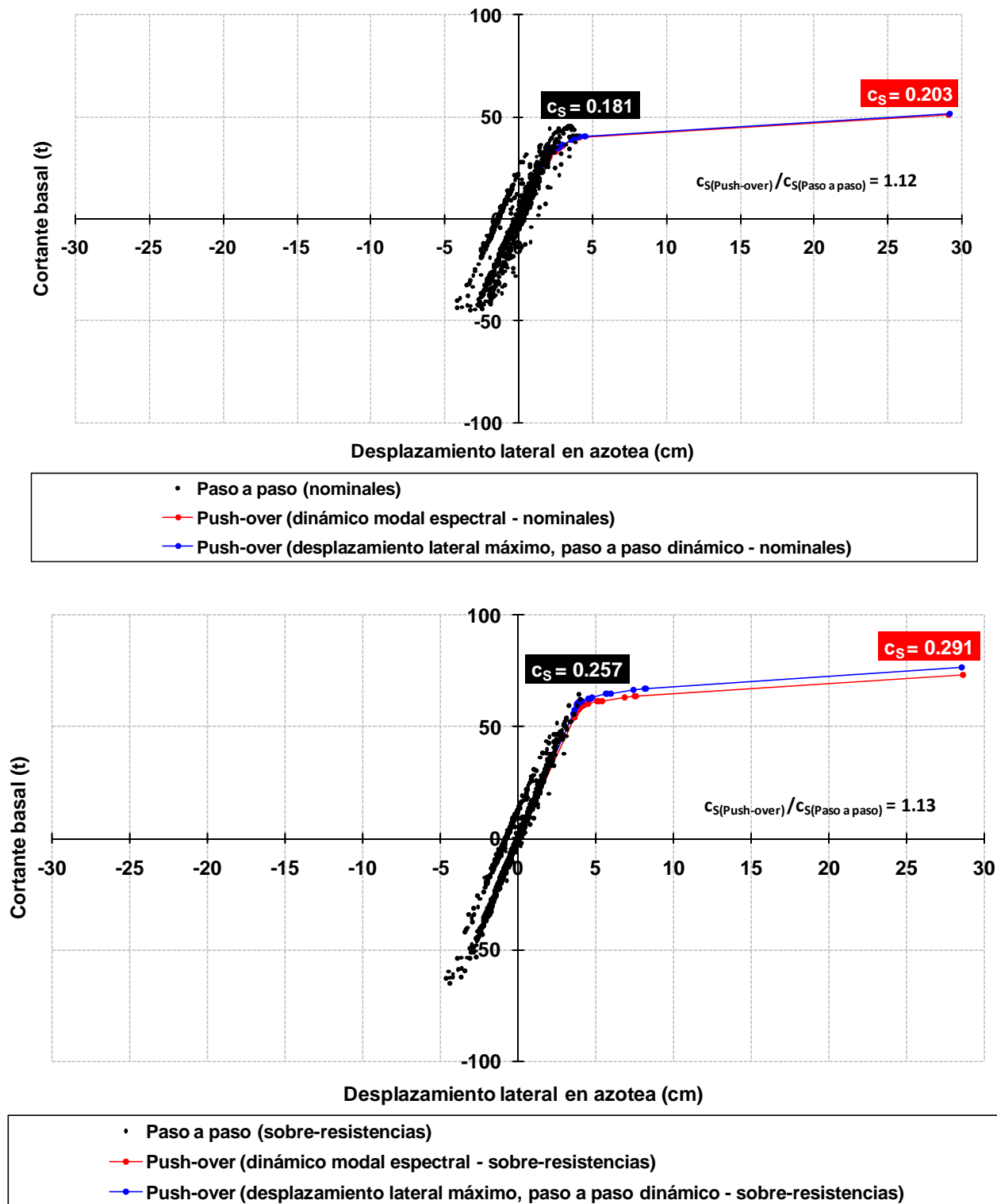
Fig 5.7 Comparación de las curvas fuerza cortante basal - desplazamiento lateral de azotea de los análisis dinámico inelástico paso a paso (con el registro SCT EW-85) y estático no-lineal Push-over (con el perfil de cargas laterales del análisis dinámico modal espectral y del dinámico inelástico paso a paso cuando ocurre el desplazamiento lateral máximo), sin y con sobre-resistencias, caso B2 del eje A del edificio de 3 niveles
