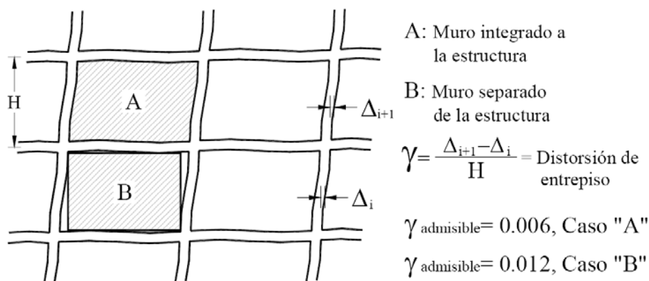
Fig 2.13 Valores permisibles de distorsiones angulares de entrepiso, según el Cuerpo Principal de las NTC-Sismo del RDF-04
