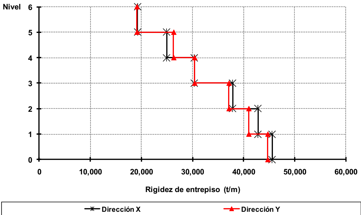
Fig 3.47 Rigideces de entrapiso, edificio 6 niveles, caso D2 (Q = 4)
