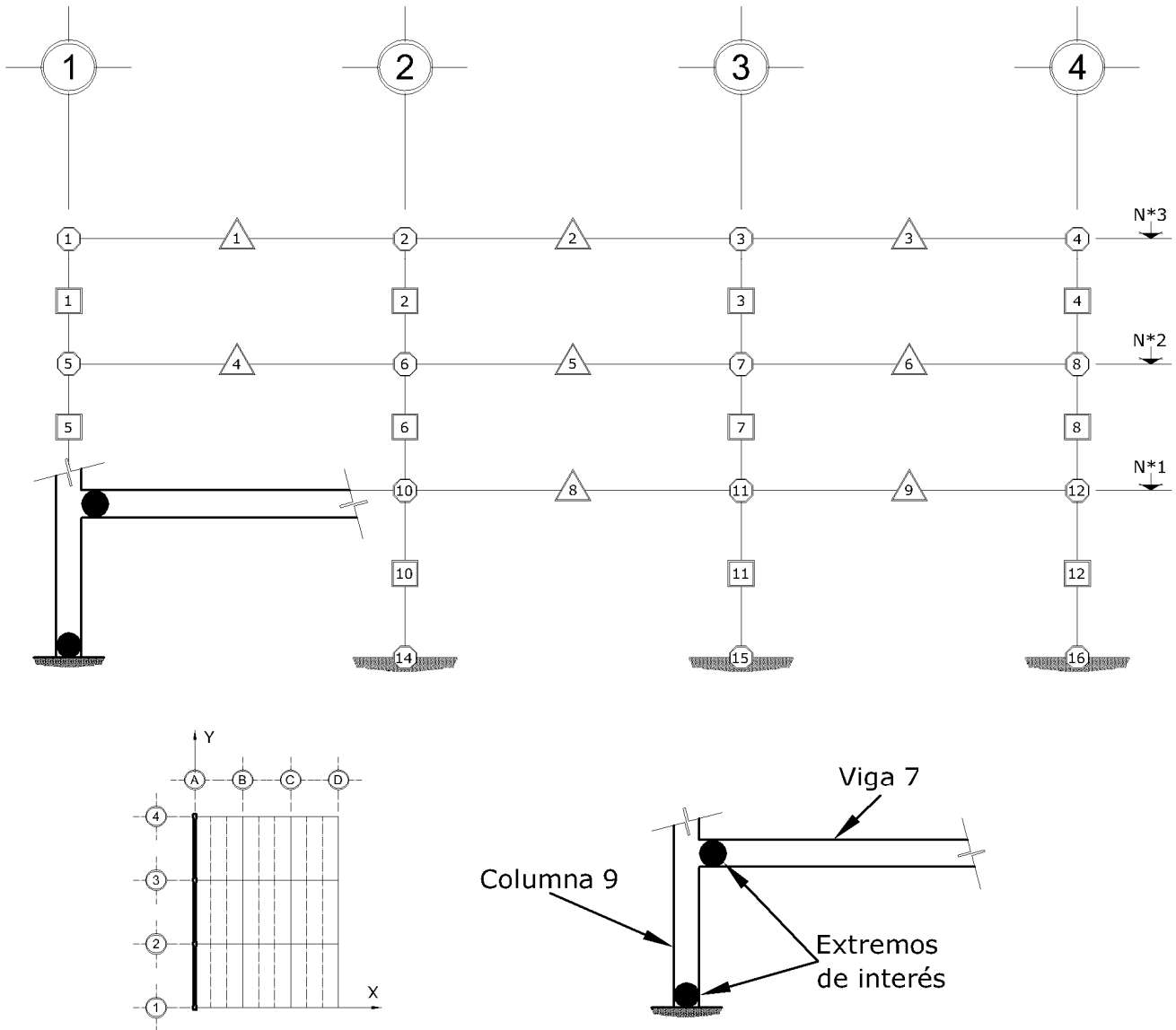
Fig 4.7 Identificación de los extremos en secciones estructurales de la viga 7 y la columna 9 para el estudio de las historias en el tiempo de las respuestas de los análisis paso a paso elásticos e inelásticos (sin y con sobre-resistencias), edificios de 3 niveles, eje A (dirección larga), casos A1 y A2 ( Q = 2 ), B1 y B2 ( Q = 4 )
