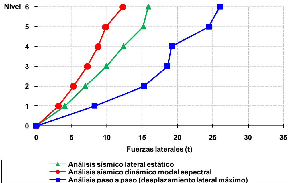
Fig 4.153 Distribución del perfil de fuerzas laterales debidas a diferentes condiciones de análisis sísmico del eje A, caso D2, (con sobre-resistencias), diseño según el Apéndice A de las NTC-Sismo del RDF-04, edificio de 6 niveles
