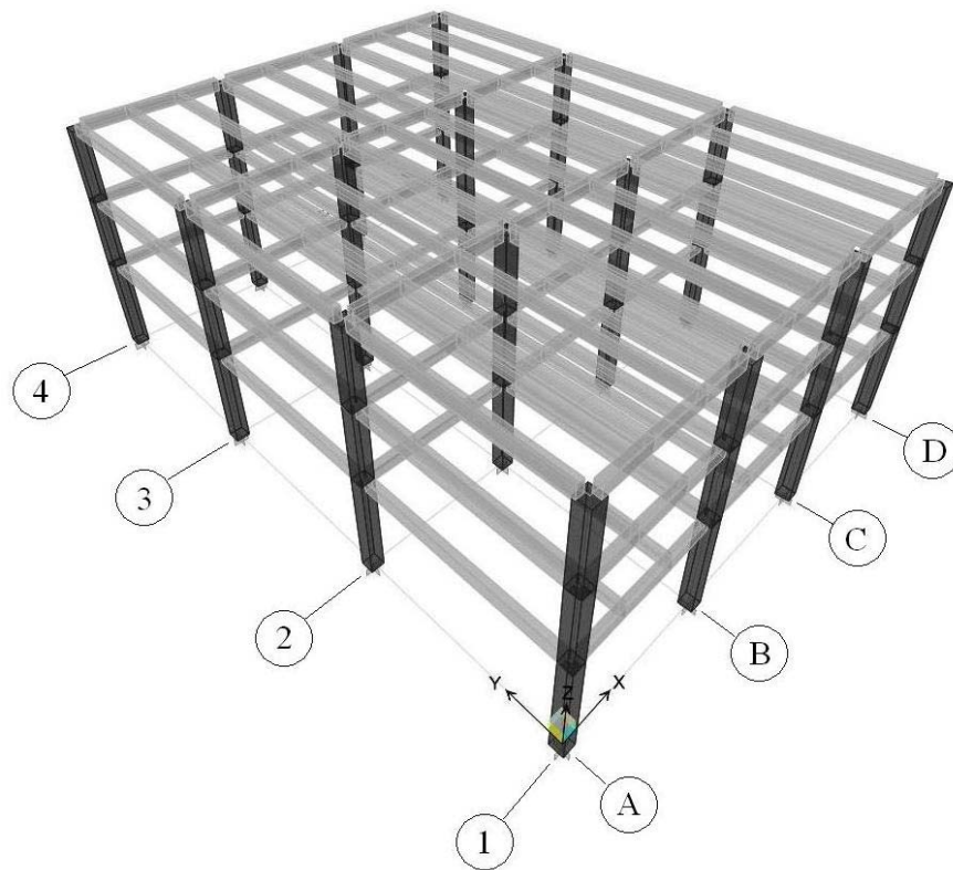
Fig 3.2 Modelo estructural del edificio de 3 niveles, casos A1, A2, B1 y B2
