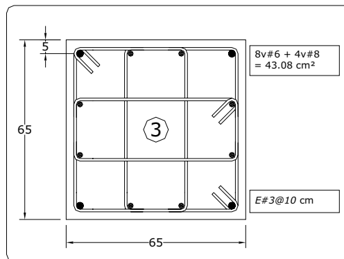
Fig 3.121 Tipos de armados de refuerzo longitudinal y transversal resultantes en los extremos de las columnas de 1 eje 2, caso D2 (Q = 4)
