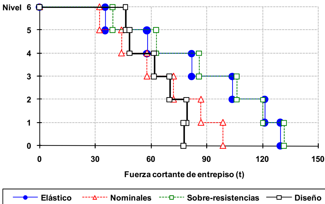
Fig 4.41 Envolventes de fuerzas cortantes de entrepiso del eje A, caso D2, análisis paso a paso elástico e inelástico (sin y con sobre-resistencias) y modal espectral, NTC-Sismo del RDF-04, edificio de 6 niveles
