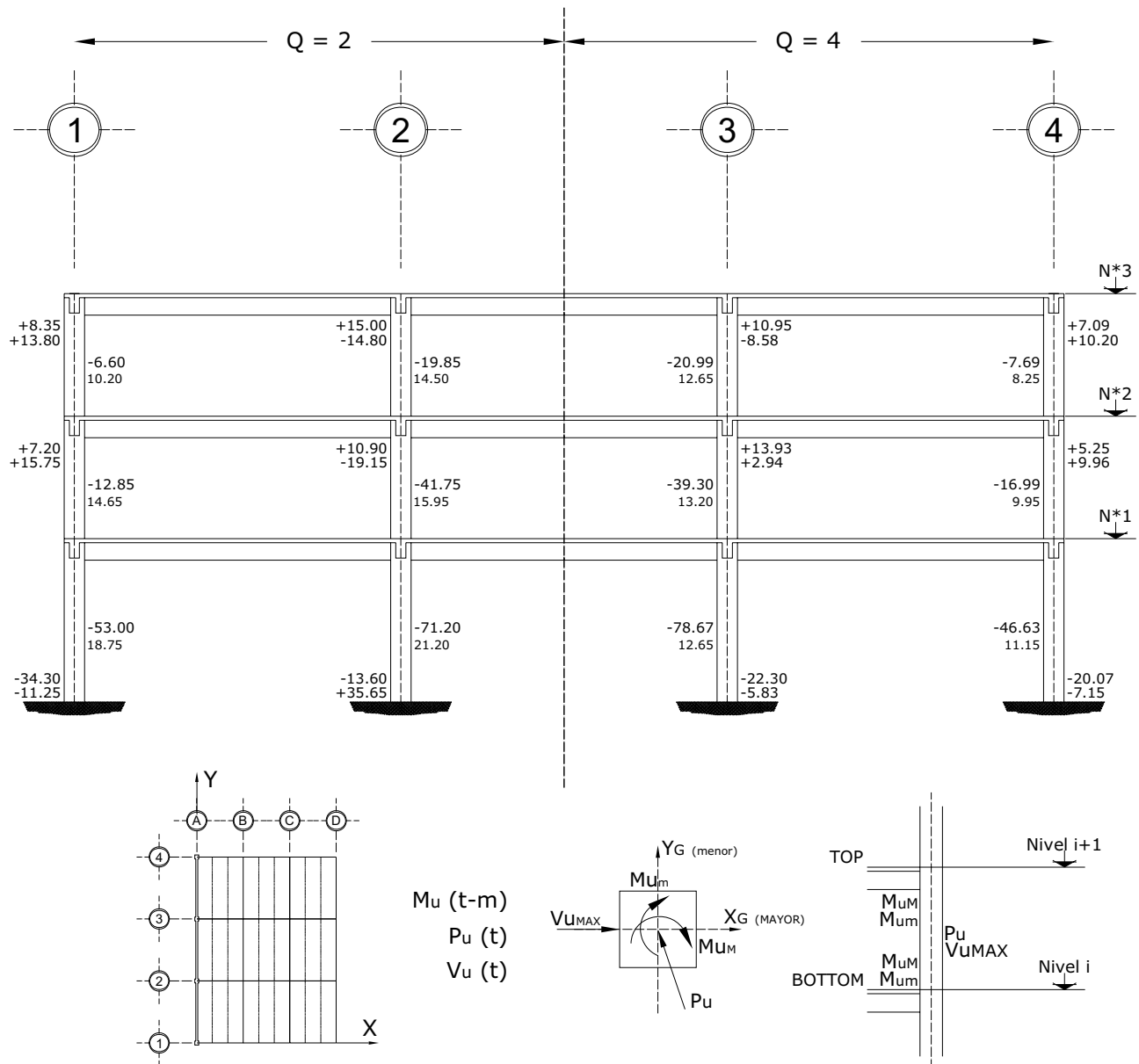
Fig 3.51 Elementos mecánicos últimos en columnas, eje A, casos A1 y B1
