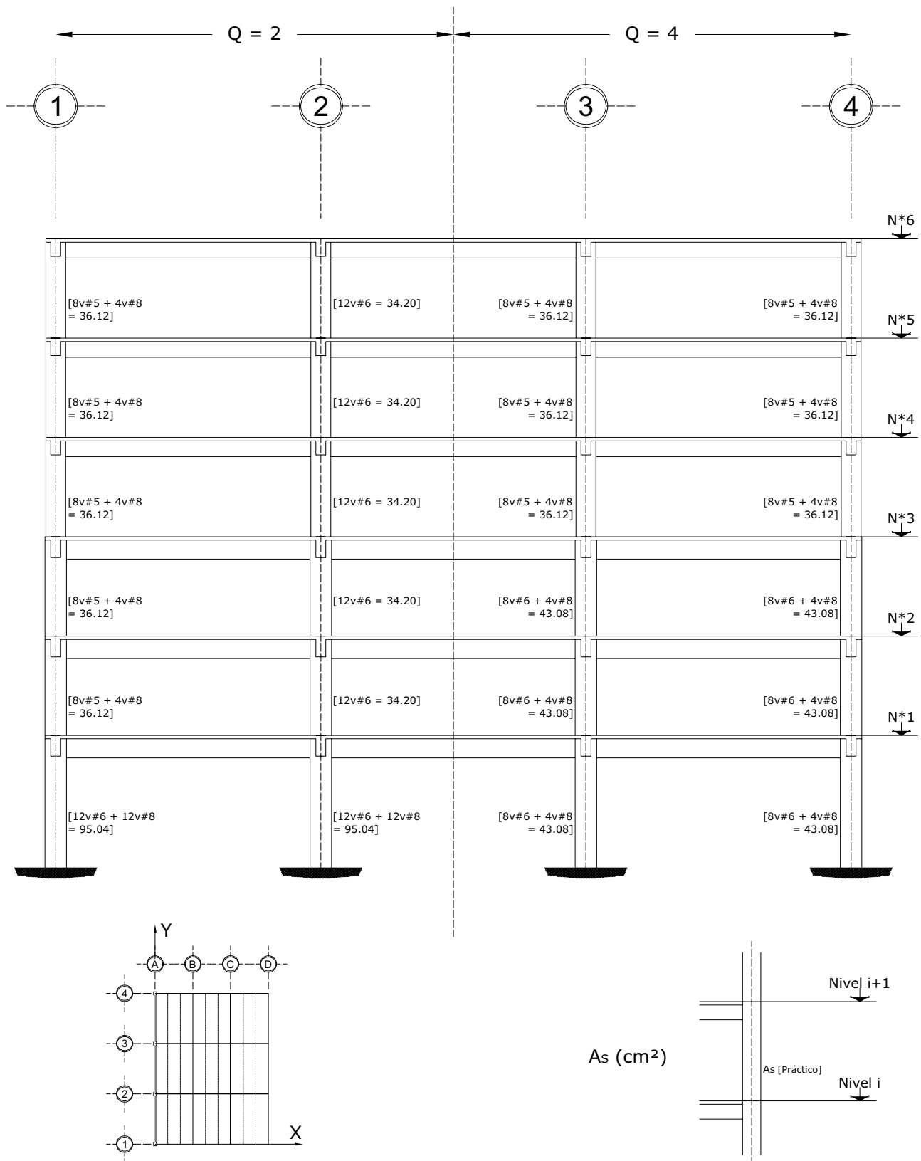
Fig 3.115b Acero de refuerzo longitudinal teórico y práctico necesario en columnas, eje A, casos C2 ( Q = 2 ) y D2 ( Q = 4 )
