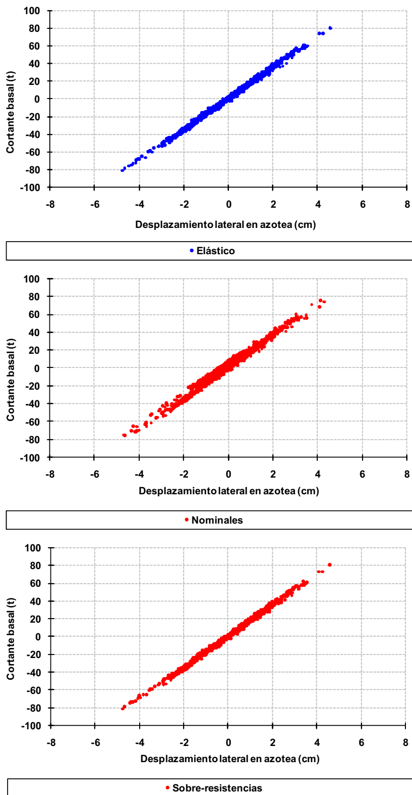
Fig 4.50 Relaciones fuerza cortante basal - desplazamiento horizontal en azotea, eje 2, caso A2, análisis paso a paso elástico e inelástico (sin y con sobre-resistencias), diseño Apéndice A, NTC-Sismo del RDF-04, edificio de 3 niveles
