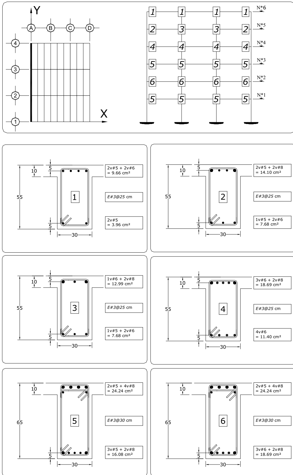
Fig 3.118 Tipos de armados de refuerzo longitudinal y transversal resultantes en los extremos de las vigas del eje A, caso C2 ( Q = 2 )
