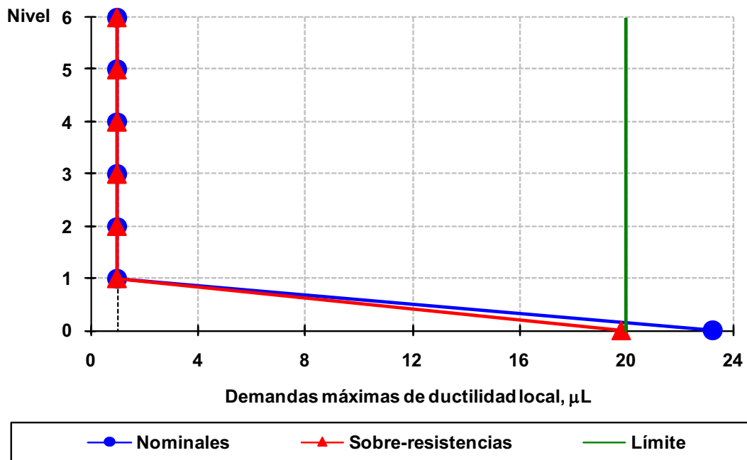
Fig 4.185 Demandas máximas de ductilidad local desarrolladas en columnas del eje A, caso D2, análisis Push-over (sin y con sobre-resistencias), perfil de cargas laterales del análisis dinámico modal espectral, diseño Apéndice A, NTC-Sismo del RDF-04, edificio de 6 niveles
