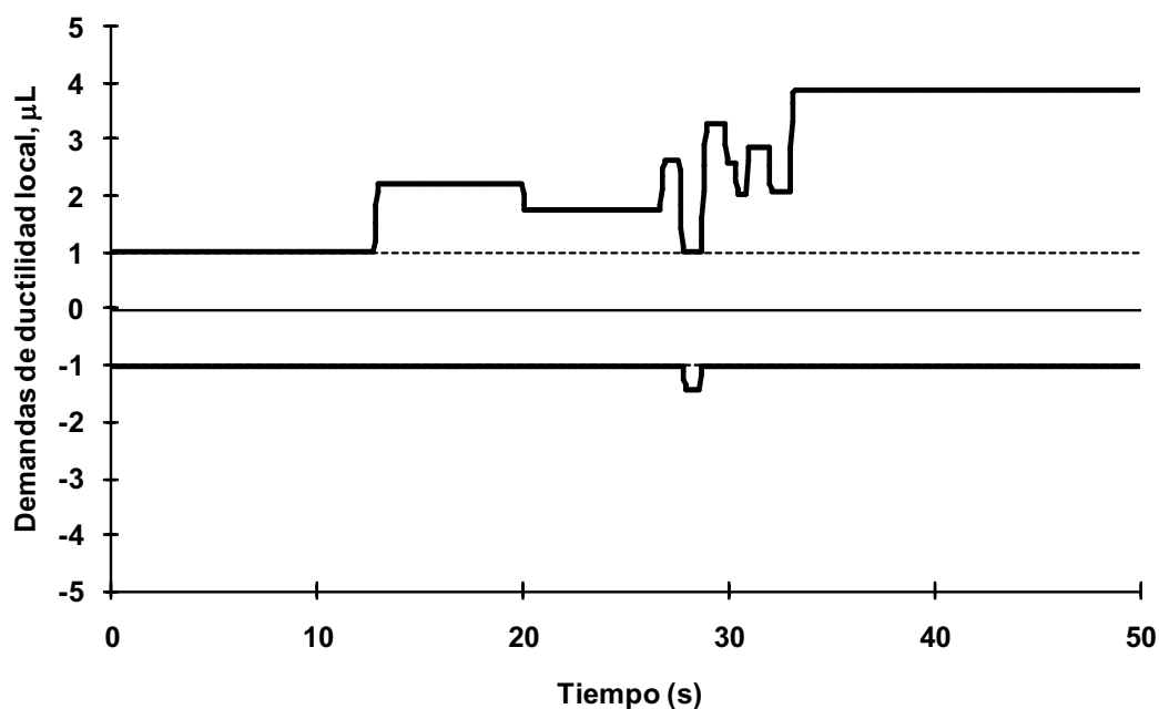
Fig 4.110 Demanda de ductilidad local desarrollada en el extremo izquierdo de la viga 16 del nivel 1, eje 2, caso D2, análisis paso a paso inelástico (sin sobre-resistencias), NTC-Sismo del RDF-04, edificio de 6 niveles
