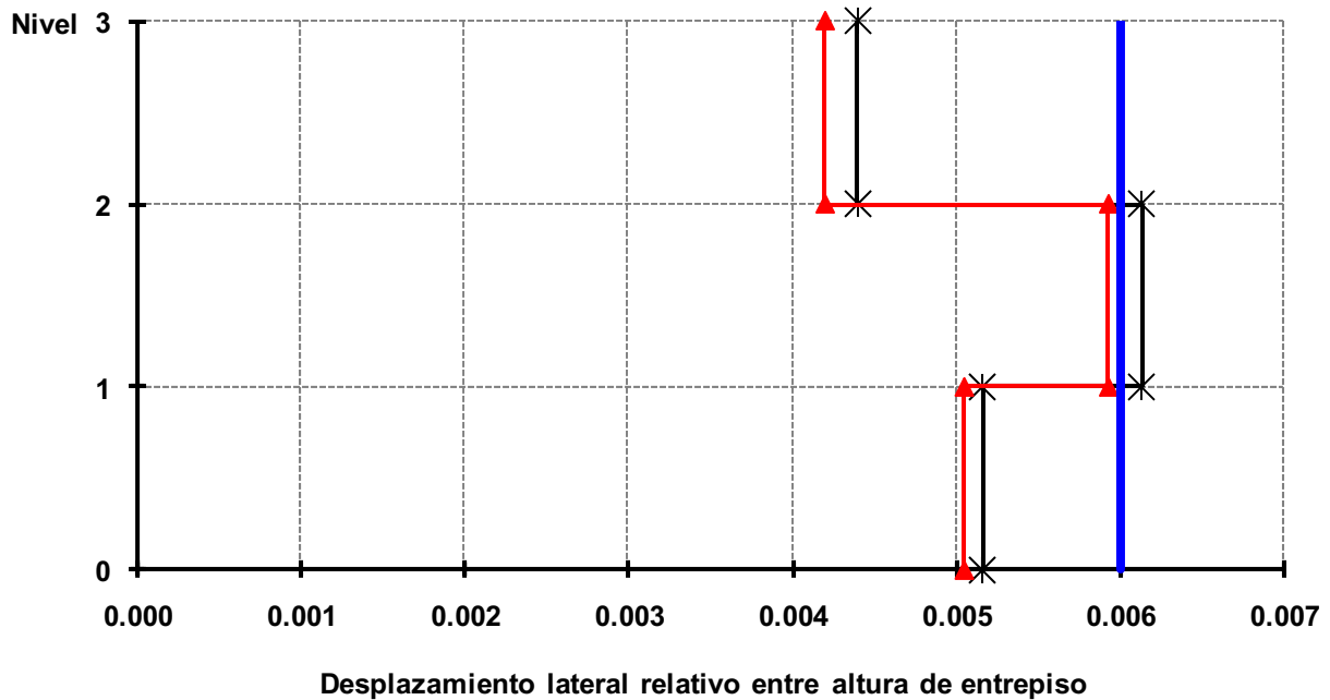
Fig 3.18 Relaciones desplazamiento lateral relativo entre altura de entrepiso (rige condición de servicio), análisis dinámico modal espectral, edificio de 3 niveles, caso B1 ( Q = 4 )
