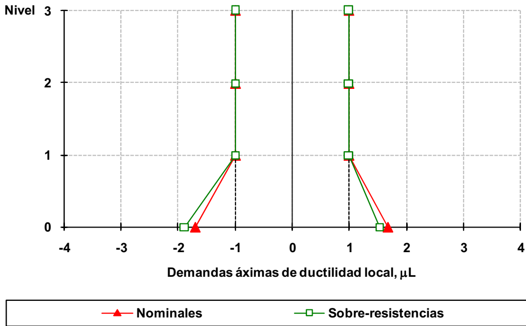
Fig 4.117 Demandas máximas de ductilidad local desarrolladas en columnas del eje A, caso B2, análisis paso a paso elástico e inelástico (sin y con sobre-resistencias), NTC-Sismo del RDF-04, edificio de 3 niveles
