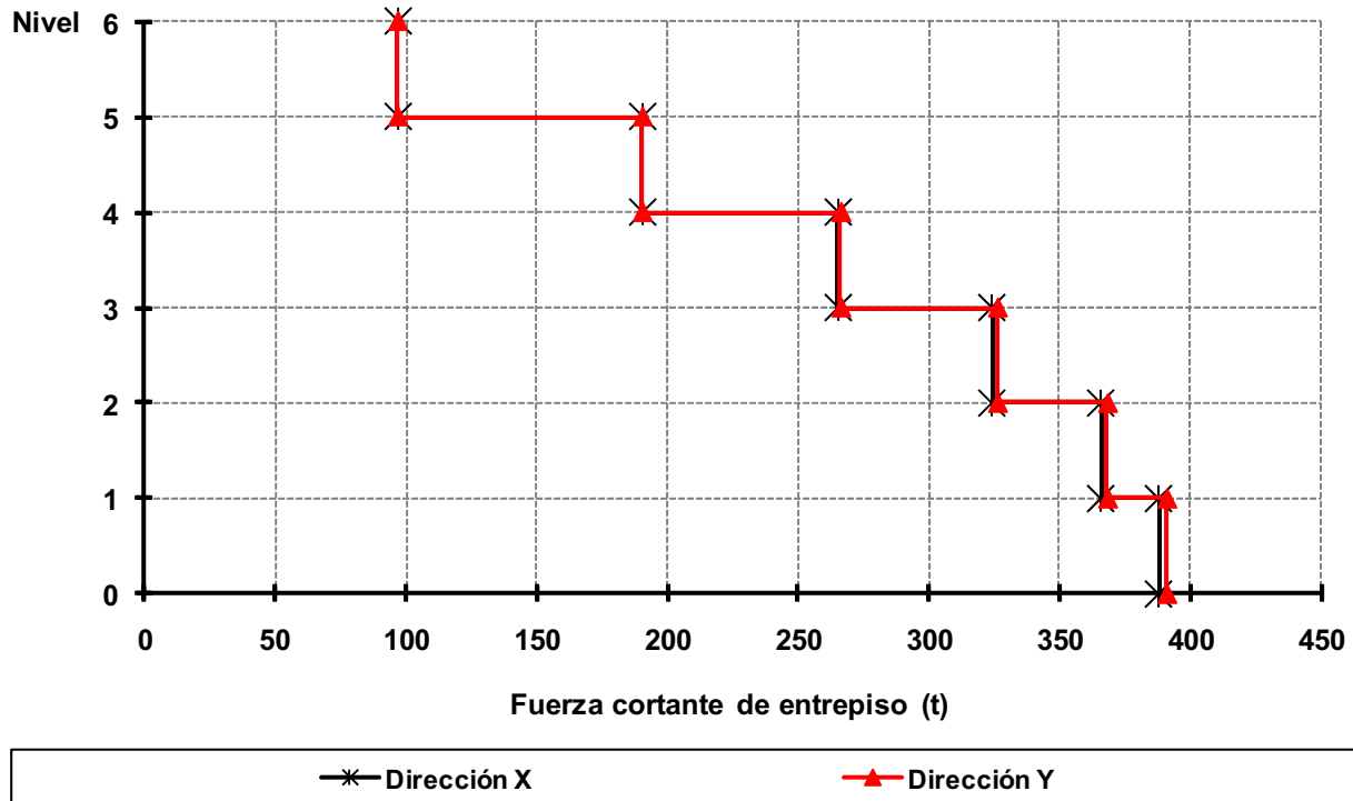
Fig 3.37 Fuerzas cortantes de entrepiso, análisis dinámico modal espectral, edificio de 6 niveles, caso C2 ( Q = 2 )
