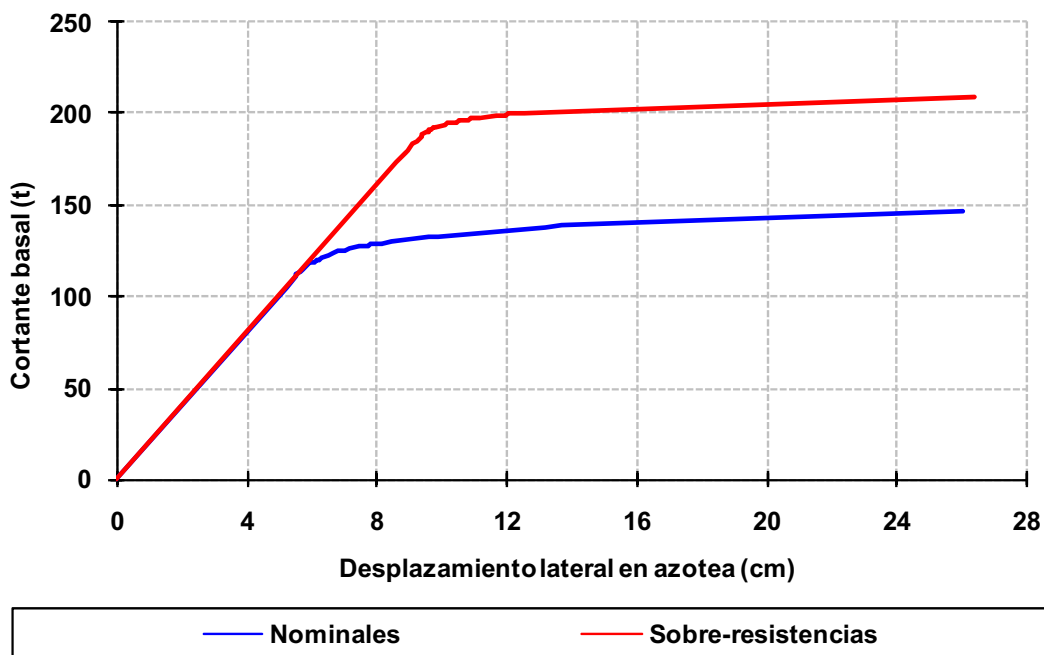
Fig 4.191 Relaciones fuerza cortante basal - desplazamiento horizontal en azotea, eje A, caso C2, análisis Push-over (sin y con sobre-resistencias), perfil de cargas laterales del análisis dinámico modal espectral, diseño Apéndice A, NTC-Sismo del RDF-04, edificio de 6 niveles
