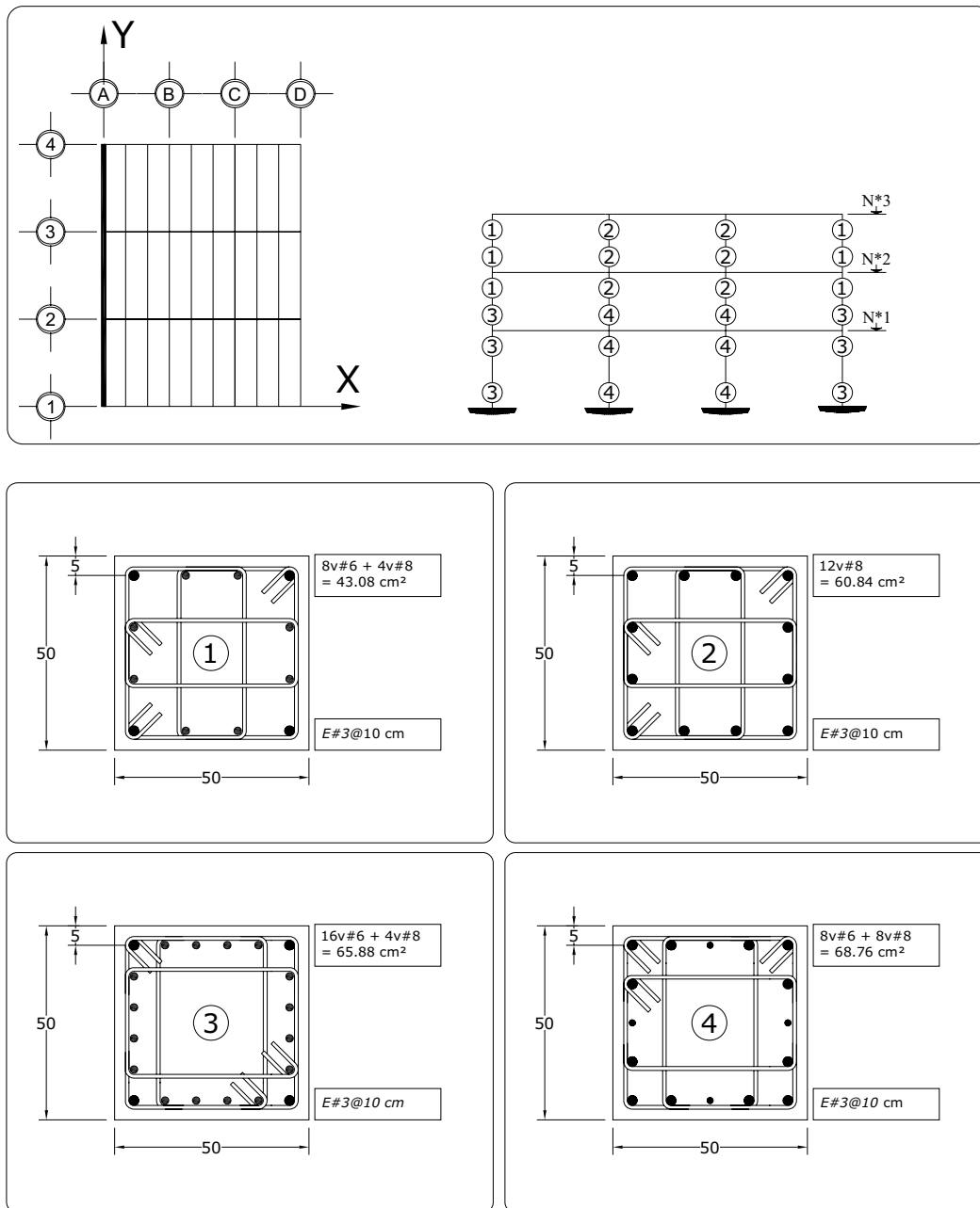
Fig 3.59 Tipos de armados de refuerzo longitudinal y transversal resultantes en los extremos de las columnas del eje A, caso A1 ( Q = 2 )
