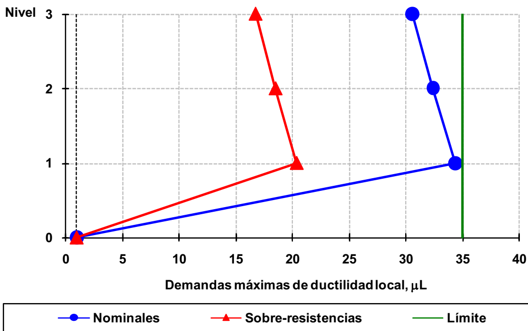
Fig 4.173 Demandas máximas de ductilidad local desarrolladas en vigas del eje A, caso B2, análisis Push-over (sin y con sobre-resistencias), perfil de cargas laterales del análisis dinámico modal espectral, diseño Apéndice A, NTC-Sismo del RDF-04, edificio de 3 niveles
