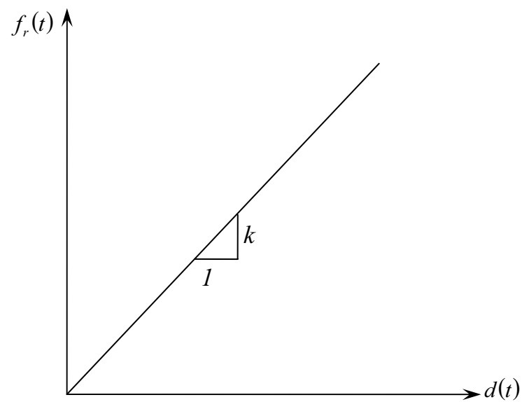
Fig 2.6 Relación matriz de rigideces laterales de columnas contra el vector de desplazamiento relativo de la masa
