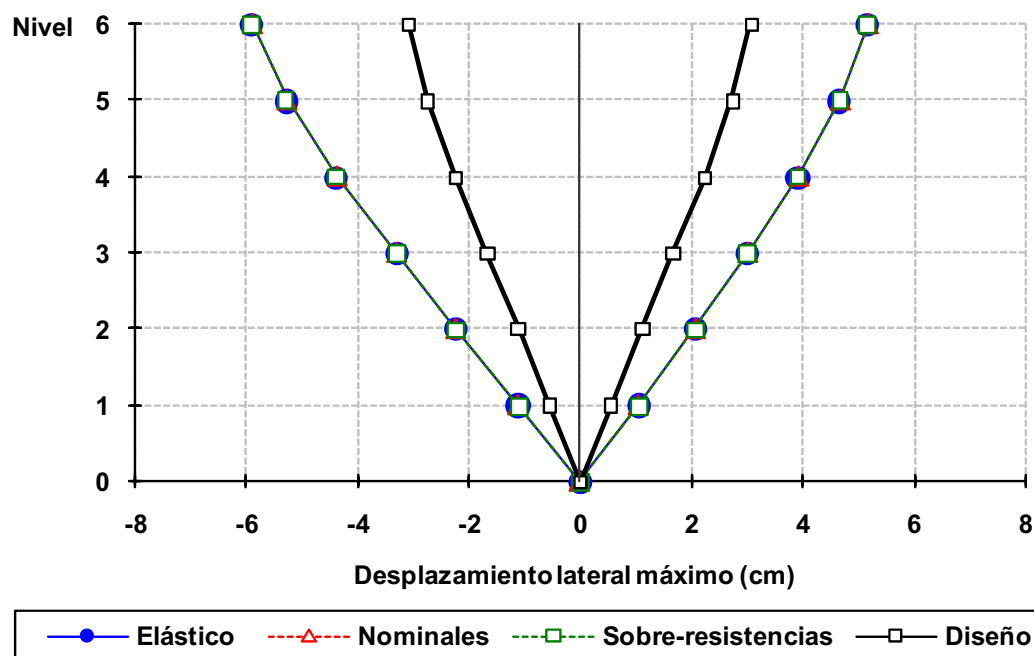
Fig 4.14 Desplazamientos horizontales máximos del eje 2, caso C2, análisis paso a paso dinámico (elástico e inelástico) y modal espectral, sin y con efectos de sobre-resistencias, diseño Apéndice A, NTC-Sismo del RDF-04, edificio de 6 niveles
