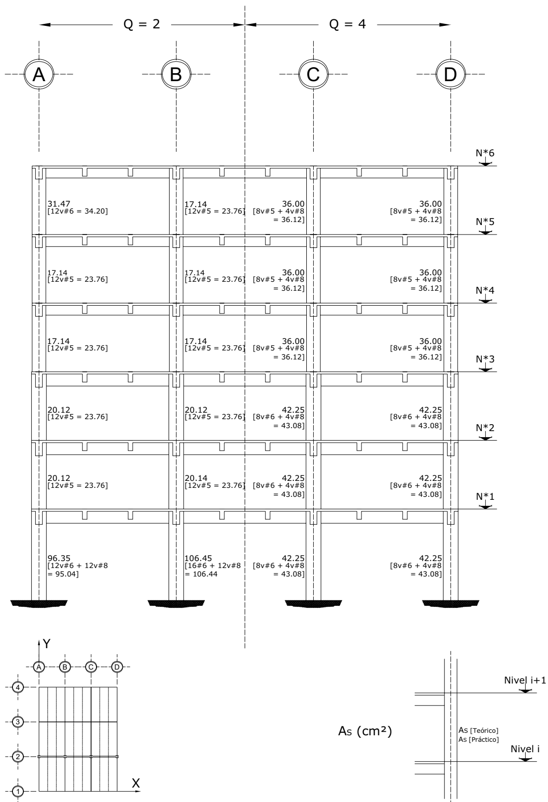
Fig 3.113a Acero de refuerzo longitudinal teórico y práctico necesario en columnas, eje 2, casos C2 (Q = 2) y D2 (Q = 4)
