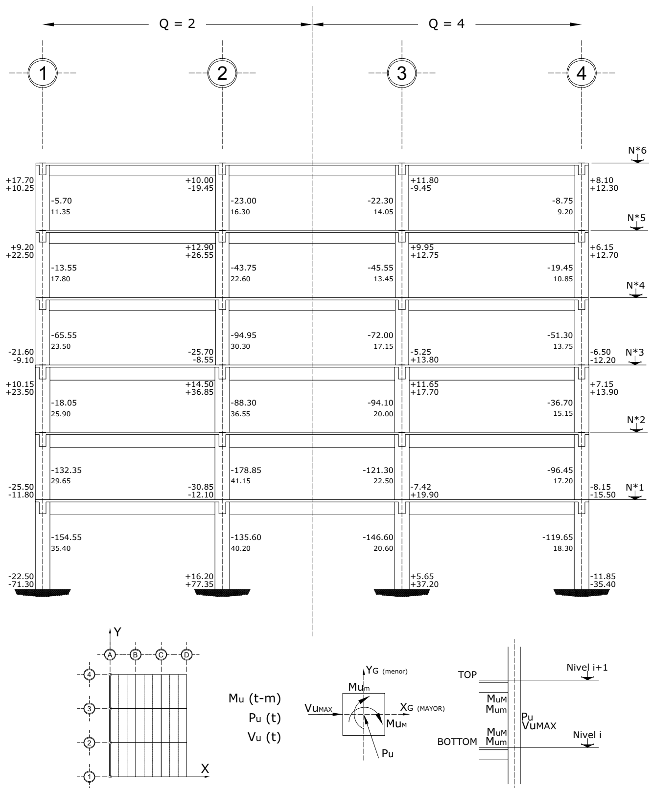
Fig 3.111 Elementos mecánicos últimos en columnas, eje A, casos C2 y D2
