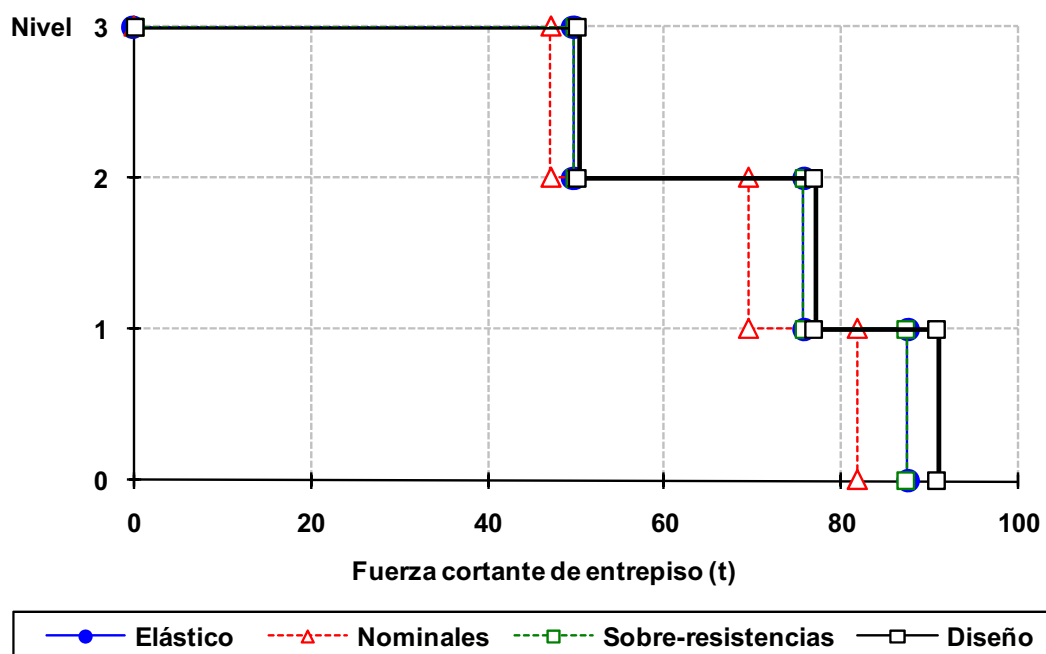
Fig 4.34 Envolventes de fuerzas cortantes de entrepiso del eje 2, caso A2, análisis paso a paso elástico e inelástico (sin y con sobre-resistencias) y modal espectral, NTC-Sismo del RDF-04, edificio de 3 niveles
