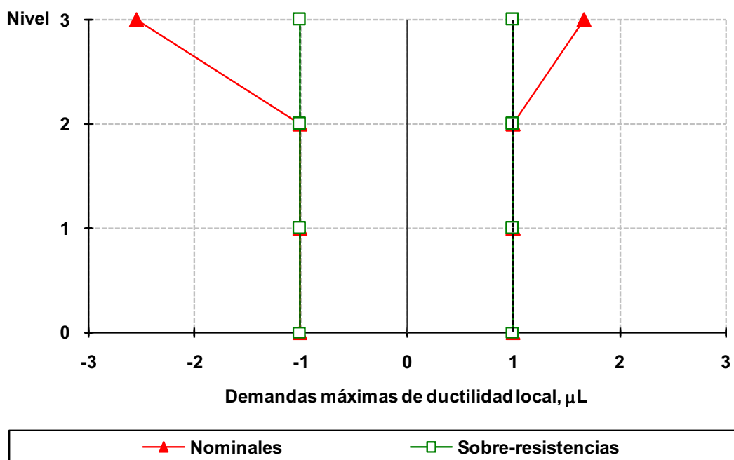
Fig 4.114 Demandas máximas de ductilidad local desarrolladas en columnas del eje 2, caso A2, análisis paso a paso elástico e inelástico (sin y con sobre-resistencias), NTC-Sismo del RDF-04, edificio de 3 niveles
