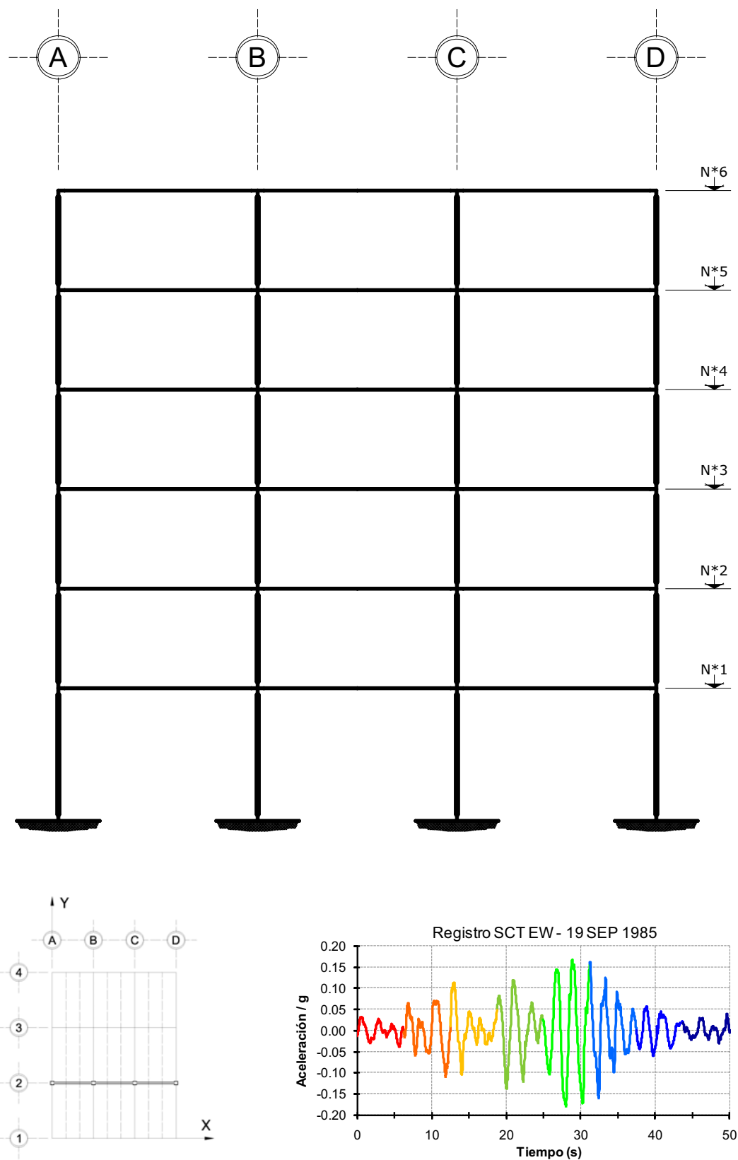
Fig 4.131 Ubicación y secuencia de formación de articulaciones plásticas, análisis paso a paso, con sobre-resistencias, edificio de 6 niveles, eje 2, caso C2
