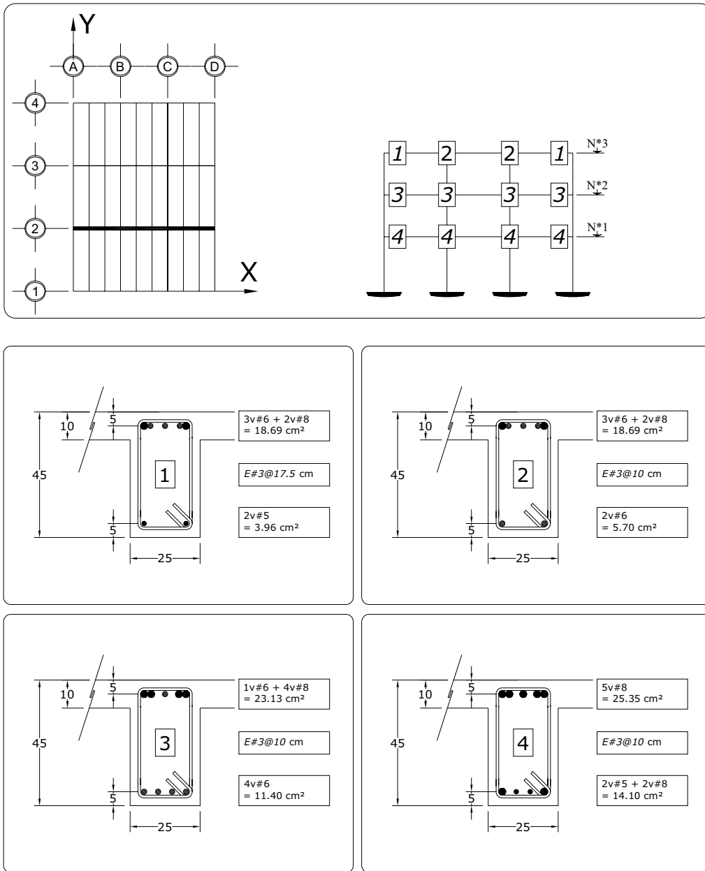
Fig 3.76 Tipos de armados de refuerzo longitudinal y transversal resultantes en los extremos de las vigas del eje 2, caso A2 (Q = 2)
