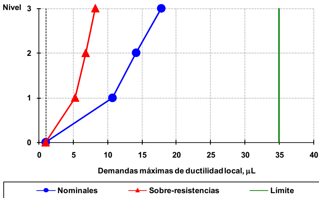
Fig 4.171 Demandas máximas de ductilidad local desarrolladas en vigas del eje A, caso A2, análisis Push-over (sin y con sobre-resistencias), perfil de cargas laterales del análisis dinámico modal espectral, diseño Apéndice A, NTC-Sismo del RDF-04, edificio de 3 niveles
