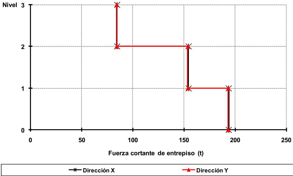
Fig 3.32 Fuerzas cortantes de entrepiso, análisis dinámico modal espectral, edificio de 3 niveles, caso A1 (Q = 2)
