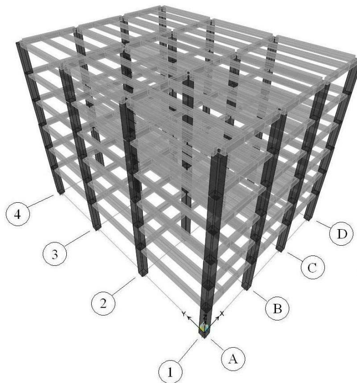
Fig 3.3 Modelo estructural del edificio de 6 niveles, casos C1, C2, D1 y D2
