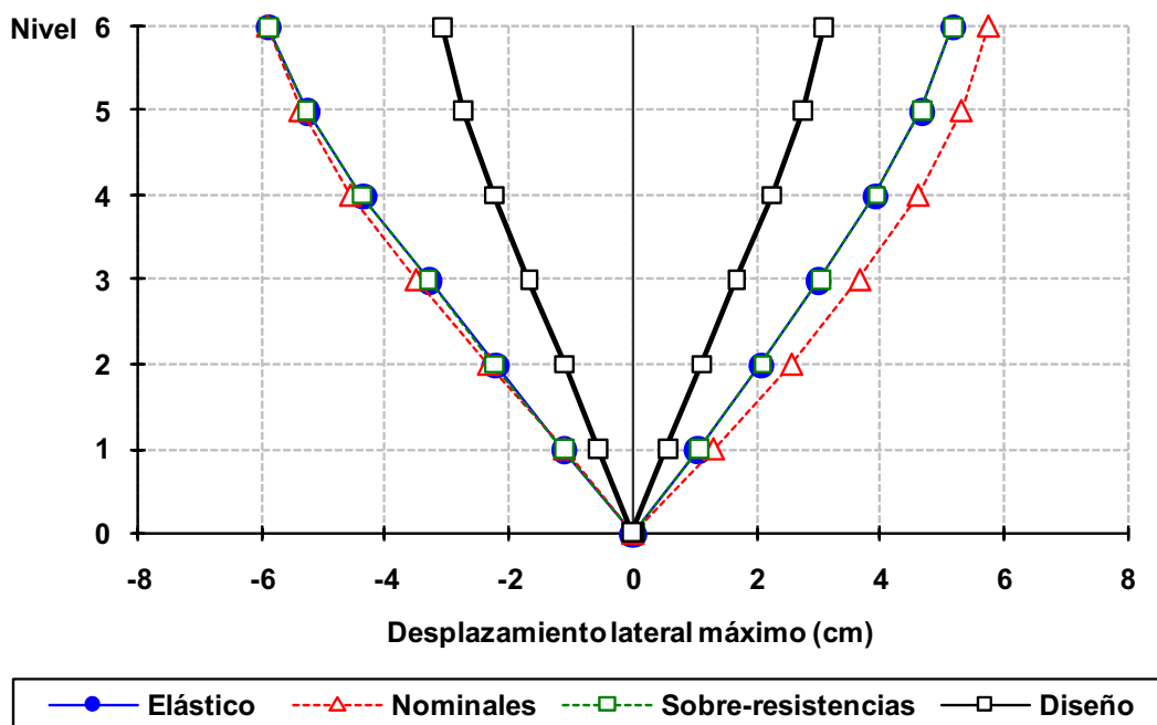
Fig 4.16 Desplazamientos horizontales máximos del eje 2, caso D2, análisis paso a paso dinámico (elástico e inelástico) y modal espectral, sin y con efectos de sobre-resistencias, diseño Apéndice A, NTC-Sismo del RDF-04, edificio de 6 niveles
