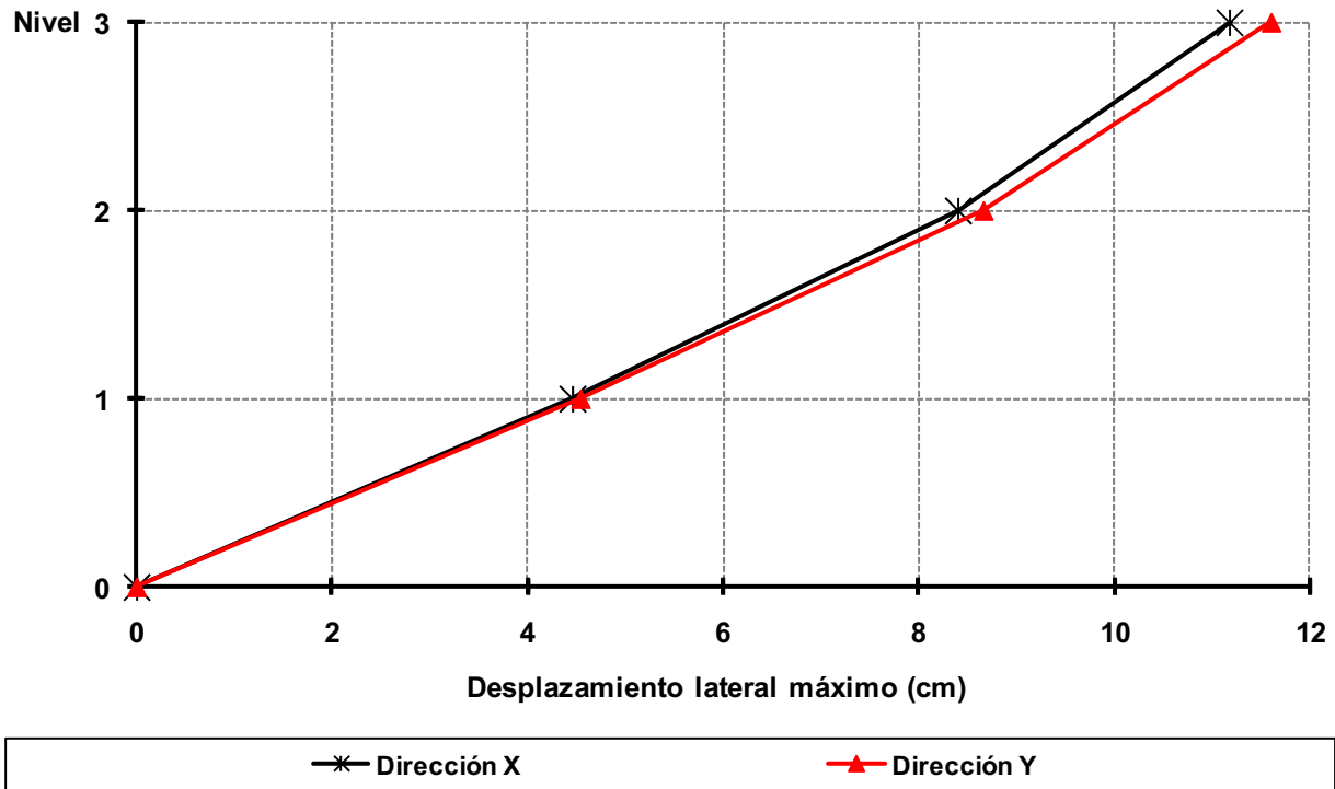
Fig 3.27b Desplazamientos laterales máximos, análisis dinámico modal espectral (condición de colapso), edificio de 3 niveles, caso B2 ( Q = 4 )
