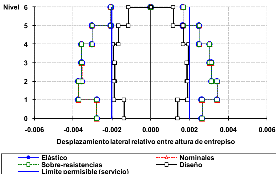
Fig 4.30 Relaciones desplazamiento lateral relativo entre altura de entrepiso del eje 2, caso C2, análisis paso a paso elástico e inelástico (sin y con sobre-resistencias) y modal espectral, NTC-Sismo del RDF-04, edificio de 6 niveles
