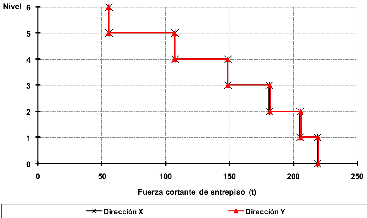
Fig 3.38 Fuerzas cortantes de entrepiso, análisis dinámico modal espectral, edificio de 6 niveles, caso D1 (Q = 4)
