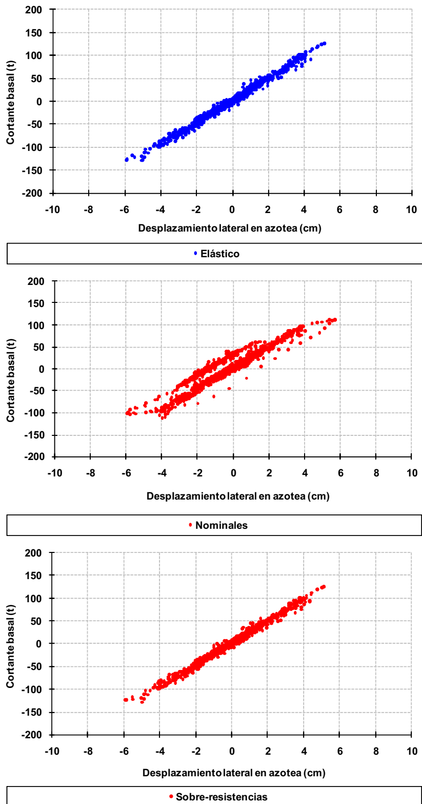
Fig 4.56 Relaciones fuerza cortante basal - desplazamiento horizontal en azotea, eje 2, caso D2, análisis paso a paso elástico e inelástico (sin y con sobre-resistencias), diseño Apéndice A, NTC-Sismo del RDF-04, edificio de 6 niveles
