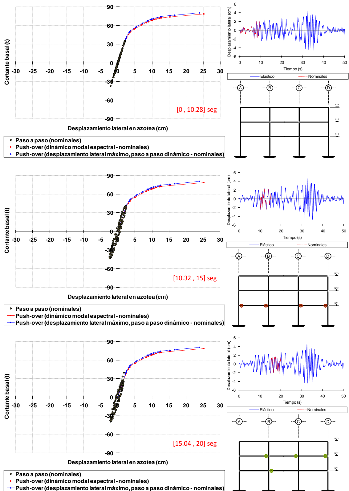
Fig 5.6a Comparación de la intensidad de la respuesta inelástica fuerza cortante basal - desplazamiento lateral de azotea para varios intervalos del tiempo (0 a 20 segundos) de los análisis paso a paso contra análisis estático no-lineal Push-over, resistencias nominales, caso B2 del eje 2 del edificio de 3 niveles
