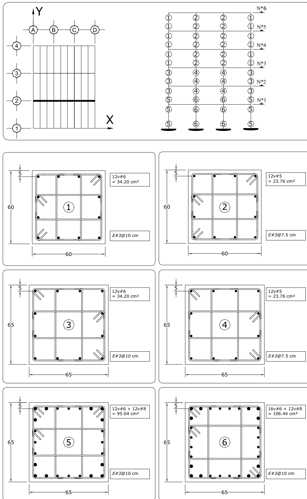
Fig 3.117 Tipos de armados de refuerzo longitudinal y transversal resultantes en los extremos de las columnas del eje 2, caso C2 (Q = 2)
