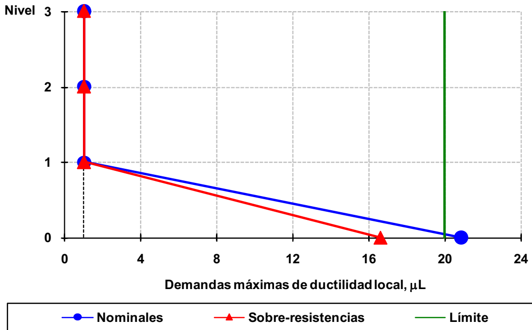
Fig 4.181 Demandas máximas de ductilidad local desarrolladas en columnas del eje A, caso B2, análisis Push-over (sin y con sobre-resistencias), perfil de cargas laterales del análisis dinámico modal espectral, diseño Apéndice A, NTC-Sismo del RDF-04, edificio de 3 niveles
