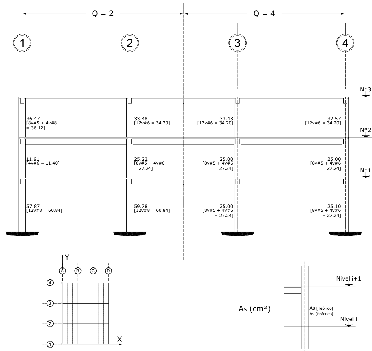
Fig 3.75a Acero de refuerzo longitudinal teórico y práctico necesario en columnas, eje A, casos A2 ( Q = 2 ) y B2 ( Q = 4 )
