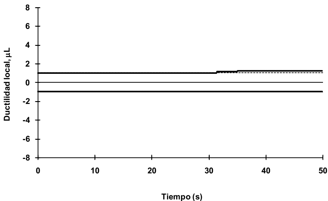
Fig 4.103 Demanda de ductilidad local desarrollada en el extremo izquierdo de la viga 7 del nivel 1, eje 2, caso B2, análisis paso a paso inelástico (con sobre-resistencias), NTC-Sismo del RDF-04, edificio de 3 niveles
