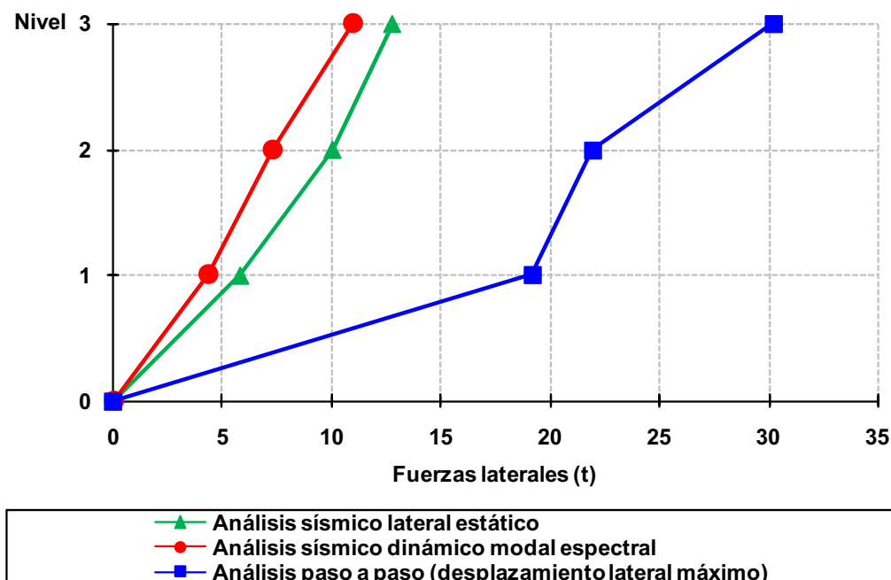
Fig 4.143 Distribución del perfil de fuerzas laterales debidas a diferentes condiciones de análisis sísmico del eje 2, caso B2, (con sobre-resistencias), diseño según el Apéndice A de las NTC-Sismo del RDF-04, edificio de 3 niveles
