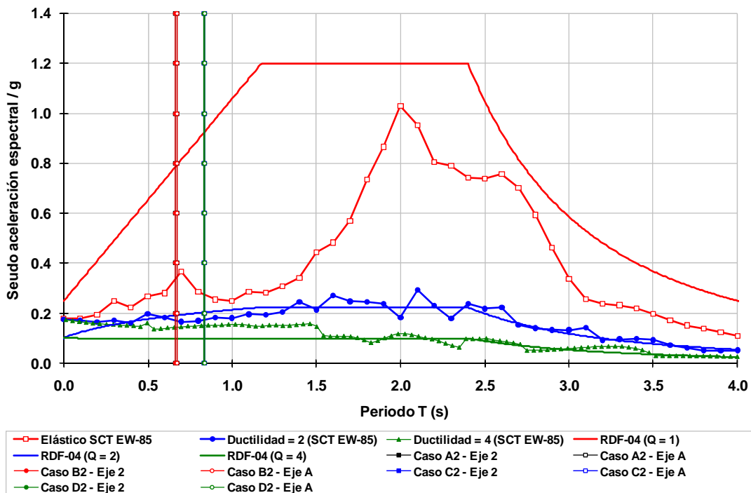
Fig 5.2 Espectros de respuesta SCT EW-85 (ductilidades 1, 2 y 4, con amortiguamiento del 5%) y de diseño ( Q=1, 2 y 4 ) del Apéndice A ( T_s=2 s) de las NTC-Sismo del RDF-04, y ubicación de los periodos fundamentales de vibración de los diferentes modelos de estudio de 6 niveles
