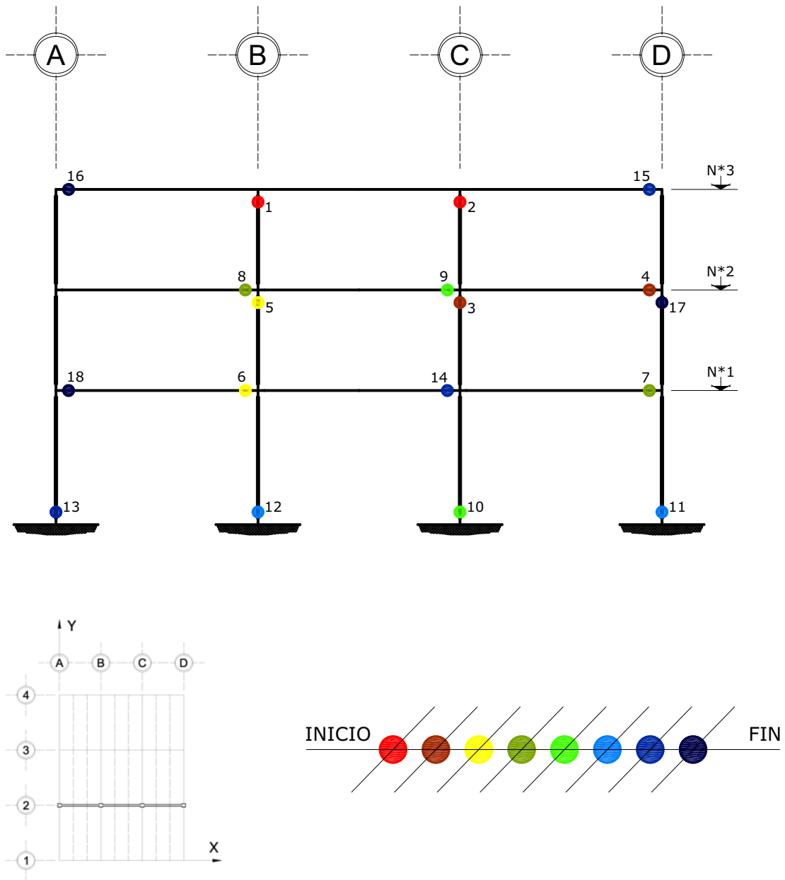
Fig 4.195 Ubicación y secuencia de formación de articulaciones plásticas, análisis Push-over, con sobre-resistencias, edificio de 3 niveles, eje 2, caso A2
