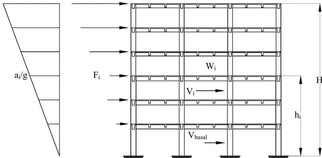
Fig 2.1 Fuerzas sísmicas estáticas equivalentes
