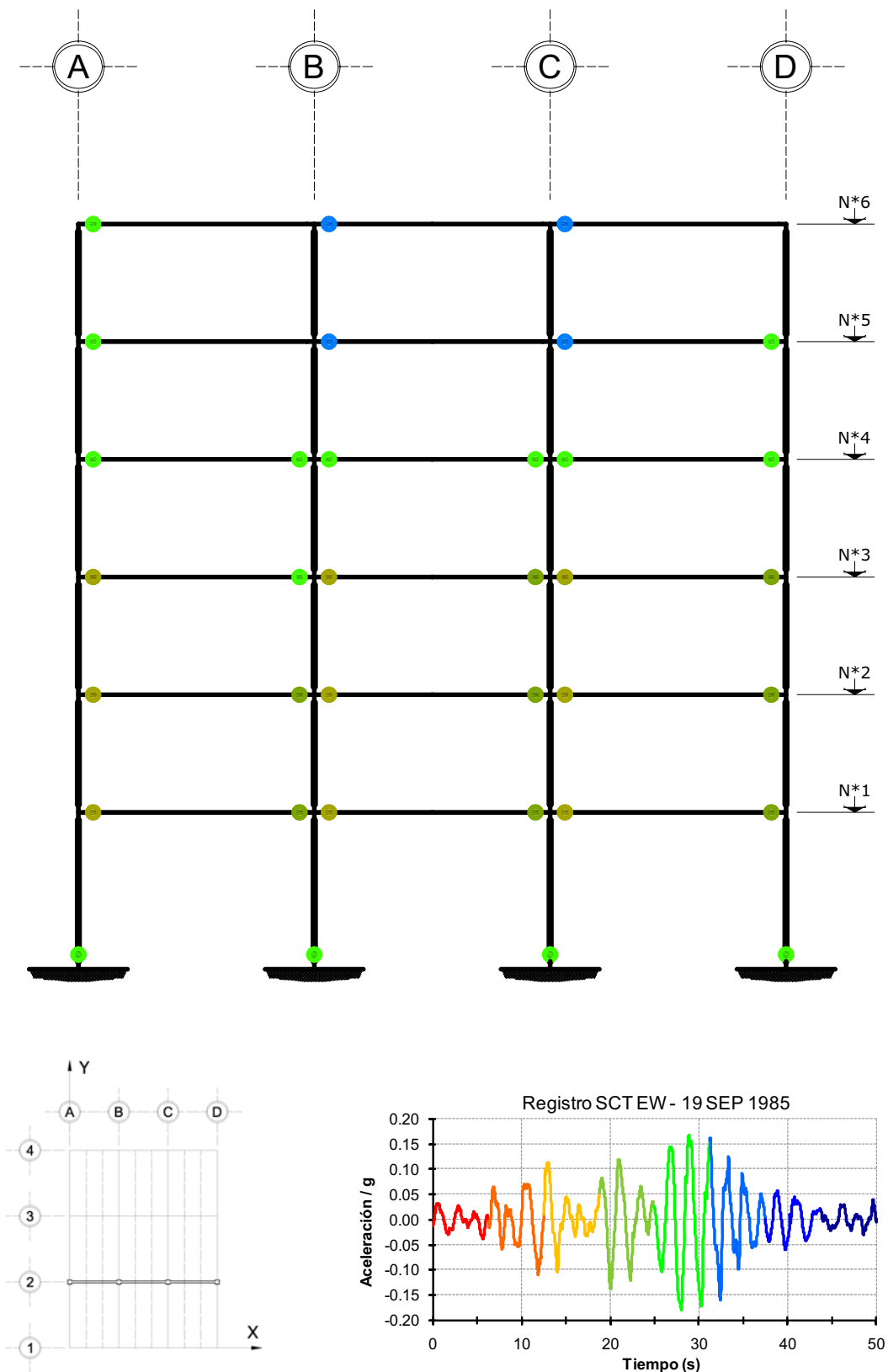
Fig 4.134 Ubicación y secuencia de formación de articulaciones plásticas, análisis paso a paso, resistencias nominales, edificio de 6 niveles, eje 2, caso D2
