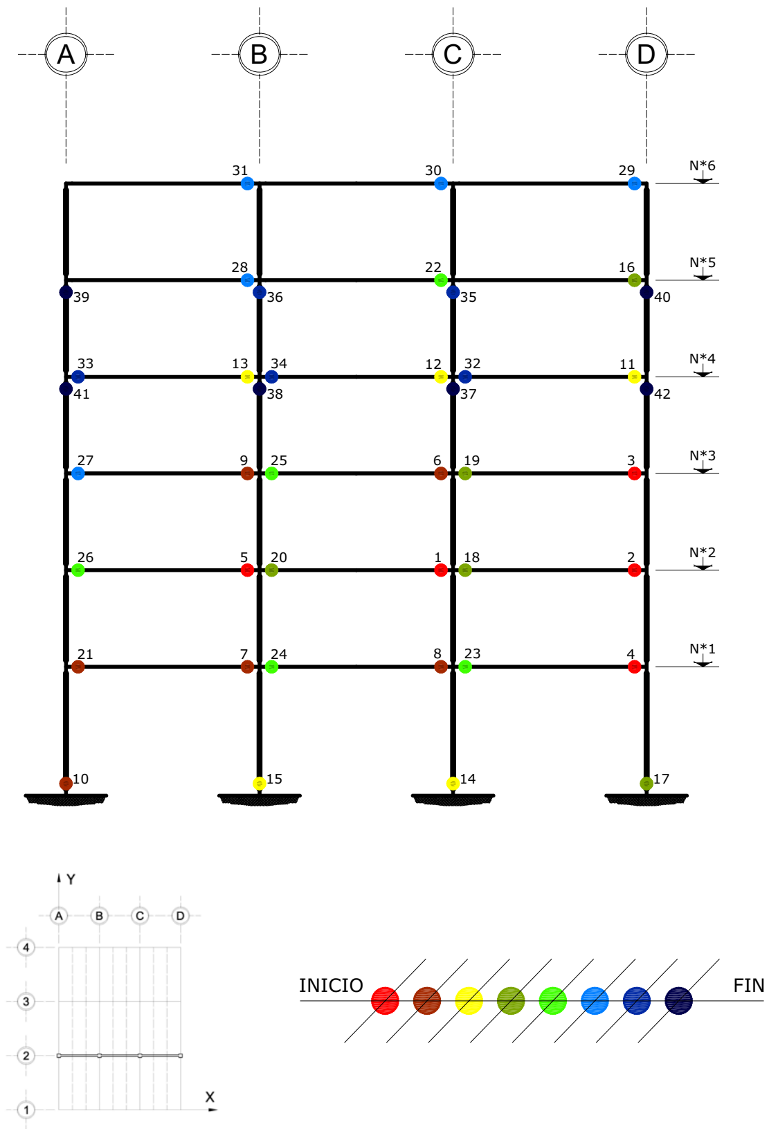
Fig 4.207 Ubicación y secuencia de formación de articulaciones plásticas, análisis Push-over, con sobre-resistencias, edificio de 6 niveles, eje 2, caso D2
