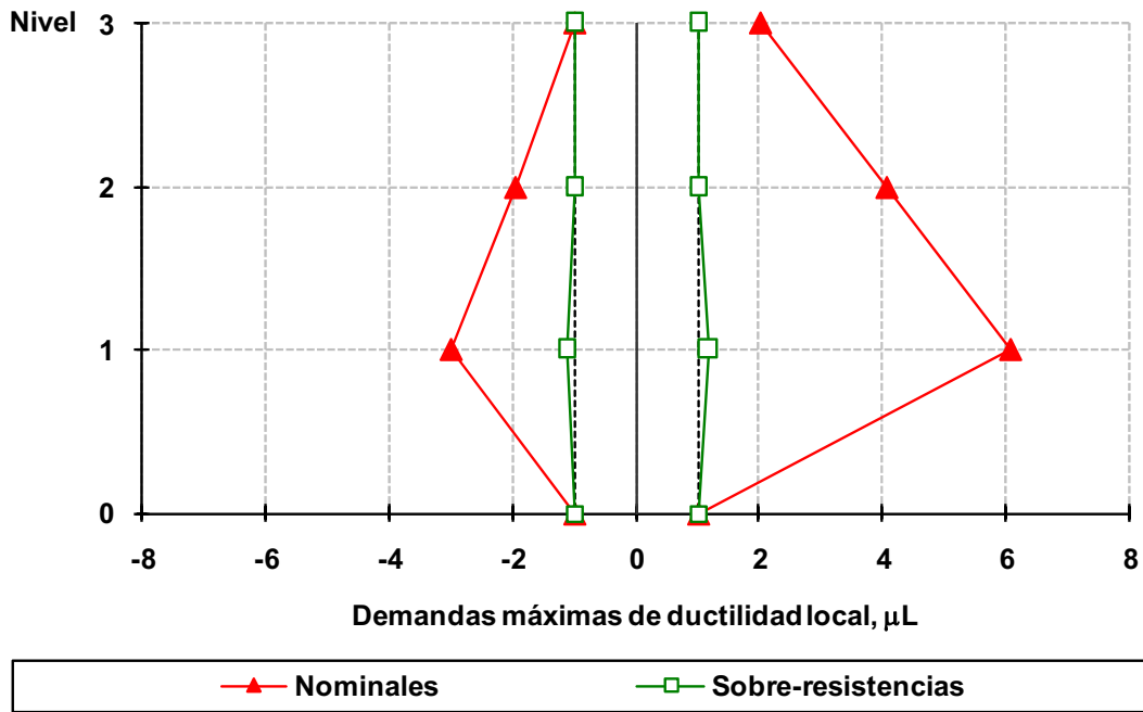
Fig 4.92 Demandas máximas de ductilidad local desarrolladas en vigas del eje 2, caso B2, análisis paso a paso elástico e inelástico (sin y con sobre-resistencias), NTC-Sismo del RDF-04, edificio de 3 niveles
