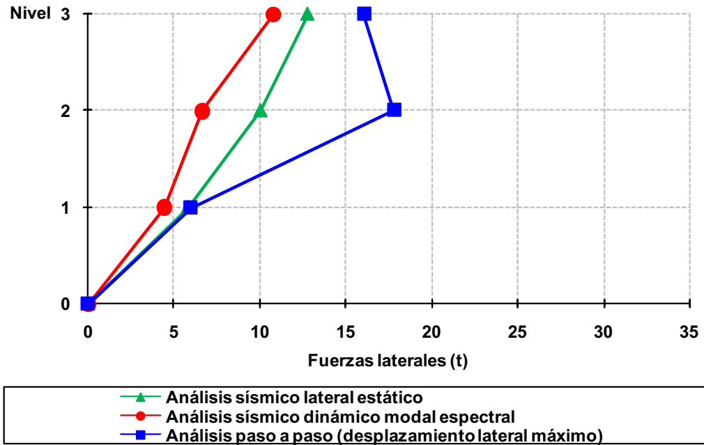
Fig 4.144 Distribución del perfil de fuerzas laterales debidas a diferentes condiciones de análisis sísmico del eje A, caso B2, (sin sobre-resistencias), diseño según el Apéndice A de las NTC-Sismo del RDF-04, edificio de 3 niveles
