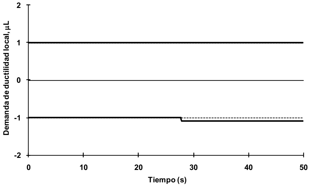
Fig 4.108 Demanda de ductilidad local desarrollada en el extremo izquierdo de la viga 16 del nivel 1, eje A, caso C2, análisis paso a paso inelástico (sin sobre-resistencias), NTC-Sismo del RDF-04, edificio de 6 niveles
