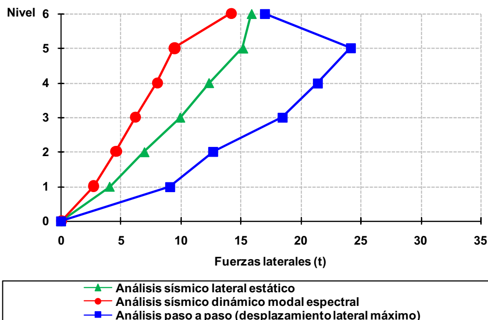
Fig 4.150 Distribución del perfil de fuerzas laterales debidas a diferentes condiciones de análisis sísmico del eje 2, caso D2, (sin sobre-resistencias), diseño según el Apéndice A de las NTC-Sismo del RDF-04, edificio de 6 niveles
