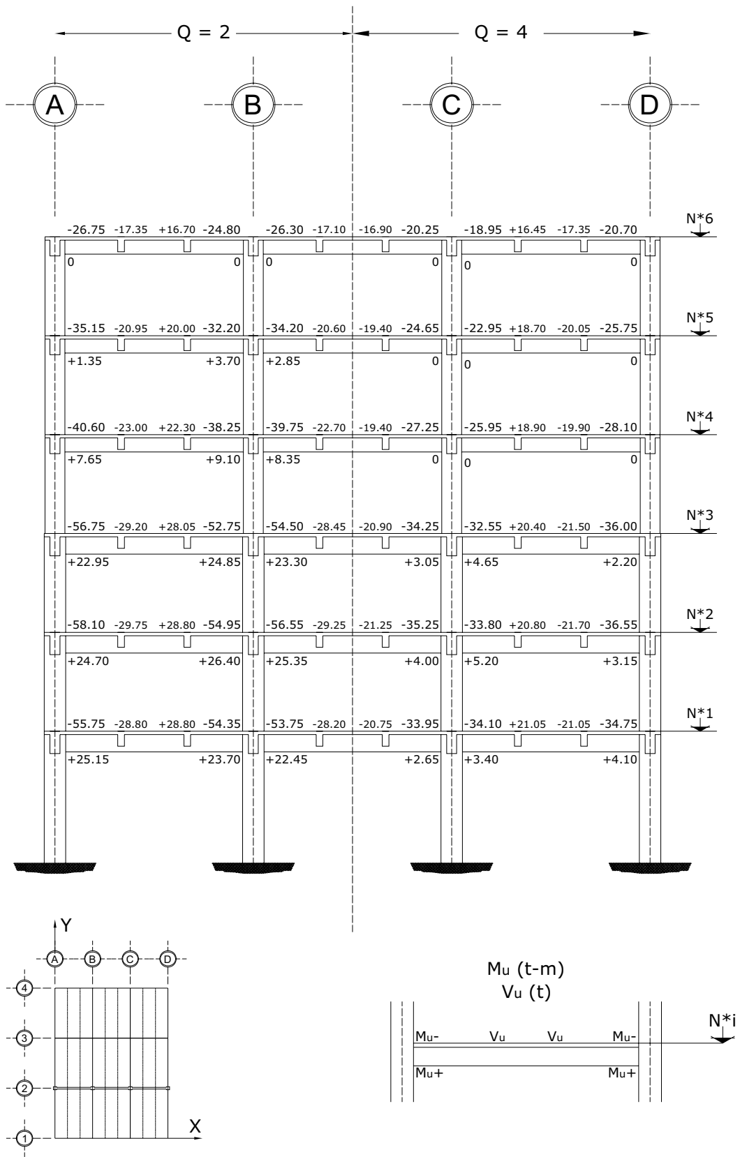
Fig 3.108 Momentos flexionantes y fuerzas cortantes últimos de vigas, eje 2, casos C2 ( Q = 2 ) y D2 ( Q = 4 )
