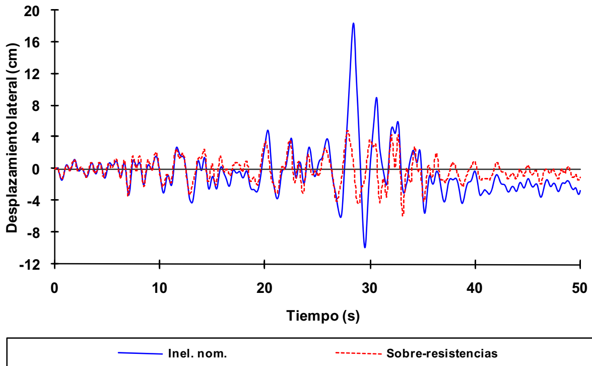
Fig 4.25 Historias de desplazamientos laterales de azotea, eje A, caso D2, análisis paso a paso elástico e inelástico (sin y con sobre-resistencias), diseño Apéndice A, NTC-Sismo del RDF-04, edificio de 6 niveles
