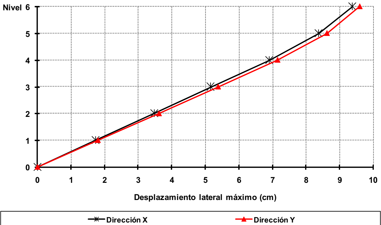
Fig 3.28 Desplazamientos laterales máximos, análisis dinámico modal espectral (rige condición de servicio), edificio de 6 niveles, caso C1 ( Q = 2 )
