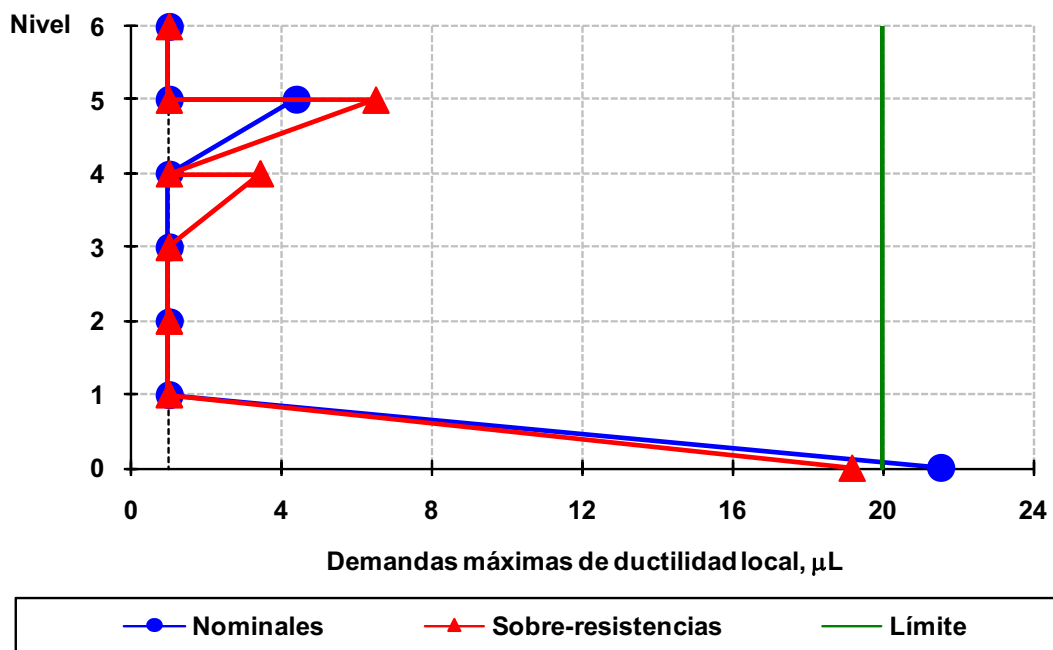
Fig 4.184 Demandas máximas de ductilidad local desarrolladas en columnas del eje 2, caso D2, análisis Push-over (sin y con sobre-resistencias), perfil de cargas laterales del análisis dinámico modal espectral, diseño Apéndice A, NTC-Sismo del RDF-04, edificio de 6 niveles
