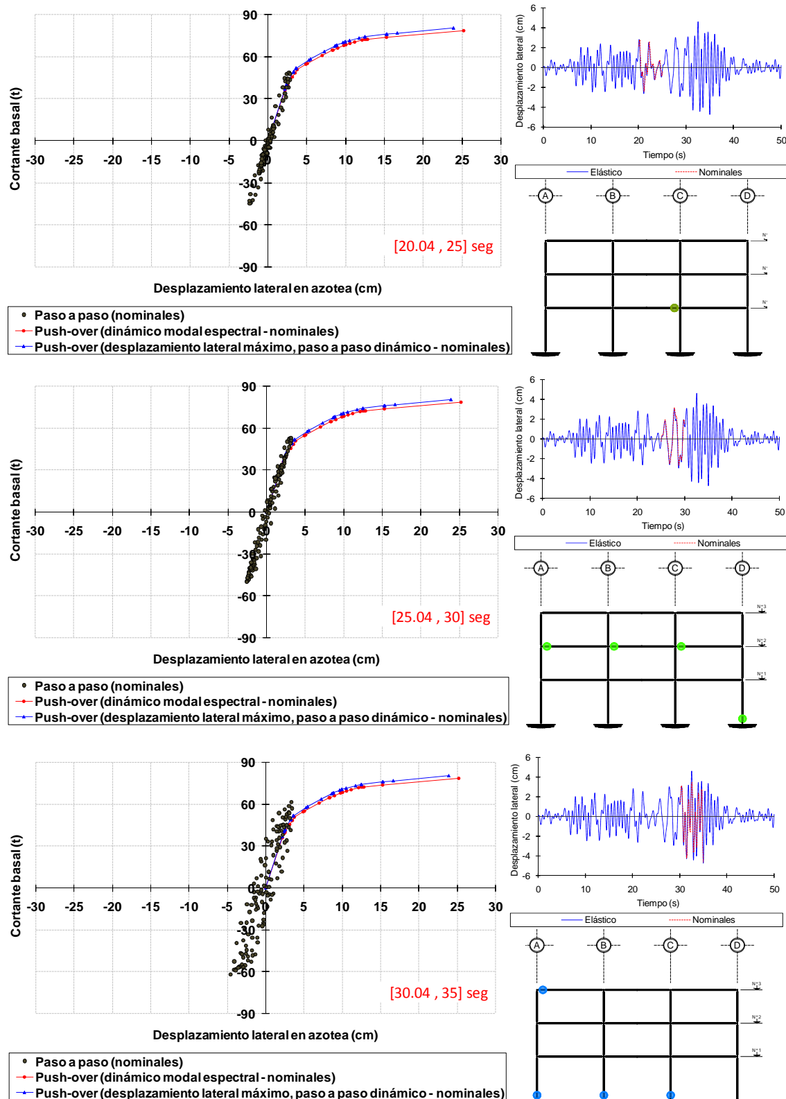
Fig 5.6b Comparación de la intensidad de la respuesta inelástica fuerza cortante basal - desplazamiento lateral de azotea para varios intervalos del tiempo (20 a 35 segundos) de los análisis paso a paso contra análisis estático no-lineal Push-over, resistencias nominales, caso B2 del eje 2 del edificio de 3 niveles
