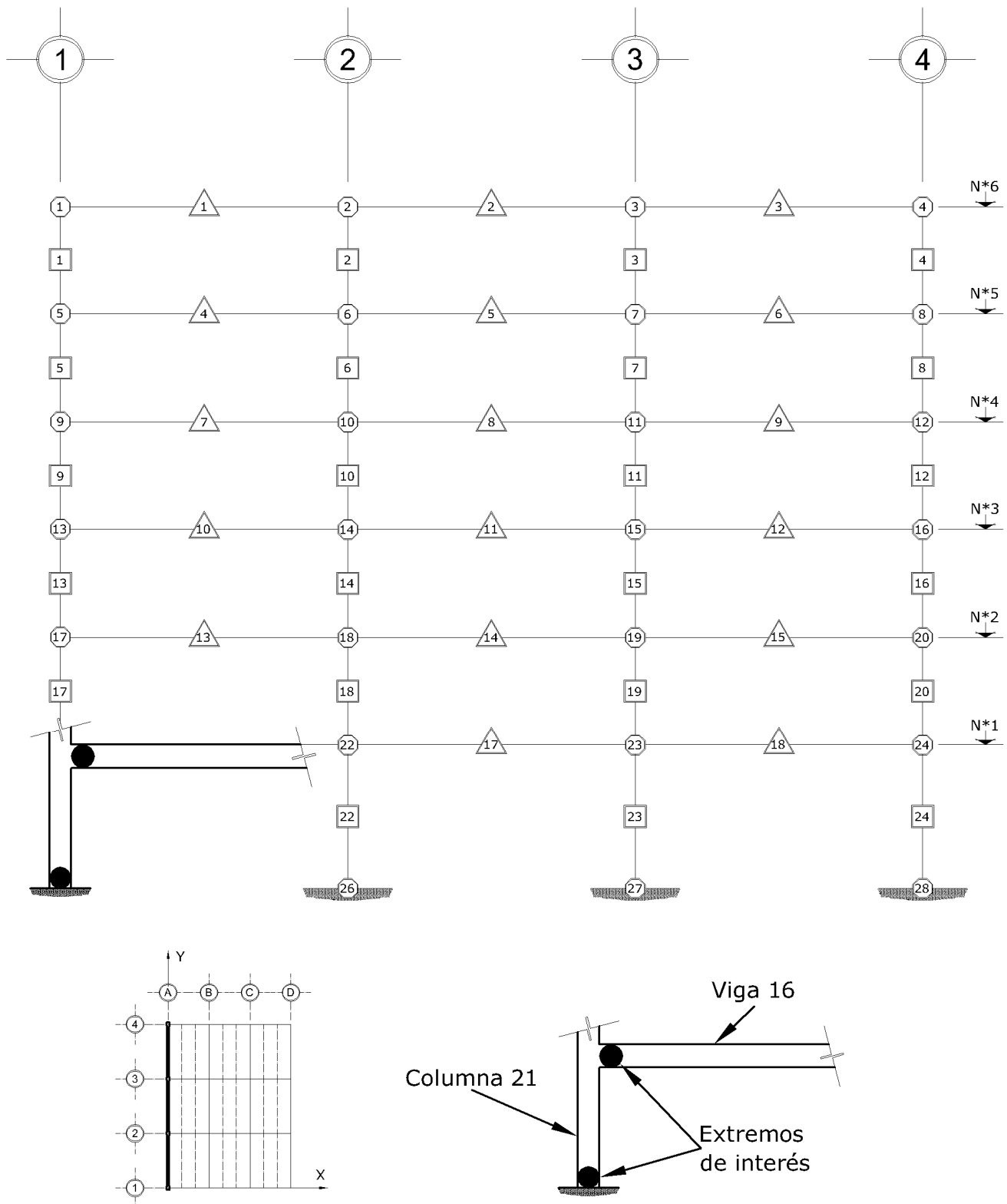
Fig 4.9 Identificación de los extremos en secciones estructurales de la viga 16 y la columna 21 para el estudio de las historias en el tiempo de las respuestas de los análisis paso a paso elásticos e inelásticos (sin y con sobre-resistencias), edificios de 6 niveles, eje A (dirección larga), casos C1 y C2 ( Q = 2 ), D1 y D2 ( Q = 4 )
