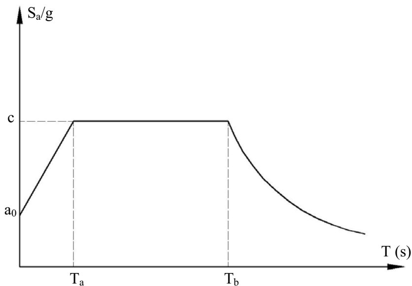
Fig 2.8a Forma típica de los espectros de diseño propuestos por las NTC-Sismo del RDF-04
