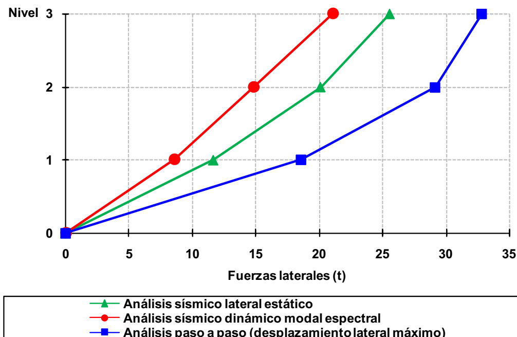
Fig 4.139 Distribución del perfil de fuerzas laterales debidas a diferentes condiciones de análisis sísmico del eje 2, caso A2, (con sobre-resistencias), diseño según el Apéndice A de las NTC-Sismo del RDF-04, edificio de 3 niveles
