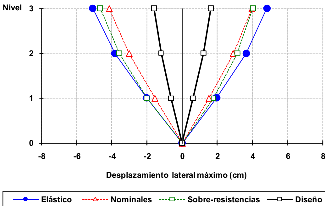
Fig 4.13 Desplazamientos horizontales máximos del eje A, caso B2, análisis paso a paso dinámico (elástico e inelástico) y modal espectral, sin y con efectos de sobre-resistencias, diseño Apéndice A, NTC-Sismo del RDF-04, edificio de 3 niveles
