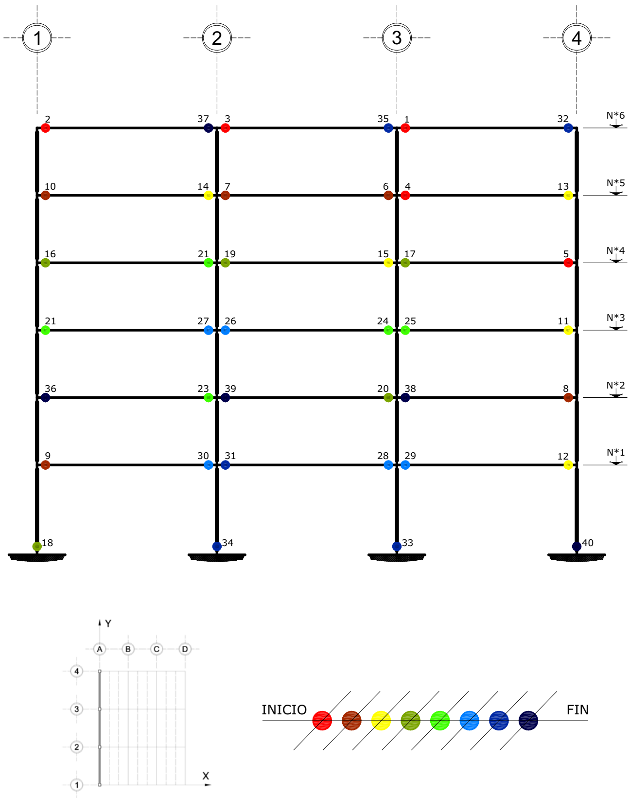
Fig 4.205 Ubicación y secuencia de formación de articulaciones plásticas, análisis Push-over, con sobre-resistencias, edificio de 6 niveles, eje A, caso C2
