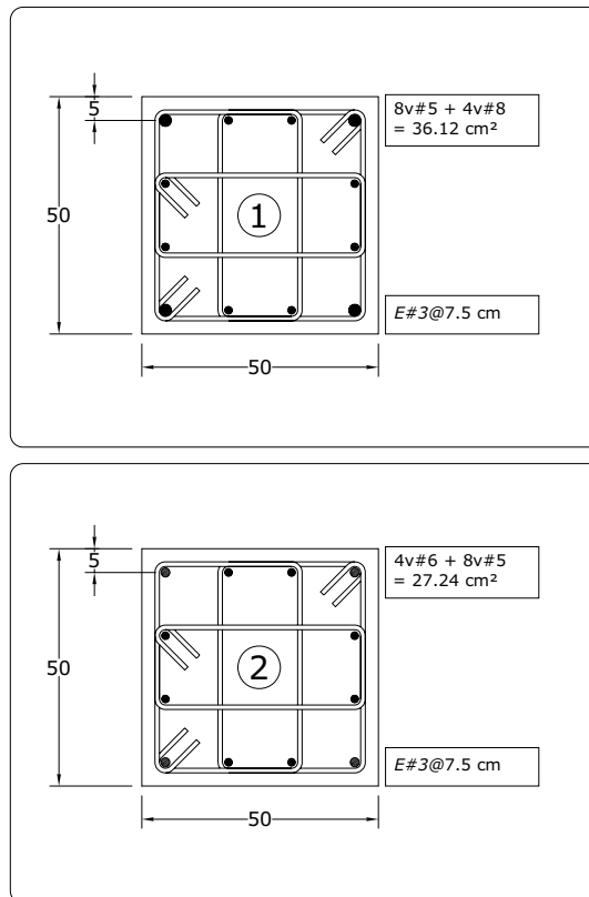
Fig 3.81 Tipos de armados de refuerzo longitudinal y transversal resultantes en los extremos de las columnas del eje 2, caso B2 ( Q = 4 )
