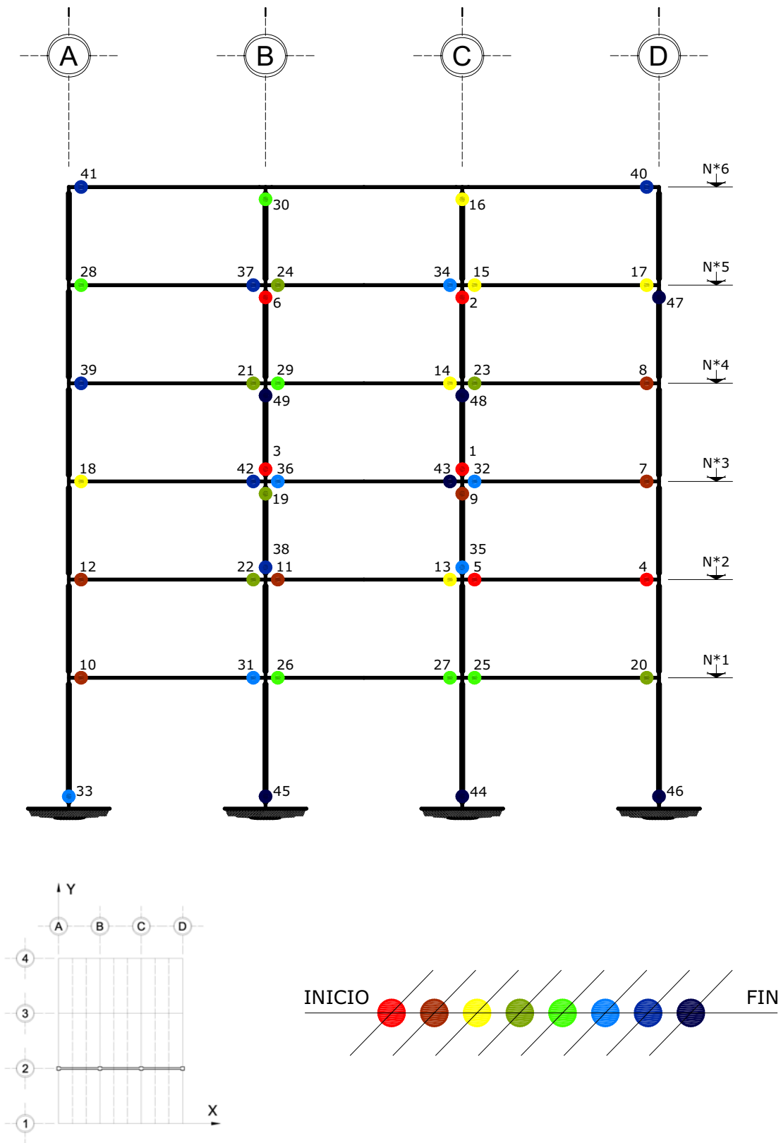
Fig 4.203 Ubicación y secuencia de formación de articulaciones plásticas, análisis Push-over, con sobre-resistencias, edificio de 6 niveles, eje 2, caso C2
