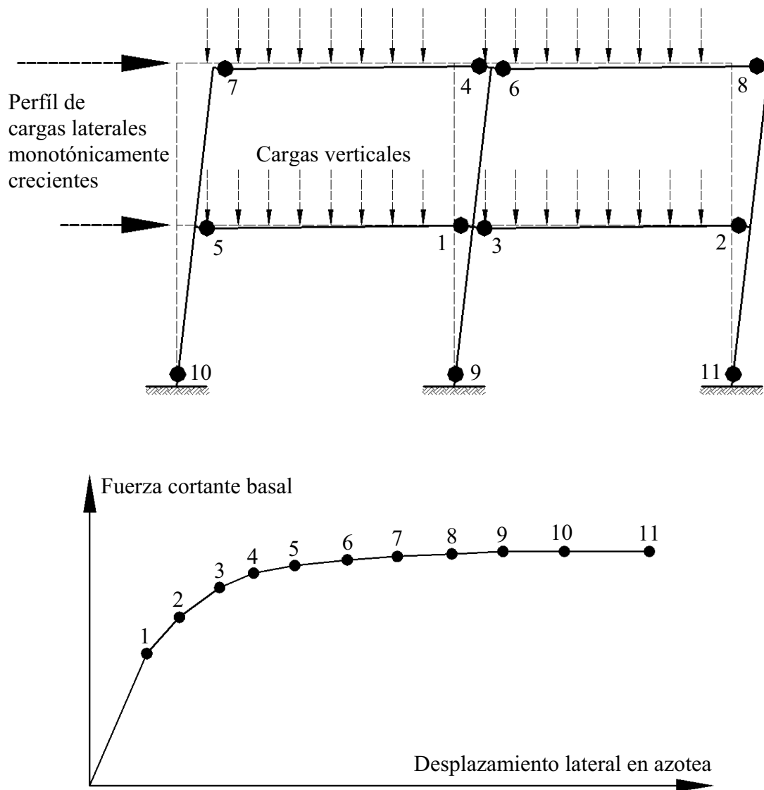
Fig 2.12 Representación del análisis estático no-lineal Push-over en función de la gráfica fuerza cortante basal – desplazamiento lateral en azotea
