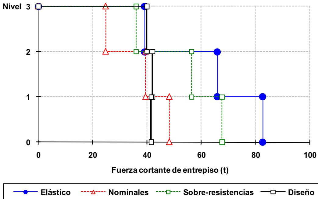
Fig 4.37 Envolventes de fuerzas cortantes de entrepiso del eje A, caso B2, análisis paso a paso elástico e inelástico (sin y con sobre-resistencias) y modal espectral, NTC-Sismo del RDF-04, edificio de 3 niveles
