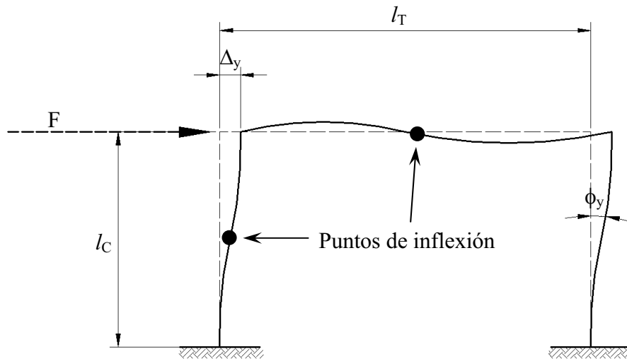
Fig 2.17 Deformada elástica de un marco sujeto a cargas laterales
