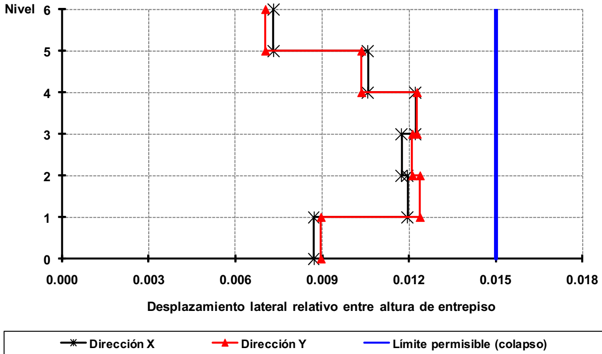
Fig 3.21b Relaciones desplazamiento lateral relativo entre altura de entrepiso (condición de colapso), análisis dinámico modal espectral, edificio de 6 niveles, caso C2 ( Q = 2 )
