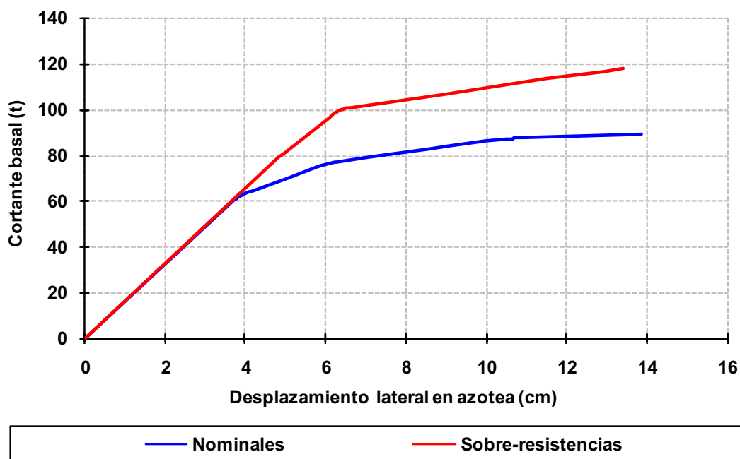
Fig 4.186 Relaciones fuerza cortante basal - desplazamiento horizontal en azotea, eje 2, caso A2, análisis Push-over (sin y con sobre-resistencias), perfil de cargas laterales del análisis dinámico modal espectral, diseño Apéndice A, NTC-Sismo del RDF-04, edificio de 3 niveles
