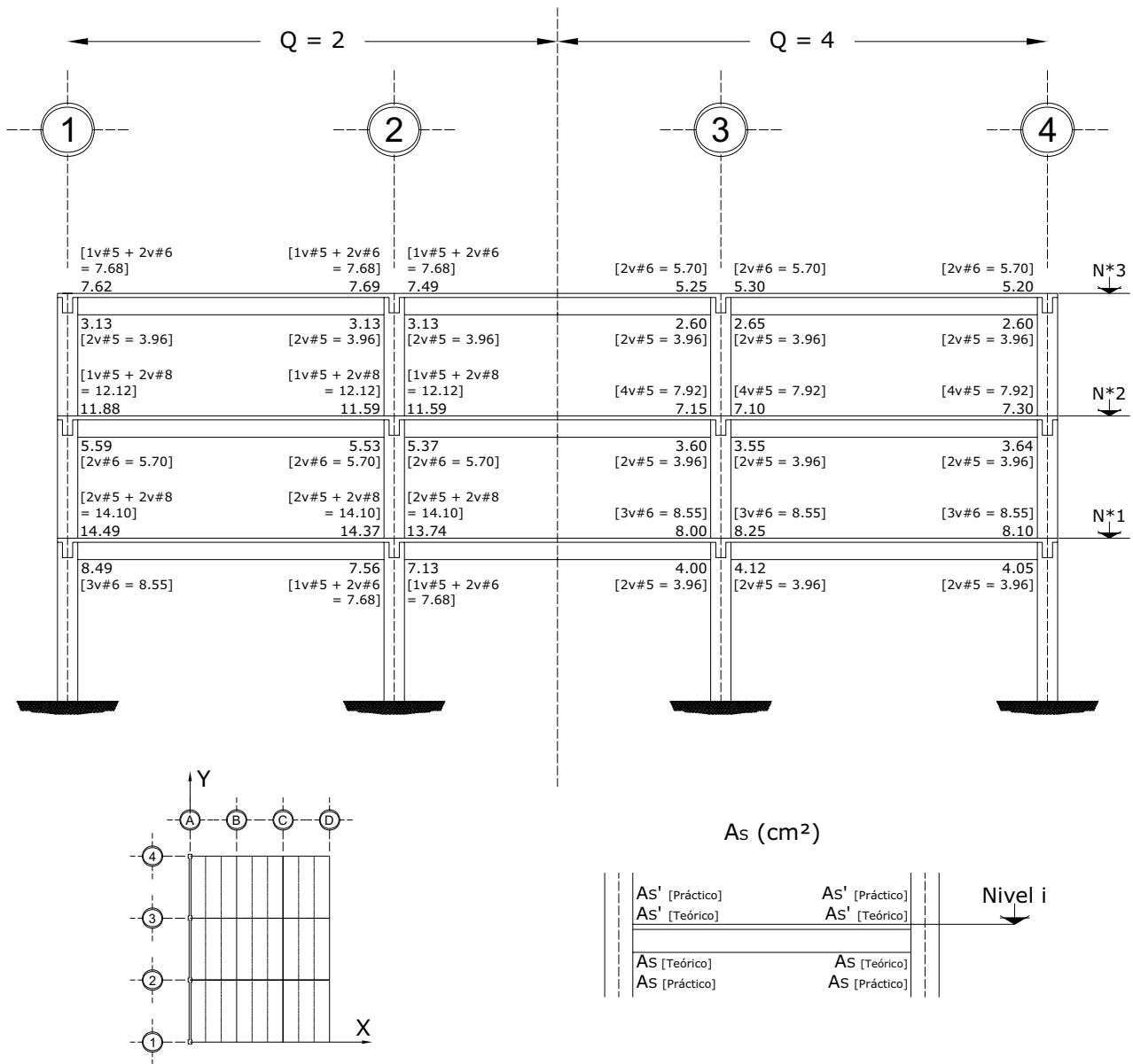
Fig 3.54 Acero de refuerzo longitudinal teórico y práctico necesario en vigas, eje A, casos A1 ( Q = 2 ) y B1 ( Q = 4 )
