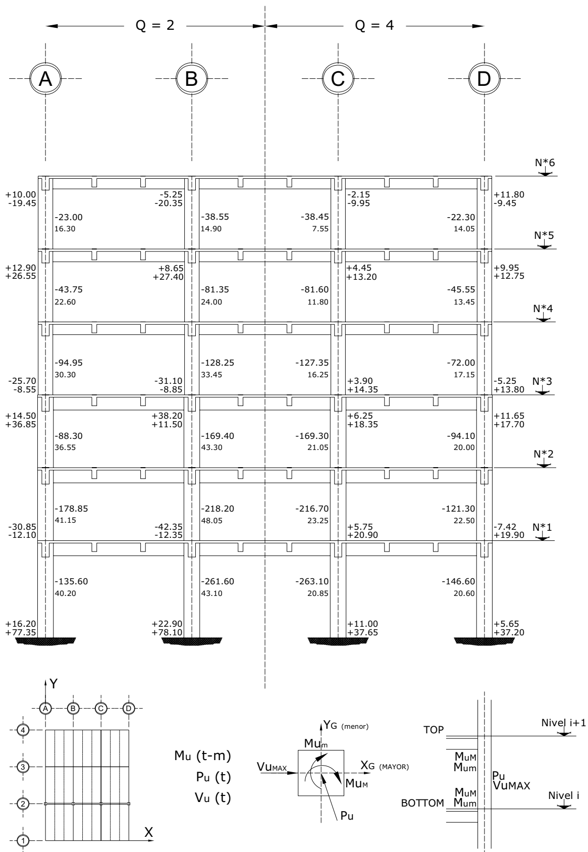
Fig 3.109 Elementos mecánicos últimos en columnas, eje 2, casos C2 (Q = 2) y D2 (Q = 4)
