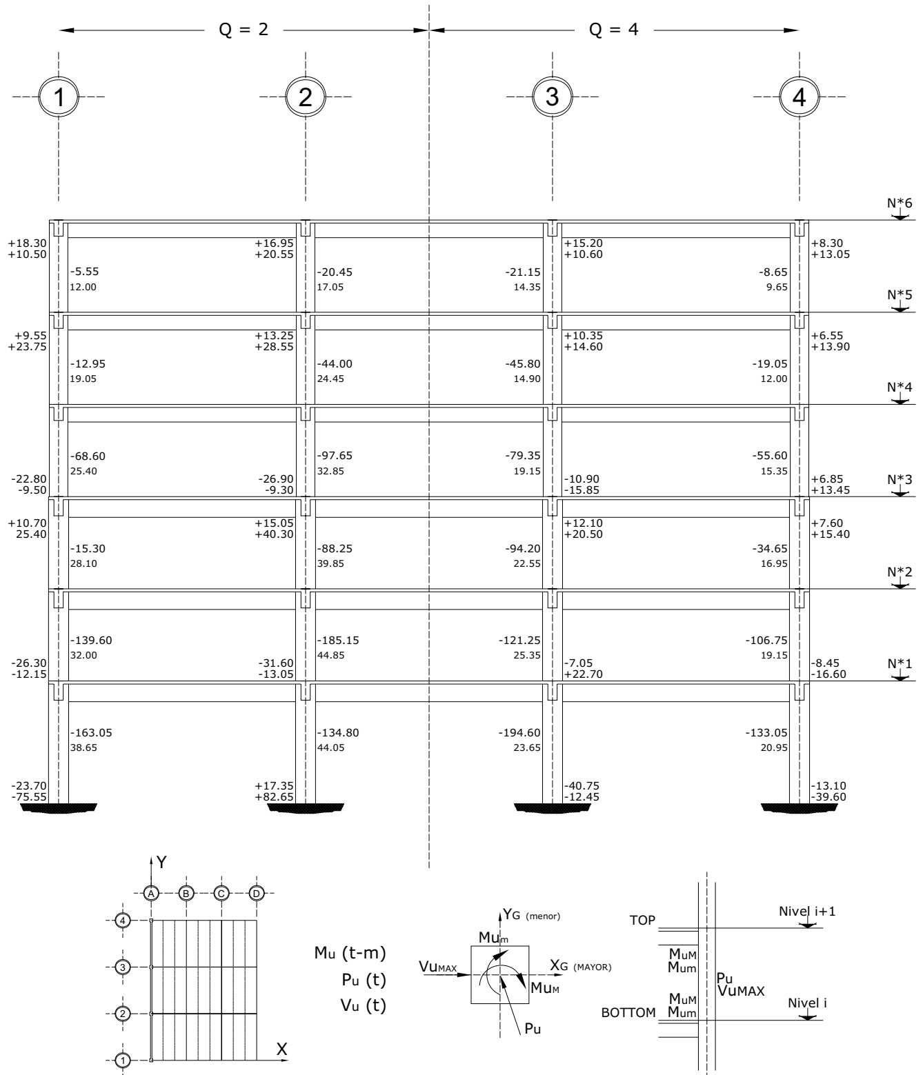
Fig 3.91 Elementos mecánicos últimos en columnas, eje A, casos C1 y D1
