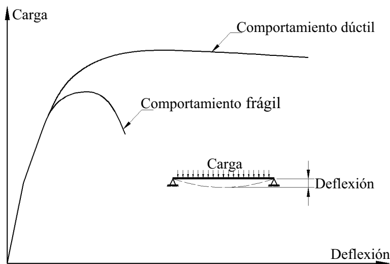
Fig 2.14 Comportamiento de la curva carga-deflexión de un miembro sometido a flexión
