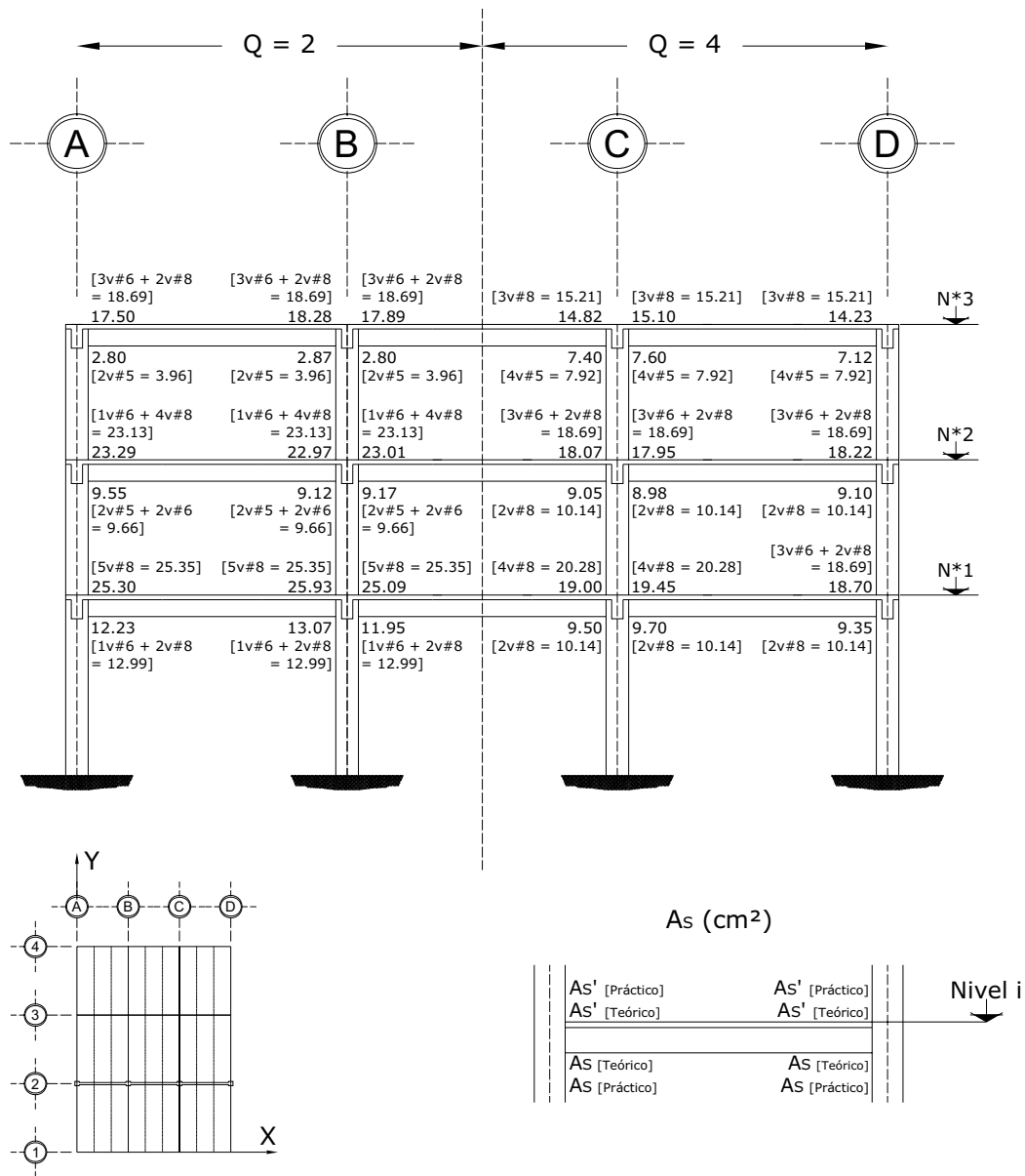
Fig 3.52 Acero de refuerzo longitudinal teórico y práctico necesario en vigas, eje 2, casos A1 (Q = 2) y B1 (Q = 4)
