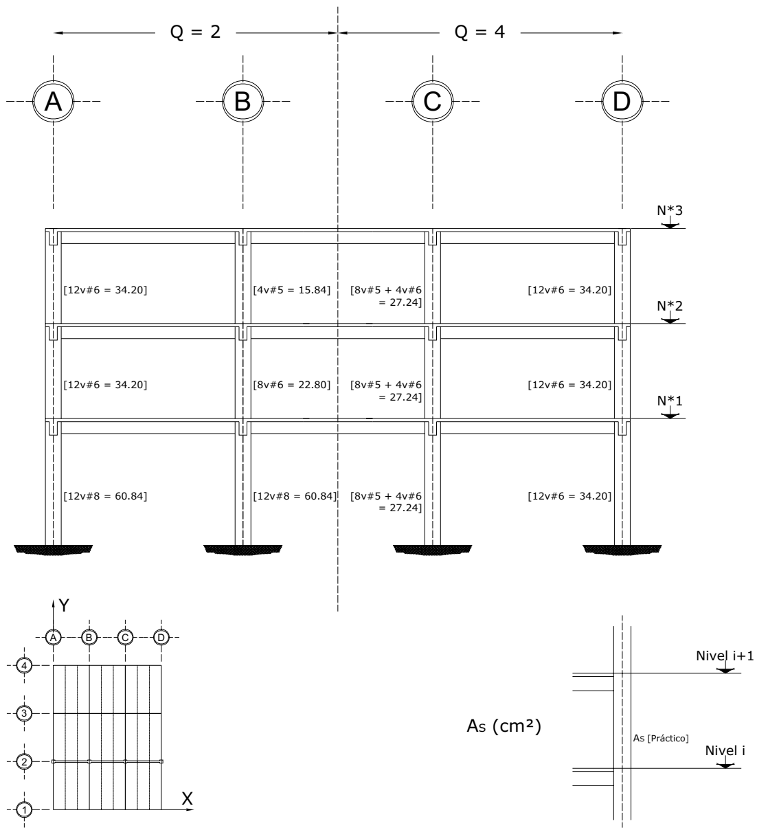
Fig 3.73b Acero de refuerzo longitudinal teórico y práctico necesario en columnas, eje 2, casos A2 (Q = 2) y B2 (Q = 4)
