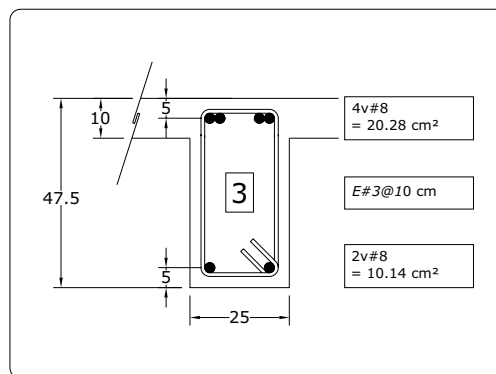
Fig 3.80 Tipos de armados de refuerzo longitudinal y transversal resultantes en los extremos de las vigas del eje 2, caso B2 (Q = 4)
