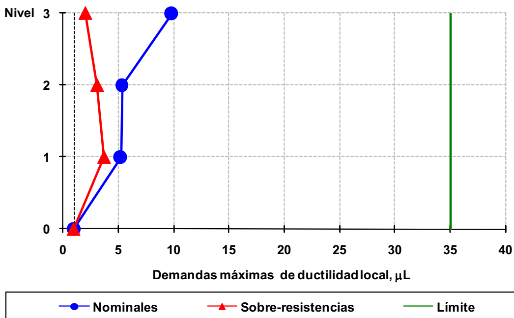
Fig 4.170 Demandas máximas de ductilidad local desarrolladas en vigas del eje 2, caso A2, análisis Push-over (sin y con sobre-resistencias), perfil de cargas laterales del análisis dinámico modal espectral, diseño Apéndice A, NTC-Sismo del RDF-04, edificio de 3 niveles
