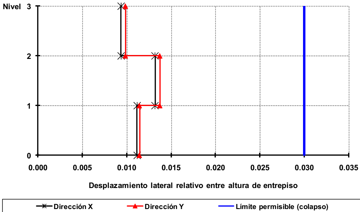
Fig 3.19b Relaciones desplazamiento lateral relativo entre altura de entrepiso (condición de colapso), análisis dinámico modal espectral, edificio de 3 niveles, caso B2 (Q = 4)
