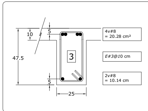
Fig 3.60 Tipos de armados de refuerzo longitudinal y transversal resultantes en los extremos de las vigas del eje 2, caso B1 (Q = 4)
