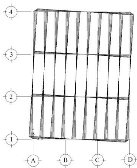
Fig 3.14 Deformada en planta del primer modo de vibración de torsión, edificio de 6 niveles
