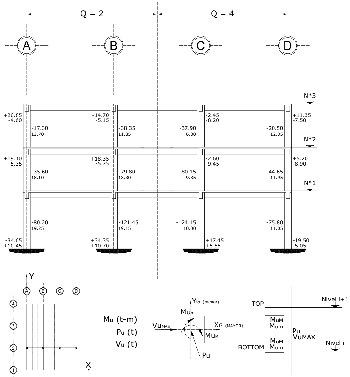
Fig 3.69 Elementos mecánicos últimos en columnas, eje 2, casos A2 ( Q = 2 ) y B2 ( Q = 4 )
