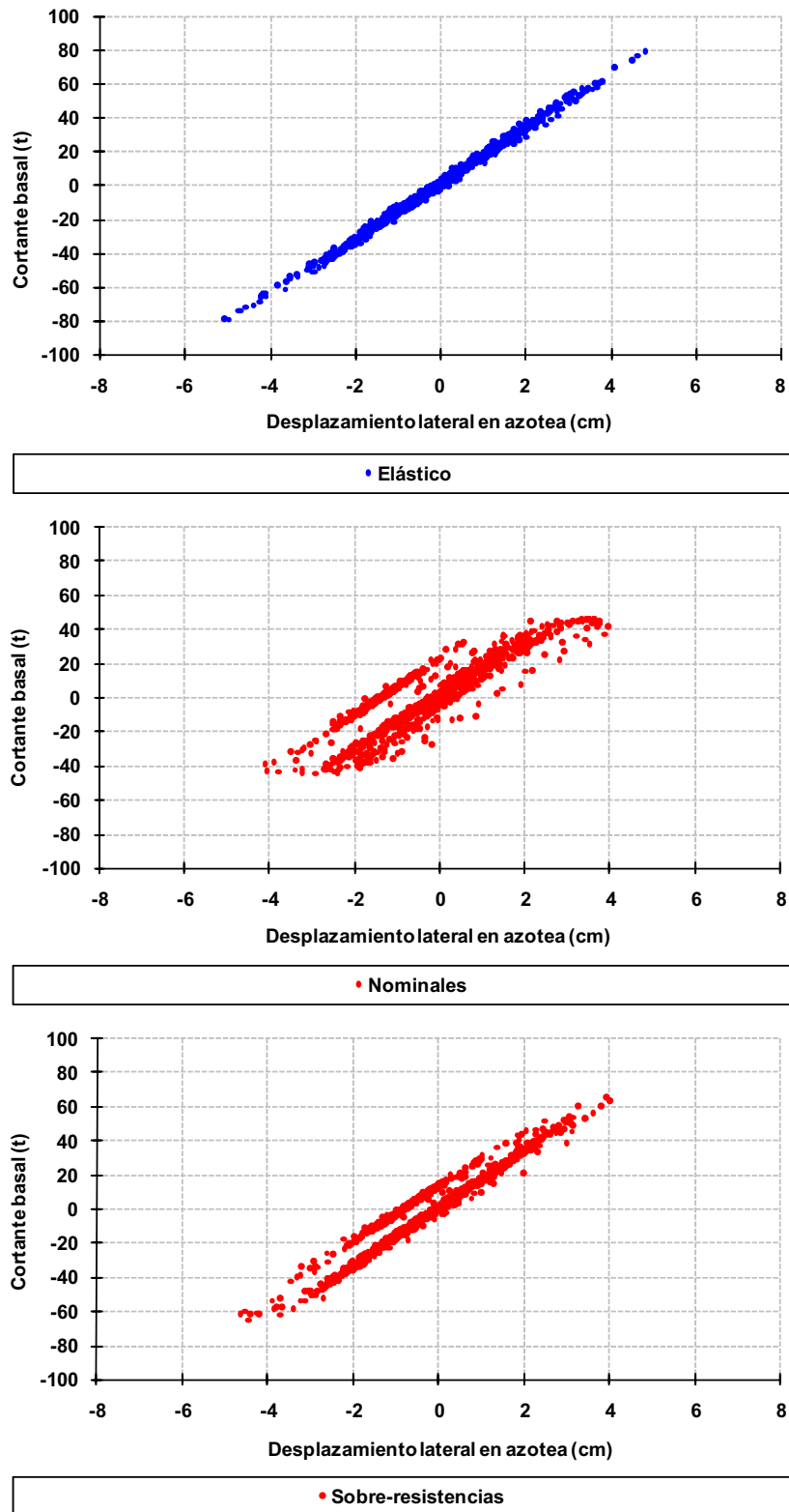
Fig 4.53 Relaciones fuerza cortante basal - desplazamiento horizontal en azotea, eje A, caso B2, análisis paso a paso elástico e inelástico (sin y con sobre-resistencias), diseño Apéndice A, NTC-Sismo del RDF-04, edificio de 3 niveles
