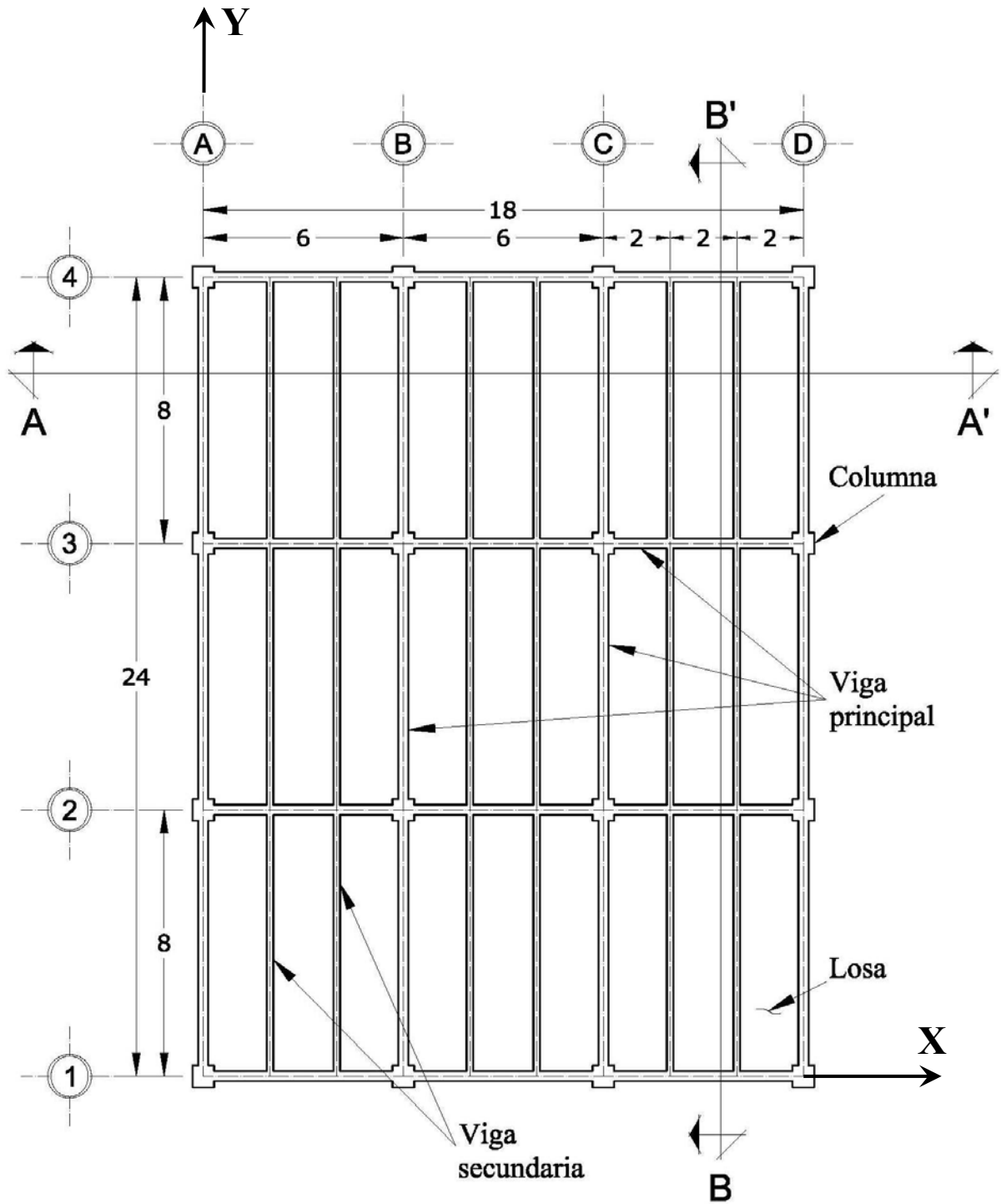
Fig 3.1 Planta estructural tipo de los modelos en estudio (cotas en metros)
