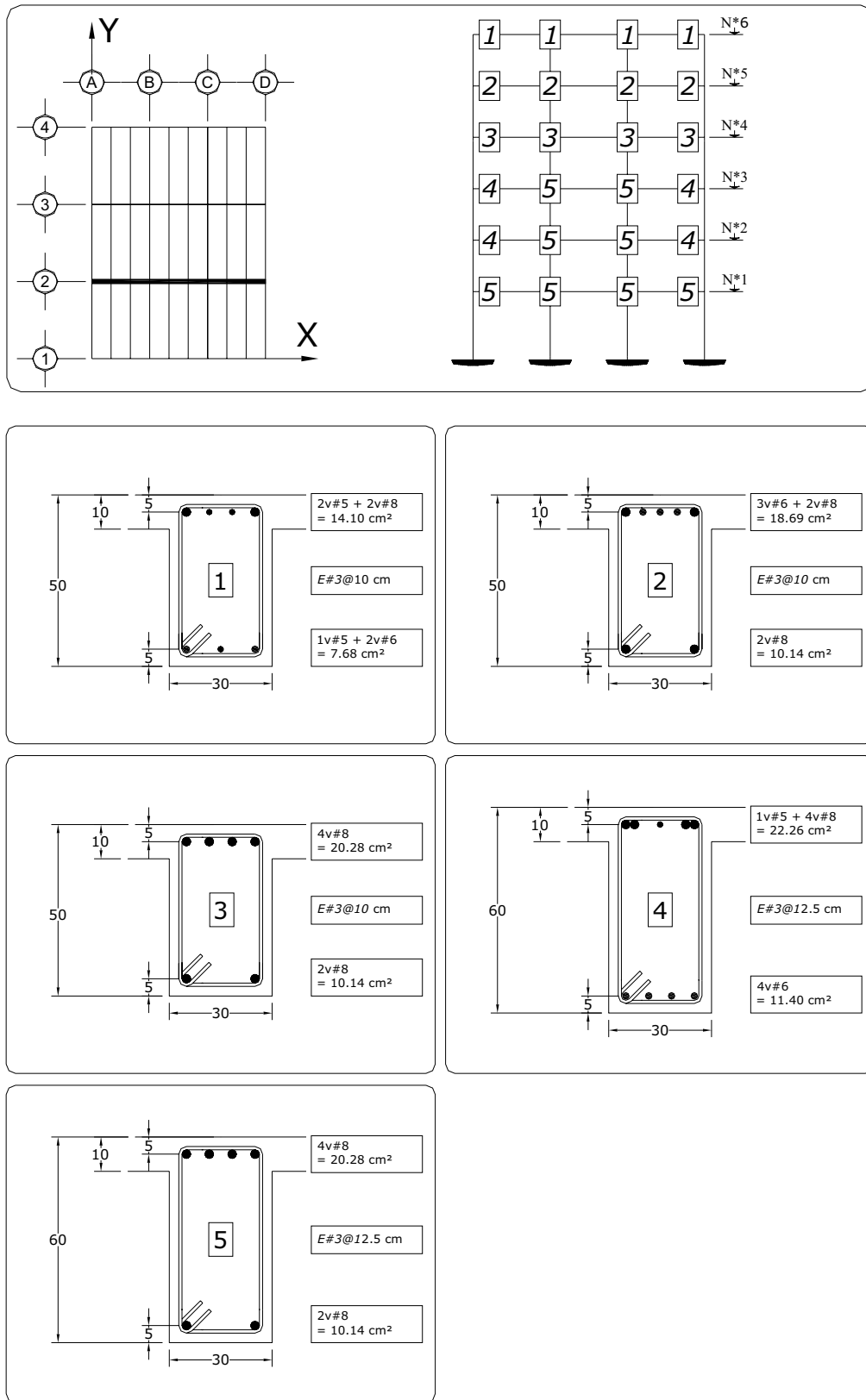
Fig 3.120 Tipos de armados de refuerzo longitudinal y transversal resultantes en los extremos de las vigas del eje 2, caso D2 (Q = 4)
