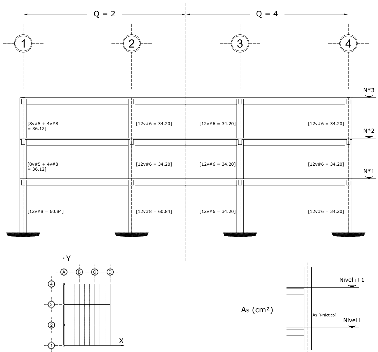
Fig 3.75b Acero de refuerzo longitudinal teórico y práctico necesario en columnas, eje A, casos A2 ( Q = 2 ) y B2 ( Q = 4 )
