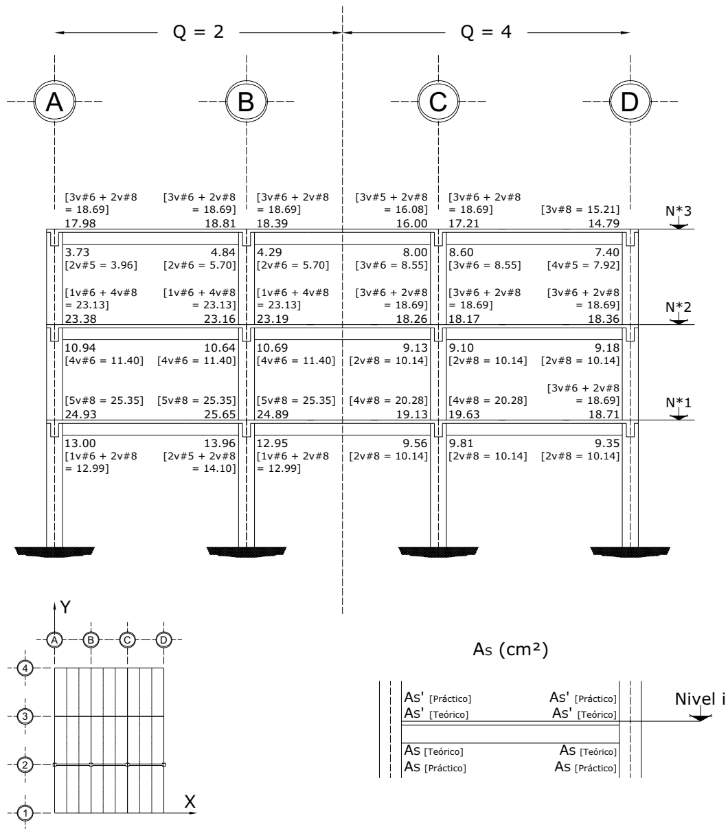
Fig 3.72 Acero de refuerzo longitudinal teórico y práctico necesario en vigas, eje 2, casos A2 (Q = 2) y B2 (Q = 4)
