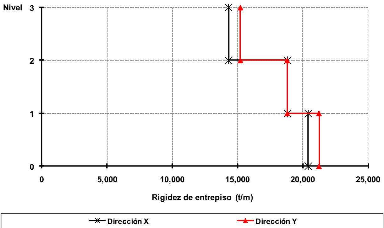
Fig 3.42 Rigideces de entrepiso, edificio 3 niveles, caso B1 (Q = 4)
