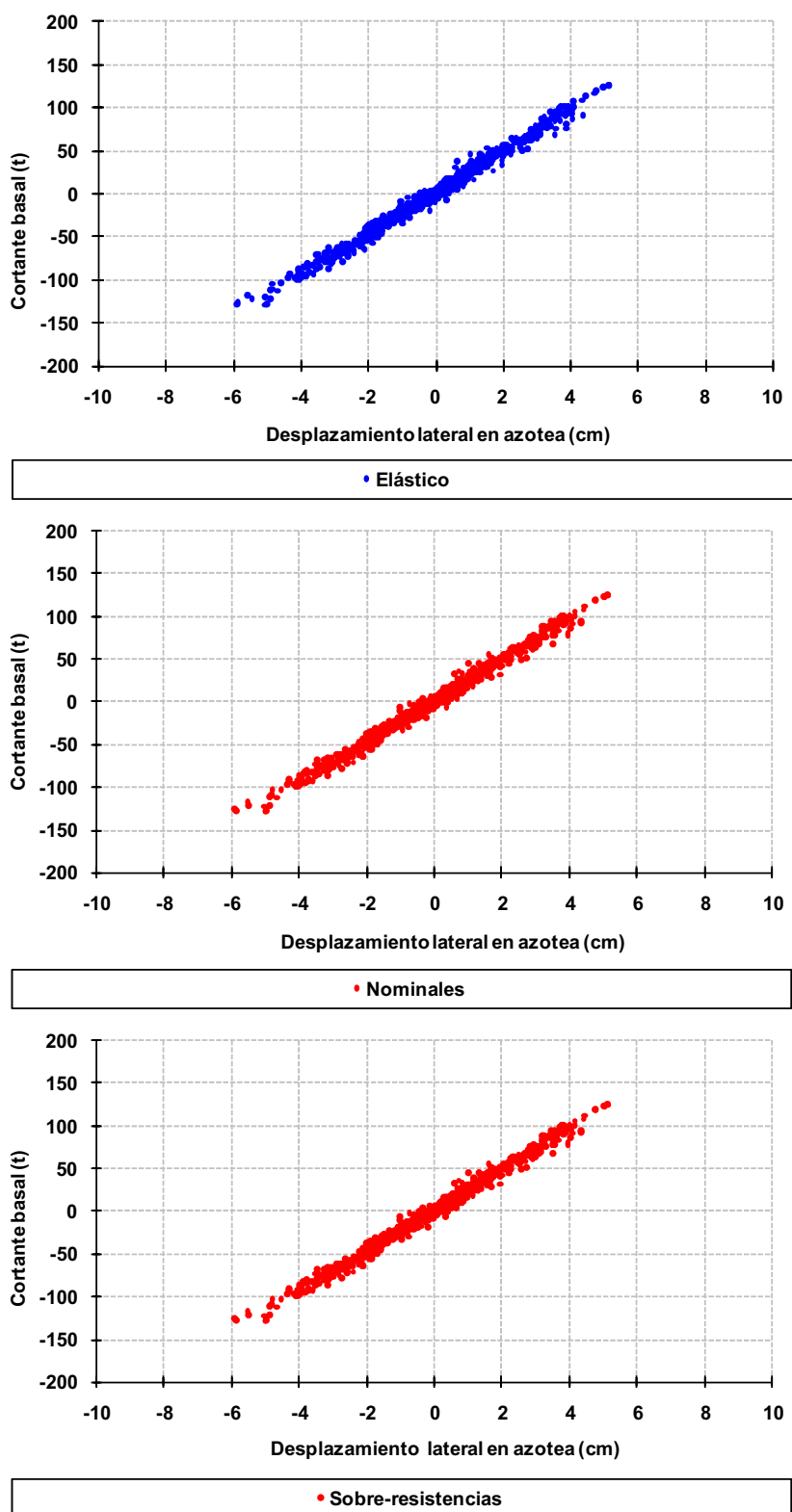
Fig 4.54 Relaciones fuerza cortante basal - desplazamiento horizontal en azotea, eje 2, caso C2, análisis paso a paso elástico e inelástico (sin y con sobre-resistencias), diseño Apéndice A, NTC-Sismo del RDF-04, edificio de 6 niveles
