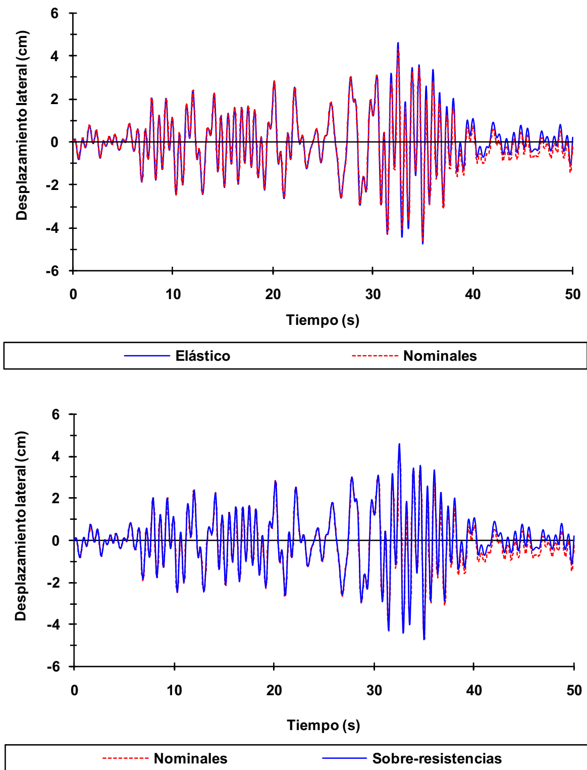
Fig 4.18 Historias de desplazamientos laterales de azotea, eje 2, caso A2, análisis paso a paso elástico e inelástico (sin y con sobre-resistencia), diseño Apéndice A, NTC-Sismo del RDF-04, edificio de 3 niveles
