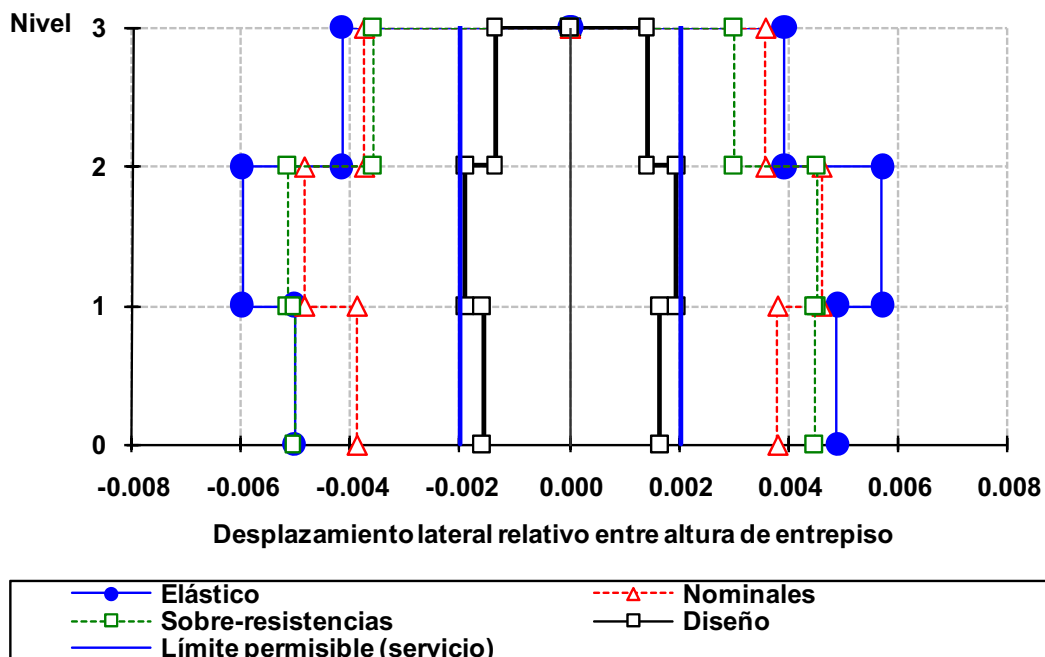
Fig 4.29 Relaciones desplazamiento lateral relativo entre altura de entrepiso del eje A, caso B2, análisis paso a paso elástico e inelástico (sin y con sobre-resistencias) y modal espectral, NTC-Sismo del RDF-04, edificio de 3 niveles
