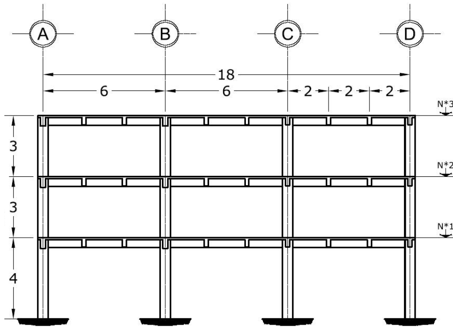
Fig 3.1a Corte estructural AA' del modelo de 3 niveles (cotas en metros)
