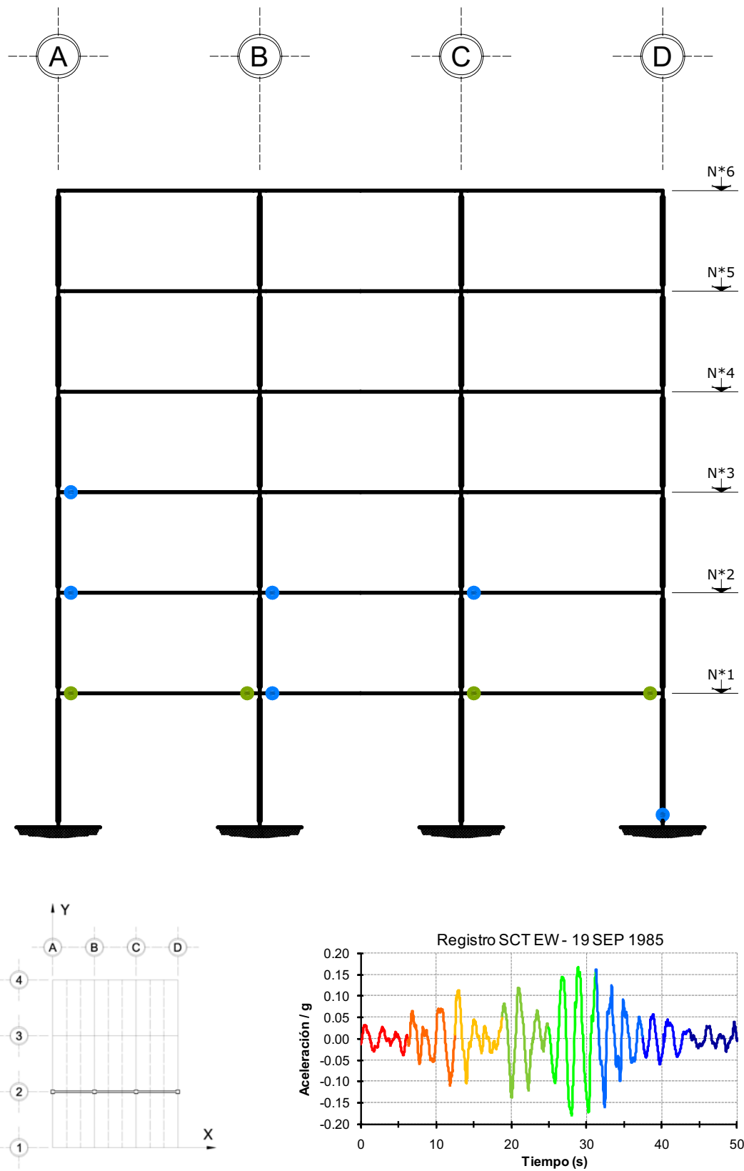
Fig 4.135 Ubicación y secuencia de formación de articulaciones plásticas, análisis paso a paso, con sobre-resistencias, edificio de 6 niveles, eje 2, caso D2
