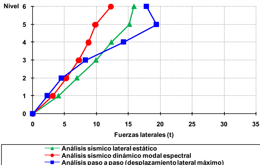
Fig 4.152 Distribución del perfil de fuerzas laterales debidas a diferentes condiciones de análisis sísmico del eje A, caso D2, (sin sobre-resistencias), diseño según el Apéndice A de las NTC-Sismo del RDF-04, edificio de 6 niveles
