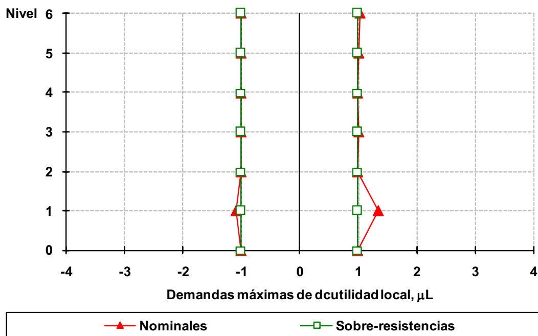
Fig 4.95 Demandas máximas de ductilidad local desarrolladas en vigas del eje A, caso C2, análisis paso a paso elástico e inelástico (sin y con sobre-resistencias), NTC-Sismo del RDF-04, edificio de 6 niveles
