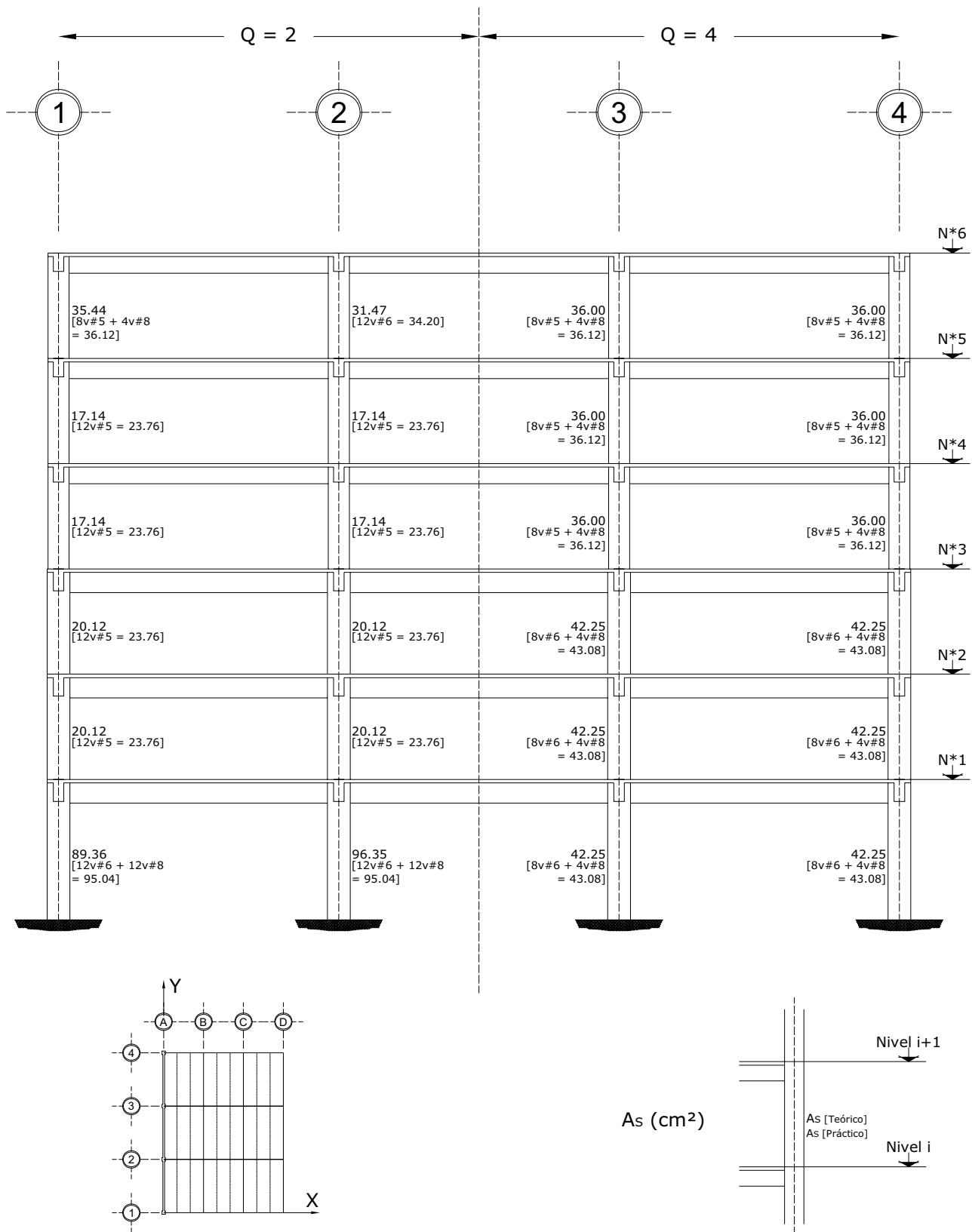
Fig 3.115a Acero de refuerzo longitudinal teórico y práctico necesario en columnas, eje A, casos C2 (Q = 2) y D2 (Q = 4)
