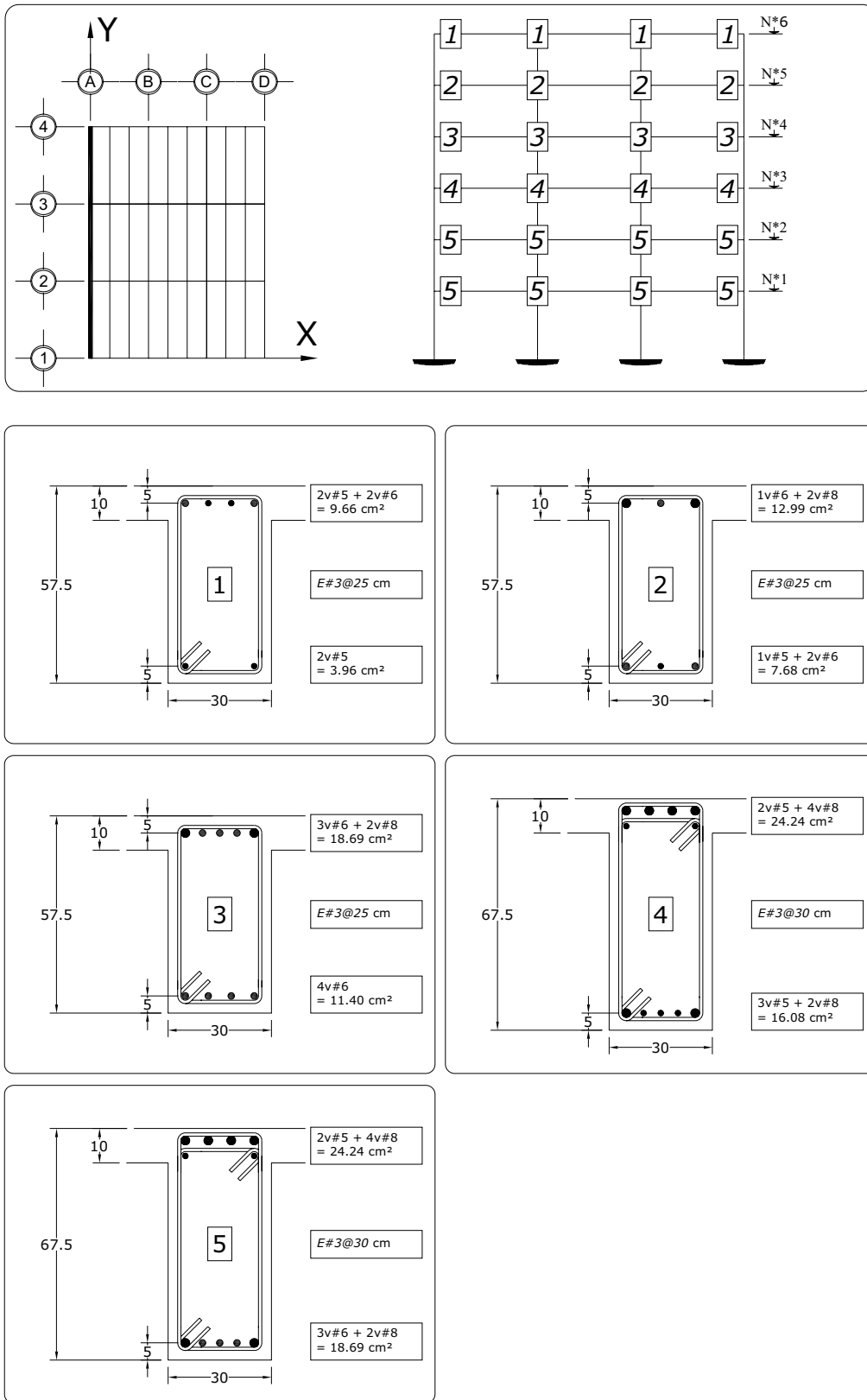
Fig 3.98 Tipos de armados de refuerzo longitudinal y transversal resultantes en los extremos de las vigas del eje A, caso C1 (Q = 2)
