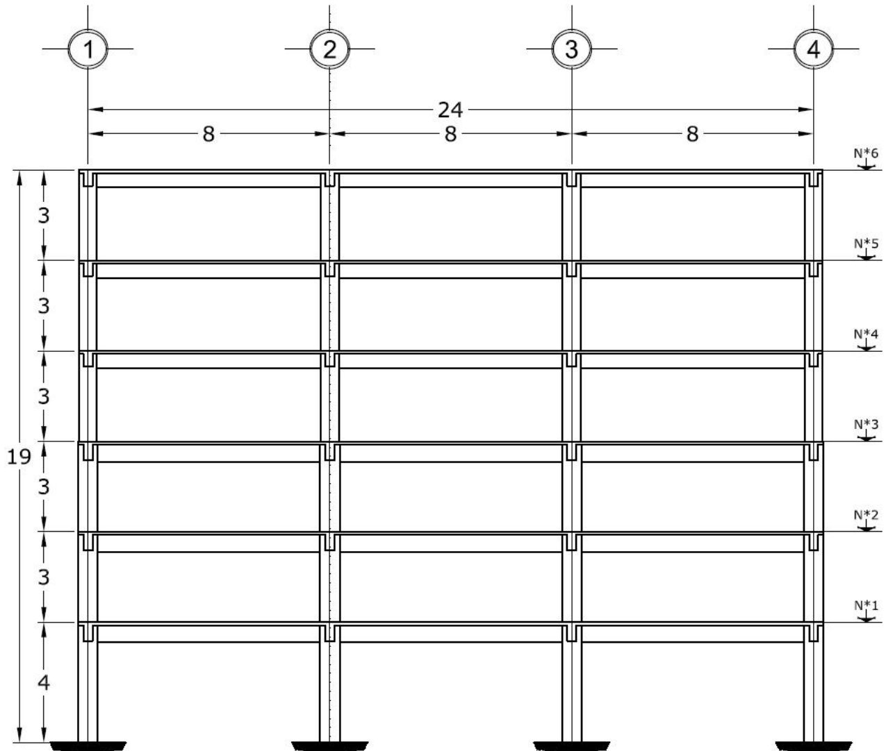
Fig 3.1d Corte estructural tipo BB' del modelo de 6 niveles (cotas en metros)
