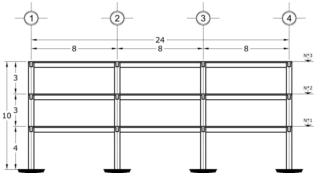
Fig 3.1b Corte estructural tipo BB' del modelo de 3 niveles (cotas en metros)
