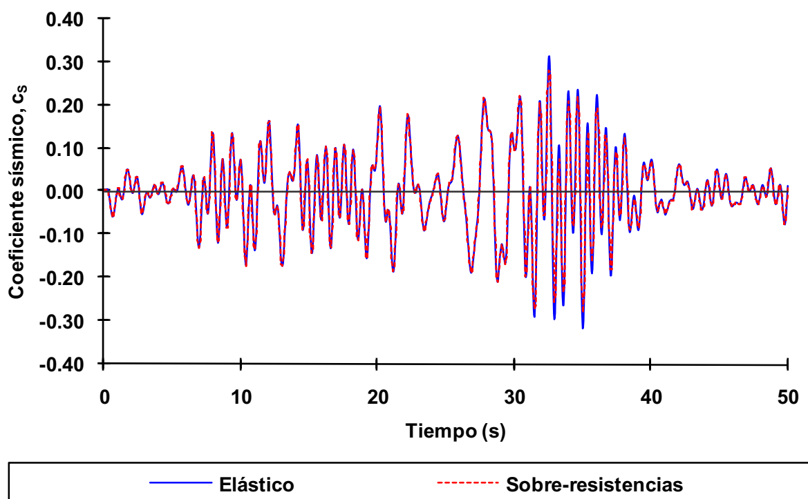
Fig 4.44 Historias de coeficientes sísmicos ( c_s ), eje 2, caso B2, análisis paso a paso elástico e inelástico (sin y con sobre-resistencias), diseño Apéndice A, NTC-Sismo del RDF-04, edificio de 3 niveles
