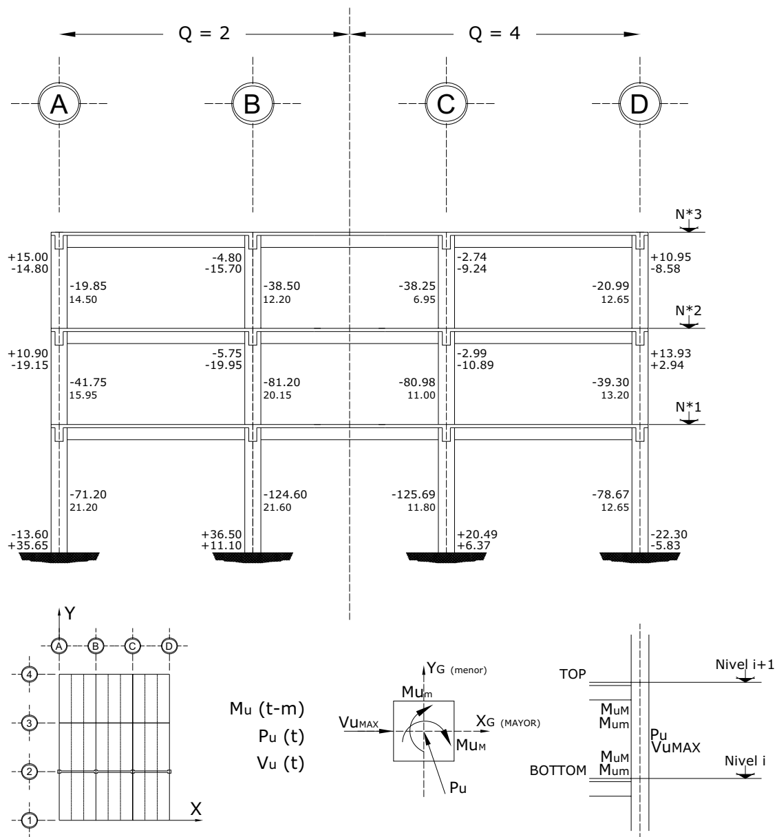
Fig 3.49 Elementos mecánicos últimos en columnas, eje 2, casos A1 ( Q = 2 ) y B1 ( Q = 4 )
