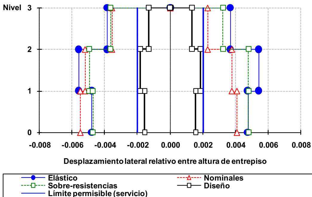
Fig 4.28 Relaciones desplazamiento lateral relativo entre altura de entrepiso del eje 2, caso B2, análisis paso a paso elástico e inelástico (sin y con sobre-resistencias) y modal espectral, NTC-Sismo del RDF-04, edificio de 3 niveles
