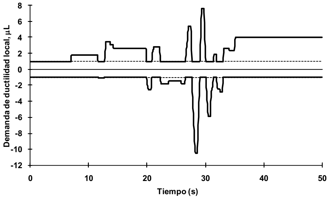
Fig 4.112 Demanda de ductilidad local desarrollada en el extremo izquierdo de la viga 16 del nivel 1, eje A, caso D2, análisis paso a paso inelástico (sin sobre-resistencias), NTC-Sismo del RDF-04, edificio de 6 niveles
