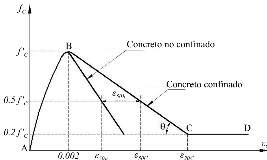
Fig 2.23 Modelo de Kent y Park modificado para el diagrama esfuerzo- deformación del concreto a compresión con y sin confinamiento
