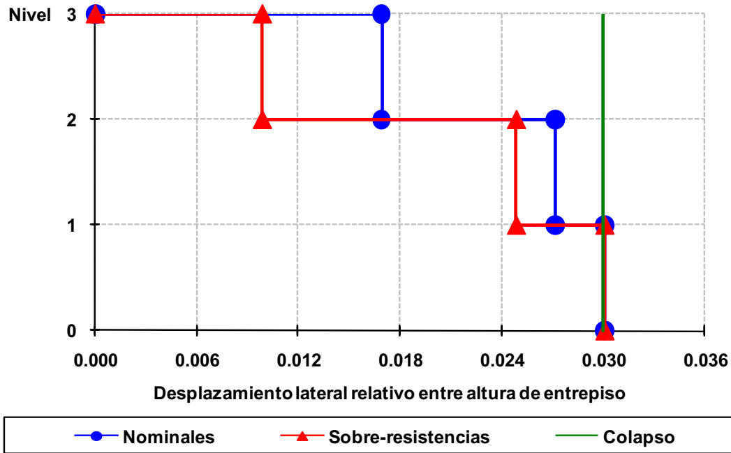
Fig 4.164 Relaciones desplazamiento lateral relativo entre altura de entrepiso del eje 2, caso B2, análisis Push-over (sin y con sobre-resistencias), perfil de cargas laterales del análisis dinámico modal espectral, diseño Apéndice A, NTC-Sismo del RDF-04, edificio de 3 niveles
