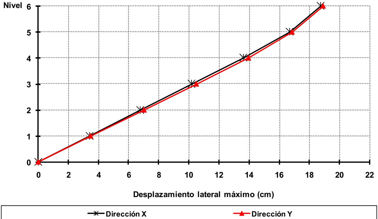
Fig 3.31b Desplazamientos laterales máximos, análisis dinámico modal espectral (condición de colapso), edificio de 6 niveles, caso D2 ( Q = 4 )
