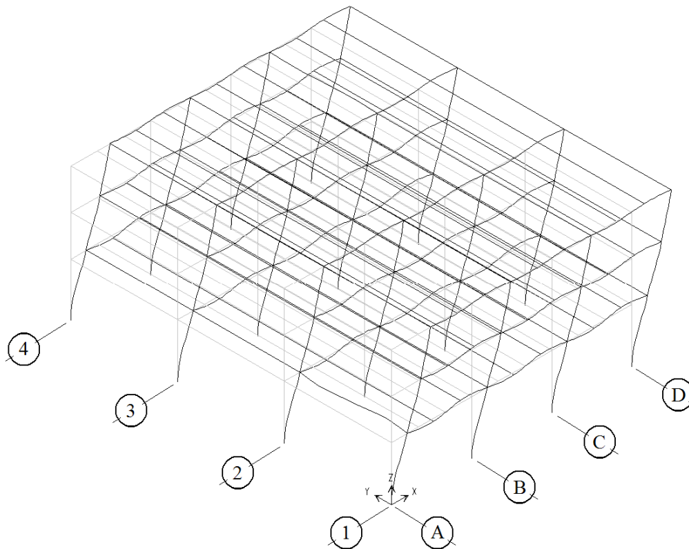
Fig 3.7 Deformada en perspectiva del primer modo de vibración, dirección corta, edificio de 3 niveles
