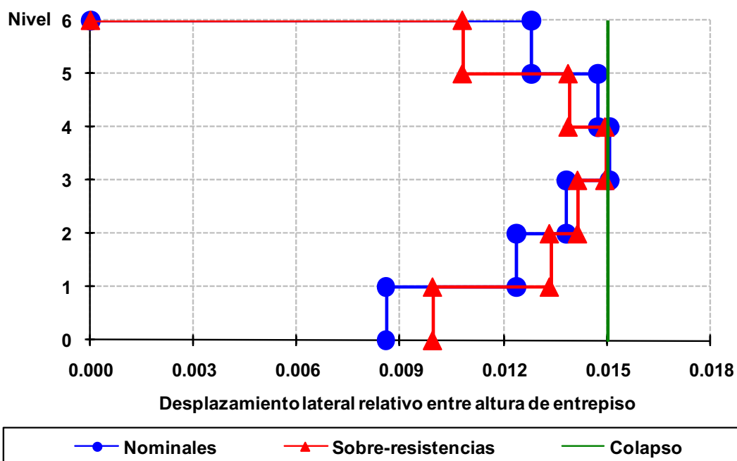
Fig 4.166 Relaciones desplazamiento lateral relativo entre altura de entrepiso del eje 2, caso C2, análisis Push-over (sin y con sobre-resistencias), perfil de cargas laterales del análisis dinámico modal espectral, diseño Apéndice A, NTC-Sismo del RDF-04, edificio de 6 niveles
