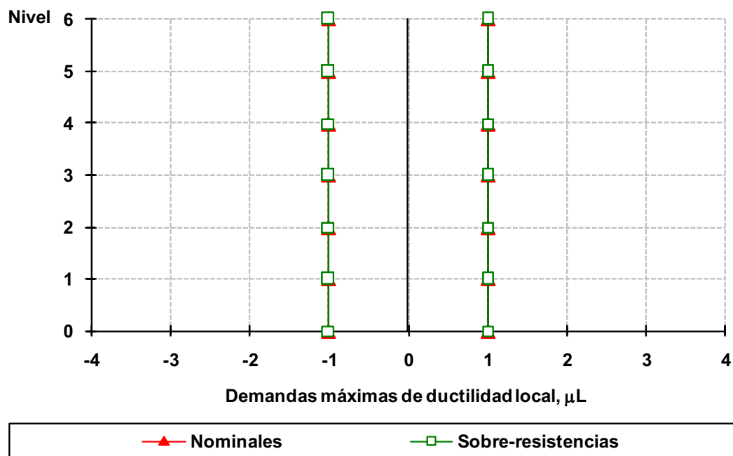
Fig 4.119 Demandas máximas de ductilidad local desarrolladas en columnas del eje A, caso C2, análisis paso a paso elástico e inelástico (sin y con sobre-resistencias), NTC-Sismo del RDF-04, edificio de 6 niveles
