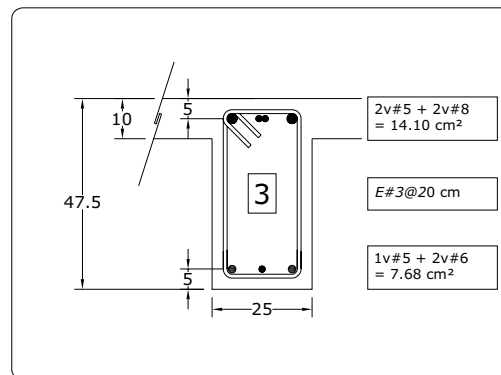
Fig 3.78 Tipos de armados de refuerzo longitudinal y transversal resultantes en los extremos de las vigas del eje A, caso A2 (Q = 2)
