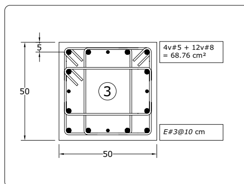
Fig 3.57 Tipos de armados de refuerzo longitudinal y transversal resultantes en los extremos de las columnas del eje 2, caso A1 (Q = 2)
