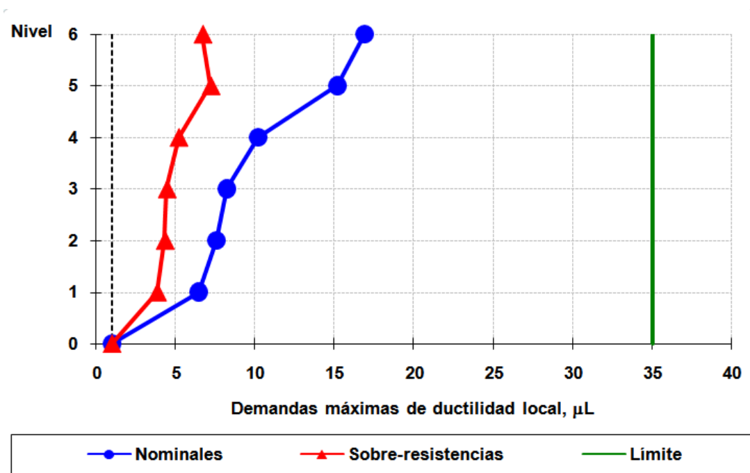
Fig 4.174 Demandas máximas de ductilidad local desarrolladas en vigas del eje 2, caso C2, análisis Push-over (sin y con sobre-resistencias), perfil de cargas laterales del análisis dinámico modal espectral, diseño Apéndice A, NTC-Sismo del RDF-04, edificio de 6 niveles
