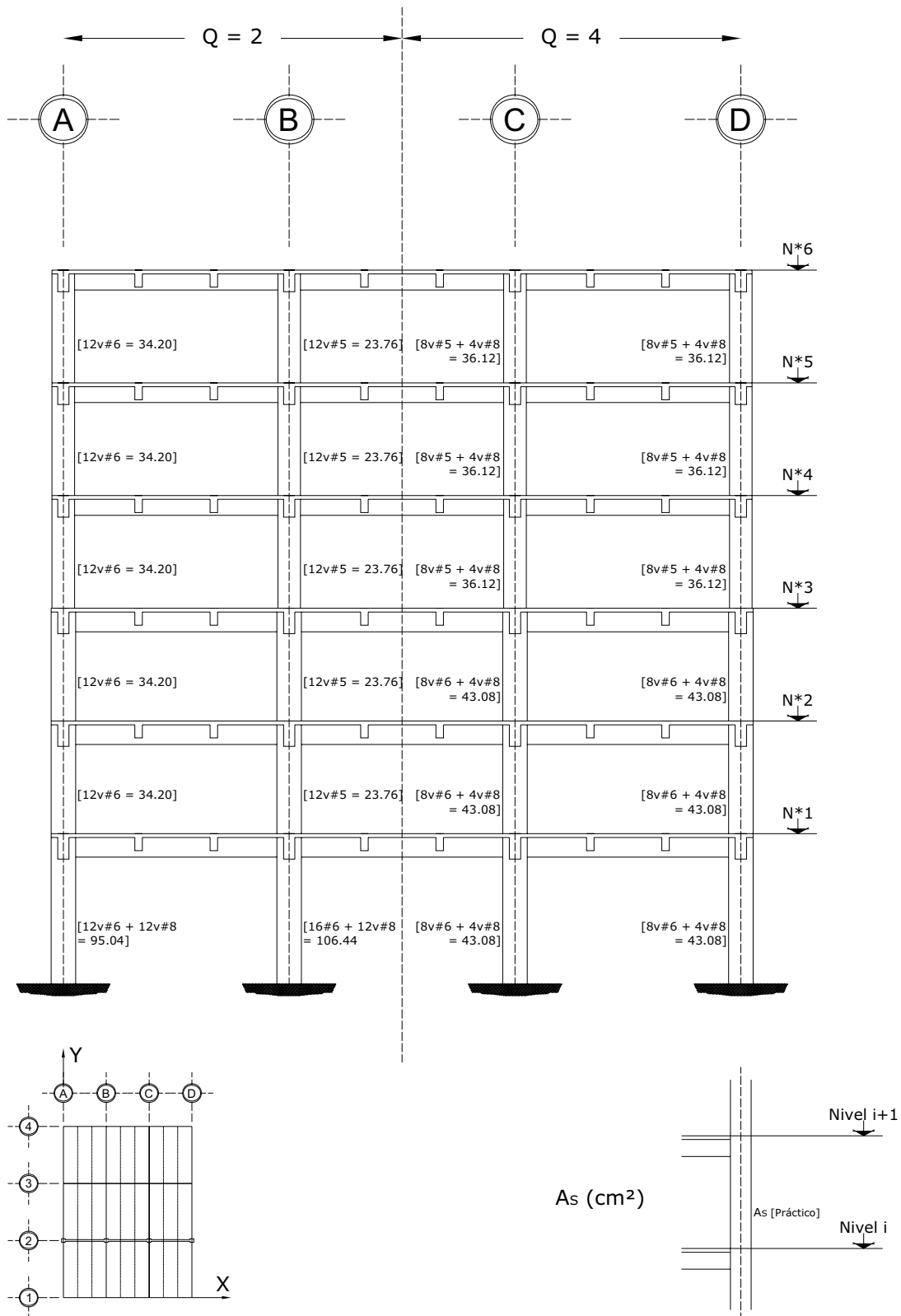
Fig 3.113b Acero de refuerzo longitudinal teórico y práctico necesario en columnas, eje 2, casos C2 (Q = 2) y D2 (Q = 4)
