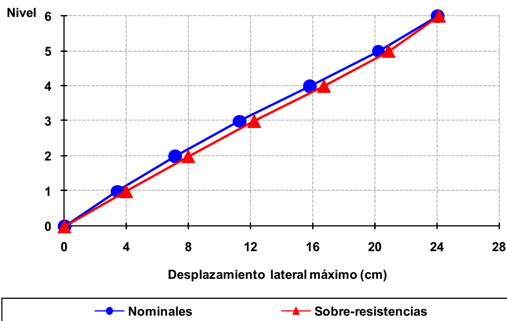
Fig 4.158 Desplazamientos laterales máximos del eje 2, caso C2, análisis Push-over (sin y con sobre-resistencias), perfil de cargas laterales del análisis dinámico modal espectral, diseño Apéndice A, NTC-Sismo del RDF-04, edificio de 6 niveles
