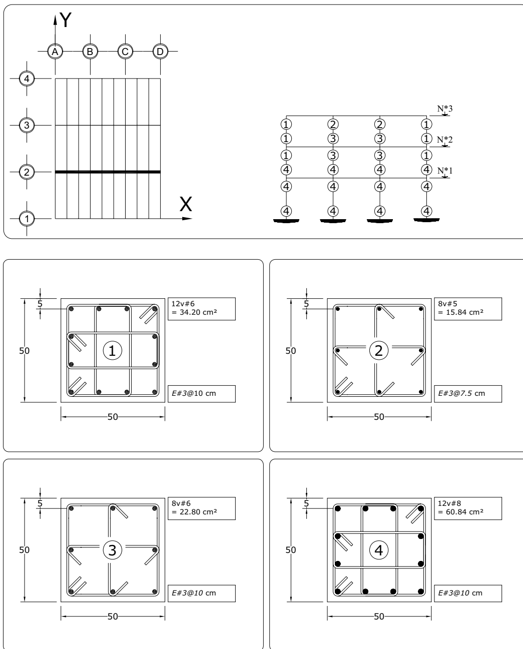
Fig 3.77 Tipos de armados de refuerzo longitudinal y transversal resultantes en los extremos de las columnas de 1 eje 2, caso A2 (Q = 2)
