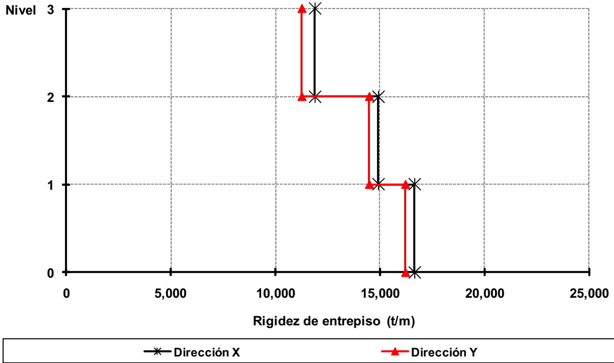
Fig 3.41 Rigideces de entrepiso, edificio 3 niveles, caso A2 (Q = 2)
