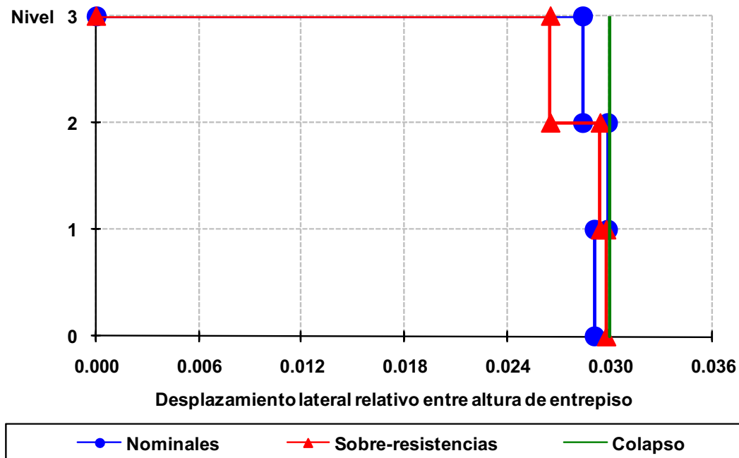
Fig 4.165 Relaciones desplazamiento lateral relativo entre altura de entrepiso del eje A, caso B2, análisis Push-over (sin y con sobre-resistencias), perfil de cargas laterales del análisis dinámico modal espectral, diseño Apéndice A, NTC-Sismo del RDF-04, edificio de 3 niveles
