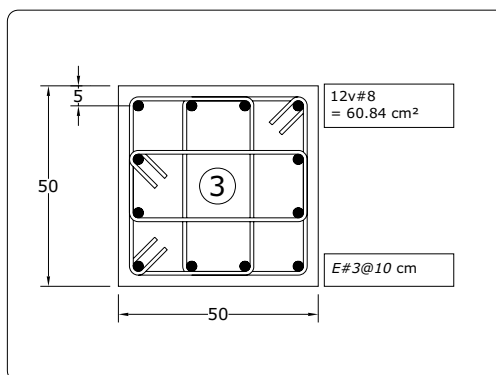
Fig 3.79 Tipos de armados de refuerzo longitudinal y transversal resultantes en los extremos de las columnas del eje A, caso A2 (Q = 2)
