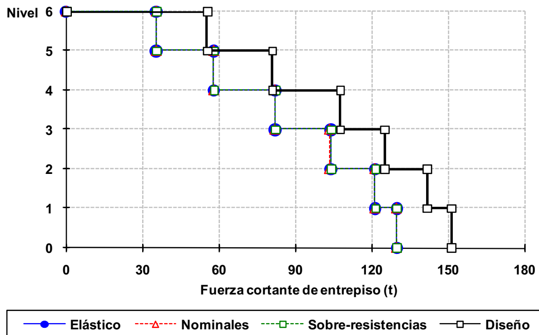
Fig 4.39 Envolventes de fuerzas cortantes de entrepiso del eje A, caso C2, análisis paso a paso elástico e inelástico (sin y con sobre-resistencias) y modal espectral, NTC-Sismo del RDF-04, edificio de 6 niveles
