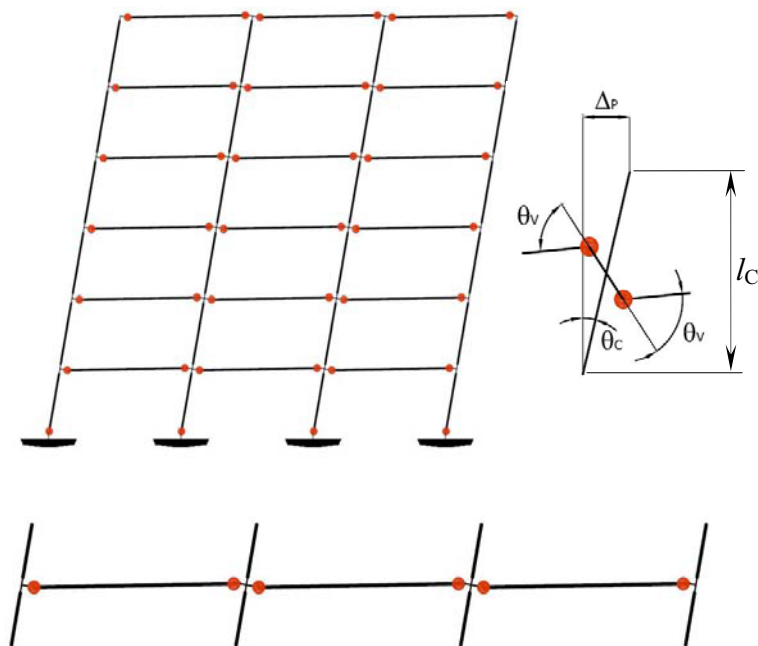
Fig 2.19 Mecanismo de falla de un entrepiso por columnas fuertes y vigas débiles
