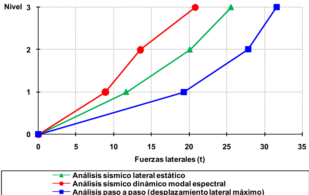
Fig 4.141 Distribución del perfil de fuerzas laterales debidas a diferentes condiciones de análisis sísmico del eje A, caso A2, (con sobre-resistencias), diseño según el Apéndice A de las NTC-Sismo del RDF-04, edificio de 3 niveles
