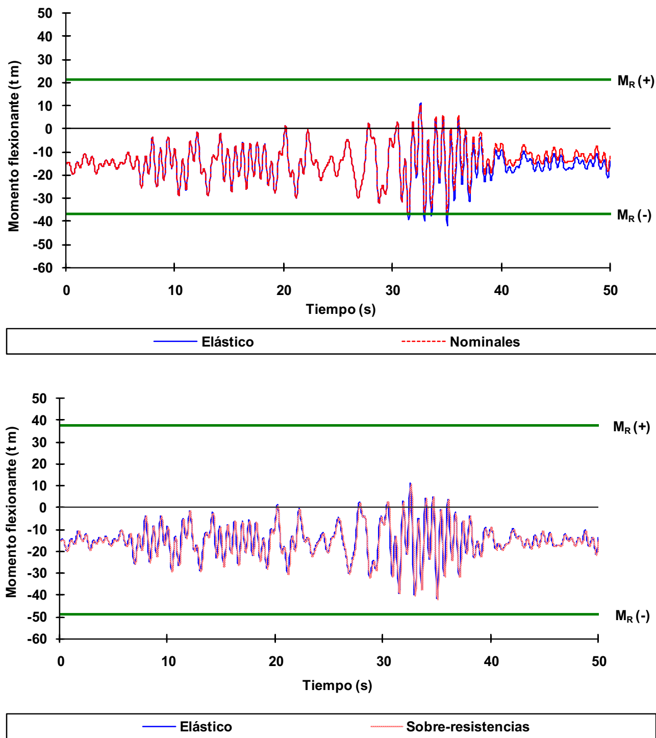
Fig 4.58 Historias de momentos flexionantes del extremo izquierdo de la viga 7 del nivel 1 del eje 2, caso A2, análisis paso a paso elástico e inelástico (sin y con sobre-resistencias), diseño Apéndice A, NTC-Sismo del RDF-04, edificio de 3 niveles
