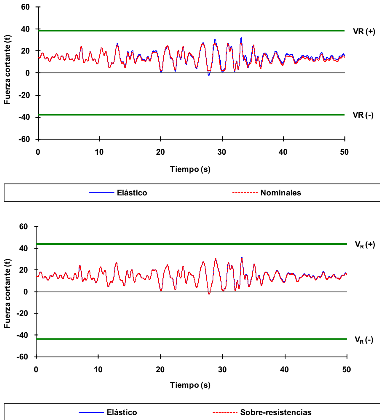
Fig 4.72 Historias de fuerzas cortantes actuantes del extremo izquierdo de la viga 16 del nivel 1 del eje 2, caso D2, análisis paso a paso elástico e inelástico (sin y con sobre-resistencias), diseño Apéndice A, NTC-Sismo del RDF-04, edificio de 6 niveles
