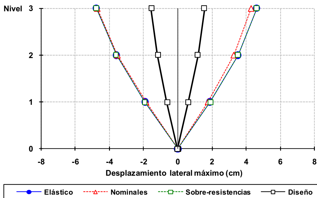
Fig 4.10 Desplazamientos horizontales máximos del eje 2, caso A2, análisis paso a paso dinámico (elástico e inelástico) y modal espectral, sin y con efectos de sobre-resistencias, diseño Apéndice A, NTC-Sismo del RDF-04, edificio de 3 niveles
