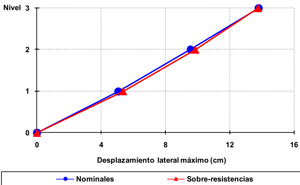
Fig 4.155 Desplazamientos laterales máximos del eje A, caso A2, análisis Push-over (sin y con sobre-resistencias), perfil de cargas laterales del análisis dinámico modal espectral, diseño Apéndice A, NTC-Sismo del RDF-04, edificio de 3 niveles
