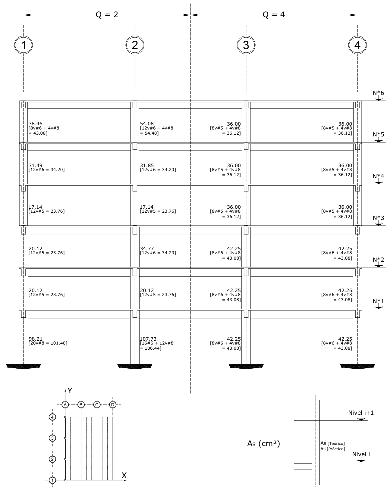
Fig 3.95a Acero de refuerzo longitudinal teórico y práctico necesario en columnas, eje A, casos C1 (Q = 2) y D1 (Q = 4)
