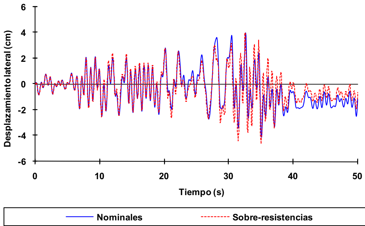
Fig 4.21 Historias de desplazamientos laterales de azotea, eje A, caso B2, análisis paso a paso elástico e inelástico (sin y con sobre-resistencias), diseño Apéndice A, NTC-Sismo del RDF-04, edificio de 3 niveles
