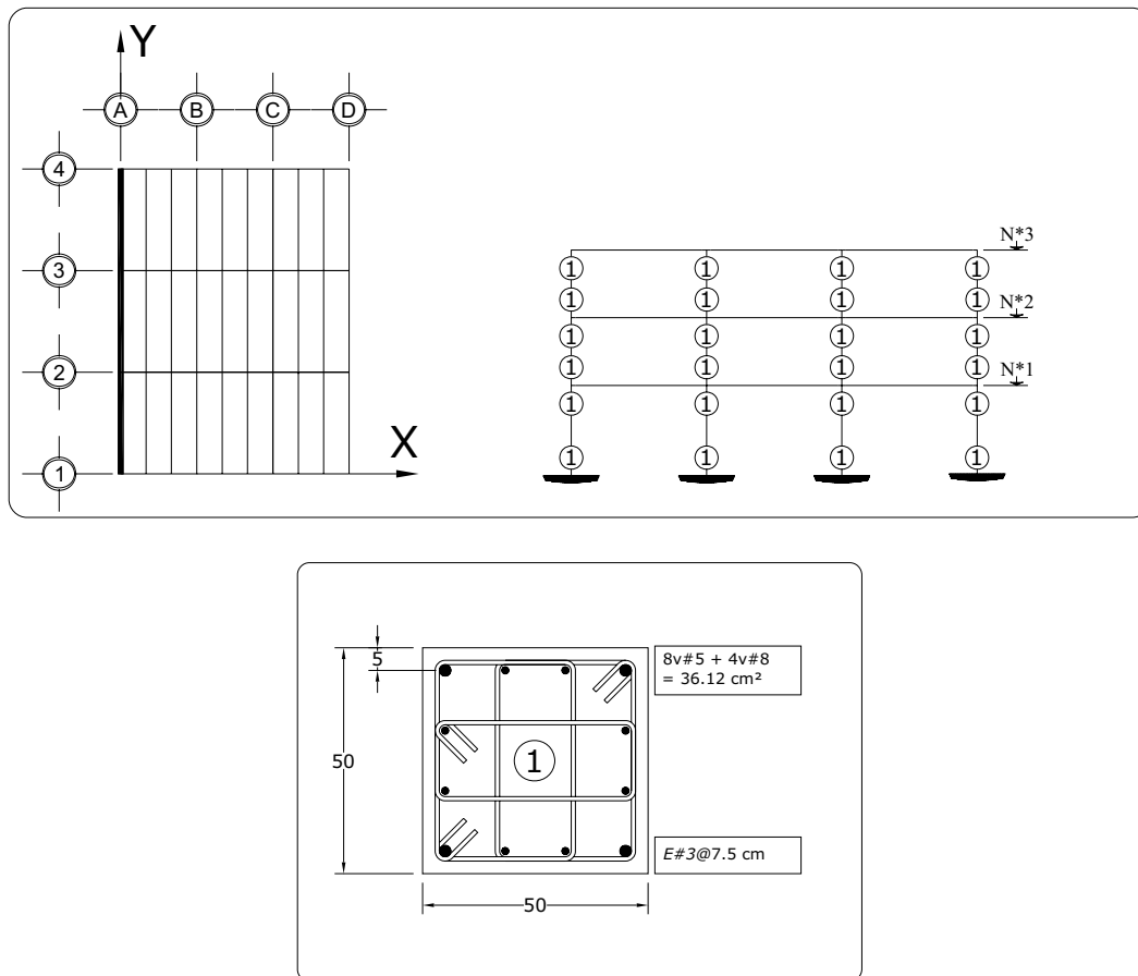
Fig 3.63 Tipos de armados de refuerzo longitudinal y transversal resultantes en los extremos de las columnas del eje A, caso B1 ( Q = 4 )
