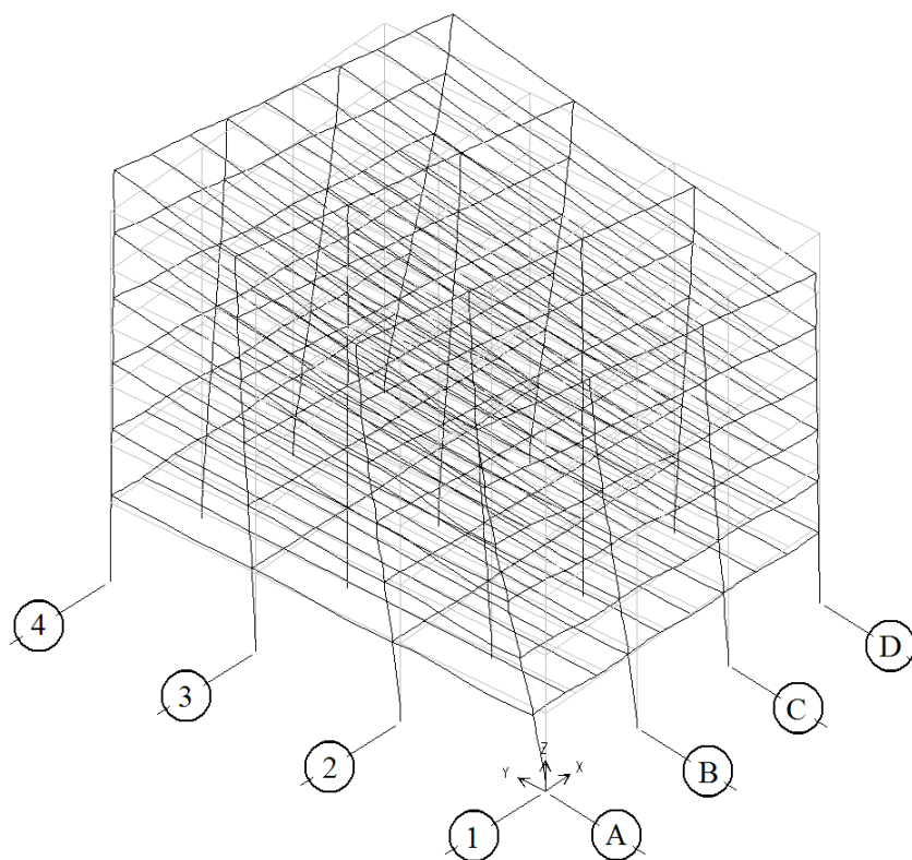
Fig 3.15 Deformada en perspectiva del primer modo de vibración en torsión, edificio de 6 niveles
