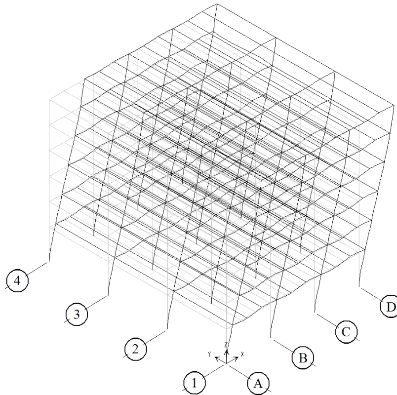
Fig 3.13 Deformada en perspectiva del primer modo de vibración, dirección corta, edificio de 6 niveles
