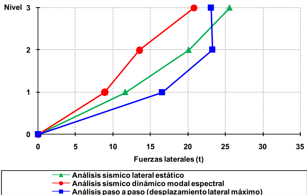
Fig 4.140 Distribución del perfil de fuerzas laterales debidas a diferentes condiciones de análisis sísmico del eje A, caso A2, (sin sobre-resistencias), diseño según el Apéndice A de las NTC-Sismo del RDF-04, edificio de 3 niveles
