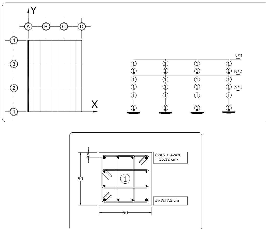
Fig 3.83 Tipos de armados de refuerzo longitudinal y transversal resultantes en los extremos de las columnas del eje A, caso B2 ( Q = 4 )
