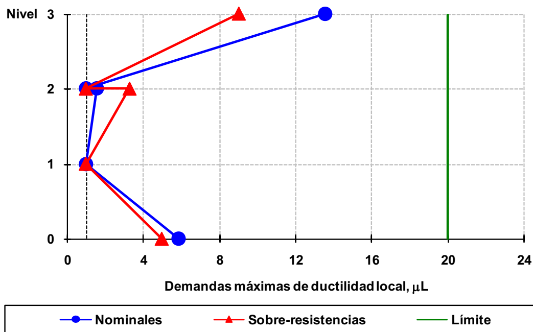
Fig 4.178 Demandas máximas de ductilidad local desarrolladas en columnas del eje 2, caso A2, análisis Push-over (sin y con sobre-resistencias), perfil de cargas laterales del análisis dinámico modal espectral, diseño Apéndice A, NTC-Sismo del RDF-04, edificio de 3 niveles
