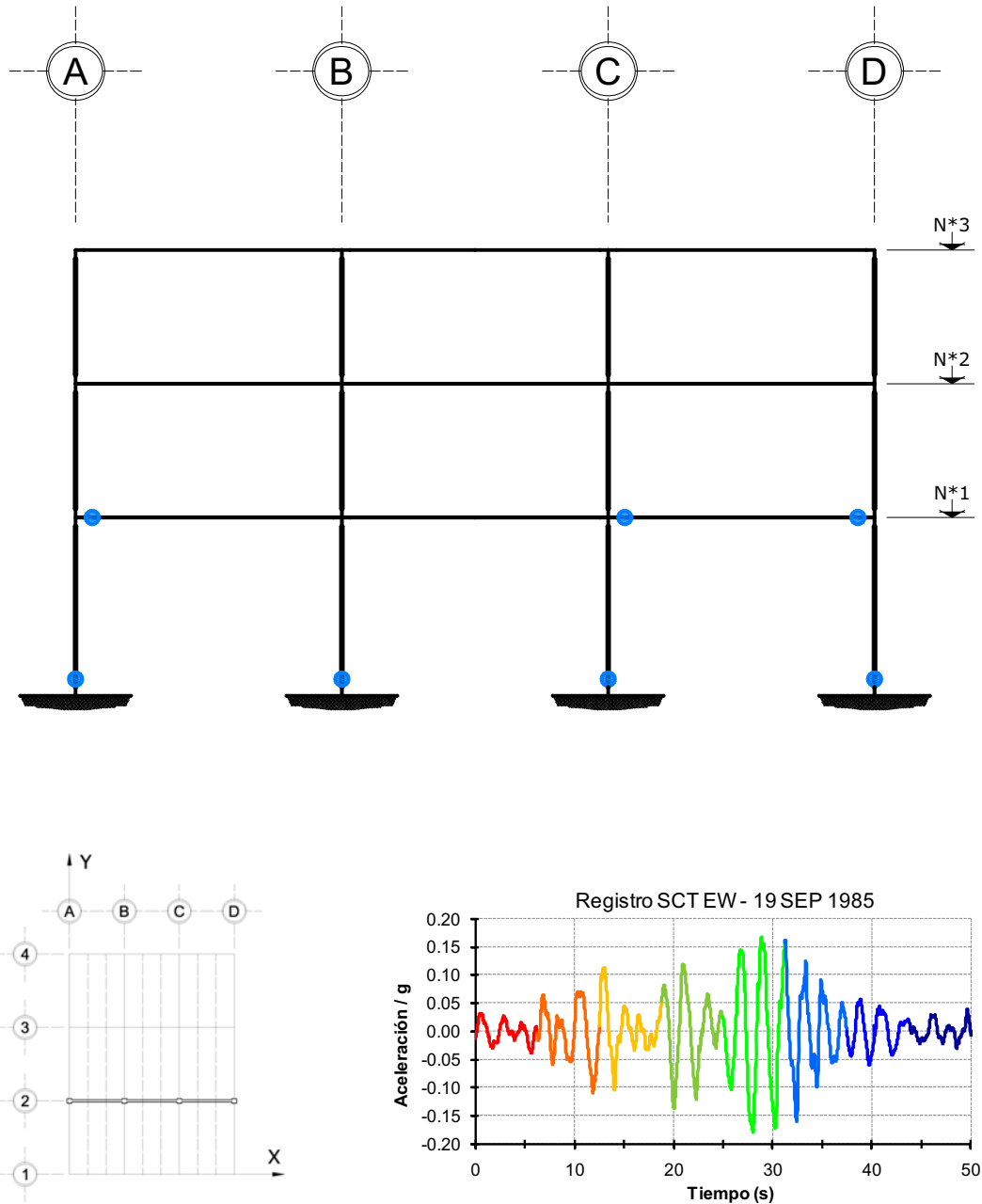
Fig 4.127 Ubicación y secuencia de formación de articulaciones plásticas, análisis paso a paso, con sobre-resistencias, edificio de 3 niveles, eje 2, caso B2
