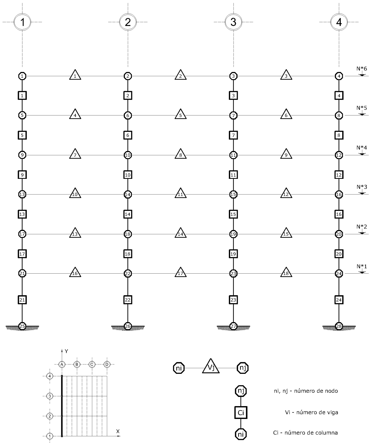
Fig 4.5 Numeración de nudos y barras en el modelo matemático bidimensional para el análisis paso a paso y el análisis tipo push-over, edificios de 6 niveles, eje A (dirección larga), casos C1 y C2 ( Q=2 ), D1 y D2 ( Q=4 )
