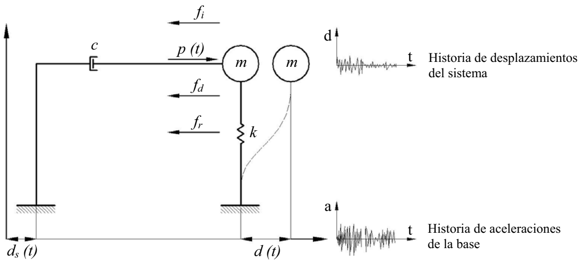
Fig 2.3 Sistema de un grado de libertad en equilibrio dinámico
