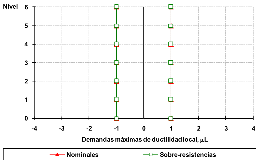
Fig 4.118 Demandas máximas de ductilidad local desarrolladas en columnas del eje 2, caso C2, análisis paso a paso elástico e inelástico (sin y con sobre-resistencias), NTC-Sismo del RDF-04, edificio de 6 niveles
