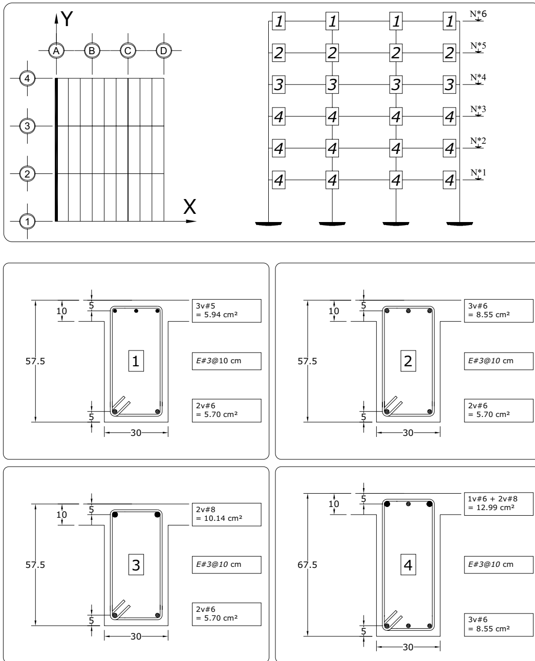
Fig 3.102 Tipos de armados de refuerzo longitudinal y transversal resultantes en los extremos de las vigas del eje A, caso D1 (Q = 4)
