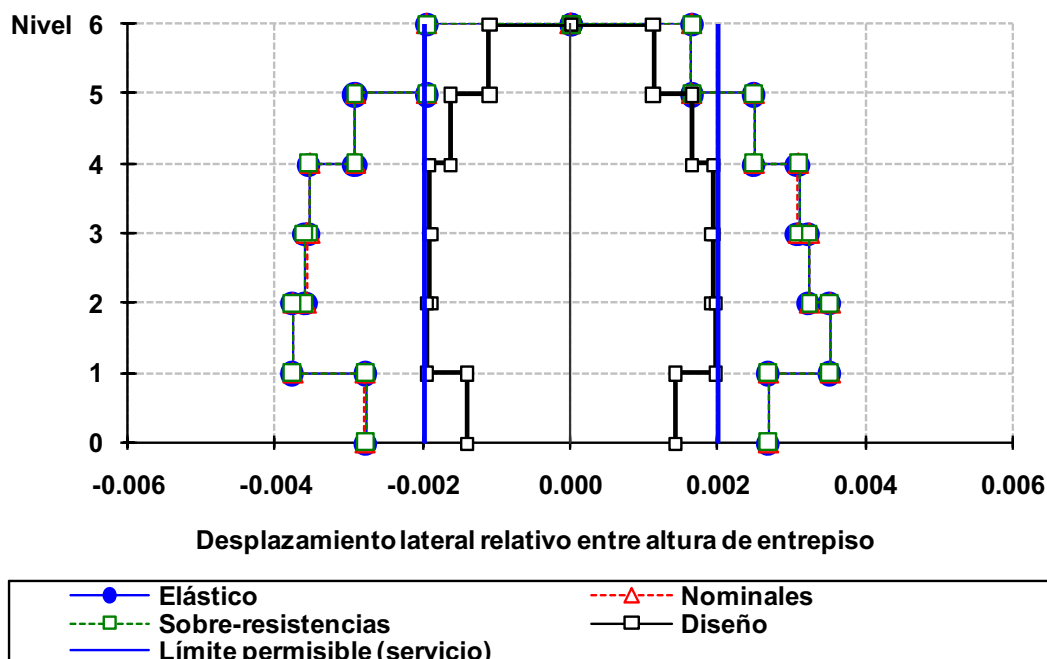
Fig 4.31 Relaciones desplazamiento lateral relativo entre altura de entrepiso del eje A, caso C2, análisis paso a paso elástico e inelástico (sin y con sobre-resistencias) y modal espectral, NTC-Sismo del RDF-04, edificio de 6 niveles
