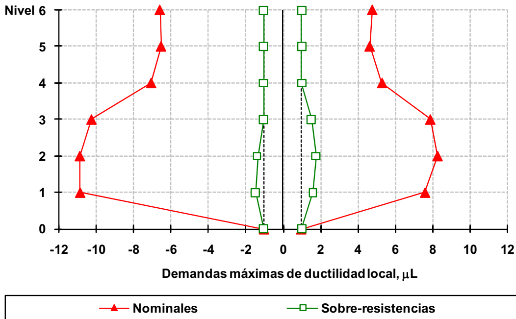
Fig 4.97 Demandas máximas de ductilidad local desarrolladas en vigas del eje A, caso D2, análisis paso a paso elástico e inelástico (sin y con sobre-resistencias), NTC-Sismo del RDF-04, edificio de 6 niveles
