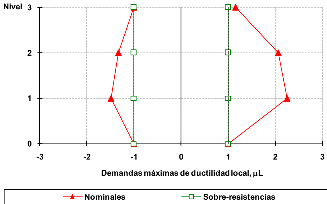
Fig 4.90 Demandas máximas de ductilidad local desarrolladas en vigas del eje 2, caso A2, análisis paso a paso elástico e inelástico (sin y con sobre-resistencias), NTC-Sismo del RDF-04, edificio de 3 niveles
