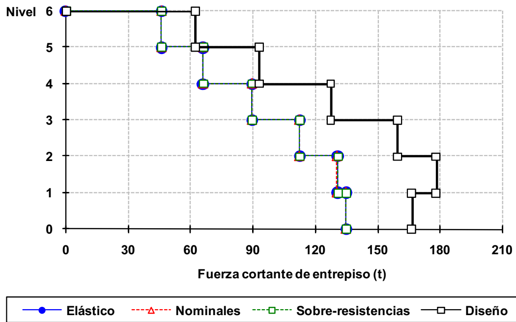
Fig 4.38 Envolventes de fuerzas cortantes de entrepiso del eje 2, caso C2, análisis paso a paso elástico e inelástico (sin y con sobre-resistencias) y modal espectral, NTC-Sismo del RDF-04, edificio de 6 niveles
