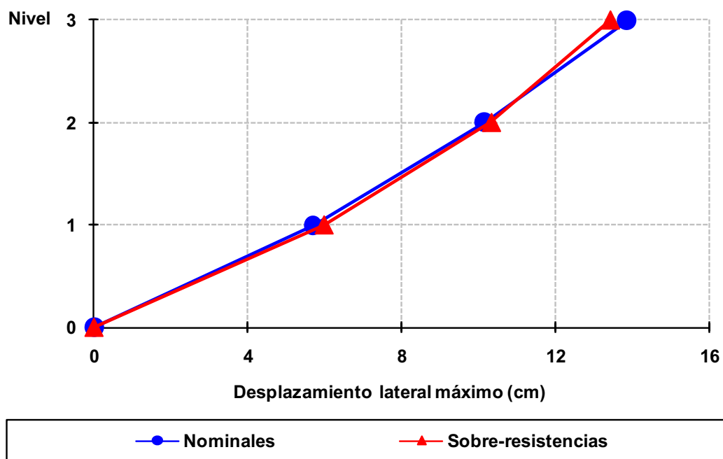
Fig 4.154 Desplazamientos laterales máximos del eje 2, caso A2, análisis Push-over (sin y con sobre-resistencias), perfil de cargas laterales del análisis dinámico modal espectral, diseño Apéndice A, NTC-Sismo del RDF-04, edificio de 3 niveles
