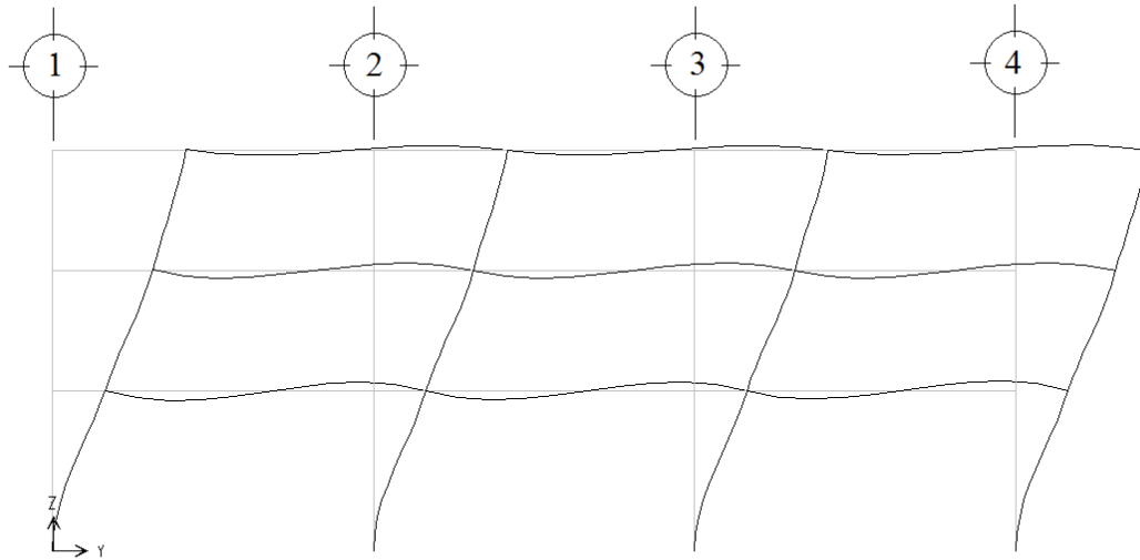
Fig 3.4 Deformada en elevación del primer modo de vibración, dirección larga, edificio de 3 niveles
