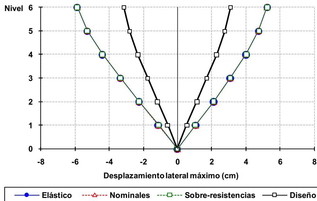
Fig 4.15 Desplazamientos horizontales máximos del eje A, caso C2, análisis paso a paso dinámico (elástico e inelástico) y modal espectral, sin y con efectos de sobre-resistencias, diseño Apéndice A, NTC-Sismo del RDF-04, edificio de 6 niveles
