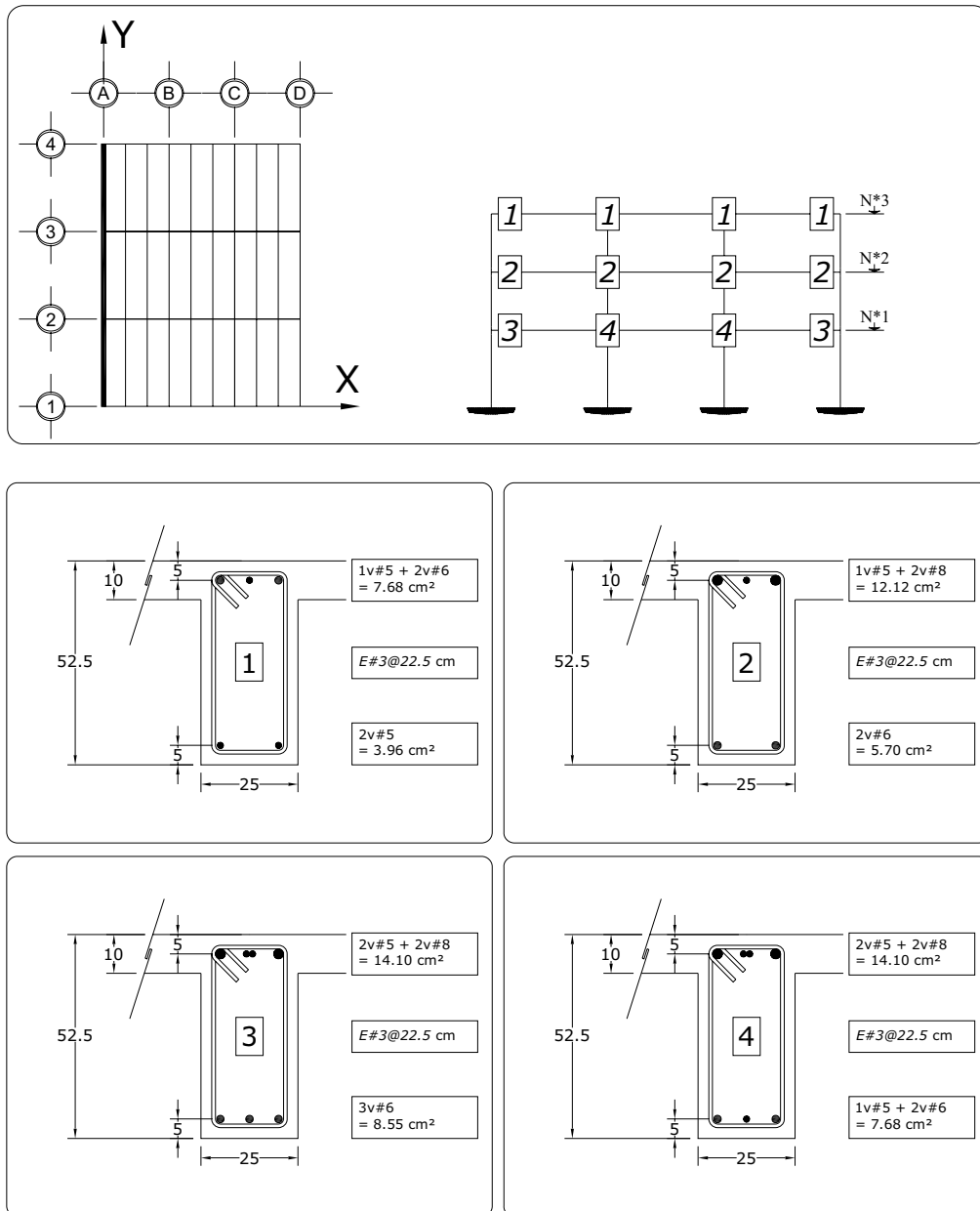
Fig 3.58 Tipos de armados de refuerzo longitudinal y transversal resultantes en los extremos de las vigas del eje A, caso A1 (Q = 2)
