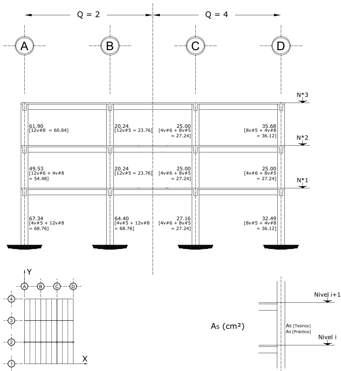
Fig 3.53a Acero de refuerzo longitudinal teórico y práctico necesario en columnas, eje 2, casos A1 (Q = 2) y B1 (Q = 4)
