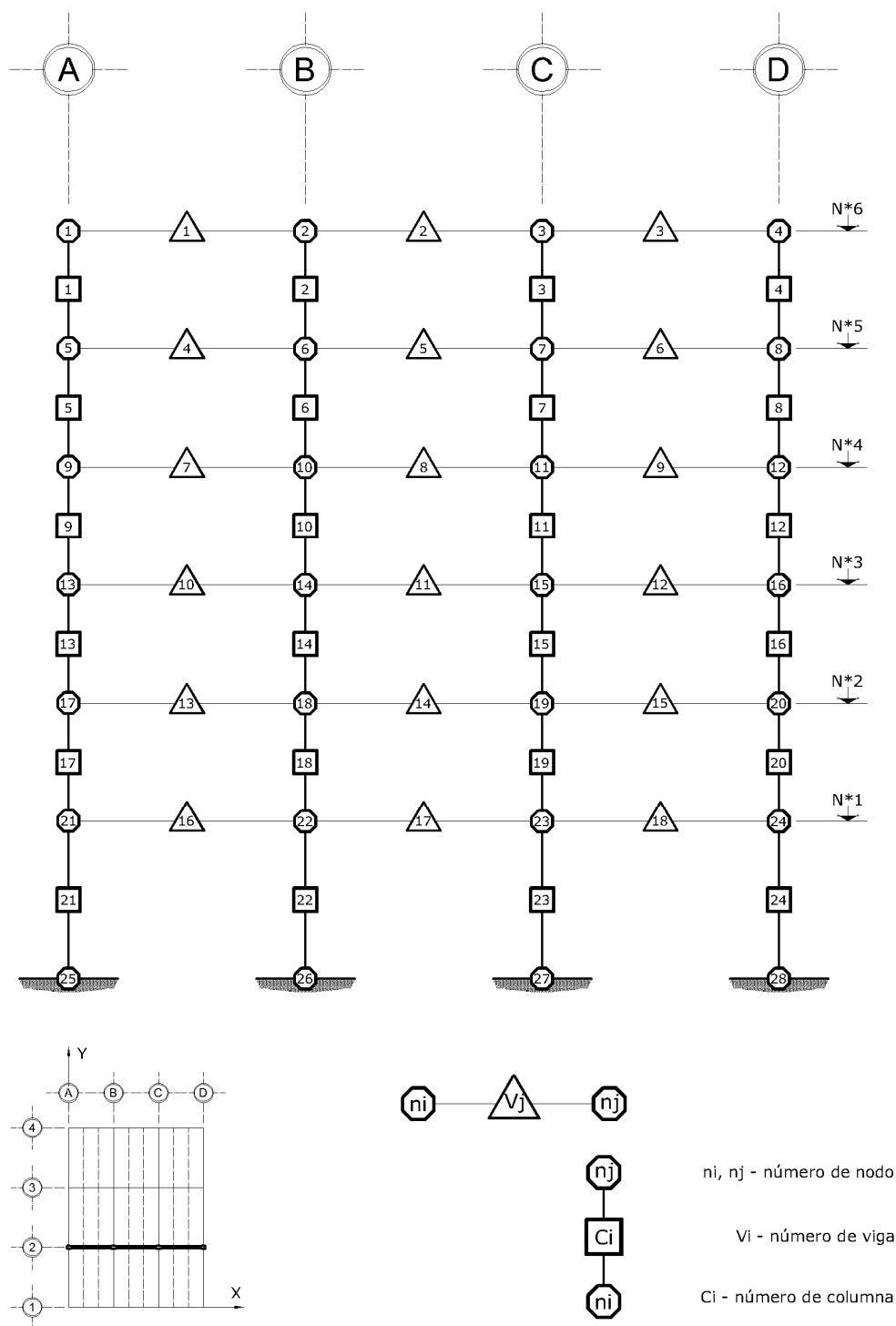
Fig 4.4 Numeración de nudos y barras en el modelo matemático bidimensional para el análisis paso a paso y el análisis tipo push-over, edificios de 6 niveles, eje 2 (dirección corta), casos C1 y C2 ( Q = 2 ), D1 y D2 ( Q = 4 )
