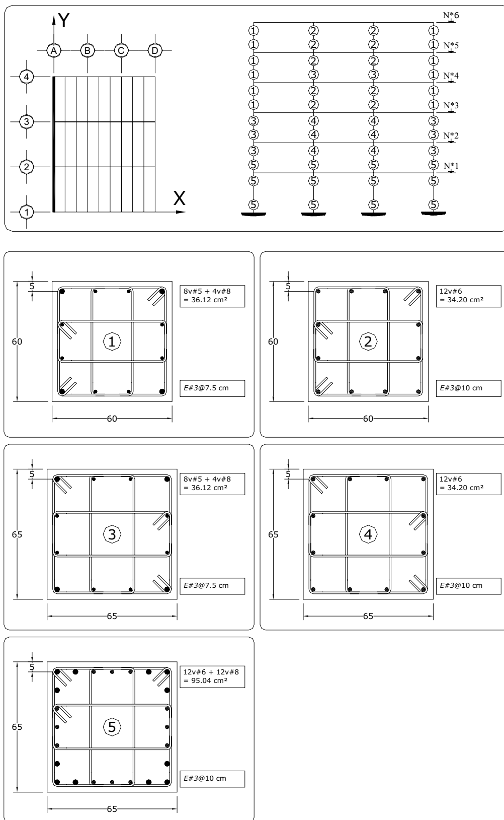
Fig 3.119 Tipos de armados de refuerzo longitudinal y transversal resultantes en los extremos de las columnas del eje A, caso C2 (Q = 2)
