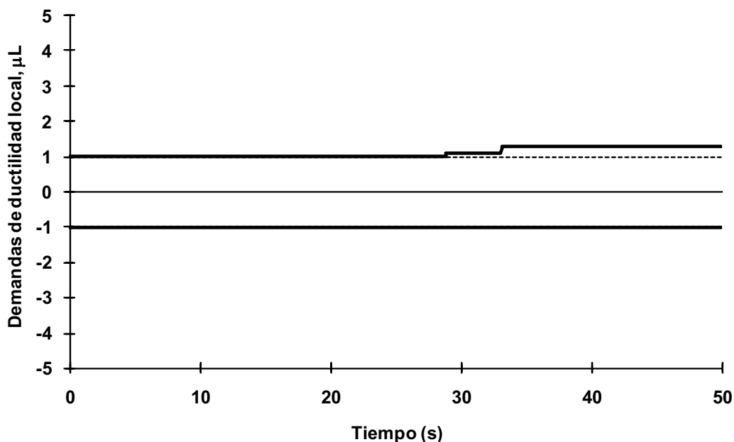
Fig 4.111 Demanda de ductilidad local desarrollada en el extremo izquierdo de la viga 16 del nivel 1, eje 2, caso D2, análisis paso a paso inelástico (con sobre-resistencias), NTC-Sismo del RDF-04, edificio de 6 niveles
