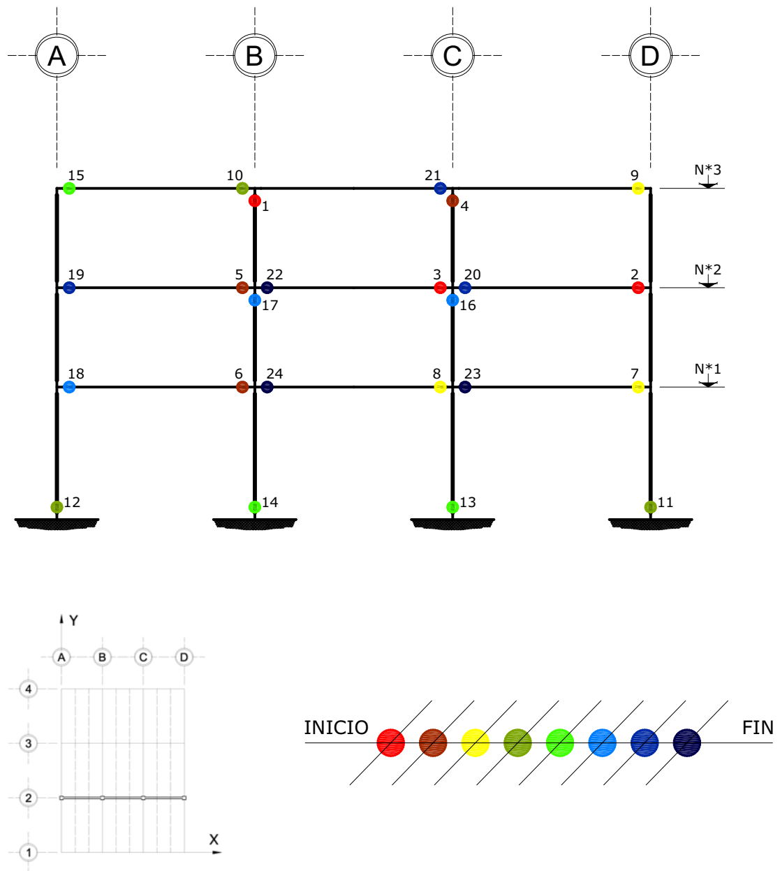
Fig 4.194 Ubicación y secuencia de formación de articulaciones plásticas, análisis Push-over, resistencias nominales, edificio de 3 niveles, eje 2, caso A2
