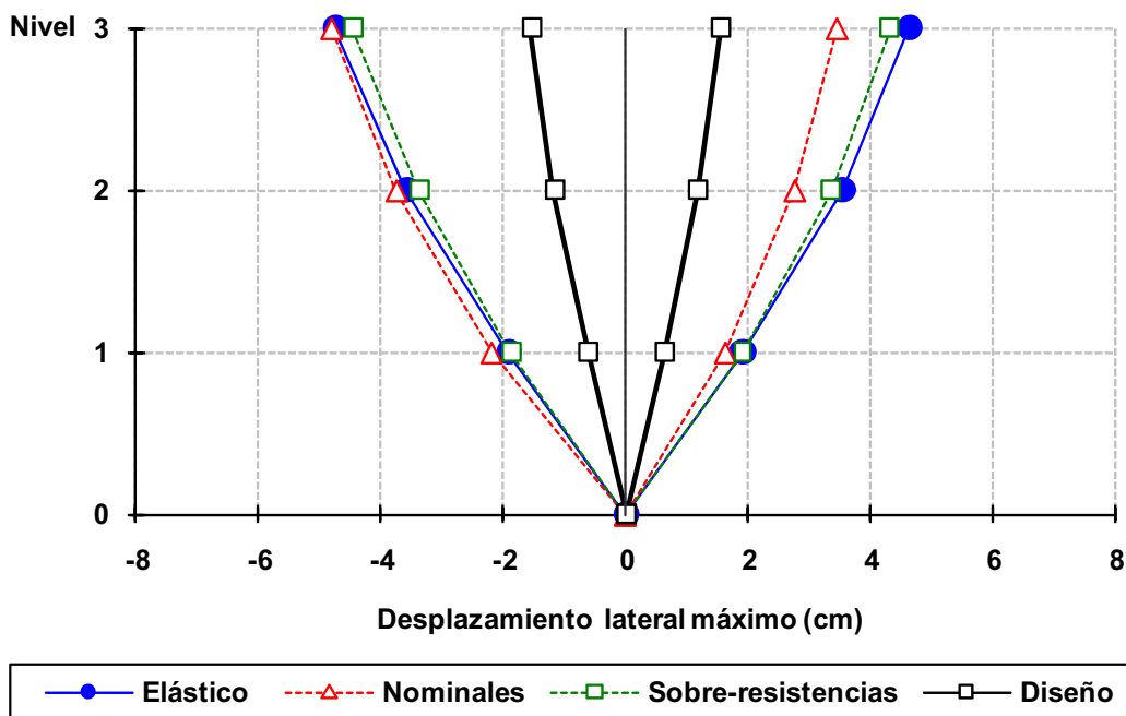
Fig 4.12 Desplazamientos horizontales máximos del eje 2, caso B2, análisis paso a paso dinámico (elástico e inelástico) y modal espectral, sin y con efectos de sobre-resistencias, diseño Apéndice A, NTC-Sismo del RDF-04, edificio de 3 niveles
