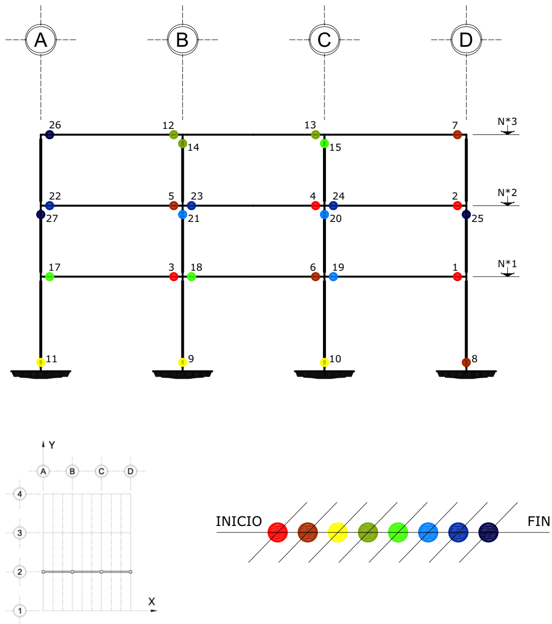
Fig 4.198 Ubicación y secuencia de formación de articulaciones plásticas, análisis Push-over, resistencias nominales, edificio de 3 niveles, eje 2, caso B2
