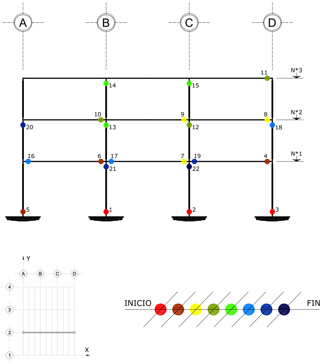
Fig 4.199 Ubicación y secuencia de formación de articulaciones plásticas, análisis Push-over, con sobre-resistencias, edificio de 3 niveles, eje 2, caso B2
