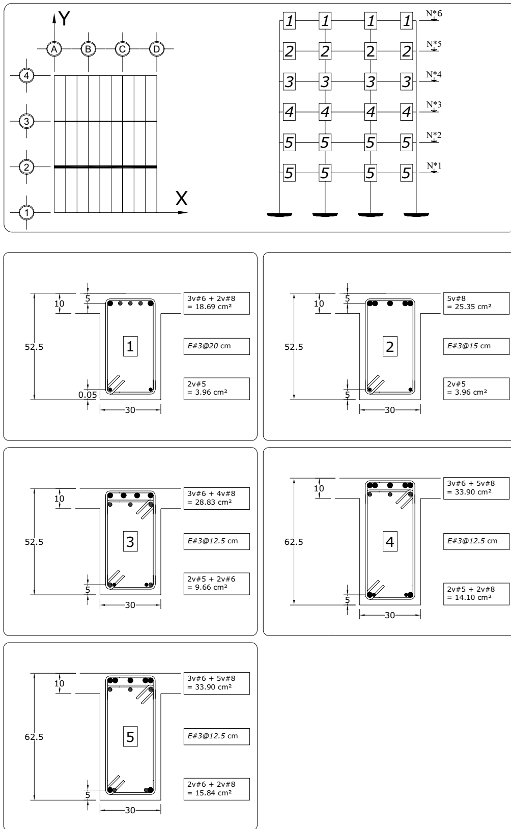
Fig 3.96 Tipos de armados de refuerzo longitudinal y transversal resultantes en los extremos de las vigas del eje 2, caso C1 (Q = 2)
