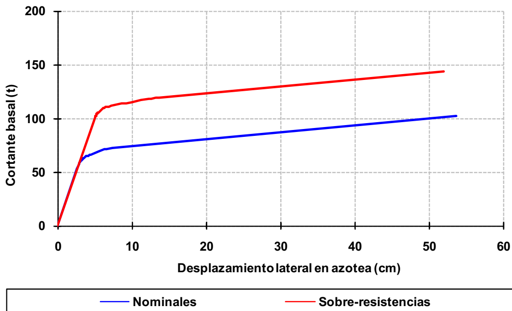
Fig 4.193 Relaciones fuerza cortante basal - desplazamiento horizontal en azotea, eje A, caso D2, análisis Push-over (sin y con sobre-resistencias), perfil de cargas laterales del análisis dinámico modal espectral, diseño Apéndice A, NTC-Sismo del RDF-04, edificio de 6 niveles
