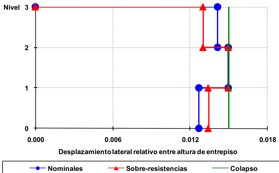
Fig 4.163 Relaciones desplazamiento lateral relativo entre altura de entrepiso del eje A, caso A2, análisis Push-over (sin y con sobre-resistencias), perfil de cargas laterales del análisis dinámico modal espectral, diseño Apéndice A, NTC-Sismo del RDF-04, edificio de 3 niveles
