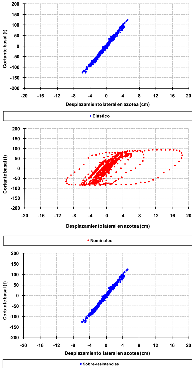
Fig 4.57 Relaciones fuerza cortante basal - desplazamiento horizontal en azotea, eje A, caso D2, análisis paso a paso elástico e inelástico (sin y con sobre-resistencias), diseño Apéndice A, NTC-Sismo del RDF-04, edificio de 6 niveles
