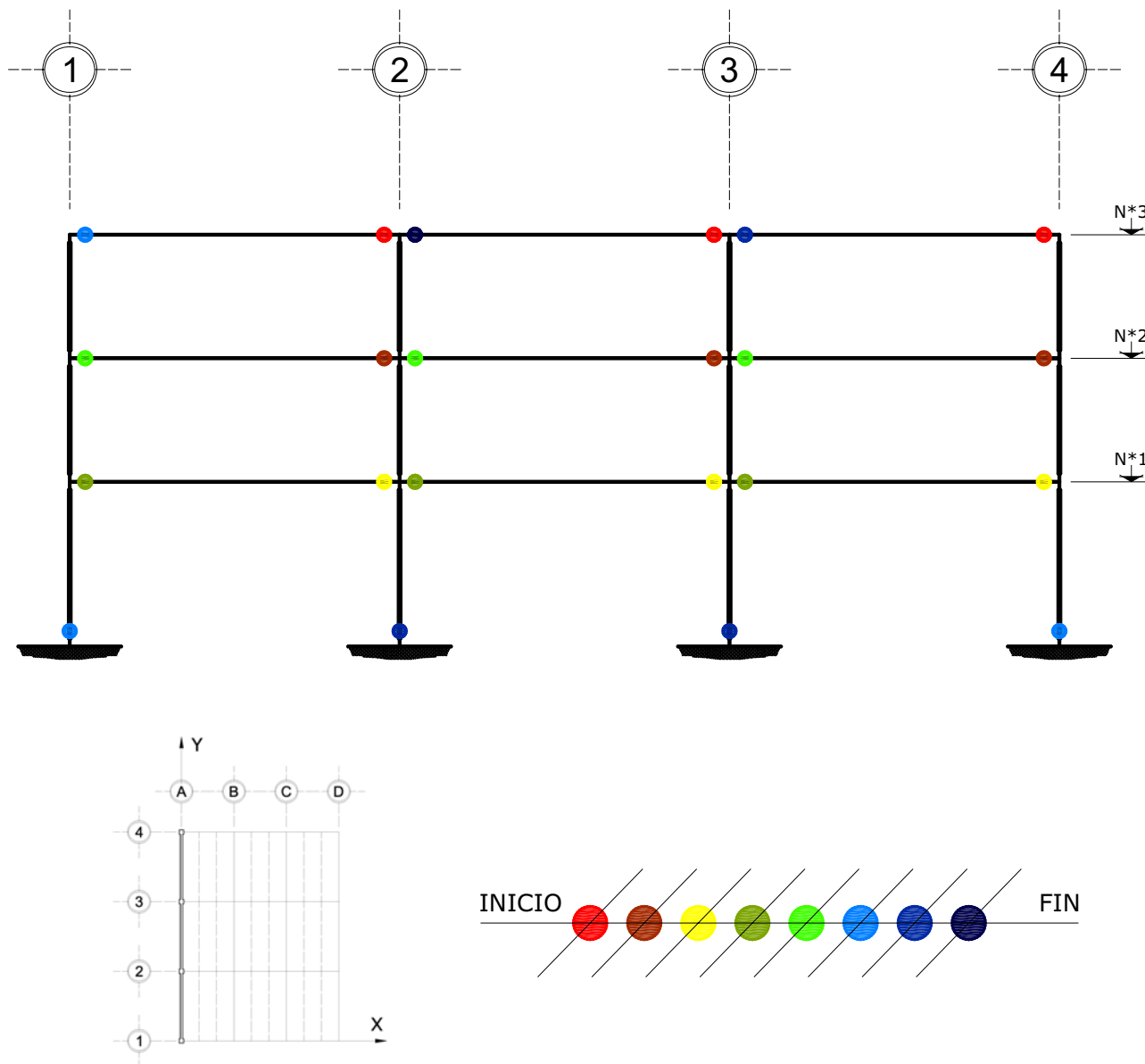
Fig 4.200 Ubicación y secuencia de formación de articulaciones plásticas, análisis Push-over, resistencias nominales, edificio de 3 niveles, eje A, caso B2
