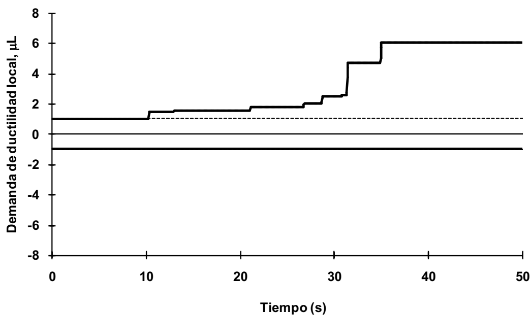
Fig 4.102 Demanda de ductilidad local desarrollada en el extremo izquierdo de la viga 7 del nivel 1, eje 2, caso B2, análisis paso a paso inelástico (sin sobre-resistencias), NTC-Sismo del RDF-04, edificio de 3 niveles
