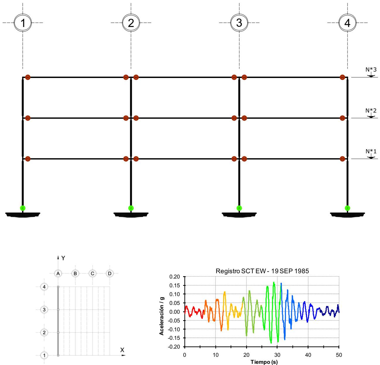
Fig 4.128 Ubicación y secuencia de formación de articulaciones plásticas, análisis paso a paso, resistencias nominales, edificio de 3 niveles, eje A, caso B2
