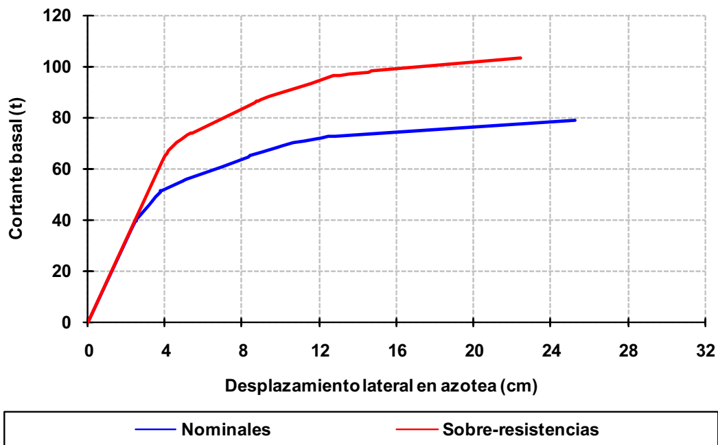
Fig 4.188 Relaciones fuerza cortante basal - desplazamiento horizontal en azotea, eje 2, caso B2, análisis Push-over (sin y con sobre-resistencias), perfil de cargas laterales del análisis dinámico modal espectral, diseño Apéndice A, NTC-Sismo del RDF-04, edificio de 3 niveles
