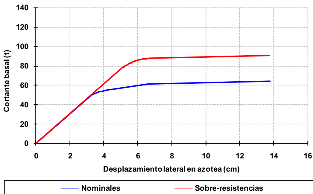
Fig 4.187 Relaciones fuerza cortante basal - desplazamiento horizontal en azotea, eje A, caso A2, análisis Push-over (sin y con sobre-resistencias), perfil de cargas laterales del análisis dinámico modal espectral, diseño Apéndice A, NTC-Sismo del RDF-04, edificio de 3 niveles
