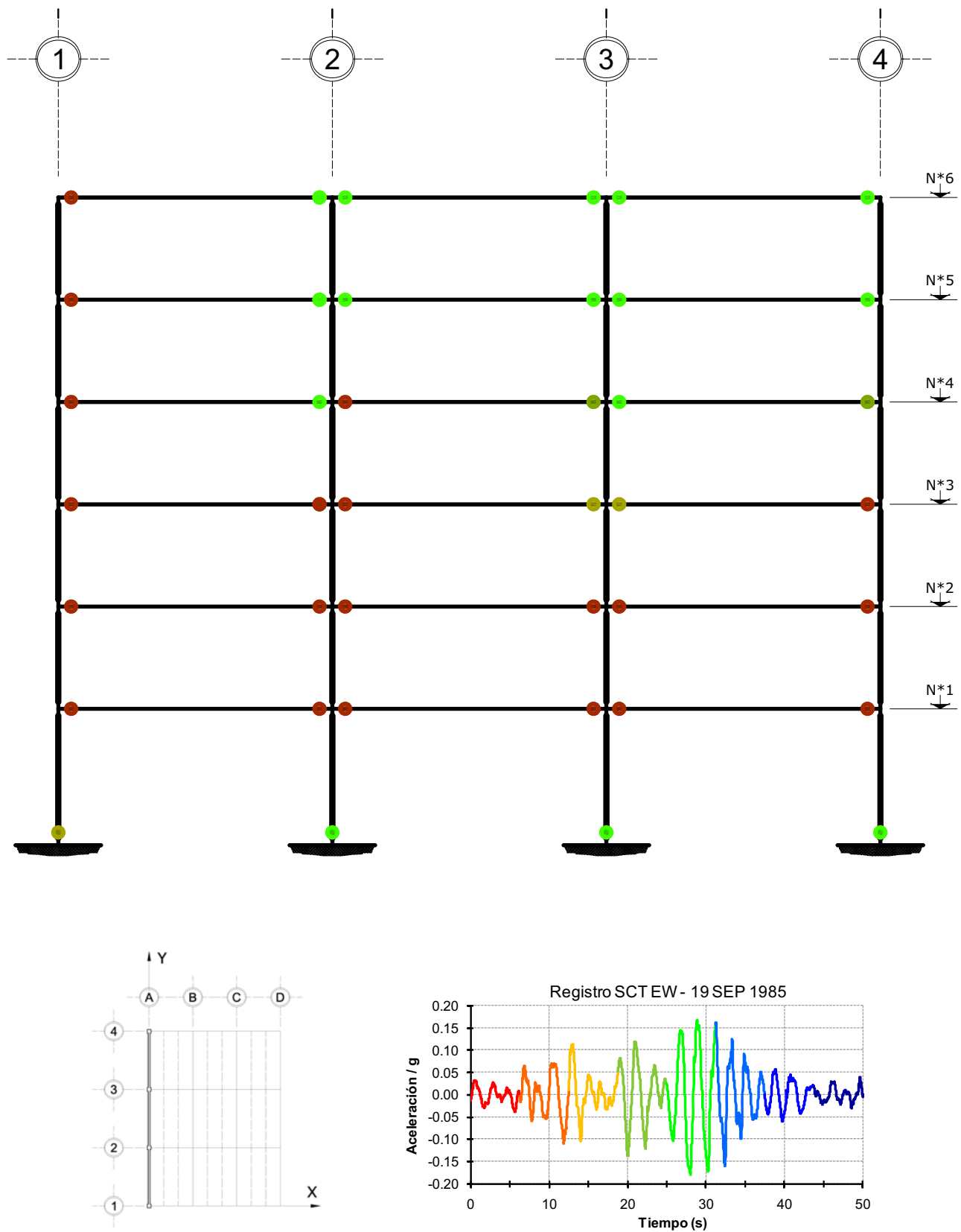
Fig 4.136 Ubicación y secuencia de formación de articulaciones plásticas, análisis paso a paso, resistencias nominales, edificio de 6 niveles, eje A, caso D2
