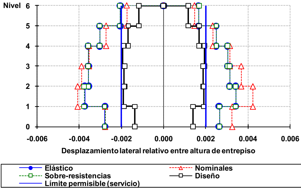
Fig 4.32 Relaciones desplazamiento lateral relativo entre altura de entrepiso del eje 2, caso D2, análisis paso a paso elástico e inelástico (sin y con sobre-resistencias) y modal espectral, NTC-Sismo del RDF-04, edificio de 6 niveles
