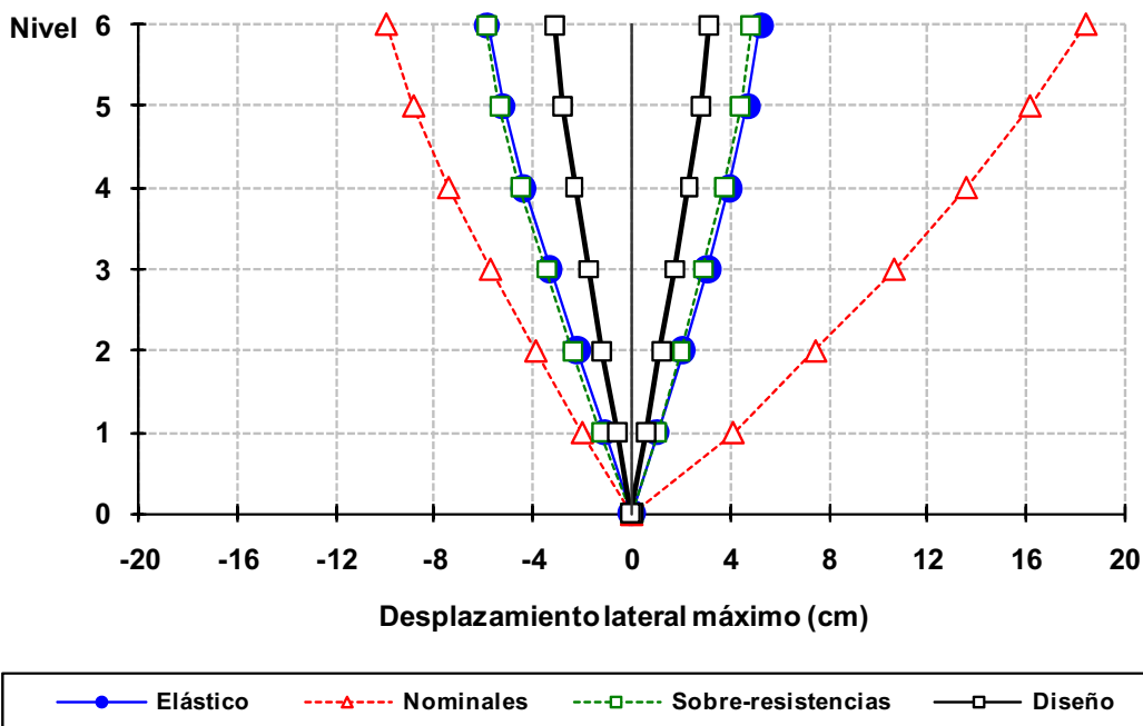
Fig 4.17 Desplazamientos horizontales máximos del eje A, caso D2, análisis paso a paso dinámico (elástico e inelástico) y modal espectral, sin y con efectos de sobre-resistencias, diseño Apéndice A, NTC-Sismo del RDF-04, edificio de 6 niveles
