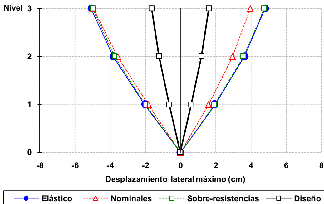
Fig 4.11 Desplazamientos horizontales máximos del eje A, caso A2, análisis paso a paso dinámico (elástico e inelástico) y modal espectral, sin y con efectos de sobre-resistencias, diseño Apéndice A, NTC-Sismo del RDF-04, edificio de 3 niveles
