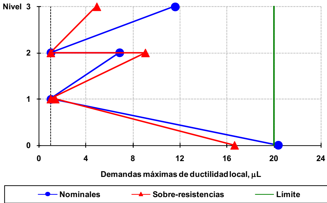
Fig 4.180 Demandas máximas de ductilidad local desarrolladas en columnas del eje 2, caso B2, análisis Push-over (sin y con sobre-resistencias), perfil de cargas laterales del análisis dinámico modal espectral, diseño Apéndice A, NTC-Sismo del RDF-04, edificio de 3 niveles
