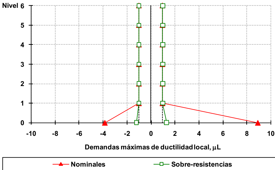
Fig 4.121 Demandas máximas de ductilidad local desarrolladas en columnas del eje A, caso D2, análisis paso a paso elástico e inelástico (sin y con sobre-resistencias), NTC-Sismo del RDF-04, edificio de 6 niveles
