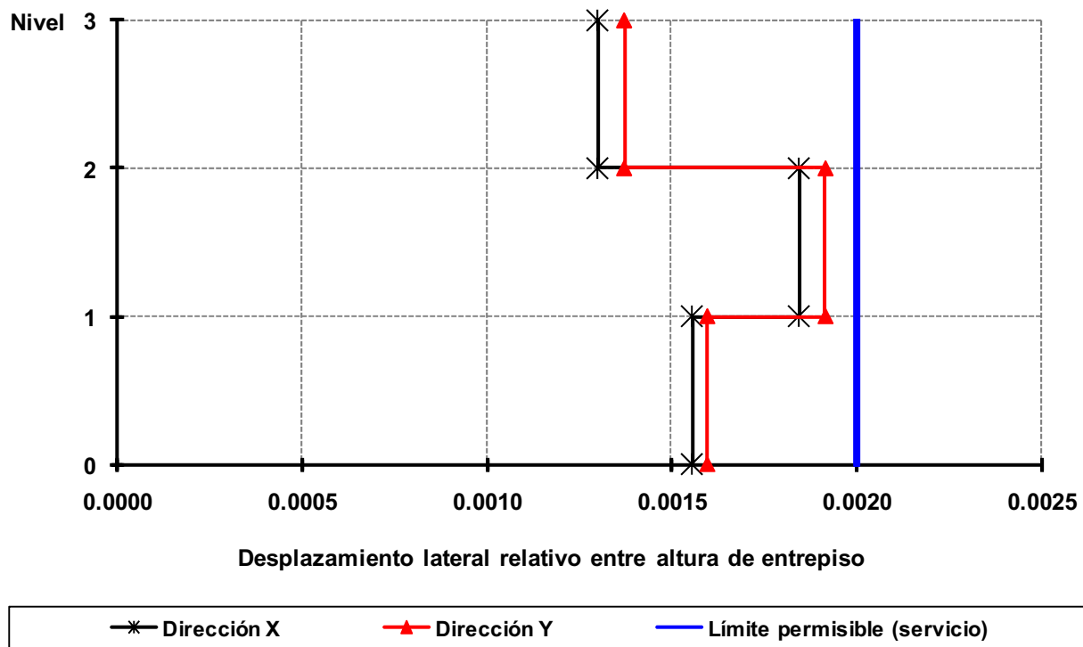
Fig 3.17a Relaciones desplazamiento lateral relativo entre altura de entrepiso (condición de servicio), análisis dinámico modal espectral, edificio de 3 niveles, caso A2 ( Q = 2 )
