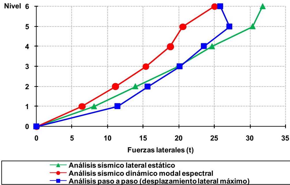
Fig 4.148 Distribución del perfil de fuerzas laterales debidas a diferentes condiciones de análisis sísmico del eje A, caso C2, (sin sobre-resistencias), diseño según el Apéndice A de las NTC-Sismo del RDF-04, edificio de 6 niveles
