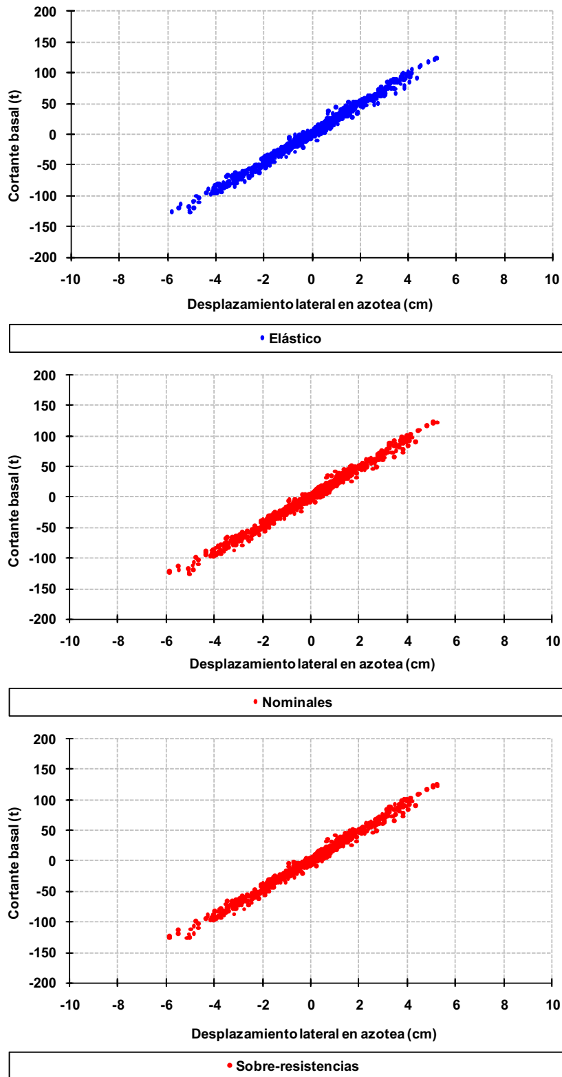
Fig 4.55 Relaciones fuerza cortante basal - desplazamiento horizontal en azotea, eje A, caso C2, análisis paso a paso elástico e inelástico (sin y con sobre-resistencias), diseño Apéndice A, NTC-Sismo del RDF-04, edificio de 6 niveles
