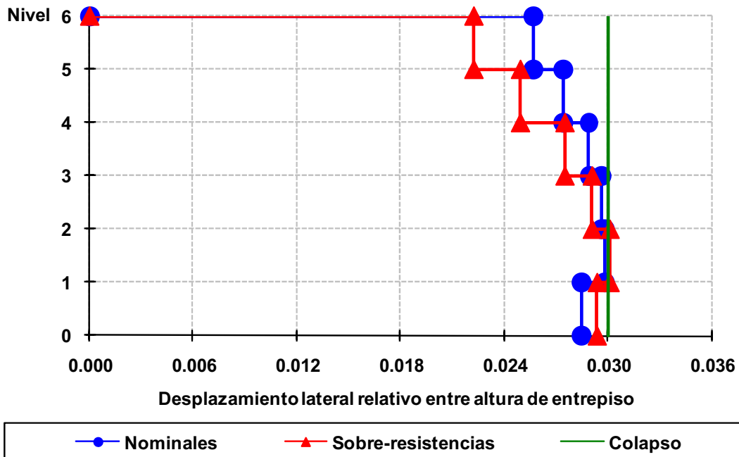
Fig 4.169 Relaciones desplazamiento lateral relativo entre altura de entrepiso del eje A, caso D2, análisis Push-over (sin y con sobre-resistencias), perfil de cargas laterales del análisis dinámico modal espectral, diseño Apéndice A, NTC-Sismo del RDF-04, edificio de 6 niveles
