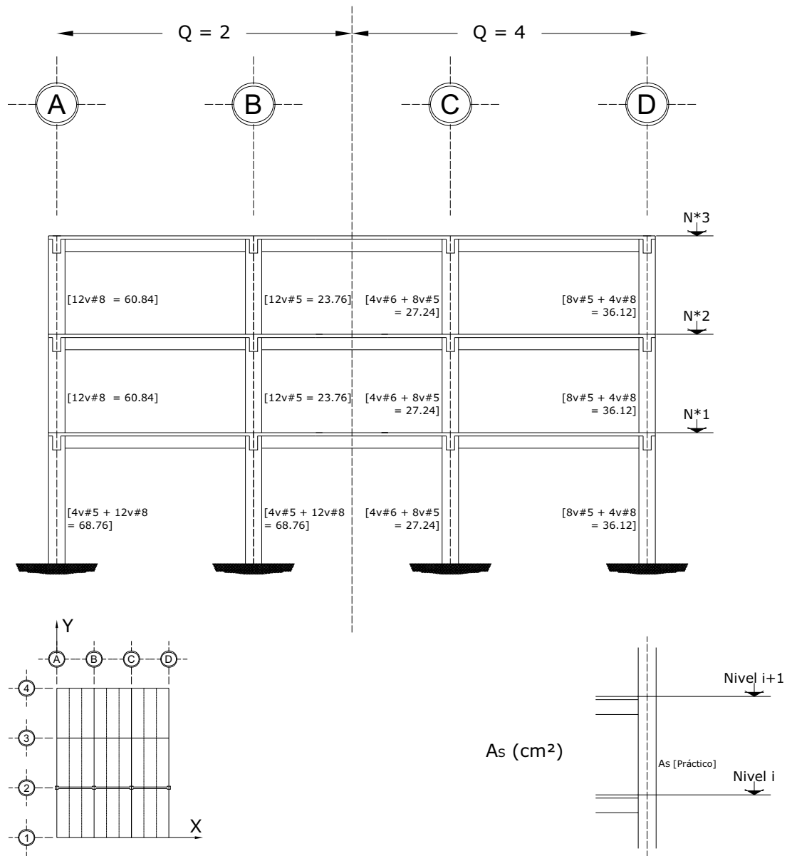
Fig 3.53b Acero de refuerzo longitudinal teórico y práctico necesario en columnas, eje 2, casos A1 (Q = 2) y B1 (Q = 4)
