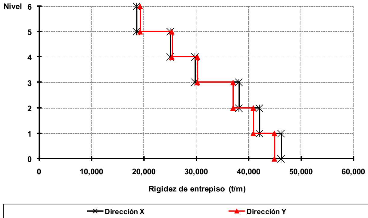
Fig 3.45 Rigideces de entrepiso, edificio 6 niveles, caso C2 (Q = 2)
