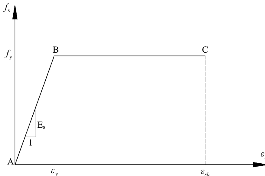
Fig 2.20 Gráfica esfuerzo-deformación EPP
