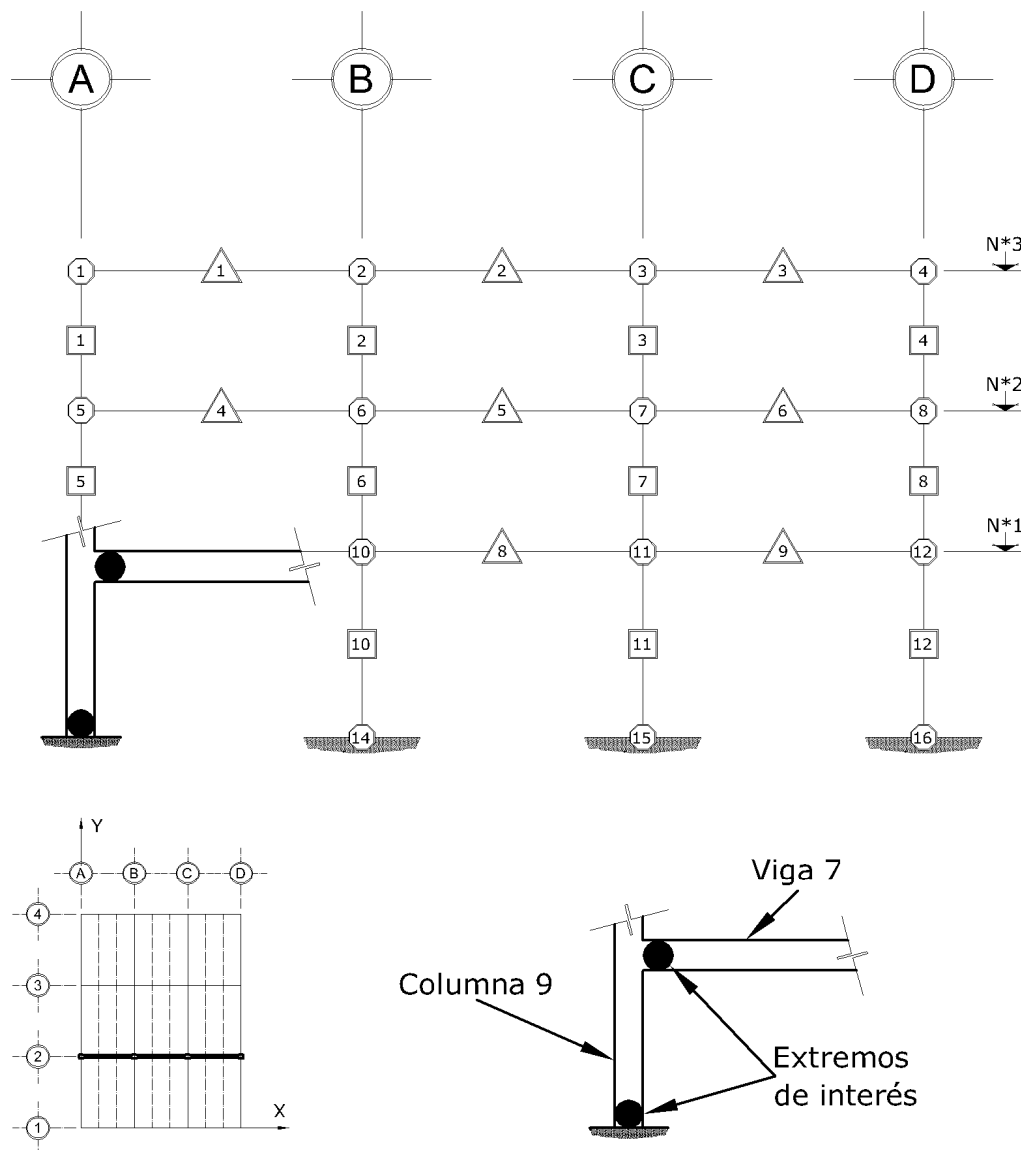
Fig 4.6 Identificación de los extremos en secciones estructurales de la viga 7 y la columna 9 para el estudio de las historias en el tiempo de las respuestas de los análisis paso a paso elásticos e inelásticos (sin y con sobre-resistencias), edificios de 3 niveles, eje 2 (dirección corta), casos A1 y A2 ( Q = 2 ), B1 y B2 ( Q = 4 )
