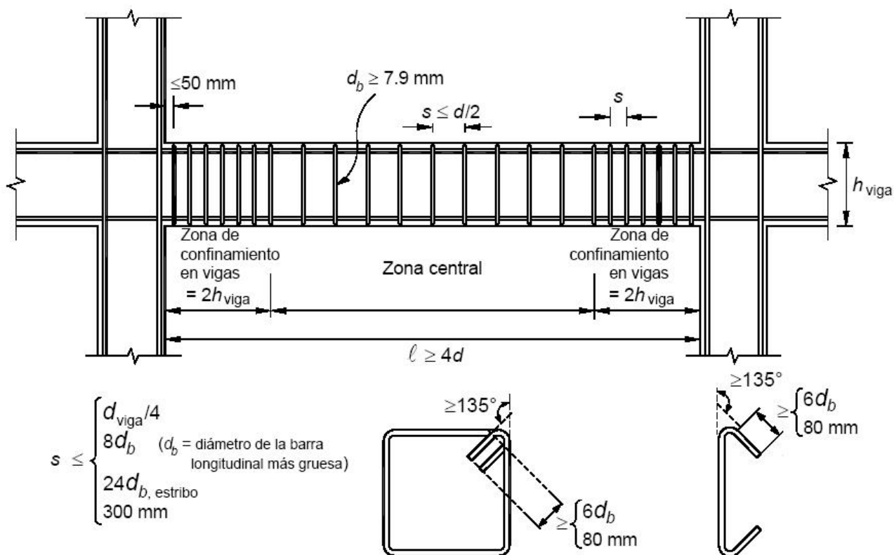
Fig 2.24 Detallado de elementos a flexión de marcos dúctiles
