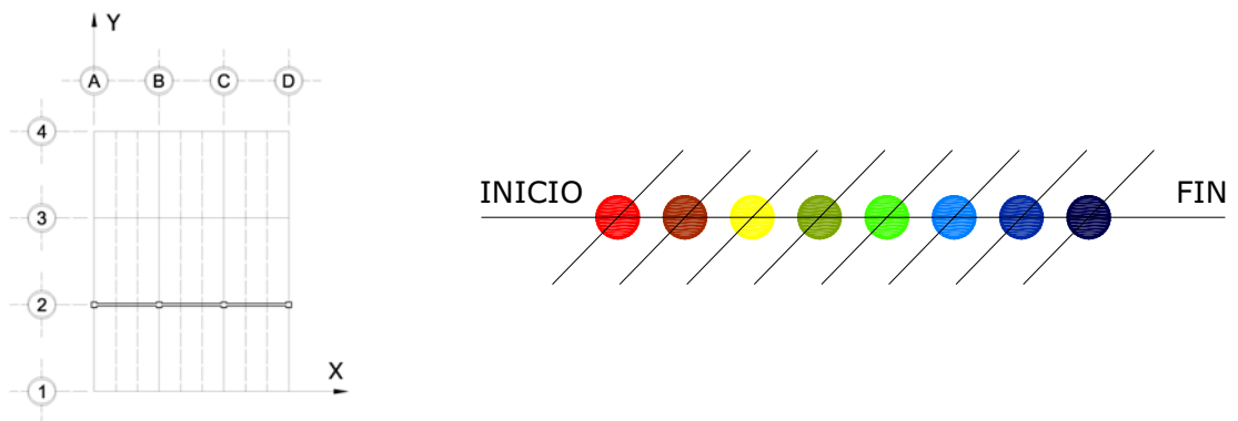
Fig 4.206 Ubicación y secuencia de formación de articulaciones plásticas, análisis Push-over, resistencias nominales, edificio de 6 niveles, eje 2, caso D2
