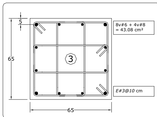
Fig 3.123 Tipos de armados de refuerzo longitudinal y transversal resultantes en los extremos de las columnas del eje A, caso D2 (Q = 4)
