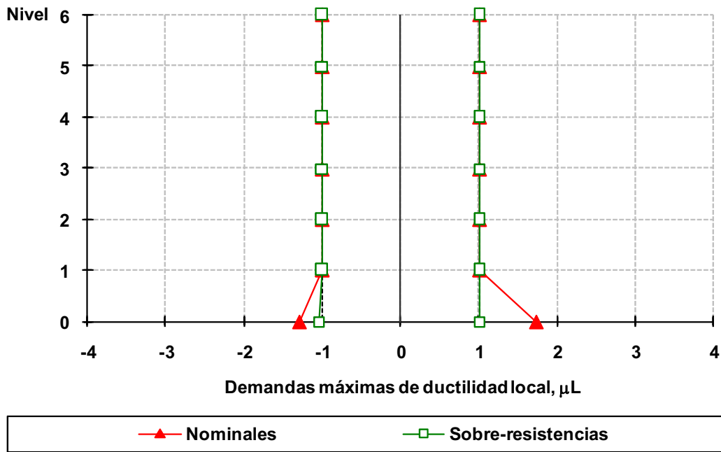
Fig 4.120 Demandas máximas de ductilidad local desarrolladas en columnas del eje 2, caso D2, análisis paso a paso elástico e inelástico (sin y con sobre-resistencias), NTC-Sismo del RDF-04, edificio de 6 niveles
