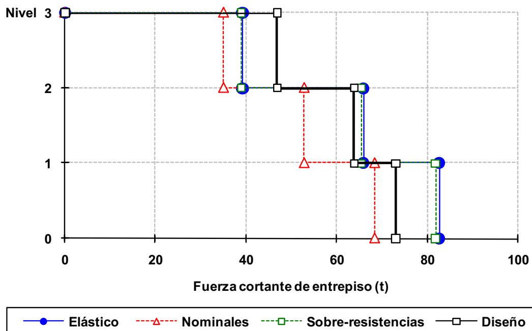
Fig 4.35 Envolventes de fuerzas cortantes de entrepiso del eje A, caso A2, análisis paso a paso elástico e inelástico (sin y con sobre-resistencias) y modal espectral, NTC-Sismo del RDF-04, edificio de 3 niveles
