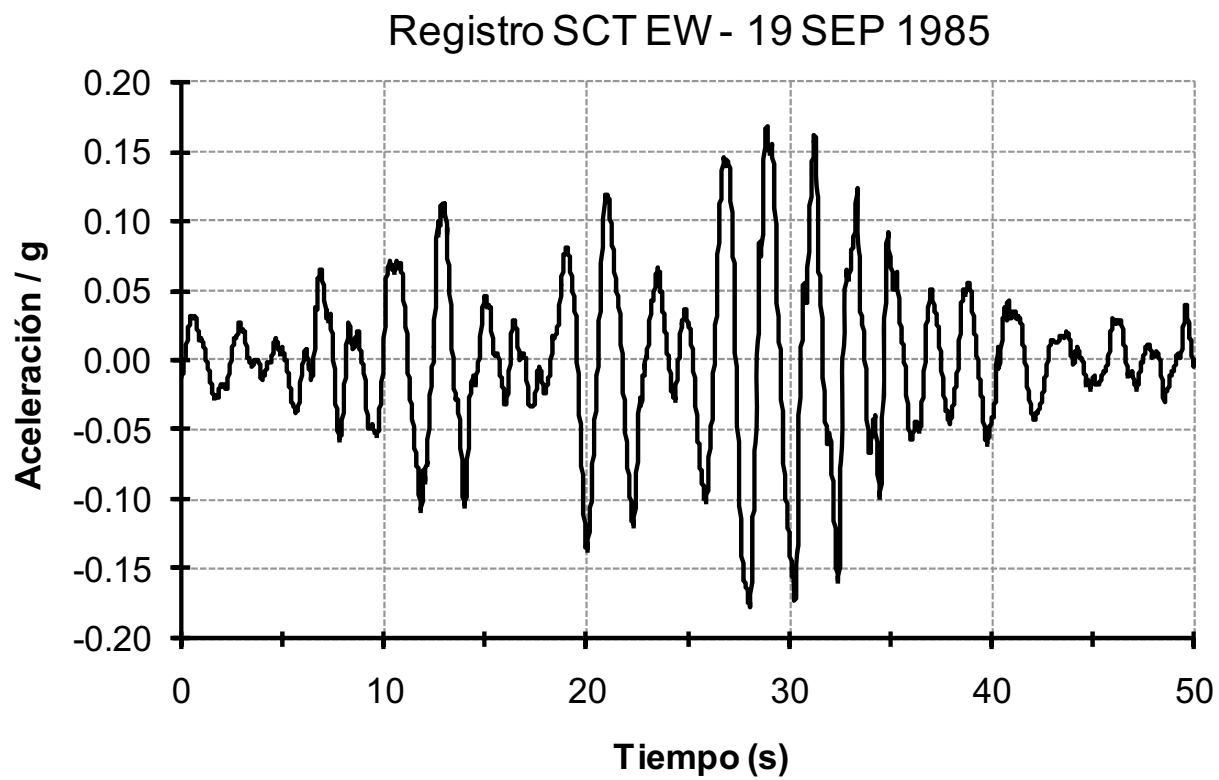
Fig 4.1 Acelerograma SCT, componente E-W, registro del sismo del 19 de septiembre de 1985
