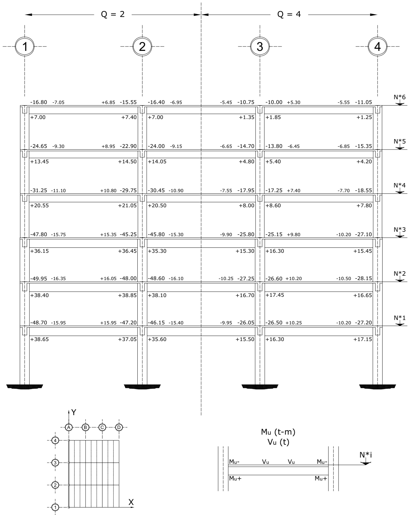
Fig 3.90 Momentos flexionantes y fuerzas cortantes últimos de vigas, eje A, casos C1 ( Q = 2 ) y D1 ( Q = 4 )
