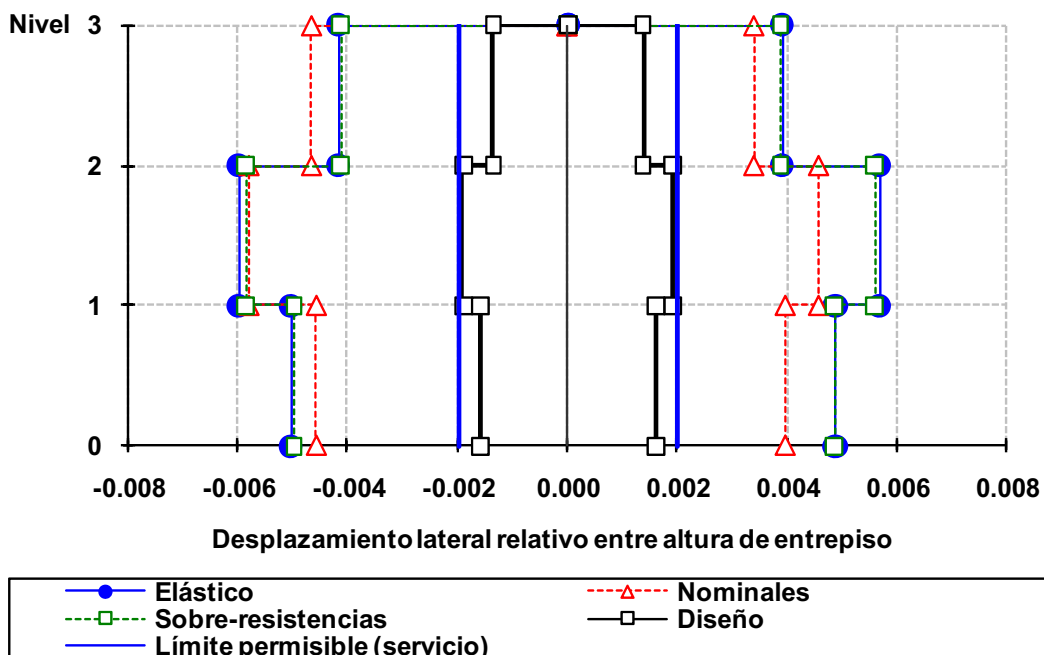
Fig 4.27 Relaciones desplazamiento lateral relativo entre altura de entrepiso del eje A, caso A2, análisis paso a paso elástico e inelástico (sin y con sobre-resistencias) y modal espectral, NTC-Sismo del RDF-04, edificio de 3 niveles
