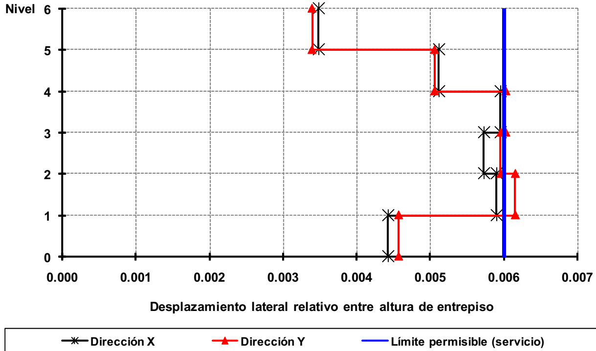
Fig 3.22 Relaciones desplazamiento lateral relativo entre altura de entrepiso (rige condición de servicio), análisis dinámico modal espectral, edificio de 6 niveles, caso D1 ( Q = 4 )
