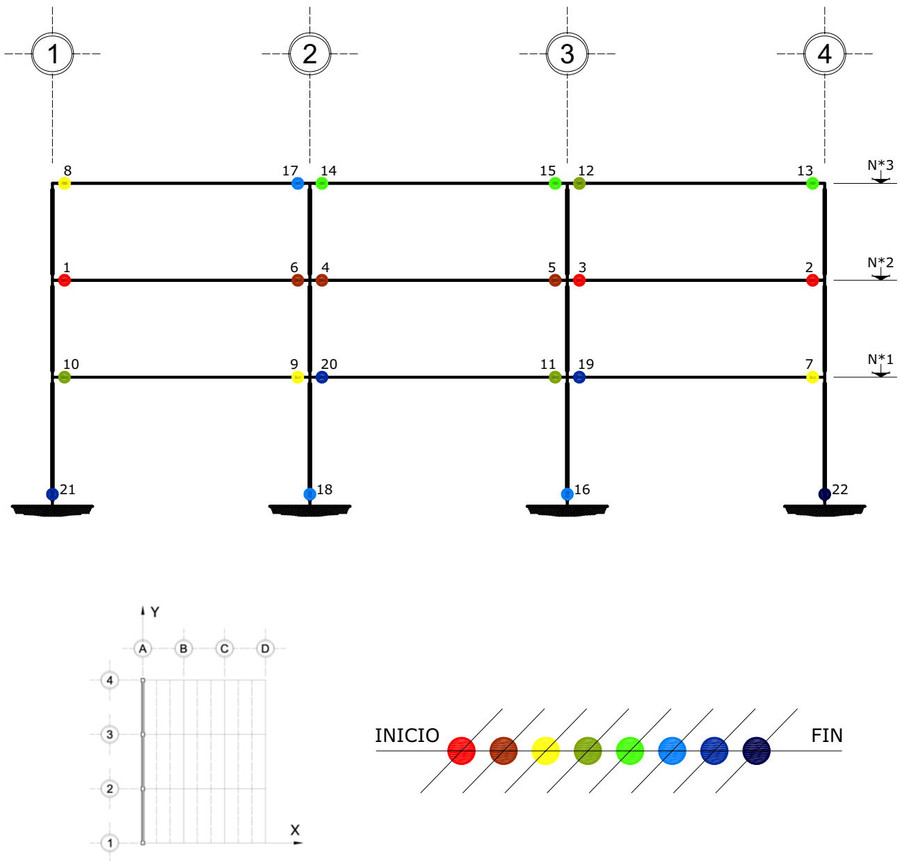
Fig 4.197 Ubicación y secuencia de formación de articulaciones plásticas, análisis Push-over, con sobre-resistencias, edificio de 3 niveles, eje A, caso A2
