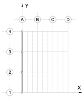
Fig 4.132 Ubicación y secuencia de formación de articulaciones plásticas, análisis paso a paso, resistencias nominales, edificio de 6 niveles, eje A, caso C2
