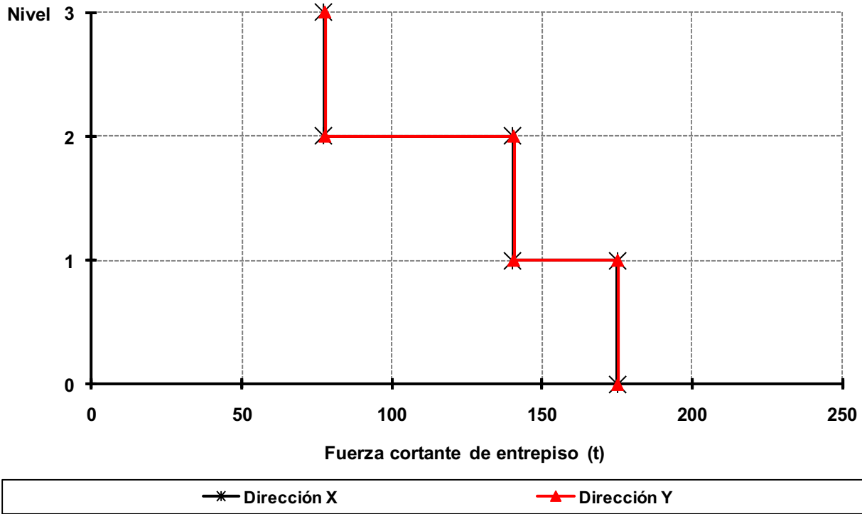
Fig 3.33 Fuerzas cortantes de entrepiso, análisis dinámico modal espectral, edificio de 3 niveles, caso A2 (Q = 2)
