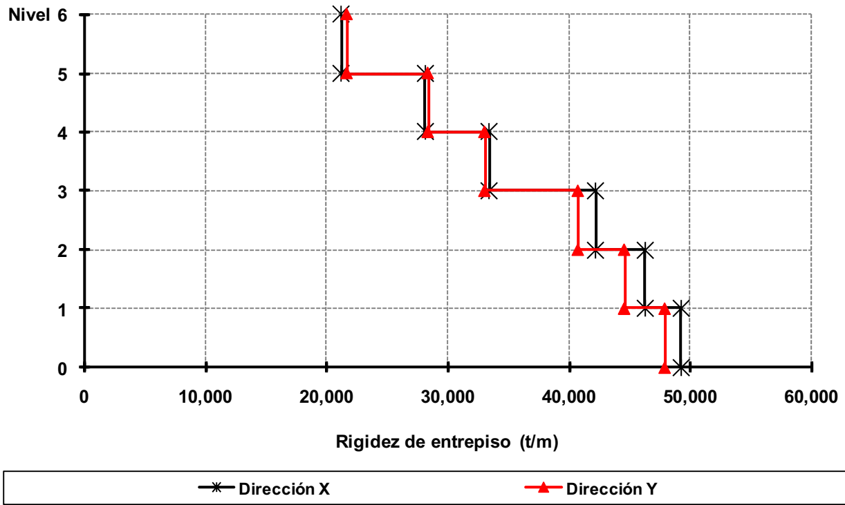
Fig 3.44 Rigideces de entrepiso, edificio 6 niveles, caso C1 (Q = 2)
