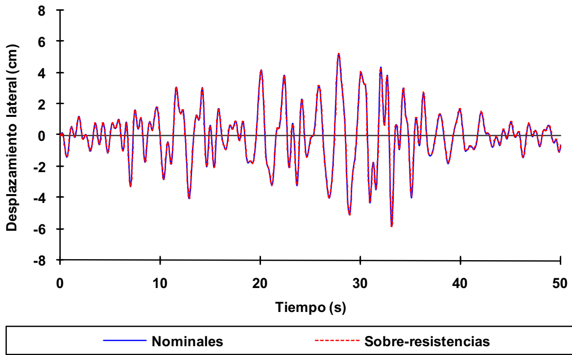
Fig 4.23 Historias de desplazamientos laterales de azotea, eje A, caso C2, análisis paso a paso elástico e inelástico (sin y con sobre-resistencias), diseño Apéndice A, NTC-Sismo del RDF-04, edificio de 6 niveles
