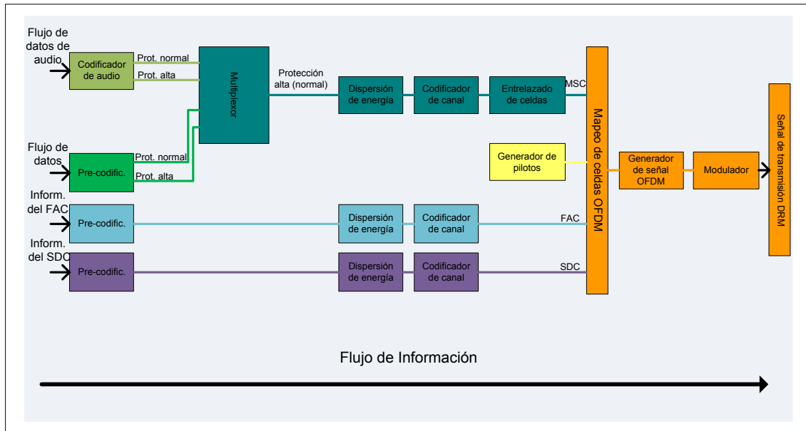
Figura 2.2. Diagrama de bloques de transmisión del sistema DRM.
