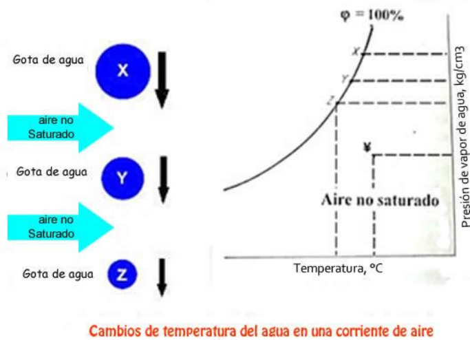
Fig.3.3. Proceso y representación en el diagrama psicrométrico de una gota de agua en una corriente de aire.
