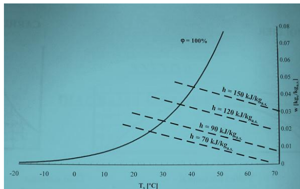
Fig.3.9 Representación de las líneas Isoentálpicas.
