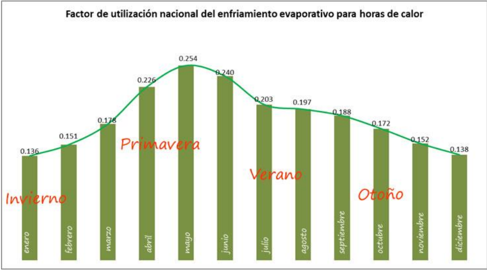
Gráfica 7.3 Factor de utilización del enfriamiento evaporativo en las principales ciudades del país considerando únicamente las horas de calor de los requerimientos bioclimáticos presentes.
