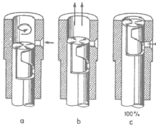
Figura A.3 Vista detallada de la posición del pistón
