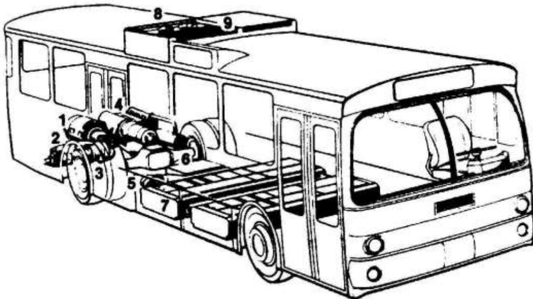
Figura 1.2 Autobús híbrido eléctrico de arreglo en serie
