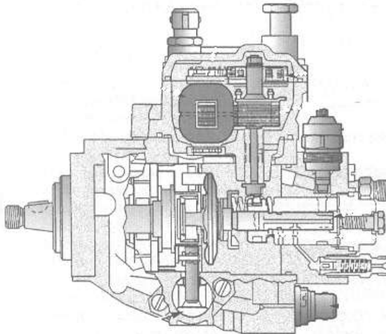
Figura A.36 Bomba de mando electrónico VP36
