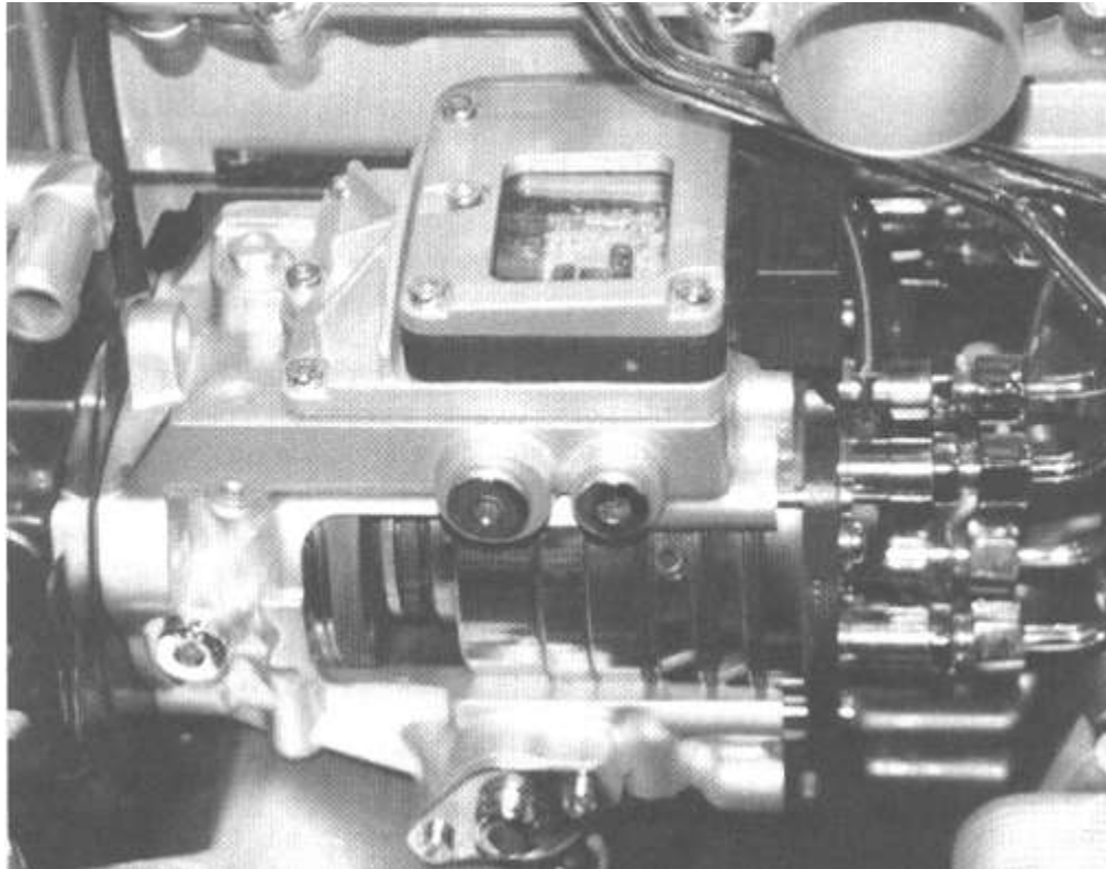
Figura A.35 Bomba VP 37 R 510
