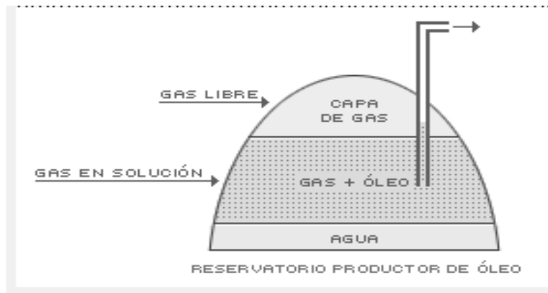
Figura 1.9 Extracción de gas asociado.
