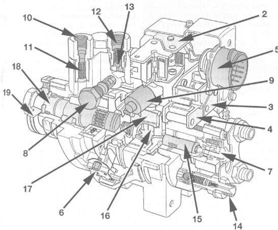
Figura A.48 Elementos de una bomba Lucas de la serie EPIC
