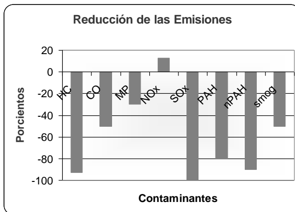
Figura 1.11 Reducción de emisiones del biodiesel
