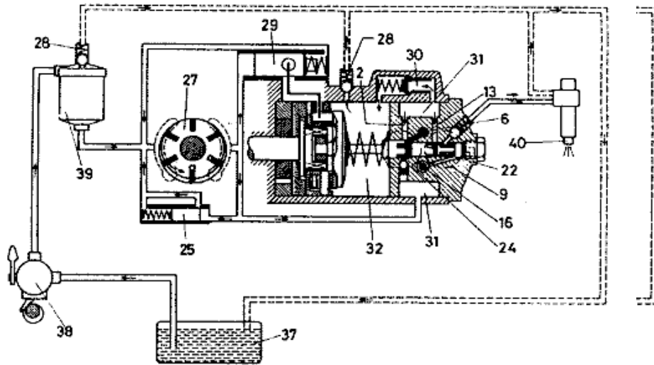
Figura A.26 Componentes hidráulicos de una bomba rotativa
