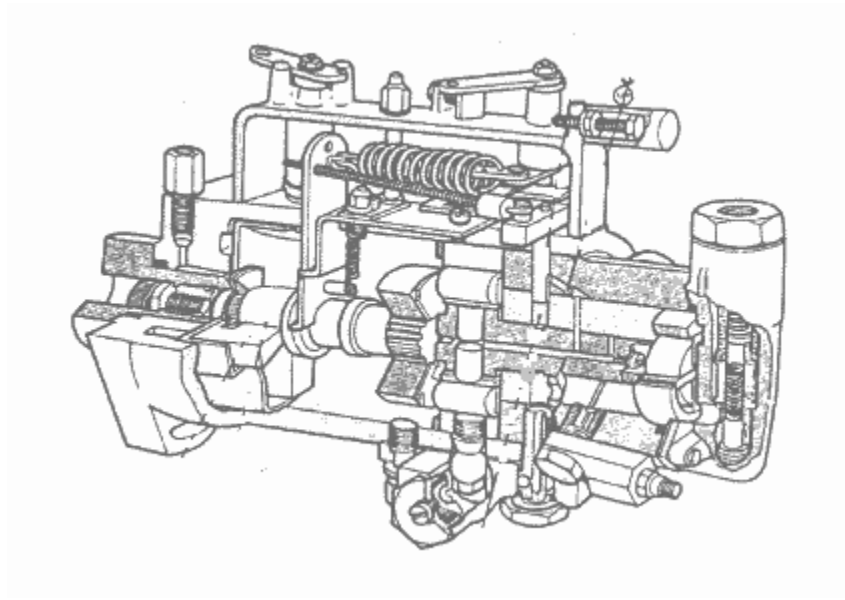
Figura A.20 Bomba provista de regulador mecánico
