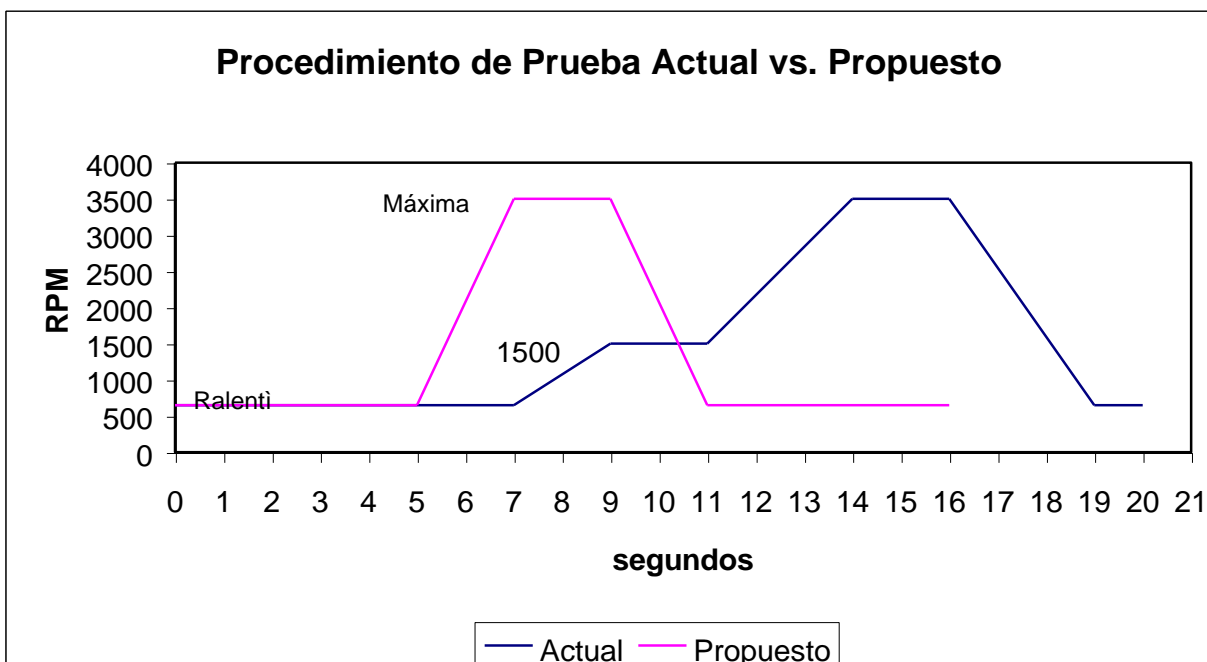
Figura 3.3 Procedimiento de prueba actual vs. propuesto
