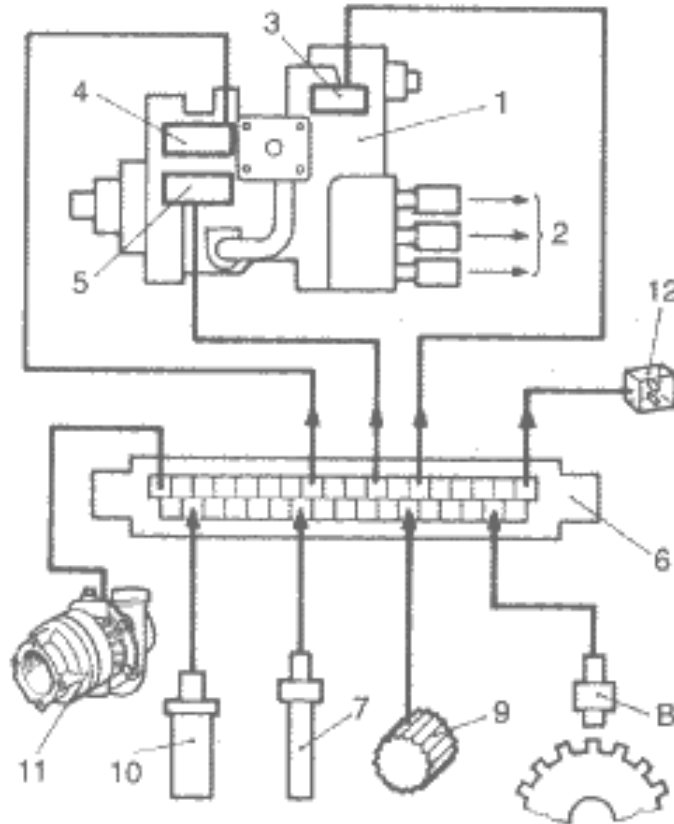
Figura A.29 Sistema de inyección electrónica
