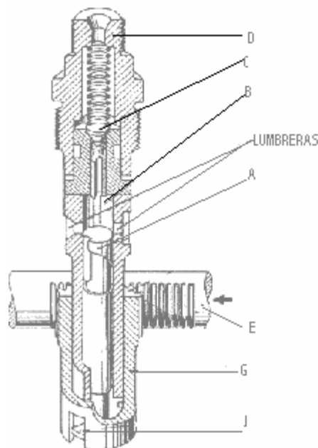
Figura A.2 Mecanismo de impulsión y regulación de caudal.
