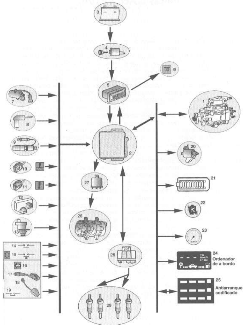
Figura A.38 Dispositivos del sistema de inyección tipo VP
