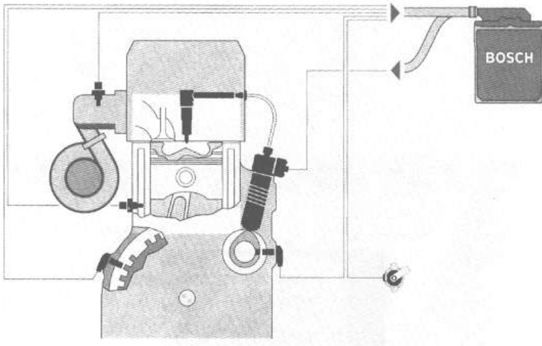
Figura A.44 Sistema Bomba-Tobera-Inyector
