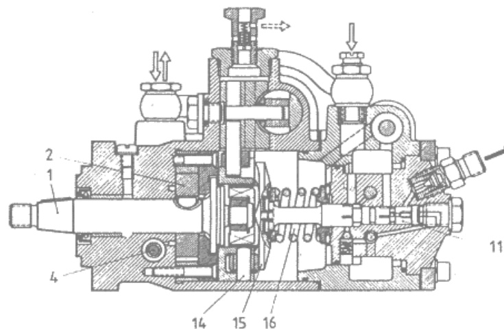
Figura A.25 Sección de una bomba rotativa bosh
