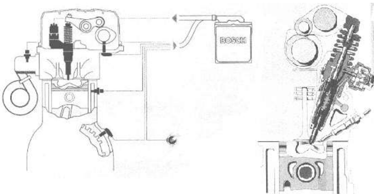
Figura A.43 Sistema Bomba-Inyector
