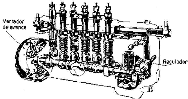
Figura 1.15 Bomba en línea o múltiples
