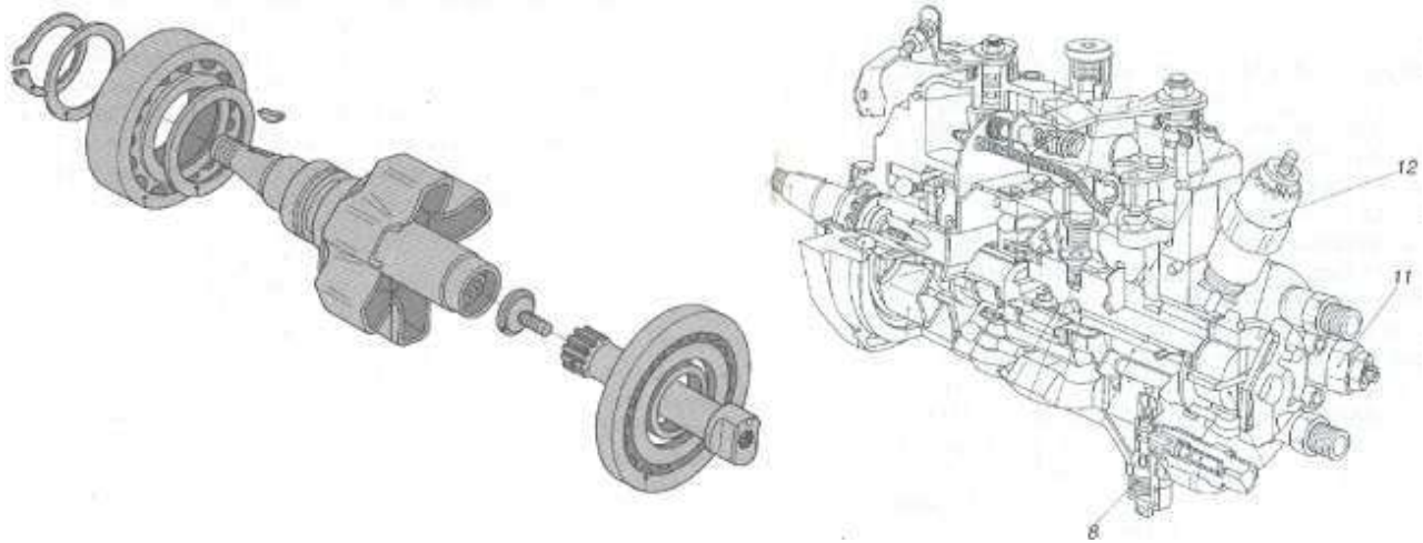
Figura A.45 Bomba electrónica Lucas
