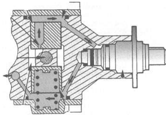
Figura A.37 Electroválvula para control de presión hidráulica
