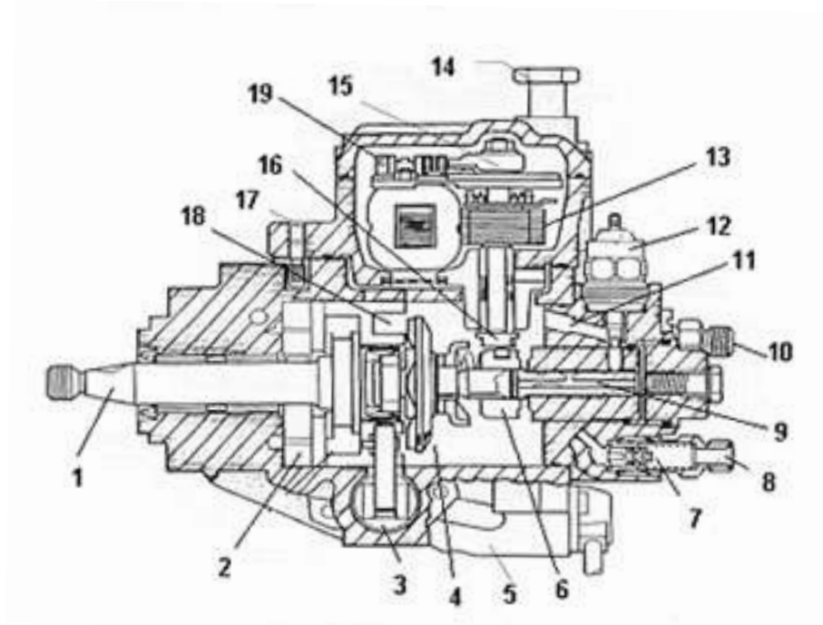
Figura 1.17 Esquema de una bomba de mando electrónico
