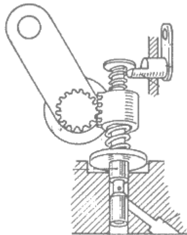
Figura A.16 Mecanismo de paro del regulador Hidráulico
