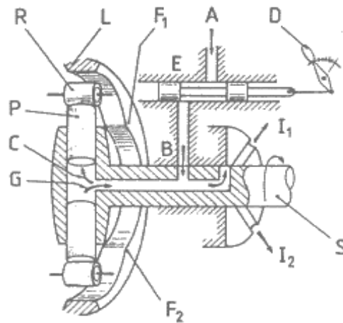
Figura A.11 Principio de funcionamiento de las bombas rotativas.
