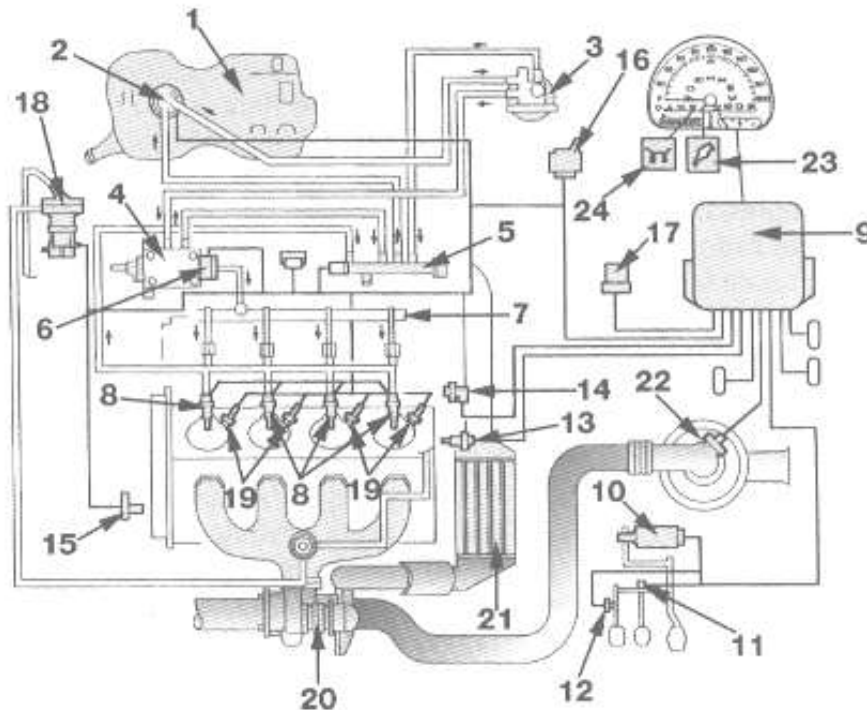
Figura A.42 Sistema de Inyección JTD
