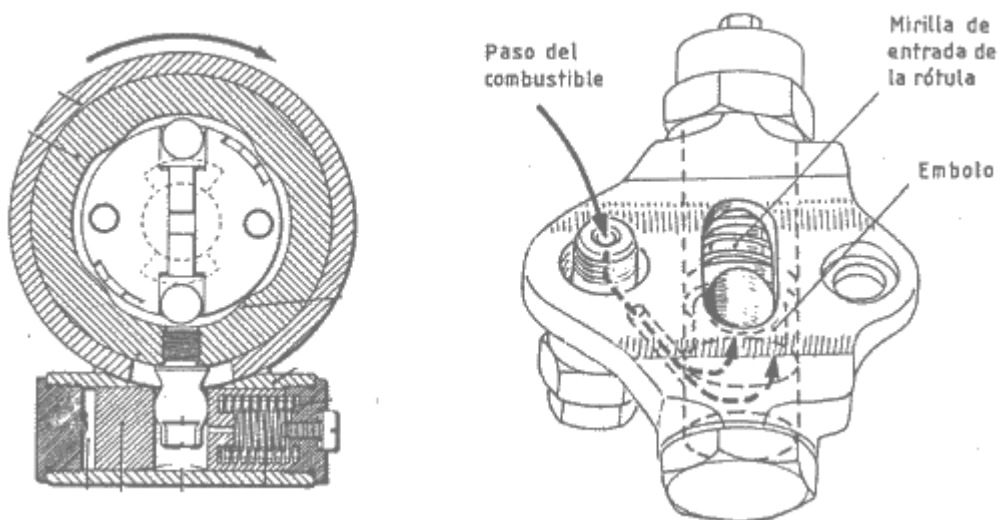
Figura A.19 Funcionamiento de Avance Automático
