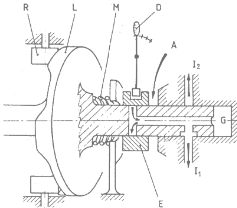
Figura A.23 Pistón de una bomba rotativa
