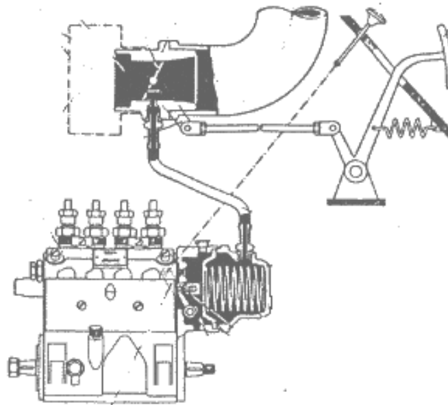
Figura A.8 Principio de funcionamiento del gobernador neumático
