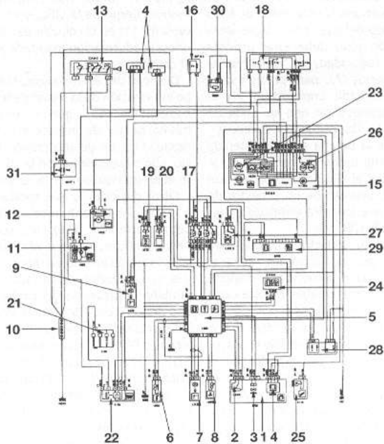
Figura A.40 Equipo de inyección electrónica diesel es el AS3 con bomba VP20
