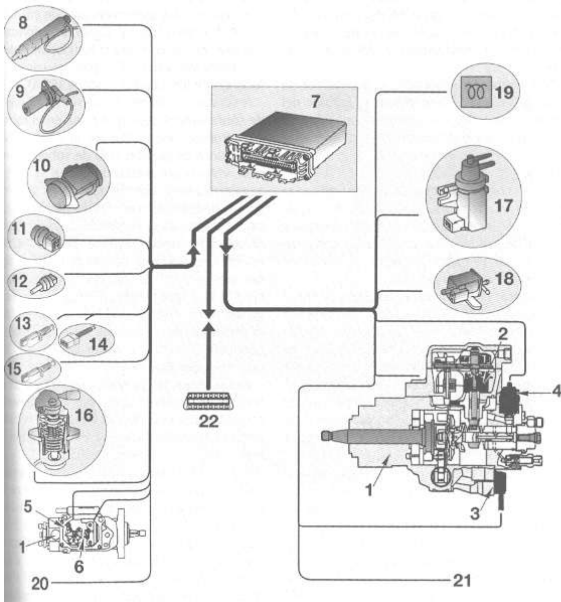
Figura A.34 Sistema de control electrónico Diesel (EDC)
