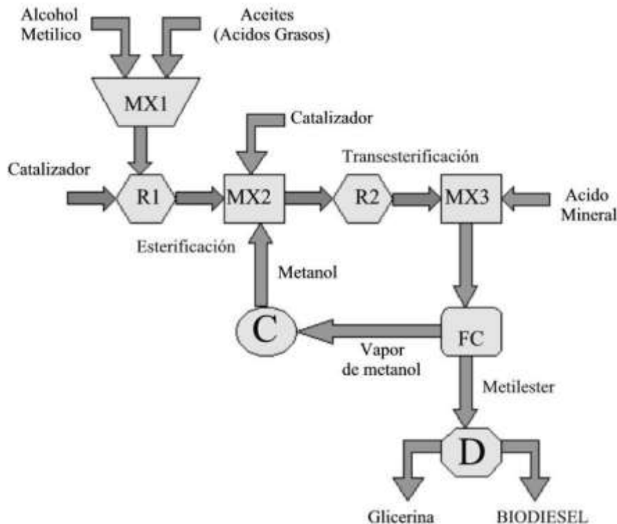
Figura 1.12 Proceso de elaboración del biodiesel.
