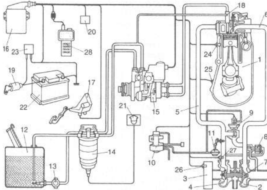
Figura A.49 Elementos de un sistema EPIC
