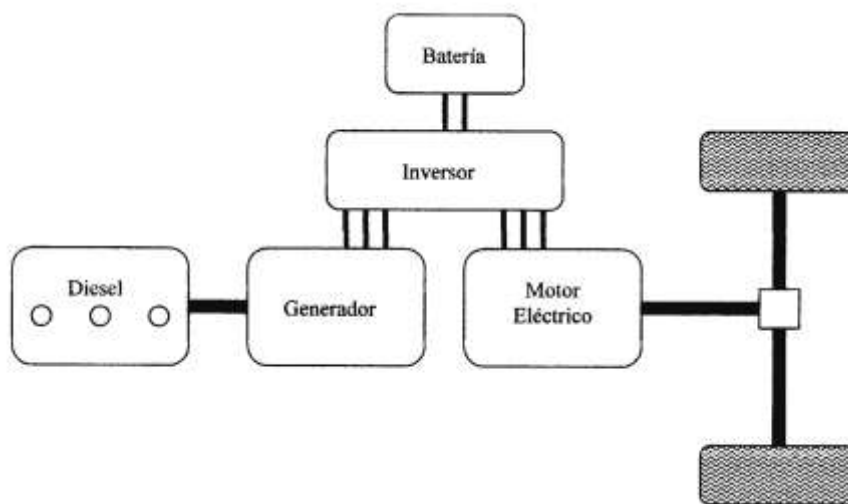
Figura 1.1 Sistema Híbrido en serie
