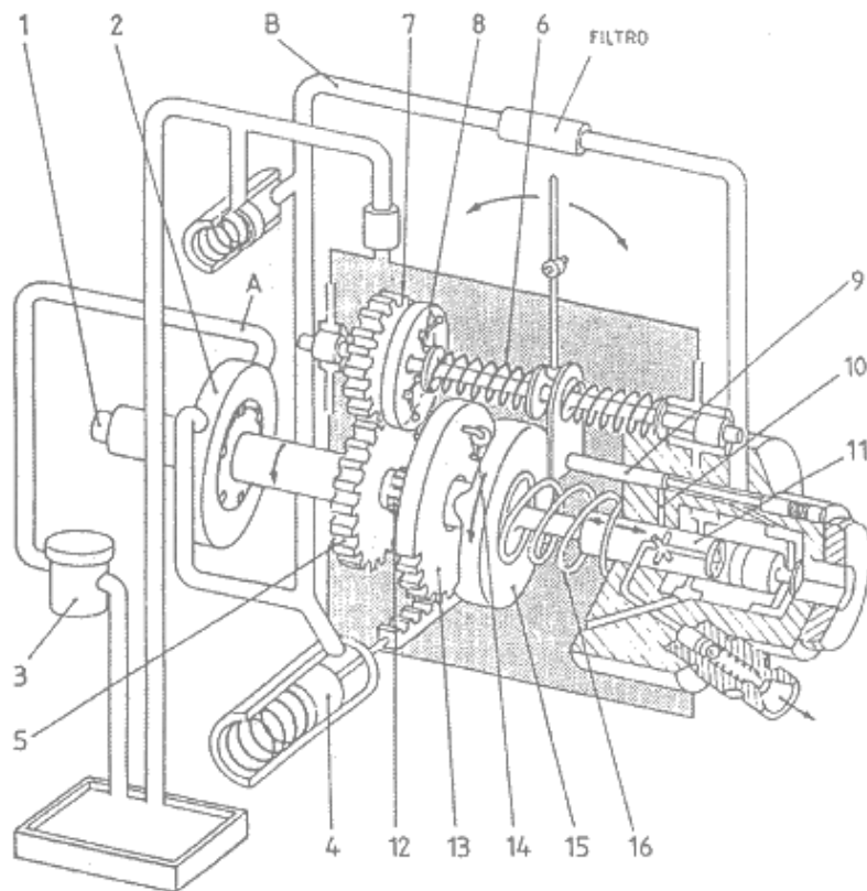
Figura A.24 Componentes mecánicos de una bomba rotativa.
