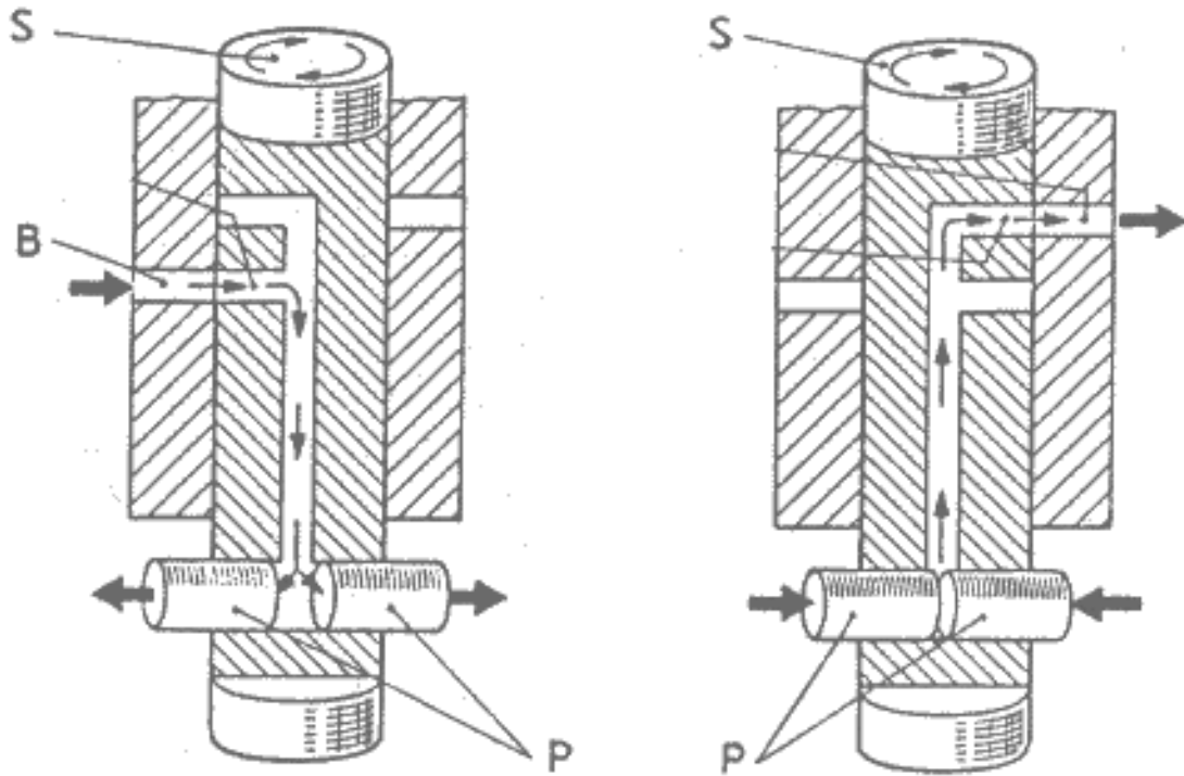
Figura A.12 Sección a detalle del funcionamiento para más cilindros.
