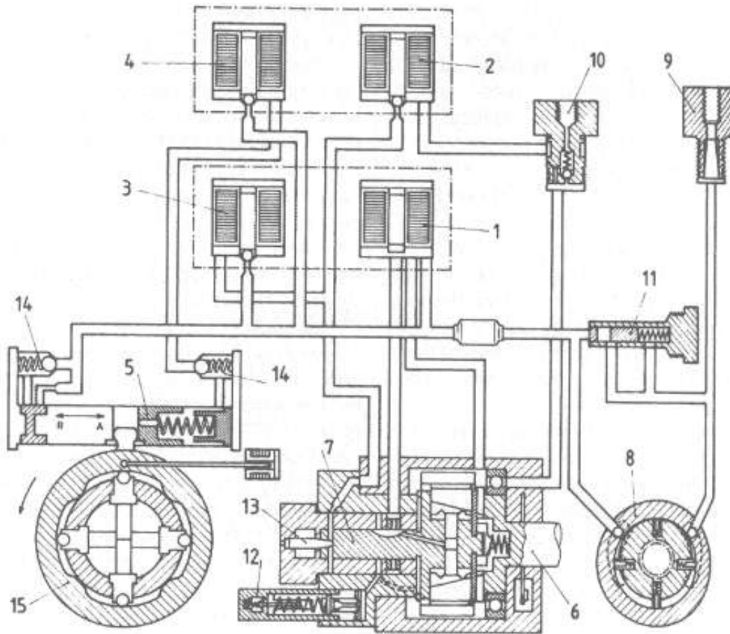
Figura A.50 Bomba utilizada en el sistema EPIC
