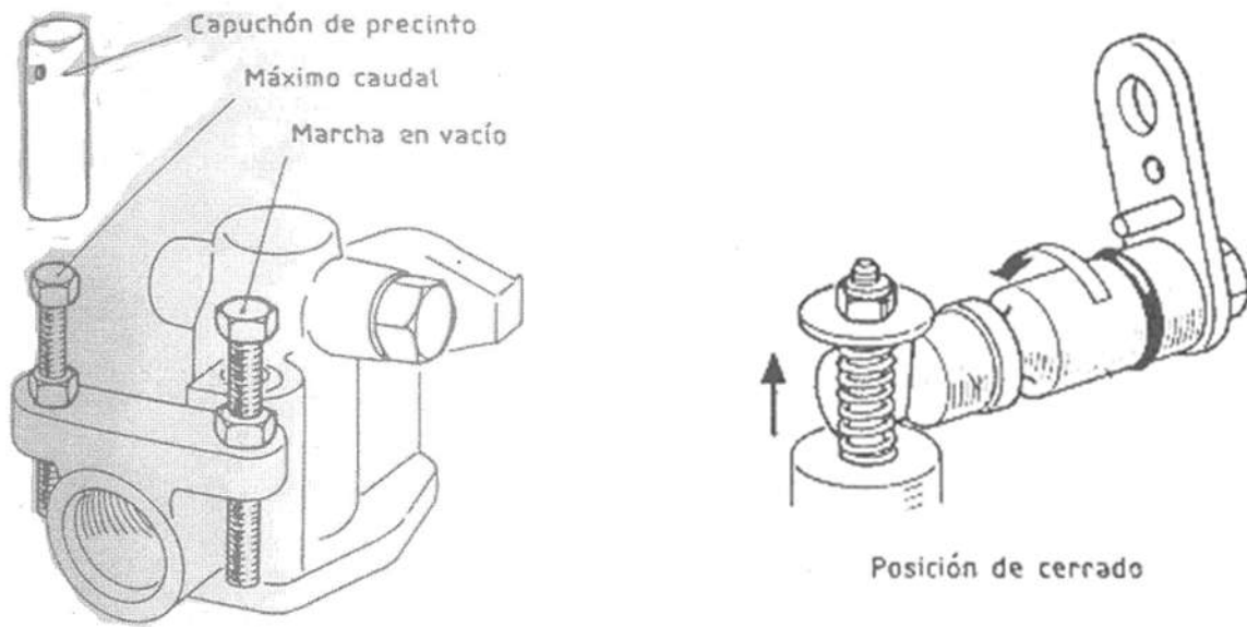
Figura A.15 Tornillo de regulación
