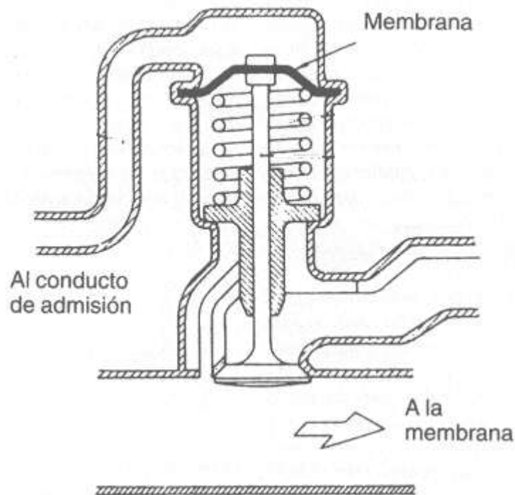
Figura A.32 Válvula de descarga
