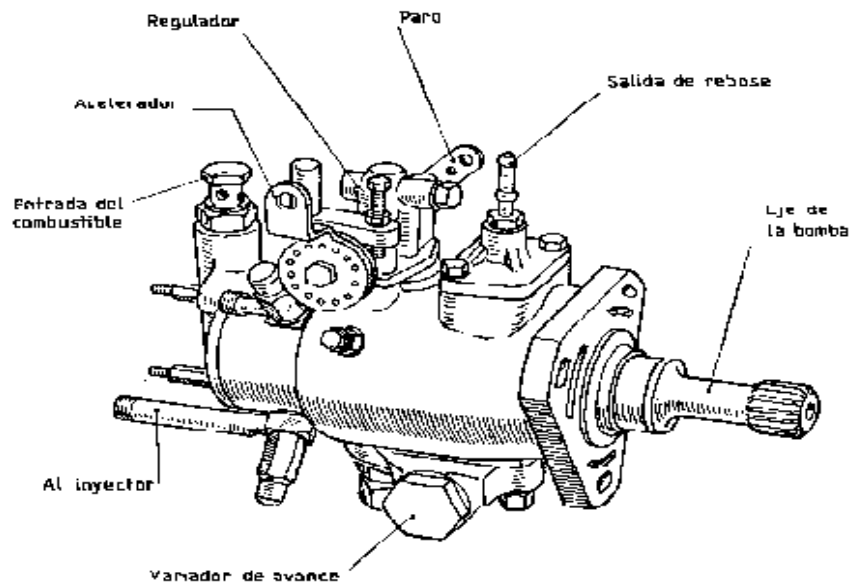
Figura 1.16 Bomba de inyección tipo mecánico rotativa
