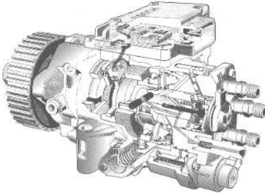
Figura A.39 Bomba de mando electrónico Bosh
