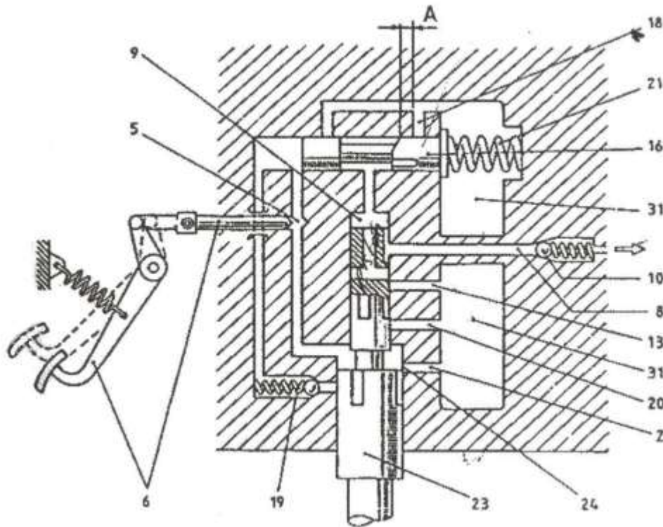
Figura A.28 Primer tiempo de admisión de combustible
