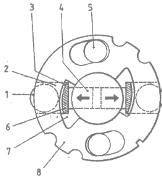
Figura A.18 Esquema del rotor de regulación de caudal
