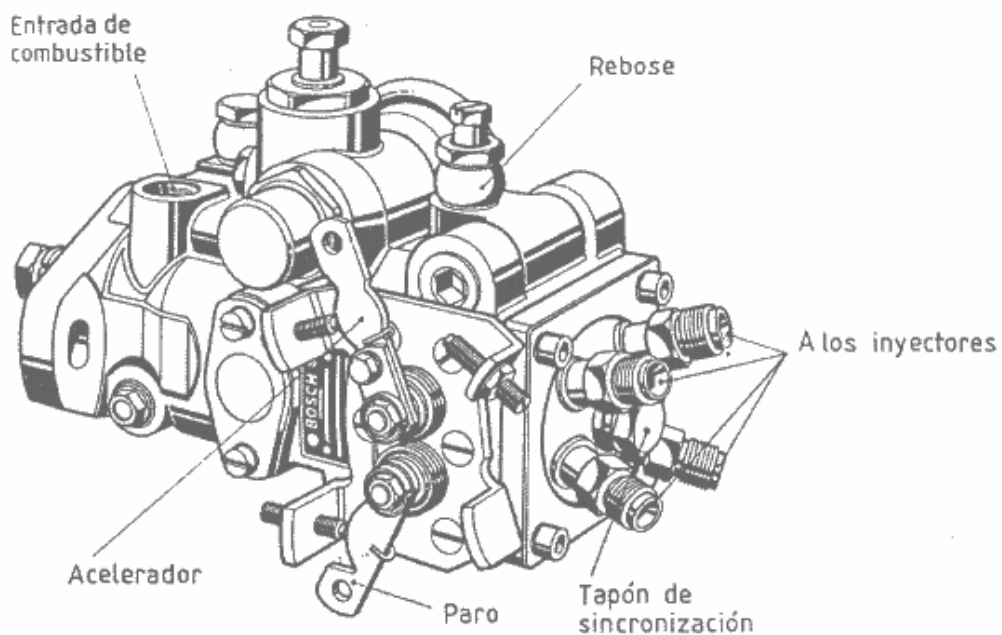
Figura A.22 Bomba Rotativa
