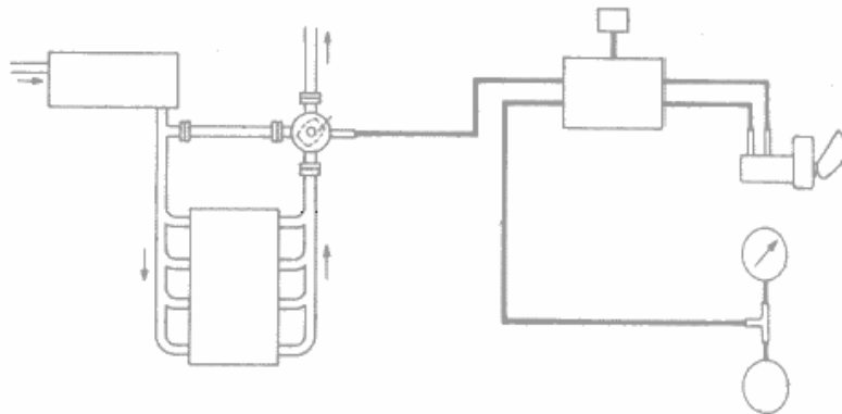
Figura A.30 Distribución de equipo EGR
