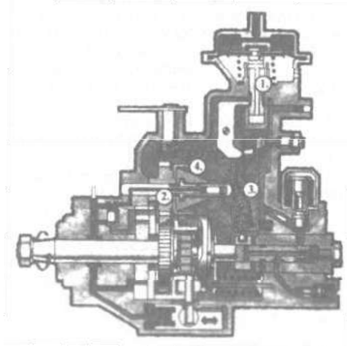
Figura A.33 Bomba Electrónica Bosh
