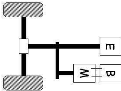
Figura 1.5 Combinación de torques
