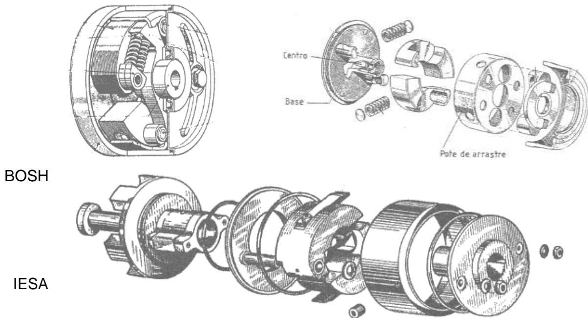
Figura A.9 Variadores de avance
