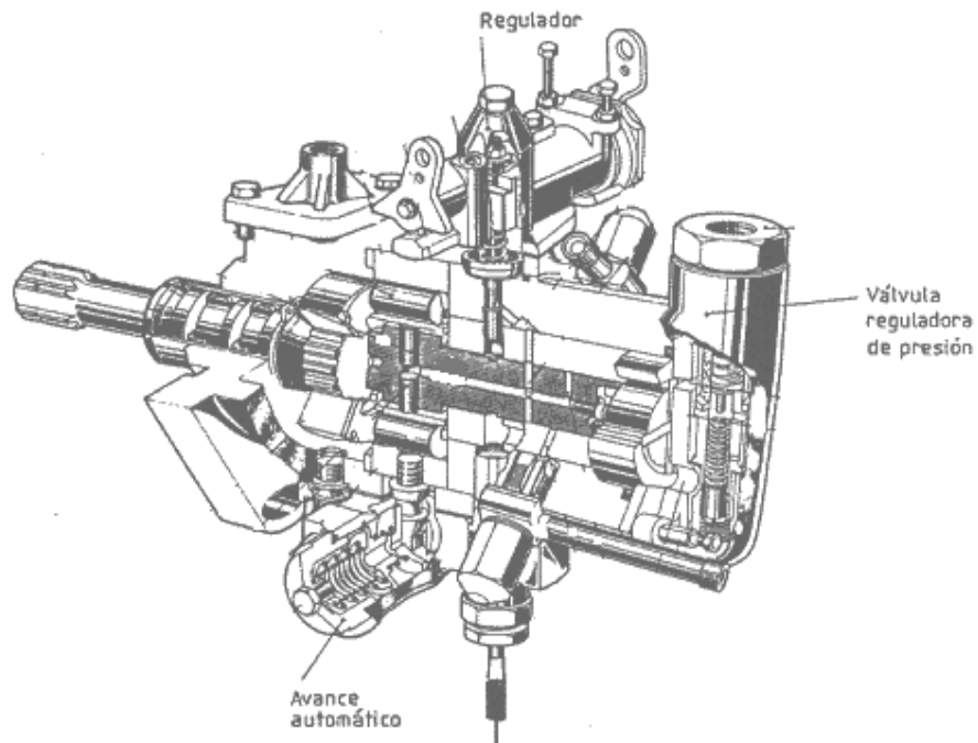
Figura A.14 Esquema seccionado de la bomba rotativa C.A.V.
