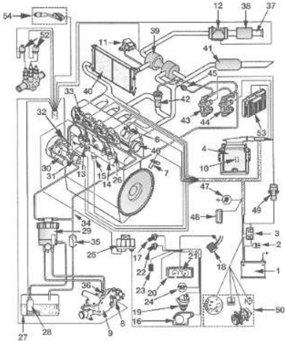
Figura A.41 Sistema de Inyección de Riel Común
