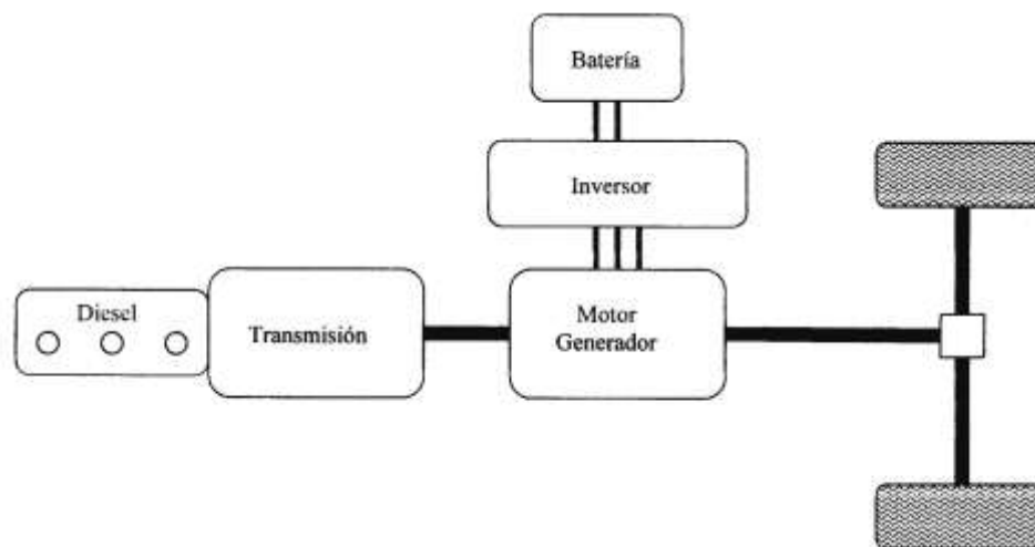
Figura 1.3 Sistema Híbrido en paralelo
