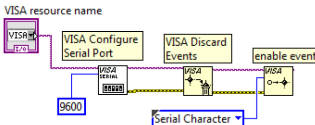
Figura 5.8 Conexión de los bloques de configuración de puerto, descarte de evento, y habilitación de evento.
