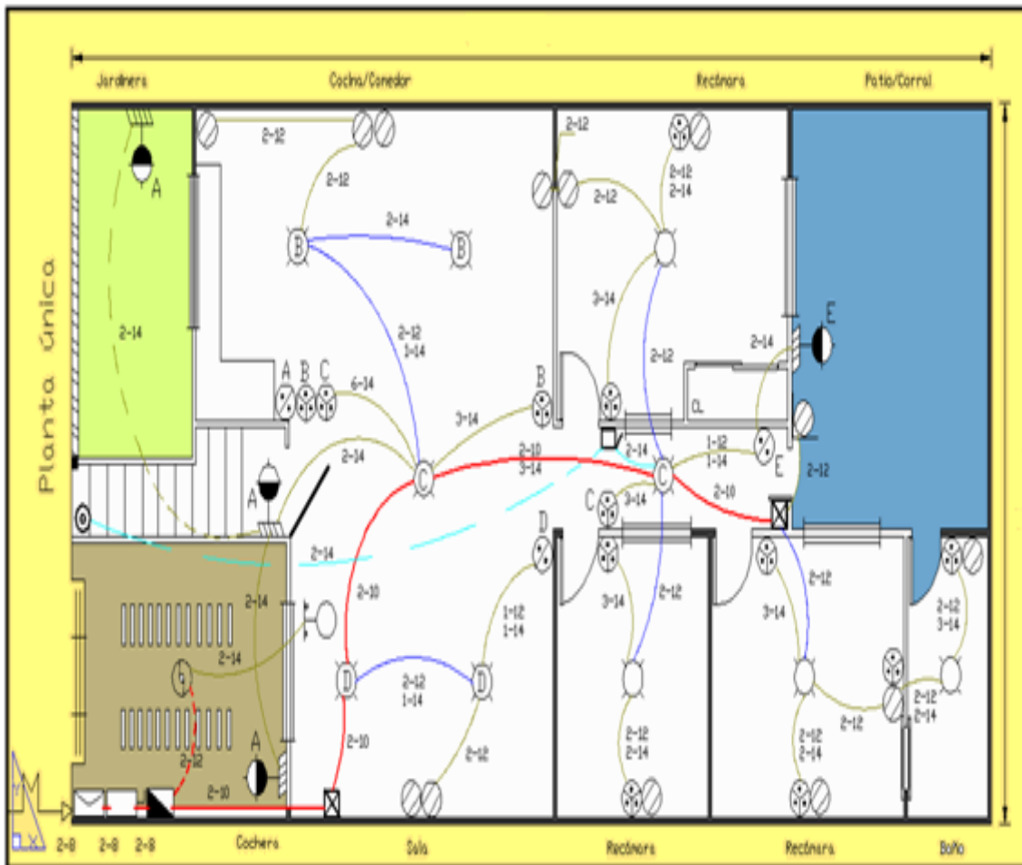
Figura 5.1 Diagrama de instalación eléctrica planta baja
