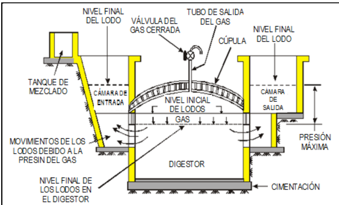
Figura 1.24 Modelo de plata de gas con biomasa (Enríquez, 2009)
